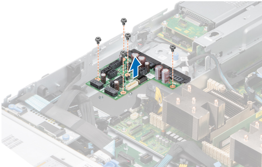
Ilustración 124. Extracción de la placa mediadora de alimentación
