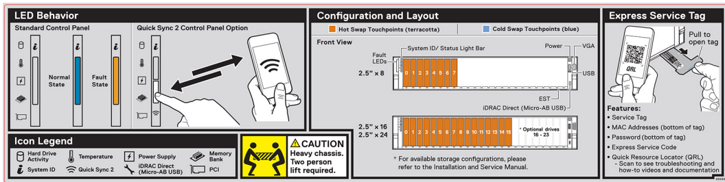
Ilustración 13. Comportamiento de LED, configuración y diseño, etiqueta de servicio exprés para el sistema de unidades de 2,5 pulgadas
