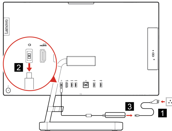
Figure 2. IdeaCentre AIO 3 22ITL6, IdeaCentre AIO 3 24ITL6, and IdeaCentre AIO 3 27ITL6
