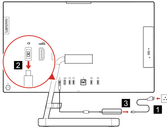
Figure 1. IdeaCentre AIO 3 22ADA6, IdeaCentre AIO 3 24ADA6, IdeaCentre AIO 3 24ALC6, and IdeaCentre AIO 3 27ALC6
