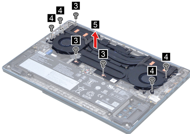
Figure 12. Remove the thermal module
