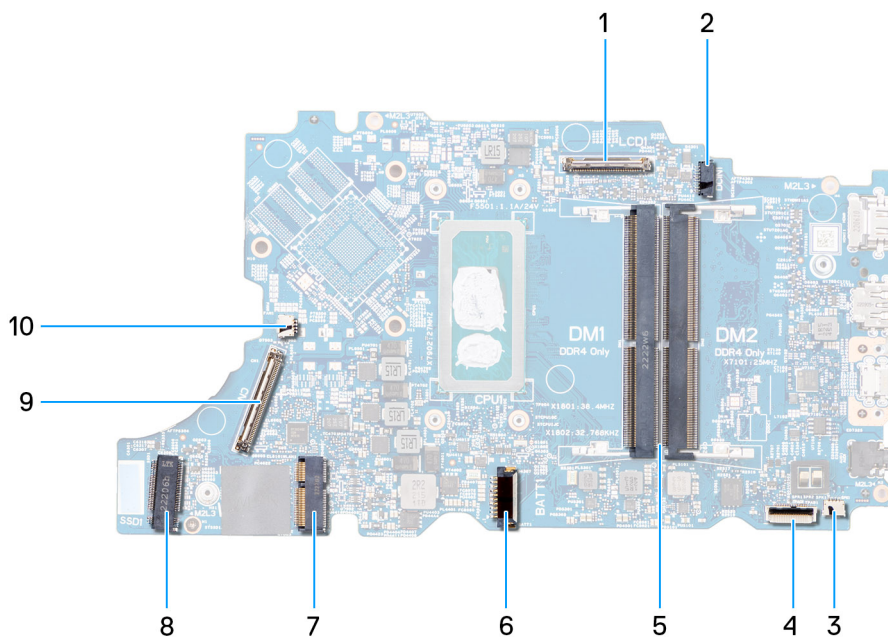
Afbeelding 2. Systeemkaartconnectoren - voorzijde
