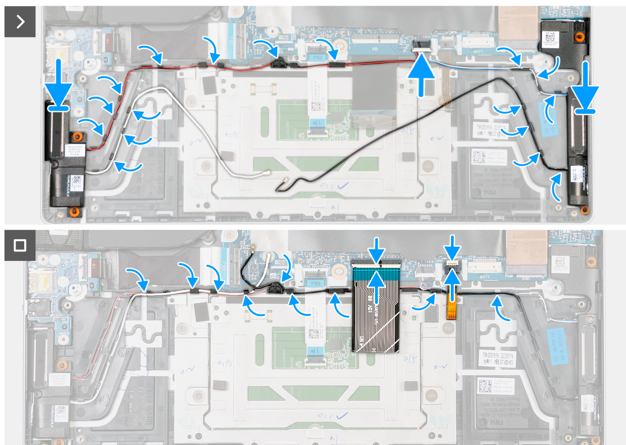
איור 31. התקנת מכלול הרמקול והאנטנה
