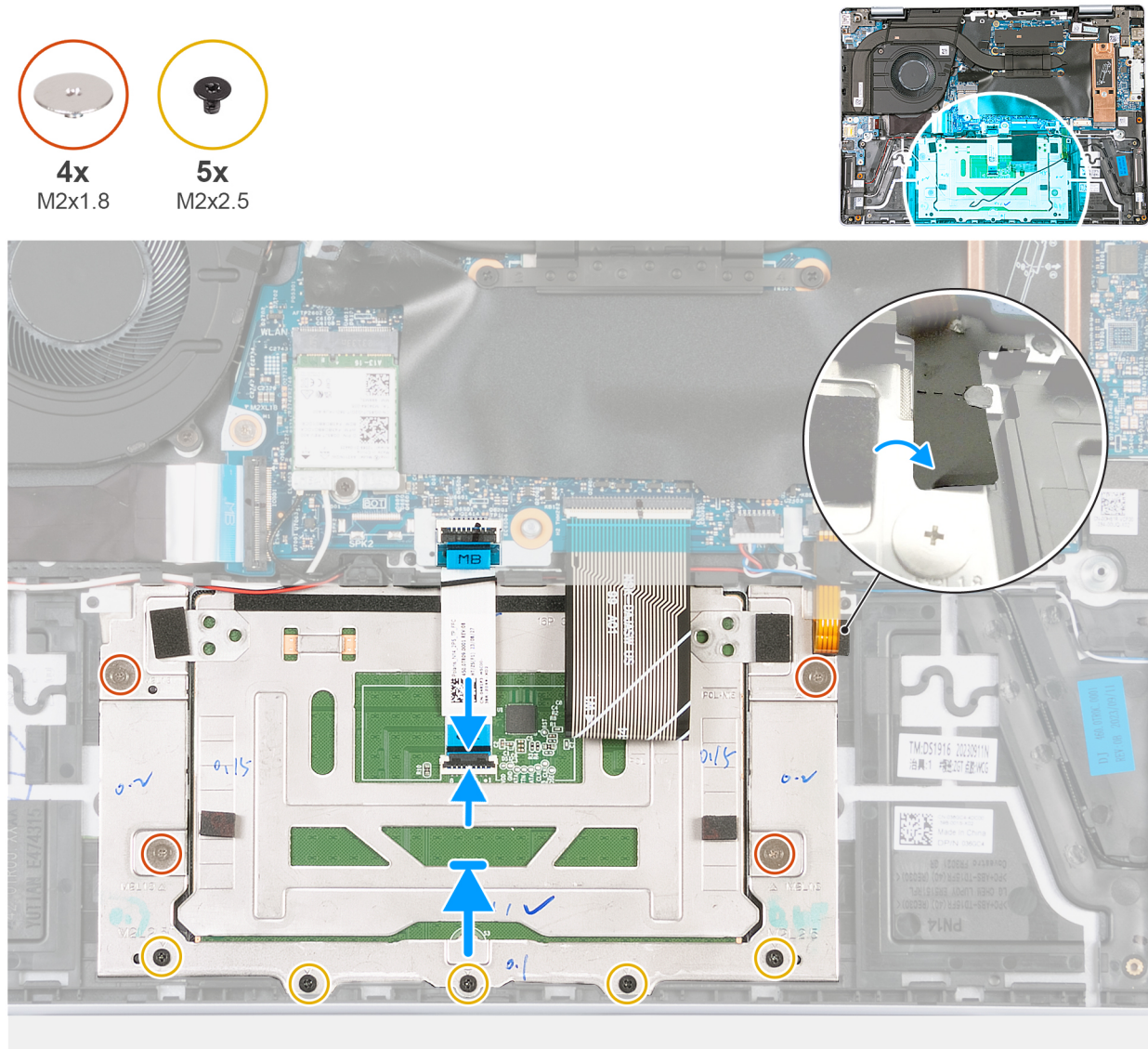
איור 48. התקנת משטח המגע
