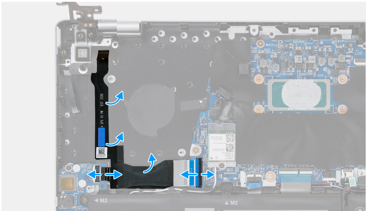
איור 49. הסרת כבל לוח הקלט/פלט ולוח ה-USB
