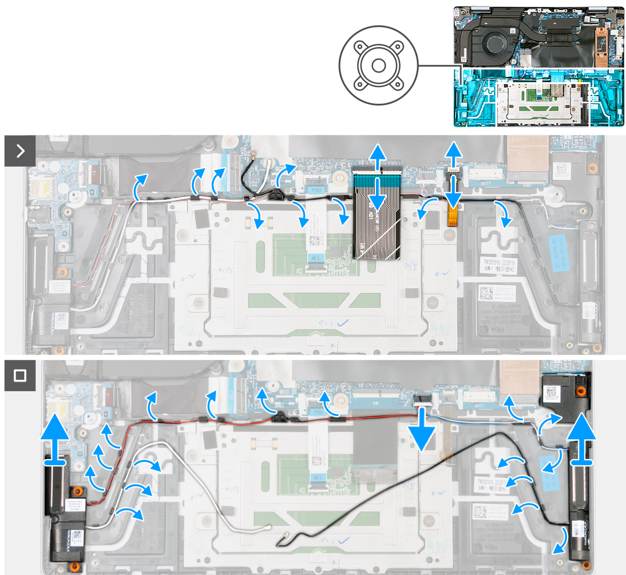
איור 30. הסרת מכלול הרמקול והאנטנה
