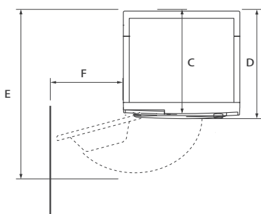
WAND DRAUFSICHT
