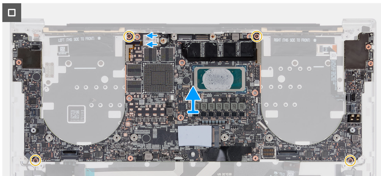
Rysunek 45. Wymontowywanie płyty głównej
