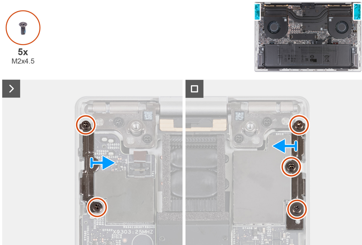
Rysunek 41. Wymontowywanie klamer złącza Type-C
