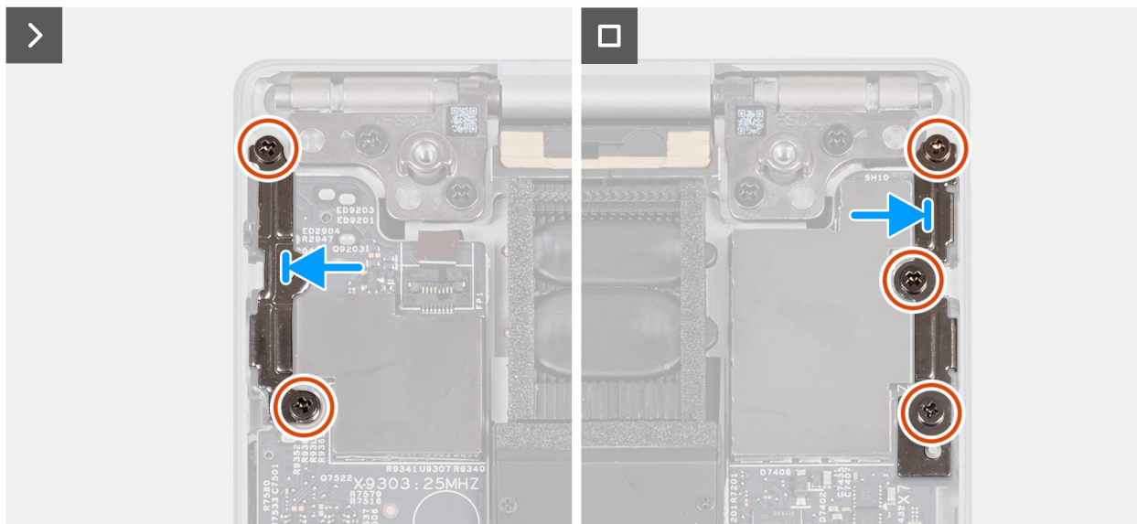
Rysunek 42. Instalowanie klamer złącza Type-C
