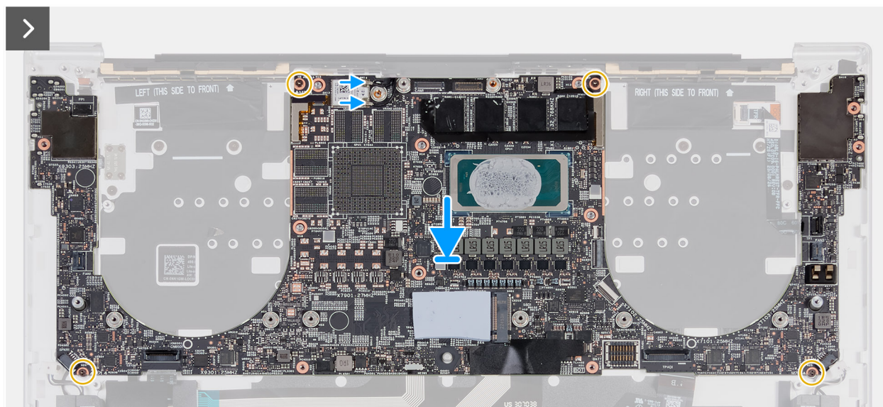
Rysunek 47. Instalowanie płyty głównej
