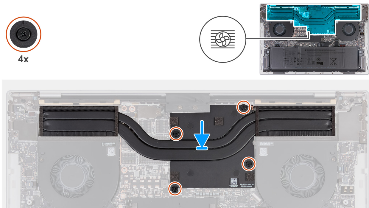
Rysunek 31. Instalowanie radiatora — konfiguracja ze zintegrowaną kartą graficzną
