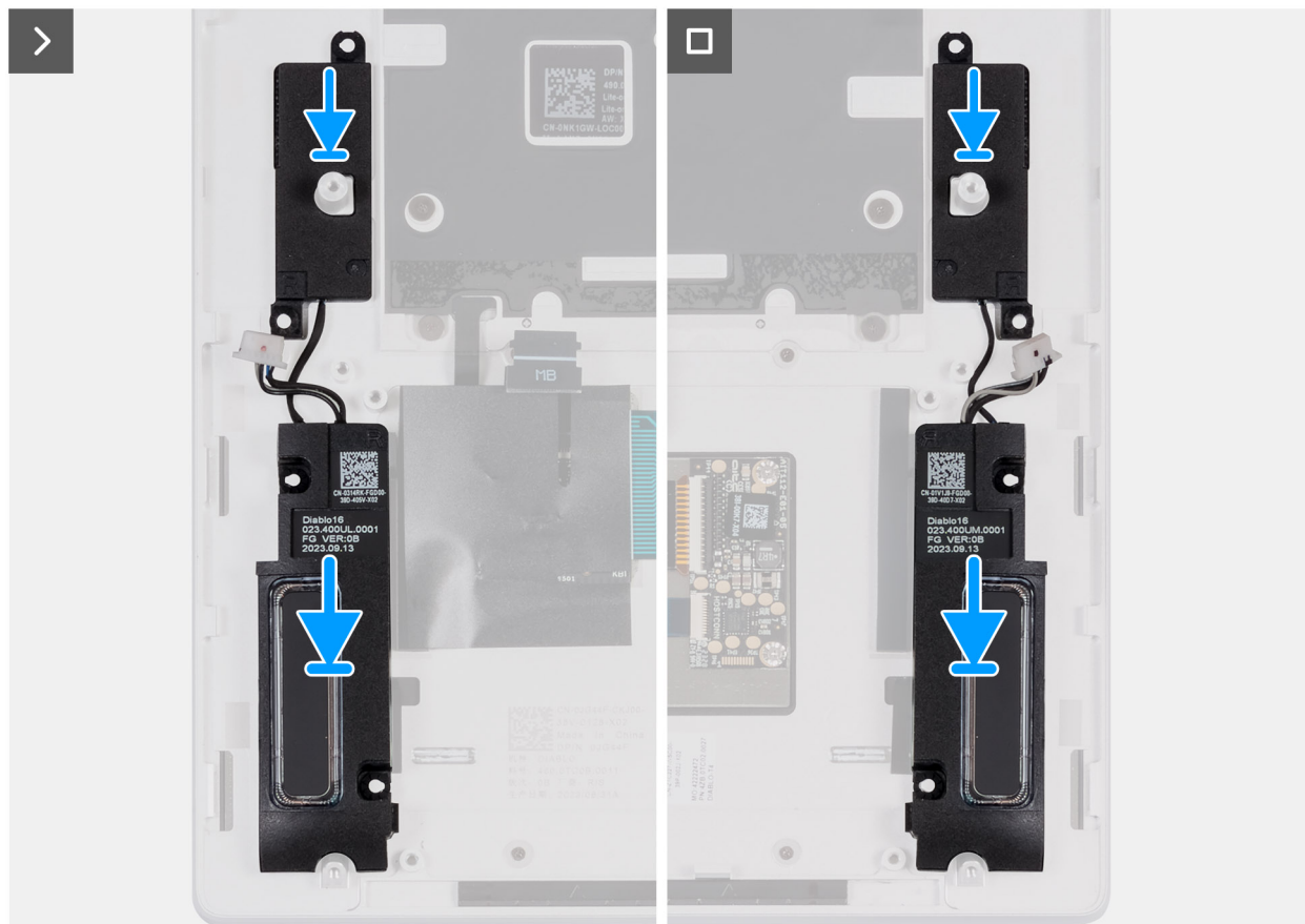
Rysunek 50. Instalowanie głośników
