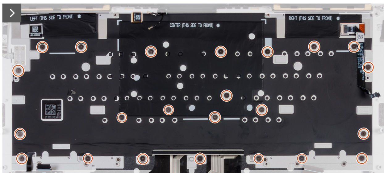
Rysunek 52. Wymontowywanie klawiatury
