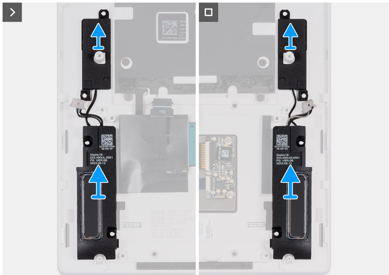
Rysunek 49. Wymontowywanie głośników
