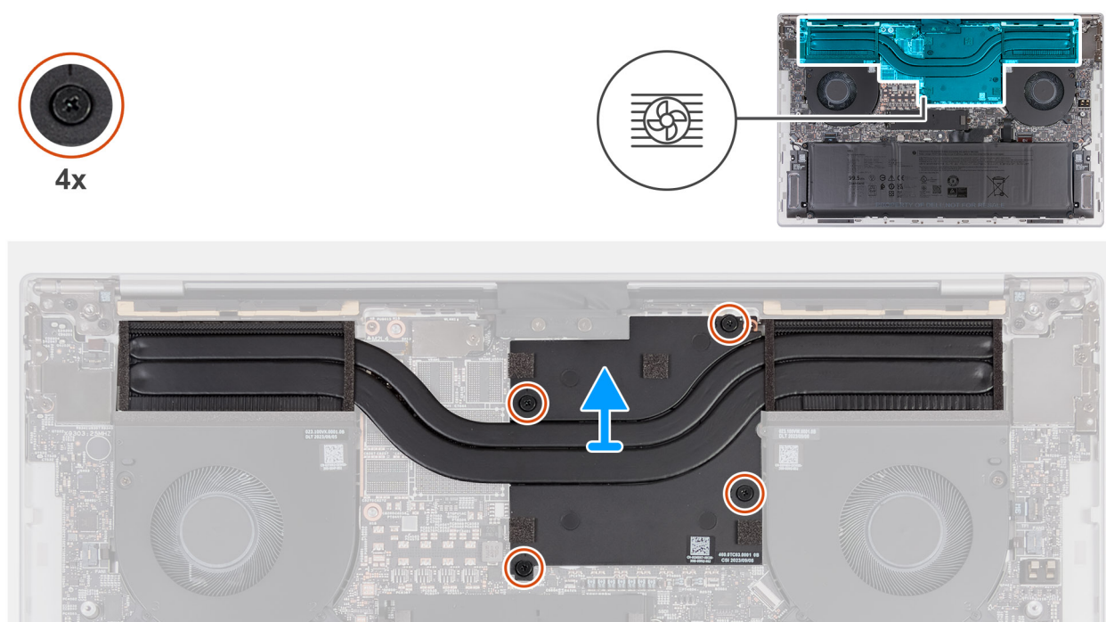
Rysunek 30. Wymontowywanie radiatora — konfiguracja ze zintegrowaną kartą graficzną
