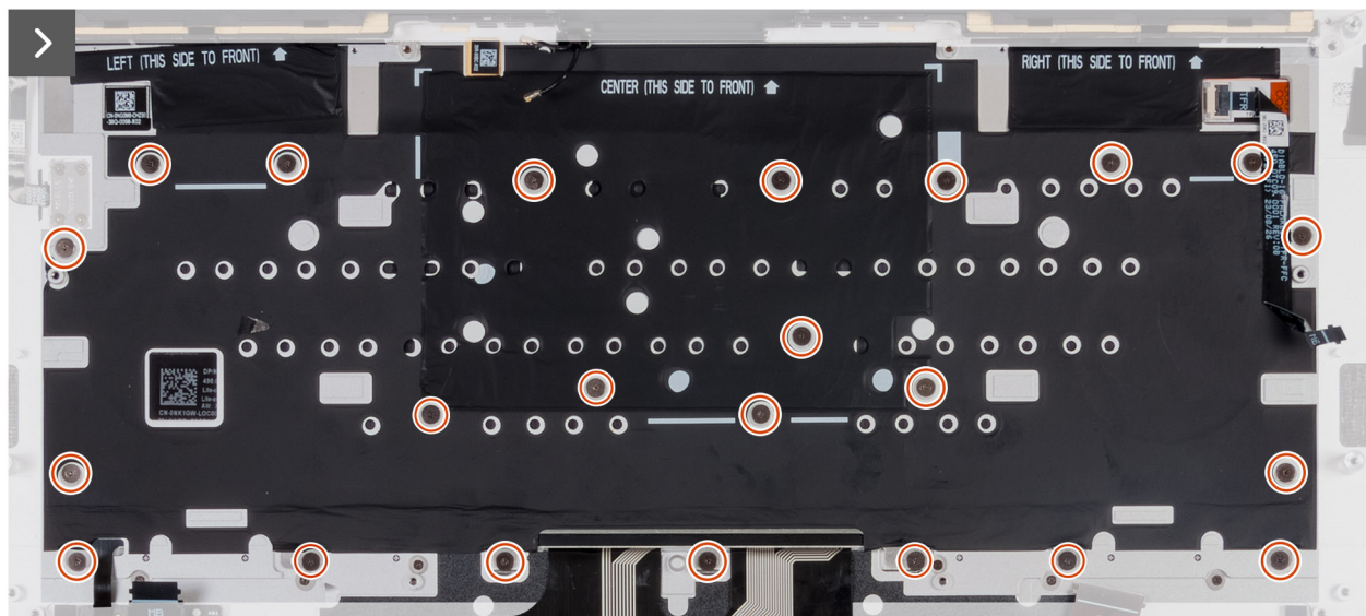
Rysunek 55. Instalowanie klawiatury
