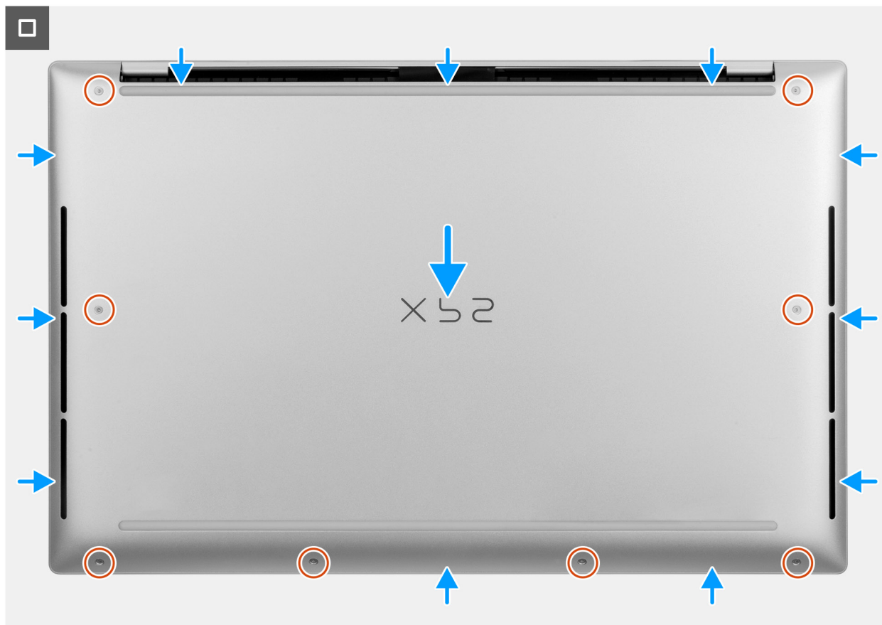
Rysunek 17. Instalowanie pokryw dolnej
