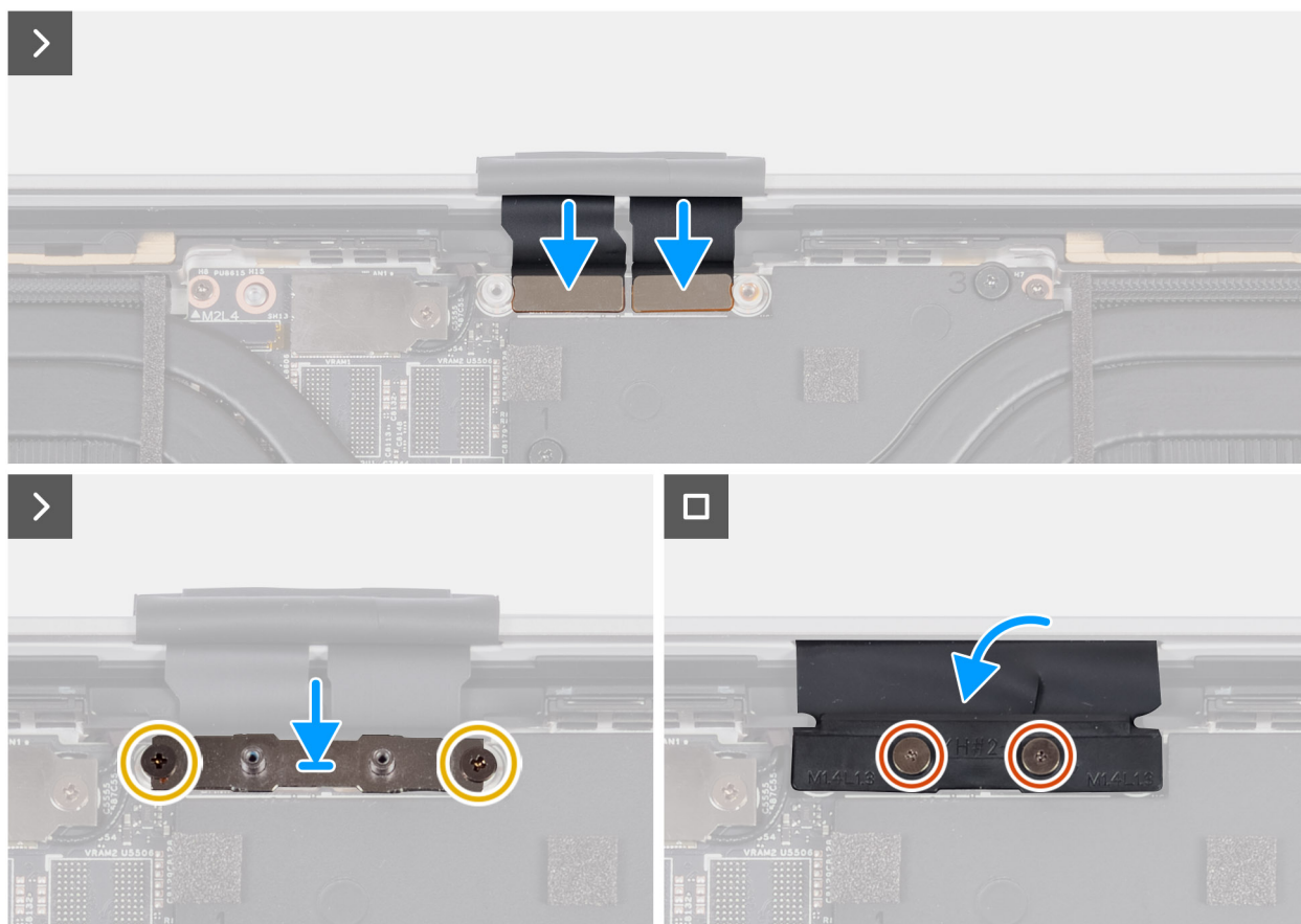
Rysunek 40. Instalowanie zestawu wyświetlacza
