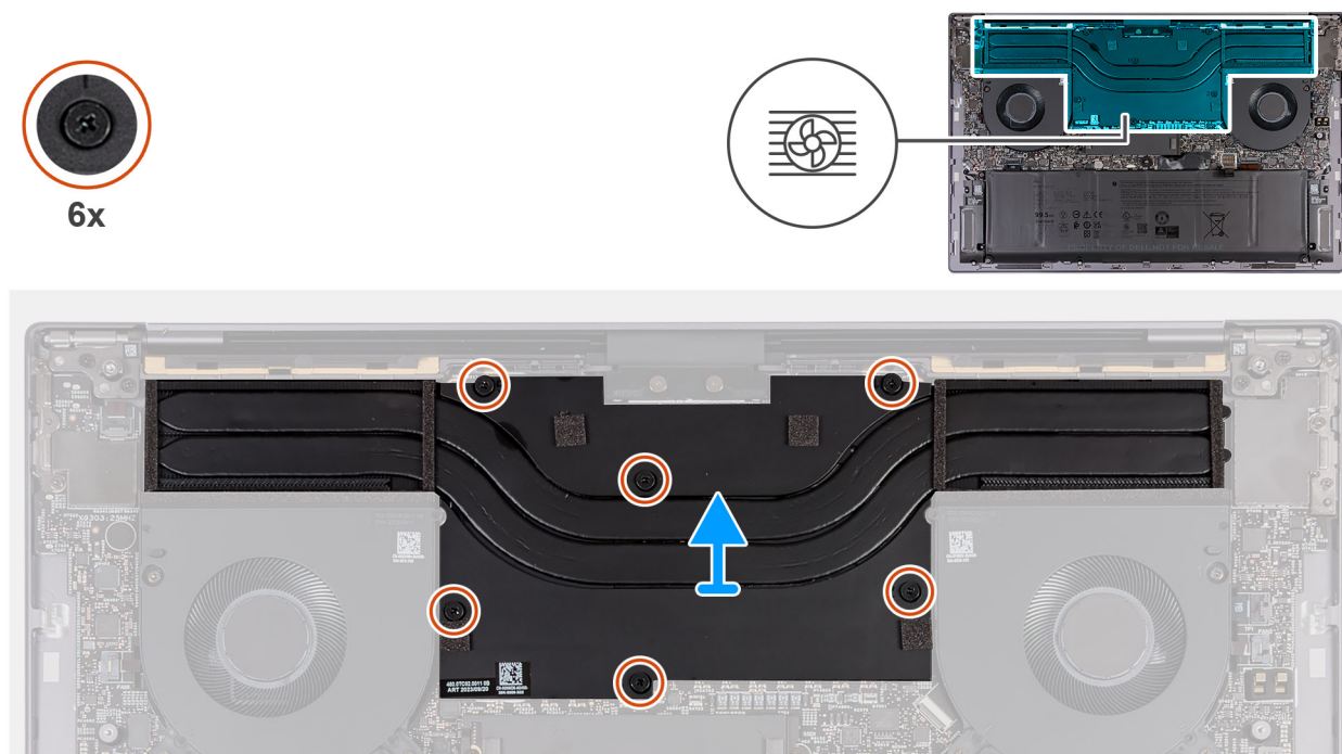
Rysunek 33. Instalowanie radiatora — konfiguracja z autonomiczną kartą graficzną
