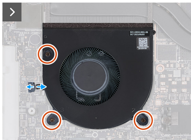
Rysunek 22. Wymontowywanie wentylatora karty graficznej
