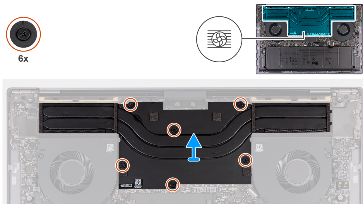
Rysunek 32. Wymontowywanie radiatora — konfiguracja z autonomiczną kartą graficzną
