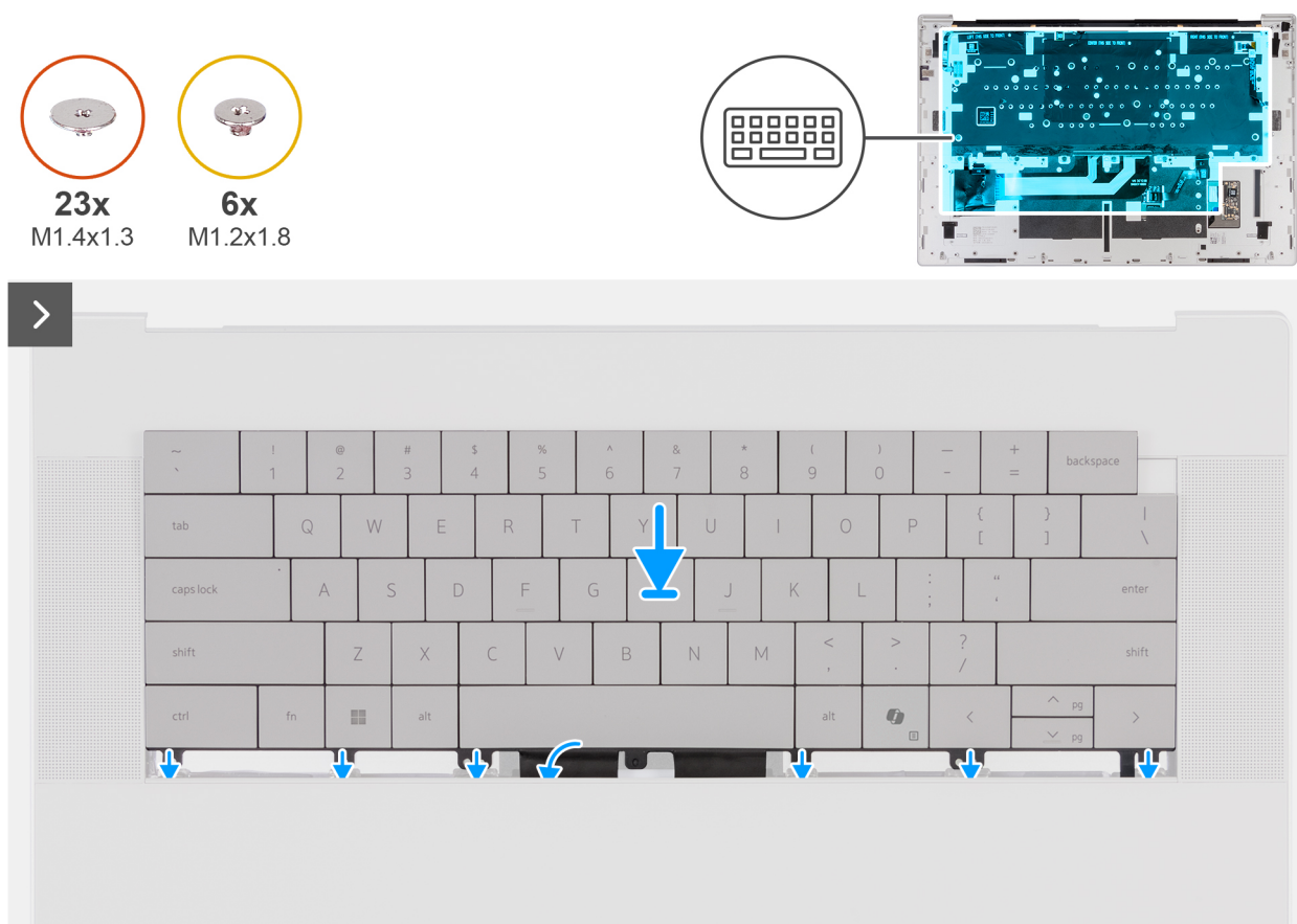
Rysunek 54. Instalowanie klawiatury
