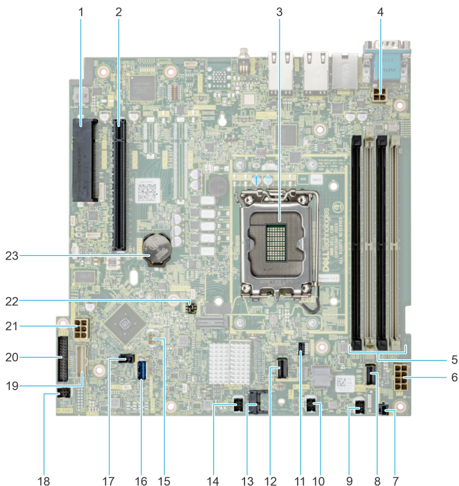
Ilustración 86. Puentes y conectores de la tarjeta madre del sistema
