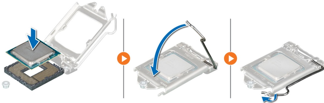
Ilustración 46. Instalación del gancho de retención
