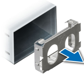
Ilustración 71. Extracción de una fuente de alimentación de relleno
