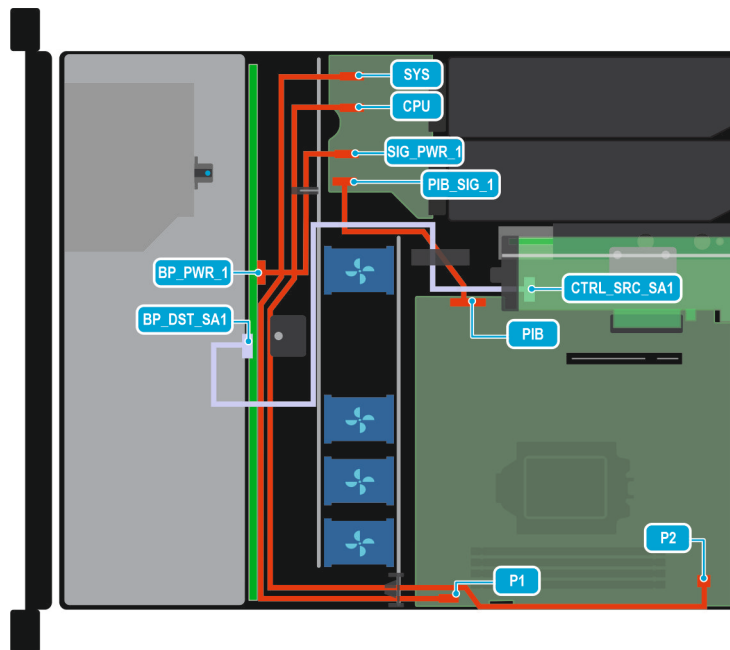
Ilustración 30. Configuración 2: 4 de SAS/SATA de 3,5 pulgadas y tarjeta PERC interna
