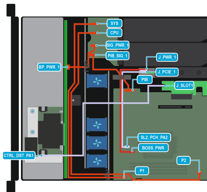
Ilustración 31. Configuración 3: tarjeta fPERC y SAS/SATA de 8 x 2,5 pulgadas con BOSS N1 opcional
