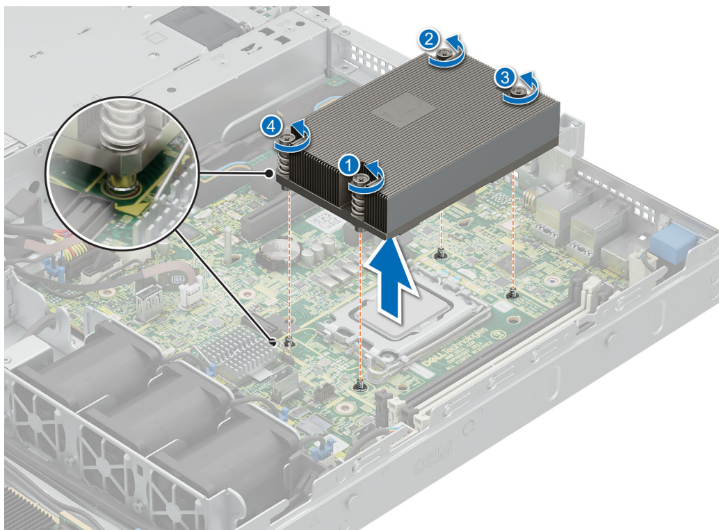
Ilustración 44. Extracción del módulo del disipador de calor
