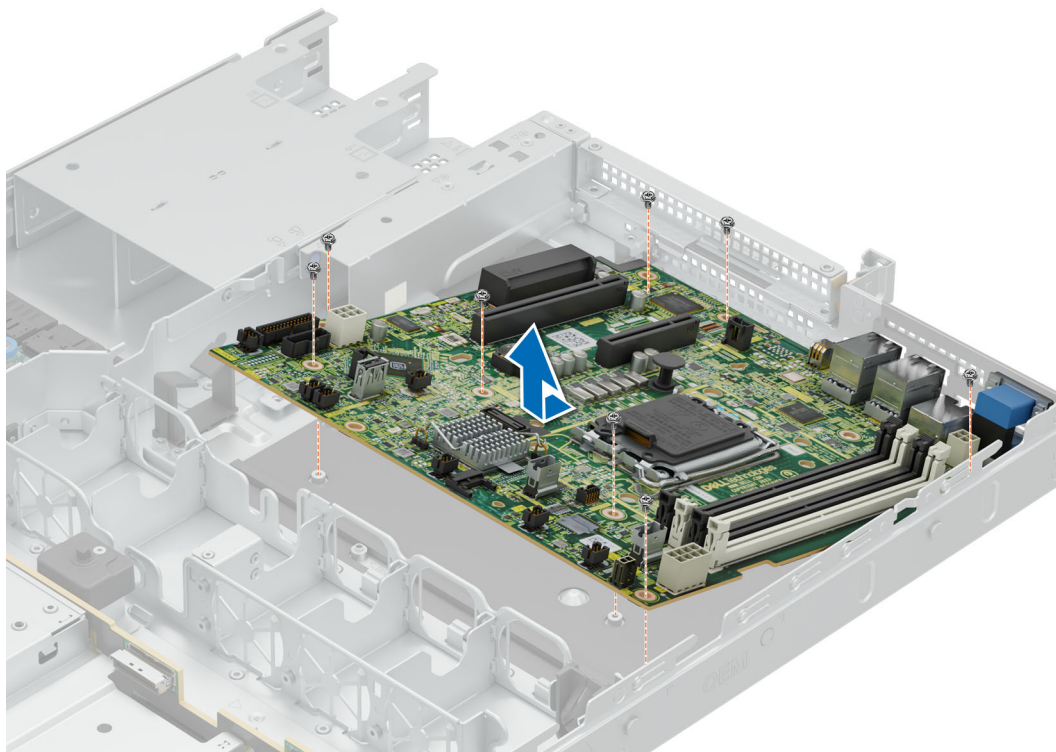
Ilustración 77. Extracción de la tarjeta madre
