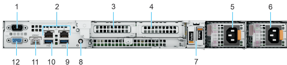
Ilustración 3. Vista posterior del sistema
