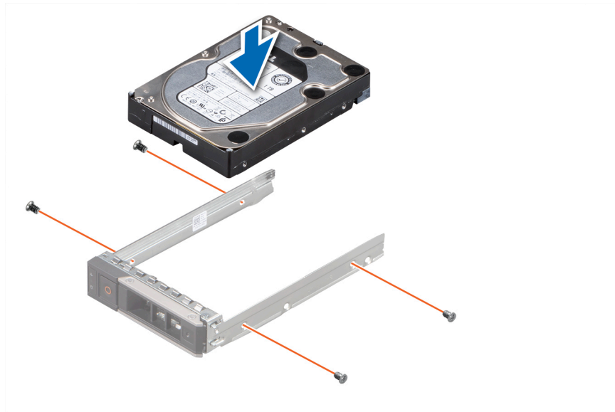
Ilustración 37. Instalación de una unidad en el portaunidades
