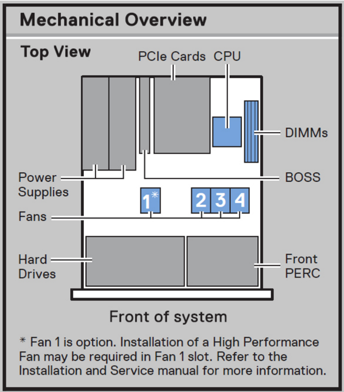
Ilustración 10. Descripción general de los aspectos mecánicos
