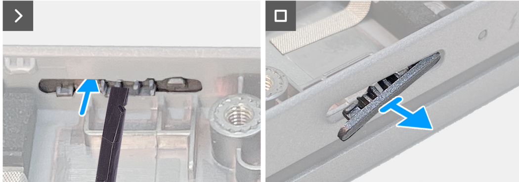
Abbildung 85. Entfernen des SIM-Karten-Platzhalters
