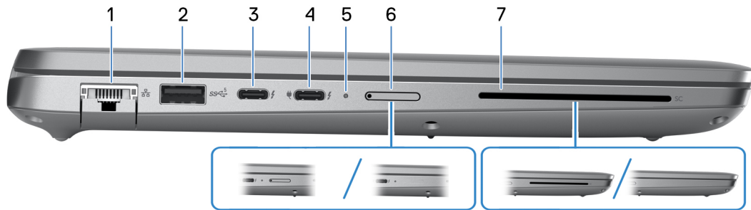
Abbildung 3. Linke Seitenansicht
