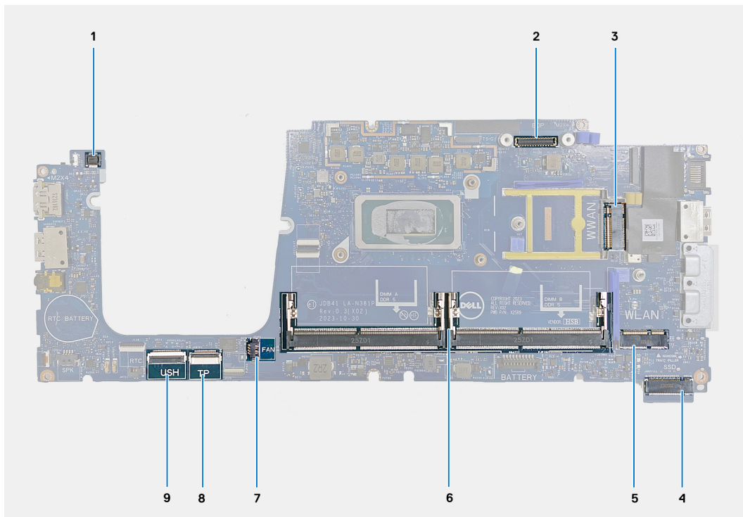
Abbildung 71. Hauptplatinenanschlüsse
