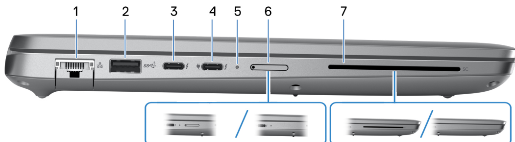
Figure 3. Vue de gauche
