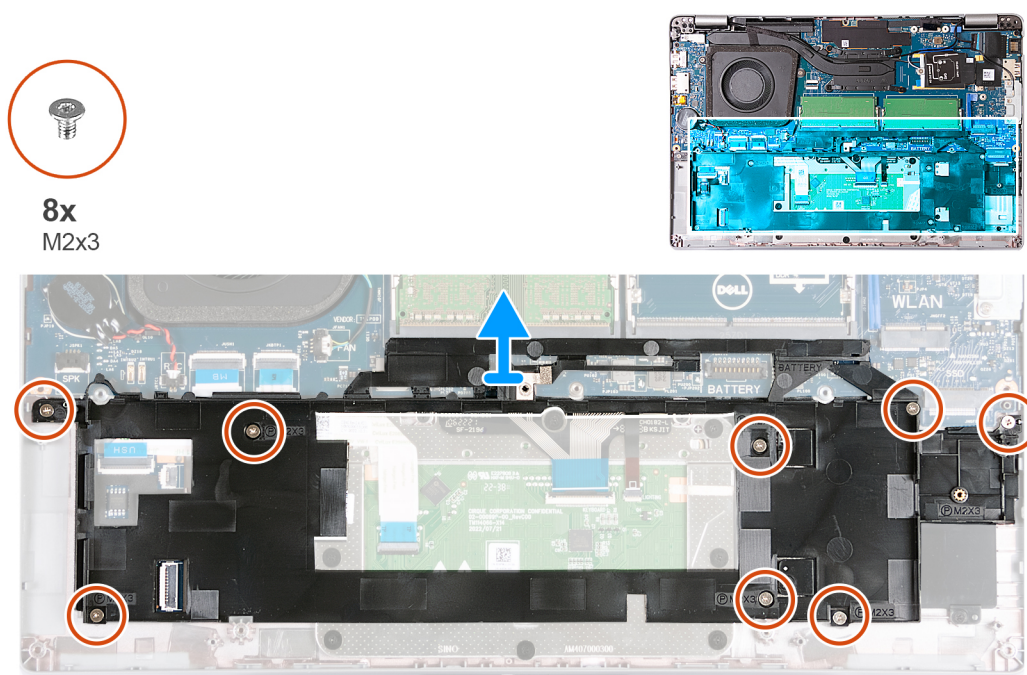
Figure 41. Retrait du cadre interne de l'assemblage
