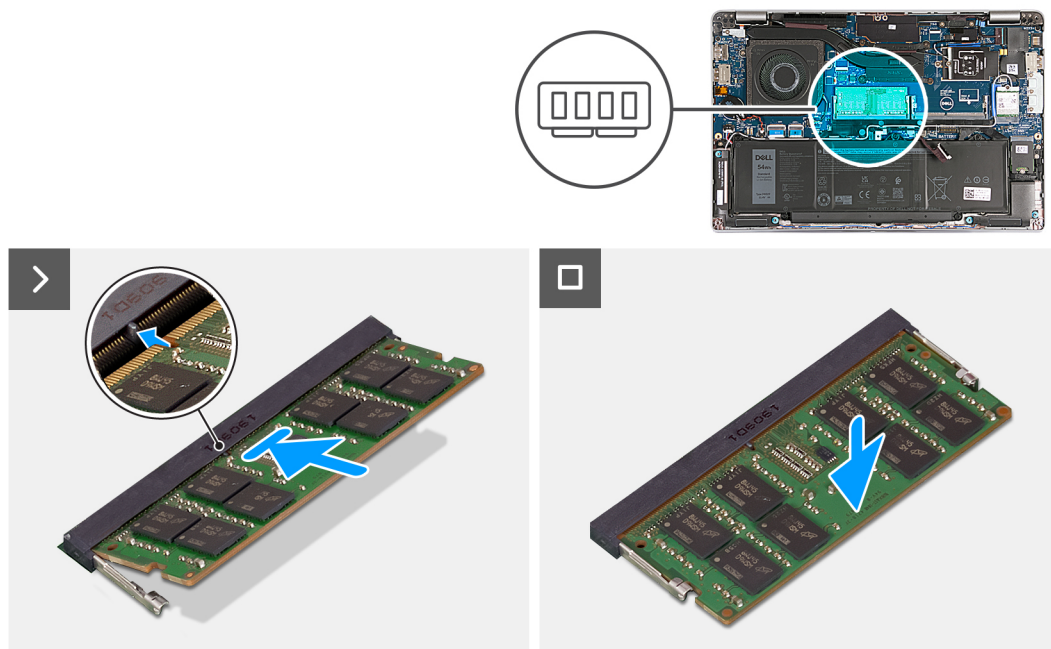
Figure 15. Installation du module de mémoire
