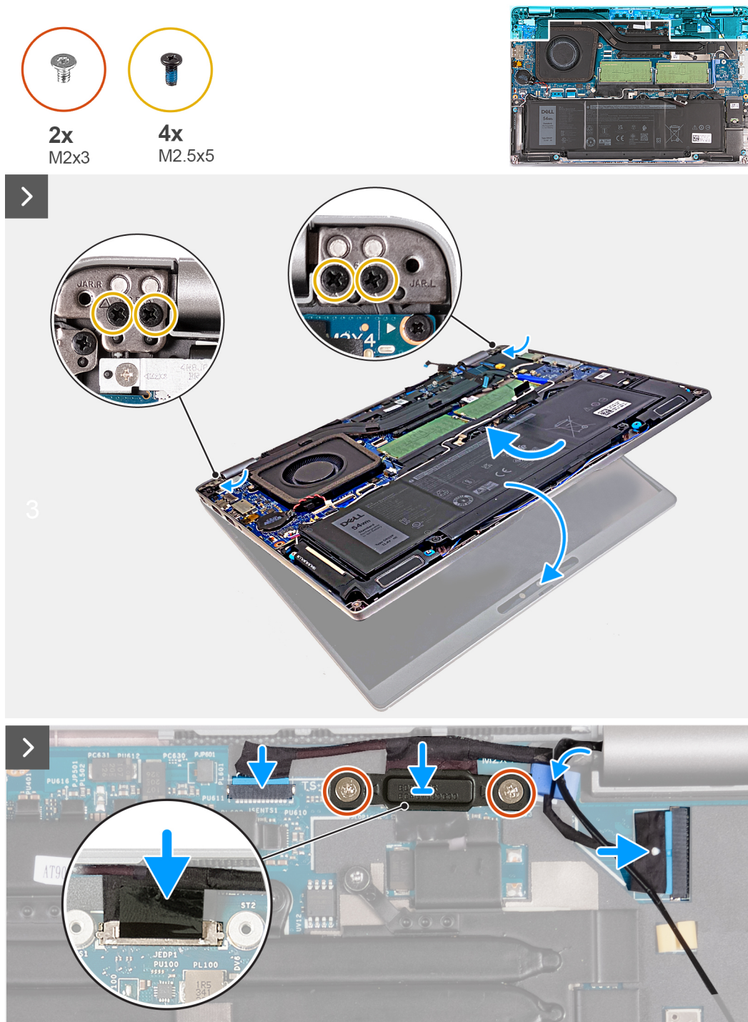
Figure 52. Installation de l'assemblage d'écran (pour les ordinateurs expédiés avec une carte graphique séparée)
