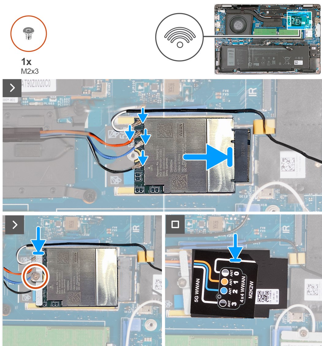
Figure 23. Installez la carte WWAN (pour les ordinateurs expédiés avec la carte 5G).
