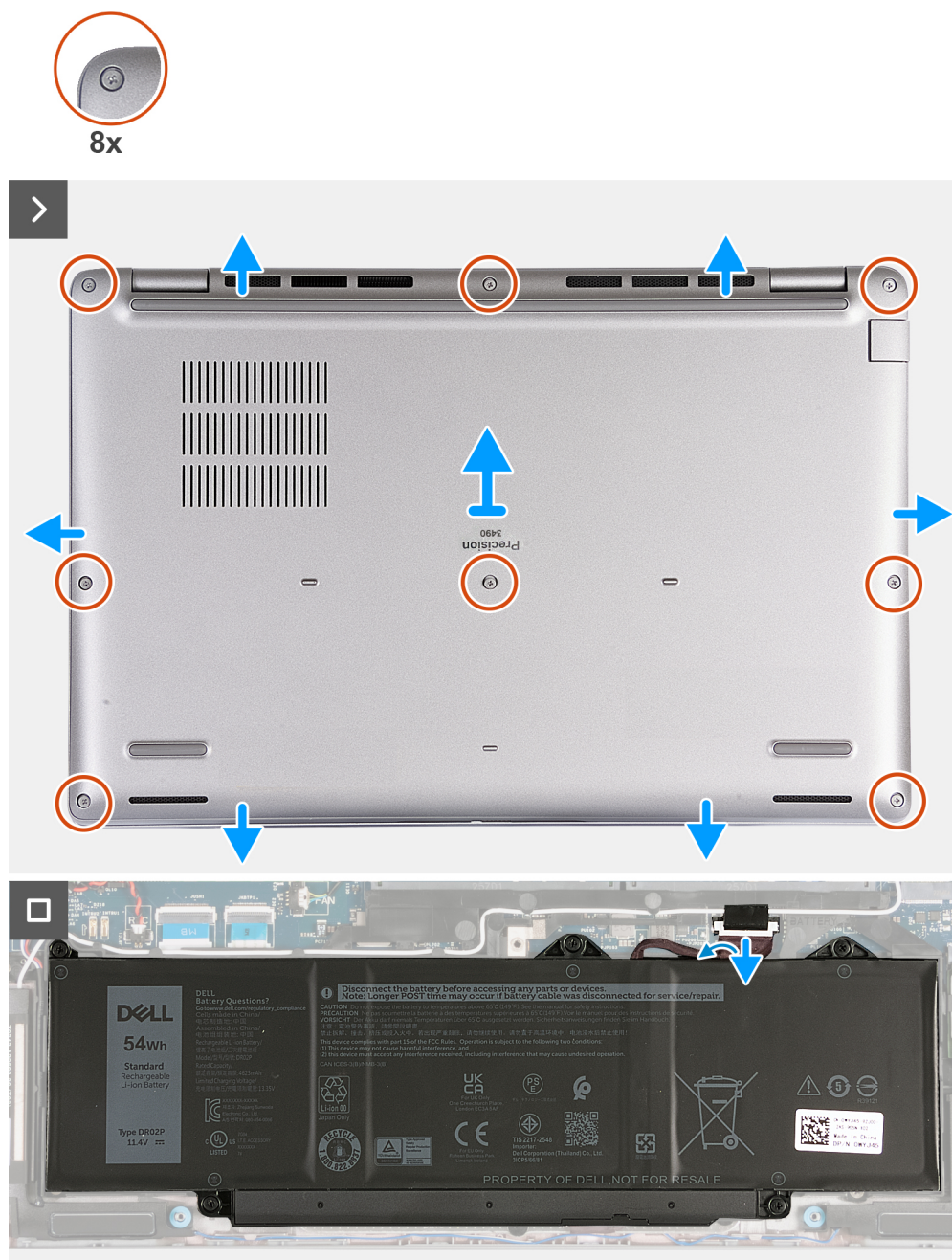
Figure 12. Retrait du cache de fond
