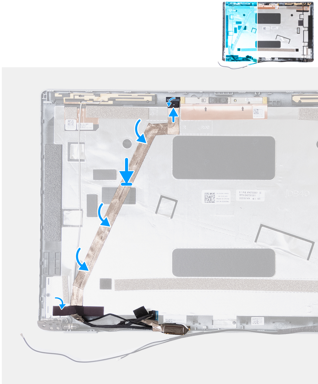
Figure 63. Installation du câble de l'écran
