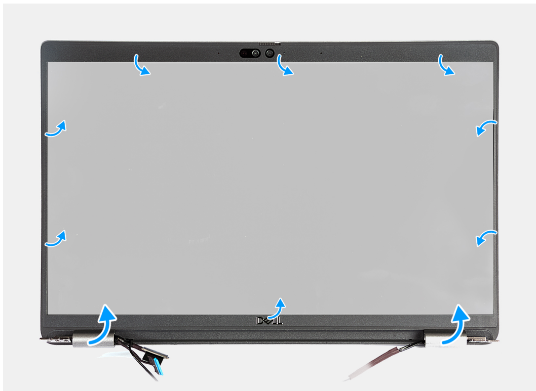
Figure 53. Retrait de la bordure d'écran
