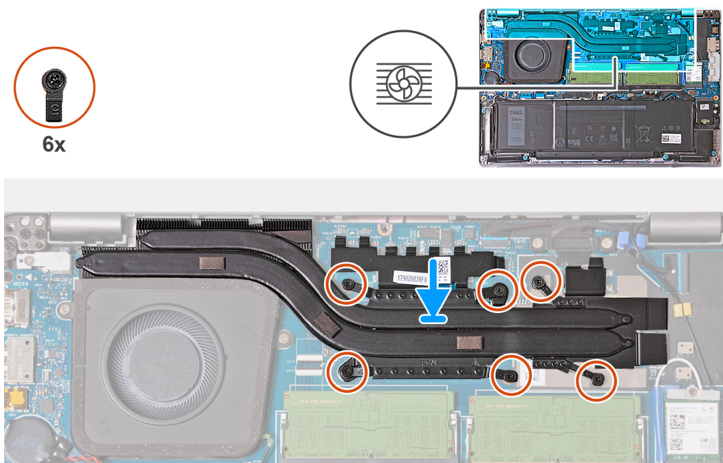
Figure 37. Installation du dissipateur de chaleur
