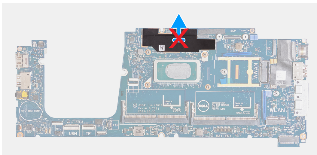
Figure 70. Capot de protection de l'alimentation (pour les ordinateurs expédiés avec une carte système U15)
