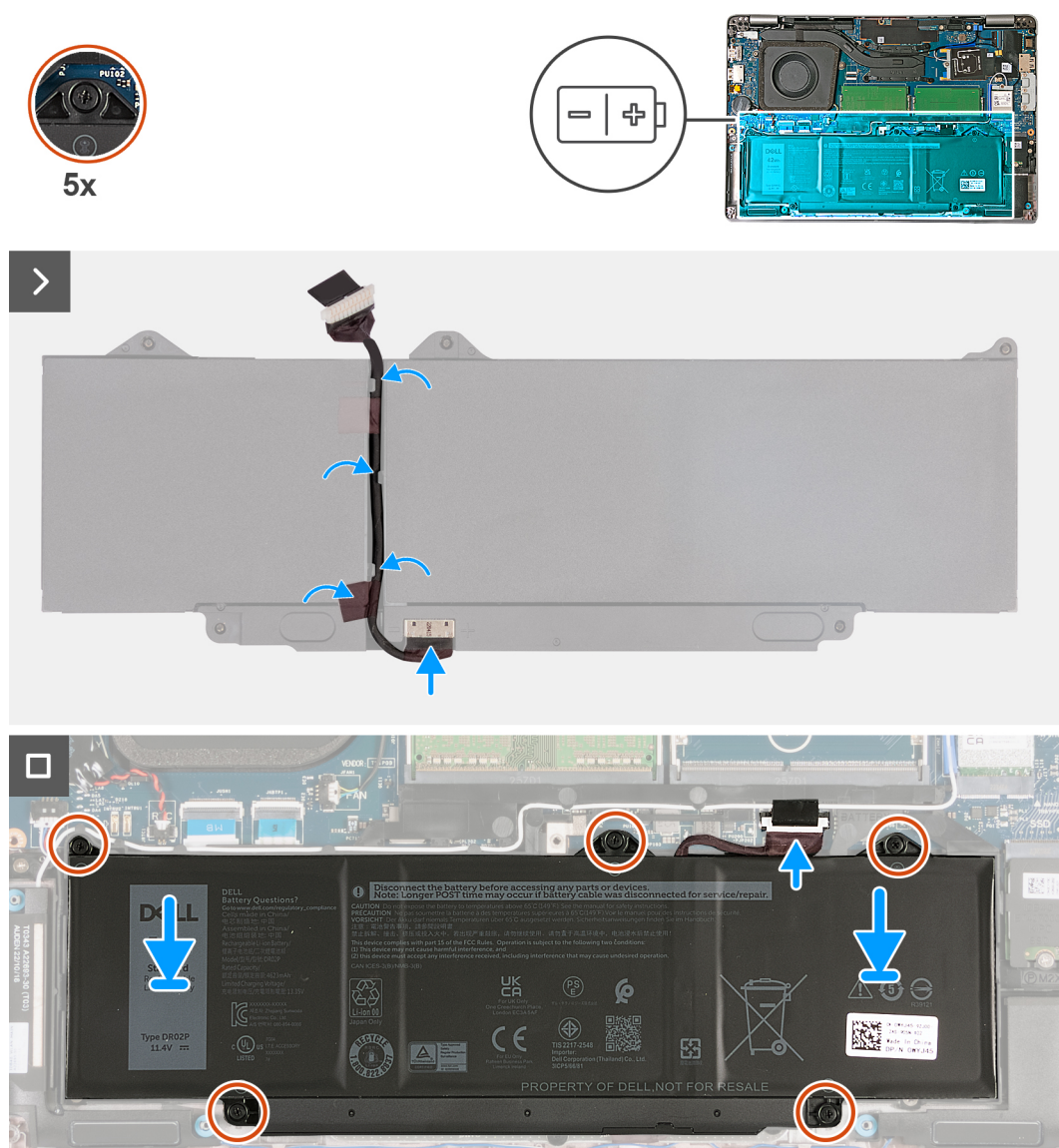
Figure 27. Installation de la batterie
