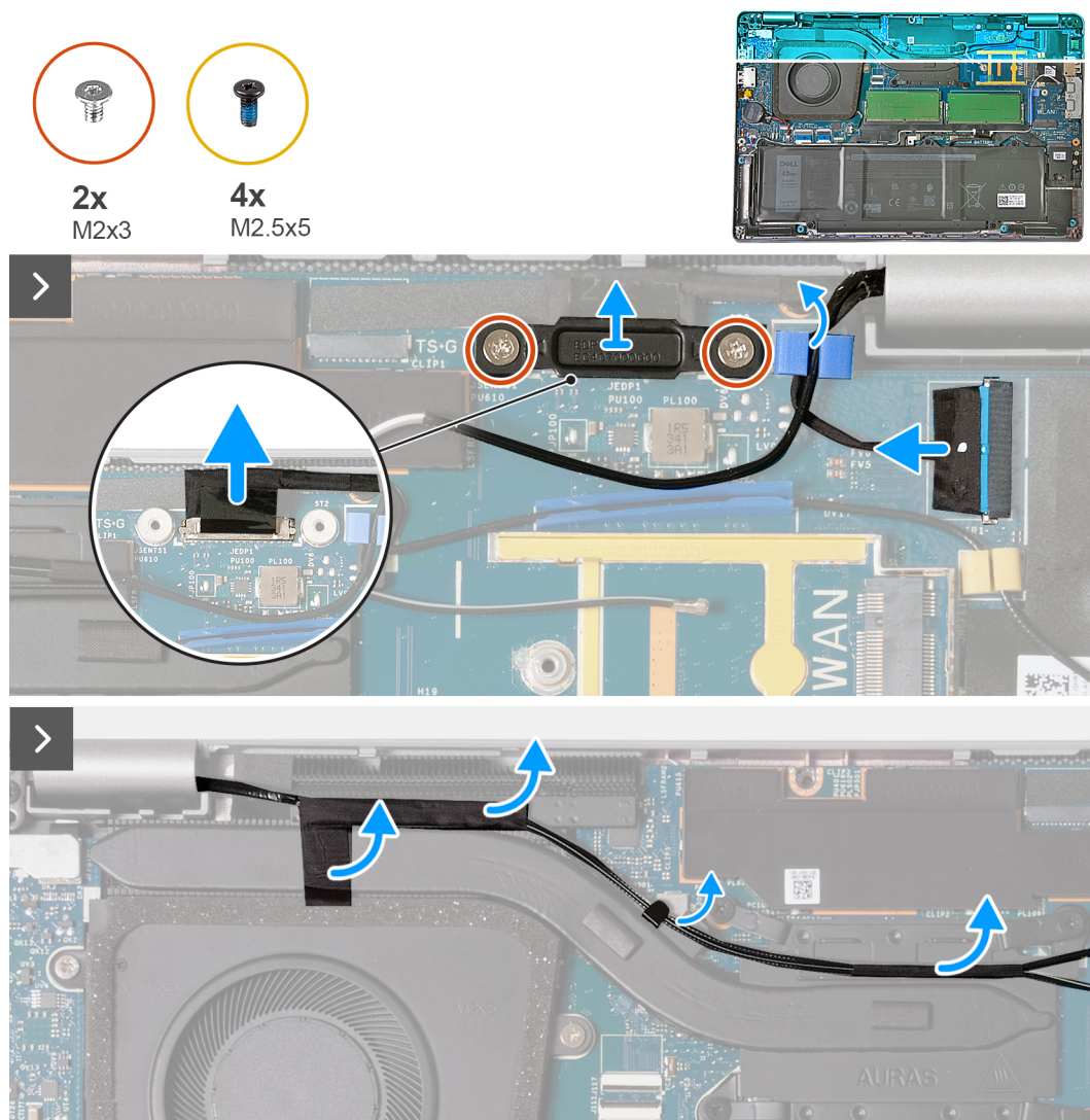
Figure 43. Retrait de l'assemblage d'écran (pour les ordinateurs expédiés avec une carte 4G)
