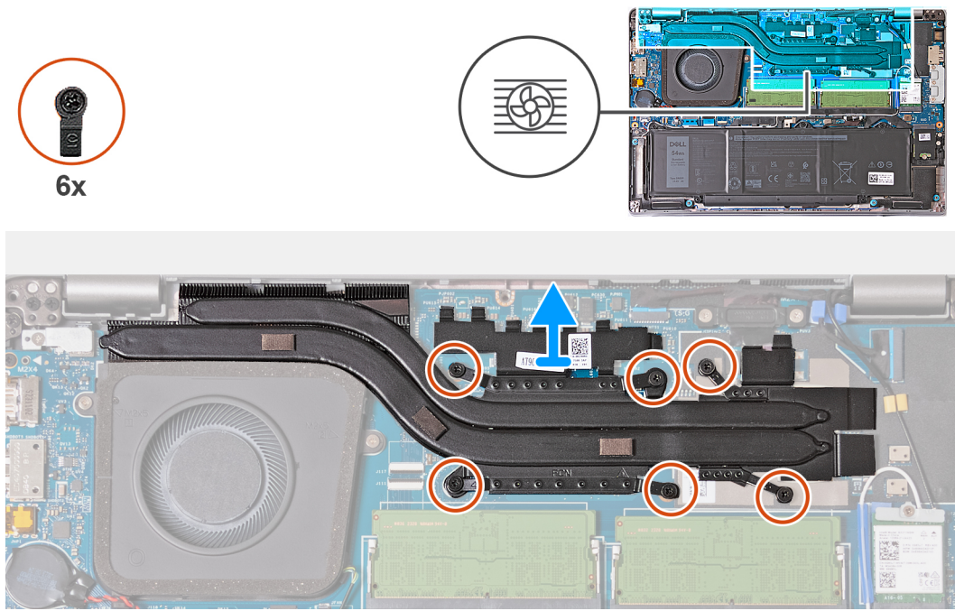
Figure 36. Retrait du dissipateur de chaleur
