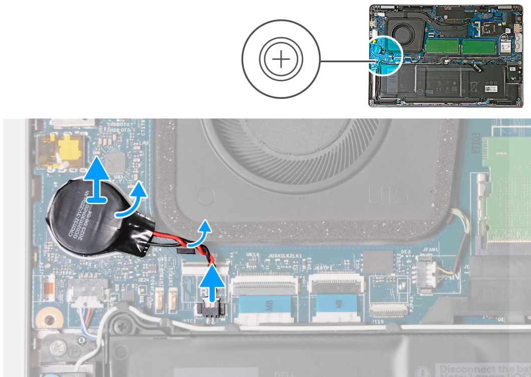
Figure 28. Retrait de la pile bouton
