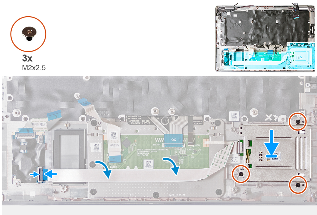
Figure 76. Installation du lecteur de carte à puce
