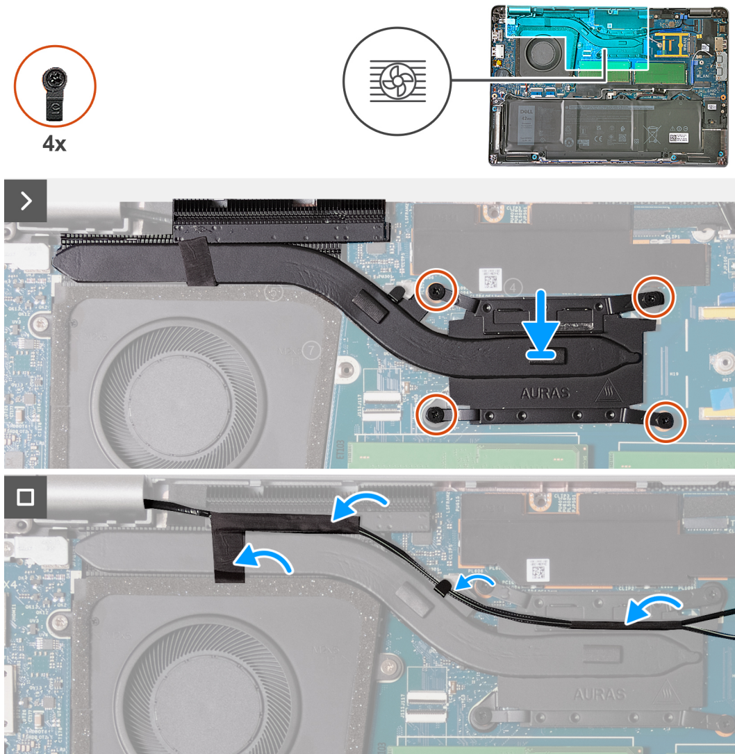
Figure 33. Installation du dissipateur de chaleur (pour les ordinateurs expédiés avec une carte 4G)
