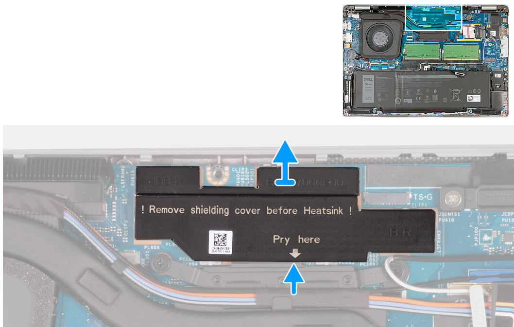
Figure 31. Retrait du capot de protection de l'alimentation (pour les ordinateurs expédiés avec une carte système UMA H28)
