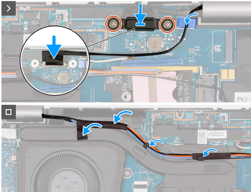
Figure 50. Installation de l'assemblage d'écran (pour les ordinateurs expédiés avec une carte 5G)
