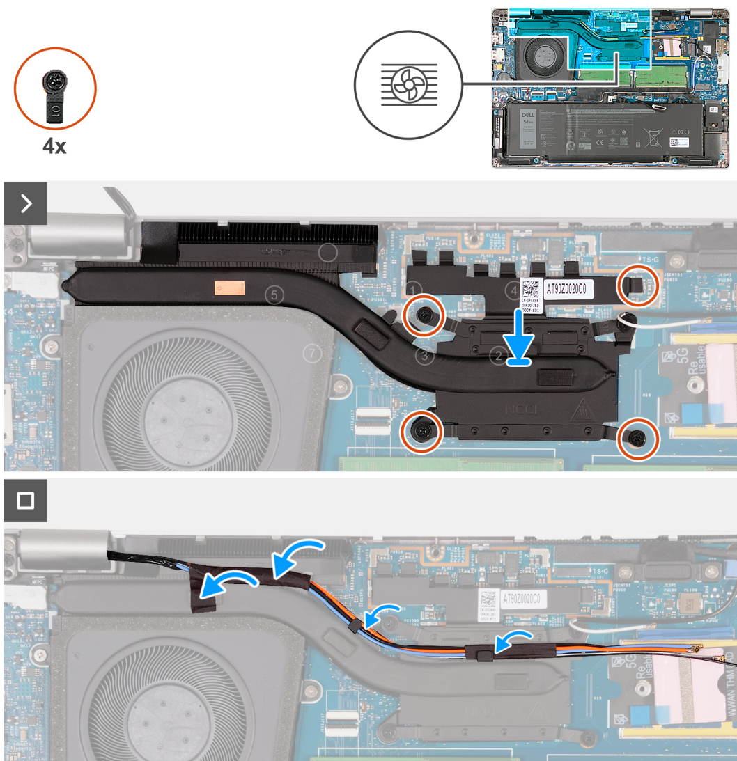
Figure 34. Installation du dissipateur de chaleur (pour les ordinateurs expédiés avec une carte 5G)
