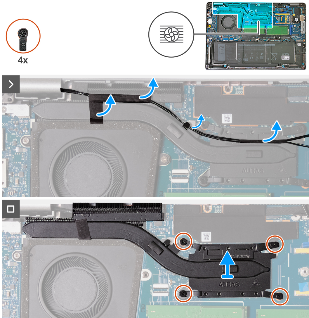
Figure 30. Retrait du dissipateur de chaleur (pour les ordinateurs expédiés avec une carte 4G)
