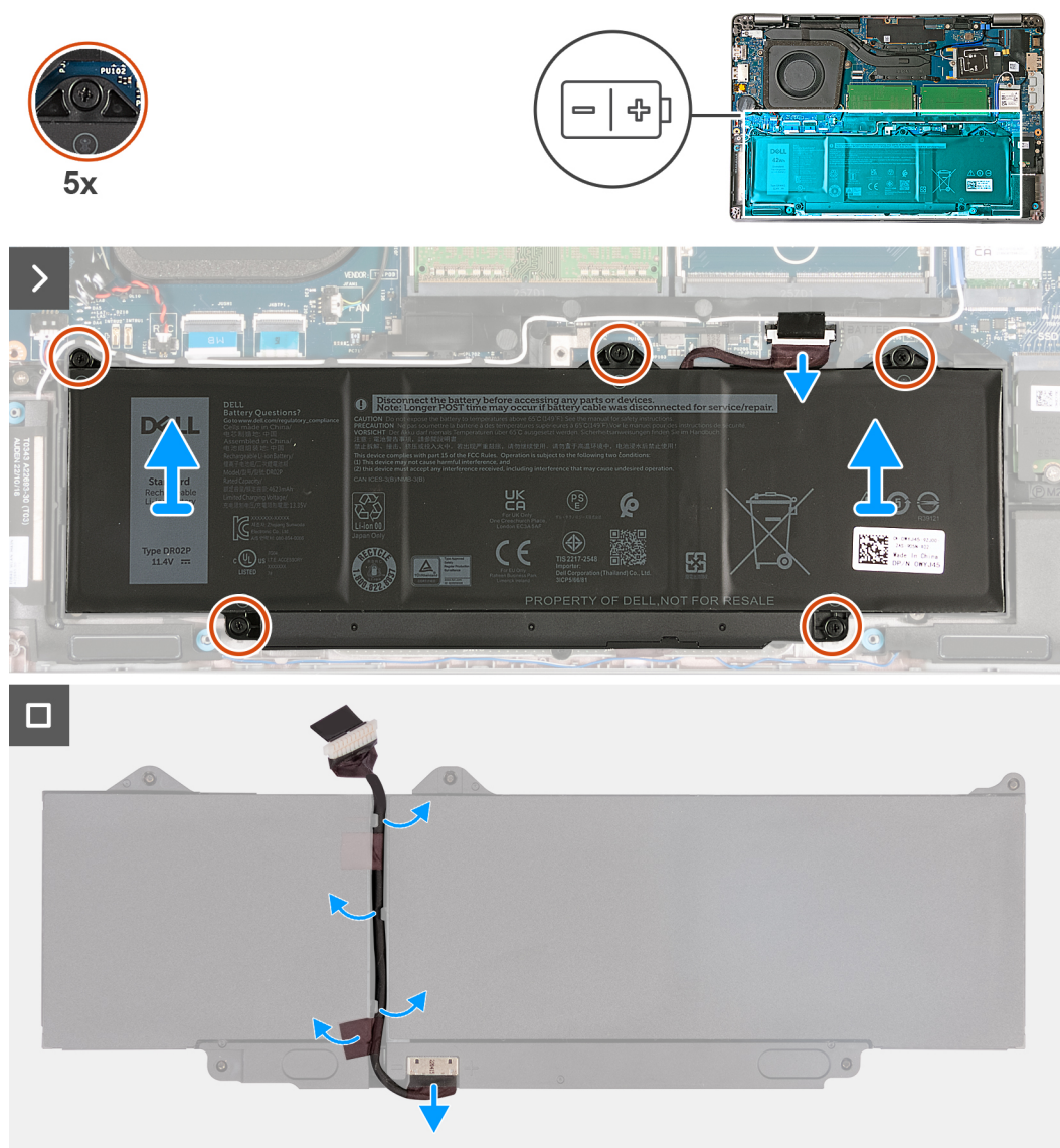
Figure 26. Retrait de la batterie
