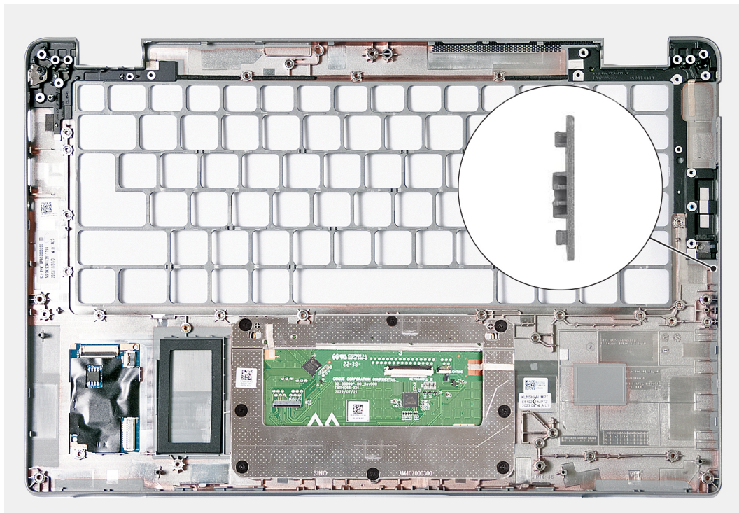
Figure 83. Retrait de l'assemblage du repose-poignets
