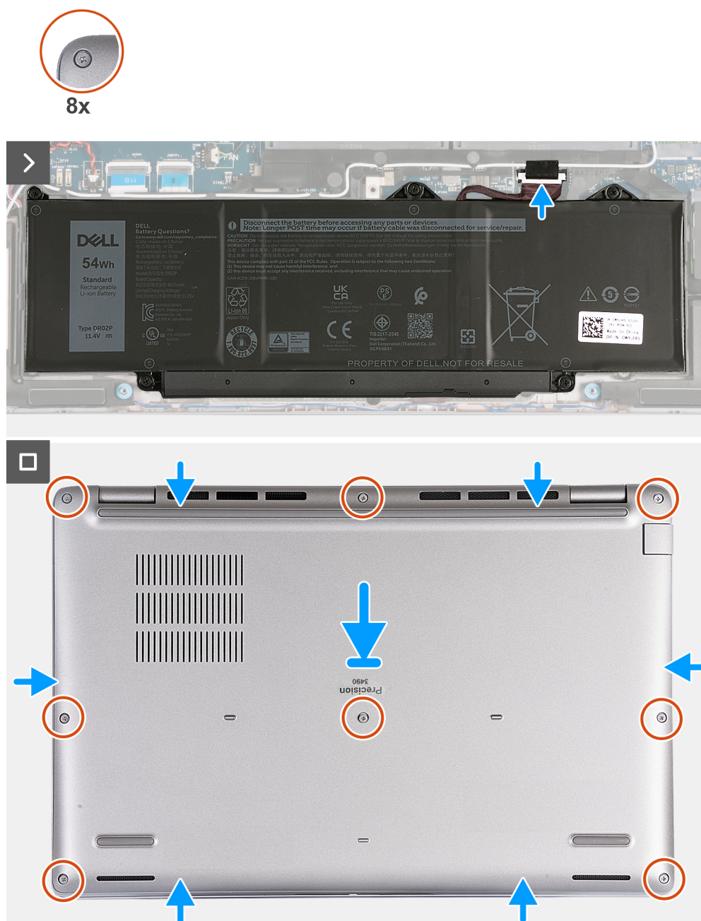
Figure 13. Installation du cache de fond
