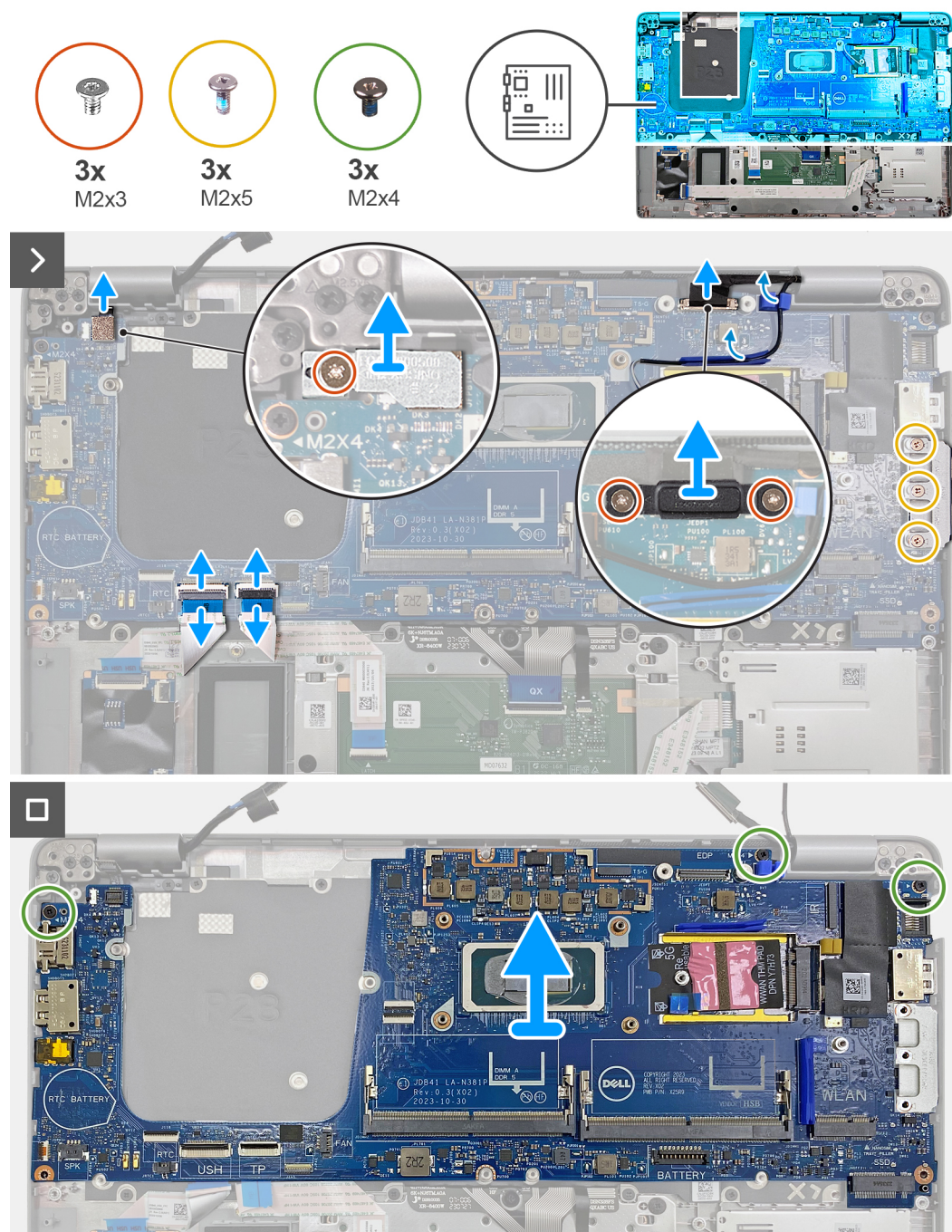
Figure 68. Retrait de la carte système
