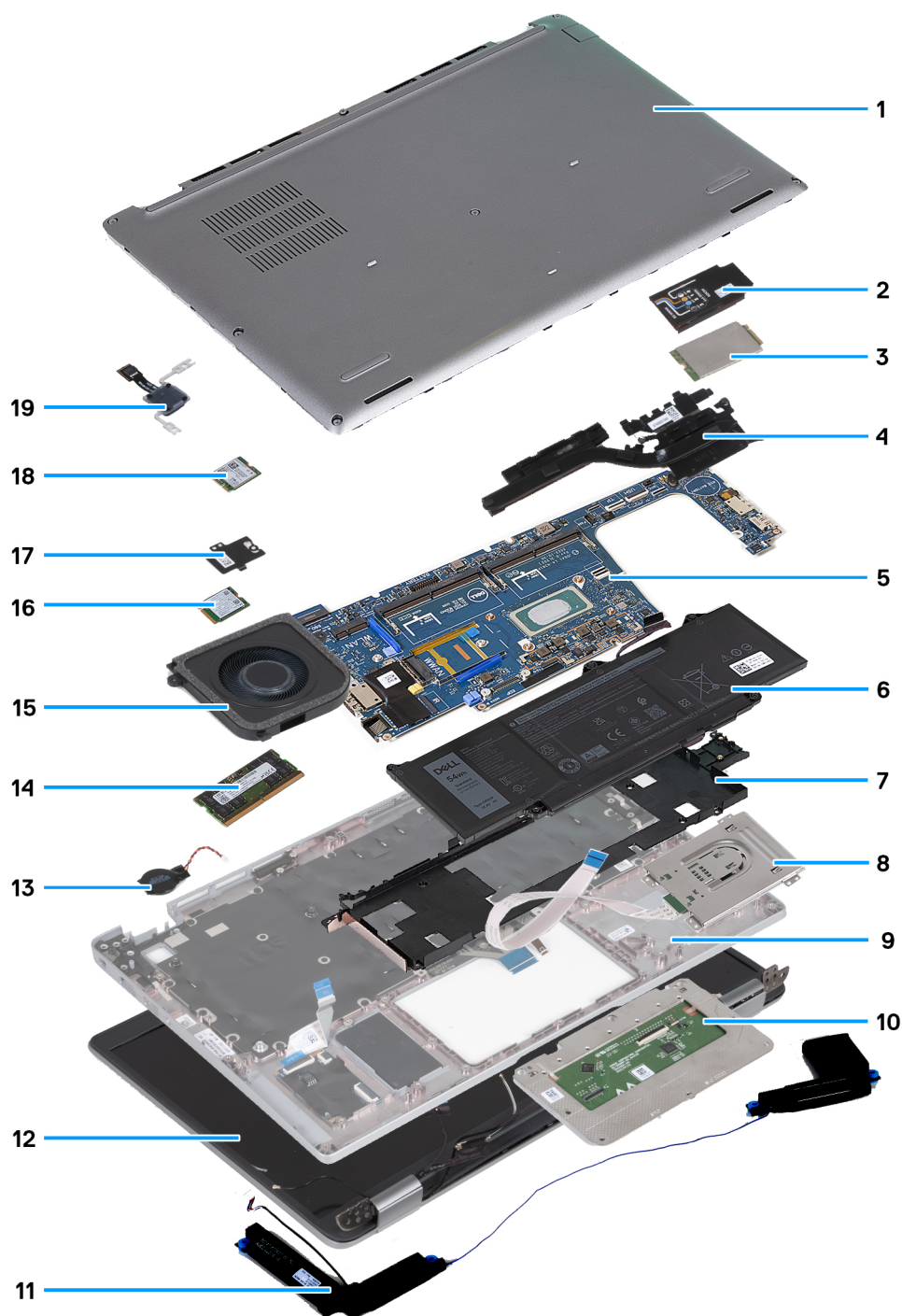
Figure 9. Principaux composants de votre ordinateur
