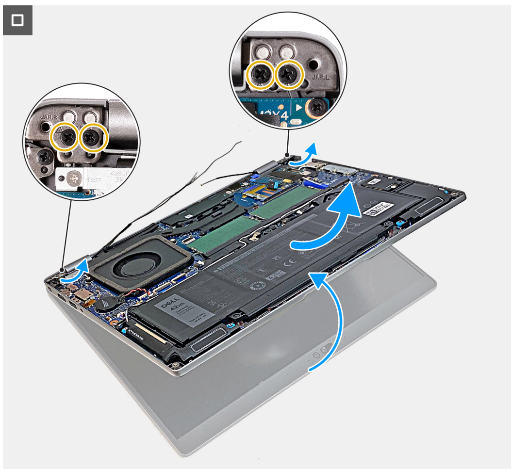
Figure 44. Retrait de l'assemblage d'écran (pour les ordinateurs expédiés avec une carte 4G)
