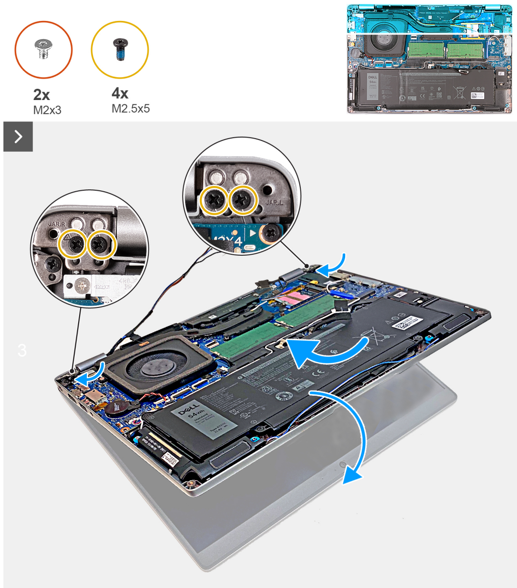
Figure 49. Installation de l'assemblage d'écran (pour les ordinateurs expédiés avec une carte 5G)
