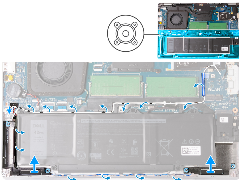
Figure 38. Retrait des haut-parleurs
