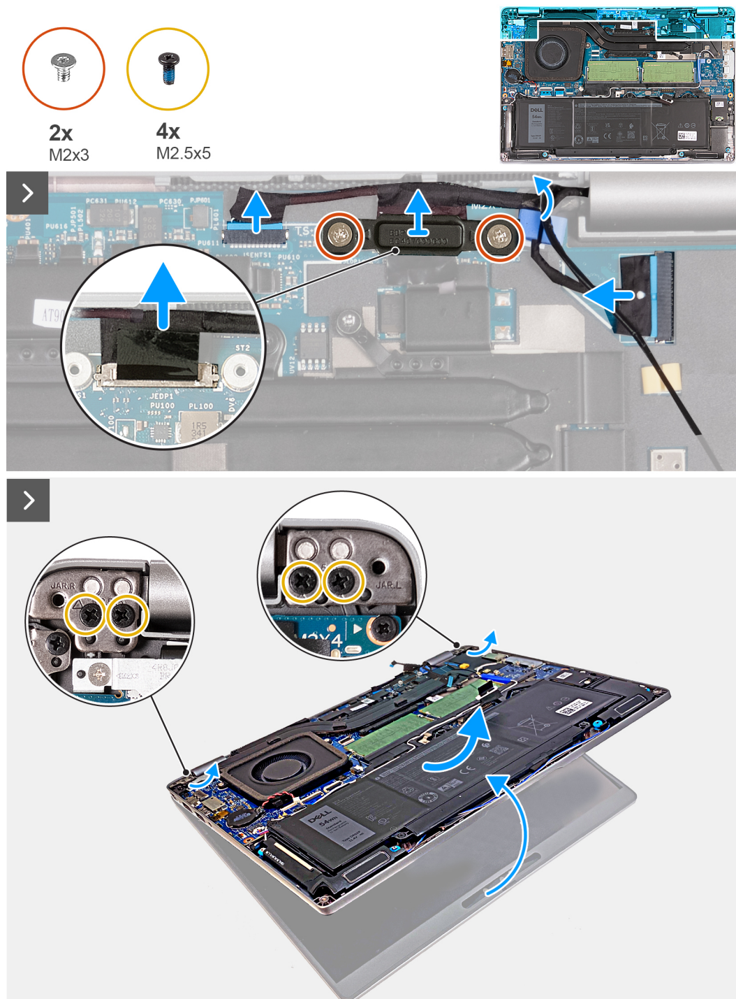
Figure 51. Retrait de l'assemblage d'écran (pour les ordinateurs expédiés avec une carte graphique séparée)
