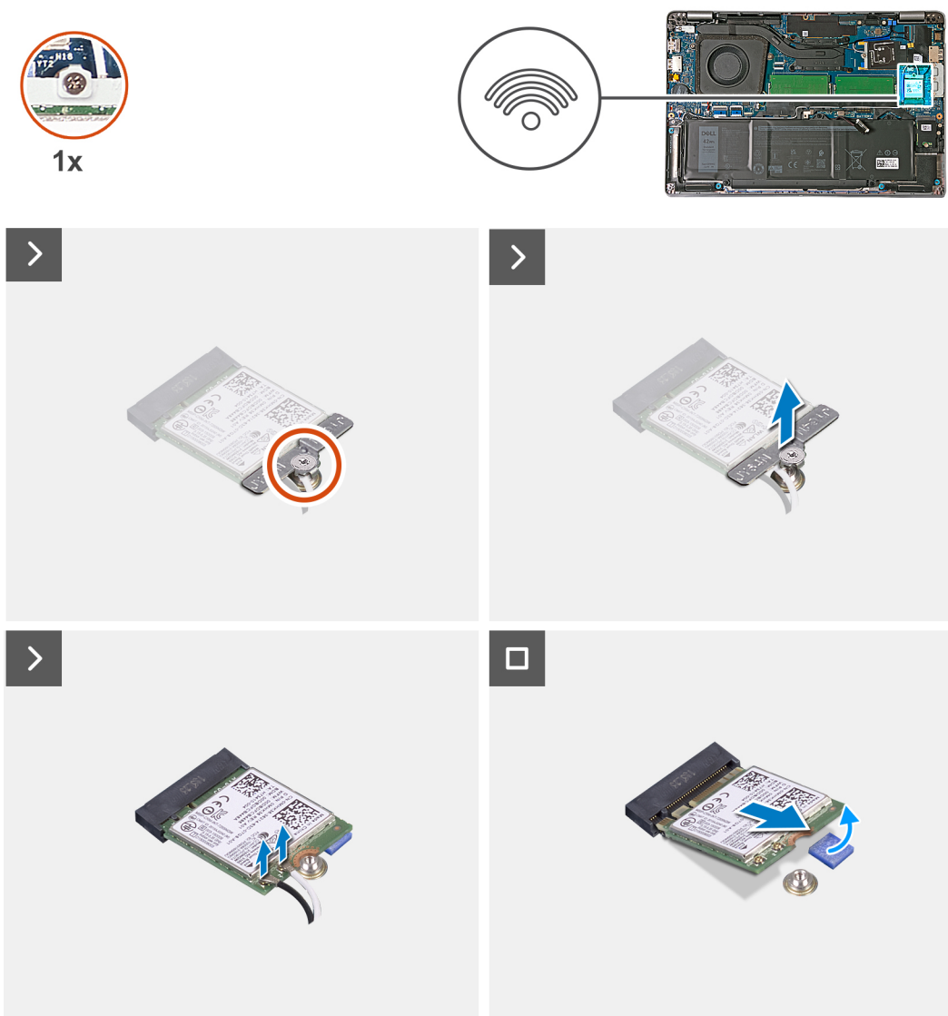
Figure 18. Retrait de la carte sans fil
