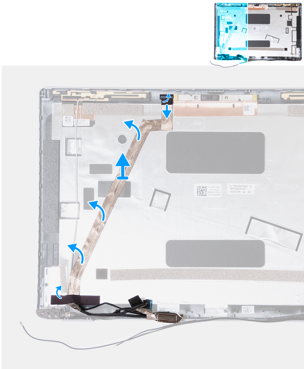
Figure 62. Retrait du câble de l'écran
