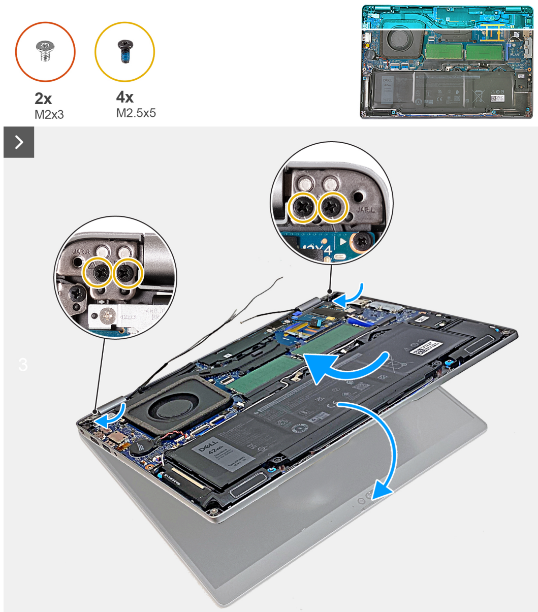
Figure 47. Installation de l'assemblage d'écran (pour les ordinateurs expédiés avec une carte 4G)
