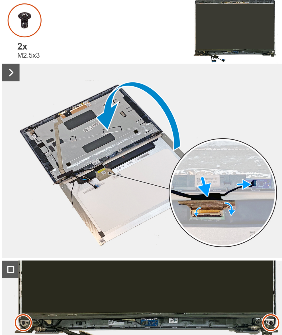
Figure 57. Installation du panneau d'écran
