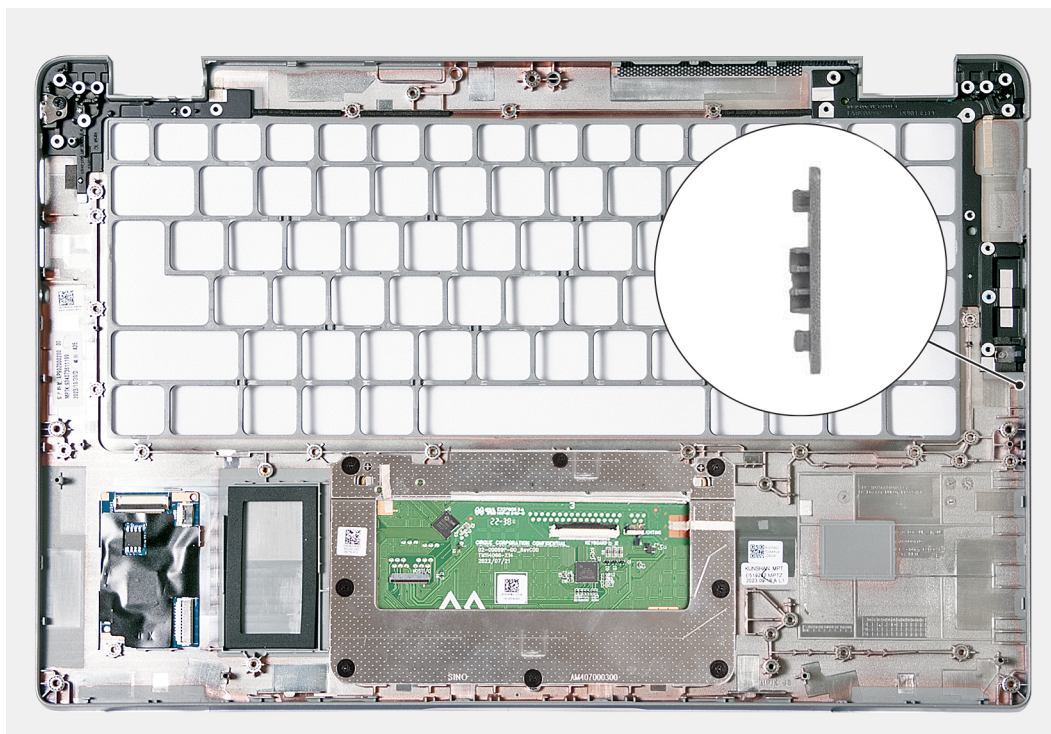
Figure 84. Installation de l'assemblage du repose-poignets
