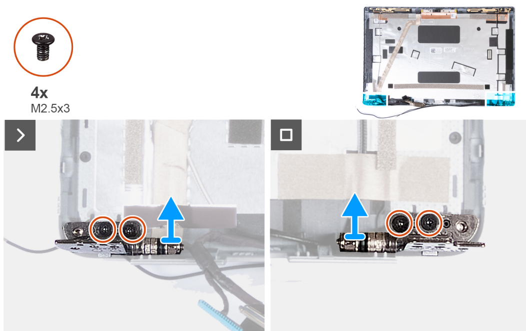
Figure 60. Retrait des charnières d'écran
