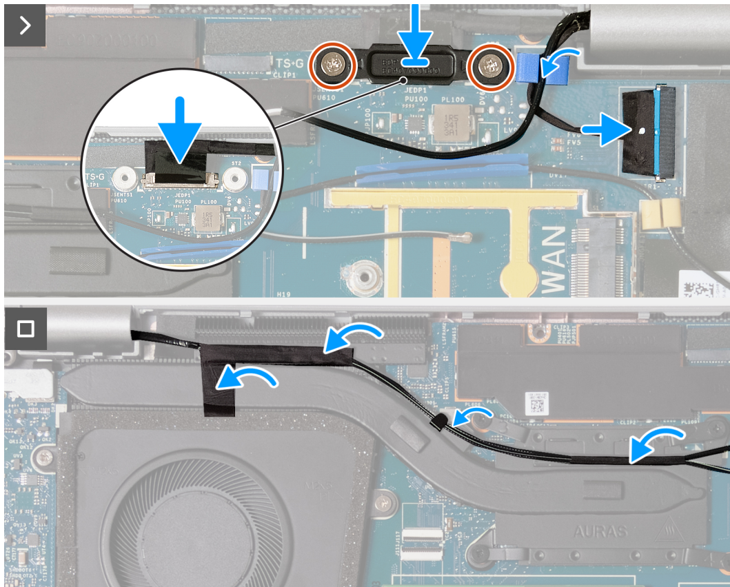
Figure 48. Installation de l'assemblage d'écran (pour les ordinateurs expédiés avec une carte 4G)
