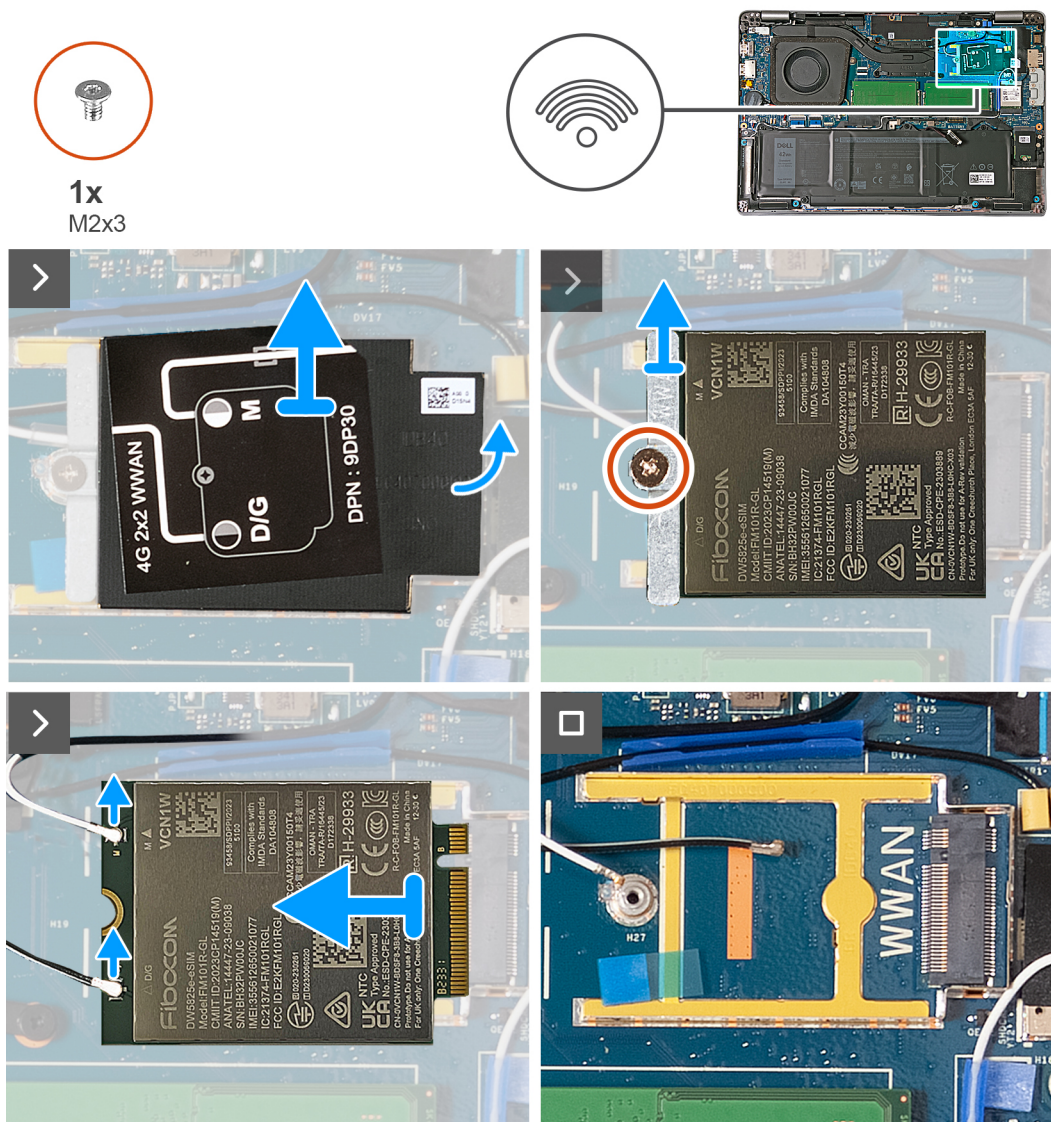
Figure 20. Retirez la carte WWAN (pour les ordinateurs expédiés avec une carte 4G)
