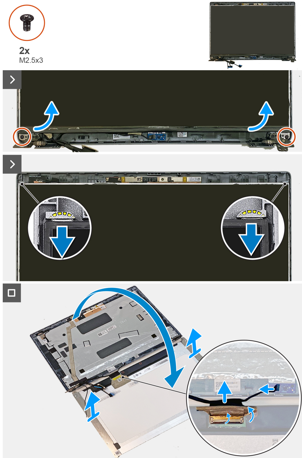
Figure 55. Retrait du panneau d'écran
