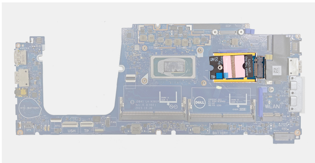
Figure 69. Tampon thermique de la carte WWAN
