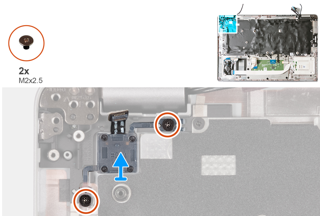
Figure 77. Retrait de la carte du bouton d'alimentation
