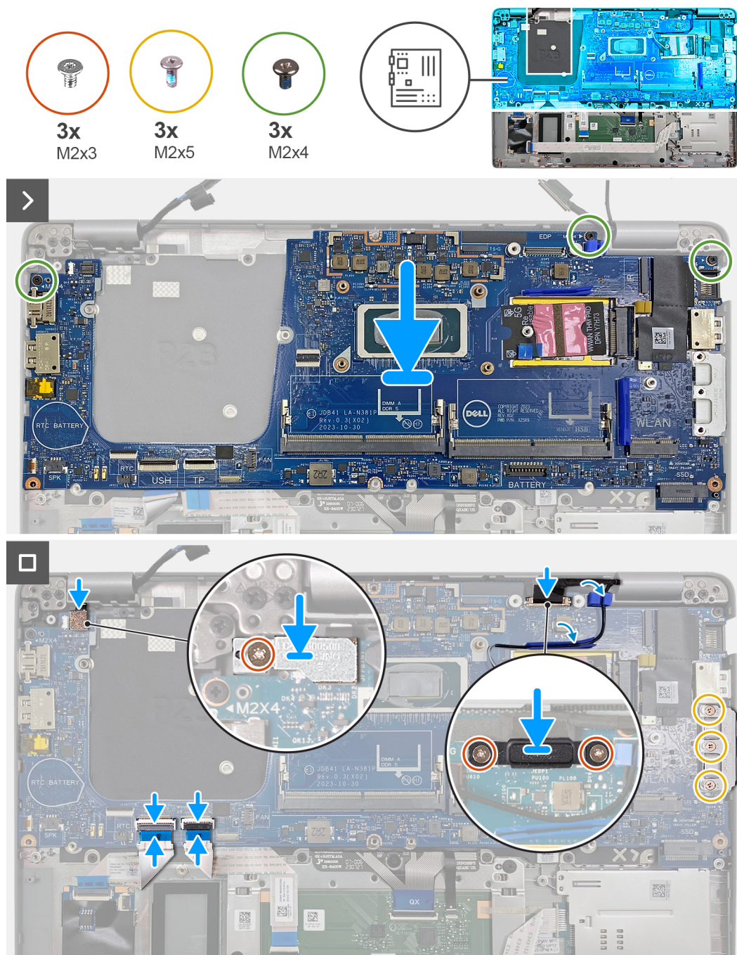
Figure 72. Installation de la carte système
