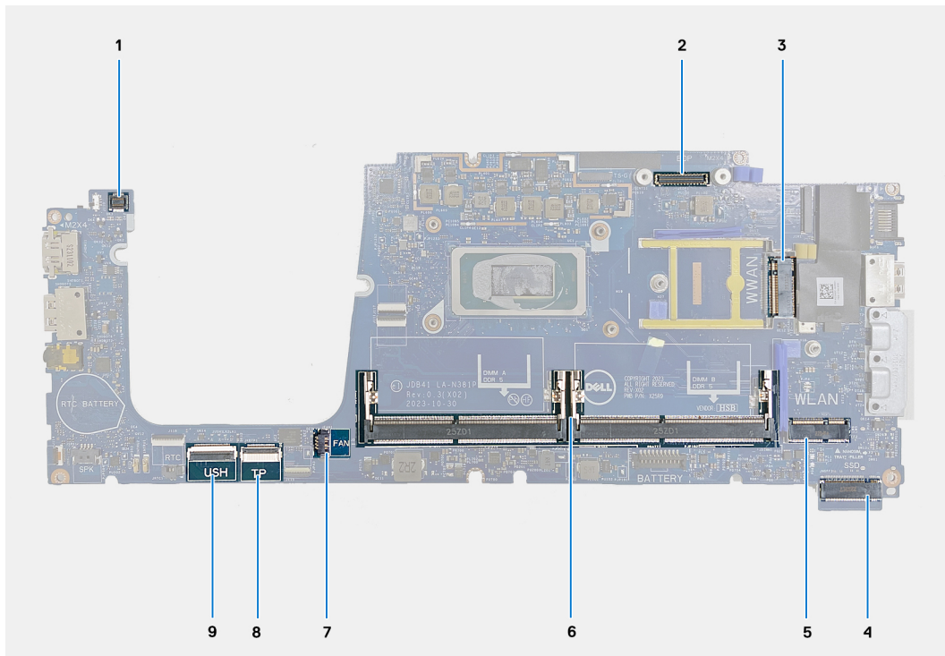
Figure 67. Connecteurs de la carte système
