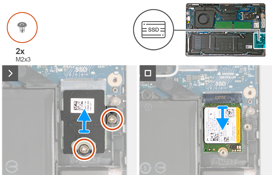
Figure 16. Retrait du disque SSD M.2 2230
