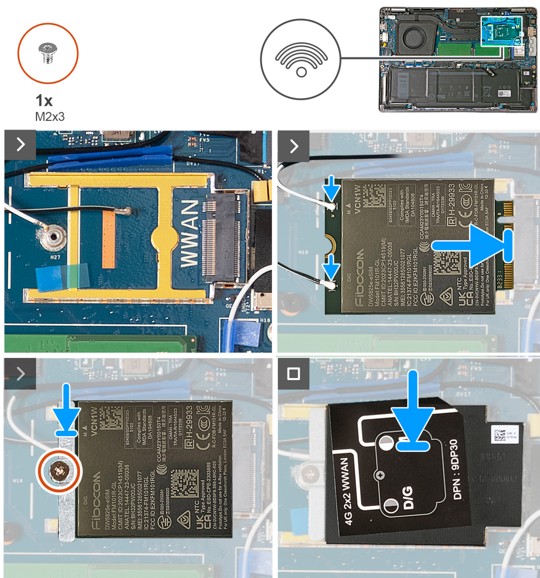
Figure 22. Installez la carte WWAN (pour les ordinateurs expédiés avec la carte 4G).
