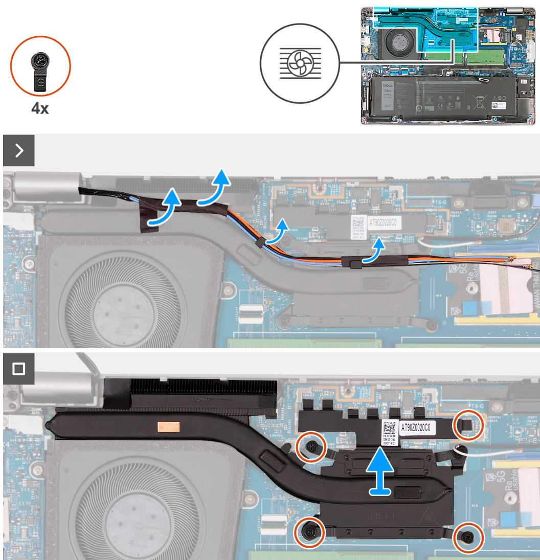
Figure 32. Retrait du dissipateur de chaleur (pour les ordinateurs expédiés avec une carte 5G)
