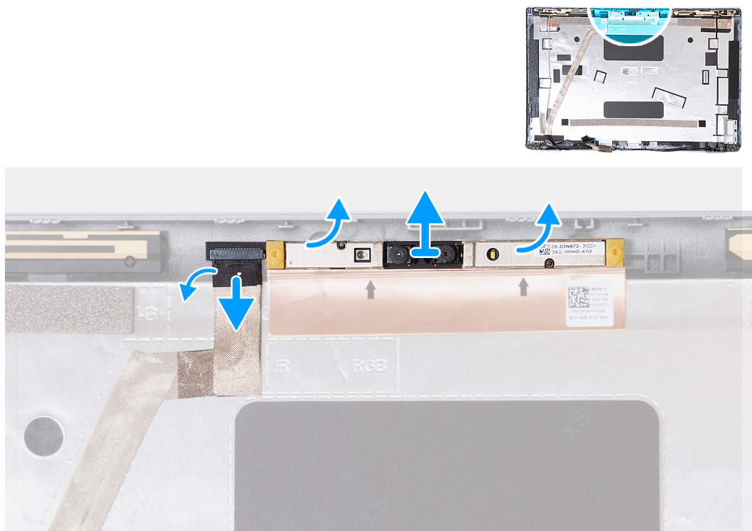
Figure 58. Retrait du module de caméra
