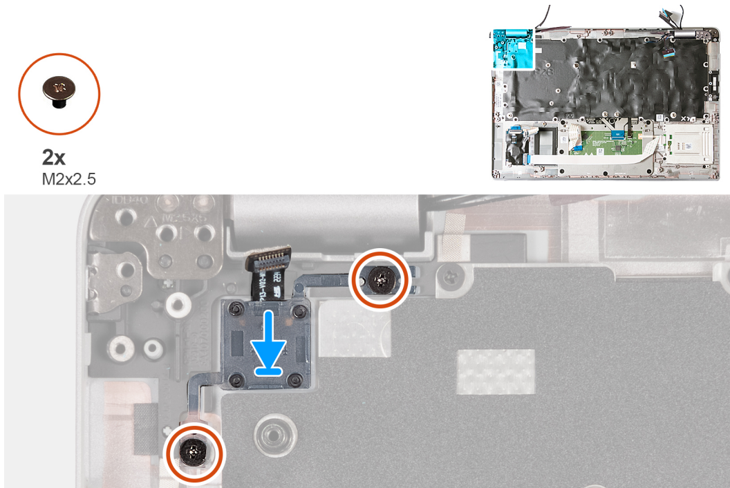
Figure 78. Installation de la carte du bouton d'alimentation
