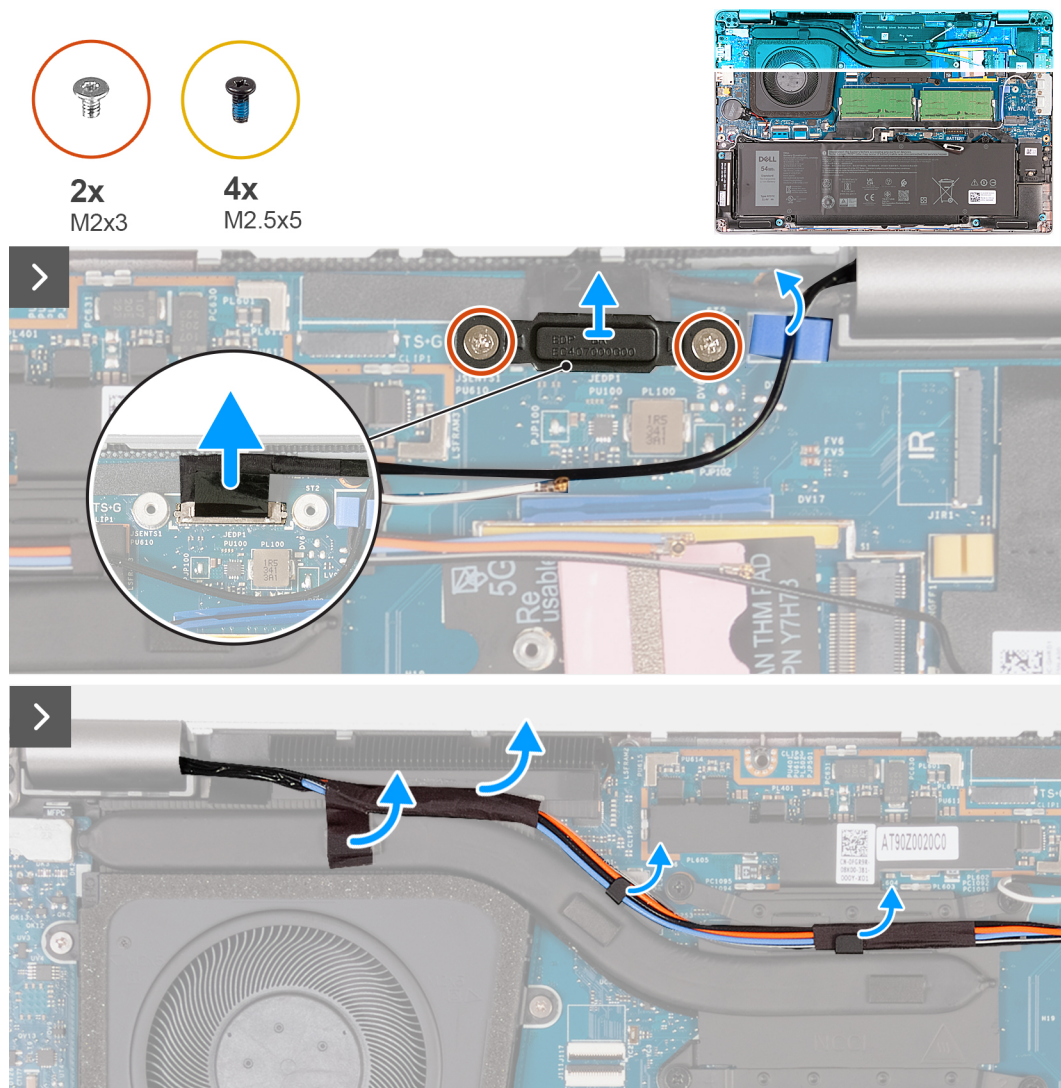
Figure 45. Retrait de l'assemblage d'écran (pour les ordinateurs expédiés avec une carte 5G)
