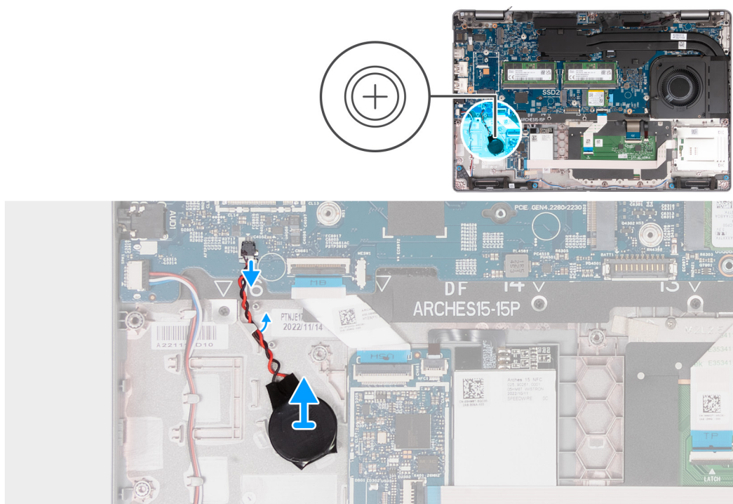
Rysunek 50. Wymontowywanie baterii pastylkowej
