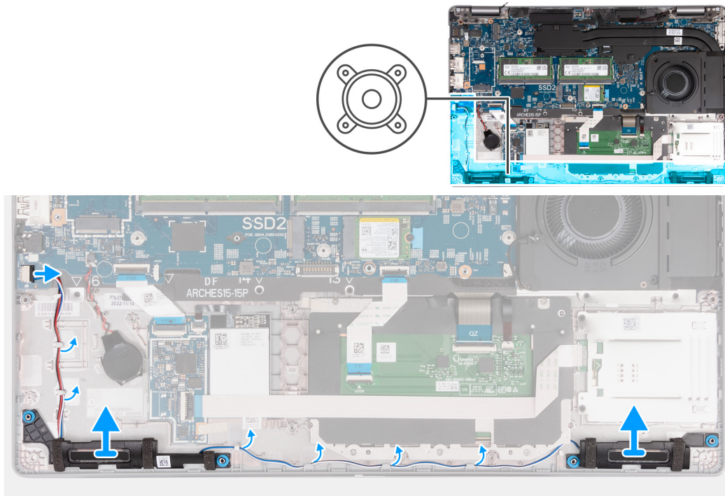
Rysunek 47. Wymontowywanie głośników
