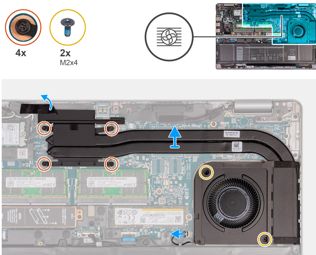
Rysunek 54. Wymontowywanie zestawu wentylatora i radiatora (zintegrowana karta graficzna)
