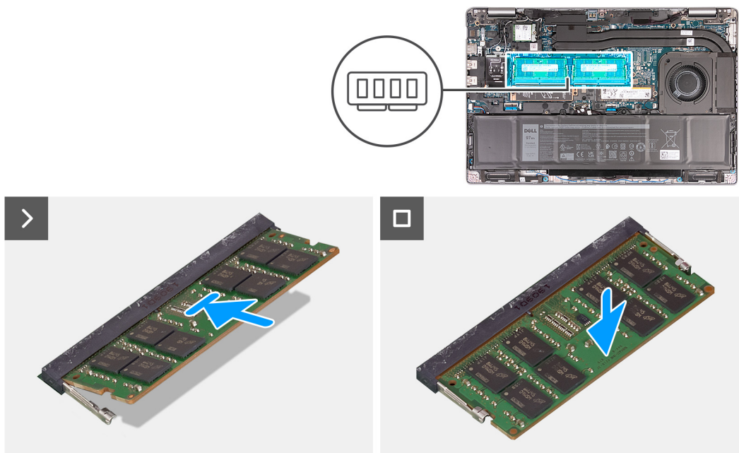
Rysunek 26. Instalowanie modułu pamięci
