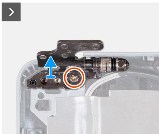
Rysunek 90. Wymontowywanie zawiasów wyświetlacza
