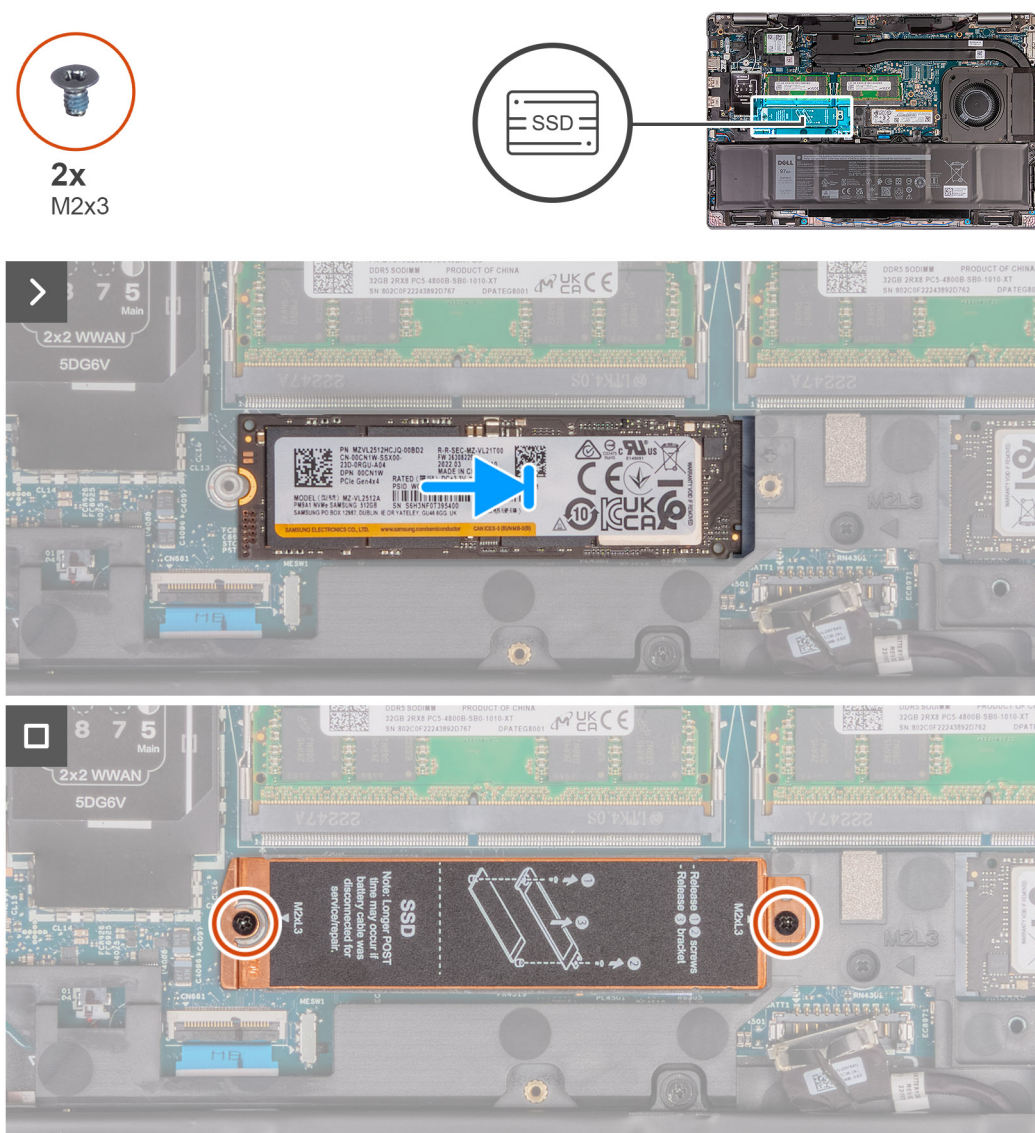
Rysunek 34. Instalowanie dysku SSD M.2 2280 w gnieździe 2
