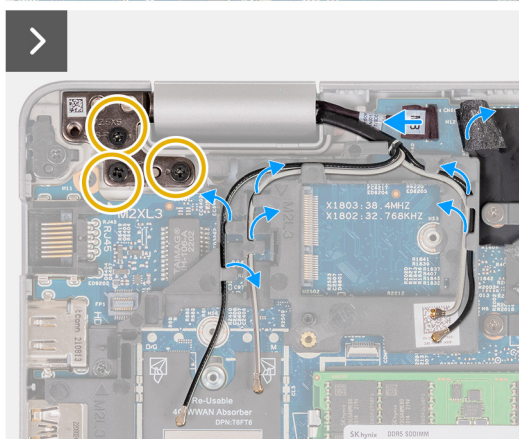
Rysunek 73. Wymontowywanie zestawu wyświetlacza
