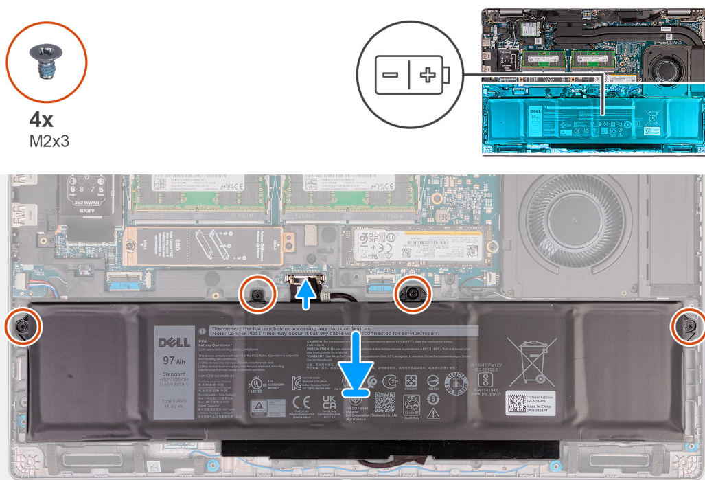
Rysunek 40. Instalowanie baterii 97 Wh
