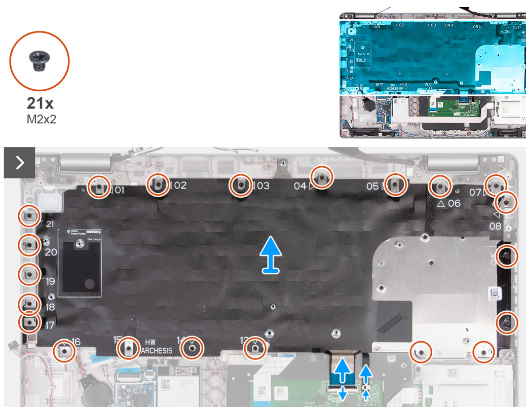
Rysunek 69. Wymontowywanie klawiatury
