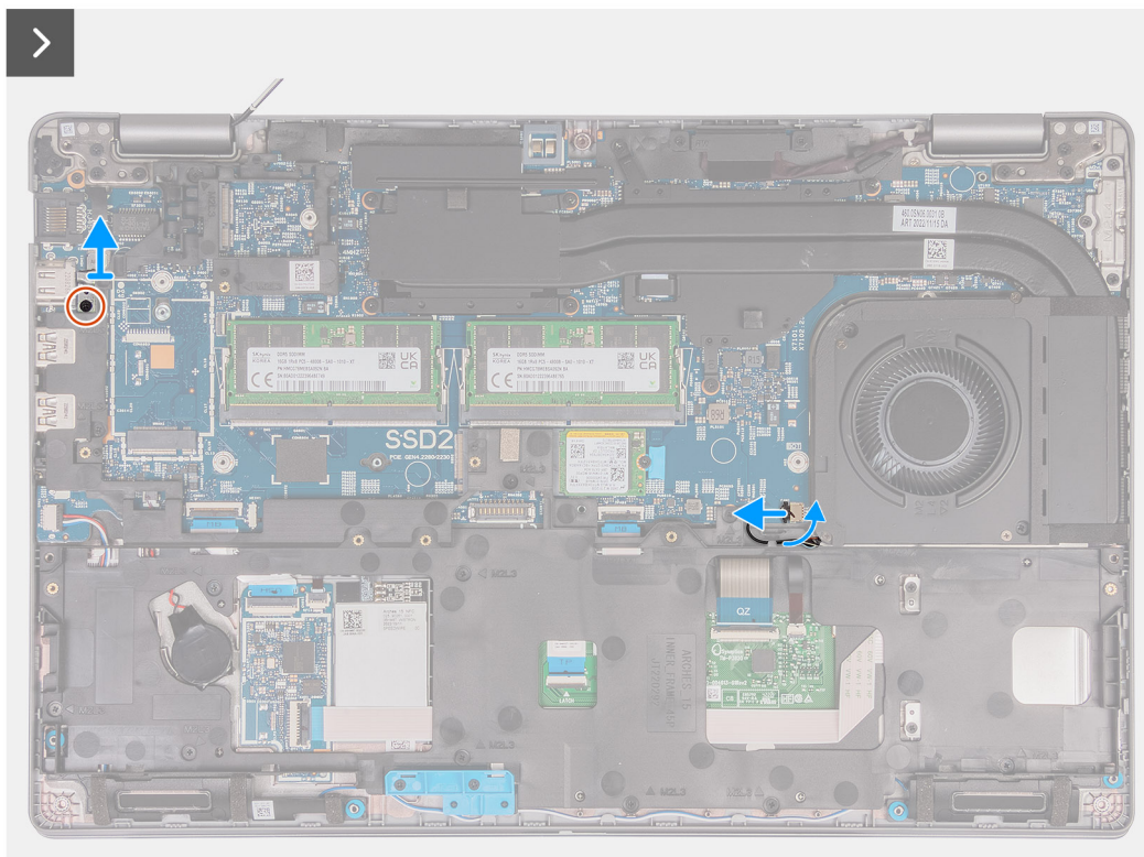
Rysunek 41. Wymontowywanie wewnętrznej ramy montażowej
