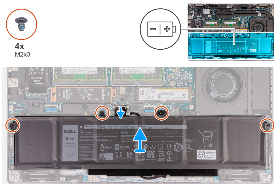
Rysunek 38. Wymontowywanie baterii 97 Wh
