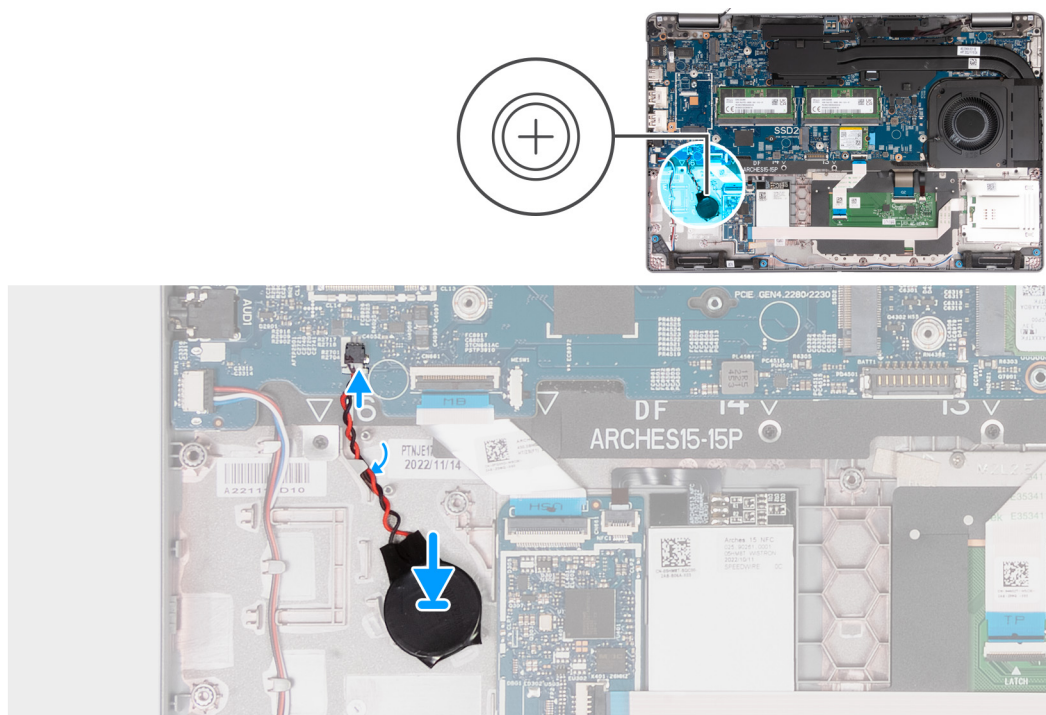
Rysunek 51. Instalowanie baterii pastylkowej
