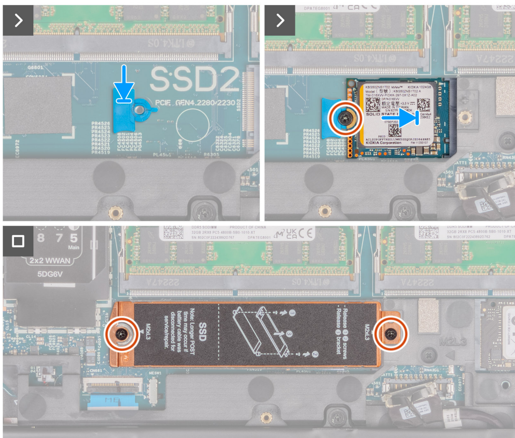
Rysunek 32. Instalowanie dysku SSD M.2 2230 w gnieździe 2
