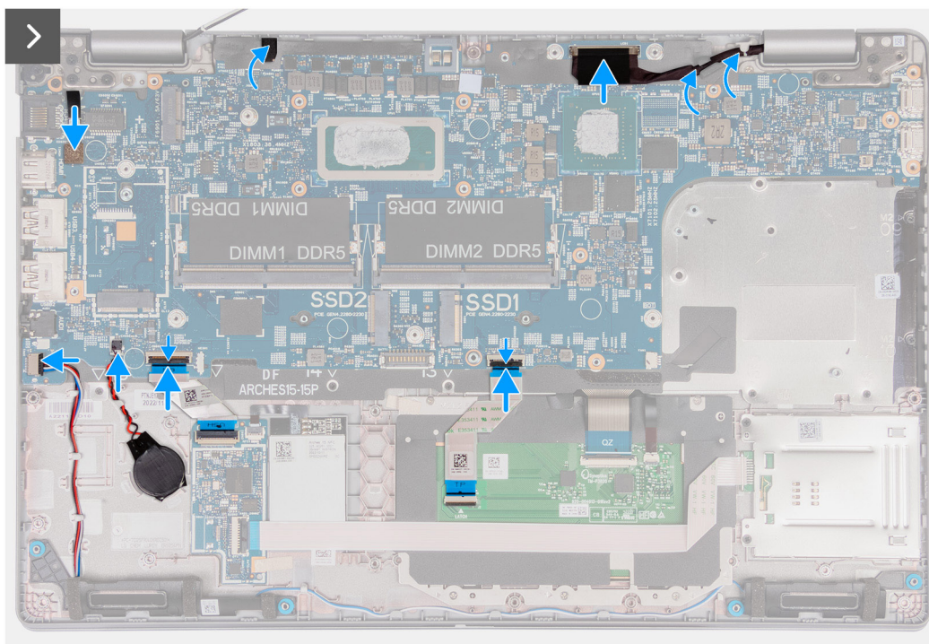
Rysunek 63. Instalowanie płyty głównej
