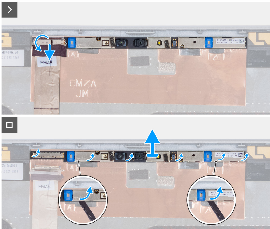
Rysunek 88. Wymontowywanie modułu kamery
