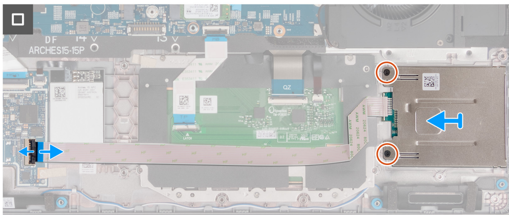
Rysunek 98. Wymontowywanie czytnika kart smart
