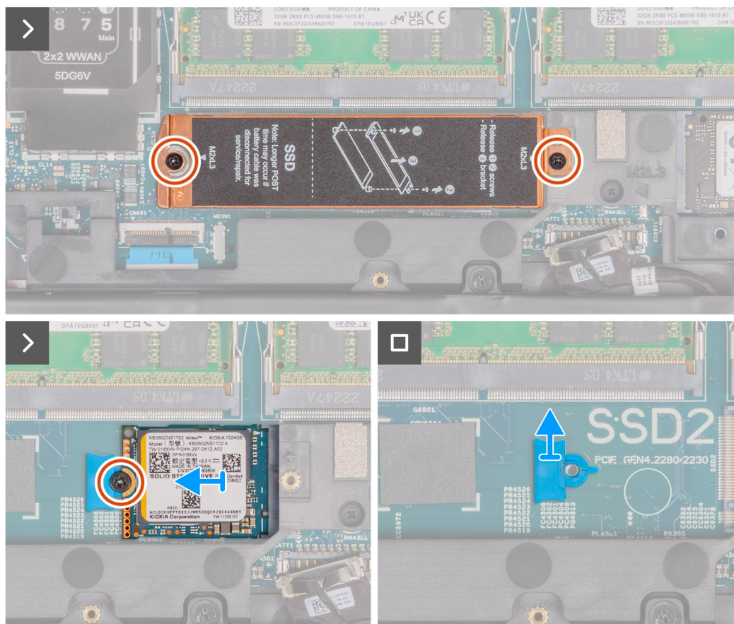
Rysunek 31. Wymontowywanie dysku SSD M.2 2230 z gniazda 2
