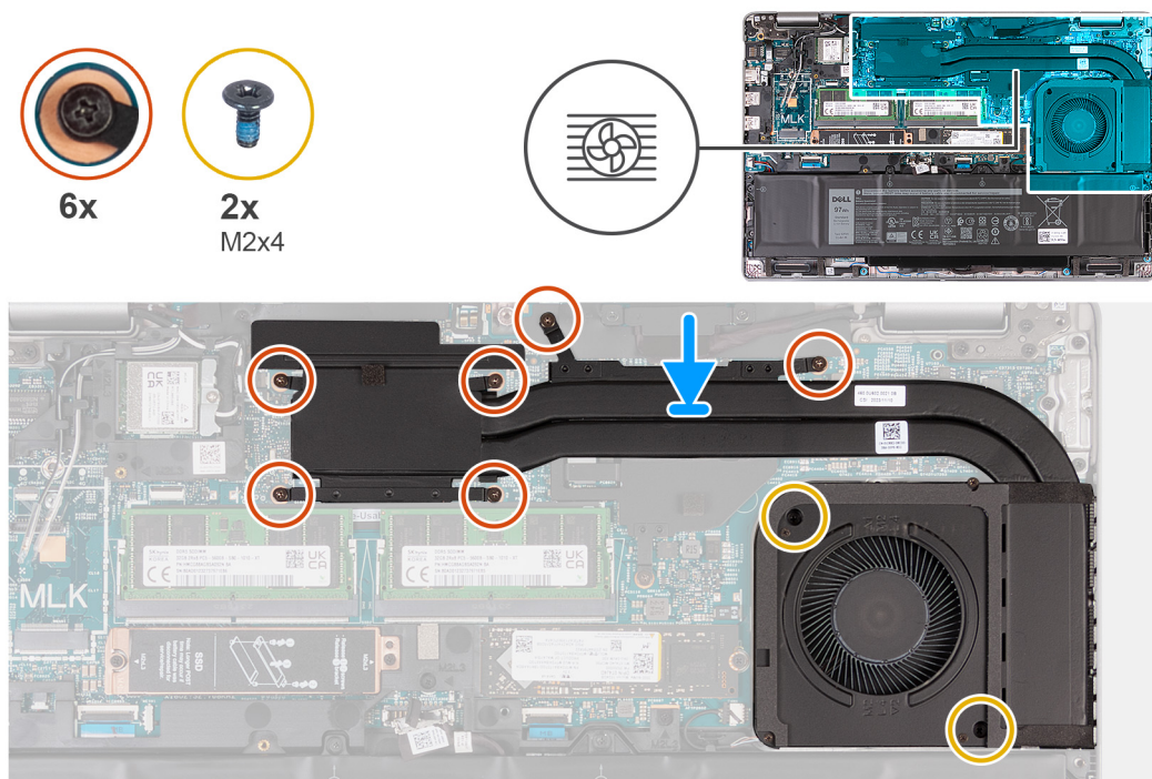
Rysunek 53. Instalowanie radiatora (konfiguracja z autonomiczną kartą graficzną)
