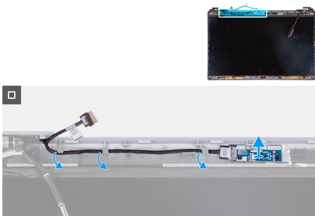
Rysunek 96. Wymontowywanie płyty czujników
