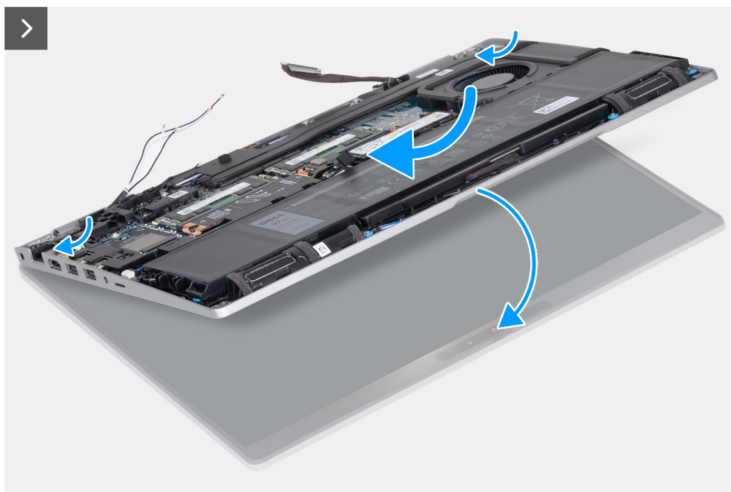
Rysunek 76. Instalowanie zestawu wyświetlacza
