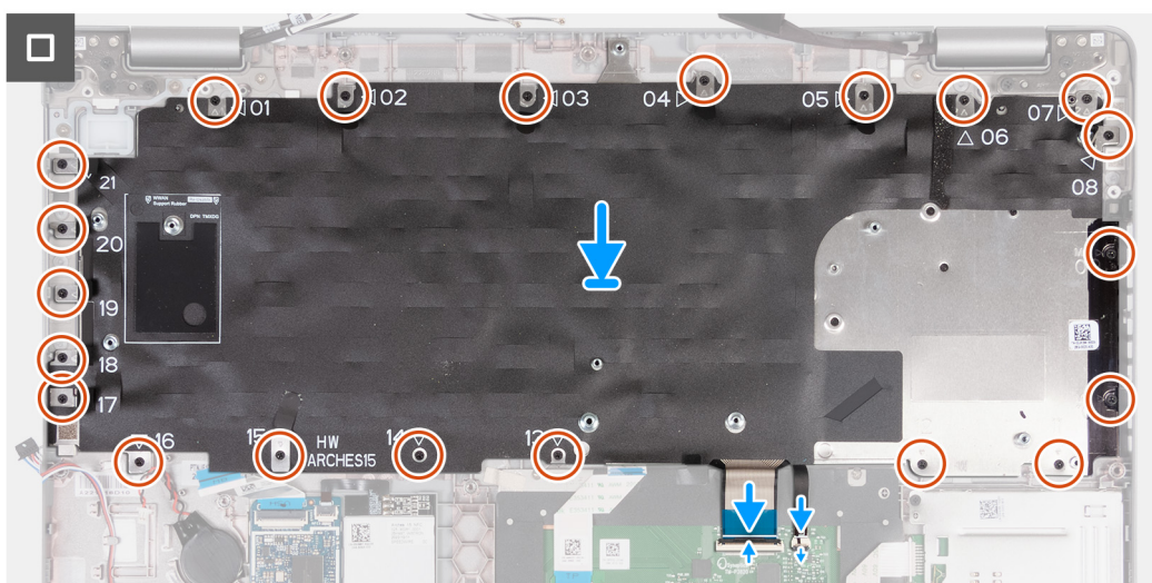
Rysunek 72. Instalowanie klawiatury
