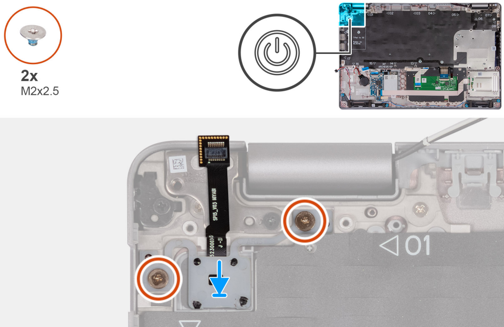
Rysunek 66. Instalowanie przycisku zasilania
