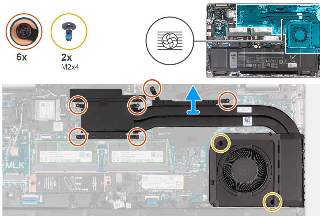
Rysunek 52. Wymontowywanie radiatora (konfiguracja z autonomiczną kartą graficzną)
