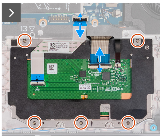
Rysunek 45. Wymontowywanie touchpada
