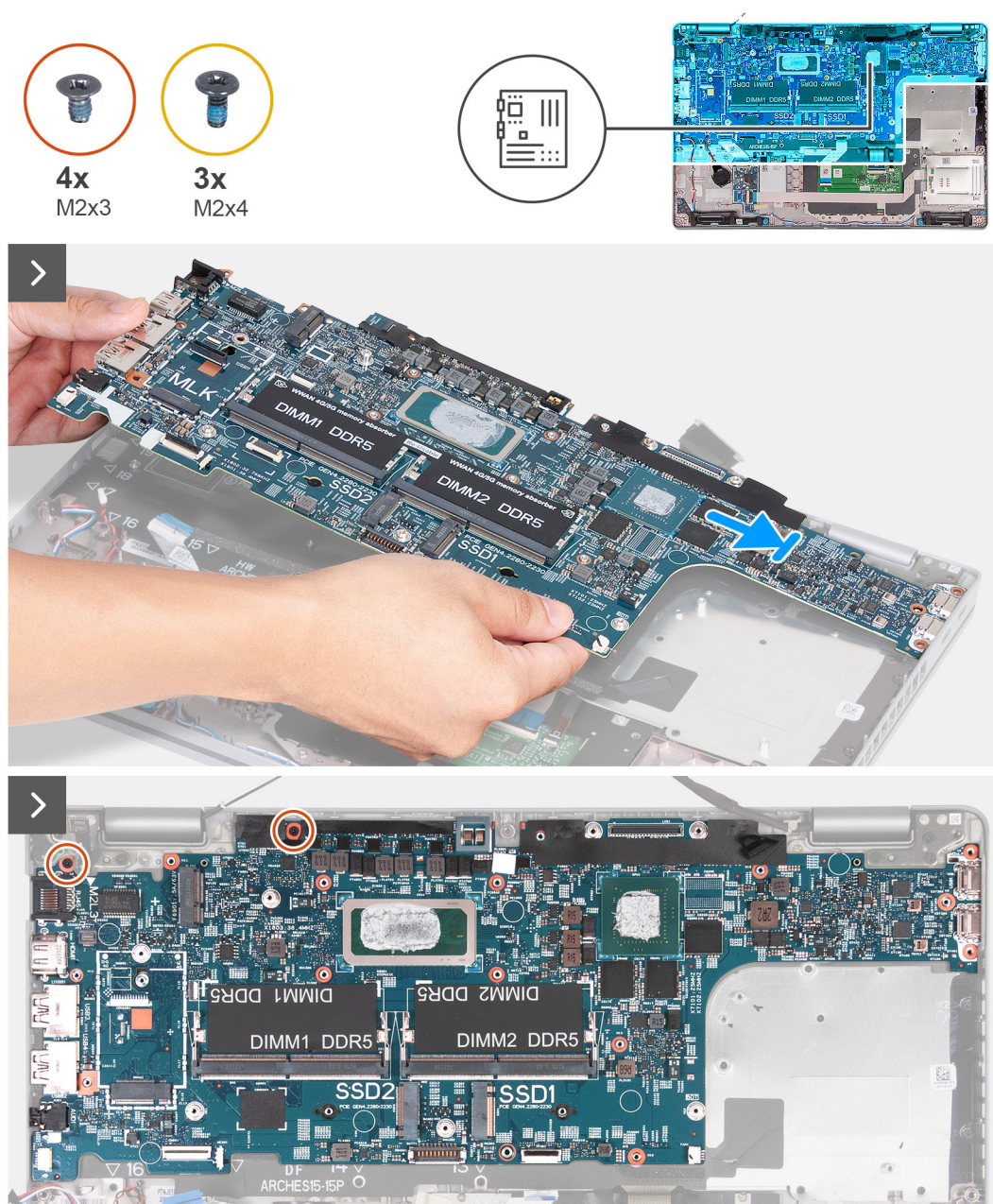
Rysunek 62. Instalowanie płyty głównej
