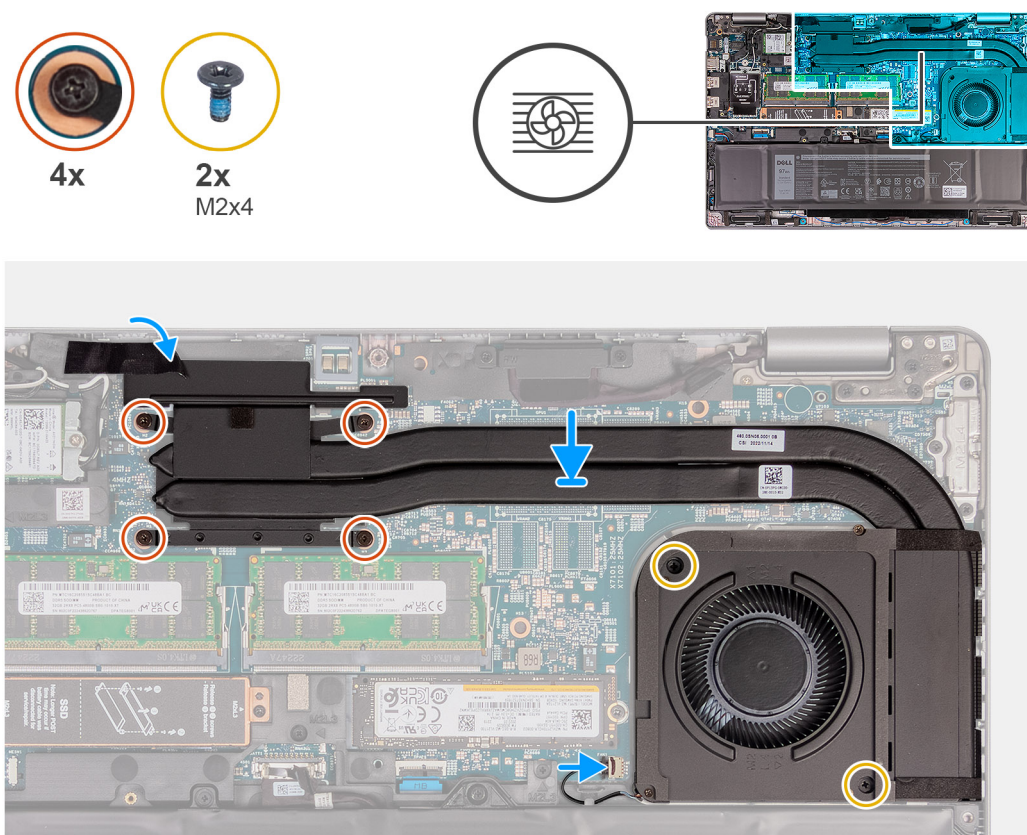
Rysunek 55. Instalowanie zestawu wentylatora i radiatora (zintegrowana karta graficzna)
