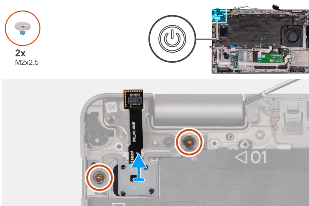
Rysunek 67. Wymontowywanie przycisku zasilania z opcjonalnym czytnikiem linii papilarnych
