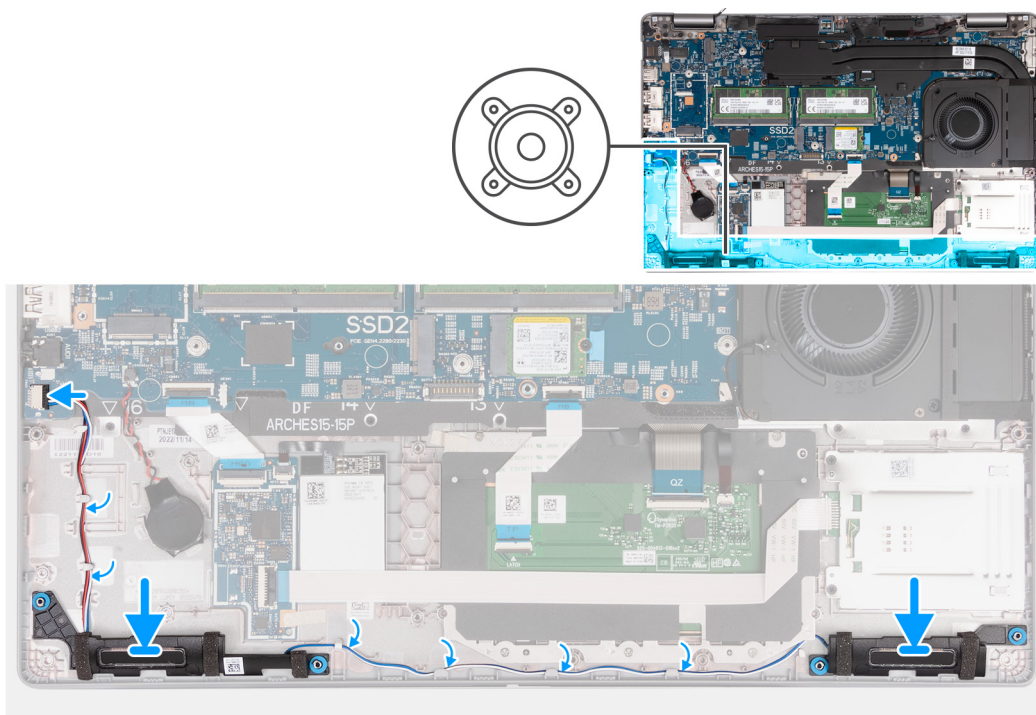
Rysunek 48. Instalowanie głośników
