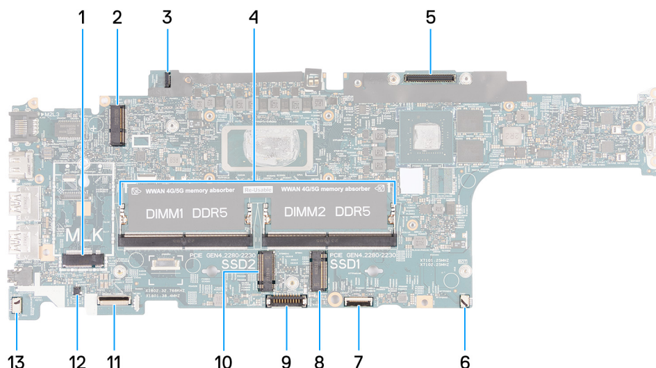
Rysunek 61. Złącza na płycie głównej
