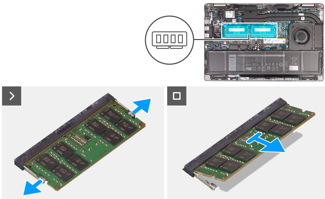
Rysunek 25. Wymontowywanie modułu pamięci
