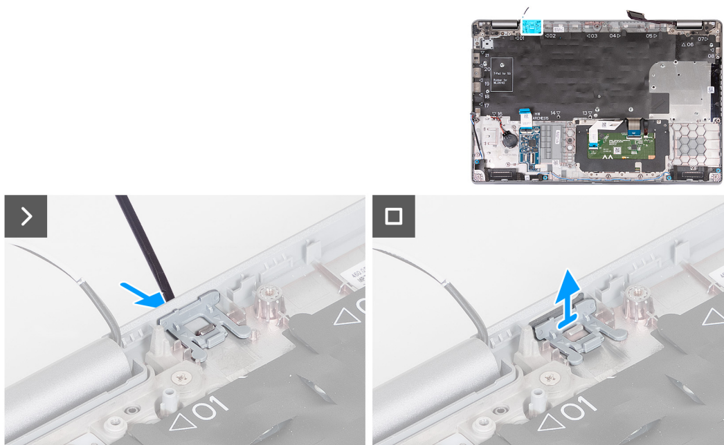
Rysunek 100. Wymontowywanie zaślepki gniazda karty SIM
