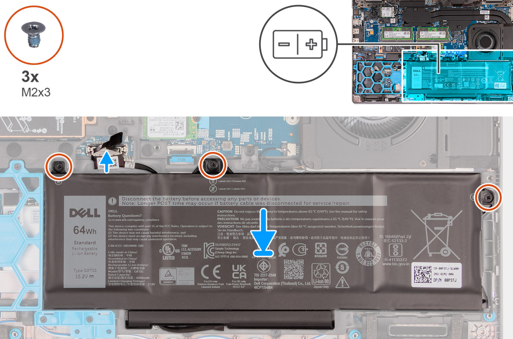
Rysunek 39. Instalowanie baterii 64 Wh
