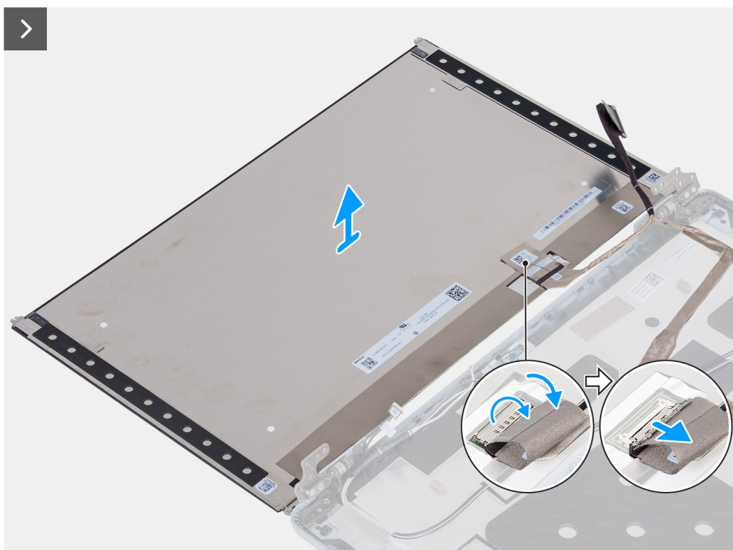
Rysunek 82. Wymontowywanie wyświetlacza
