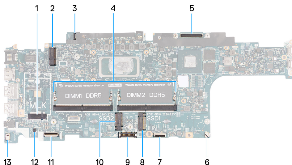
Rysunek 56. Złącza na płycie głównej
