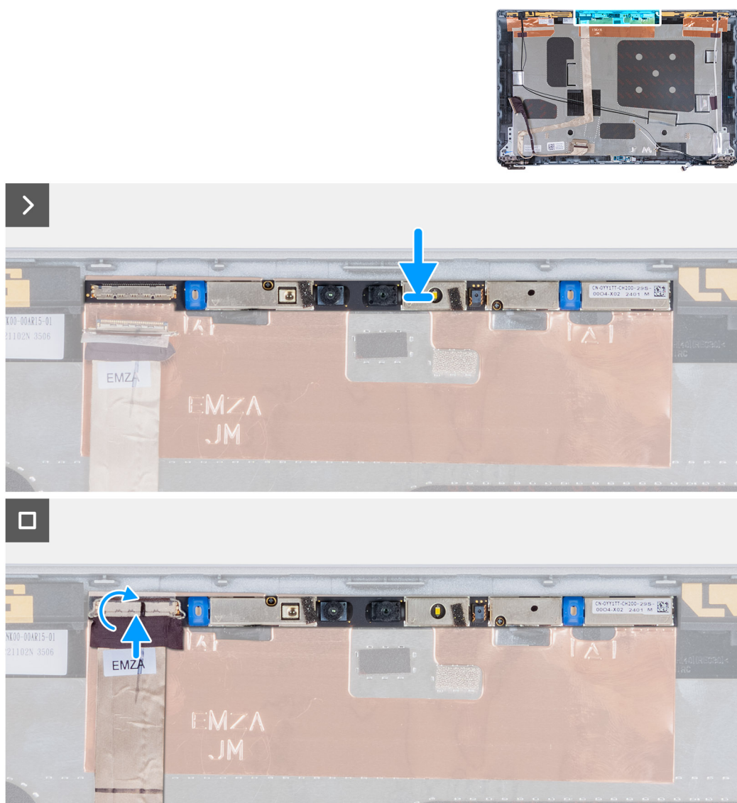
Rysunek 89. Instalowanie modułu kamery
