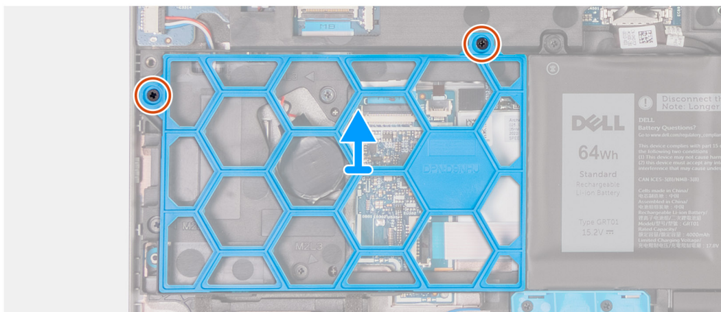
Rysunek 35. Wymontowywanie plastikowej zaślepki
