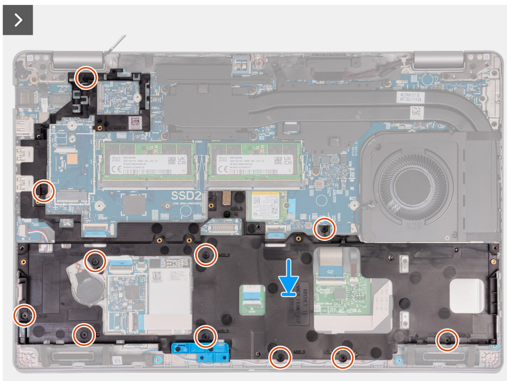
Rysunek 43. Instalowanie wewnętrznej ramy montażowej
