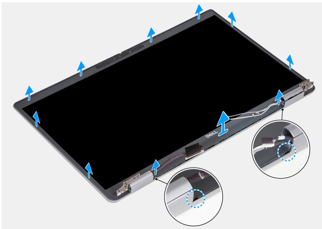
Rysunek 78. Wymontowywanie ramki wyświetlacza
