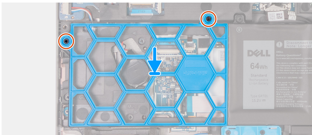
Rysunek 36. Instalowanie plastikowej zaślepki
