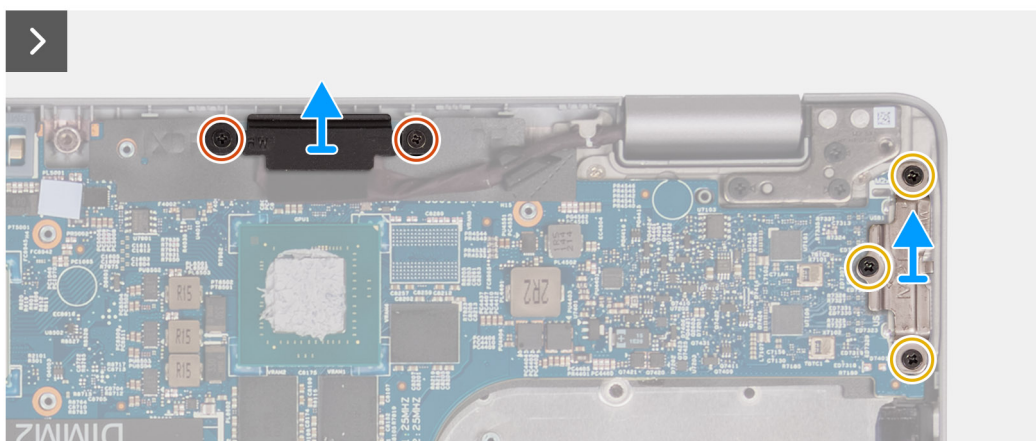
Rysunek 57. Wymontowywanie płyty głównej
