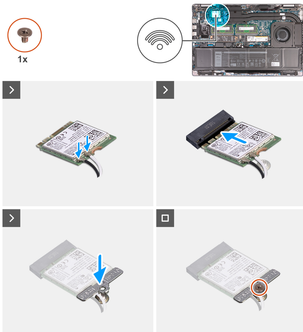
Rysunek 20. Instalowanie karty sieci bezprzewodowej
