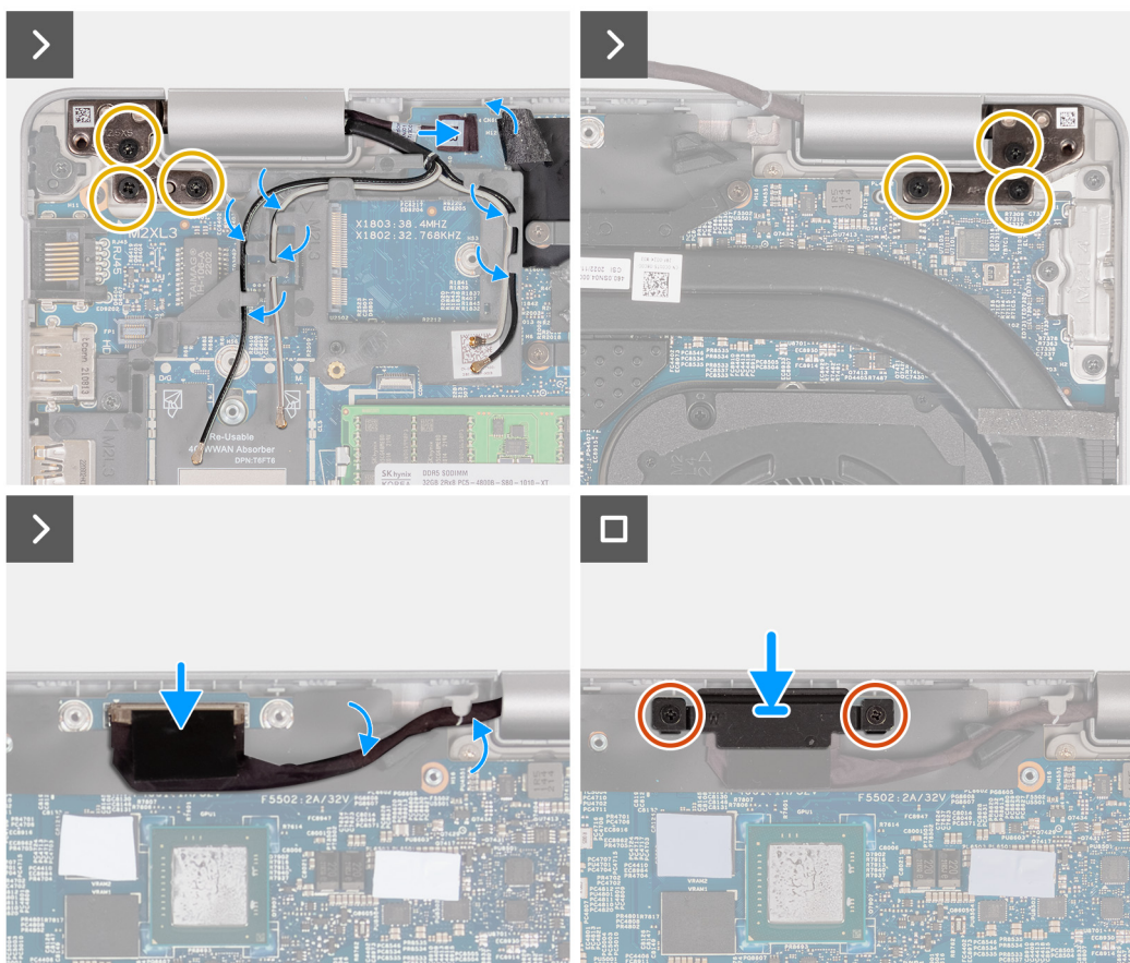
Rysunek 77. Instalowanie zestawu wyświetlacza
