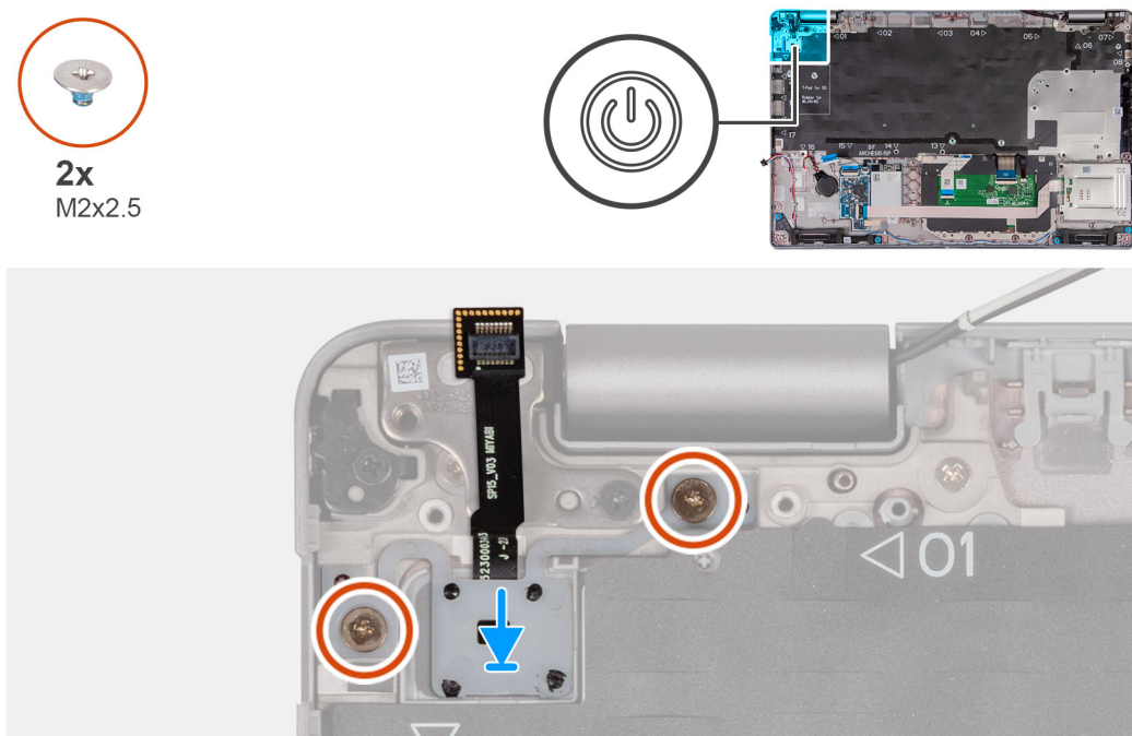
Rysunek 68. Instalowanie przycisku zasilania z opcjonalnym czytnikiem linii papilarnych
