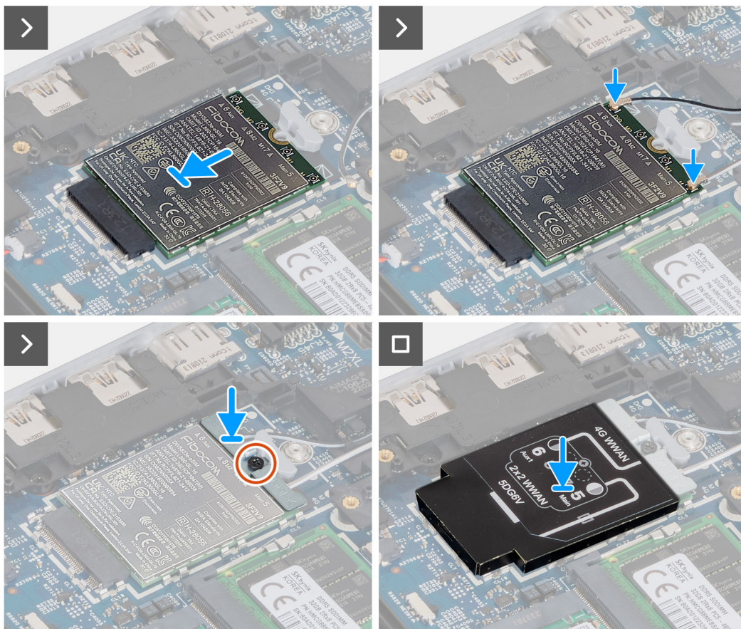
Rysunek 22. Instalowanie karty sieci WWAN 4G
