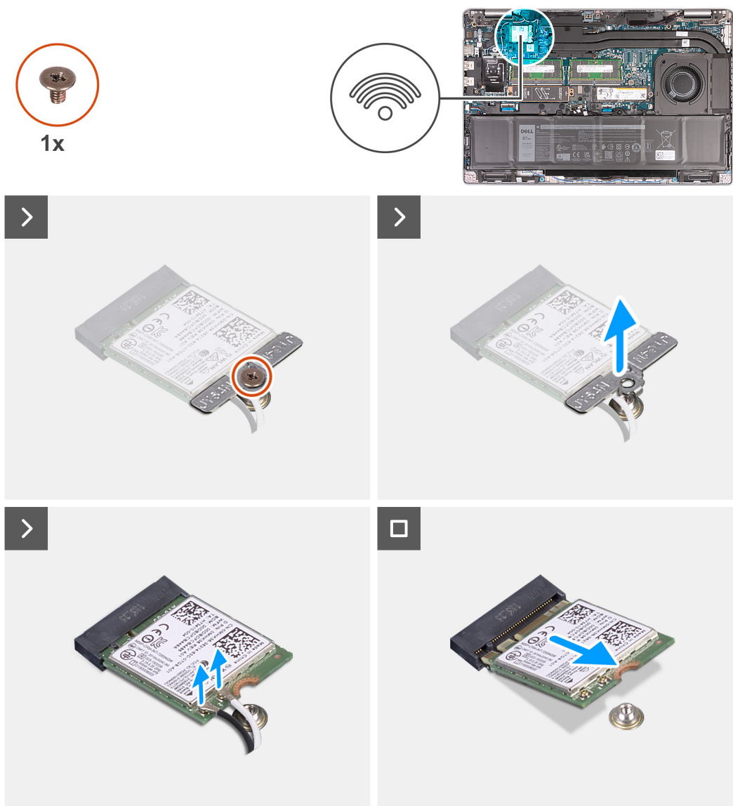
Rysunek 19. Wymontowywanie karty sieci bezprzewodowej
