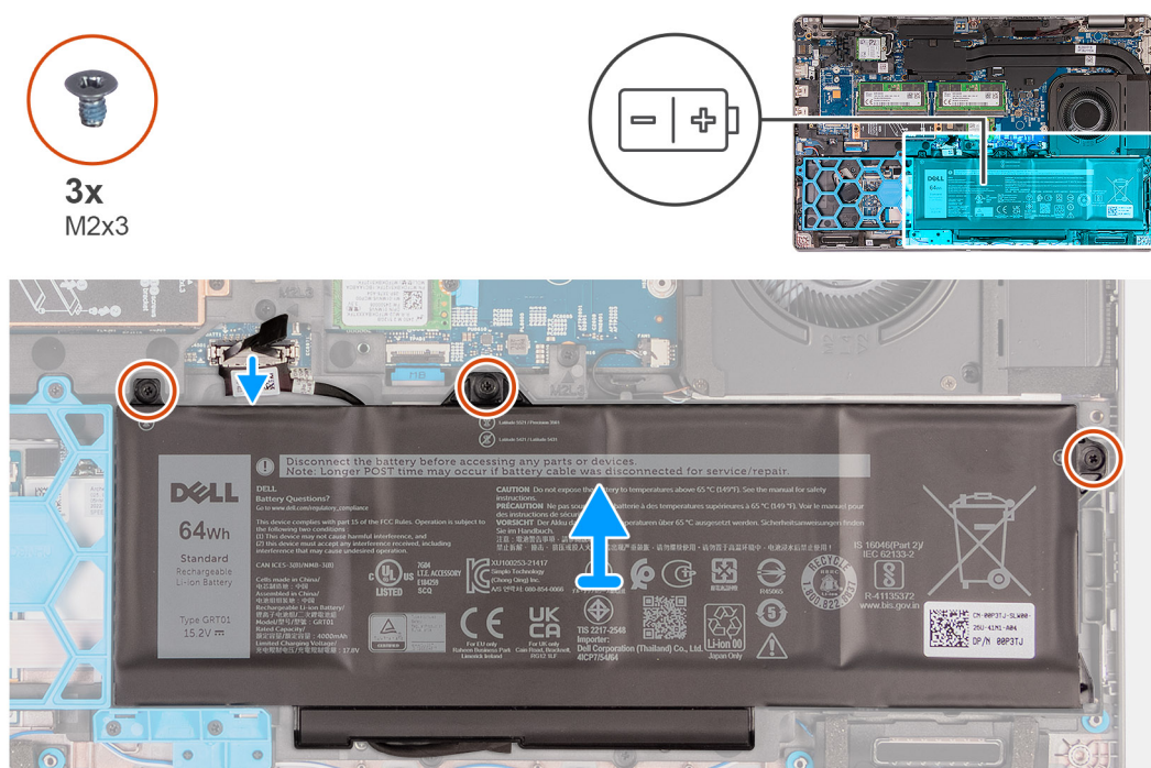
Rysunek 37. Wymontowywanie baterii 64 Wh
