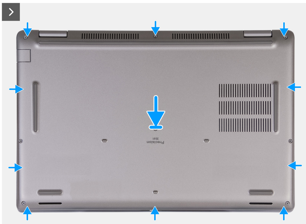
Rysunek 17. Instalowanie pokryw dolnej
