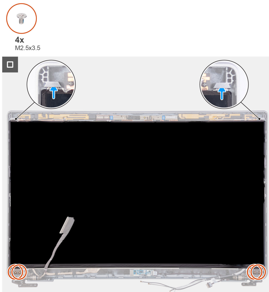
Rysunek 87. Instalowanie wyświetlacza
