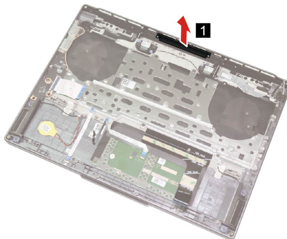
Figure 40. Remove the thermal fin
