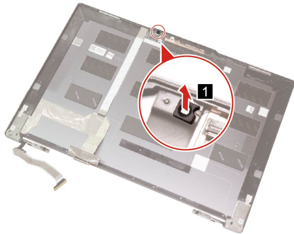
Figure 50. Remove the ALS rubber
