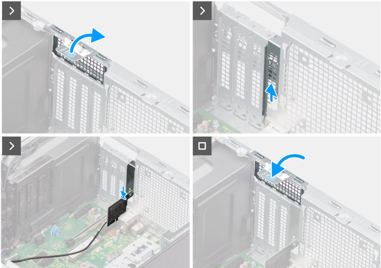
איור 37. התקנת אנטנת ה-PCIe החיצונית
