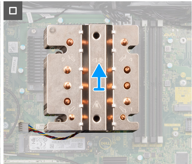
איור 52. הסרת מכלול מאוורר המעבד וגוף הקירור של 125W
