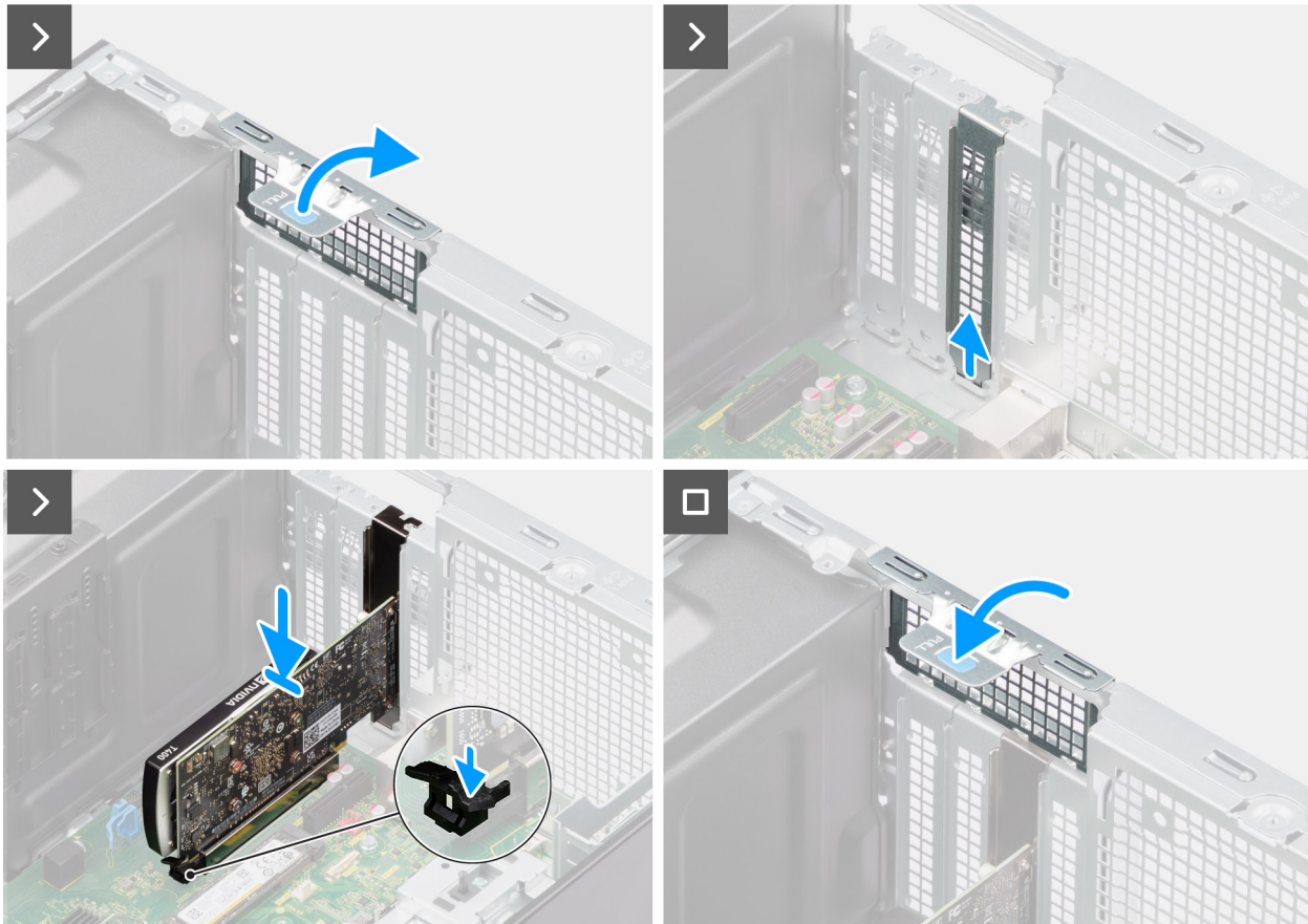
איור 39. התקנת הכרטיס הגרפי
