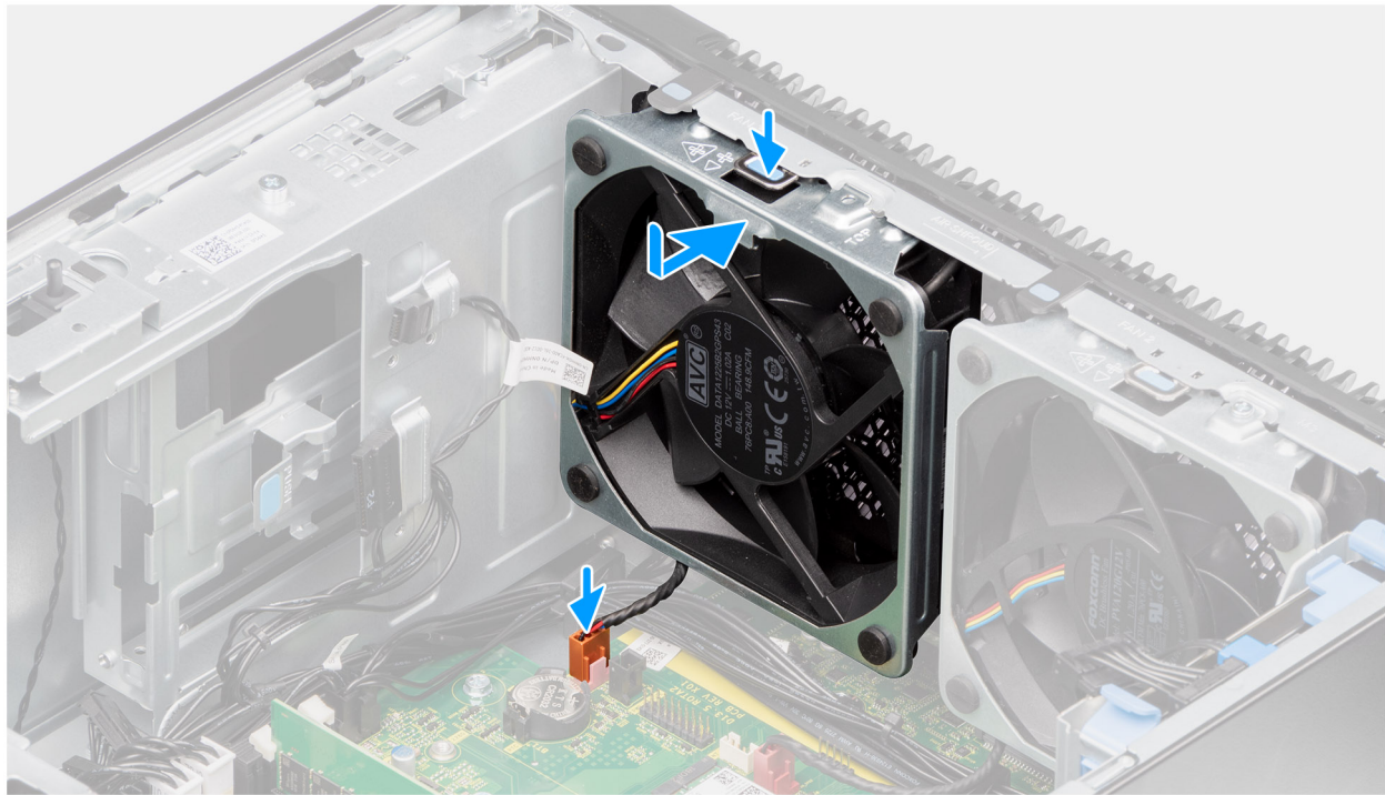
איור 63. מאוורר קדמי 2
