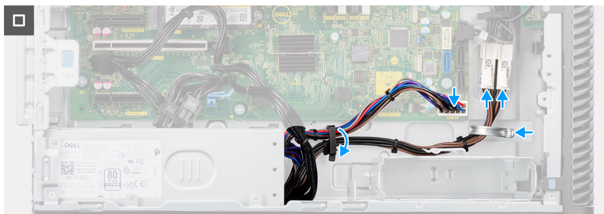
איור 50. התקנת יחידת ספק הכוח של 1000W
