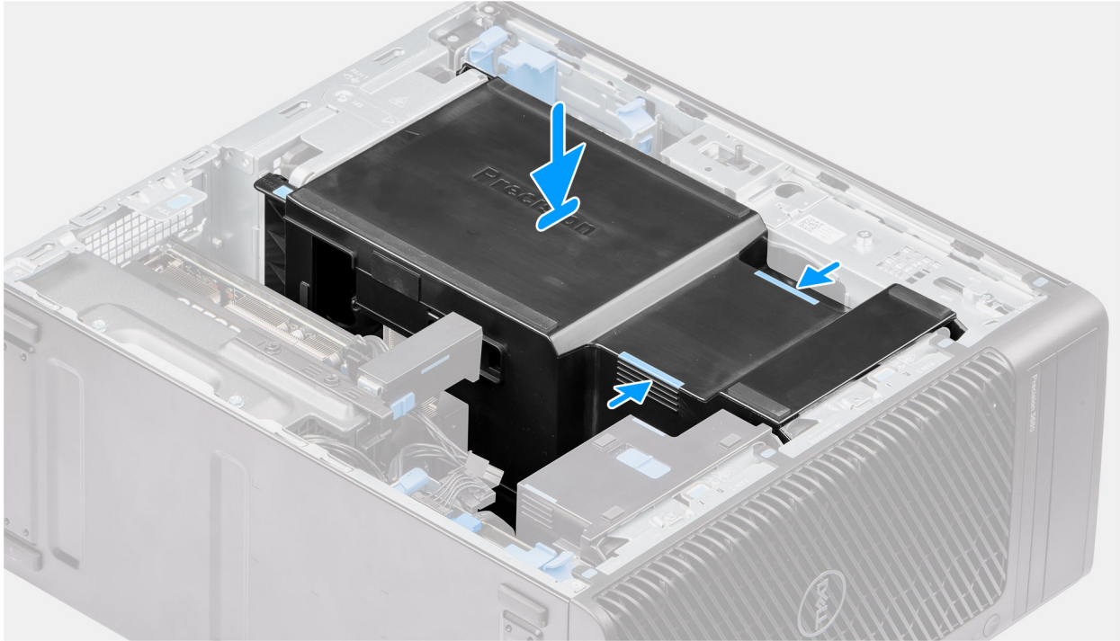
איור 15. התקנת חיפוי האוויר
