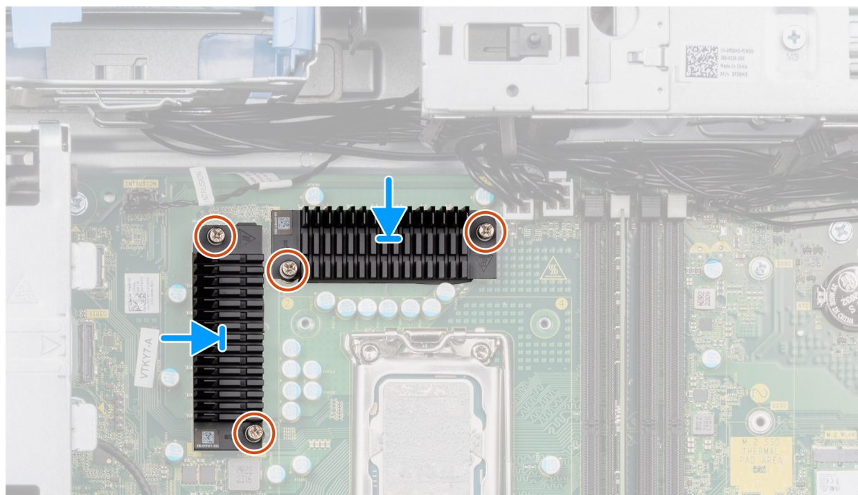
איור 59. התקנת גוף הקירור של ה-VR
