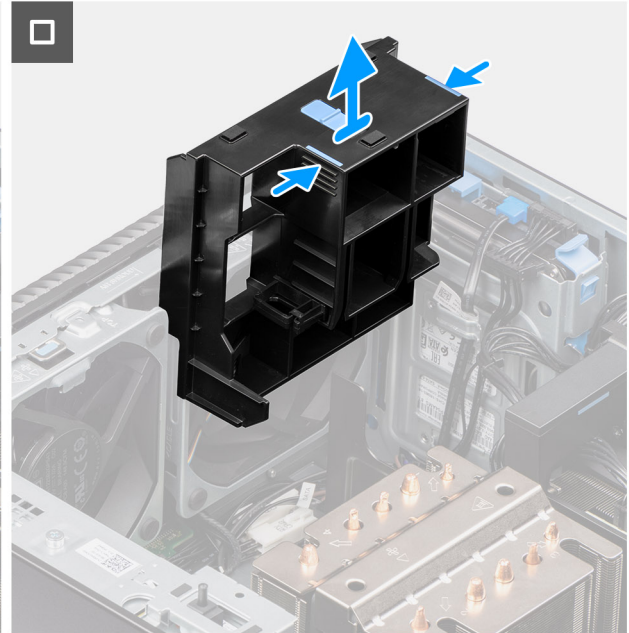
איור 34. הסרת מחזיק הקצה של ה-GPU
