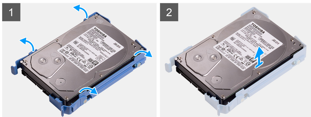
איור 18. הסרת תושבת כונן הדיסק הקשיח בגודל 3.5 אינץ'
