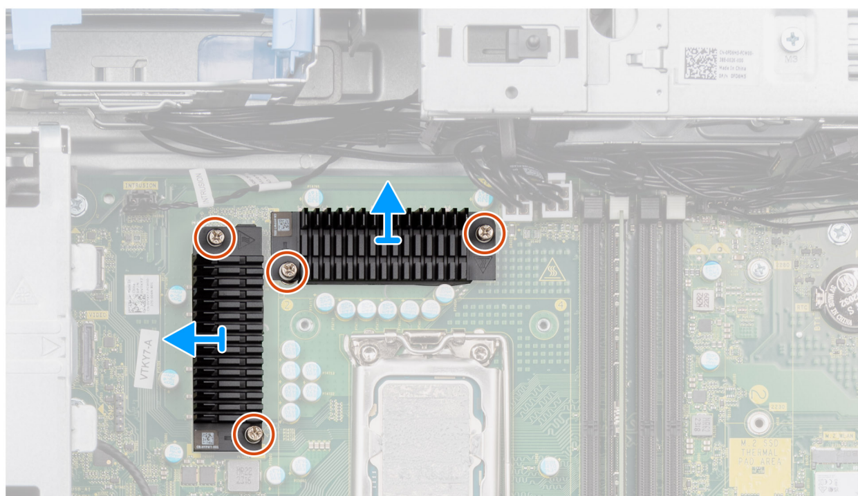
איור 58. הסרת גוף הקירור של ה-VR
