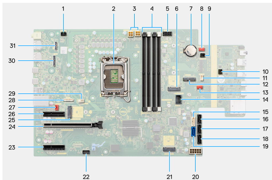
איור 79. הסברים על לוח המערכת
