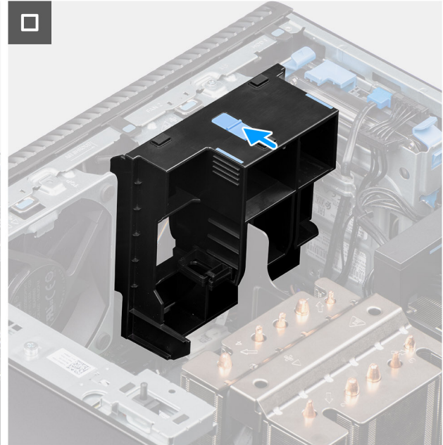
איור 35. התקנת מחזיק הקצה של ה-GPU
