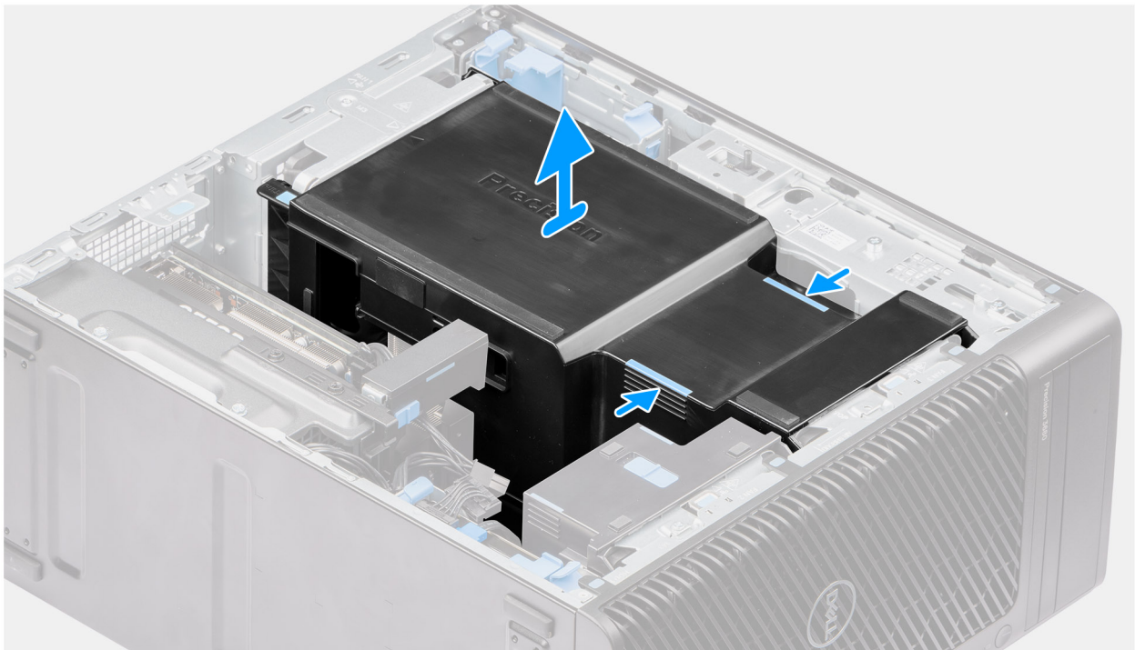
איור 14. הסרת חיפוי האוויר
