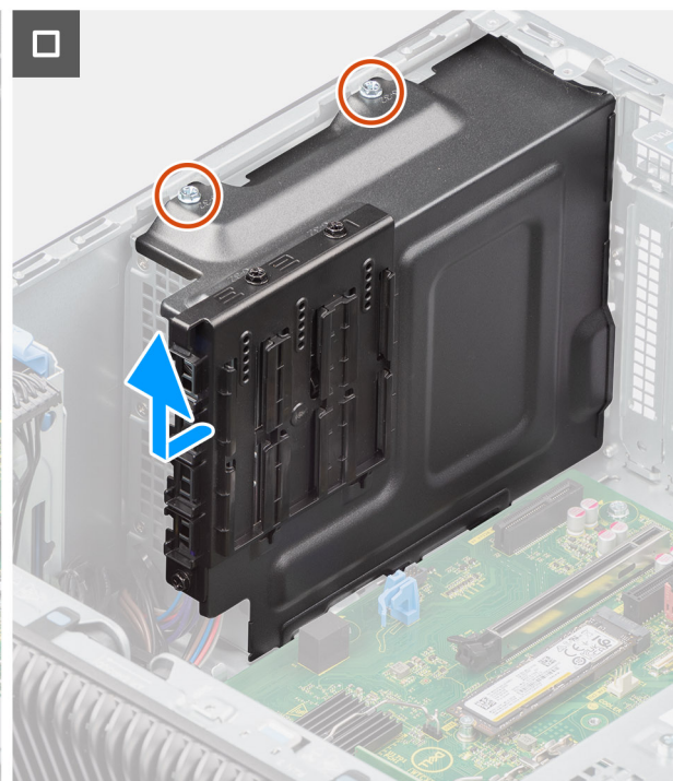
איור 46. הסרת הכיסוי של יחידת ספק הכוח
