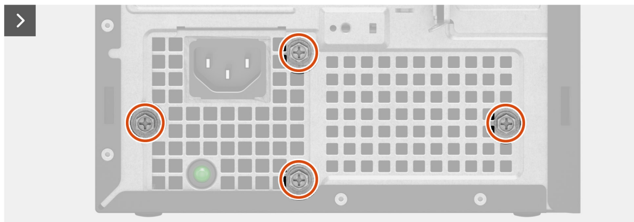
איור 48. הסרת יחידת ספק הכוח של 1000W
