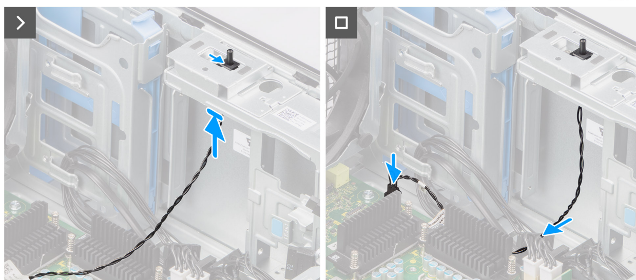
איור 71. התקנת מתג החדירה למארז
