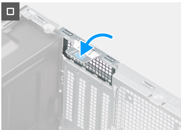
איור 36. הסרת אנטנת ה-PCIe החיצונית
