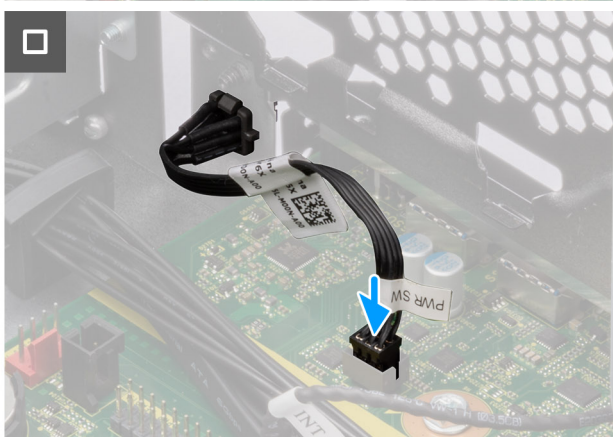
איור 69. התקנת לחצן ההפעלה
