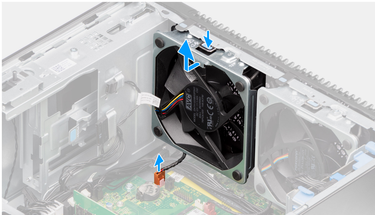
איור 61. מאוורר קדמי 2
