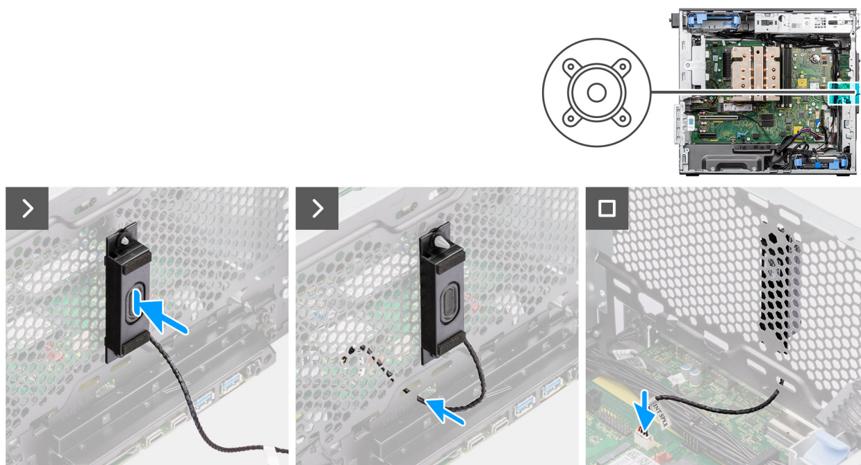
איור 73. התקנת הרמקול הפנימי
