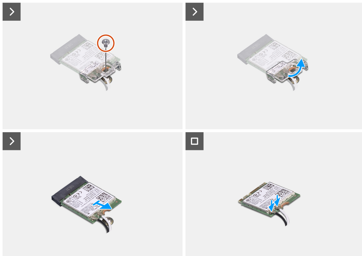
איור 26. הסרת כרטיס ה-WLAN
