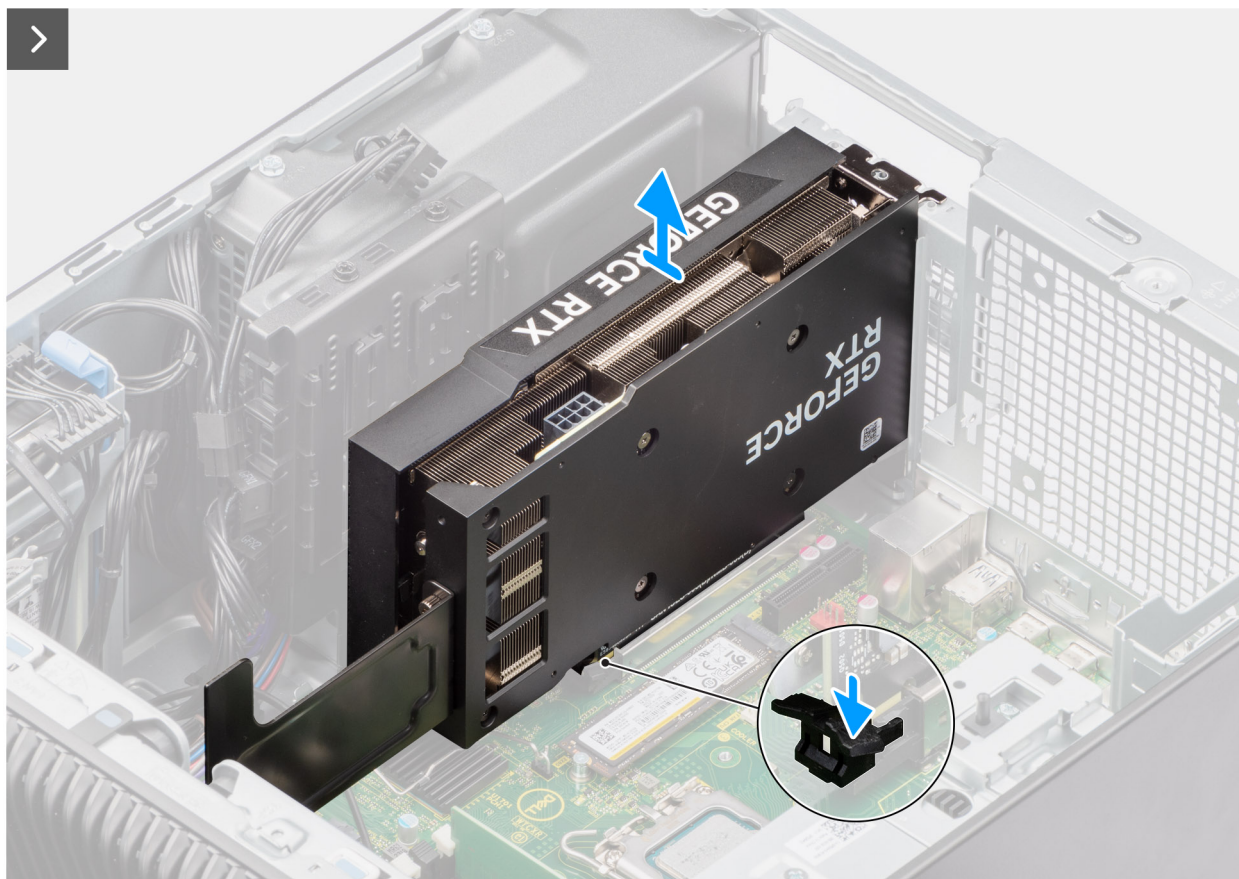
איור 41. הסרת ה-GPU המופעל
