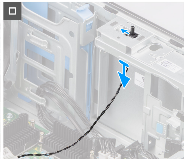
איור 70. הסרת מתג החדירה
