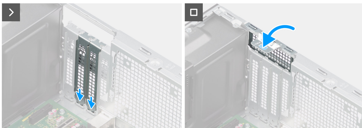
איור 42. הסרת ה-GPU המופעל
