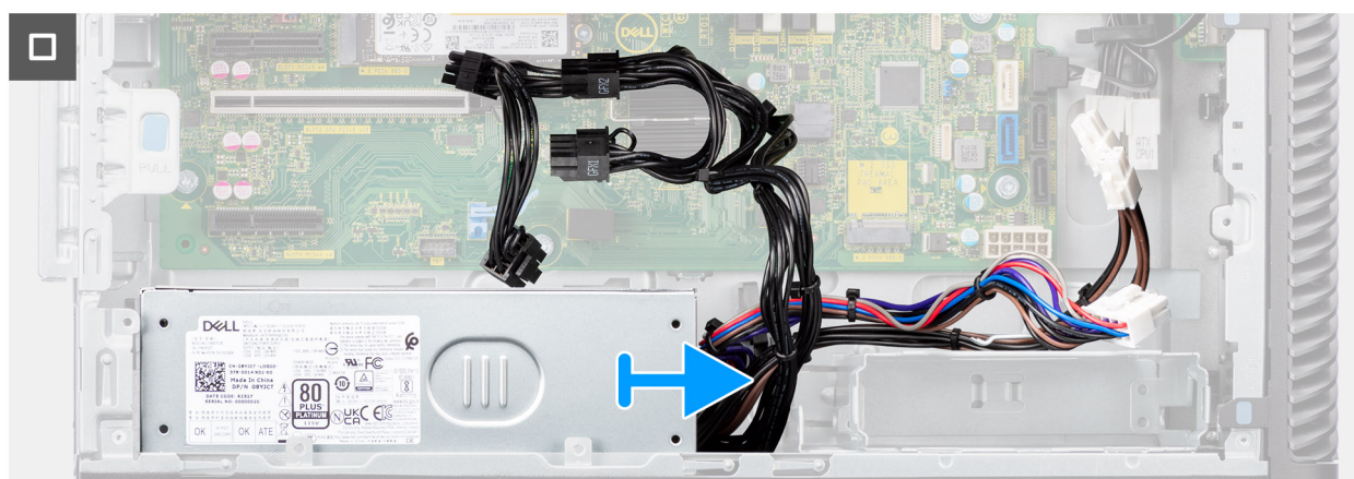
איור 49. הסרת יחידת ספק הכוח של 1000W
