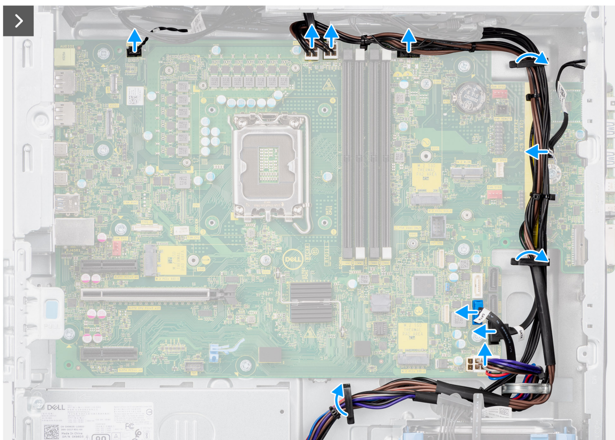
איור 76. הסרת לוח המערכת
