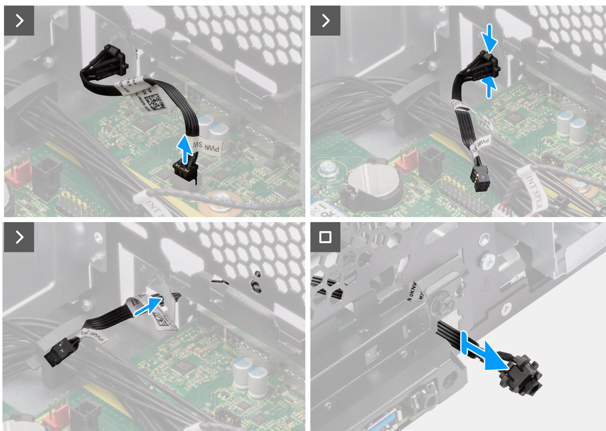
איור 68. הסרת לחצן ההפעלה
