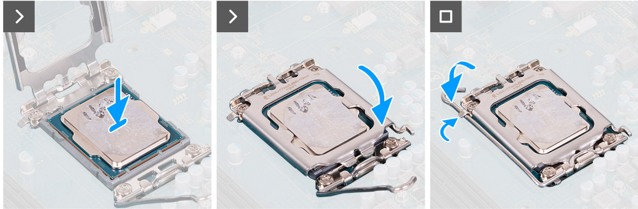
איור 57. התקנת המעבד
