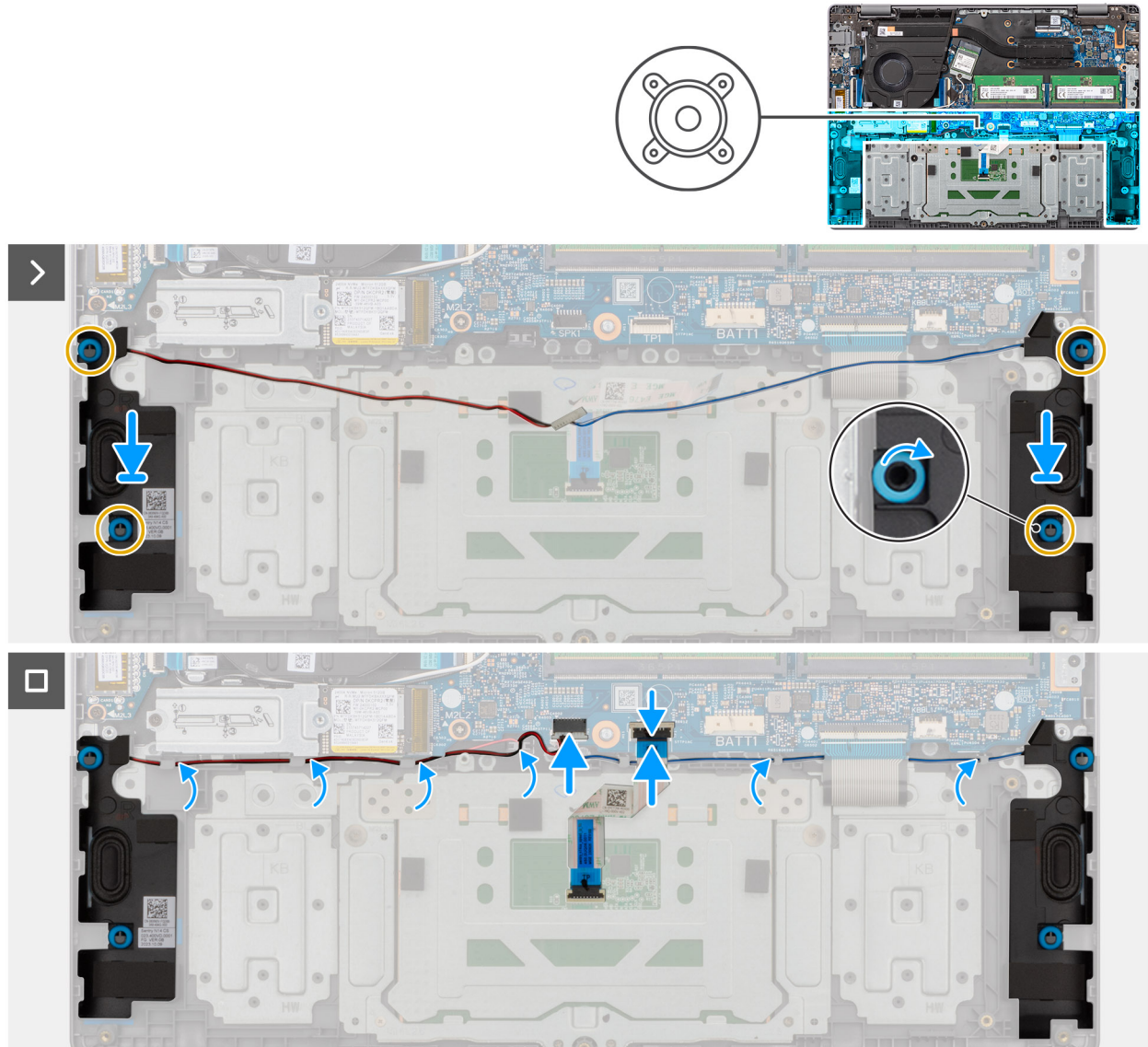
איור 29. התקנת הרמקולים
