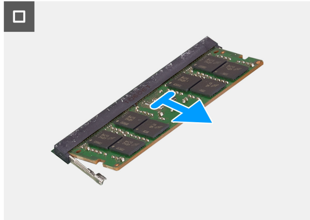
איור 14. הסרת מודול הזיכרון
