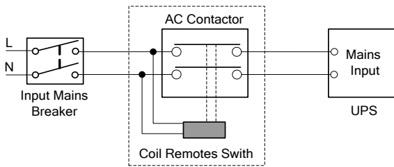
Abb. 1: Typische Installation eines externen Isoliergeräts
