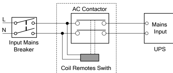
Fig. 1: Instalação típica do dispositivo isolador externo
