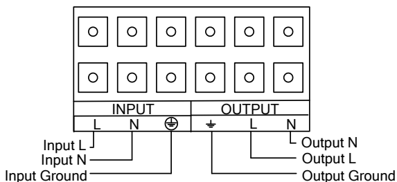
Fig. 2: Diagrama de cabeado del bloque de terminales de entrada y salida
