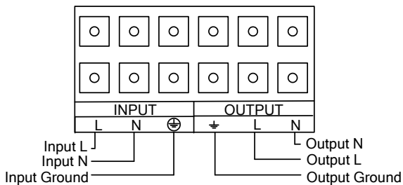
Abb. 2: Schaltplan für die Verdrahtung des Ein- und Ausgangs-Anschlussblocks
