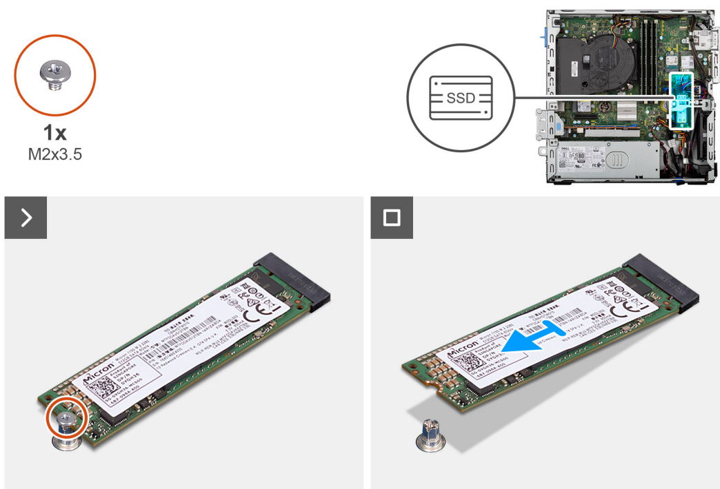
Figure 21. Retrait du disque SSD M.2 2280
