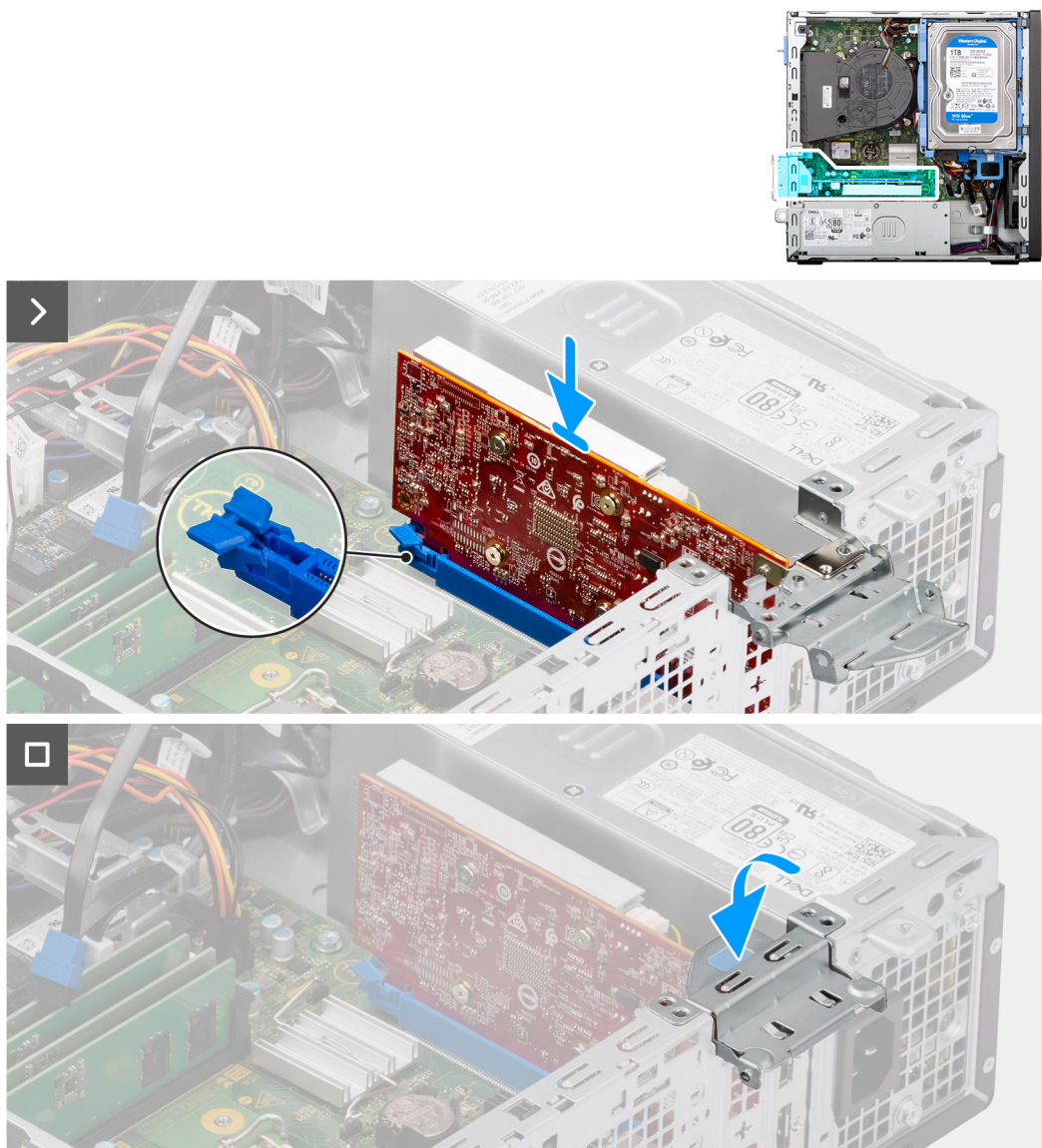
Figure 34. Installation de la carte graphique
