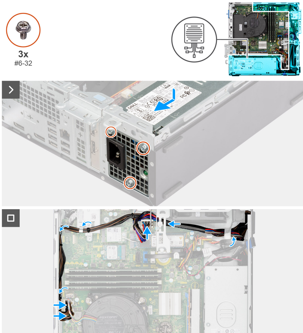
Figure 49. Installation du bloc d'alimentation
