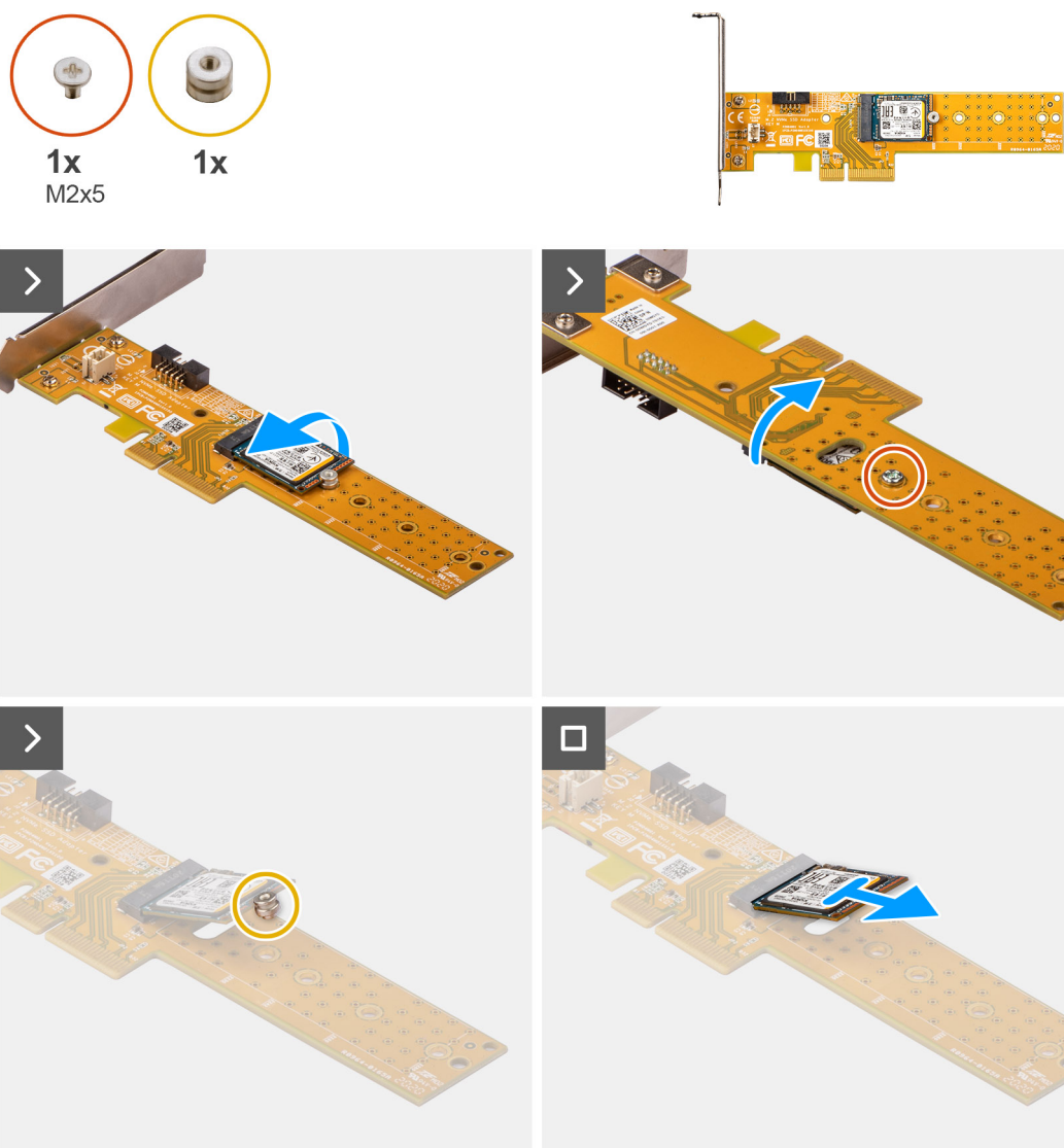
Figure 24. Retrait du disque SSD M.2 2230 de la carte Dell Ultra Speed Drive Gen 3
