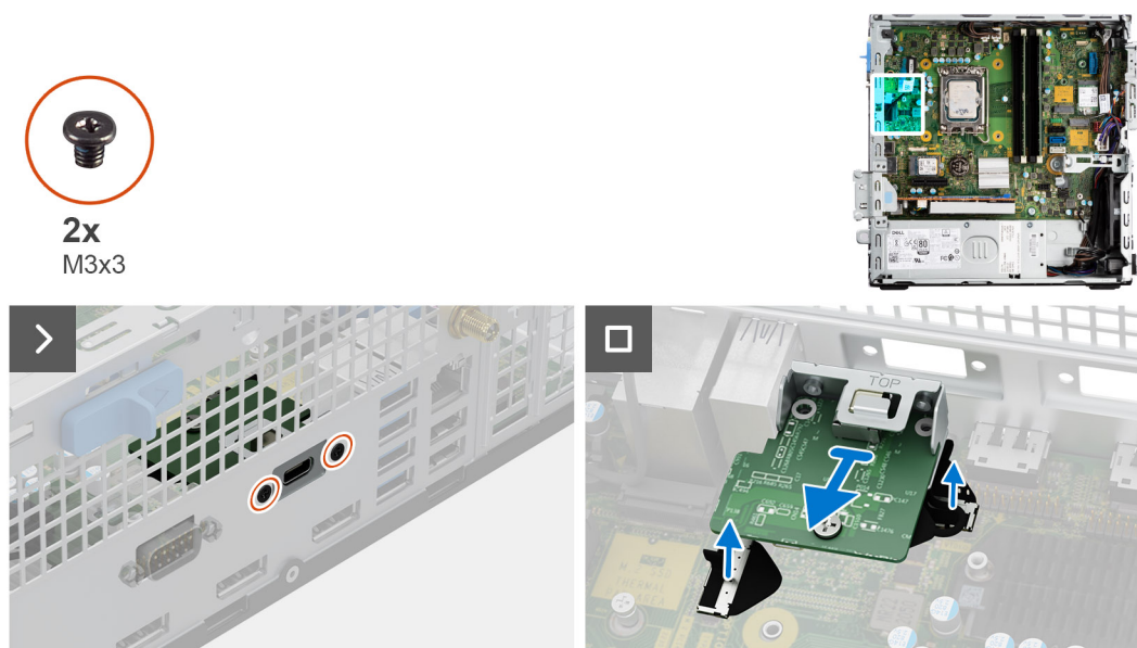
Figure 62. Retrait du module USB-C
