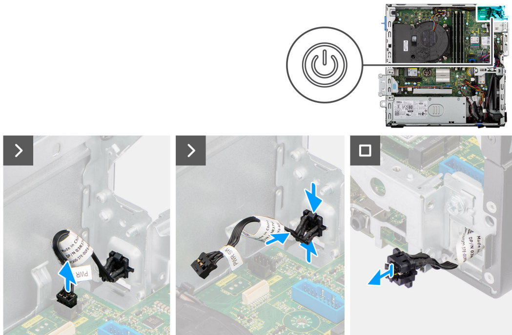
Figure 39. Retrait du bouton d'alimentation
