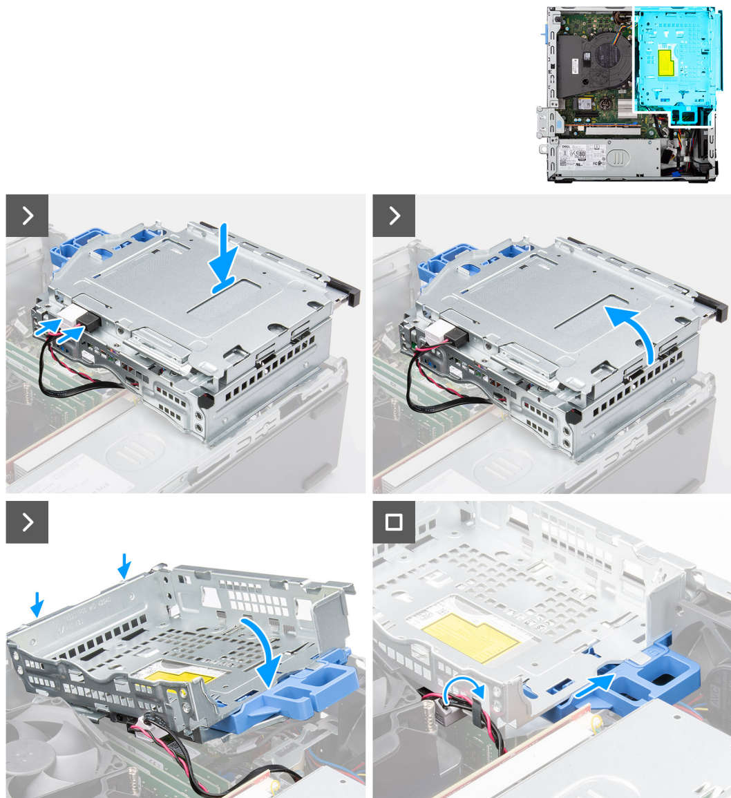
Figure 12. Installation du bâti du lecteur de disque
