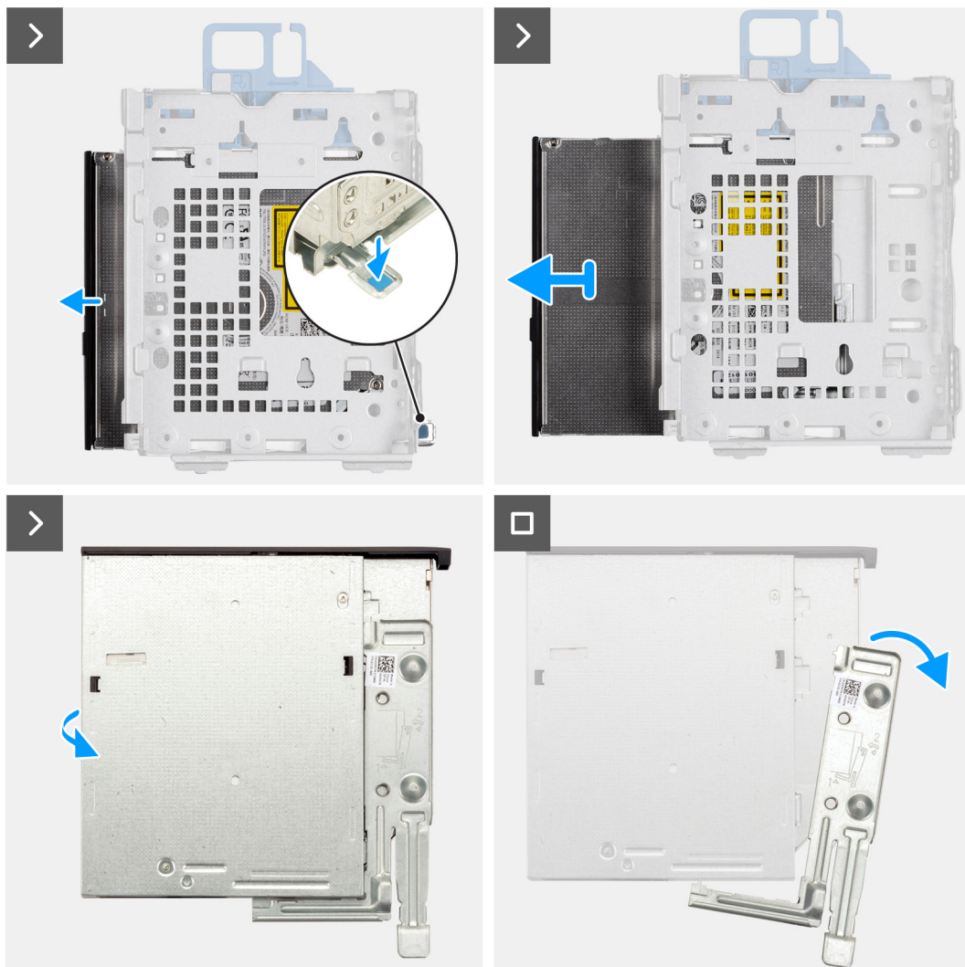
Figure 13. Retrait du lecteur optique
