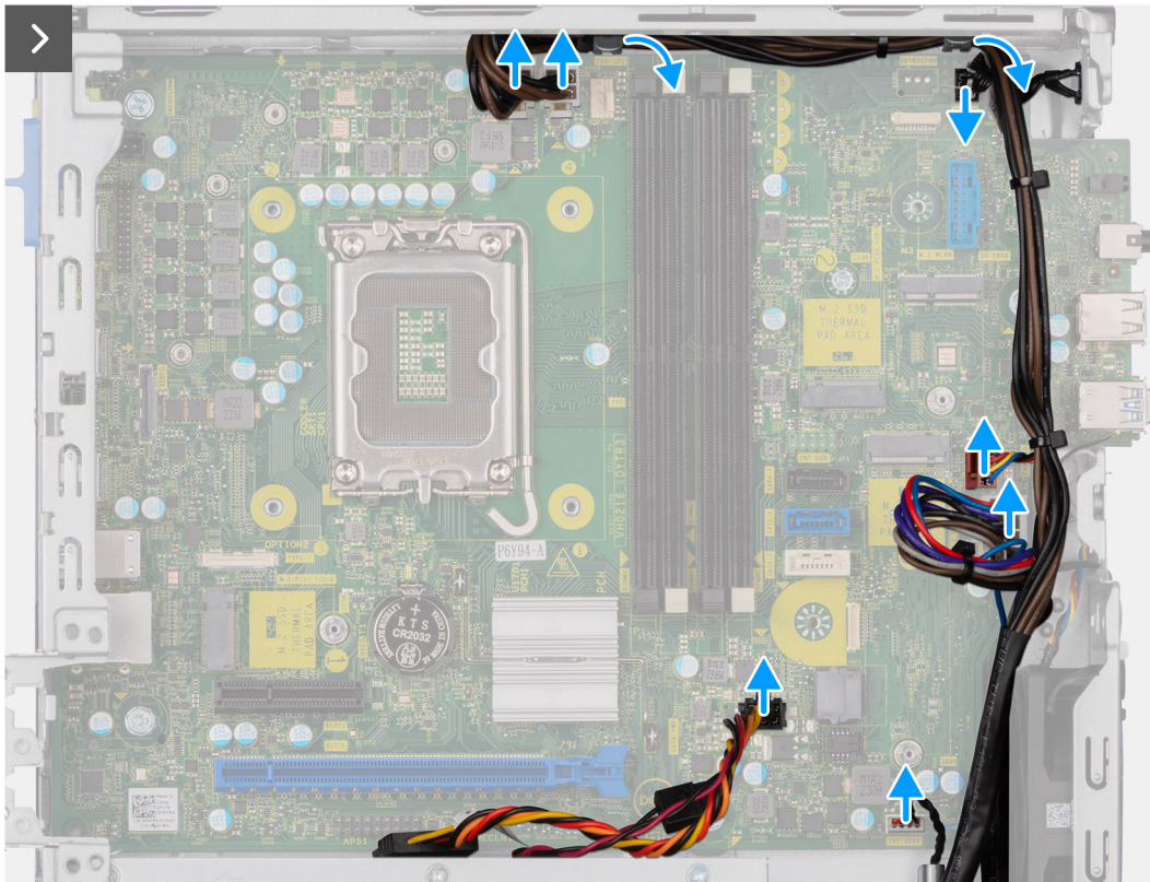
Figure 66. Retrait de la carte système
