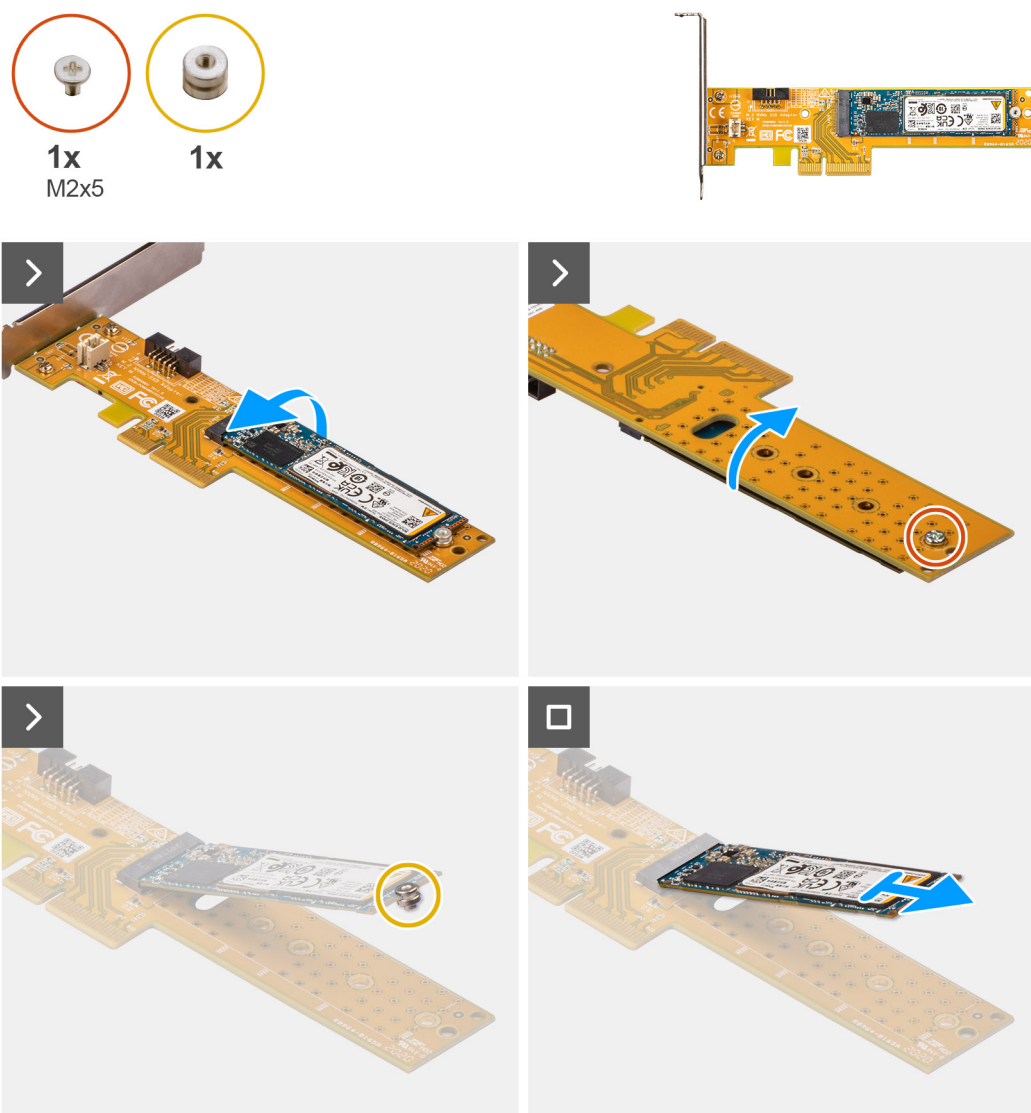
Figure 25. Retrait du disque SSD M.2 2280 de la carte Dell Ultra Speed Drive Gen 3
