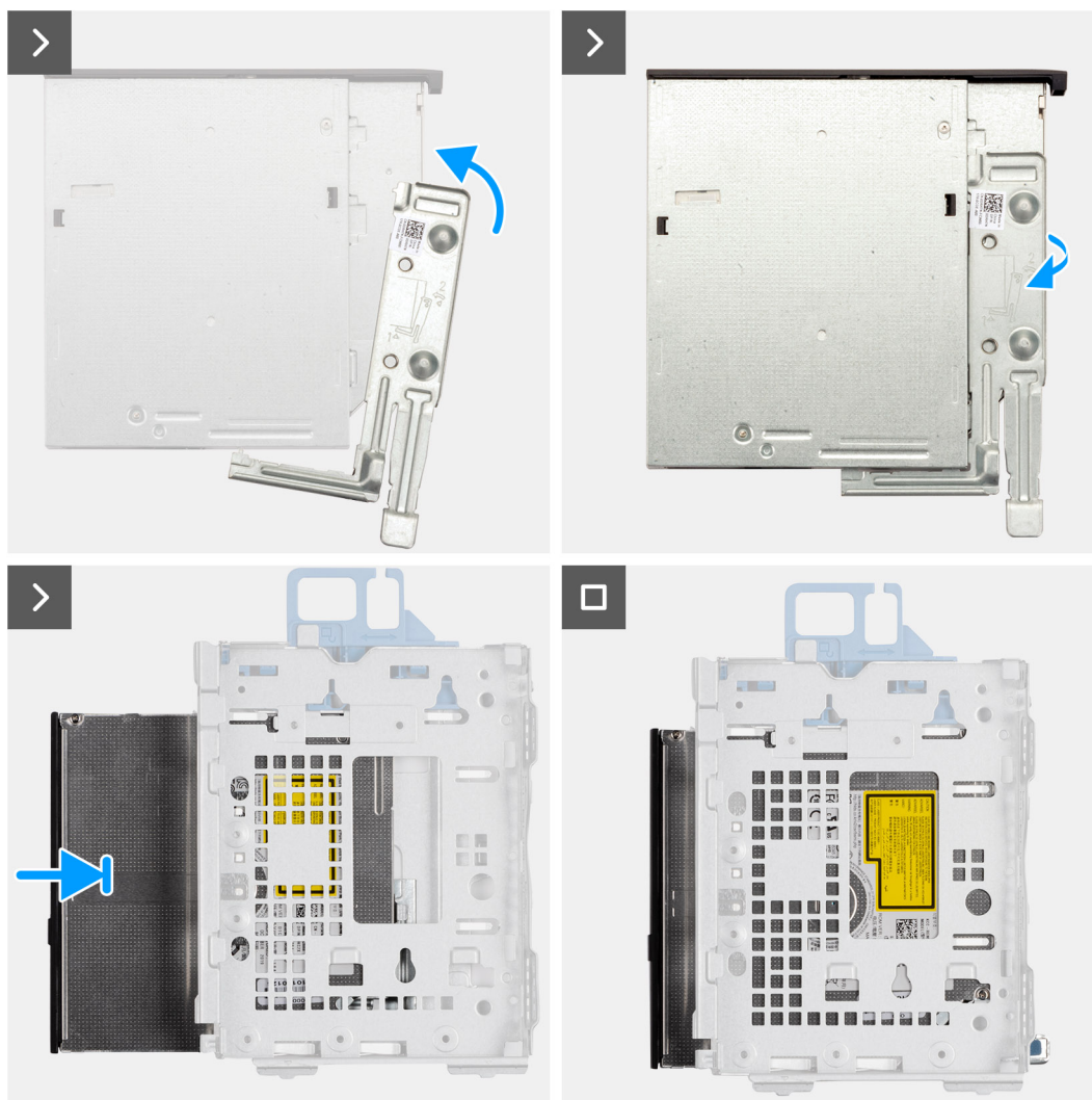
Figure 14. Installation du lecteur optique
