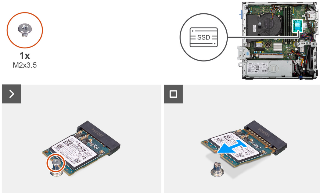
Figure 19. Retrait du disque SSD M.2 2230
