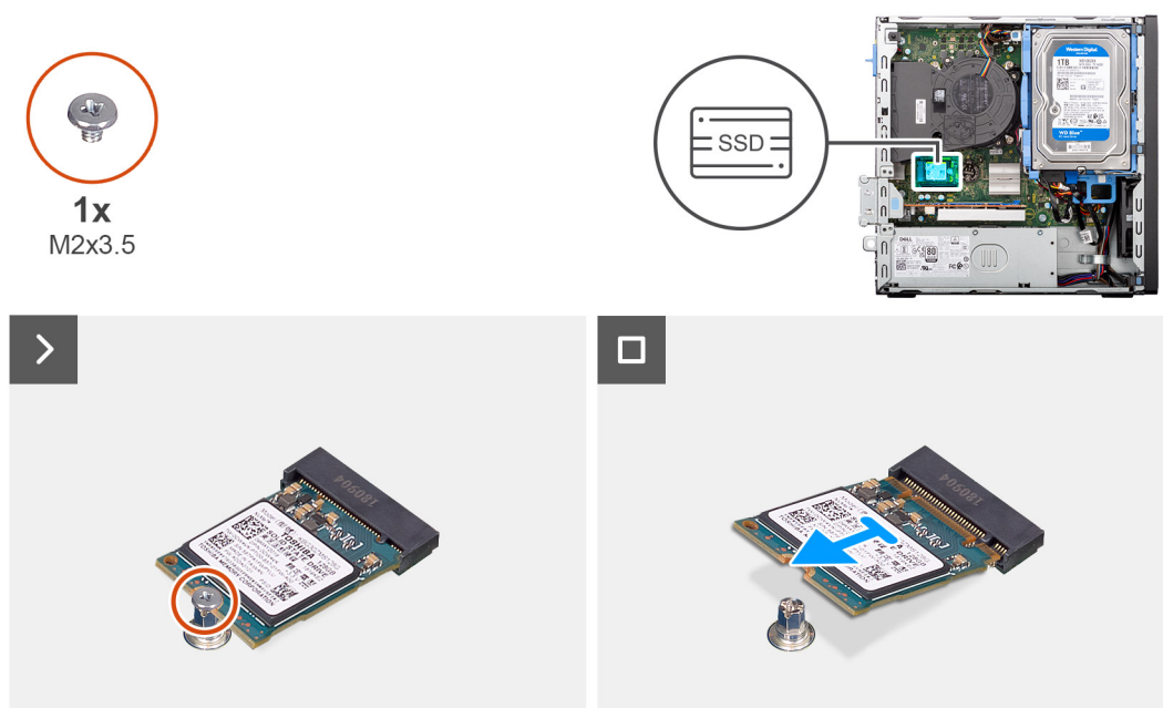
Figure 17. Retrait du disque SSD M.2 2230
