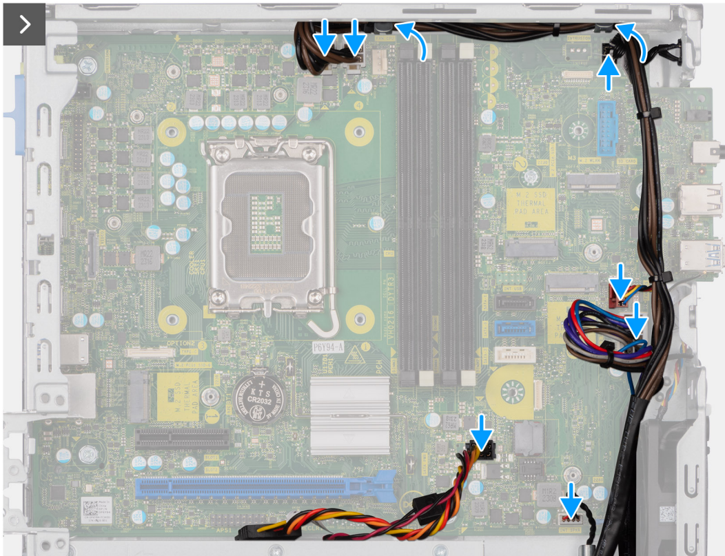
Figure 72. Installation de la carte système
