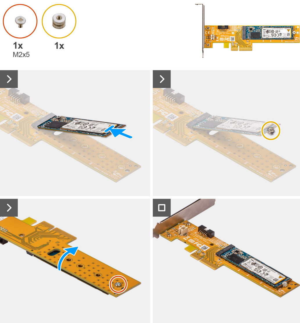
Figure 27. Installation du disque SSD M.2 2280 sur la carte Dell Ultra Speed Drive Gen 3
