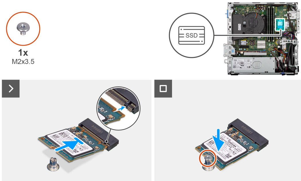
Figure 20. Installation du disque SSD M.2 2230 dans le logement 1
