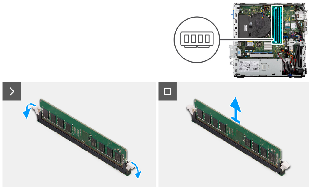
Figure 15. Retrait de la mémoire
