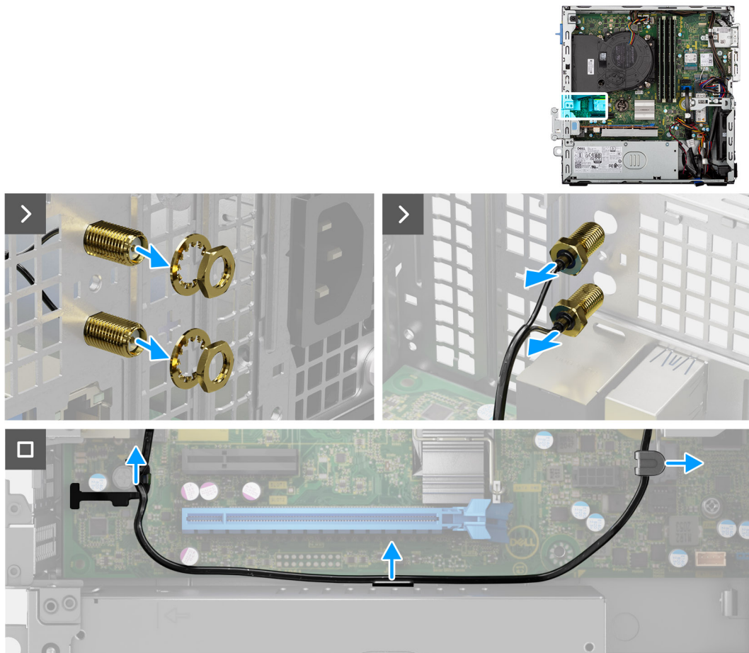
Figure 46. Retrait du module d'antenne SMA externe
