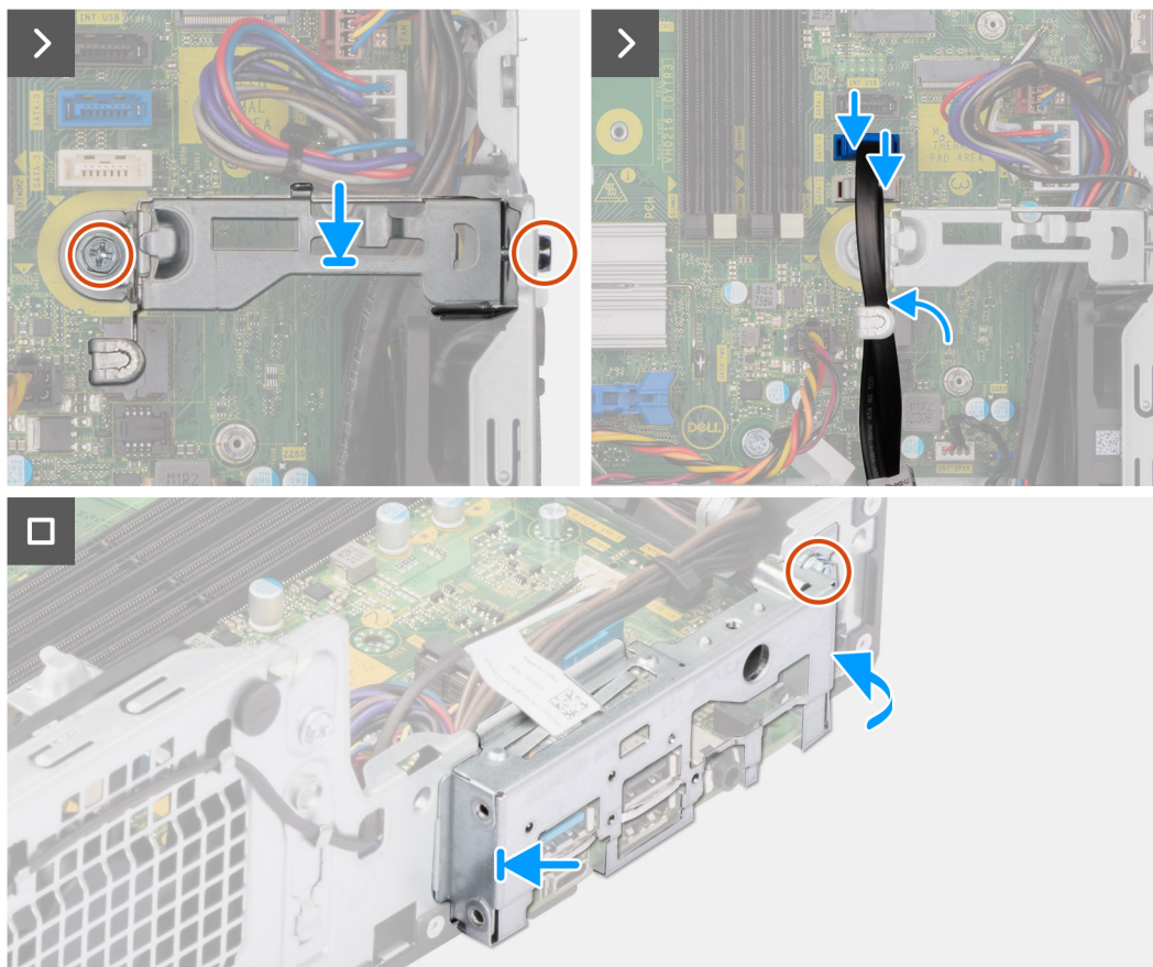
Figure 73. Installation de la carte système
