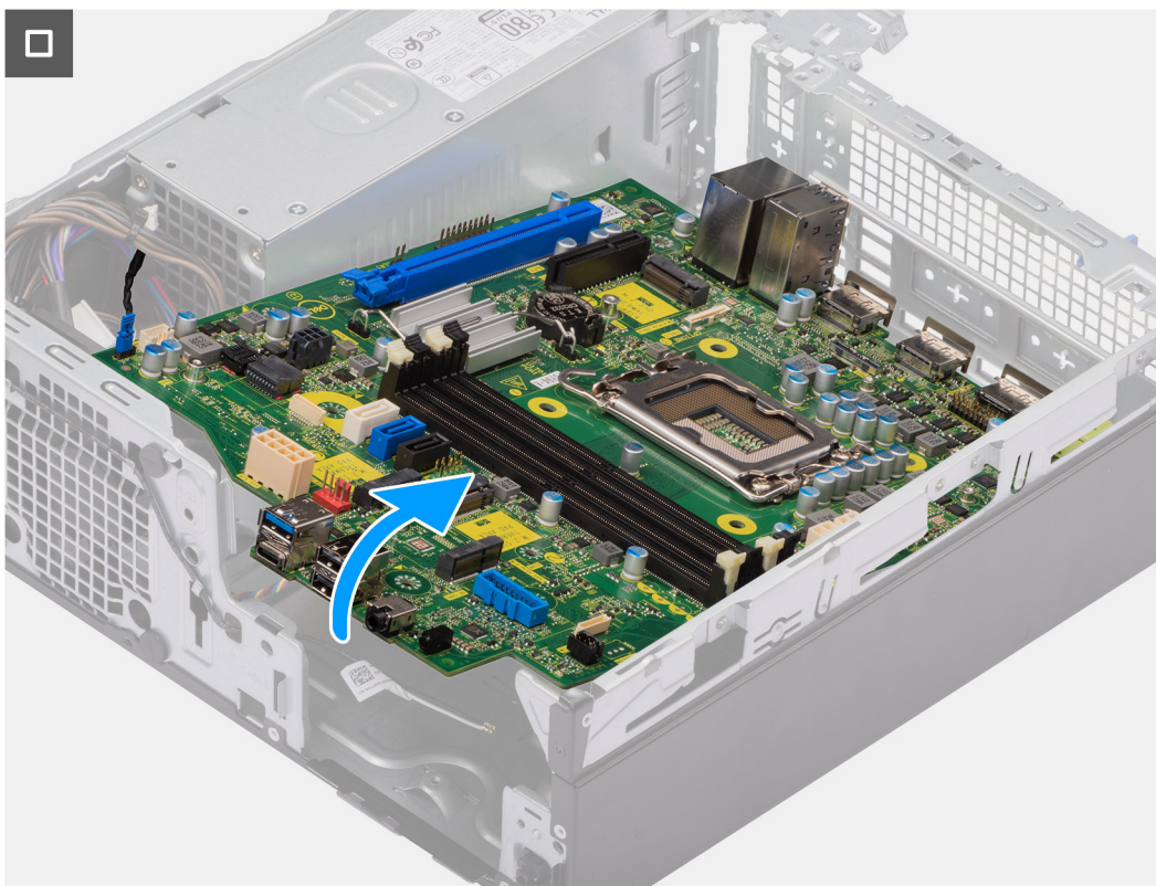
Figure 68. Retrait de la carte système
