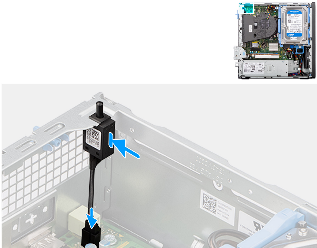
Figure 38. Installation du commutateur d'intrusion
