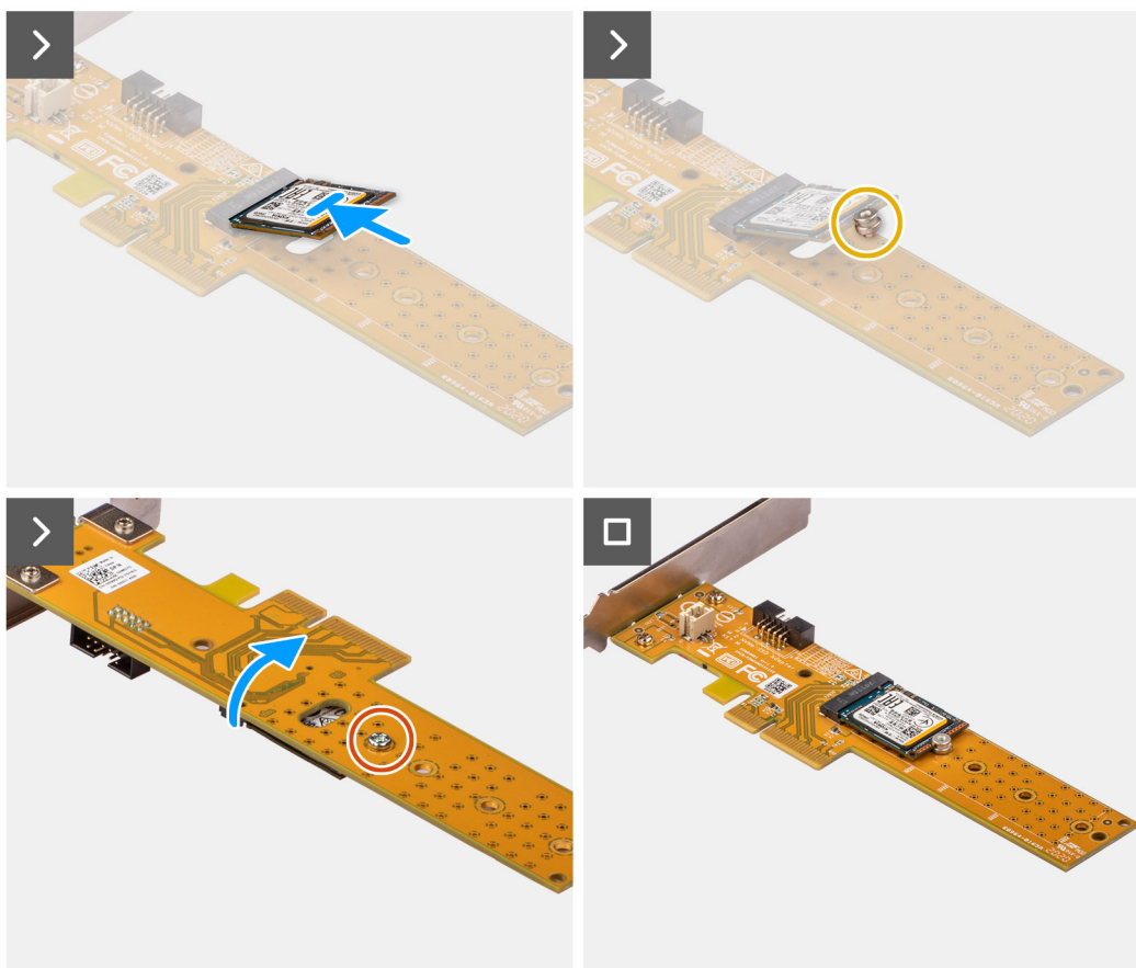
Figure 26. Installation du disque SSD M.2 2230 sur la carte Dell Ultra Speed Drive Gen 3
