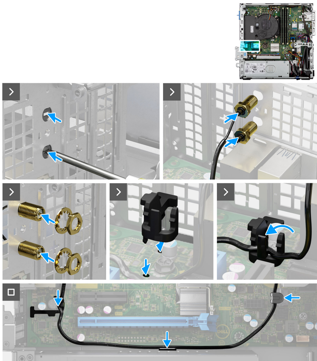
Figure 47. Installation du module d'antenne SMA externe
