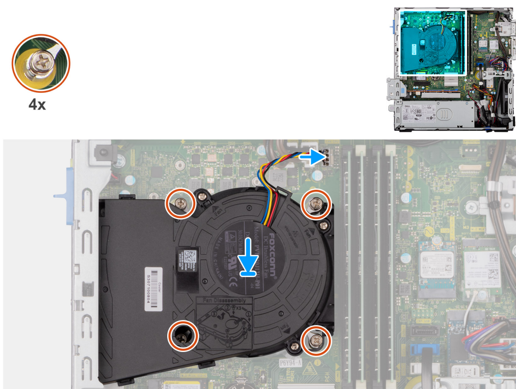
Figure 51. Installation de l'assemblage du ventilateur et du dissipateur de chaleur du processeur
