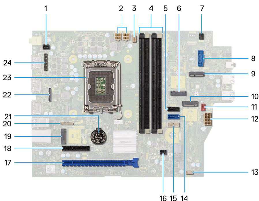
Figure 64. Présentation de la carte système
