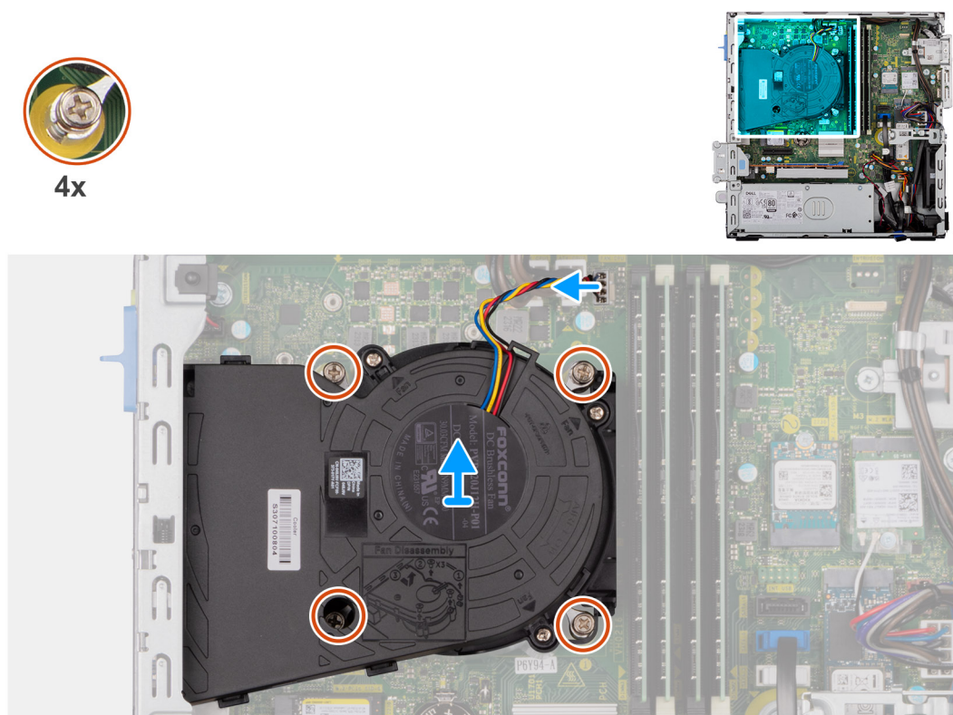
Figure 50. Retrait de l'assemblage du ventilateur et du dissipateur de chaleur du processeur
