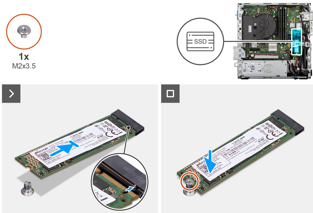
Figure 22. Installation du disque SSD M.2 2280
