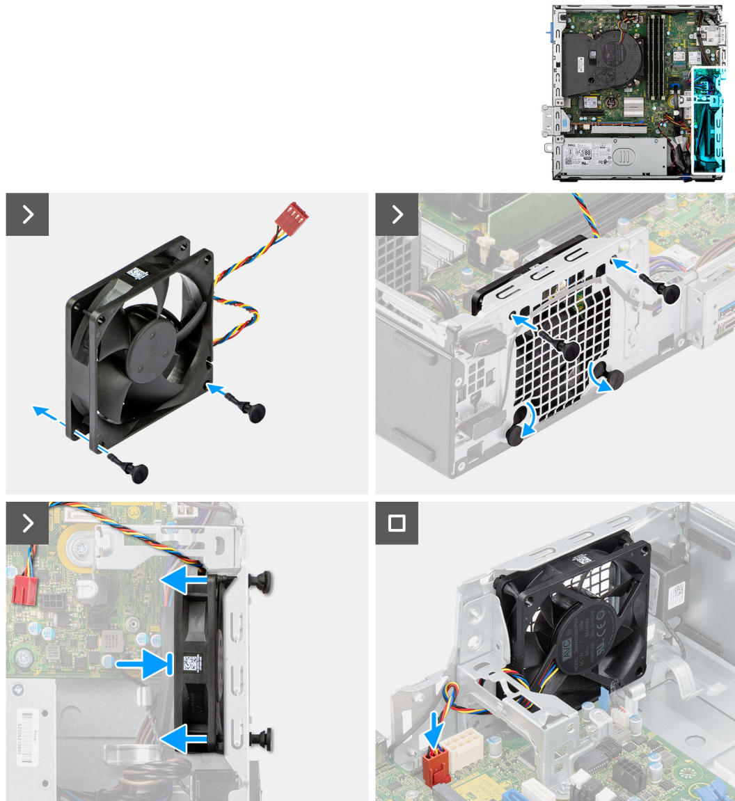
Figure 42. Installation du ventilateur système
