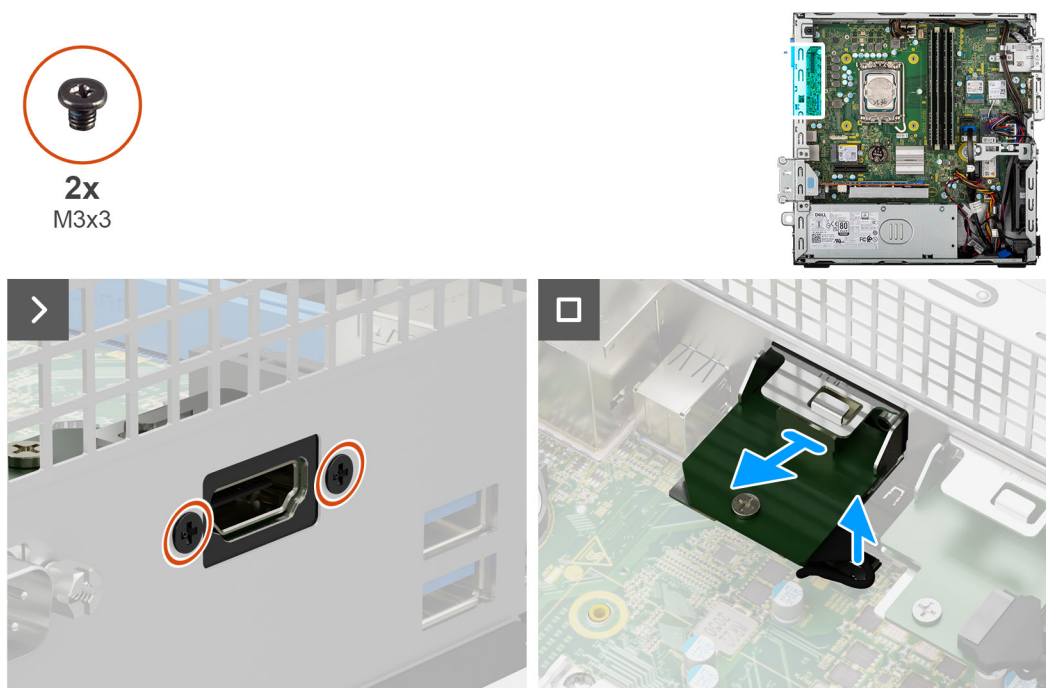
Figure 58. Retrait du module HDMI
