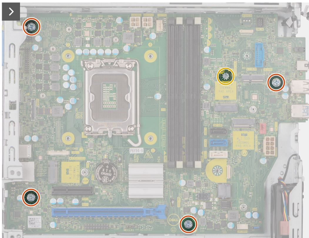
Figure 67. Retrait de la carte système
