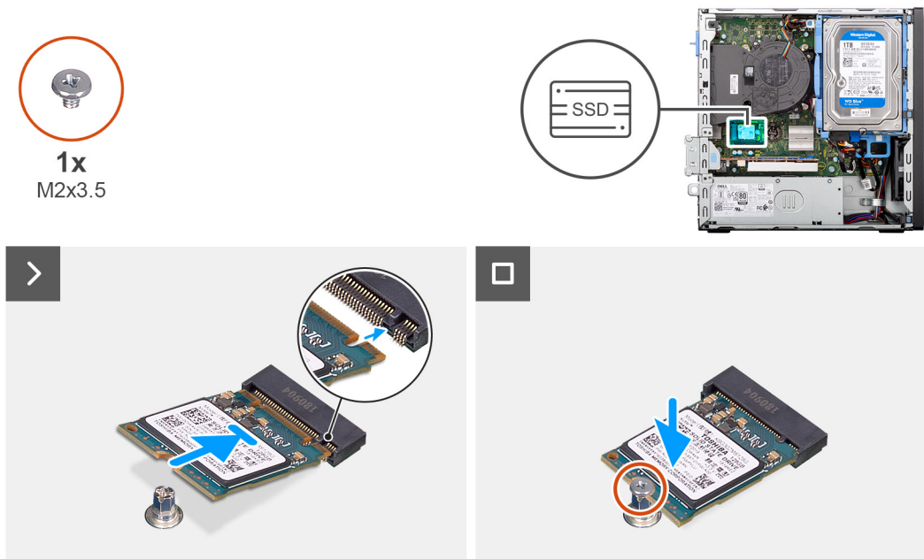
Figure 18. Installation du disque SSD M.2 2230 dans le logement 0
