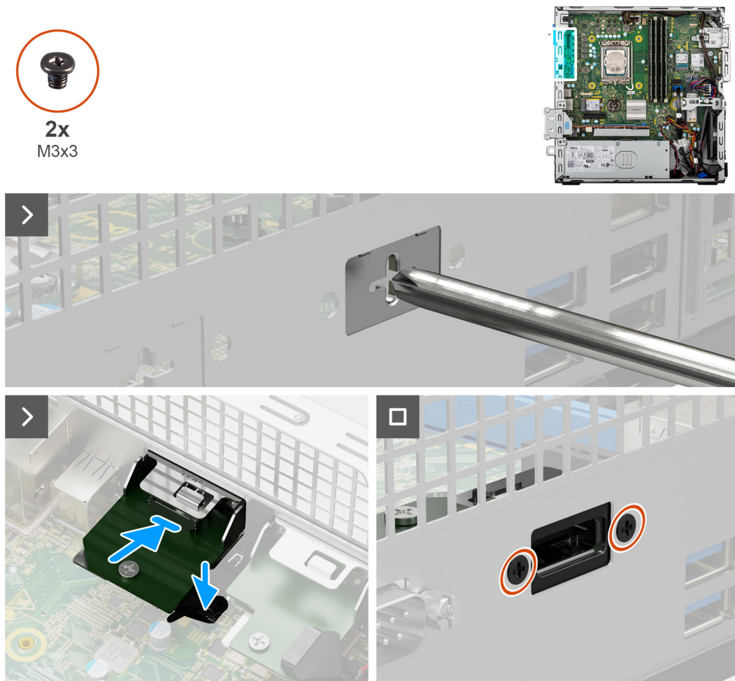
Figure 57. Installation du module DisplayPort
