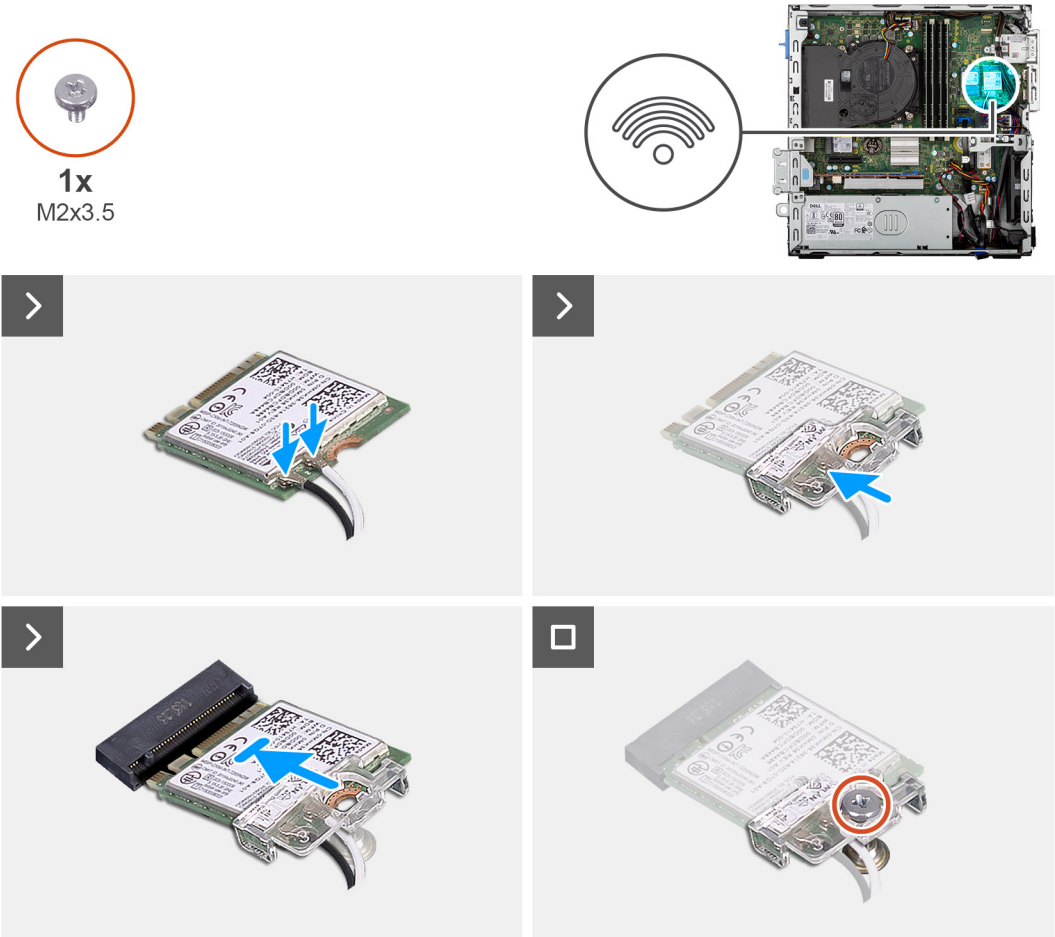
Figure 30. Installation de la carte sans fil
