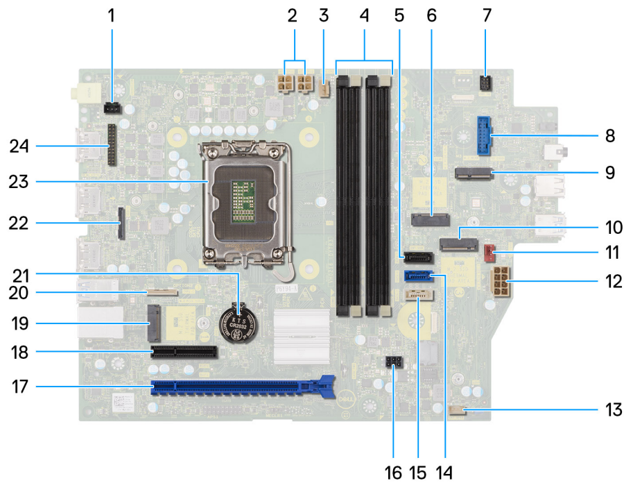
Figure 69. Présentation de la carte système
