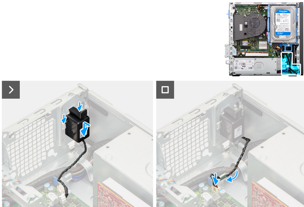
Figure 36. Installation du haut-parleur
