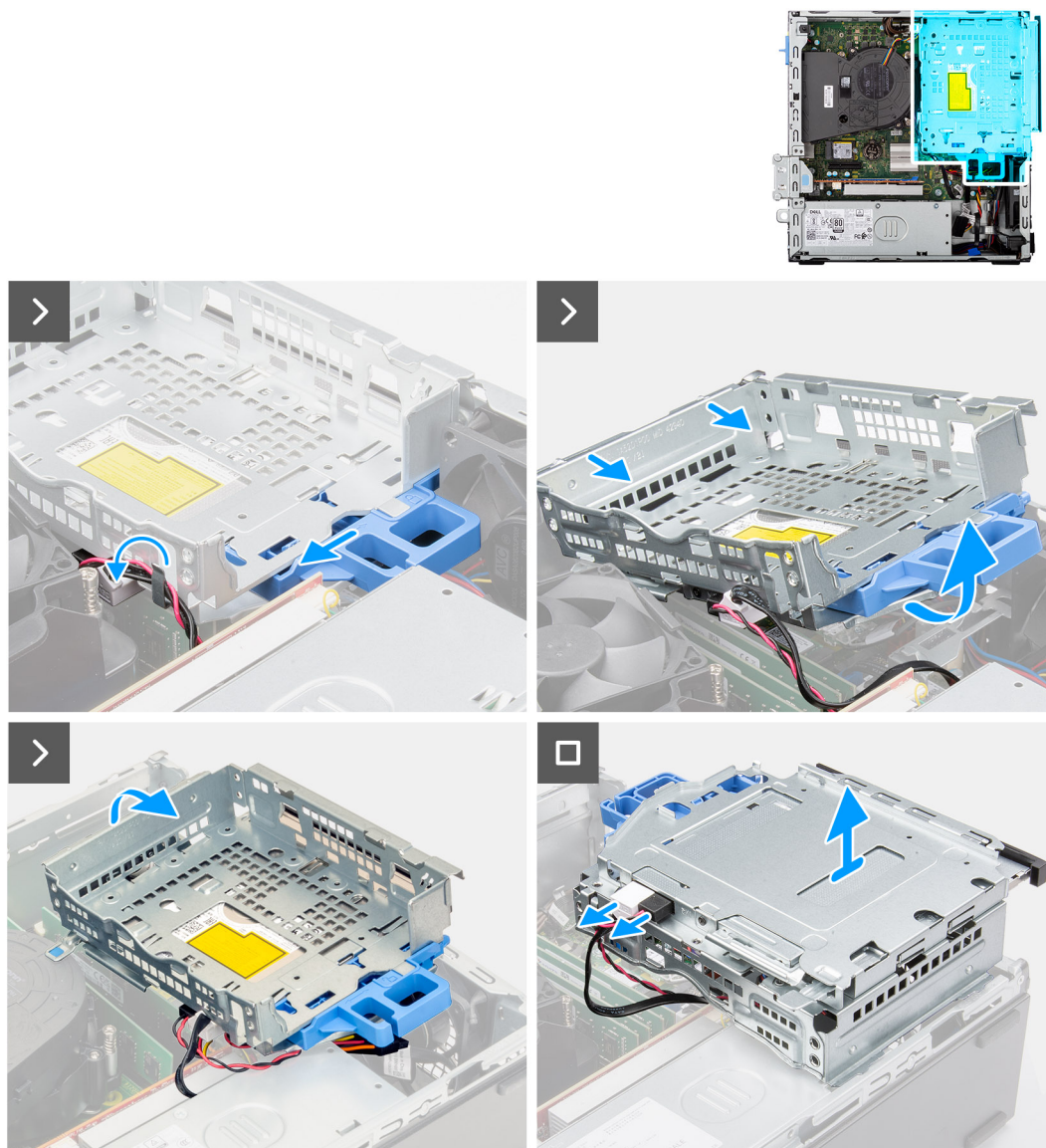
Figure 11. Retrait du bâti du lecteur de disque
