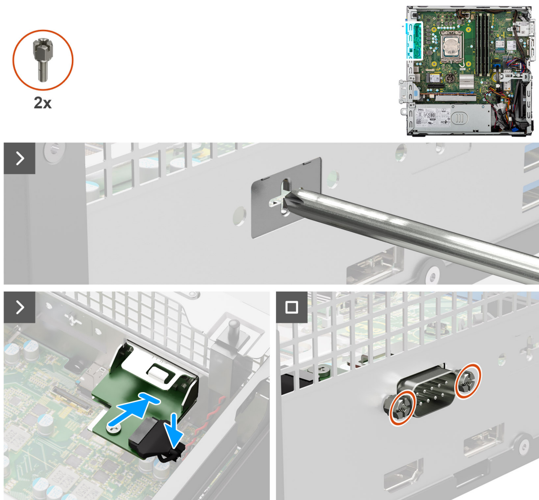
Figure 55. Installation du module série
