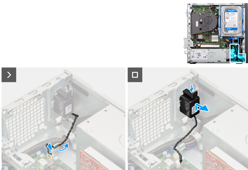
Figure 35. Retrait du haut-parleur
