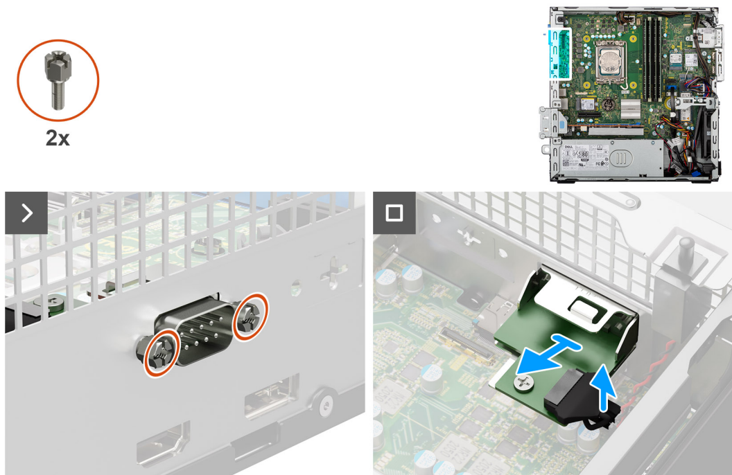
Figure 54. Retrait du module série
