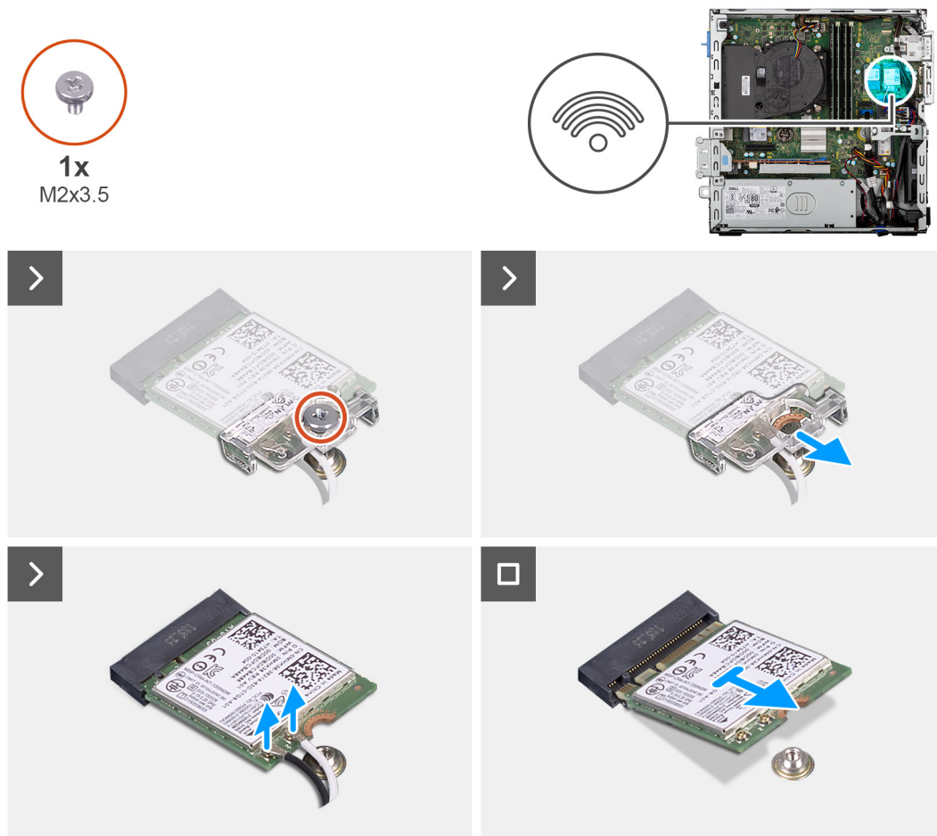
Figure 29. Retrait de la carte sans fil
