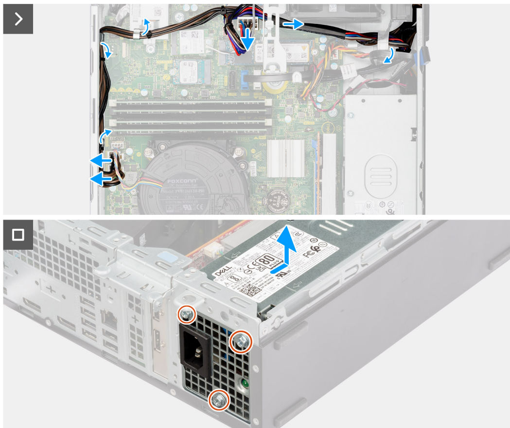
Figure 48. Retrait du bloc d'alimentation
