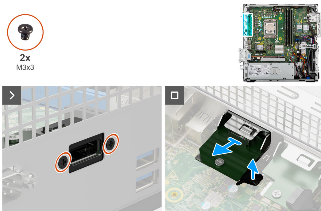
Figure 56. Retrait du module DisplayPort
