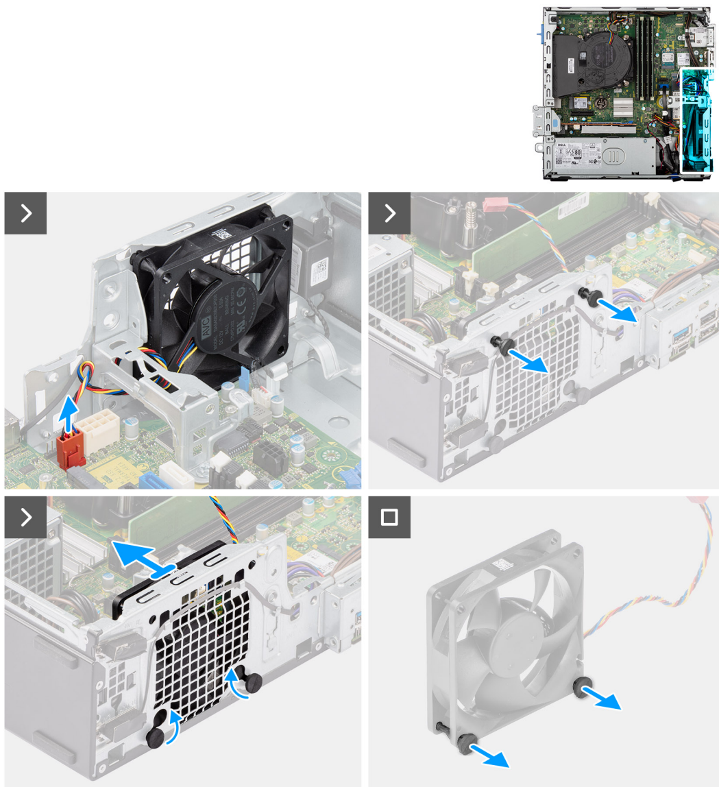
Figure 41. Retrait du ventilateur système
