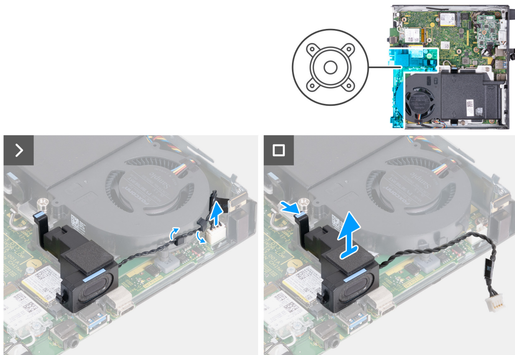
Figura 17. Rimozione dell'altoparlante
