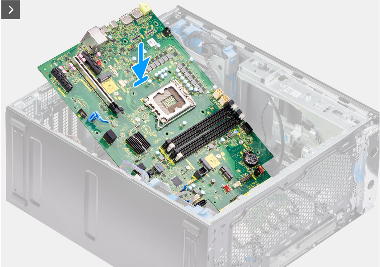
Afbeelding 80. De systeemkaart installeren
