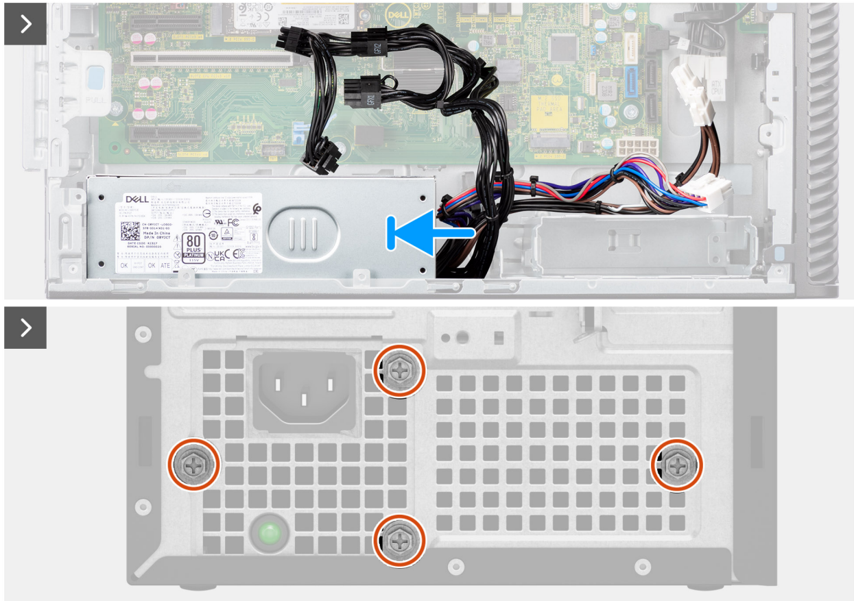
Afbeelding 51. De voedingseenheid van 1000 W plaatsen
