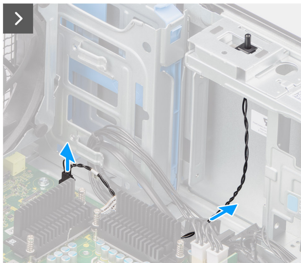
Afbeelding 70. De intrusieswitch verwijderen
