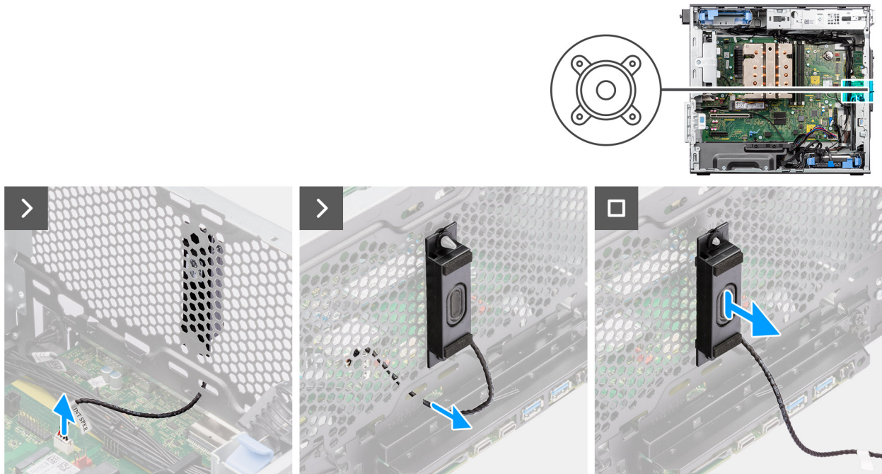
Afbeelding 72. De interne luidspreker verwijderen
