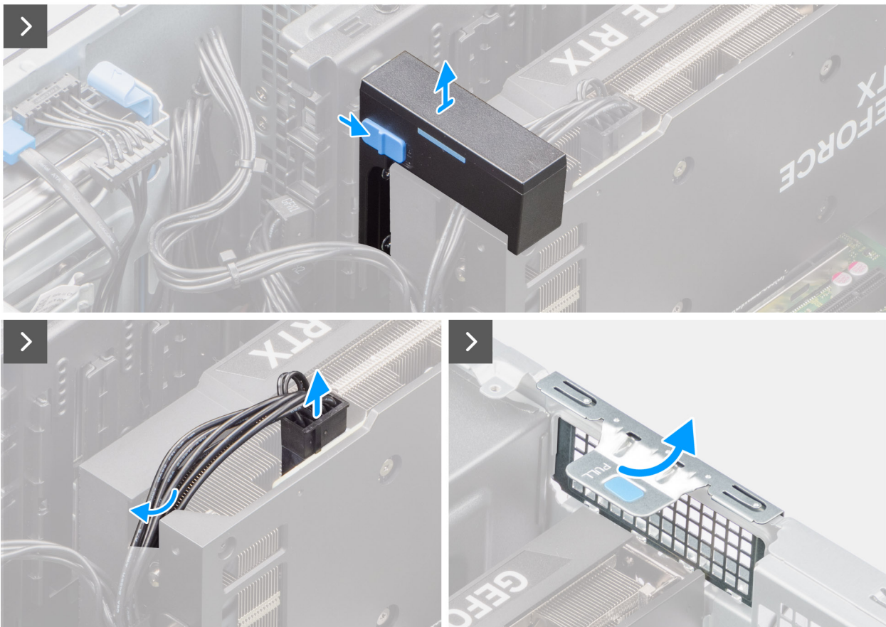
Afbeelding 40. De Powered GPU verwijderen
