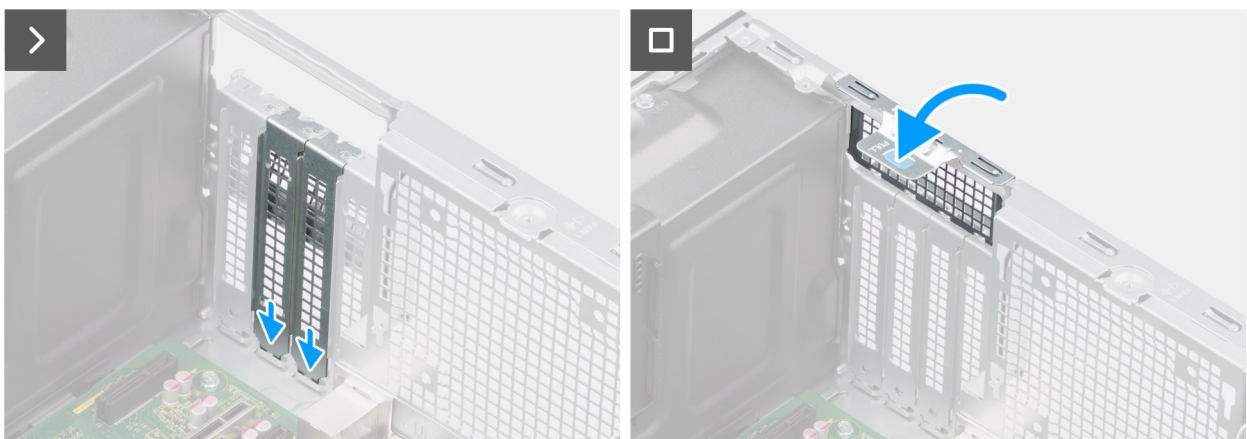
Afbeelding 42. De Powered GPU verwijderen
