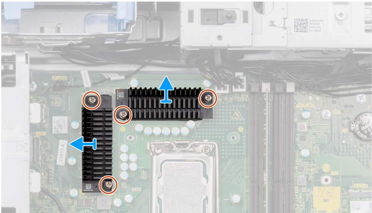
Afbeelding 58. De VR-koelplaat verwijderen
