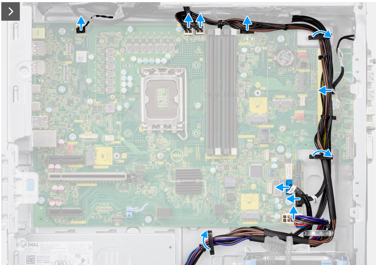
Afbeelding 76. De systeemkaart verwijderen
