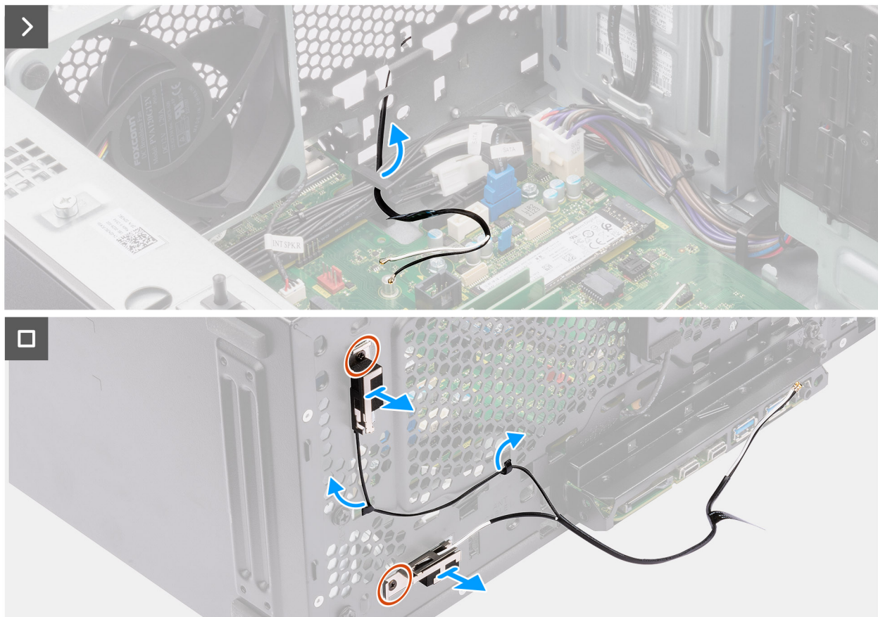
Afbeelding 28. De interne WLAN-antenne verwijderen
