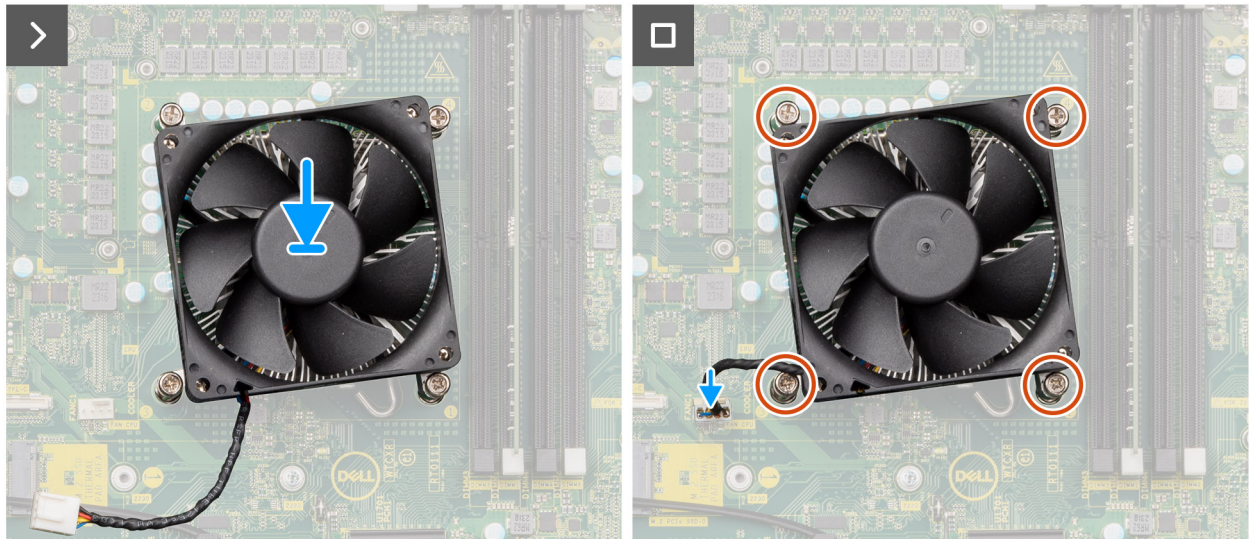
Afbeelding 55. De processorventilator en 65 W koelplaat eenheid plaatsen
