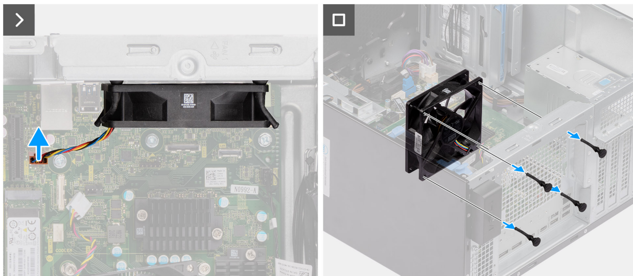
Afbeelding 64. De achterste ventilator voor 300 W PSU-systemen verwijderen
