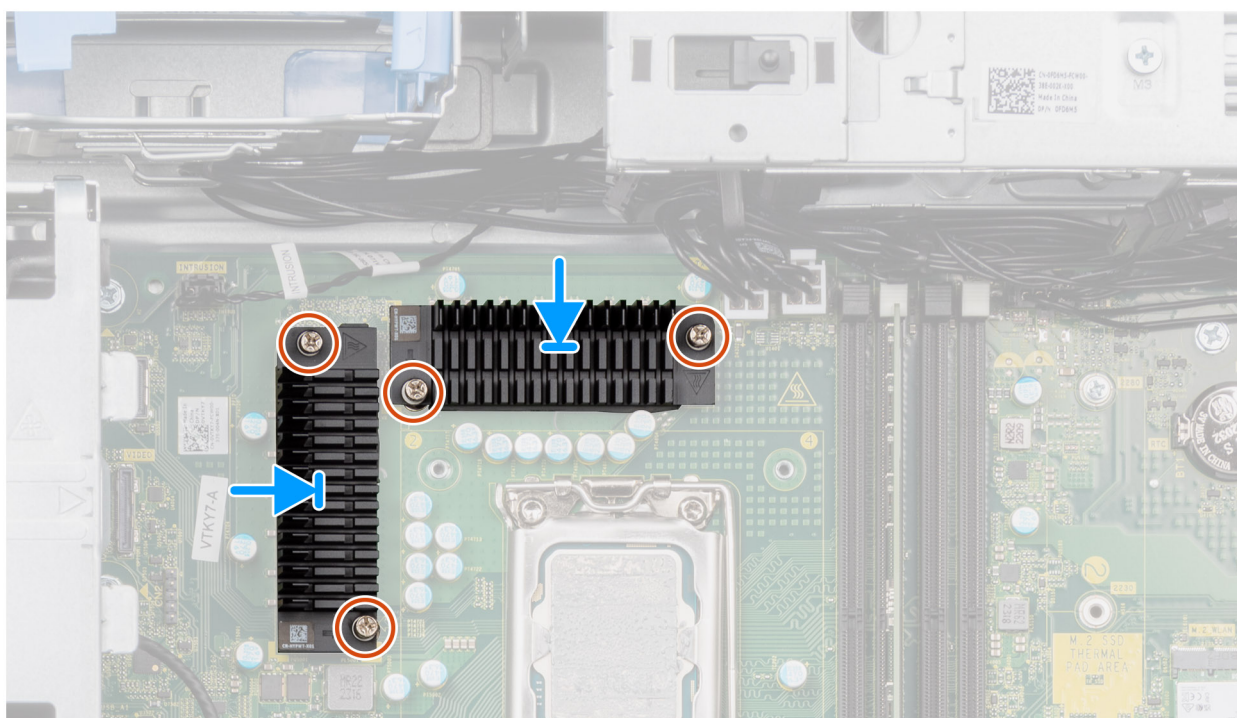
Afbeelding 59. De VR-koelplaat plaatsen
