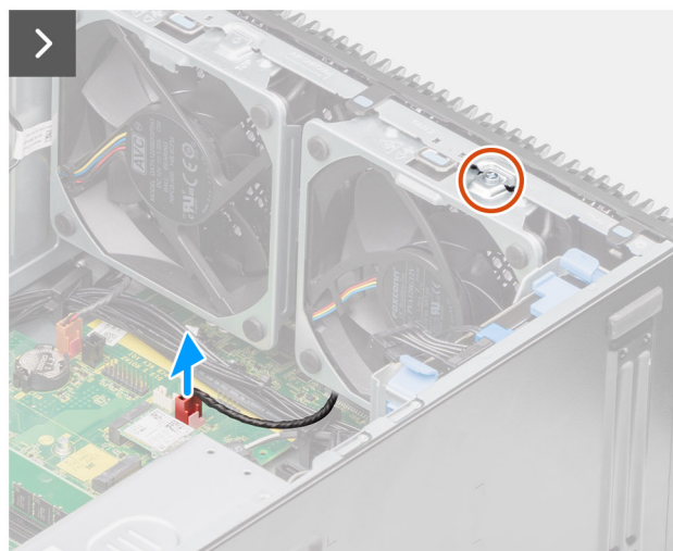
Afbeelding 60. Voorste ventilator 1
