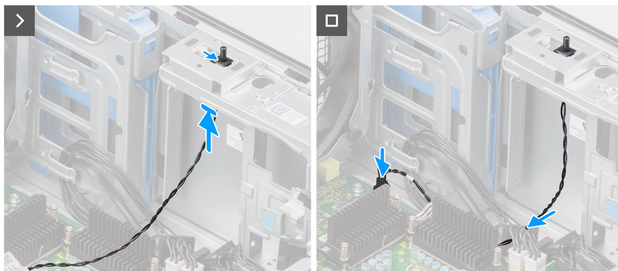
Afbeelding 71. De intrusieschakelaar plaatsen
