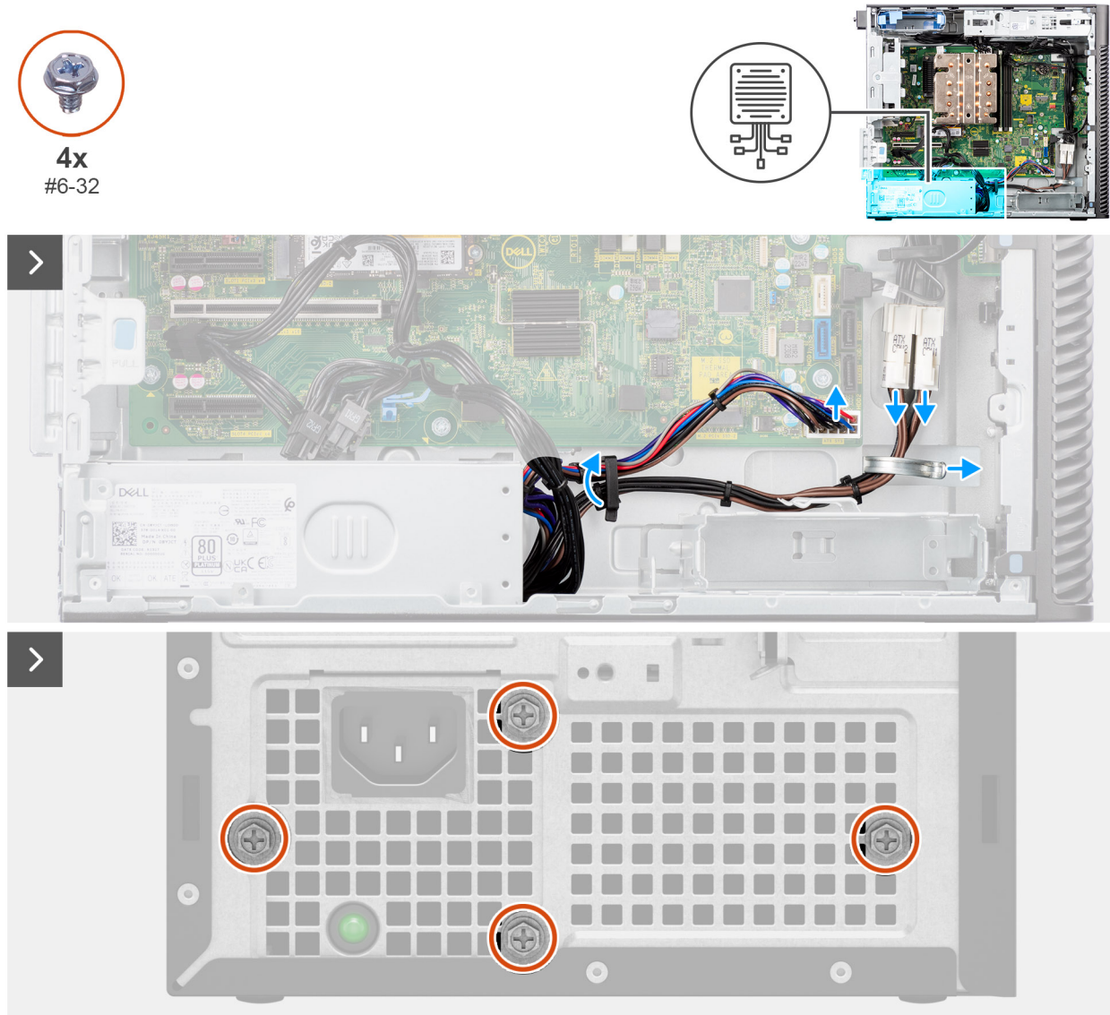
Afbeelding 48. De voedingseenheid van 1000 W verwijderen
