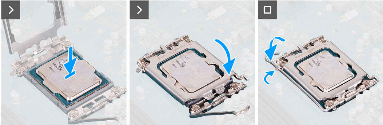
Afbeelding 57. De processor plaatsen
