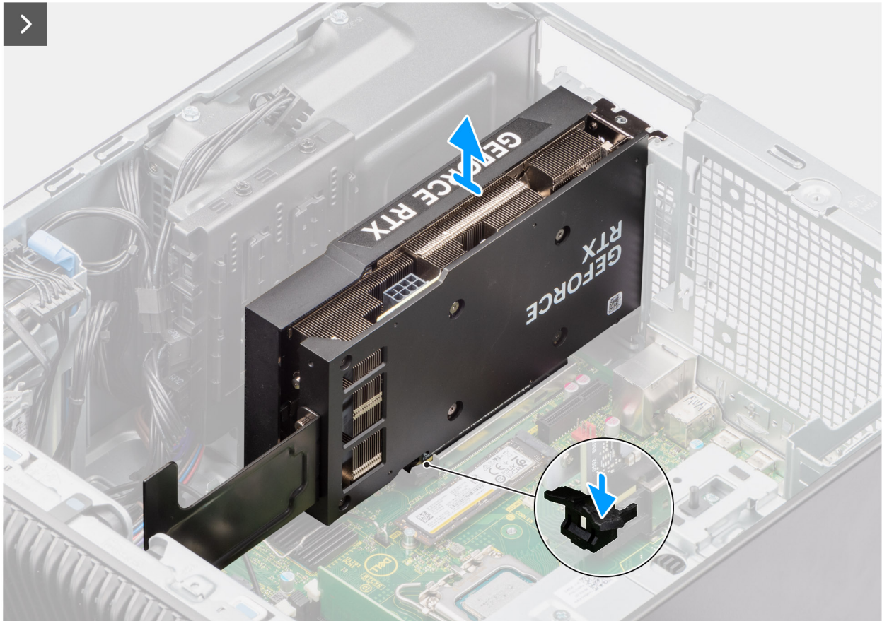
Afbeelding 41. De Powered GPU verwijderen
