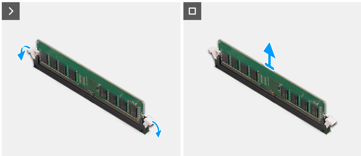
Afbeelding 32. De geheugenmodule verwijderen
