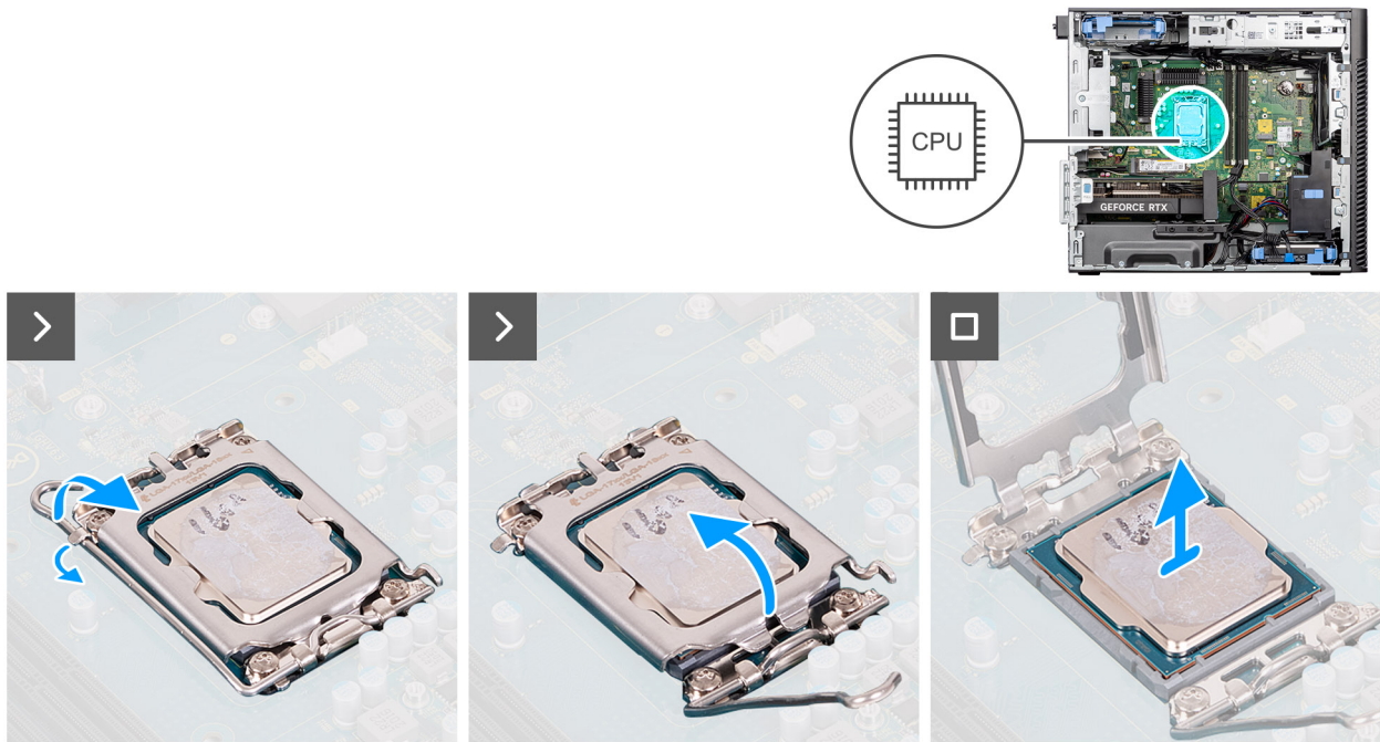
Afbeelding 56. De processor verwijderen
