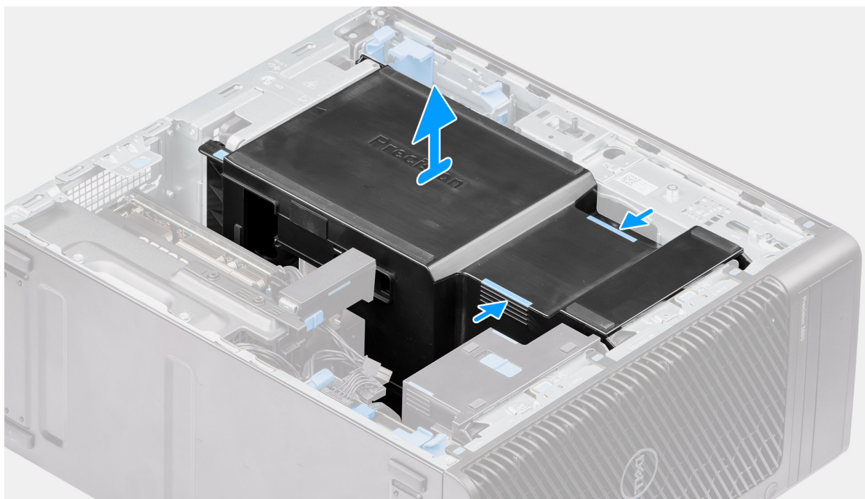
Afbeelding 14. De luchtkap verwijderen
