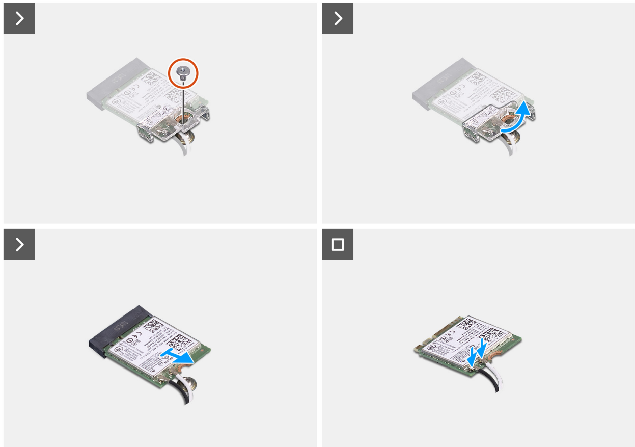
Afbeelding 26. De WLAN-kaart verwijderen
