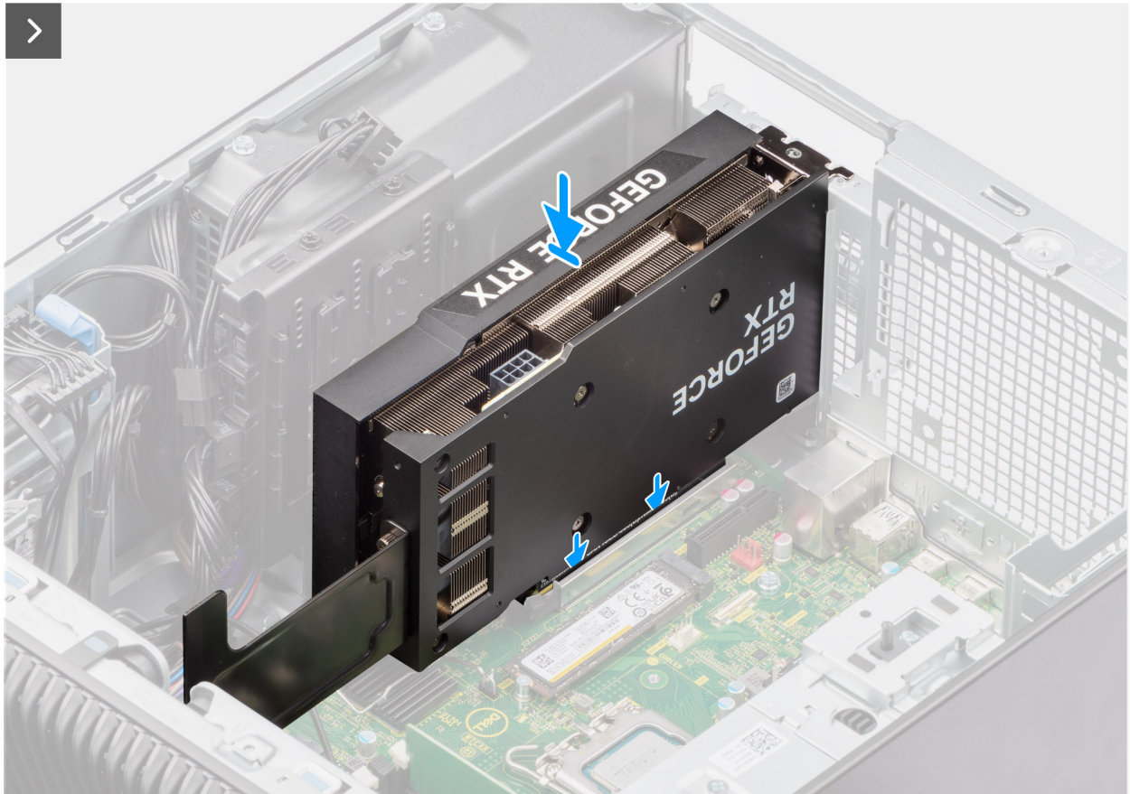
Afbeelding 44. De Powered GPU installeren
