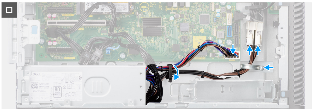
Afbeelding 50. De voedingseenheid van 1000 W plaatsen
