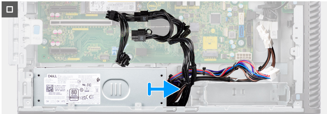
Afbeelding 49. De voedingseenheid van 1000 W verwijderen
