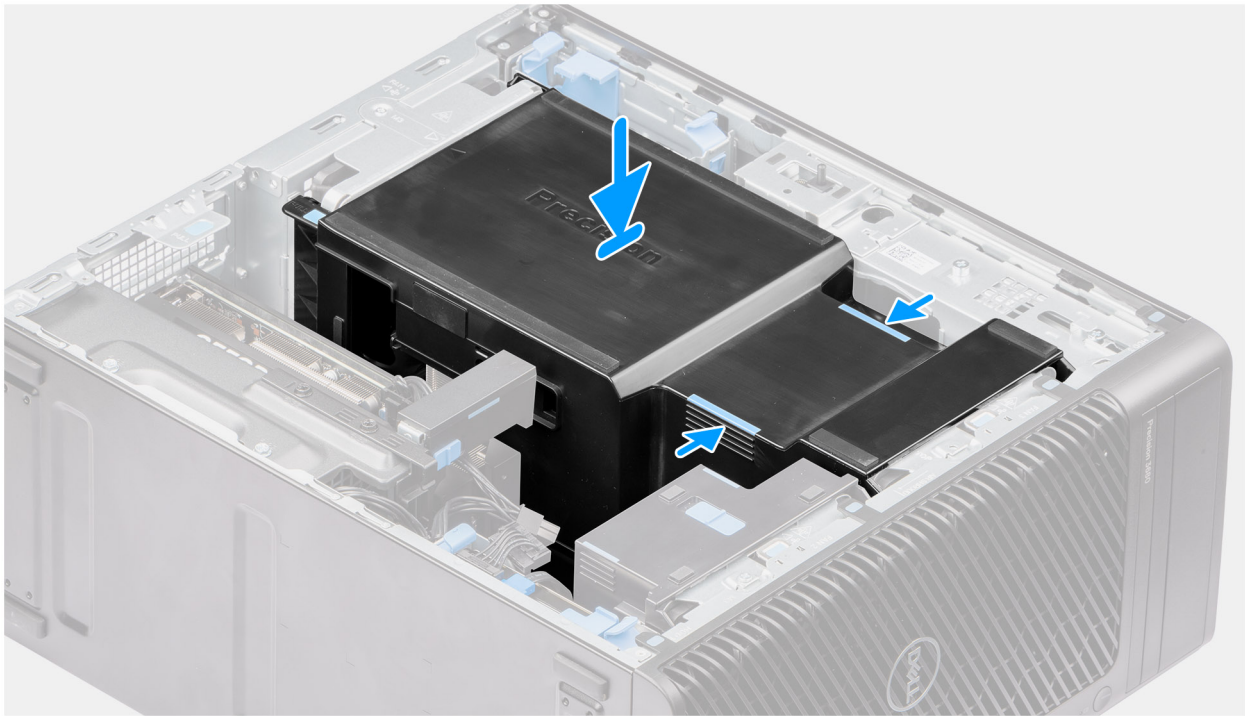
Afbeelding 15. De luchtkap plaatsen
