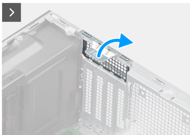
Afbeelding 43. De Powered GPU installeren
