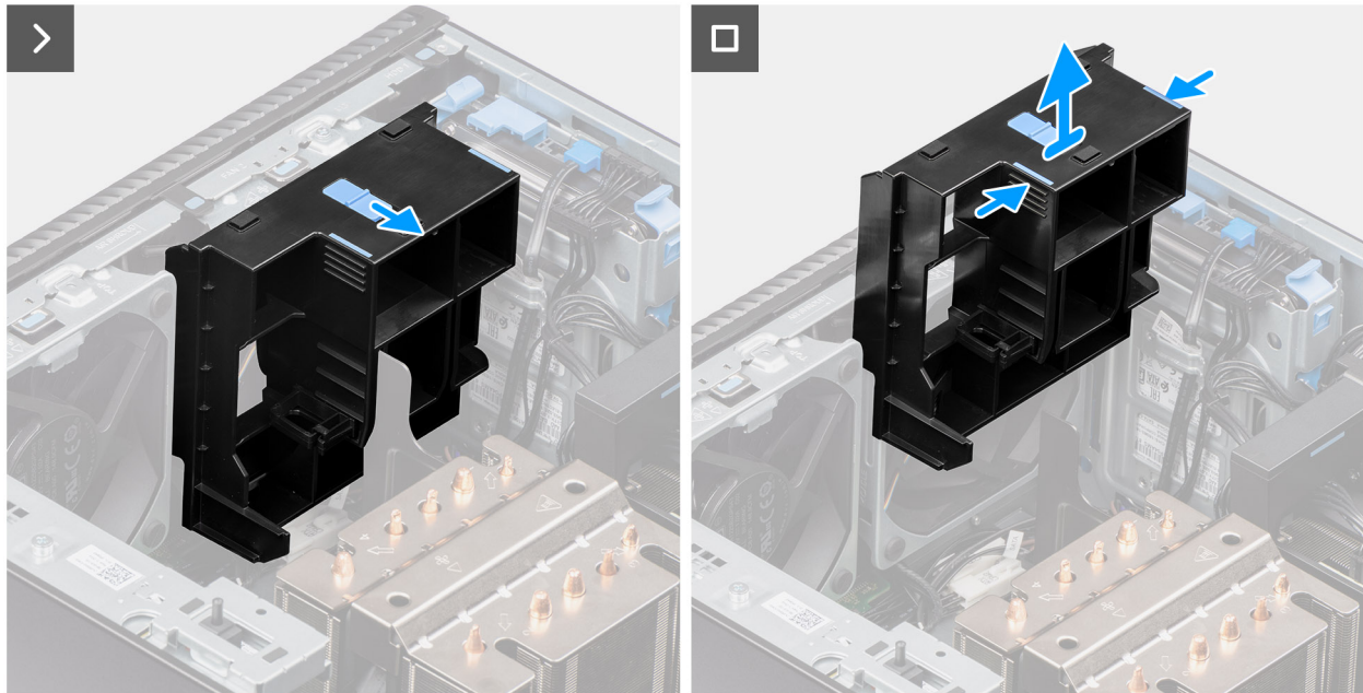
Afbeelding 34. De GPU-eindhouders verwijderen
