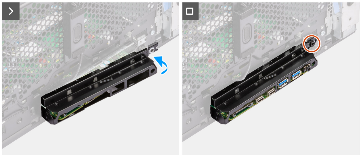
Afbeelding 83. De systeemkaart installeren
