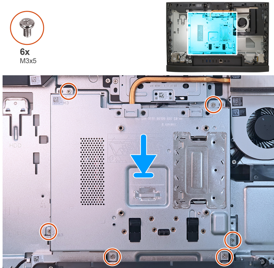
Ilustración 87. Instalación del protector de la tarjeta madre
