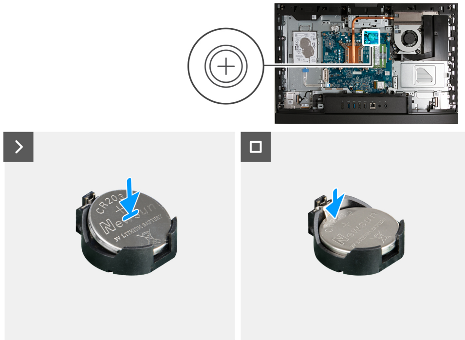
Ilustración 96. Instalación de la batería de tipo botón
