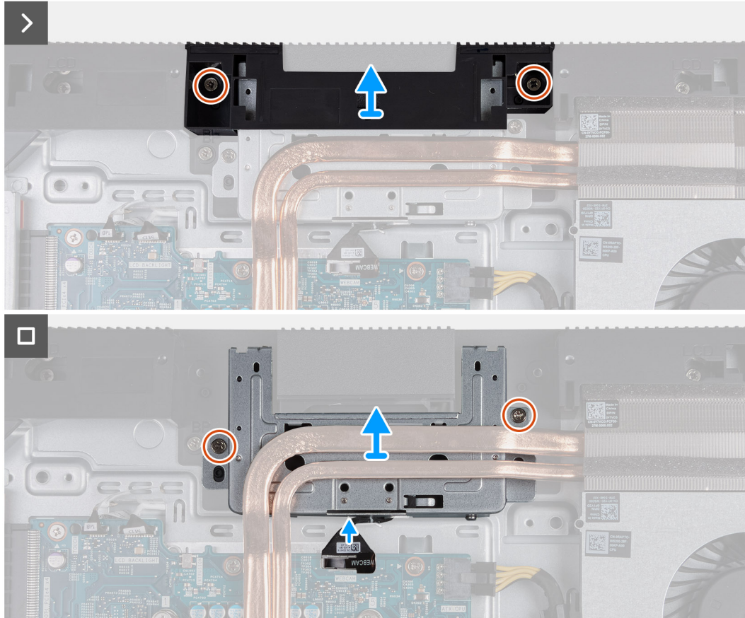
Ilustración 46. Extracción del ensamblaje de la cámara retráctil
