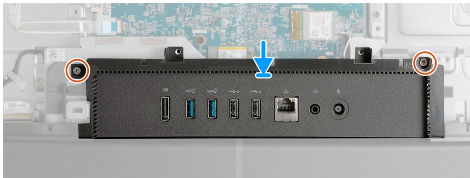
Ilustración 98. Instalación de la cubierta de I/O
