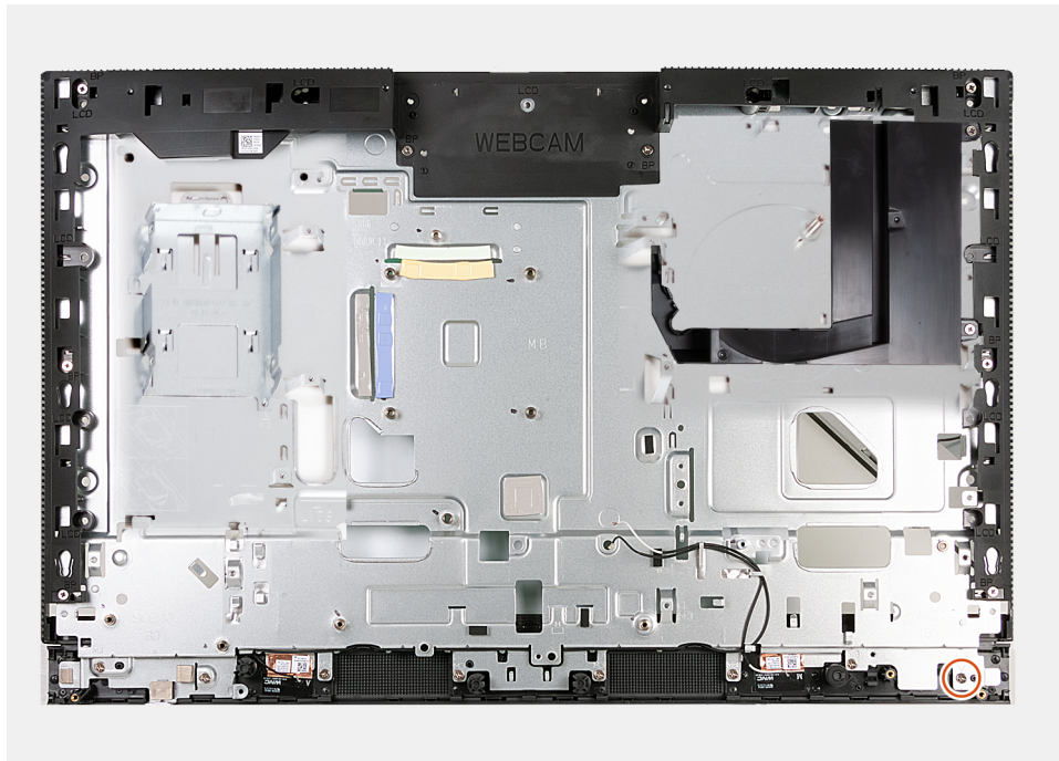
Ilustración 123. Extracción de la base del ensamblaje de la pantalla
