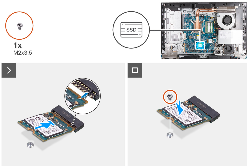
Ilustración 36. Instalación de la unidad de estado sólido M.2 2230 en la ranura M.2 1
