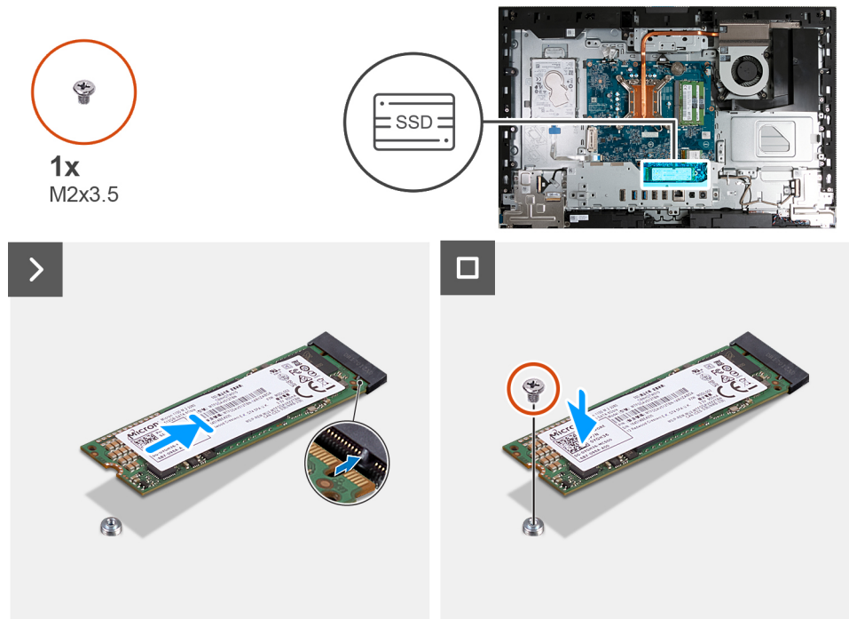
Ilustración 93. Instalación de la unidad de estado sólido M.2 2280
