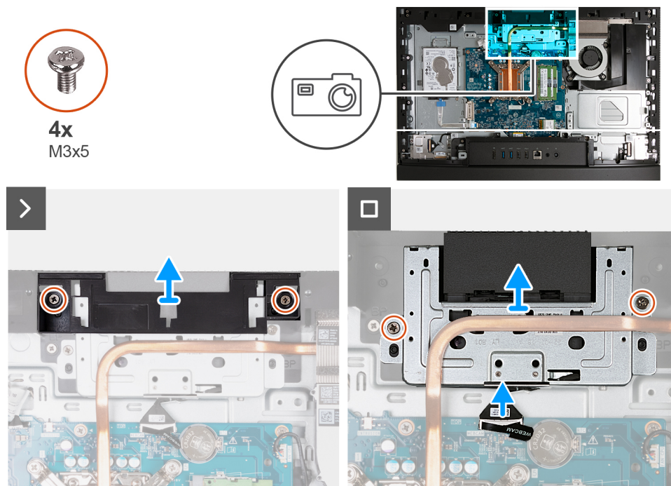
Ilustración 101. Extracción del ensamblaje de la cámara retráctil
