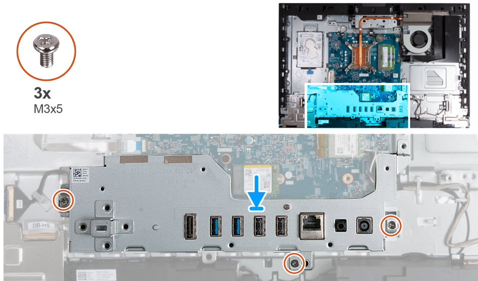
Ilustración 106. Instalación del soporte de I/O
