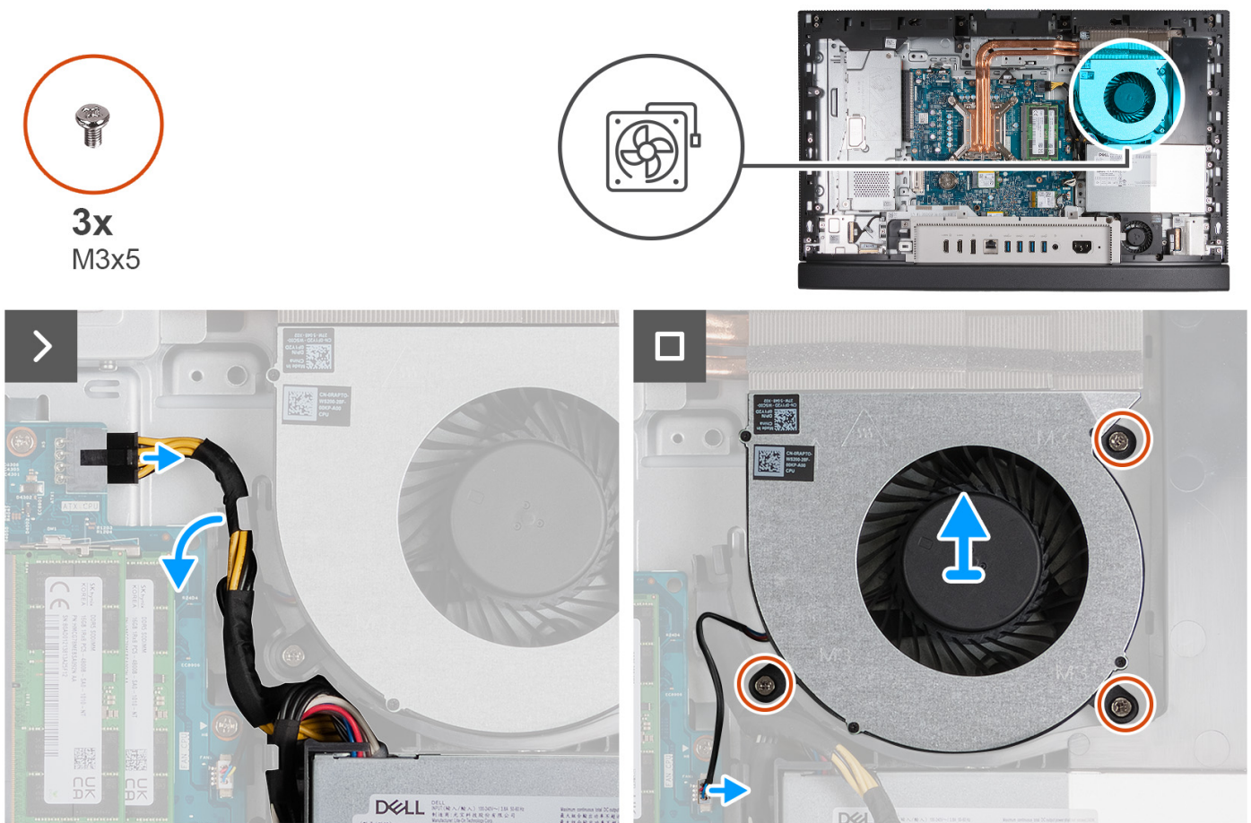
Ilustración 48. Extracción del ventilador
