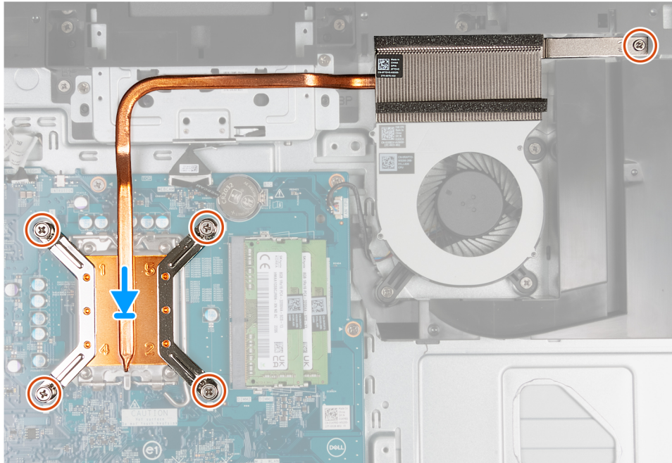
Ilustración 110. Instalación del disipador de calor
