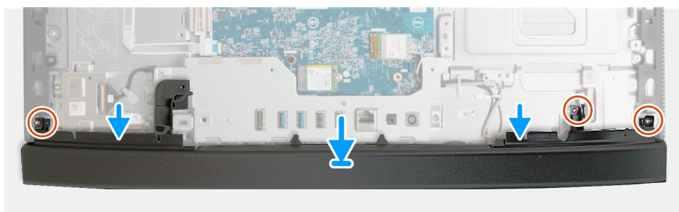
Ilustración 100. Instalación de la cubierta inferior
