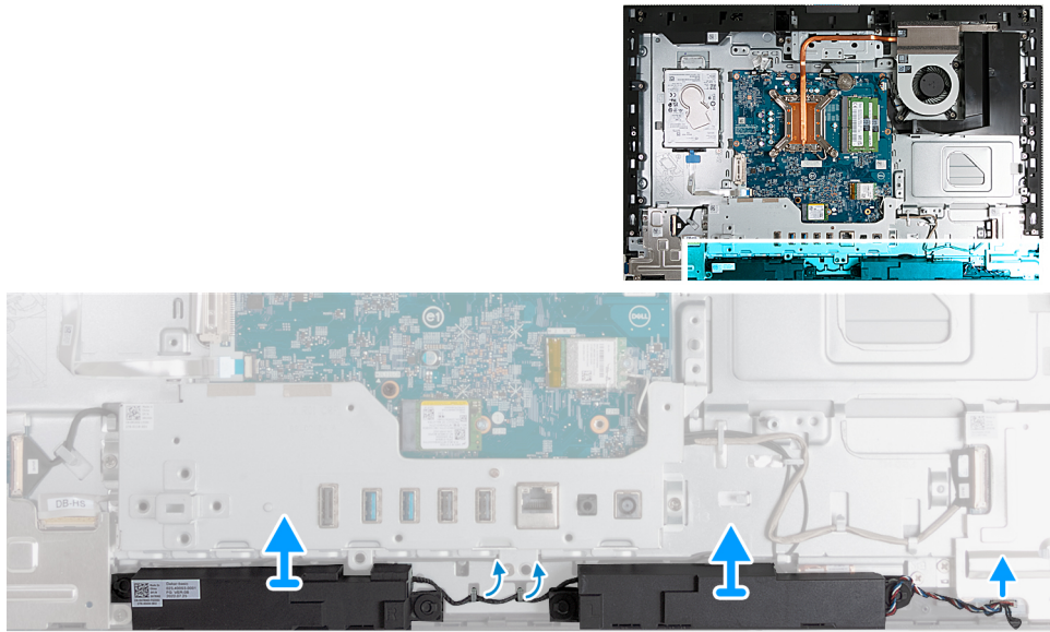
Ilustración 107. Extracción de los parlantes
