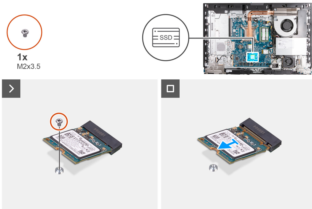
Ilustración 35. Extracción de la unidad de estado sólido M.2 2230 de la ranura M.2 1
