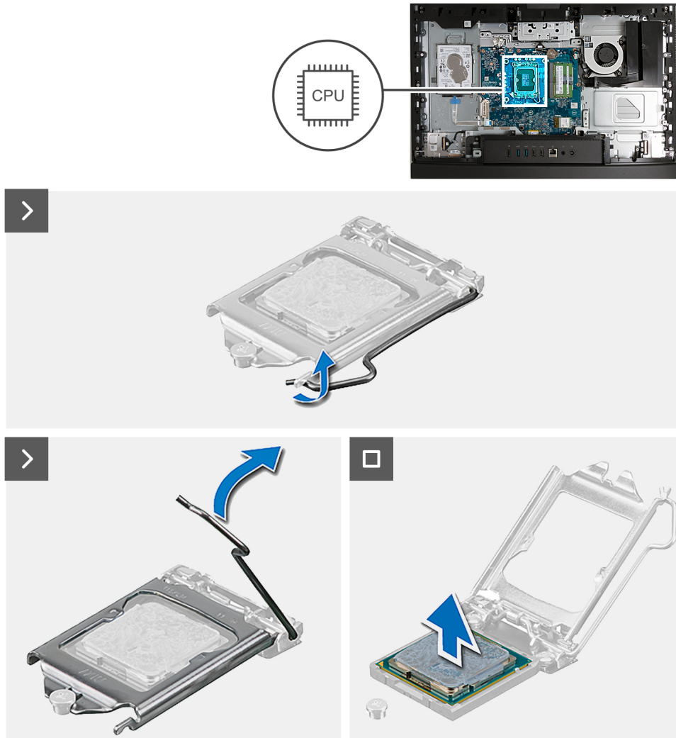
Ilustración 111. Extracción del procesador
