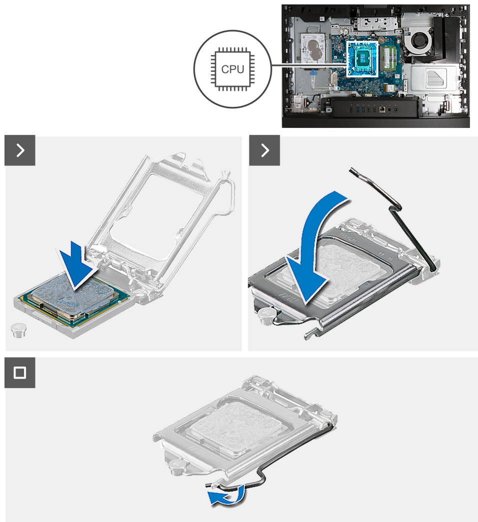
Ilustración 112. Instalación del procesador
