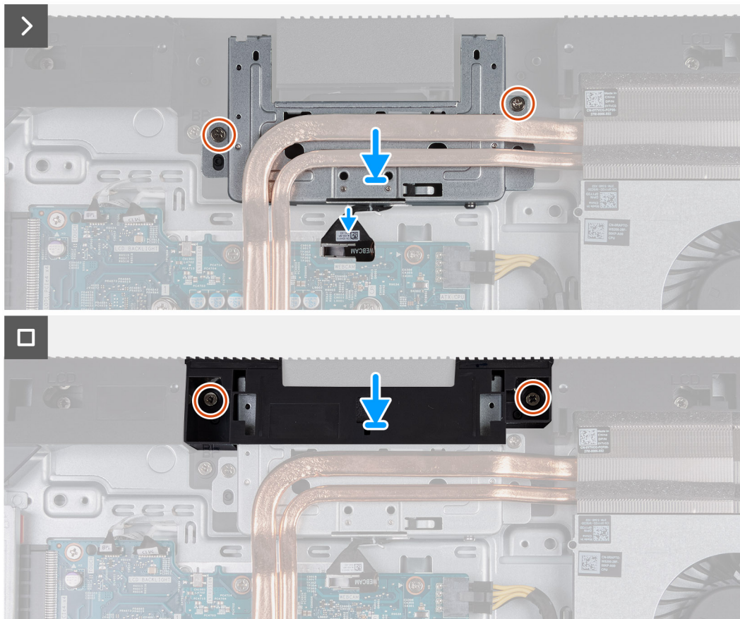
Ilustración 47. Instalación del ensamblaje de la cámara retráctil
