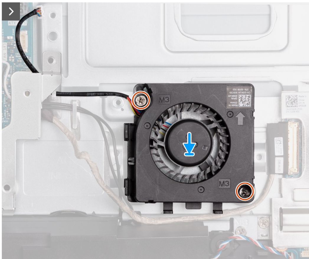
Ilustración 55. Instalación de la fuente de alimentación del ventilador
