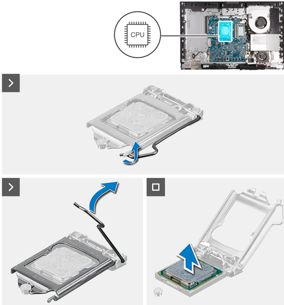
Ilustración 64. Extracción del procesador
