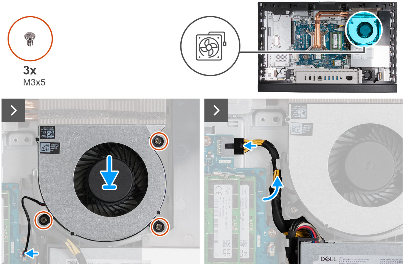
Ilustración 49. Instalación del ventilador
