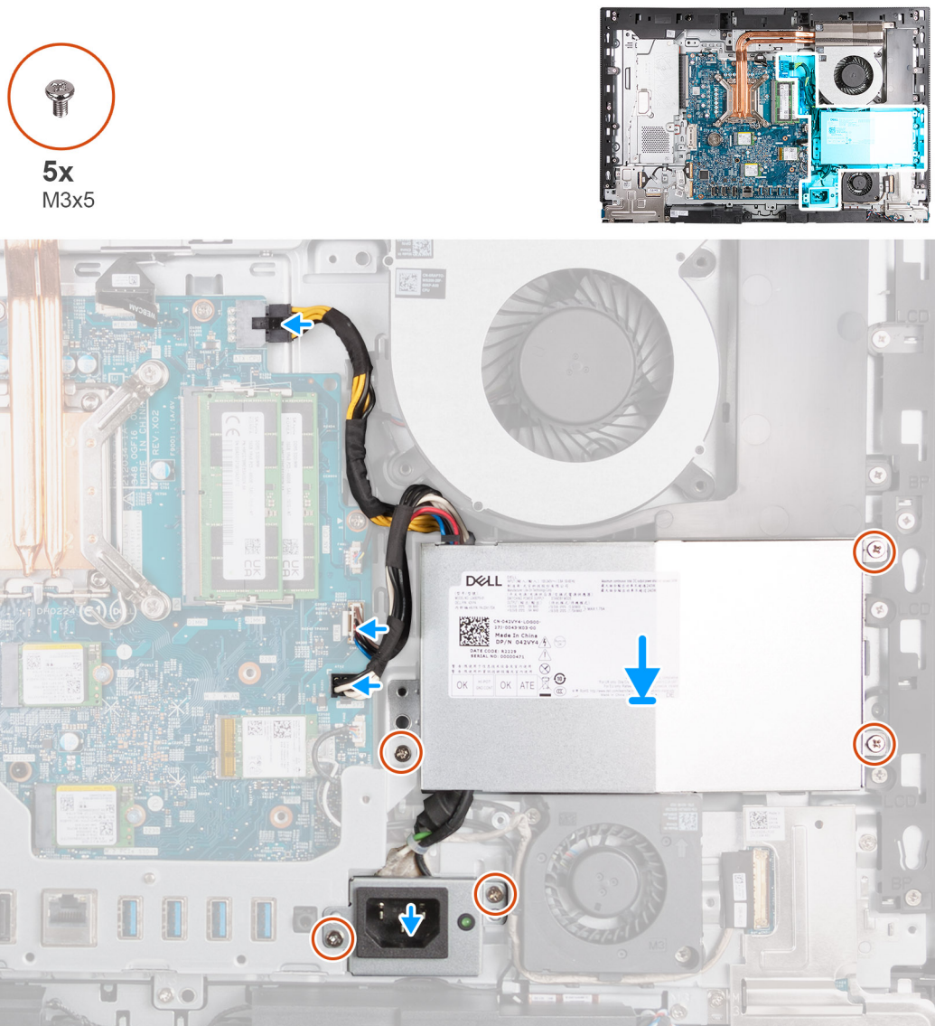
Ilustración 51. Instalación de la fuente de alimentación
