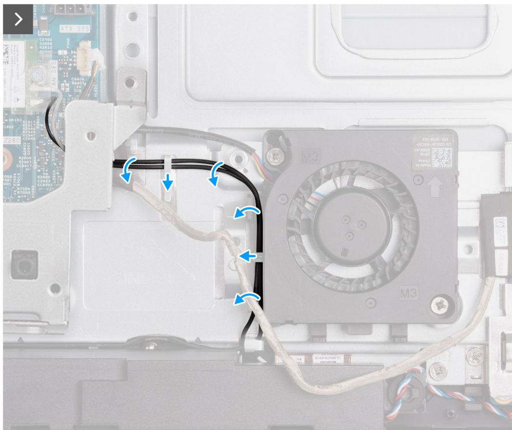
Ilustración 53. Extracción del ventilador de la fuente de alimentación
