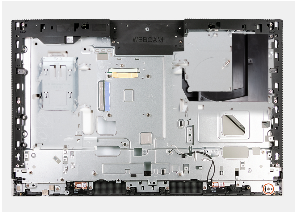
Ilustración 124. Instalación de la base del ensamblaje de la pantalla
