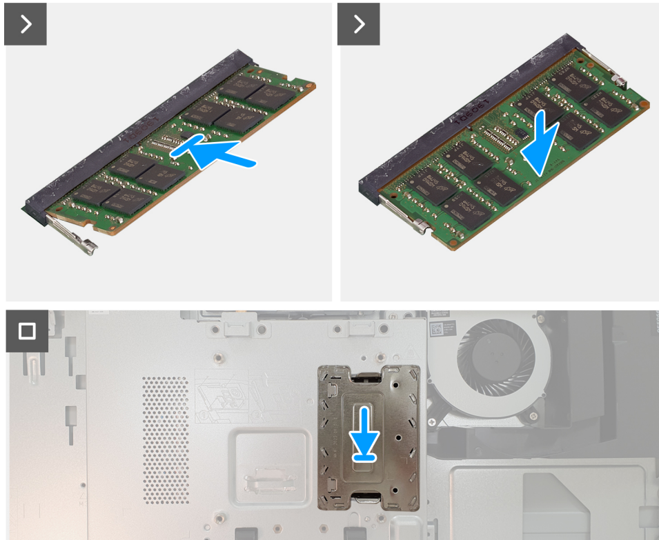
Ilustración 85. Instalación de la memoria
