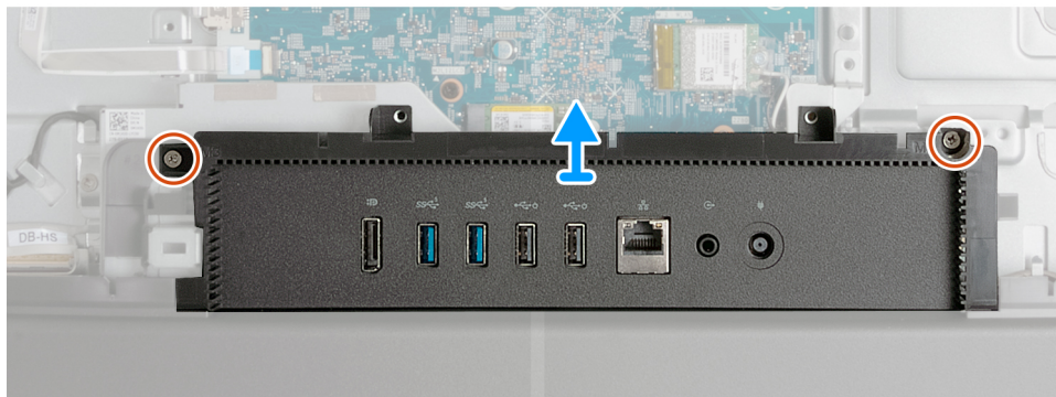
Ilustración 97. Extracción de la cubierta de I/O
