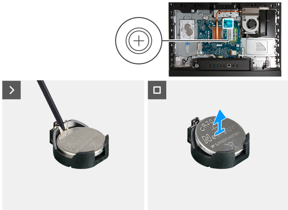
Ilustración 95. Extracción de la batería de tipo botón
