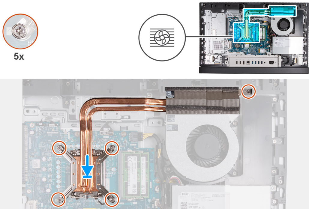
Ilustración 63. Instalación del disipador de calor
