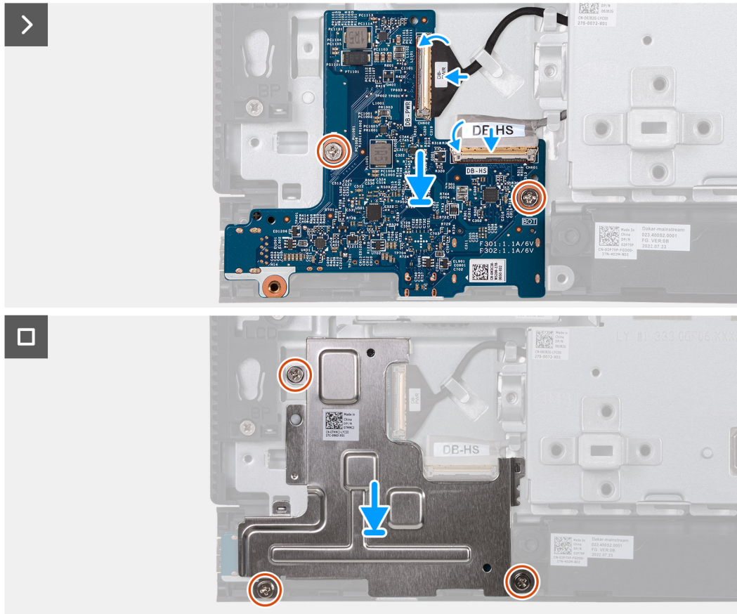
Ilustración 73. Instalación de la placa de I/O y del botón de encendido
