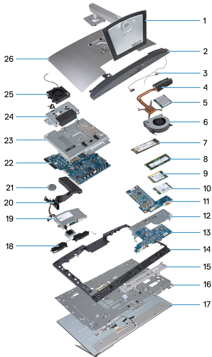
Ilustración 16. Componentes principales de la OptiPlex All-in-One 7420 con un procesador de alto rendimiento
