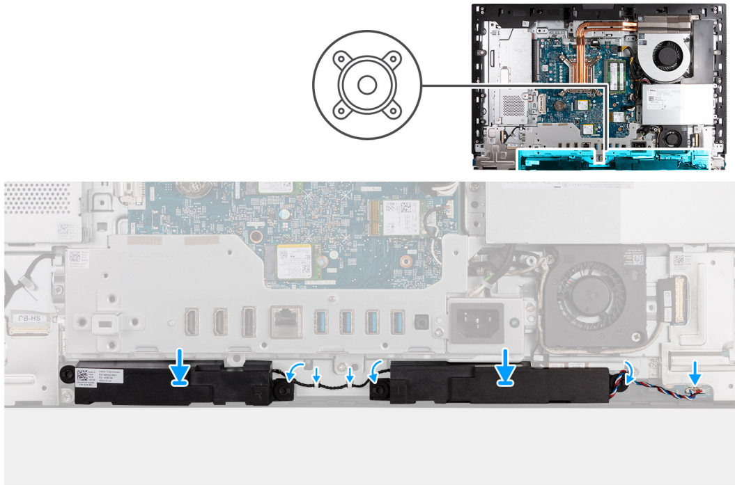
Ilustración 61. Instalación de los parlantes
