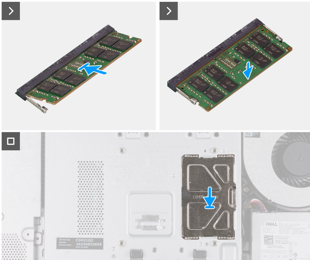
Ilustración 25. Instalación de la memoria
