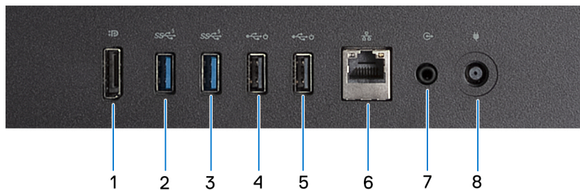
Ilustración 7. Vista del panel posterior de OptiPlex All-in-One 7420 con un procesador con uso eficiente de la energía
