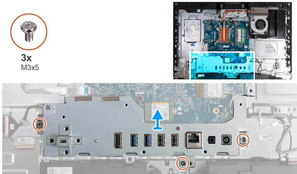
Ilustración 105. Extracción del soporte de I/O
