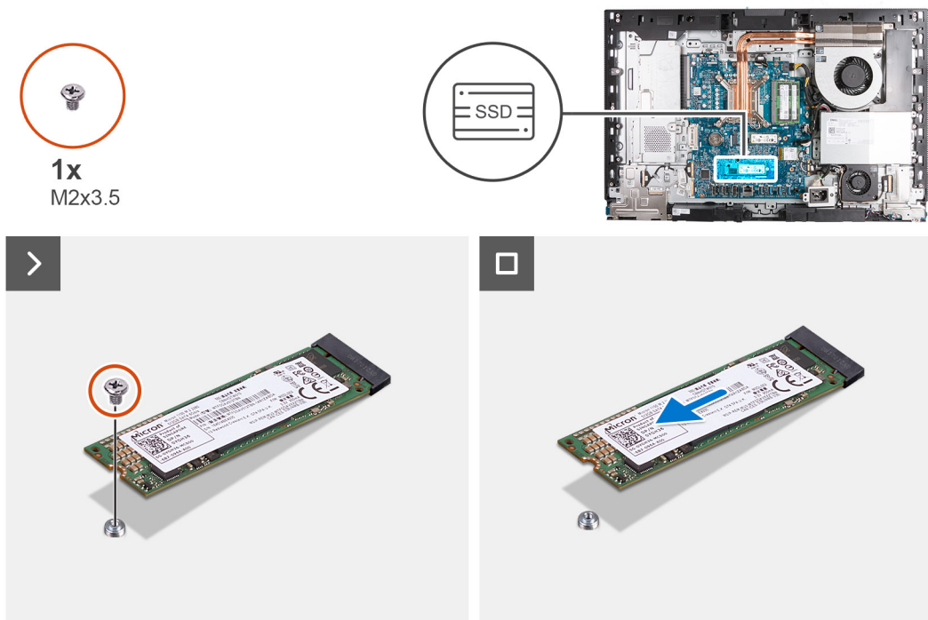
Ilustración 37. Extracción de la unidad de estado sólido M.2 2280 de la ranura M.2 1
