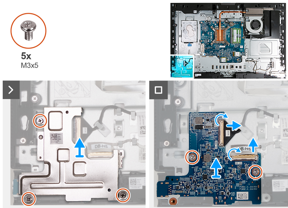
Ilustración 119. Extracción de la placa de I/O y del botón de encendido
