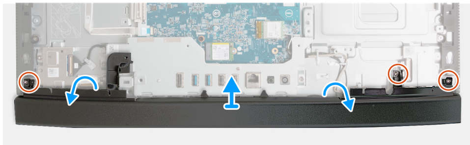
Ilustración 99. Extracción de la cubierta inferior
