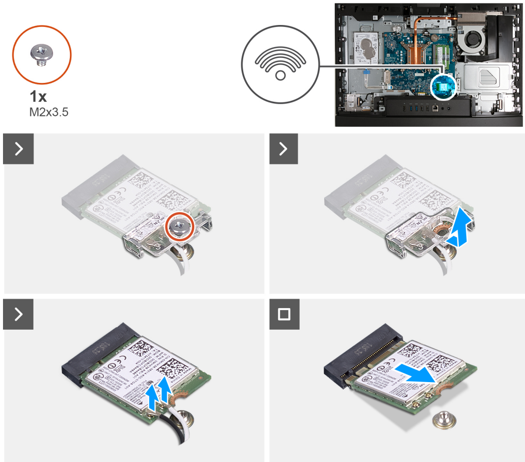
Ilustración 88. Extracción de la tarjeta inalámbrica
