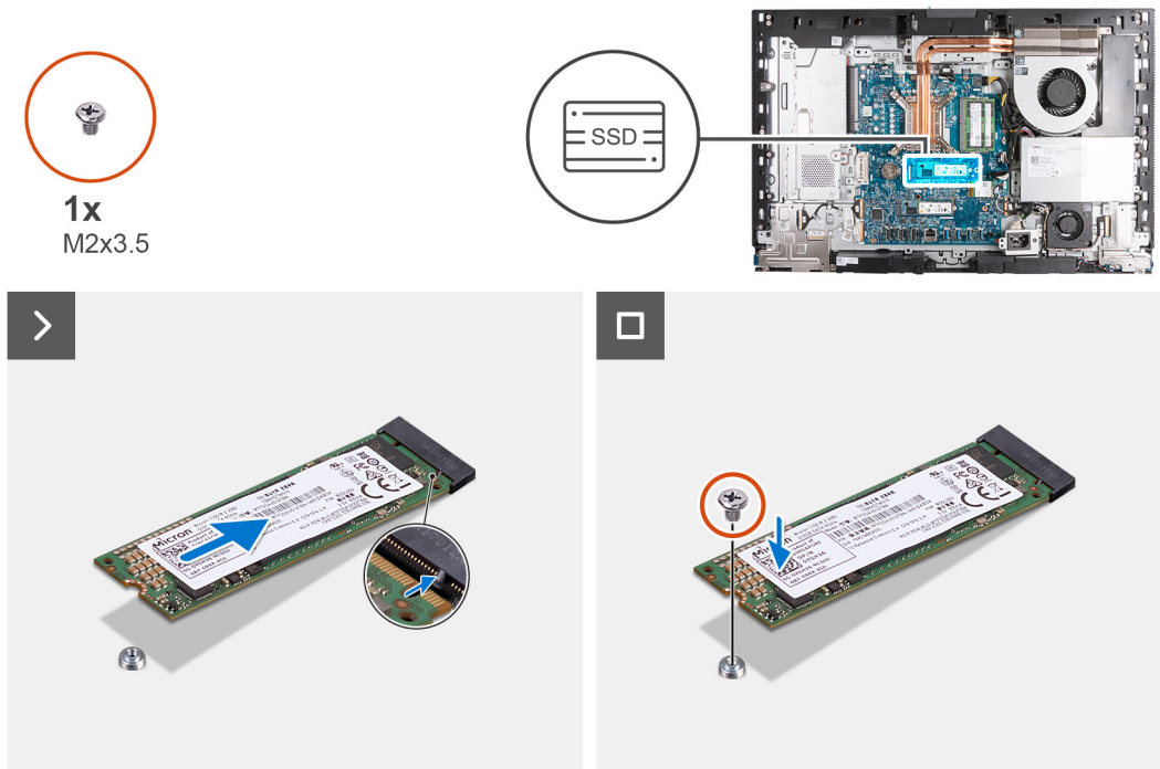
Ilustración 33. Instalación de la unidad de estado sólido M.2 2280 en la ranura M.2 0
