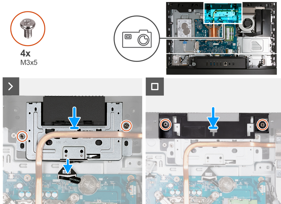
Ilustración 102. Instalación del ensamblaje de la cámara retráctil
