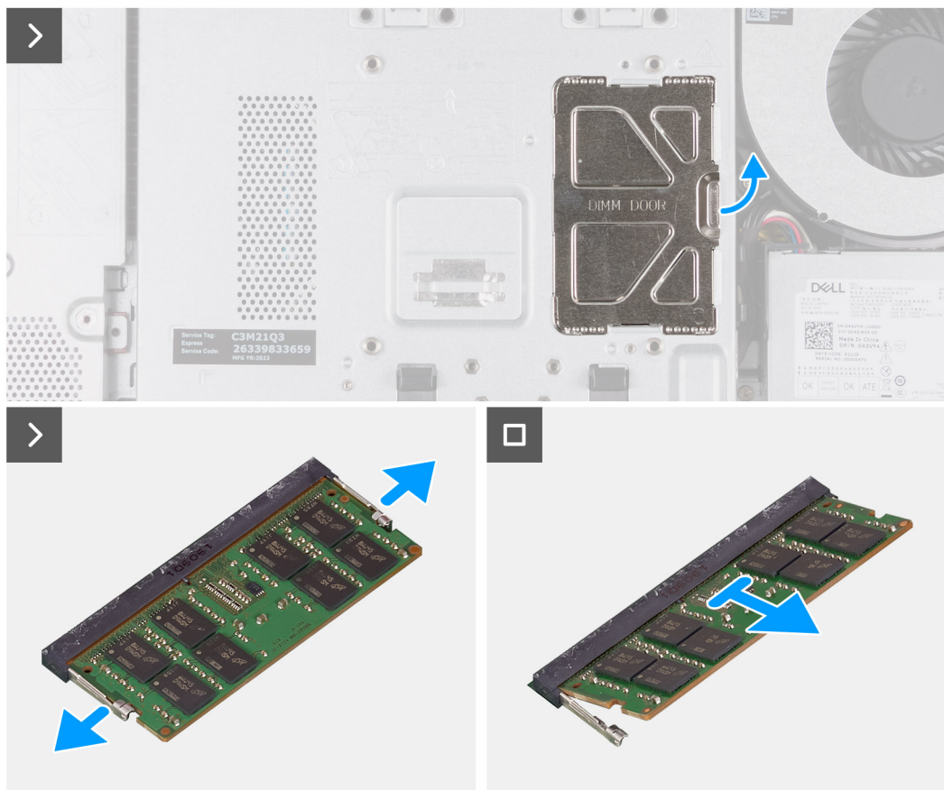
Ilustración 24. Extracción de la memoria
