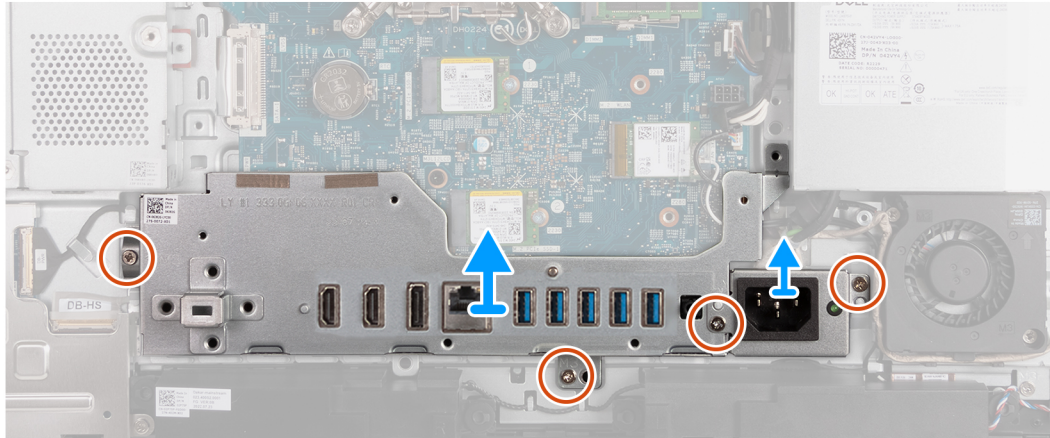
Ilustración 58. Extracción del soporte de I/O
