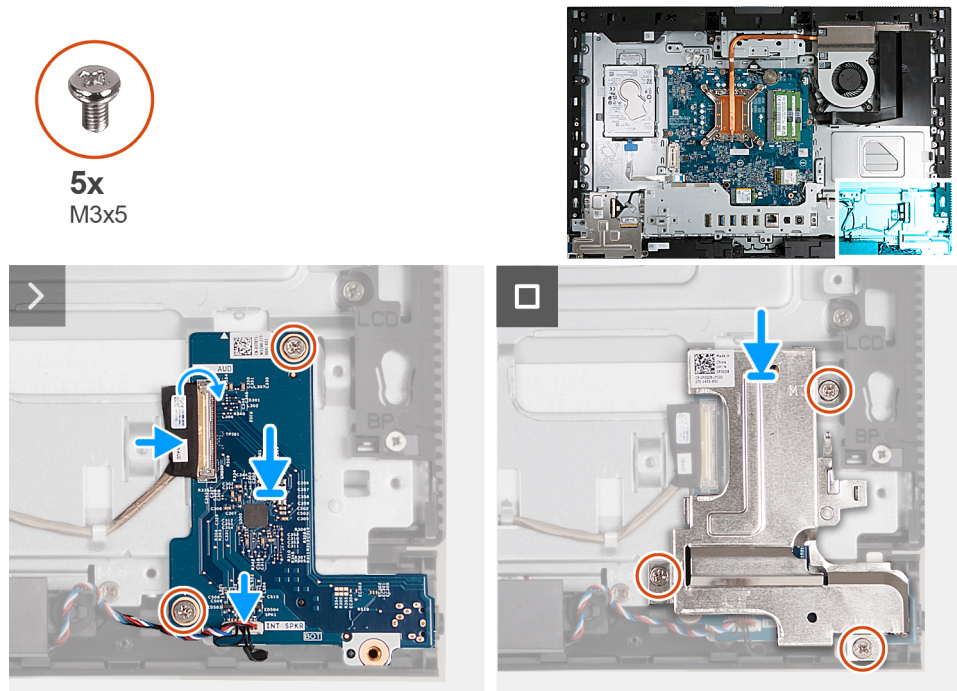
Ilustración 122. Instalación de la placa de audio
