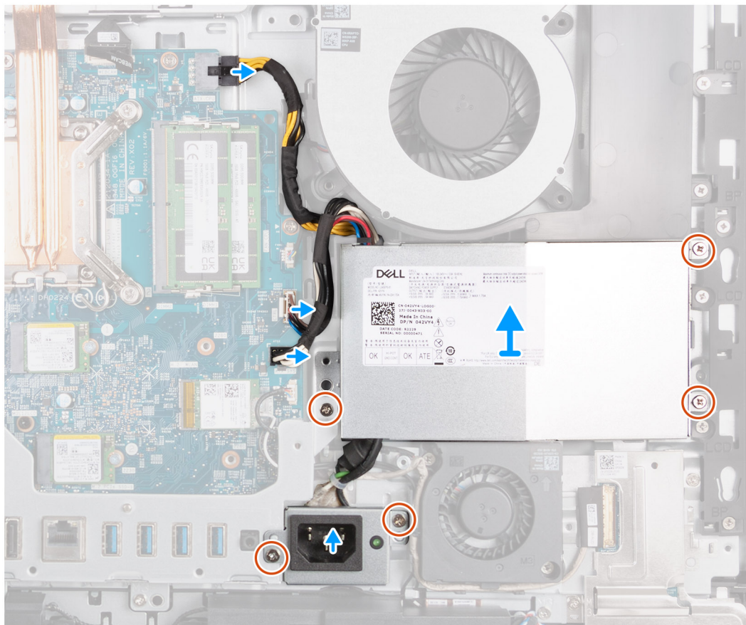
Ilustración 50. Extracción de la fuente de alimentación
