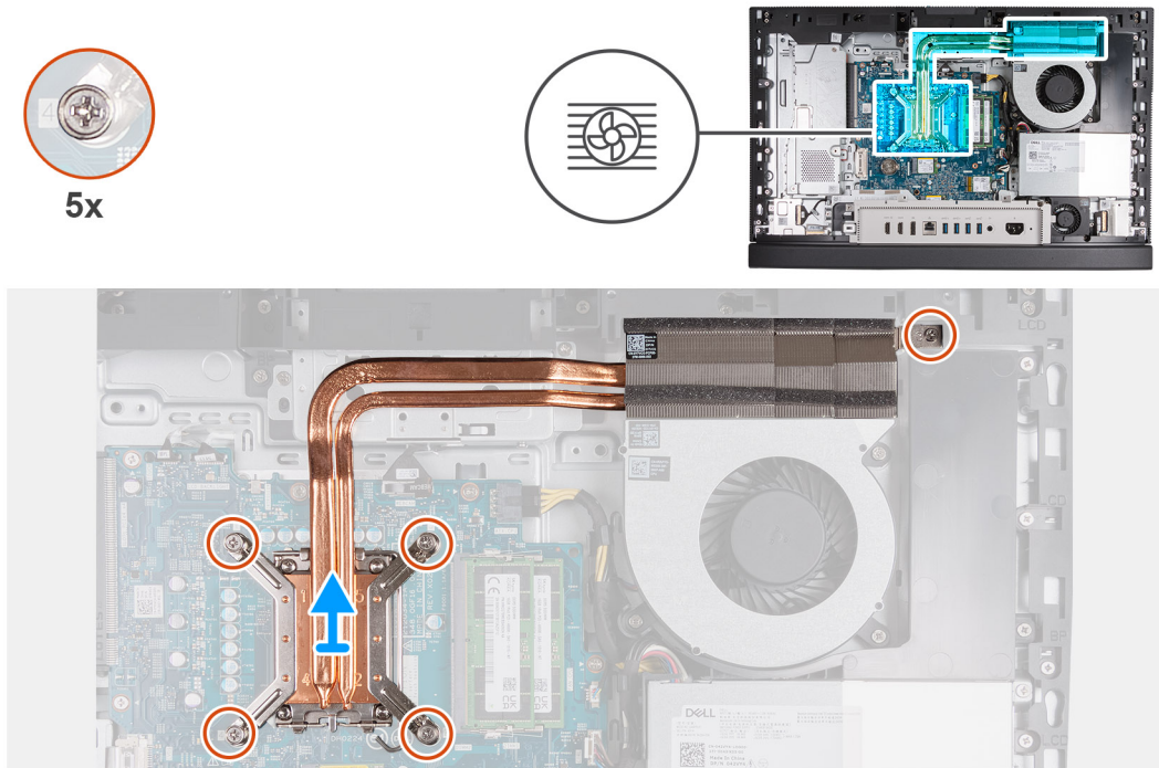
Ilustración 62. Extracción del disipador de calor
