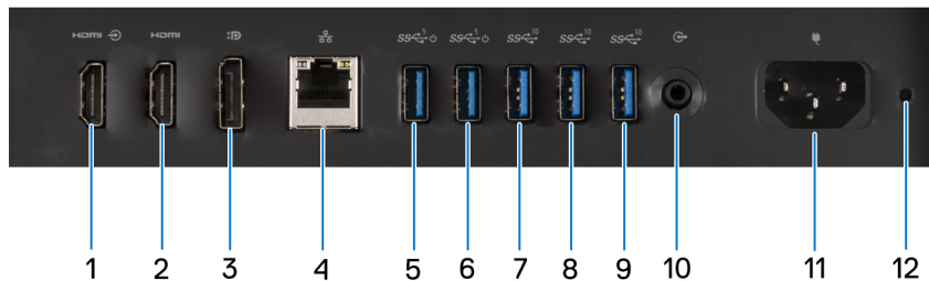
Ilustración 8. Vista del panel posterior de OptiPlex All-in-One 7420 con un procesador de alto rendimiento
