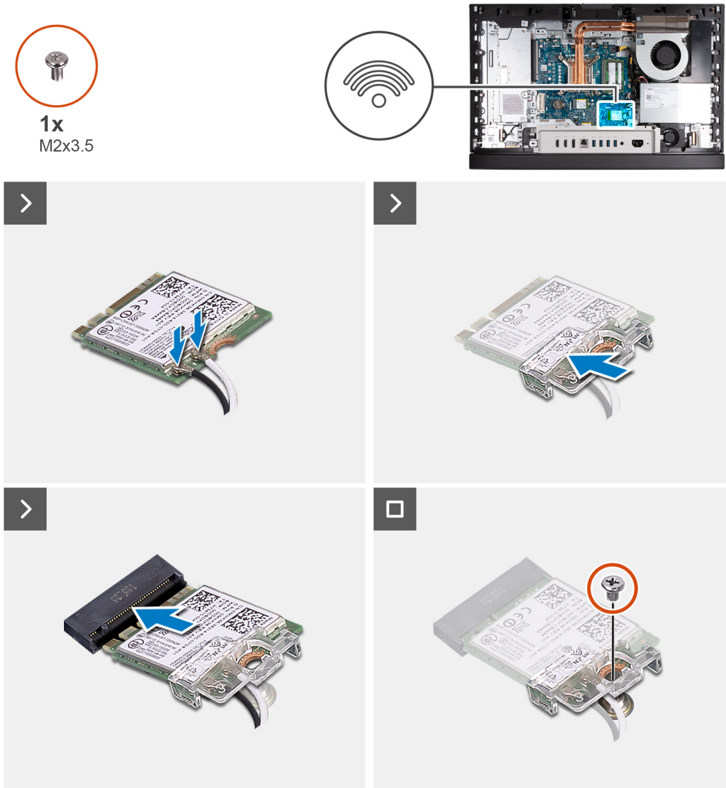
Ilustración 29. Instalación de la tarjeta inalámbrica
