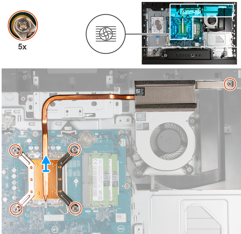
Ilustración 109. Extracción del disipador de calor
