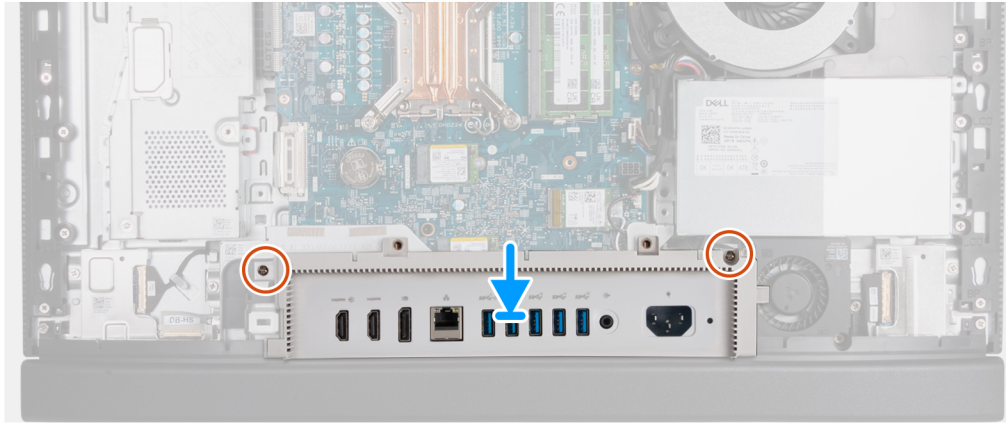
Ilustración 43. Instalación de la cubierta de I/O
