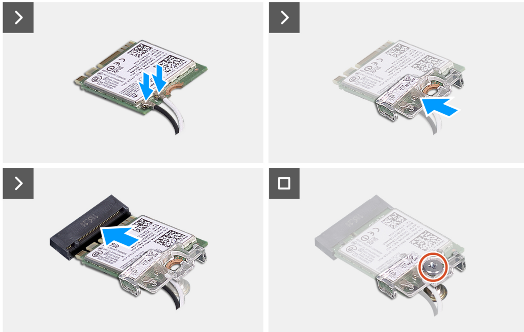
Ilustración 89. Instalación de la tarjeta inalámbrica
