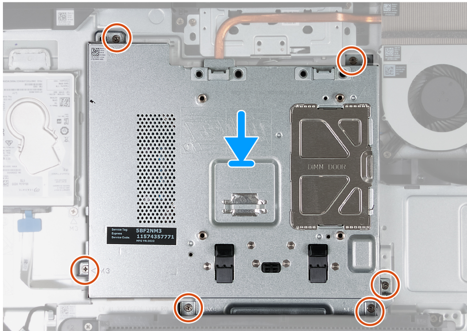
Ilustración 27. Instalación del protector de la tarjeta madre
