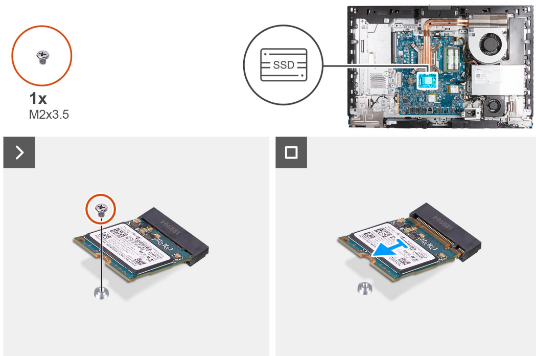
Ilustración 30. Extracción de la unidad de estado sólido M.2 2230 de la ranura M.2 0
