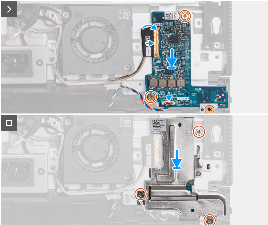
Ilustración 75. Instalación de la placa de audio
