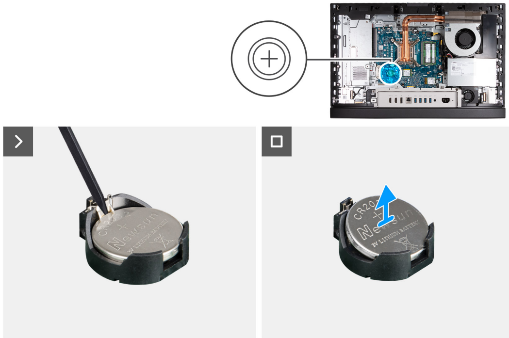
Ilustración 40. Extracción de la batería de tipo botón
