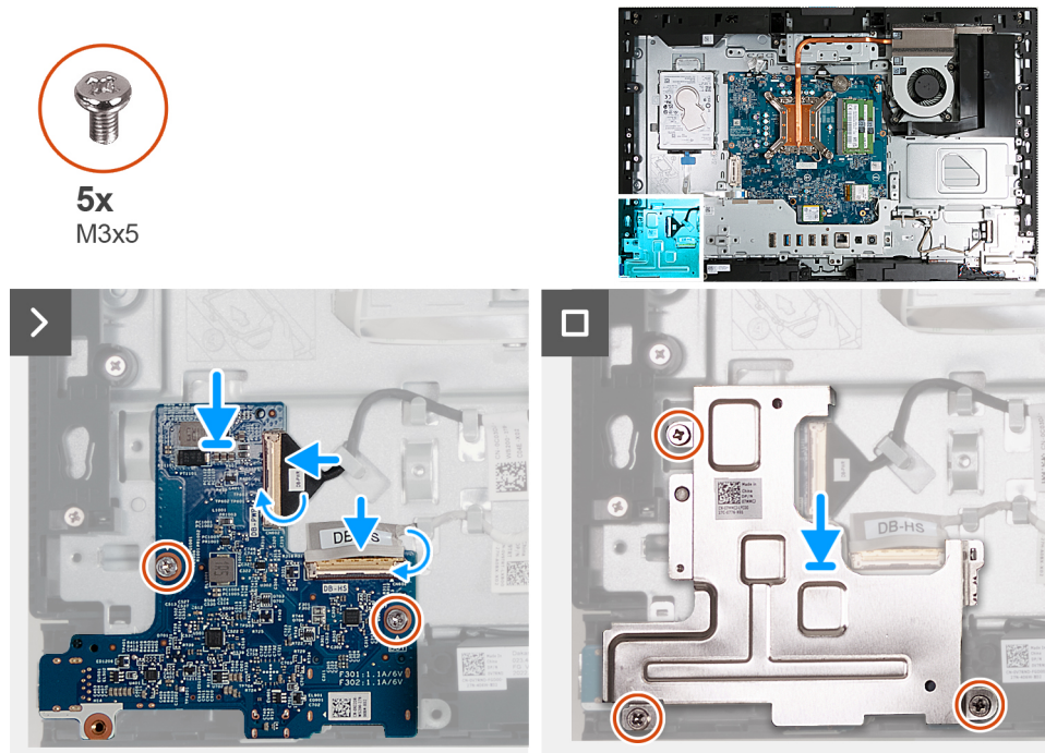
Ilustración 120. Instalación de la placa de I/O y del botón de encendido
