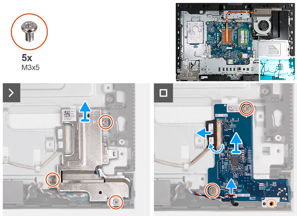
Ilustración 121. Extracción de la placa de audio
