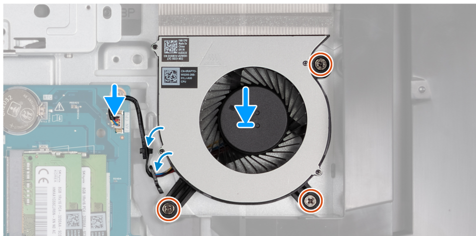
Ilustración 104. Instalación del ventilador
