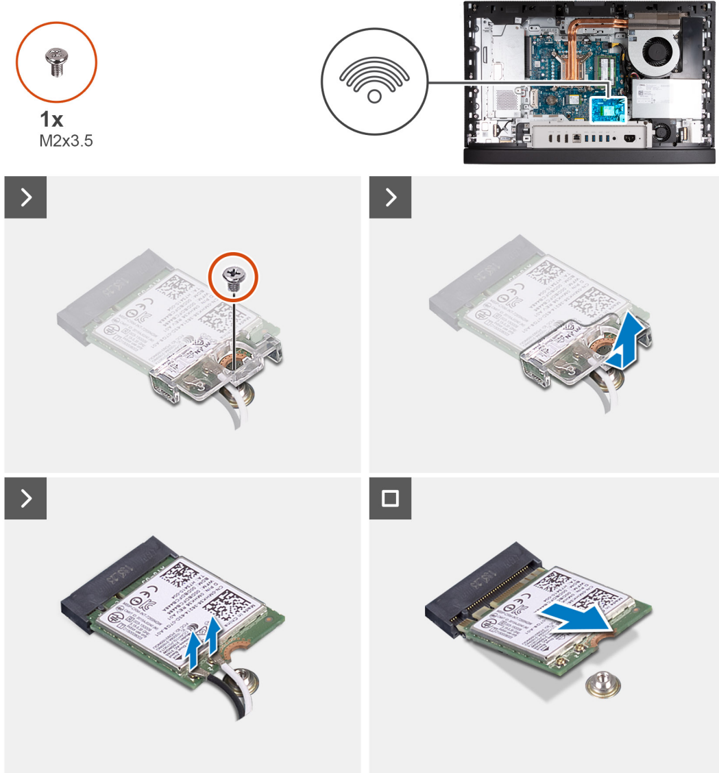
Ilustración 28. Extracción de la tarjeta inalámbrica
