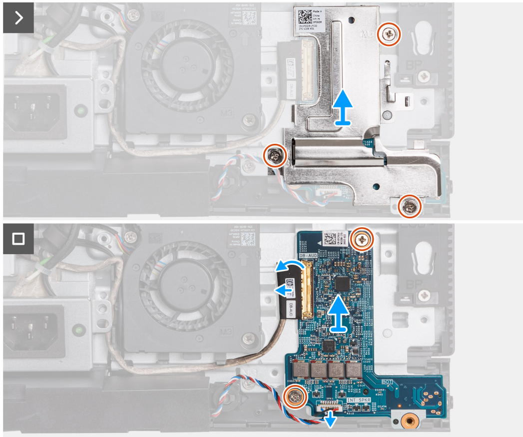
Ilustración 74. Extracción de la placa de audio
