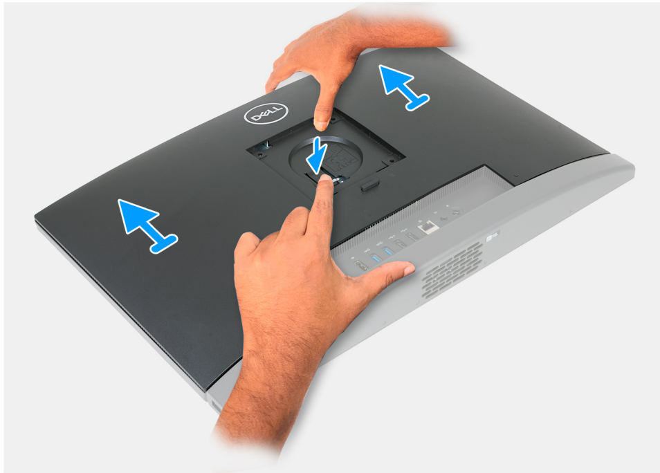
Ilustración 82. Extracción de la cubierta posterior
