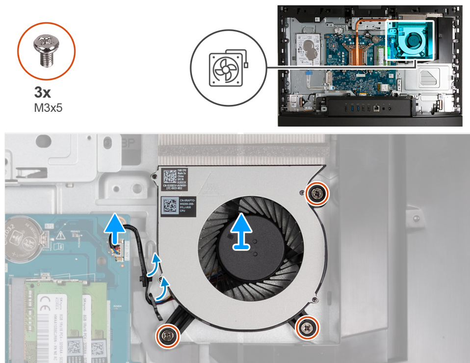
Ilustración 103. Extracción del ventilador
