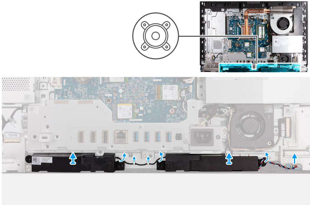
Ilustración 60. Extracción de los parlantes
