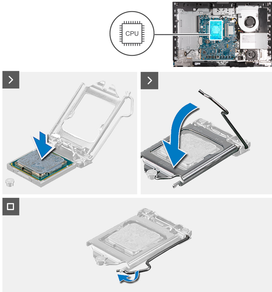
Ilustración 65. Instalación del procesador
