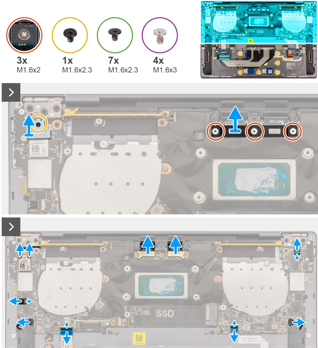
Figura 37. Rimozione della scheda di sistema
