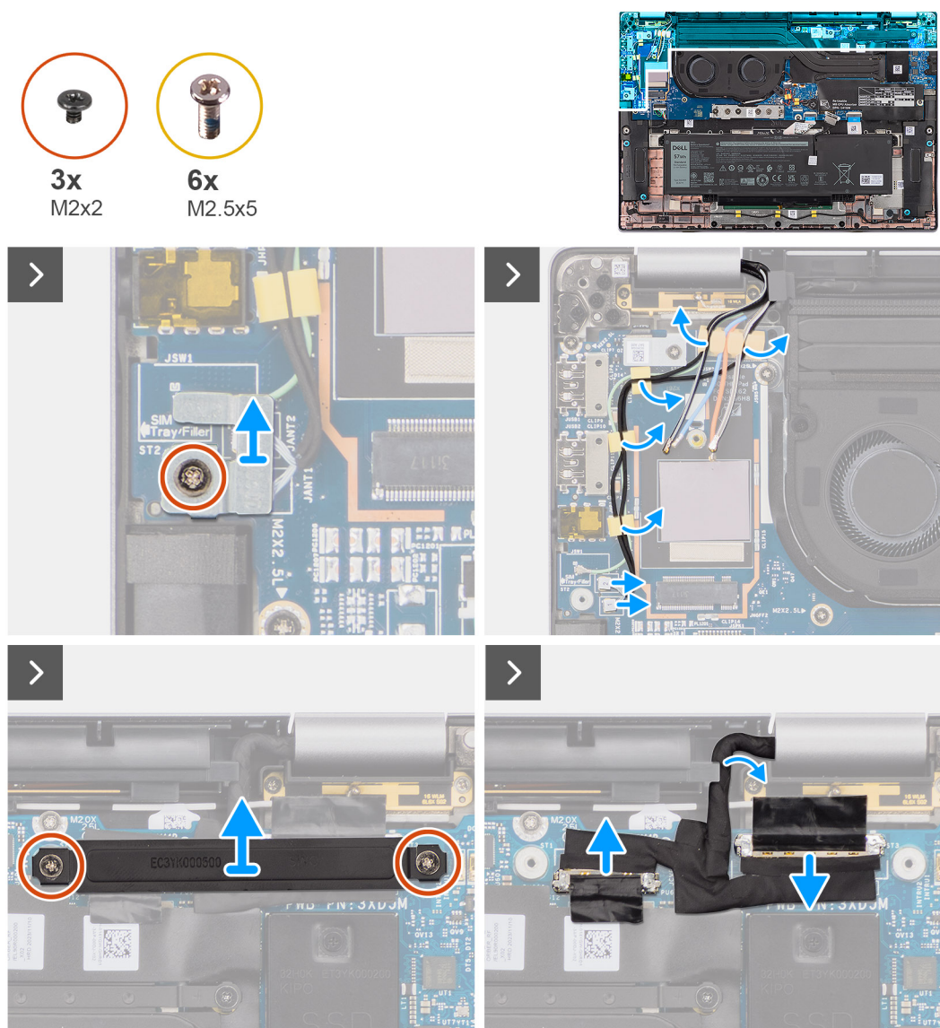
Figura 38. Rimozione del gruppo del display
