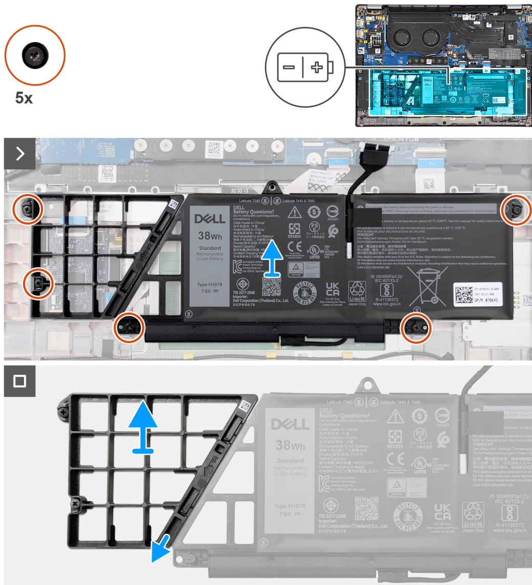
Figura 29. Rimozione della batteria a 2 celle
