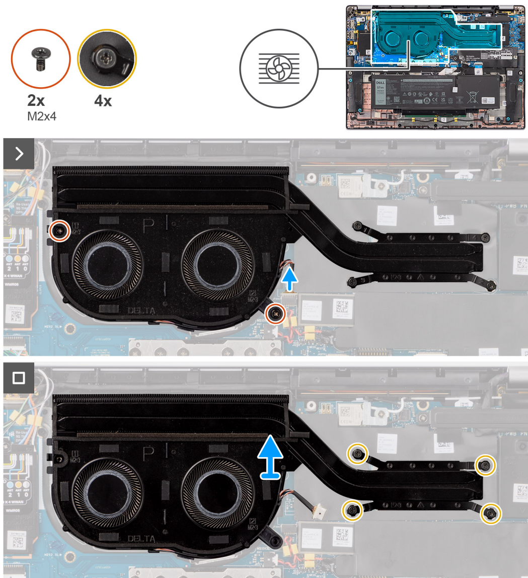
Figura 36. Rimozione del gruppo dissipatore di calore e ventola
