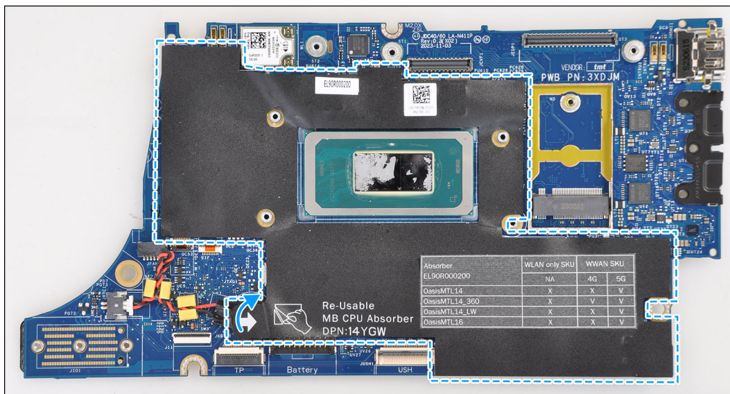
Figura 52. Ammortizzatore della CPU
