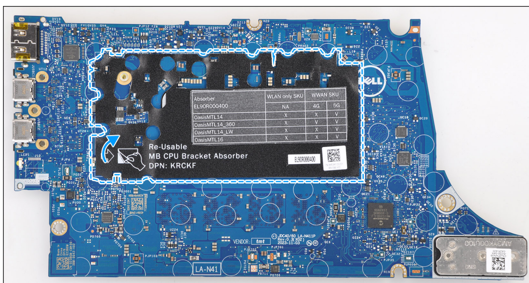
Figura 53. Ammortizzatore della staffa della CPU
