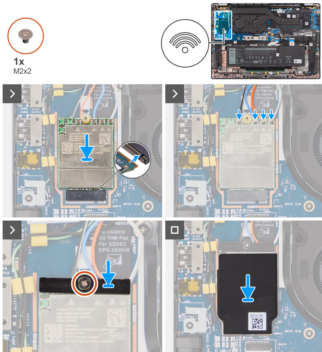
Figura 23. Installazione della scheda WWAN 5G
