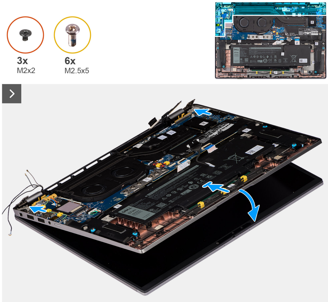
Figura 42. Installazione del gruppo del display
