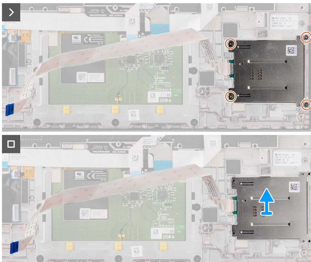
Figura 46. Rimozione del lettore di smart card
