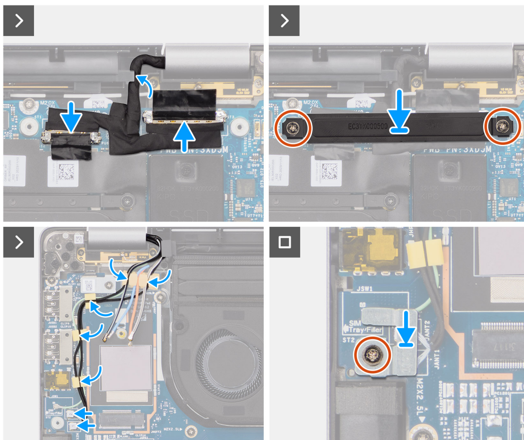
Figura 44. Installazione del gruppo del display
