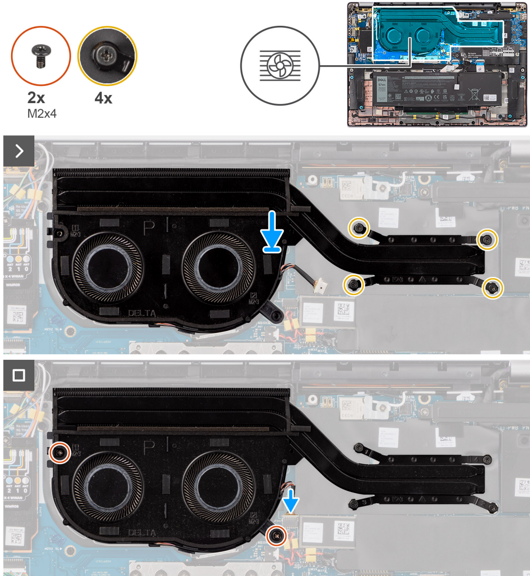
Figura 37. Installazione del gruppo dissipatore di calore e ventola
