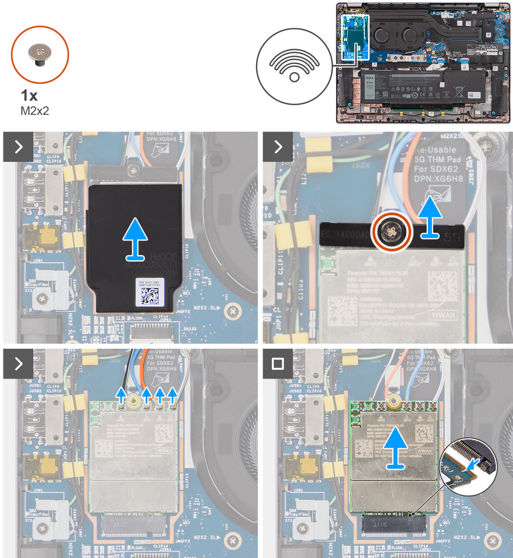
Figura 22. Rimozione della scheda WWAN 5G
