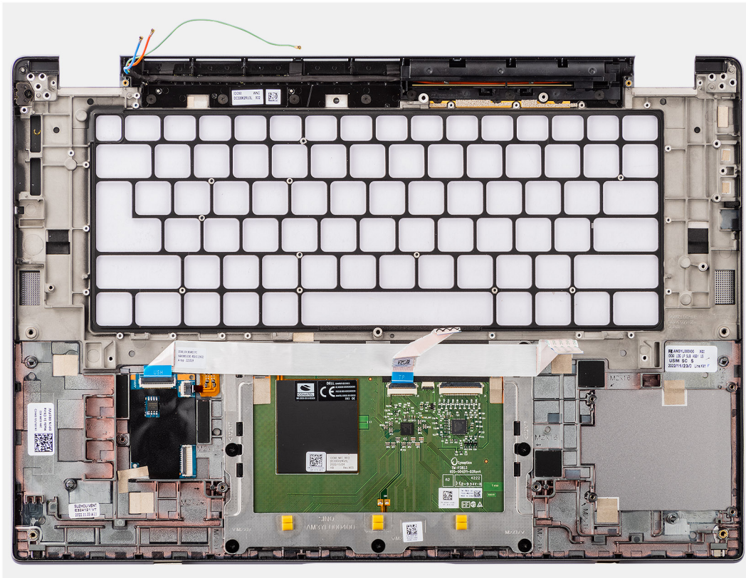
Figura 69. Rimozione del gruppo del poggiapolsi
