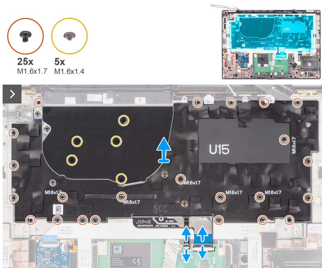
Figura 65. Rimozione della tastiera
