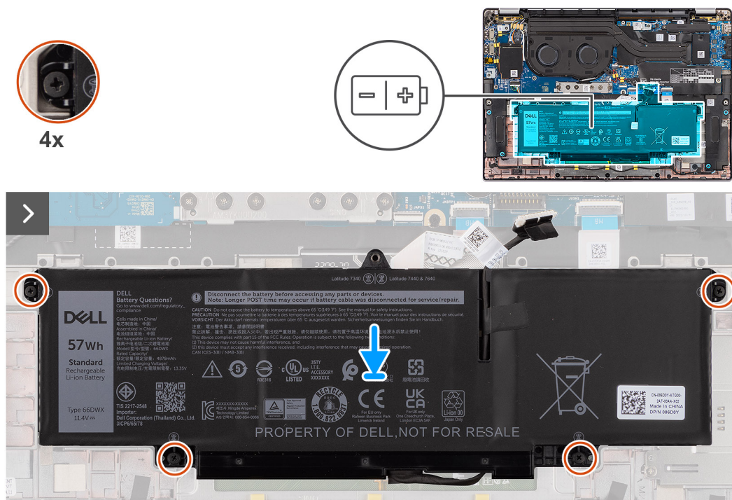
Figura 33. Installazione della batteria a 3 celle
