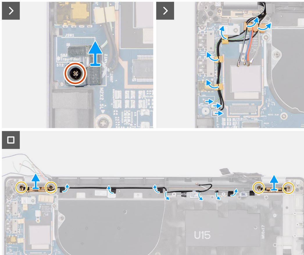
Figura 57. Rimozione del modulo dell'antenna WLAN
