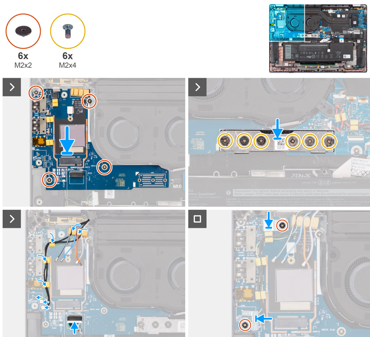
Figura 62. Installazione della scheda figlia di I/O
