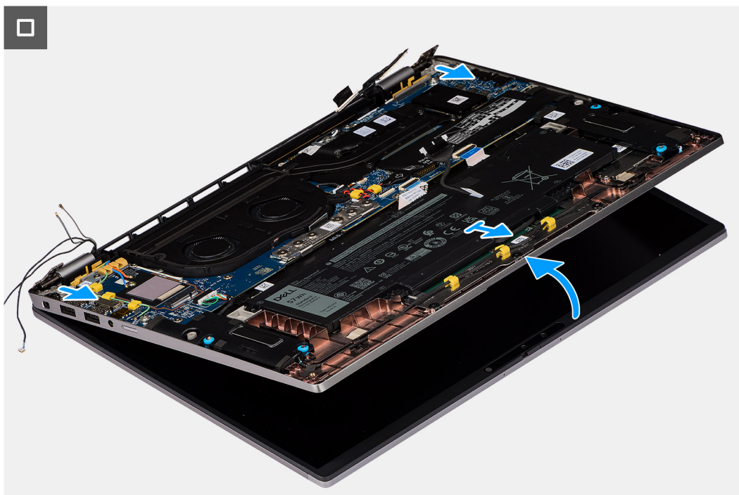
Figura 40. Rimozione del gruppo del display
