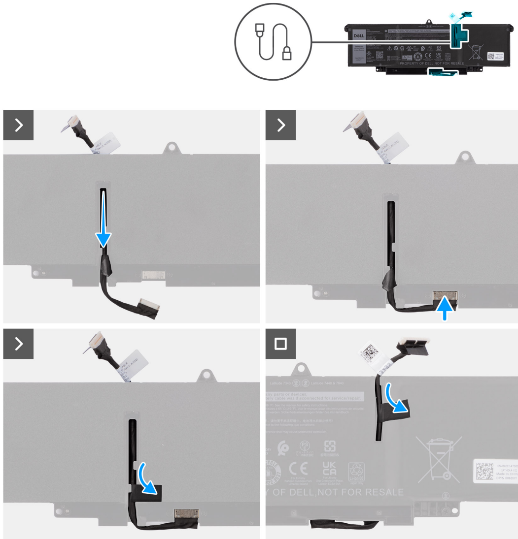
Figura 35. Installazione del cavo della batteria
