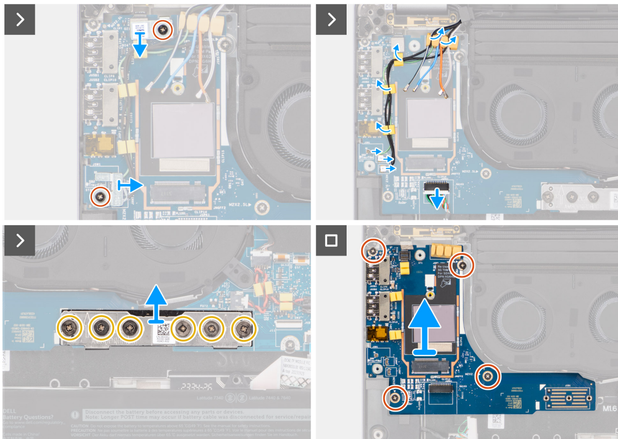
Figura 59. Rimozione della scheda figlia di I/O
