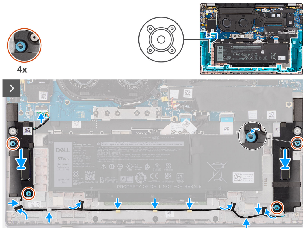
Figura 26. Installazione degli altoparlanti
