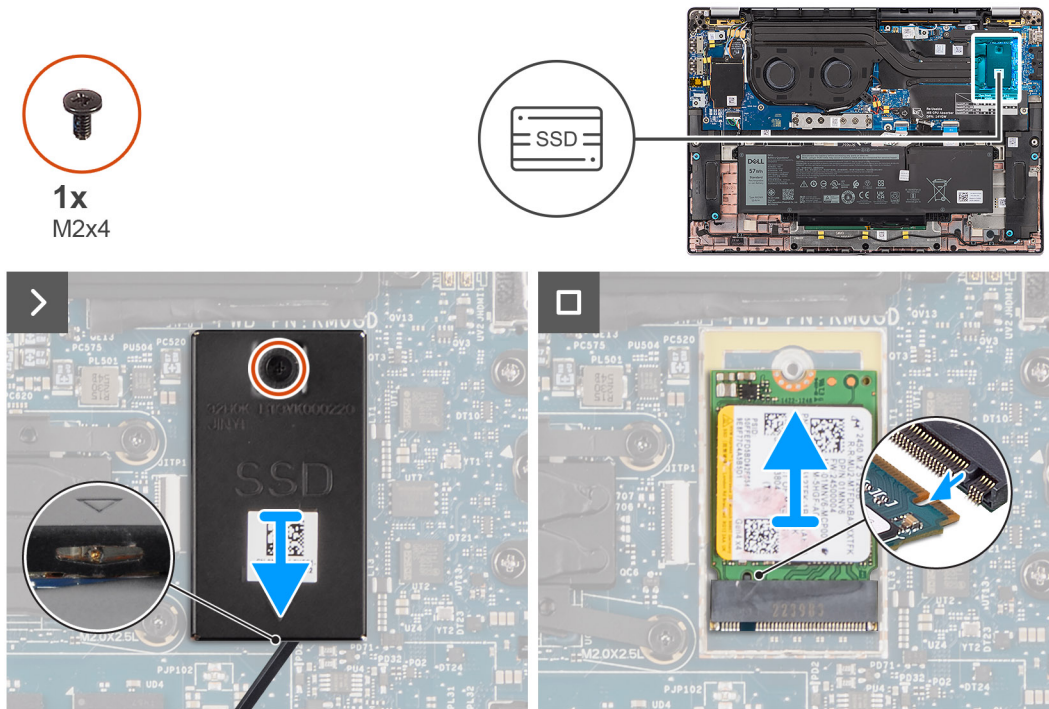
Figura 18. Rimozione dell'unità SSD M.2 2230
