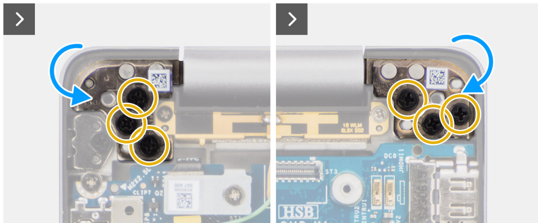
Figura 43. Installazione del gruppo del display
