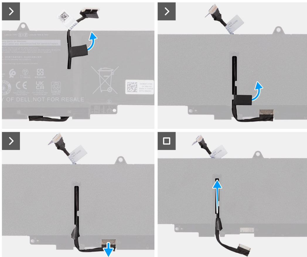
Figura 34. Rimozione del cavo della batteria
