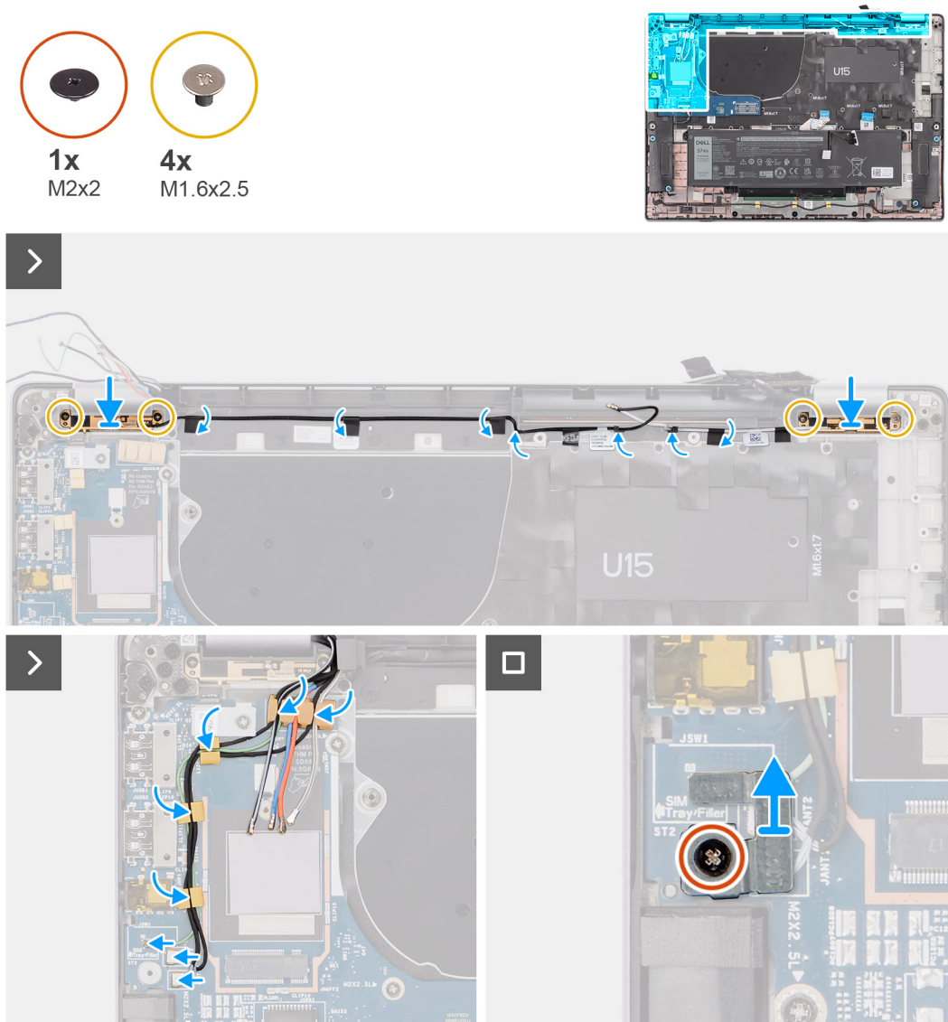
Figura 58. Installazione del modulo dell'antenna WLAN
