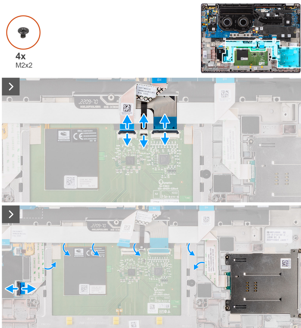
Figura 45. Rimozione del lettore di smart card
