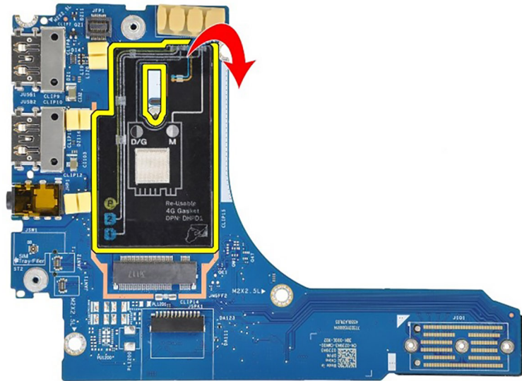
Figura 60. Configurazione Latitude 7650 4G WWAN (adesivo a guarnizione)
