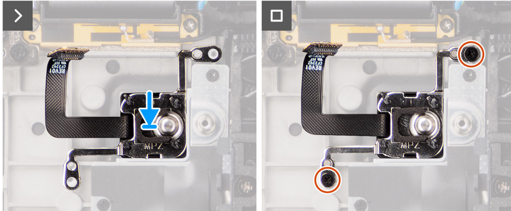
Figura 64. Installazione del pulsante di accensione con lettore di impronte digitali opzionale
