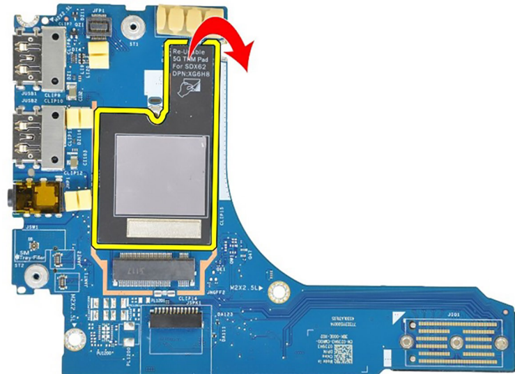
Figura 61. Configurazione Latitude 7650 5G WWAN (adesivo cuscinetto termico)
