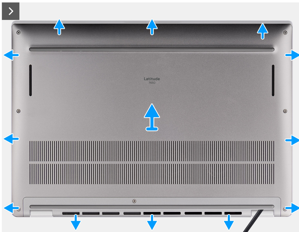
Figura 13. Rimozione del coperchio della base
