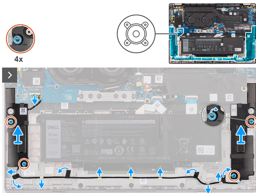
Figura 25. Rimozione degli altoparlanti
