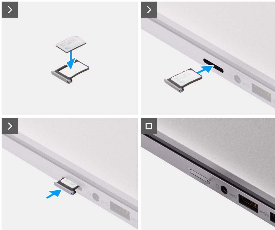
Figura 11. Installazione del vassoio della scheda SIM
