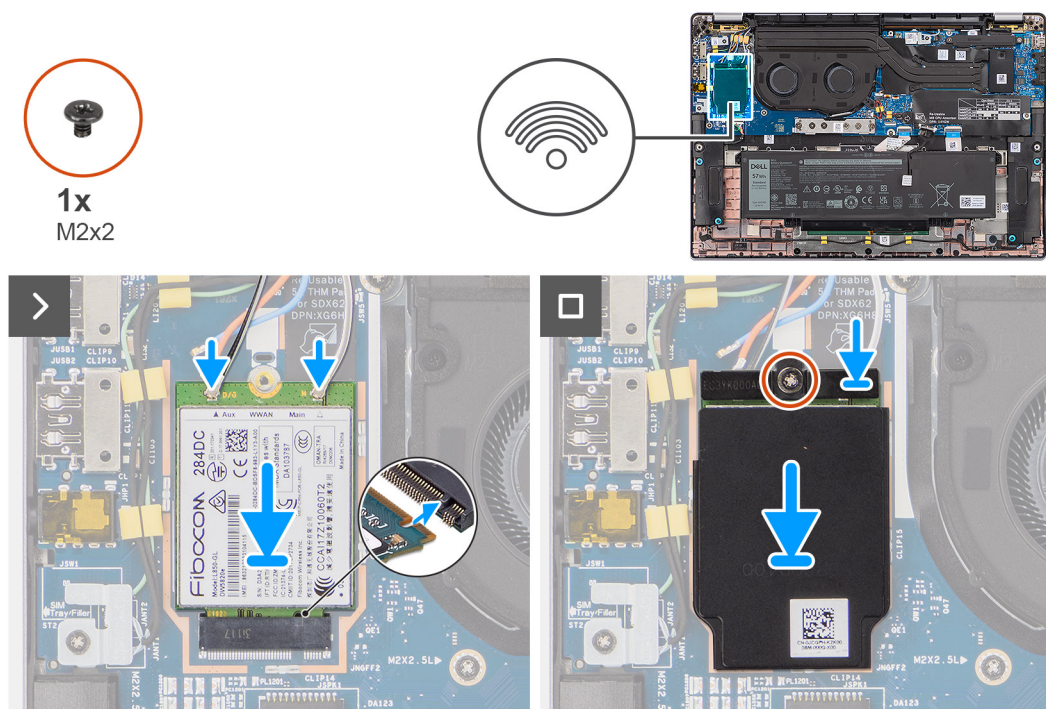
Figura 21. Installazione della scheda WWAN 4G
