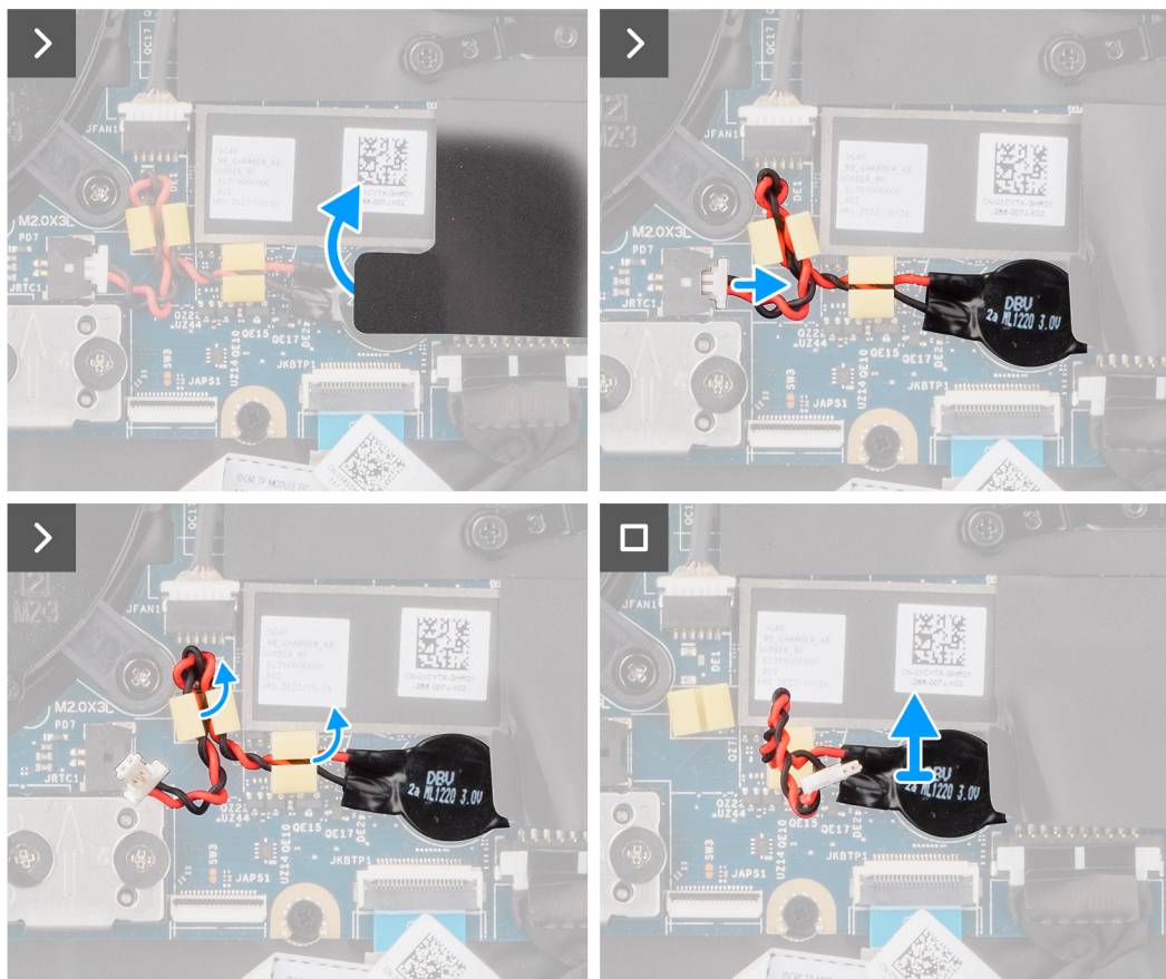
Figura 27. Rimozione della batteria a bottone
