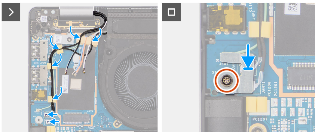
Figure 55. Installation de l'assemblage d'écran
