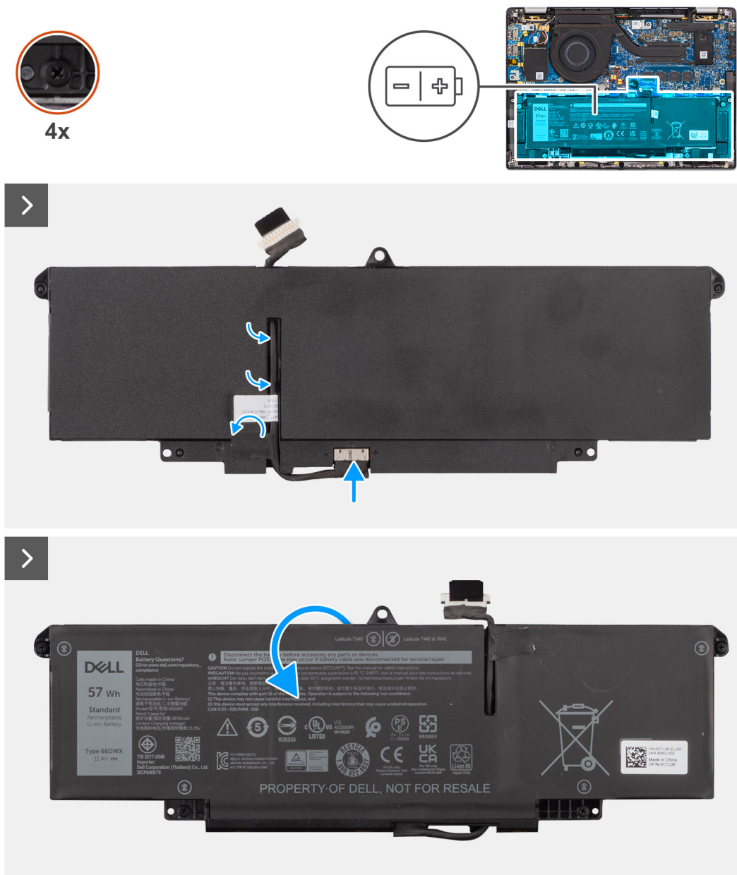
Figure 45. Installation du câble de la batterie
