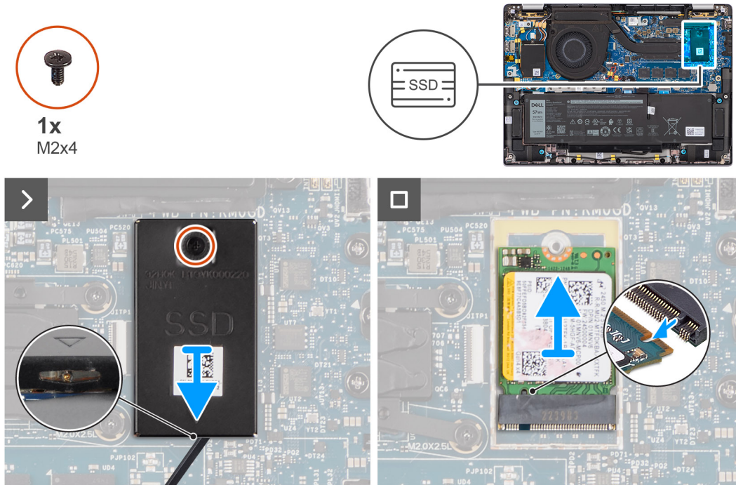
Figure 22. Retrait du disque SSD M.2 2230
