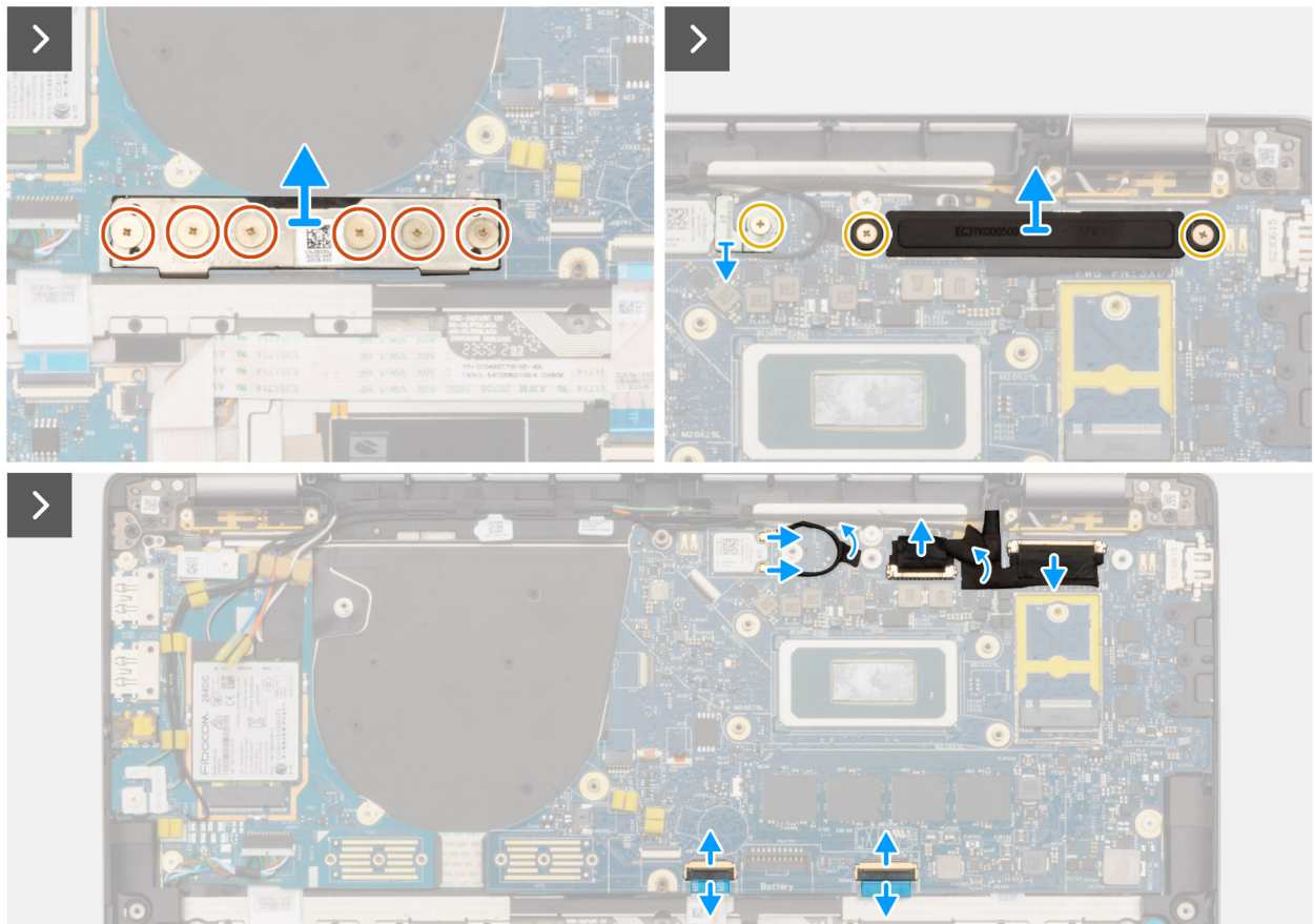
Figure 59. Retrait de la carte système
