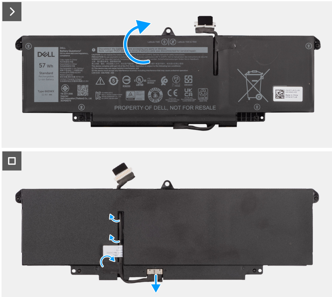
Figure 41. Retrait de la batterie à 3 cellules
