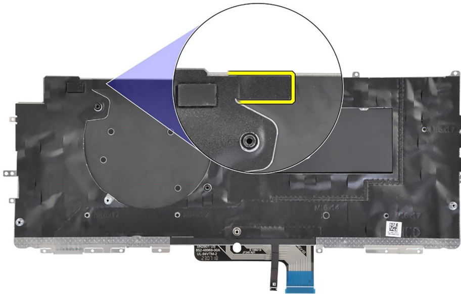
Figure 83. Installation du ruban en mylar du clavier
