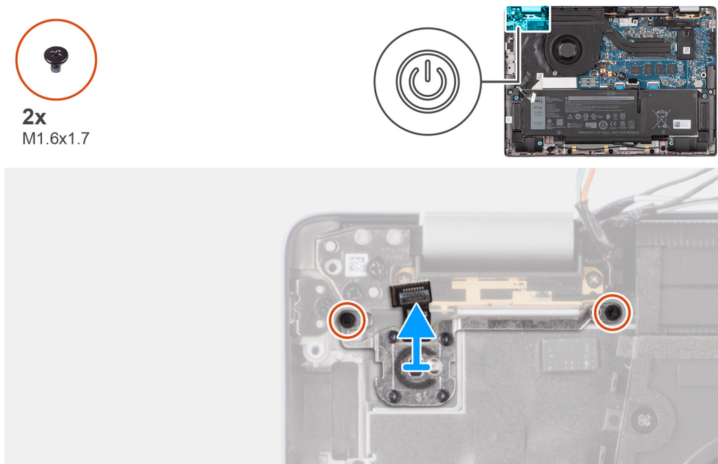
Figure 76. Retrait du bouton d'alimentation avec lecteur d'empreintes digitales (en option)
