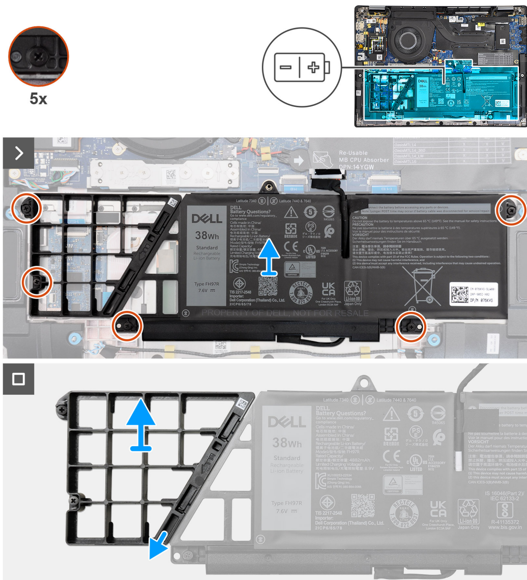
Figure 37. Retrait de la batterie à 2 cellules
