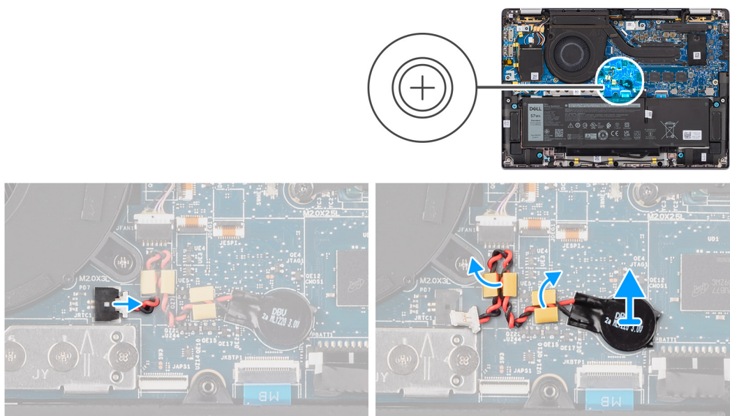
Figure 35. Retrait de la pile bouton
