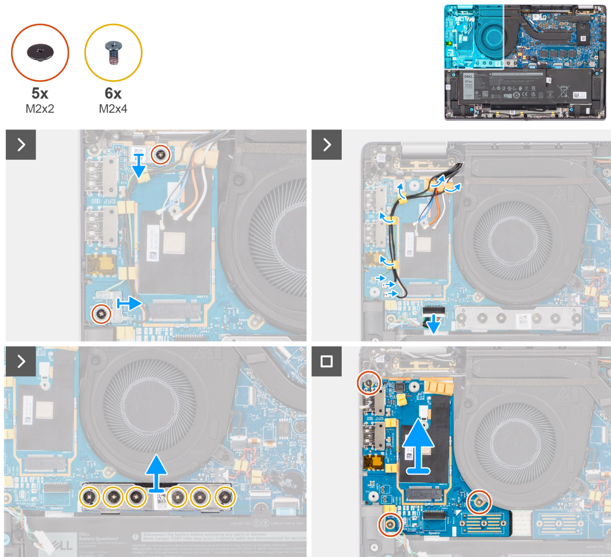
Figure 71. Retrait de la carte fille d'E/S
