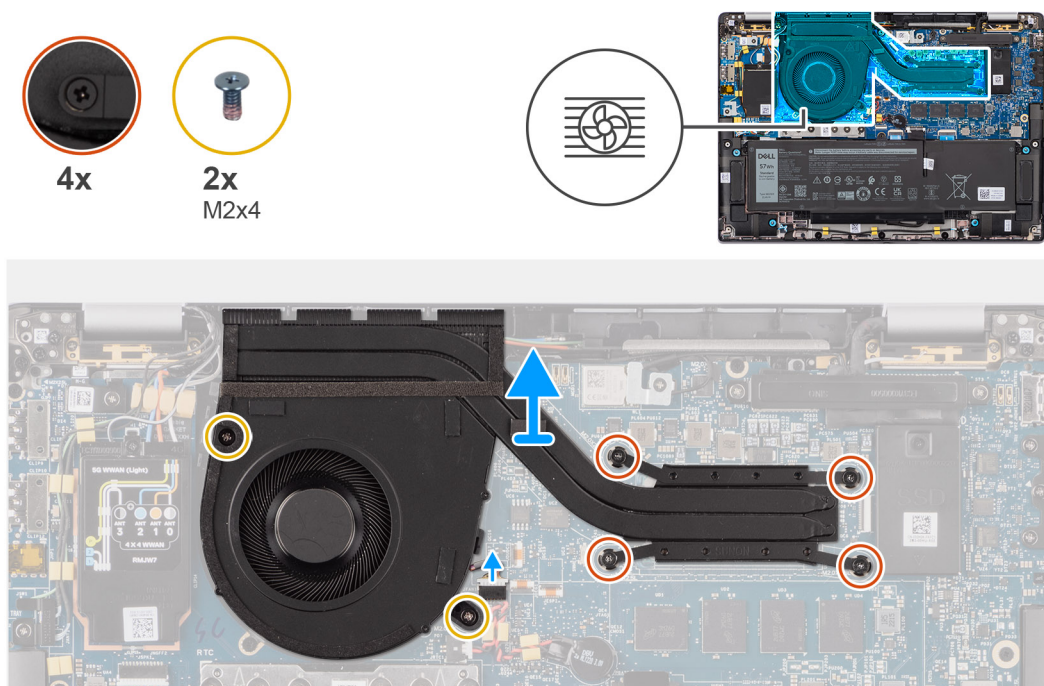
Figure 46. Retrait de l'assemblage du dissipateur de chaleur et des ventilateurs
