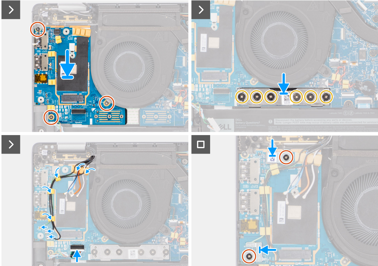
Figure 75. Installation de la carte fille d'E/S
