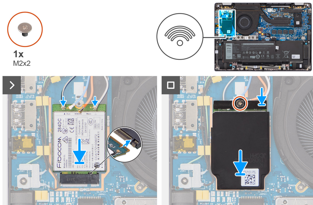
Figure 25. Installation de la carte WWAN 4G
