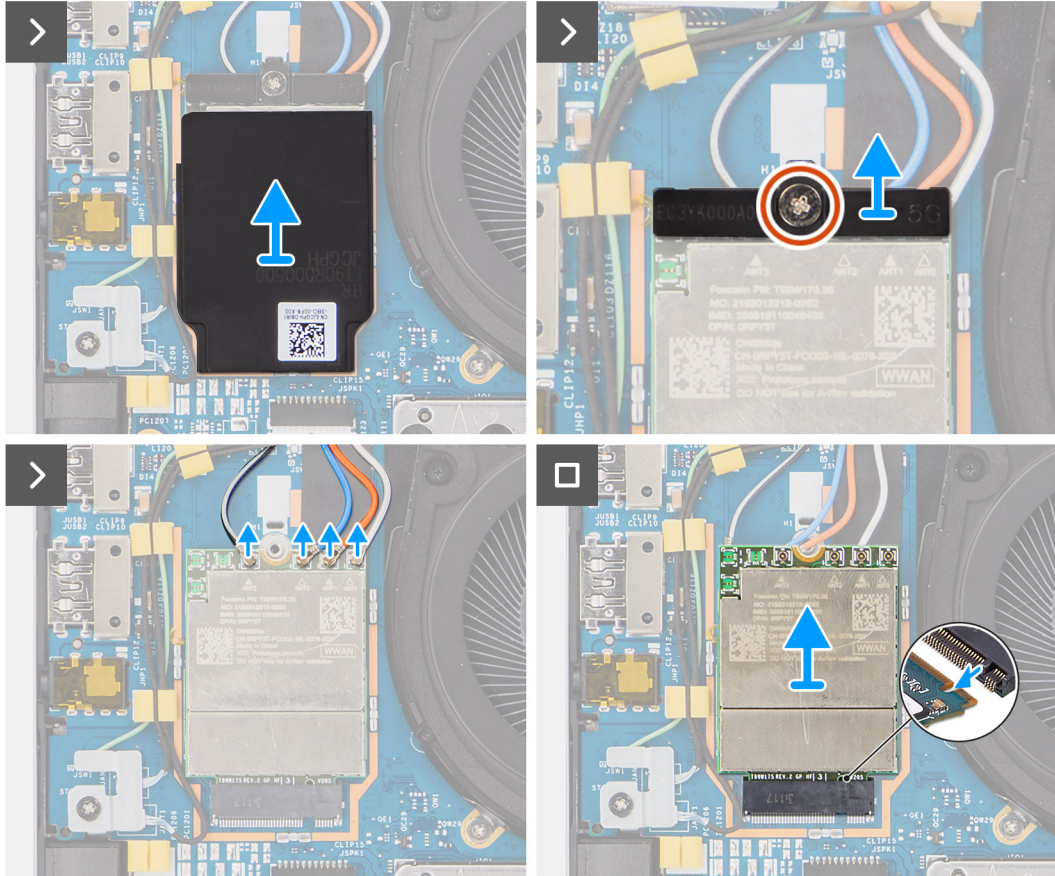
Figure 26. Retrait de la carte WWAN 5G
