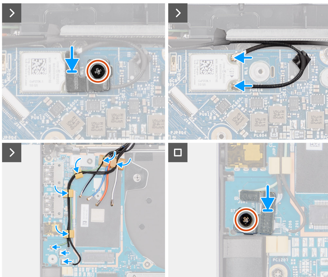
Figure 69. Installation du module d'antenne WLAN
