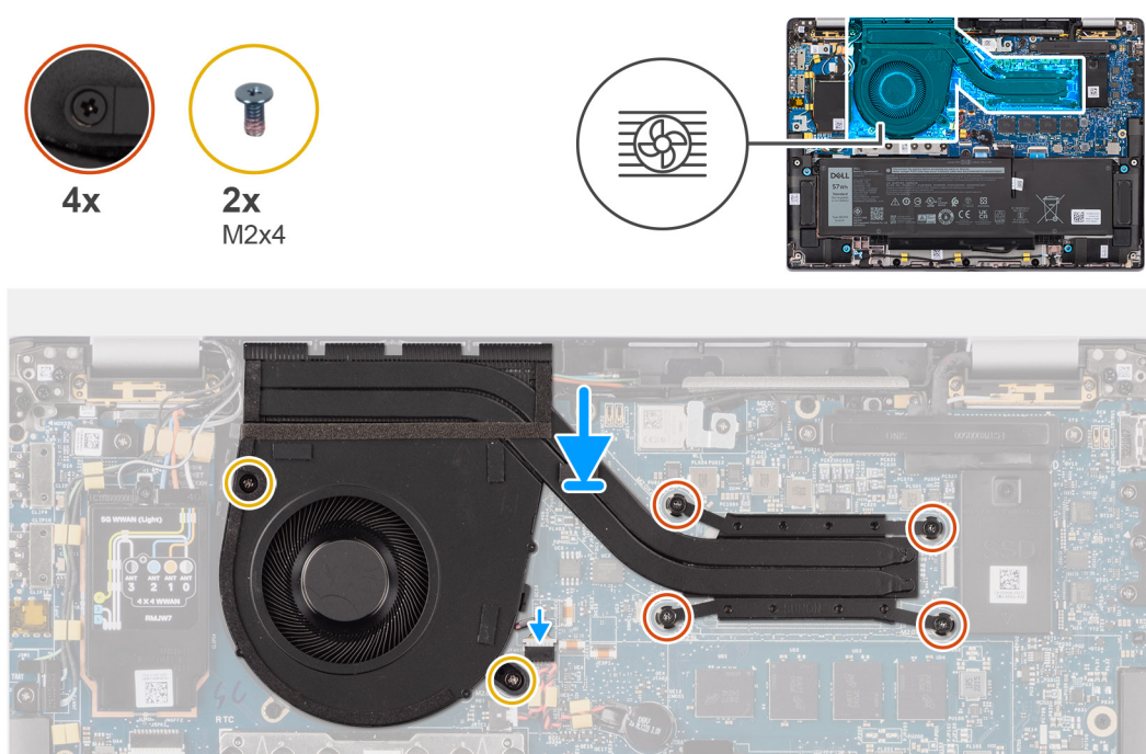
Figure 47. Installation de l'assemblage du dissipateur de chaleur et du ventilateur
