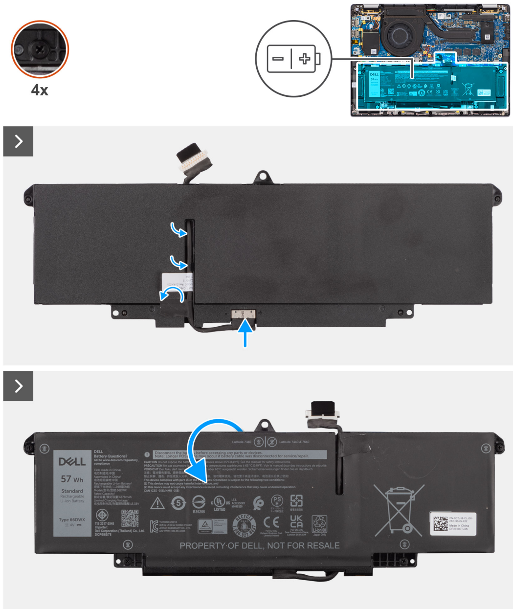
Figure 42. Installation de la batterie à 3 cellules
