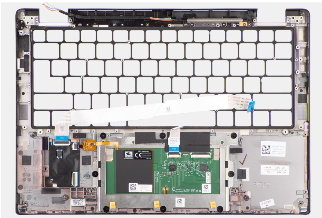
Figure 84. Retrait de l'assemblage du repose-poignets
