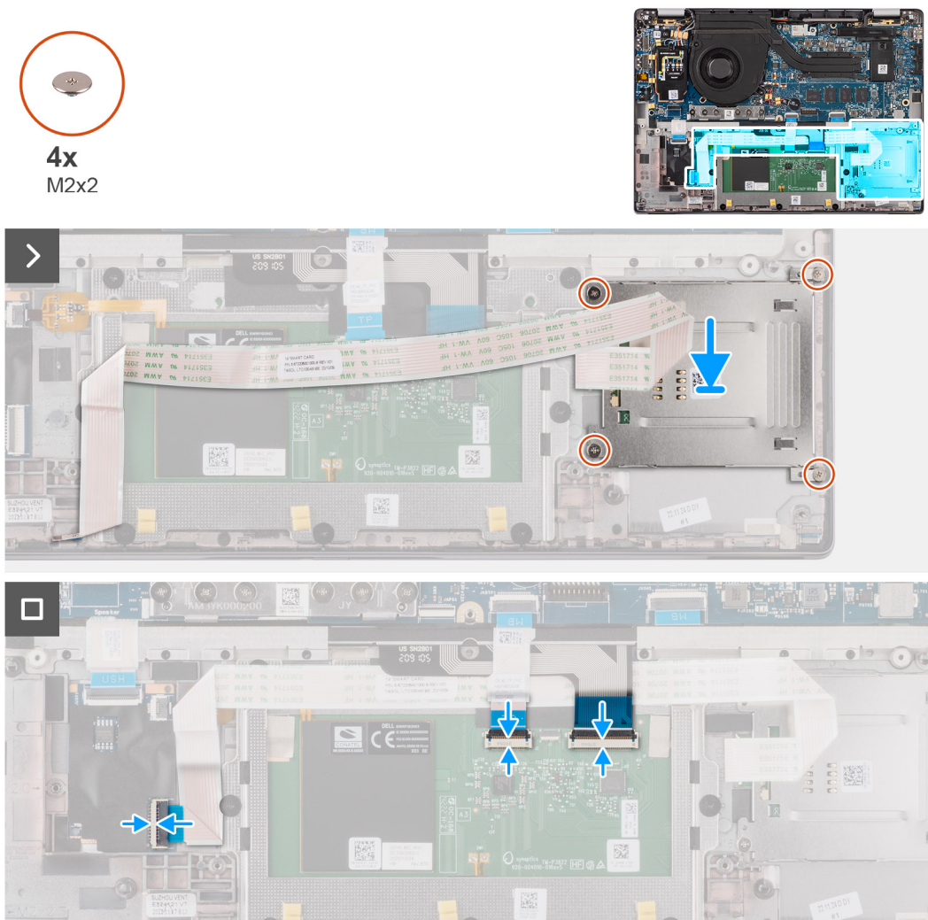
Figure 57. Installation du lecteur de carte à puce
