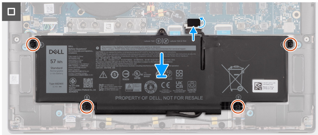
Figure 43. Installation de la batterie à 3 cellules
