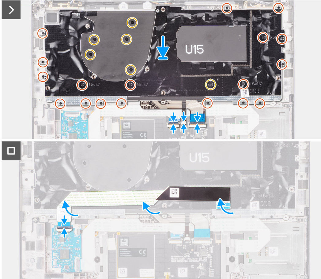
Figure 81. Installation du clavier
