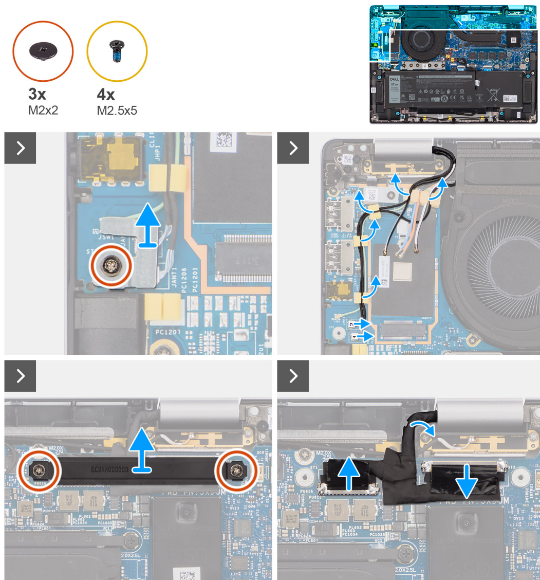
Figure 48. Retrait de l'assemblage d'écran
