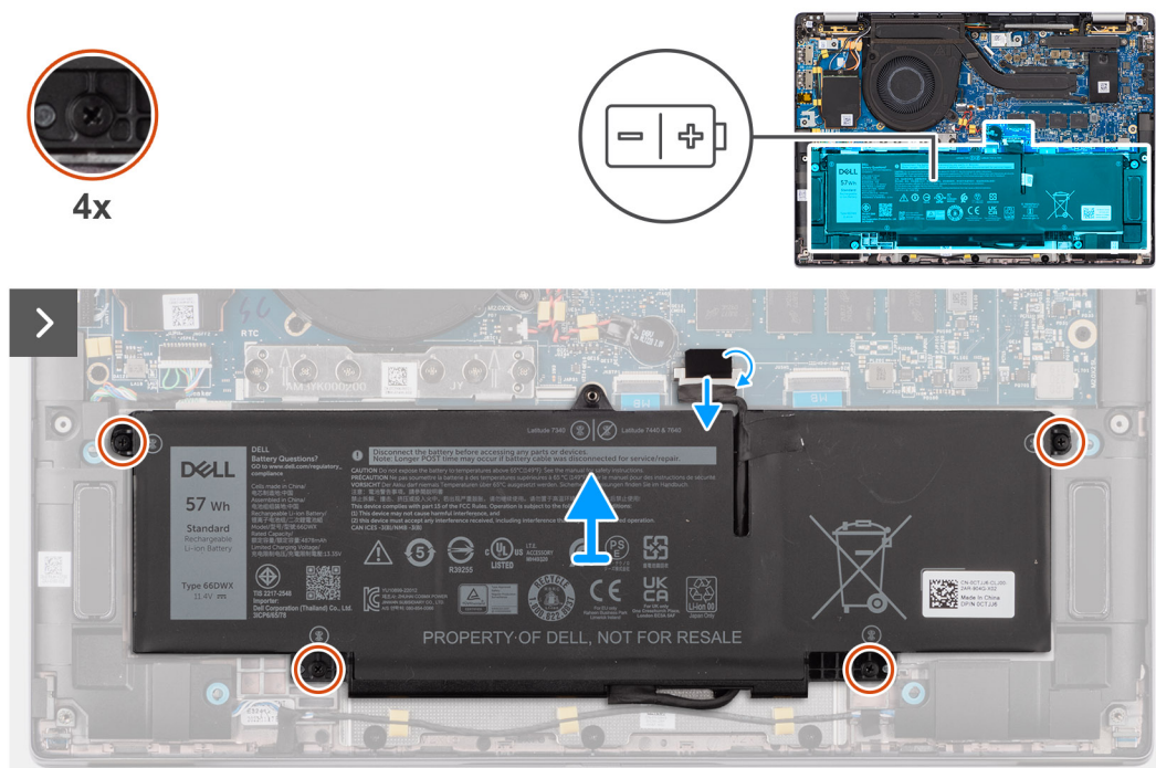
Figure 40. Retrait de la batterie à 3 cellules
