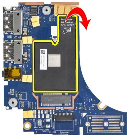
Figure 73. Latitude 7450 2-en-1, configuration WWAN 4G (autocollant de joint)
