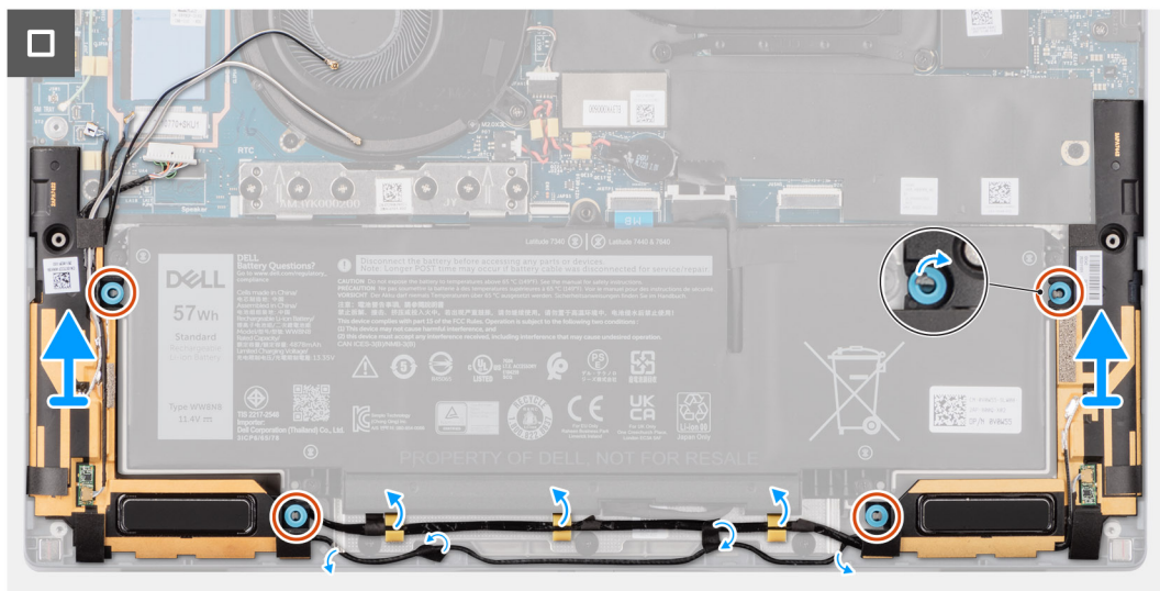
Figure 30. Retrait des haut-parleurs pour l'ultralight
