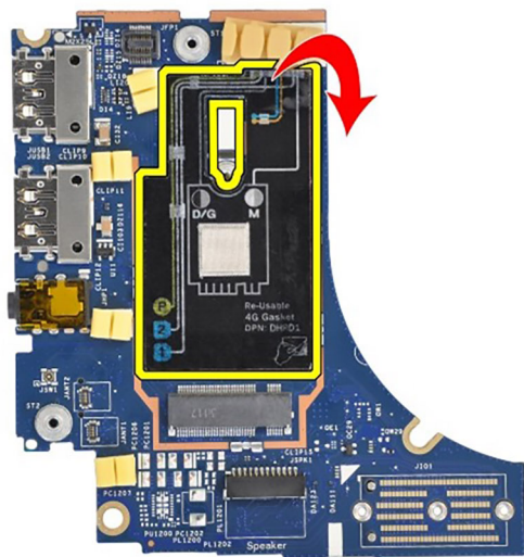
Figure 72. Latitude 7450 portable, configuration WWAN 4G (autocollant de joint)
