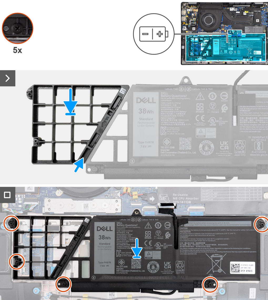
Figure 39. Installation de la batterie à 2 cellules
