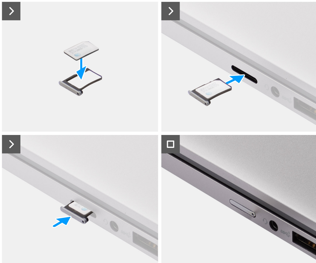
Figure 15. Installation du plateau de la carte SIM
