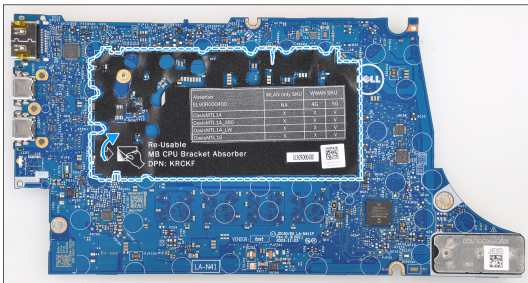
Figure 62. Absorbeur du support du processeur
