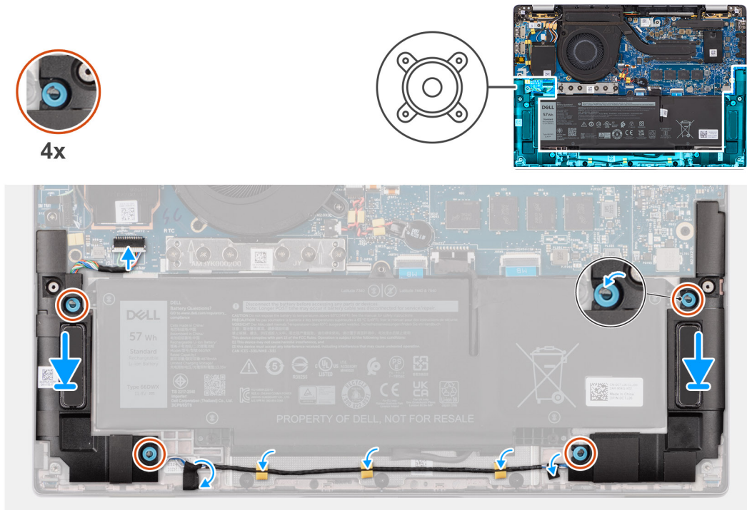
Figure 34. Installation des haut-parleurs pour standard
