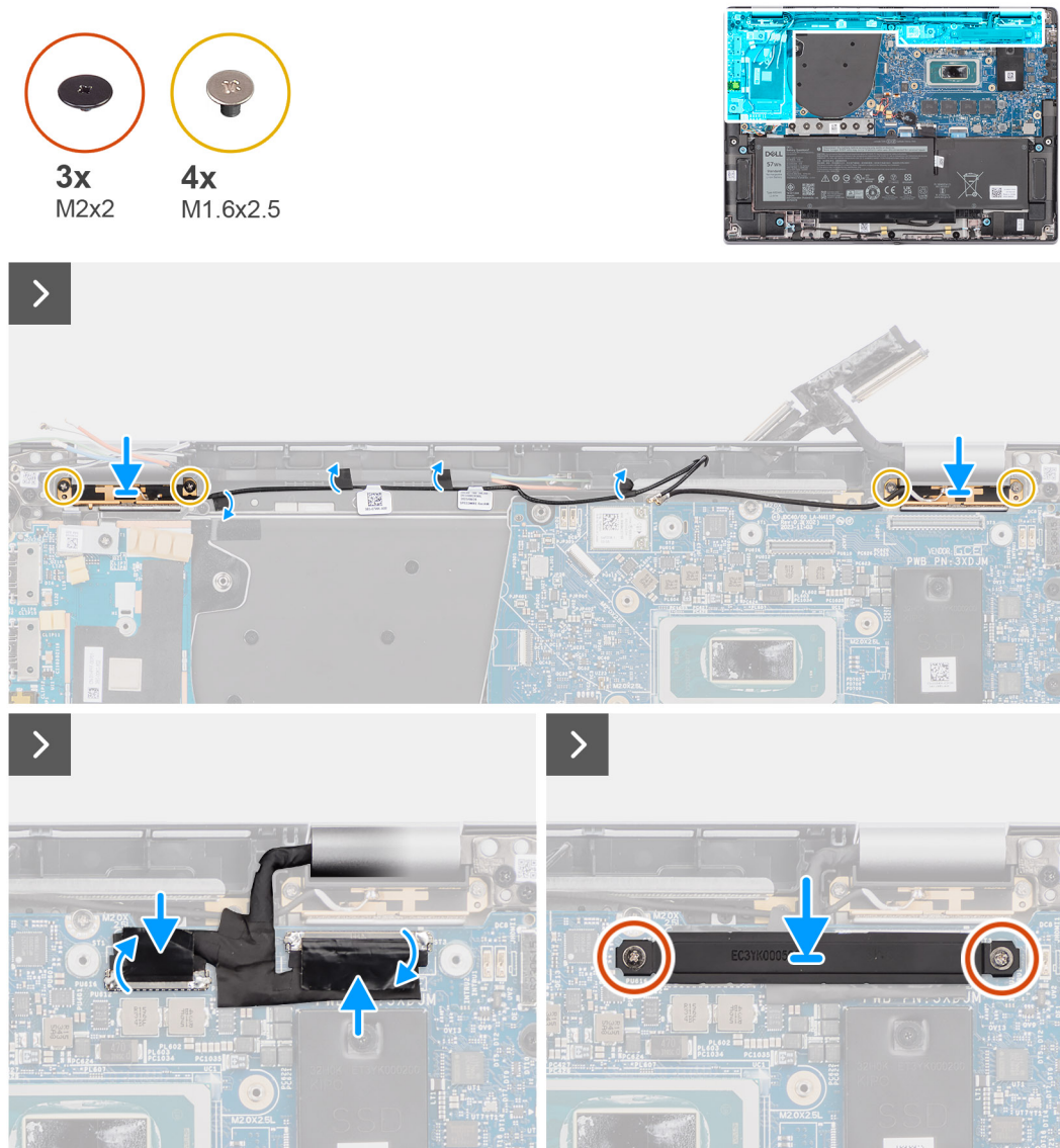
Figure 68. Installation du module d'antenne WLAN
