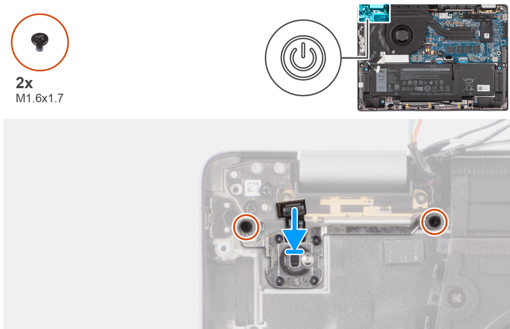
Figure 77. Installation du bouton d'alimentation avec lecteur d'empreintes digitales (en option)
