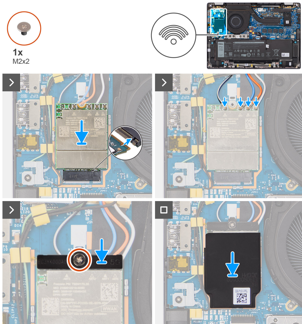
Figure 27. Installation de la carte WWAN 5G
