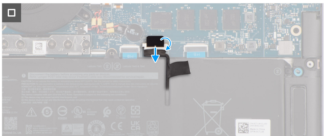
Figure 18. Retrait du cache de fond
