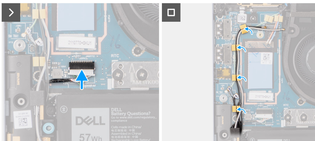
Figure 32. Installation des haut-parleurs pour l'ultralight
