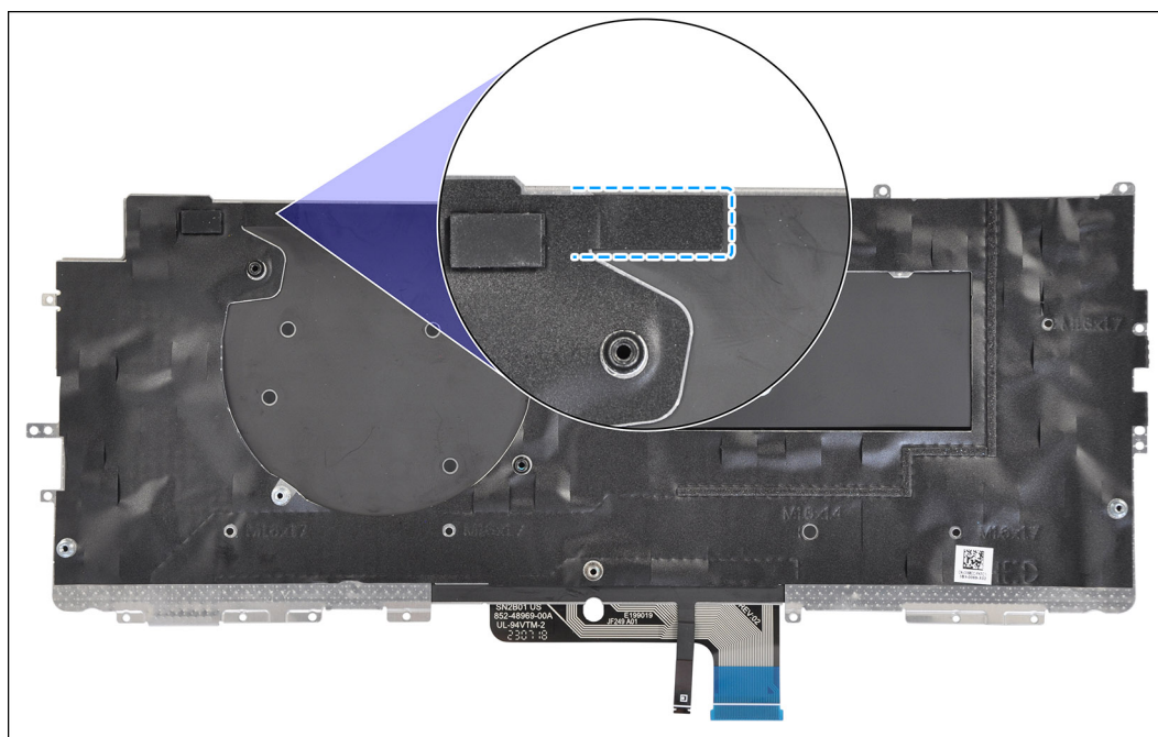
Figure 80. Retrait du ruban adhésif en mylar du clavier
