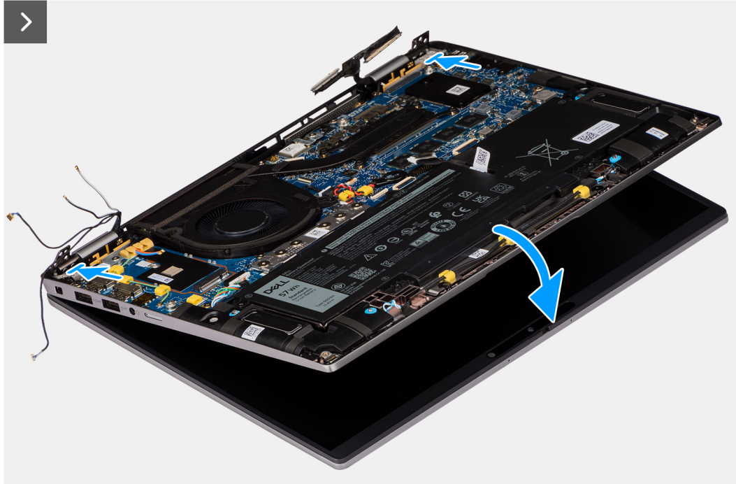
Figure 53. Installation de l'assemblage d'écran
