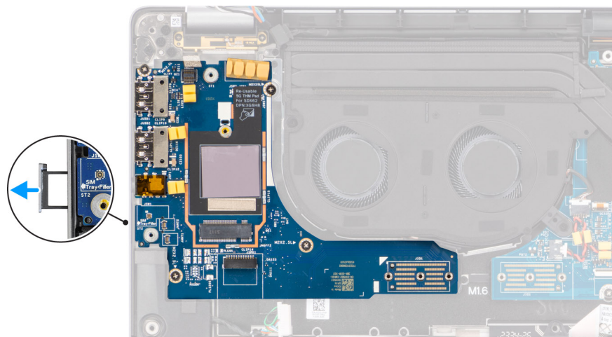
Figure 70. Retrait de la carte fille d'E/S
