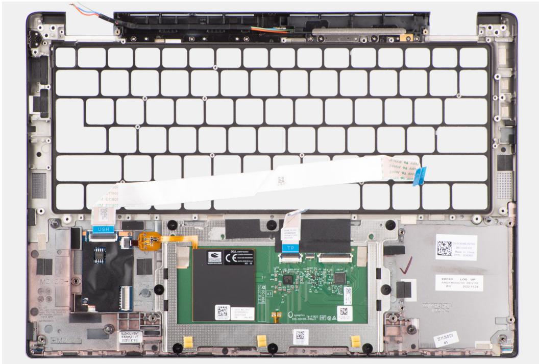
Figure 85. Installation de l'assemblage du repose-poignets
