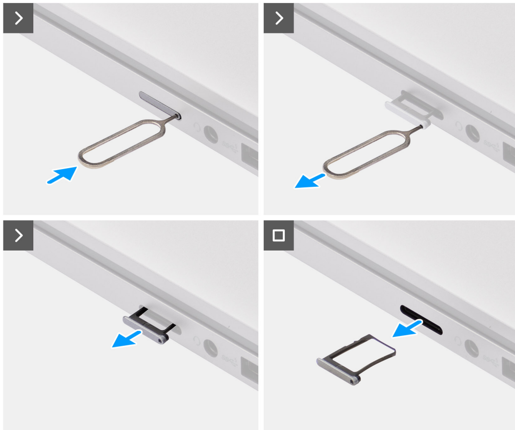
Figure 13. Retrait du plateau de carte SIM
