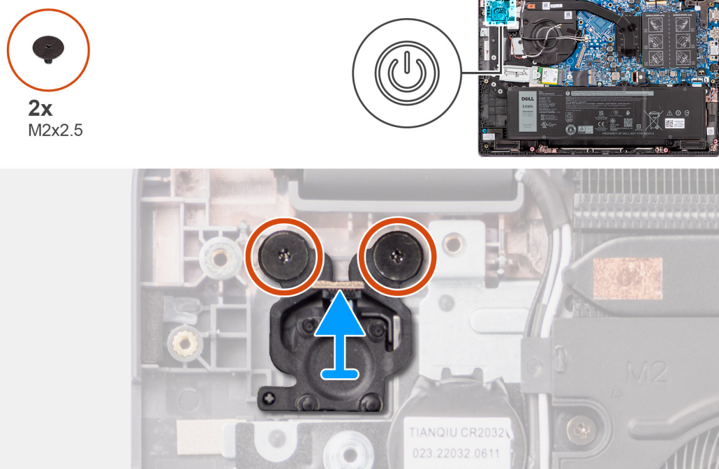
Ilustración 39. Extracción del botón de encendido
