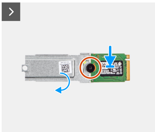
Ilustración 20. Instalación de la unidad de estado sólido M.2 2230
