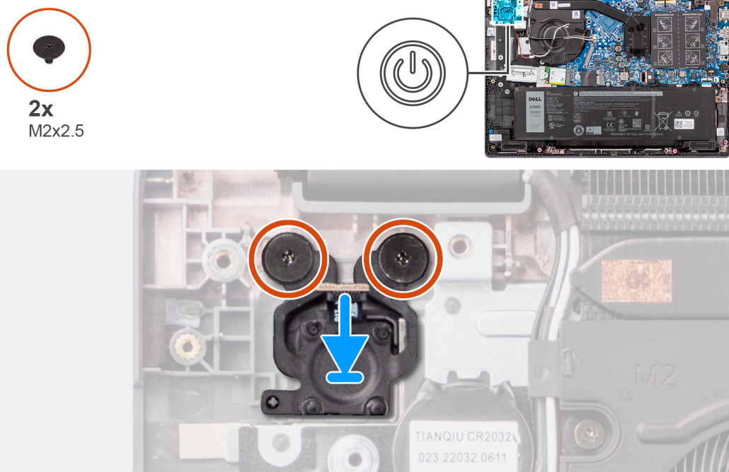
Ilustración 40. Instalación del botón de encendido
