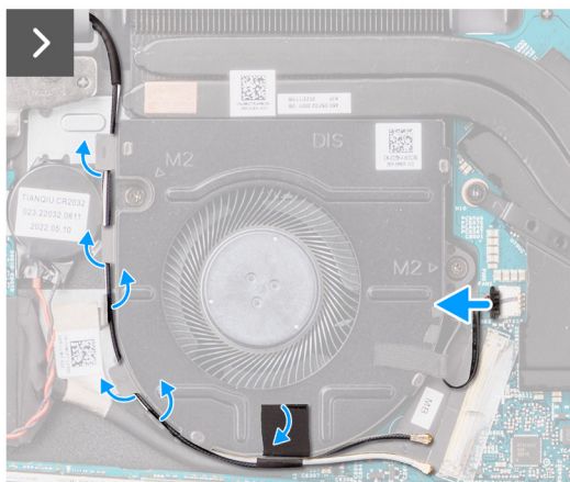
Ilustración 33. Extracción del ventilador
