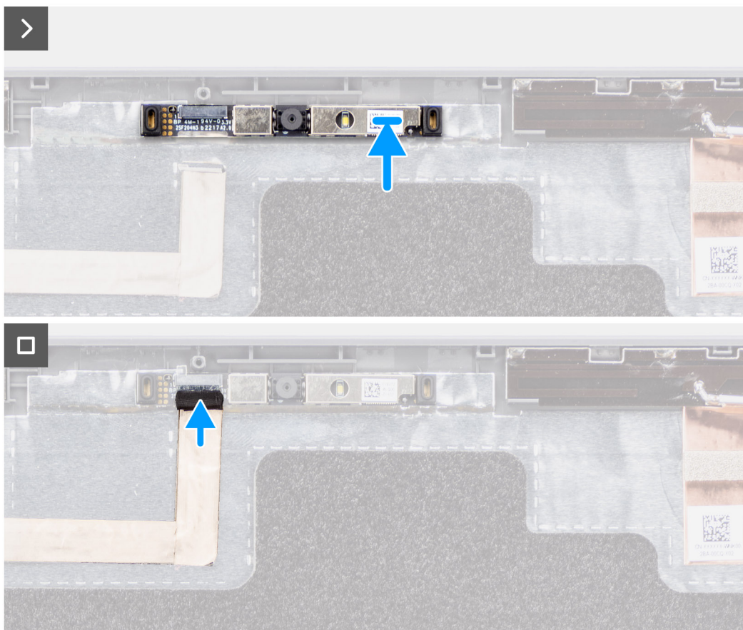
Ilustración 65. Instalación de la cámara
