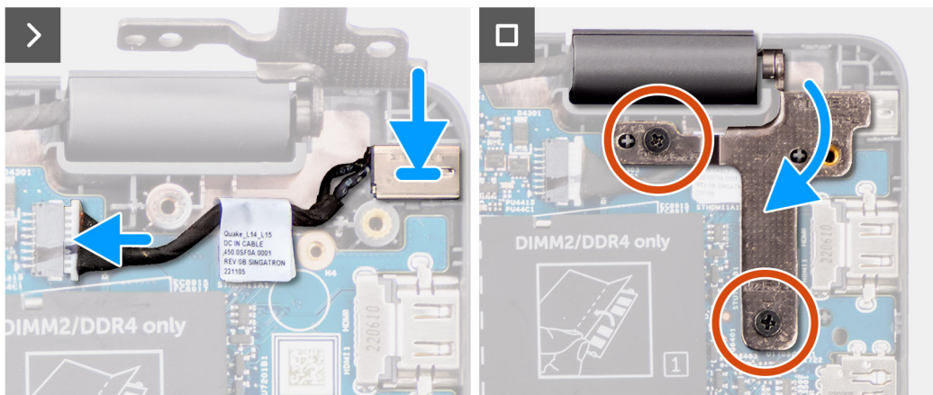
Ilustración 28. Instalación del puerto del adaptador de alimentación
