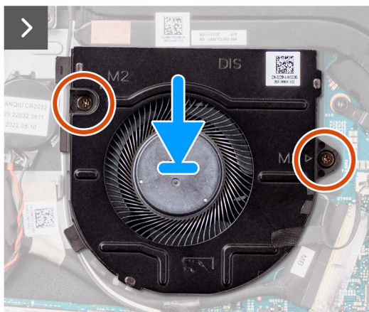
Ilustración 34. Instalación del ventilador
