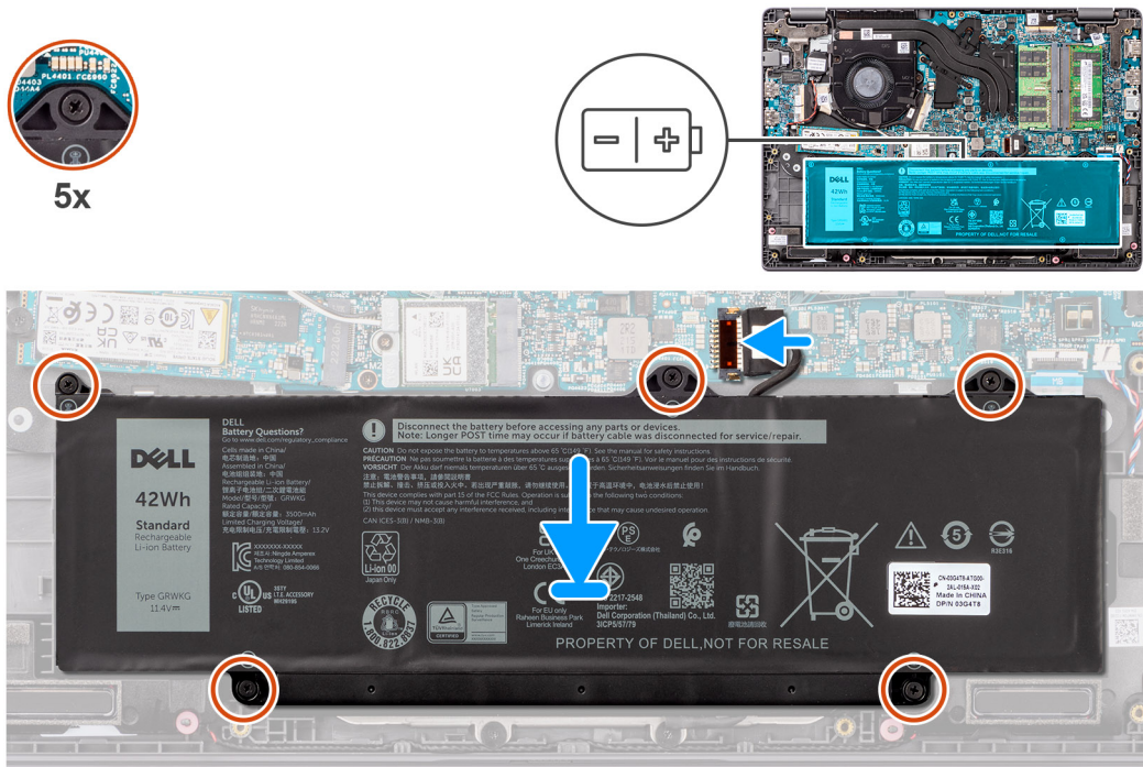
Abbildung 24. Einsetzen des Akkus
