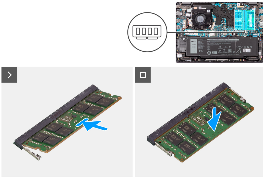
Abbildung 14. Einsetzen der Speichermodule
