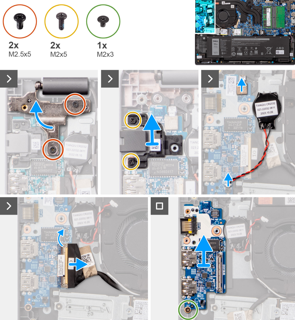
Abbildung 37. Entfernen der E/A-Platine
