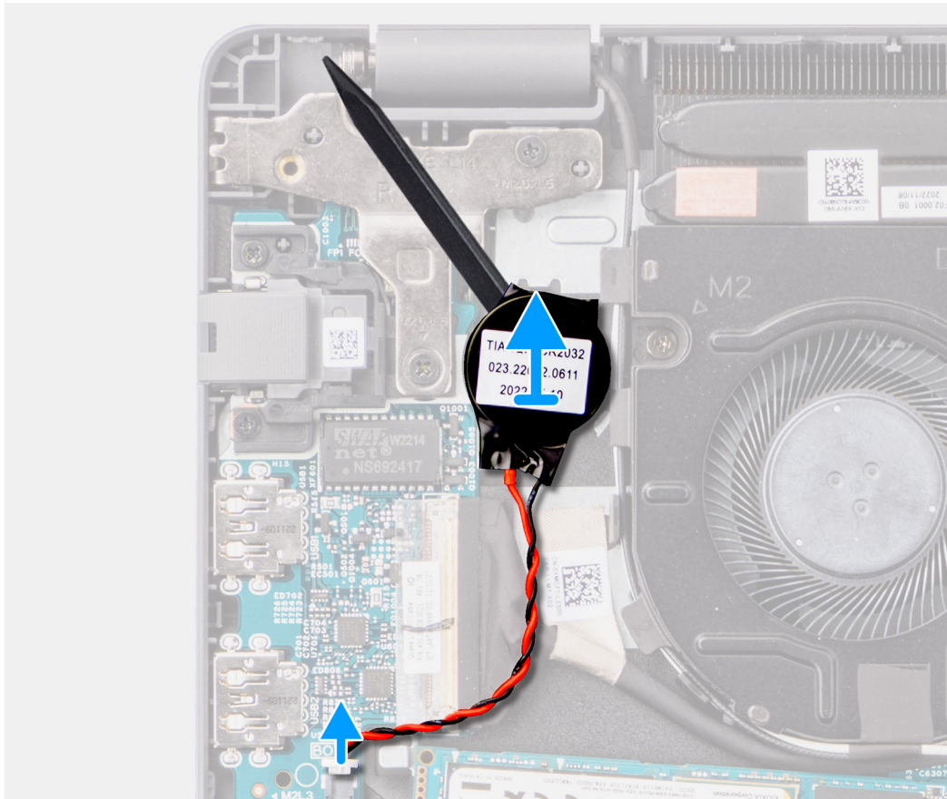
Abbildung 17. Entfernen der Knopfzellenbatterie
