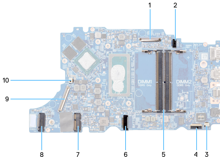
Abbildung 41. Systemplatinenanschlüsse
