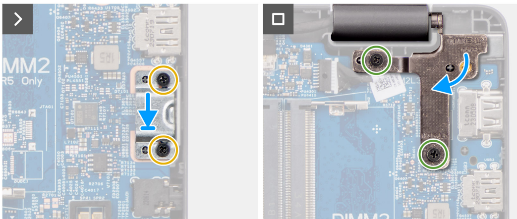
Abbildung 44. Einbauen der Systemplatine
