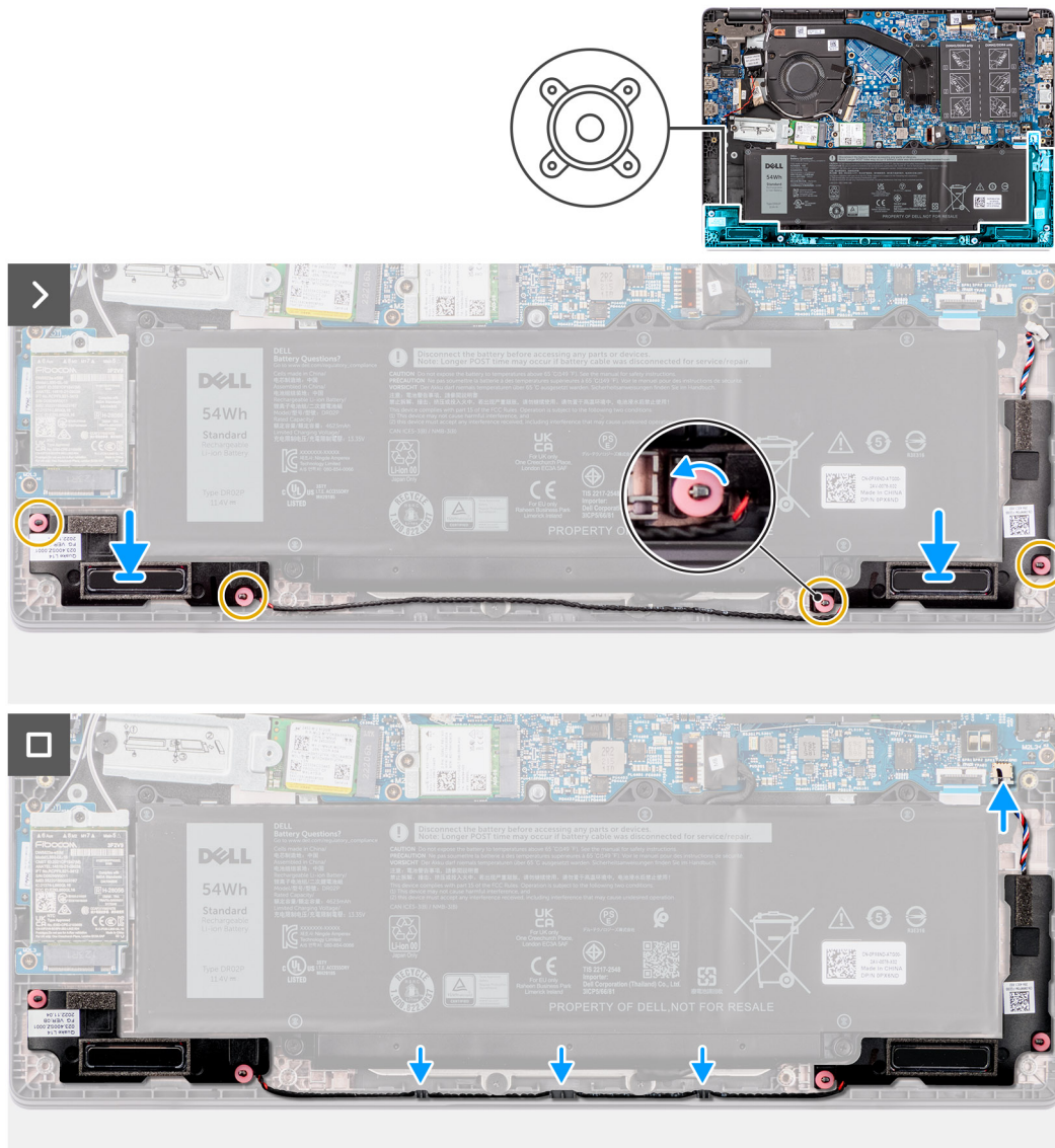
Abbildung 22. Einbau der Lautsprecher
