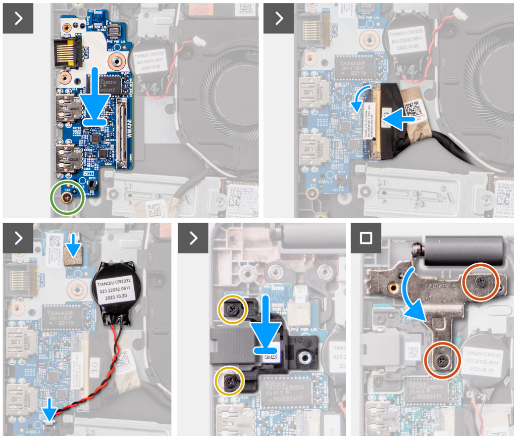
Abbildung 38. E/A-Platine einbauen
