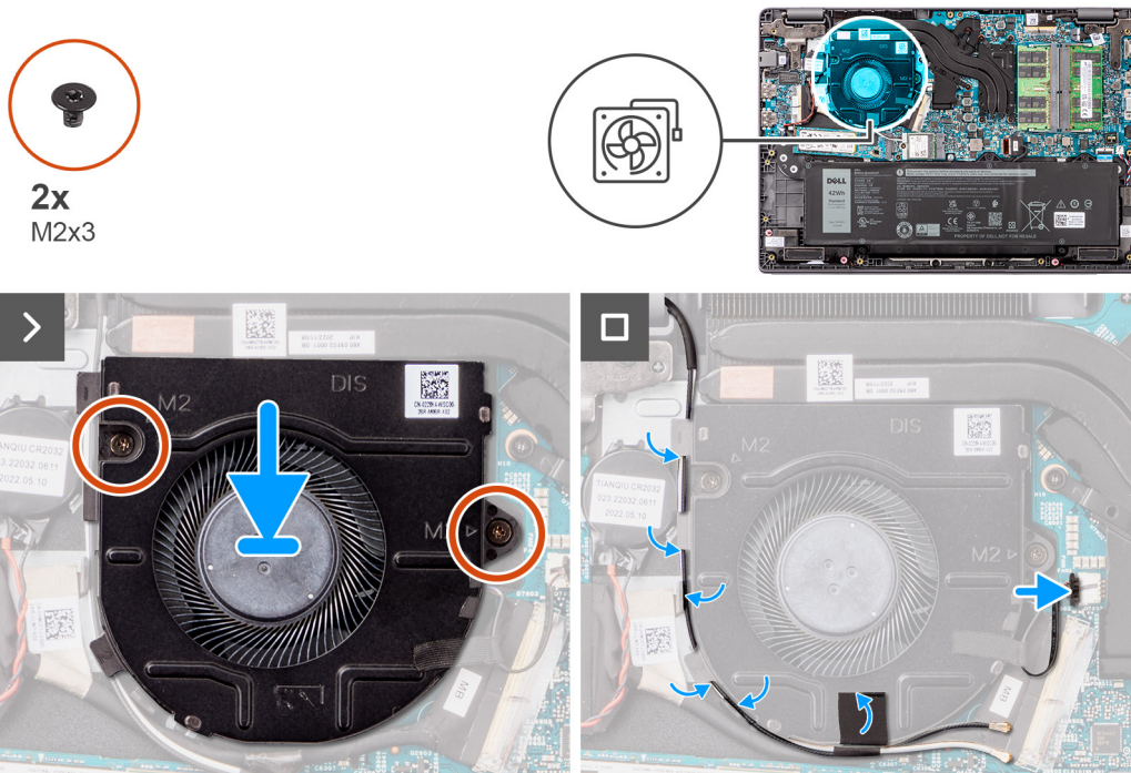
Abbildung 34. Einbauen des Lüfters
