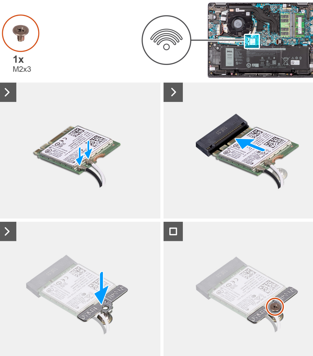
Abbildung 16. Einbauen der Wireless-Karte
