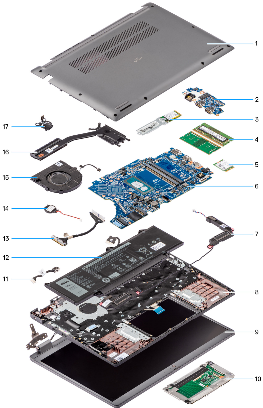
Abbildung 8. Explosionsansicht des Latitude 3450
