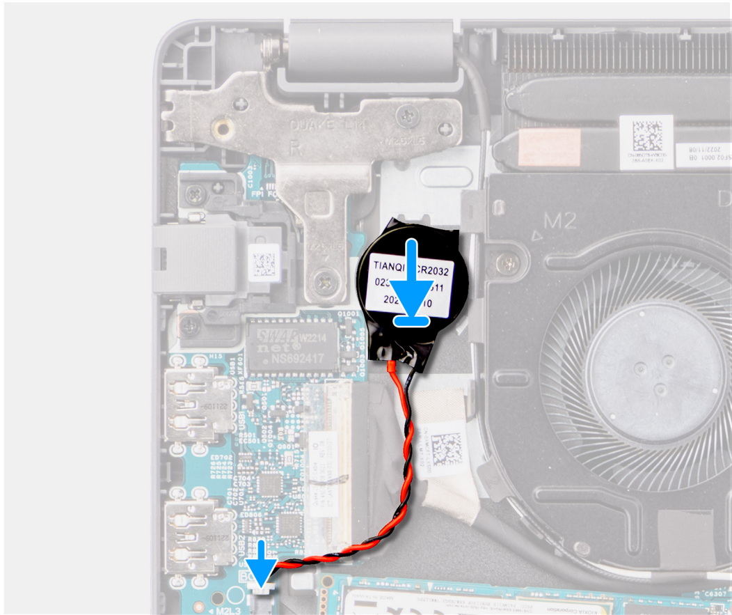
Abbildung 18. Einsetzen der Knopfzellenbatterie
