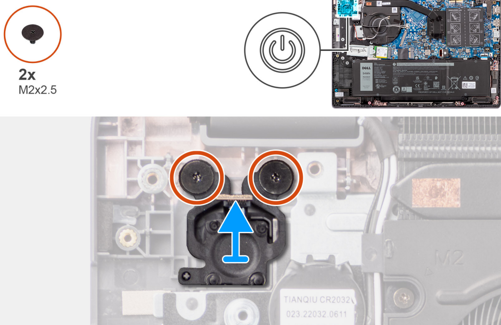
Abbildung 39. Entfernen des Netzschalters
