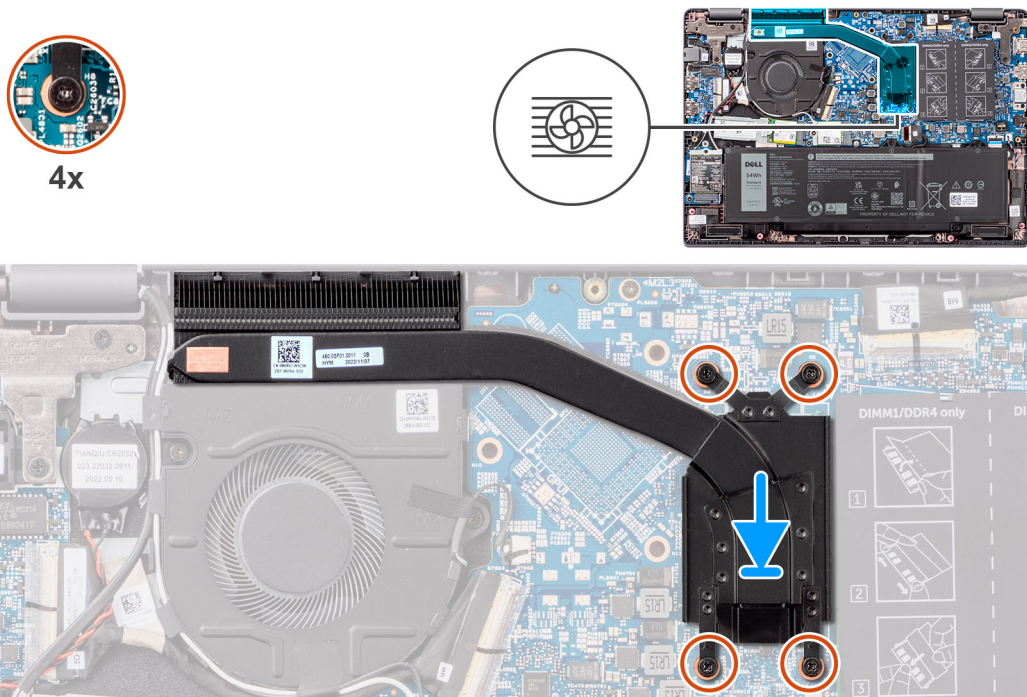
Abbildung 30. Installieren des Kühlkörpers für integrierte Grafikkarten
