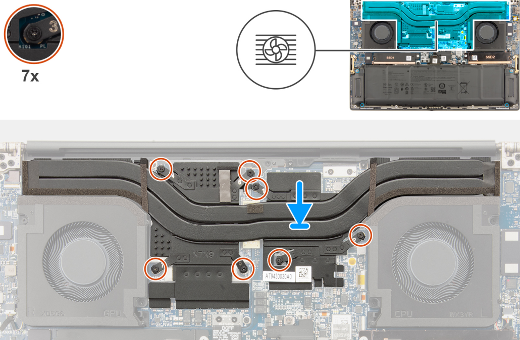
Abbildung 29. Installieren des Kühlkörpers für die separate Grafikkarte
