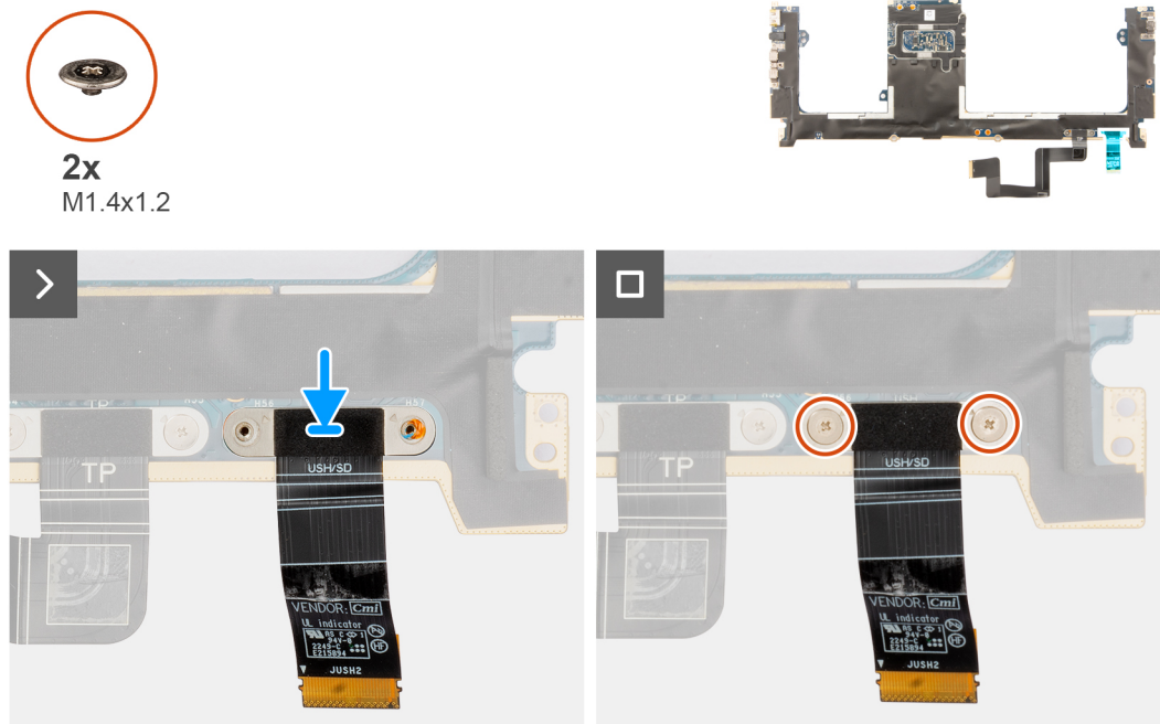
Abbildung 76. Installieren des FPC-Kabels der USH/SD-Karten-Zusatzplatine
