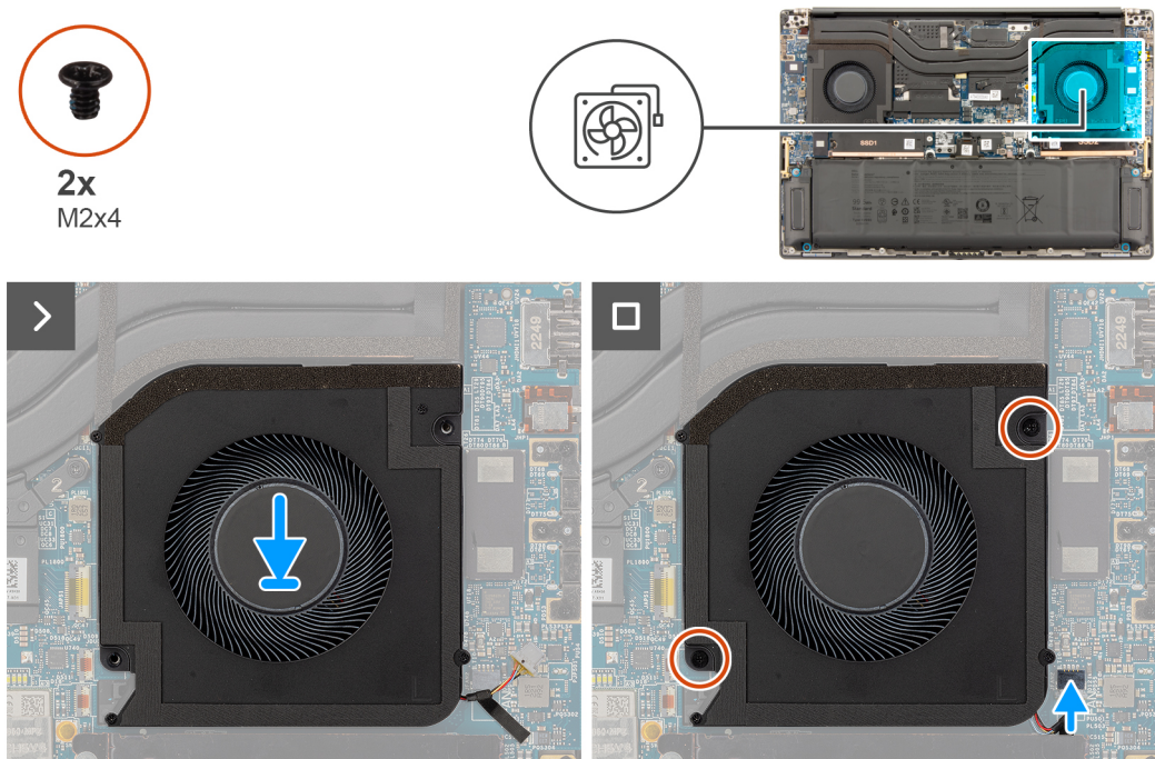
Abbildung 23. Installieren des Prozessorlüfters
