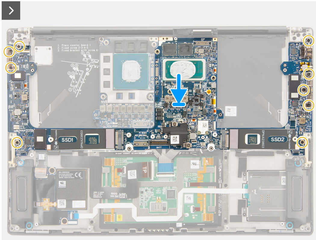
Abbildung 63. Installieren der Hauptplatine
