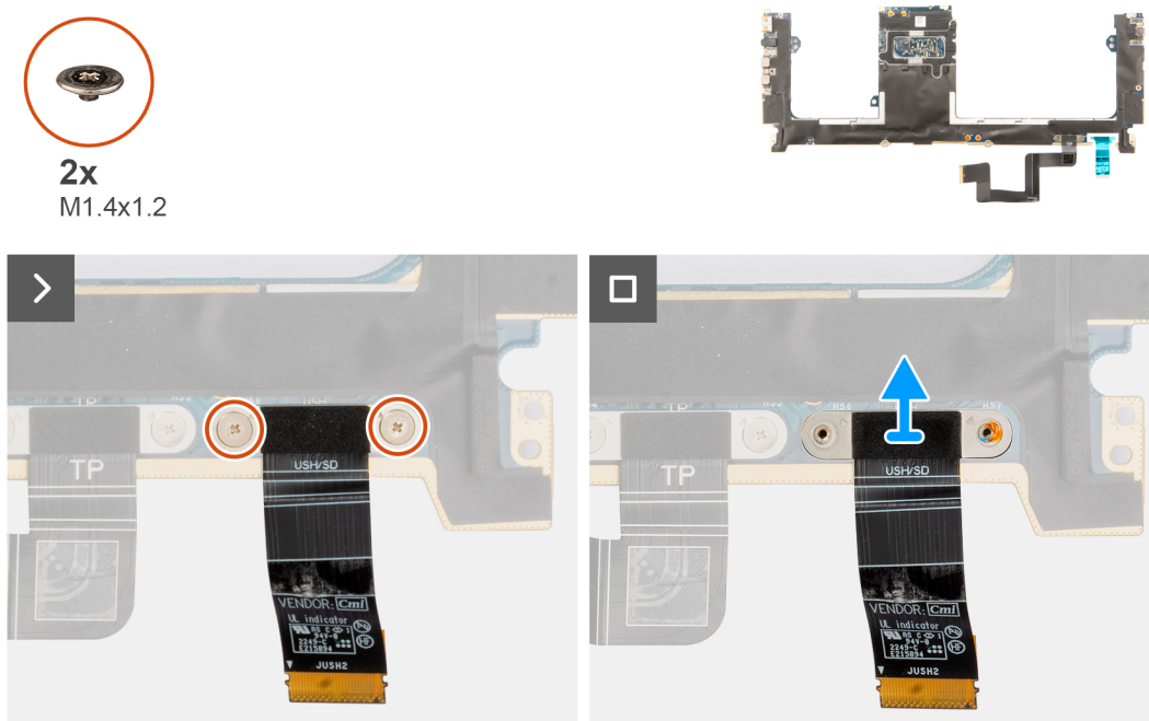
Abbildung 73. Entfernen des FPC-Kabels der SD-Karten-Zusatzplatine
