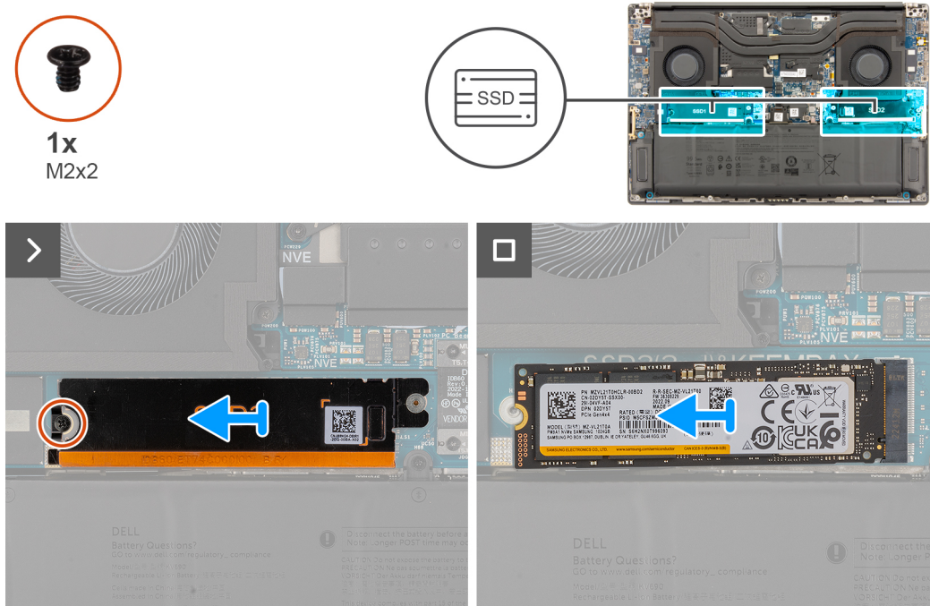
Abbildung 18. Entfernen der M.2-2280-SSD
