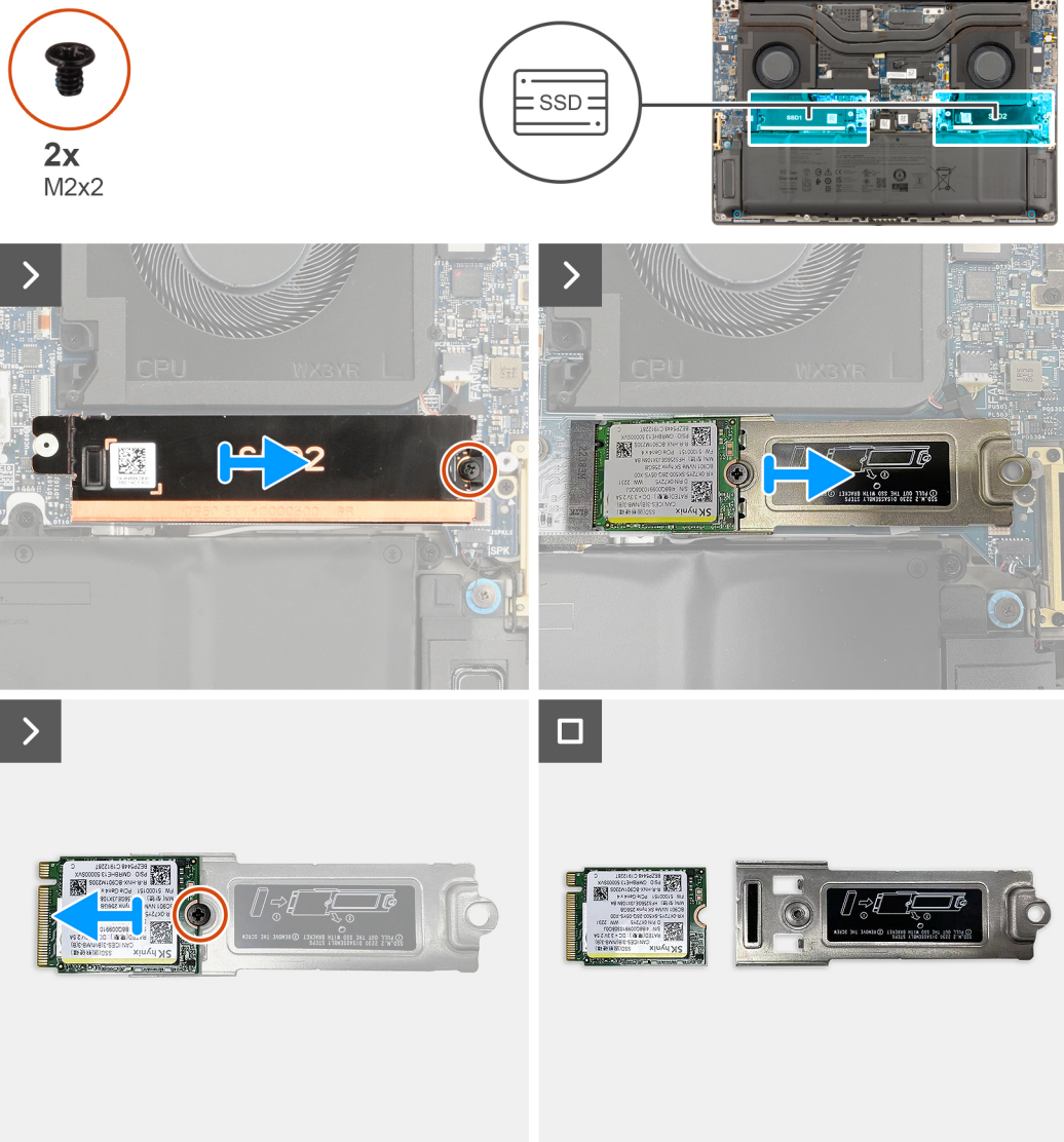
Abbildung 16. Entfernen des M.2-2230-Solid-State-Laufwerks
