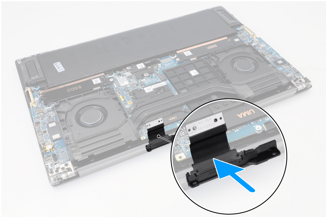
Abbildung 36. FPC-Kabel des Displays
