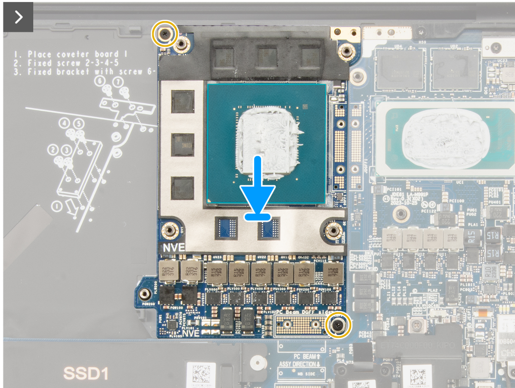
Abbildung 47. Entfernen der Grafikkarte
