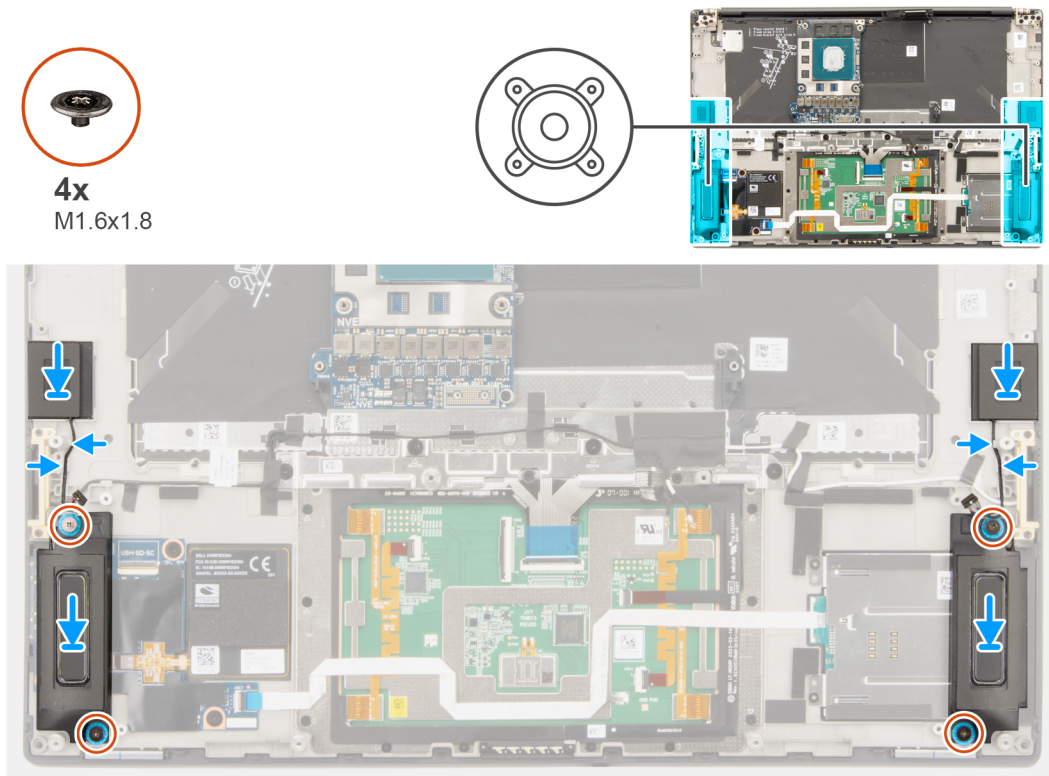
Abbildung 69. Einbauen der Lautsprecher
