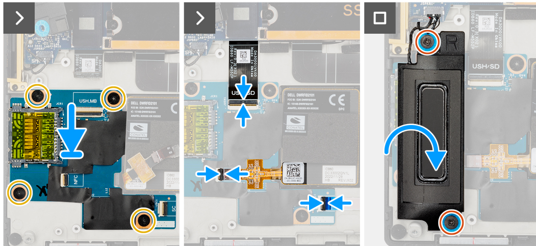
Abbildung 42. Installieren der USH/SD-Karten-Zusatzplatine
