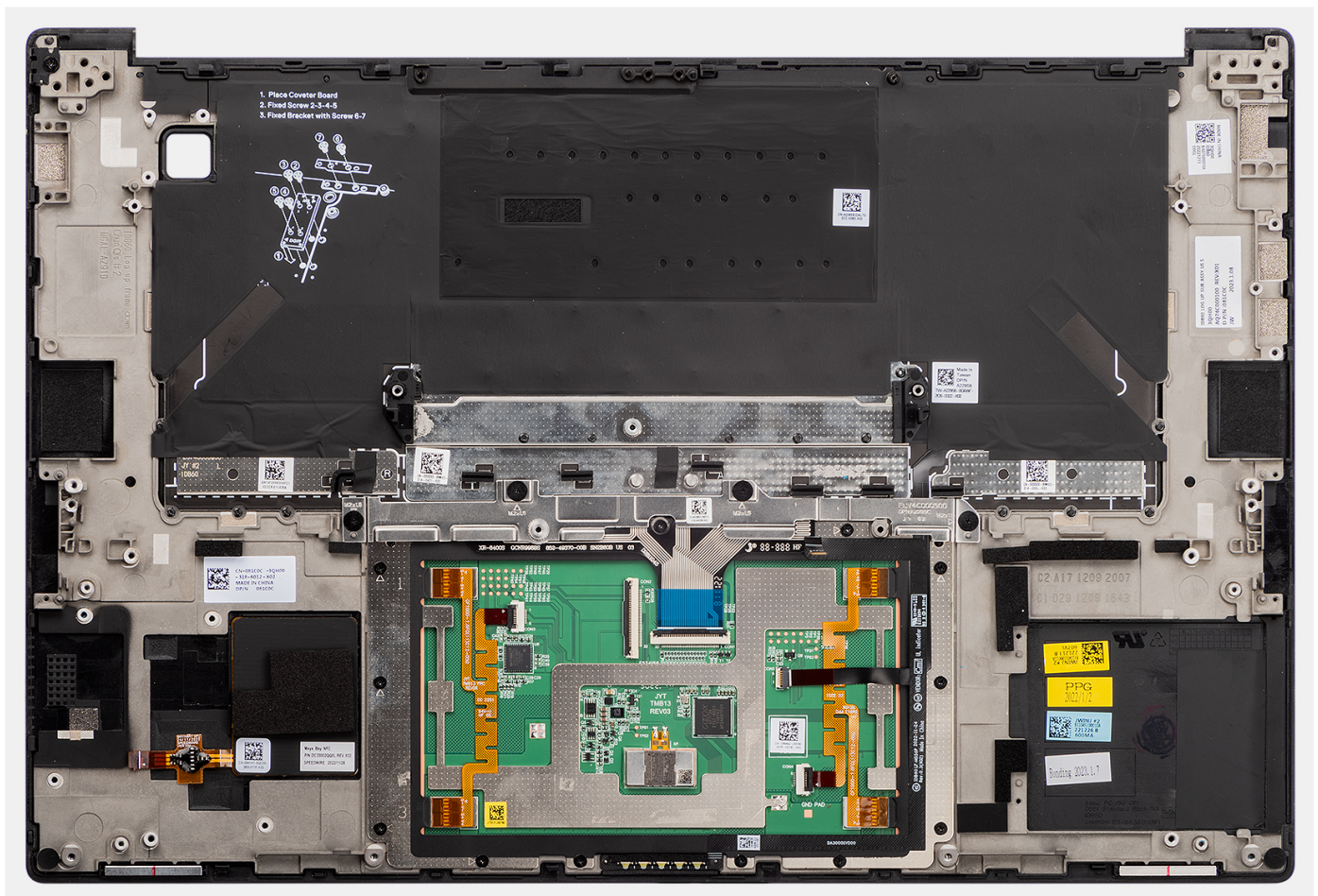
Abbildung 81. Entfernen der Handauflage/Tastatur-Baugruppe
