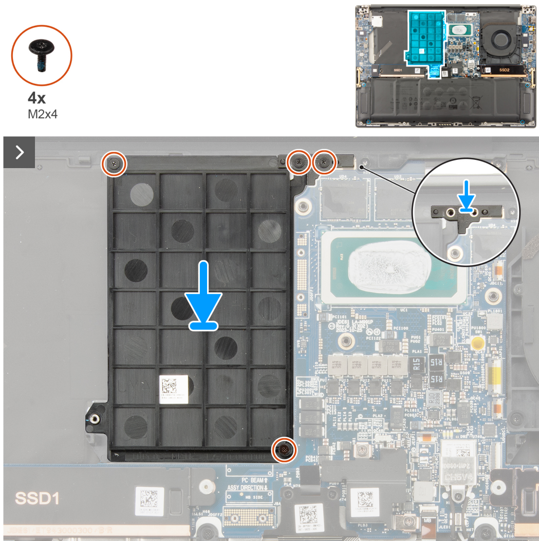
Abbildung 52. Installieren des Grafikkartenplatzhalters
