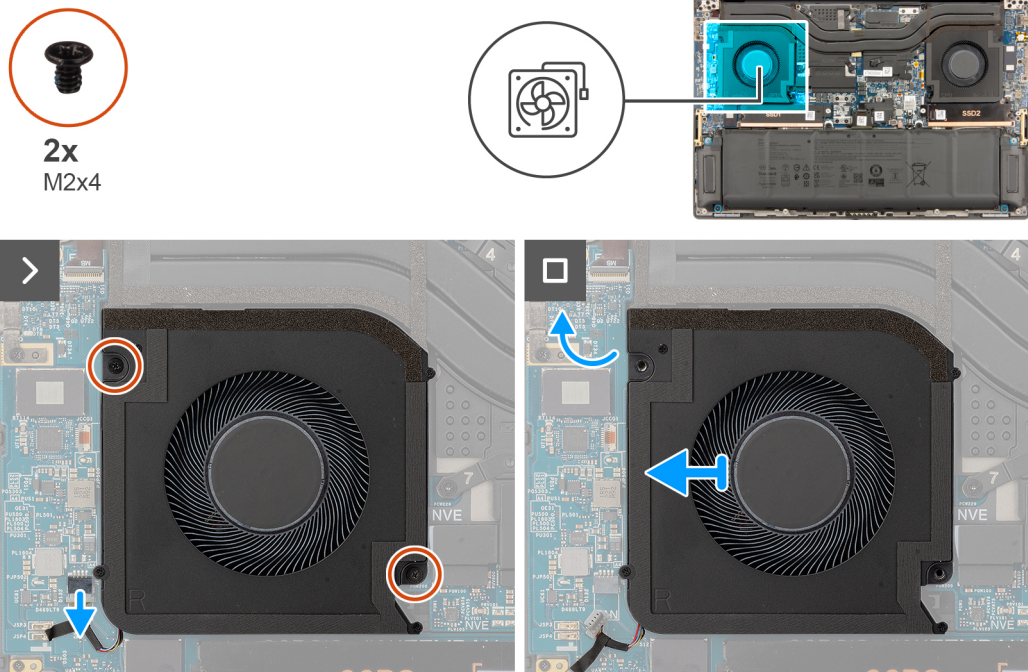
Abbildung 24. Entfernen des Grafikkartenlüfters
