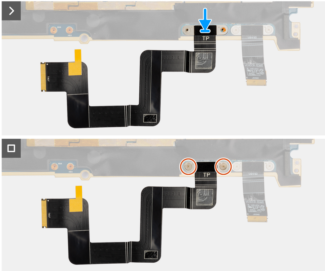
Abbildung 72. Installieren der haptischen Touchpad-FPC
