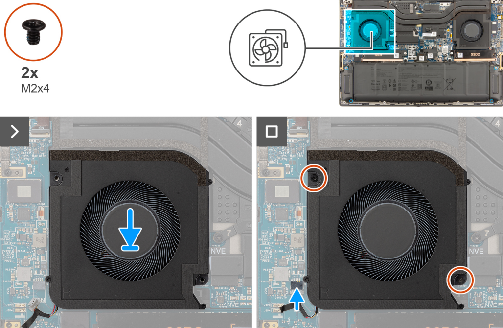
Abbildung 25. Installieren des Grafikkartenlüfters
