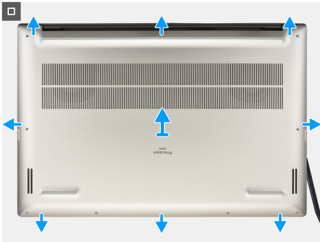
Abbildung 12. Entfernen der Bodenabdeckung
