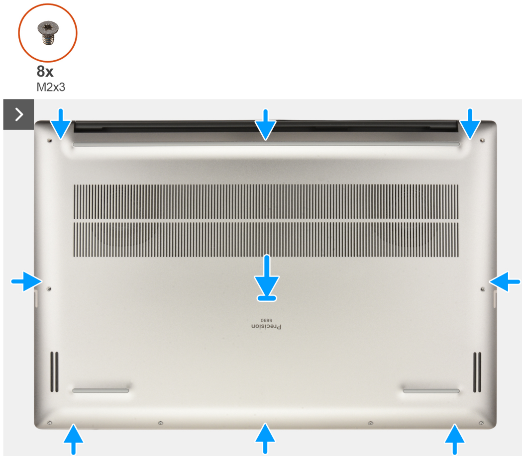
Abbildung 14. Installieren der Bodenabdeckung
