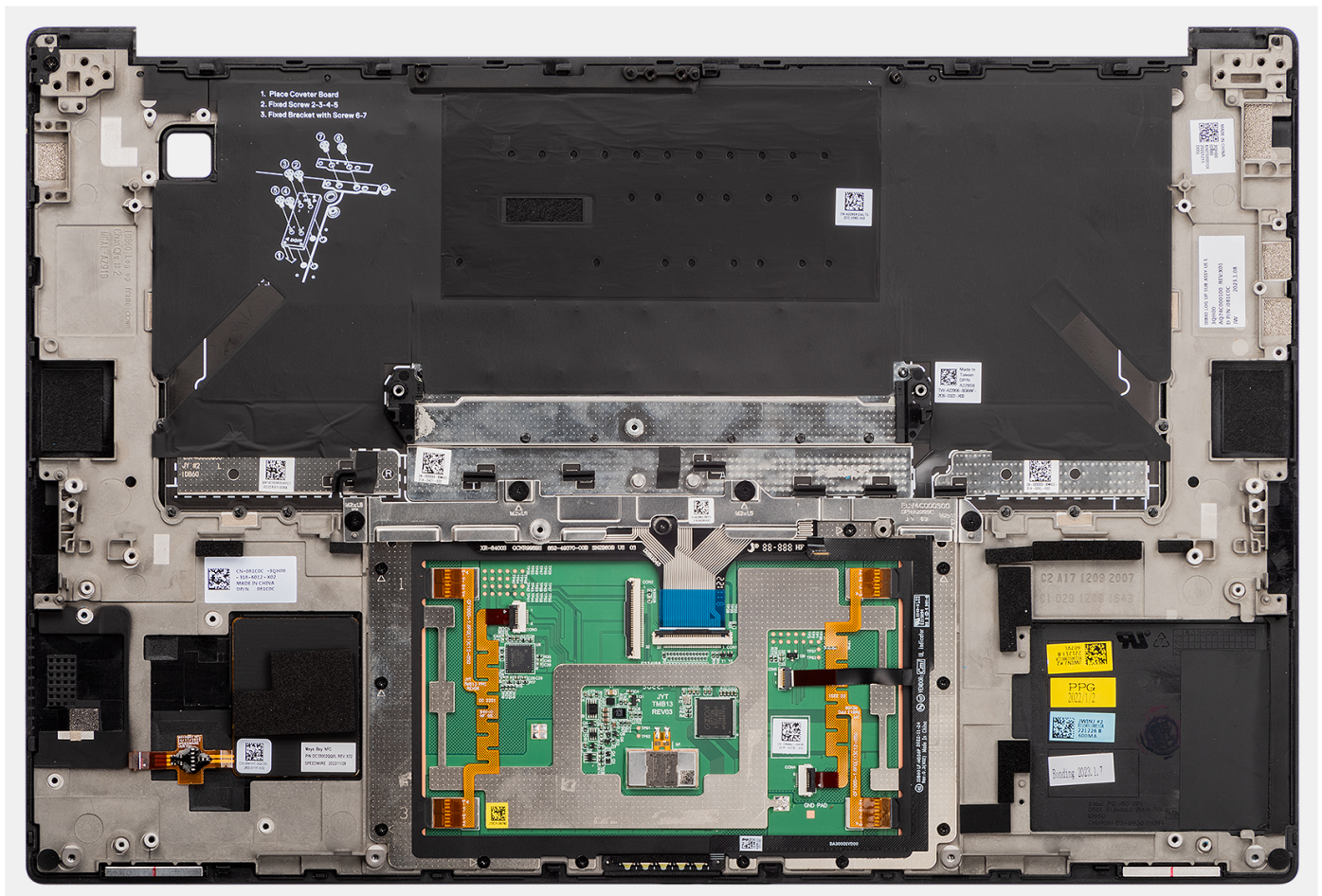
Abbildung 82. Installieren der Handauflage/Tastatur-Baugruppe
