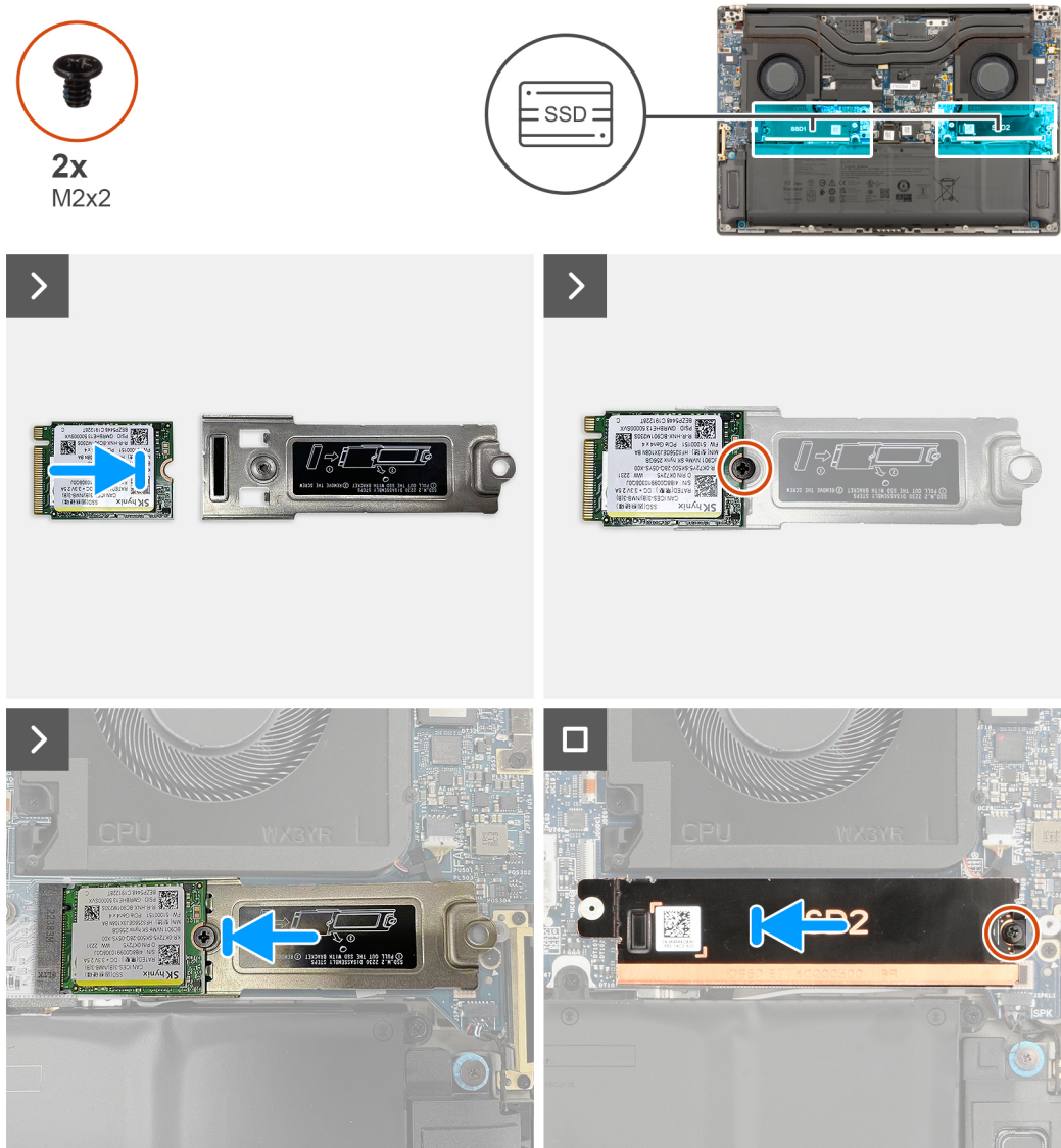
Abbildung 17. Installieren der M.2-2230-SSD
