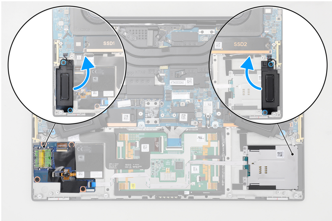
Abbildung 41. Lautsprecher
