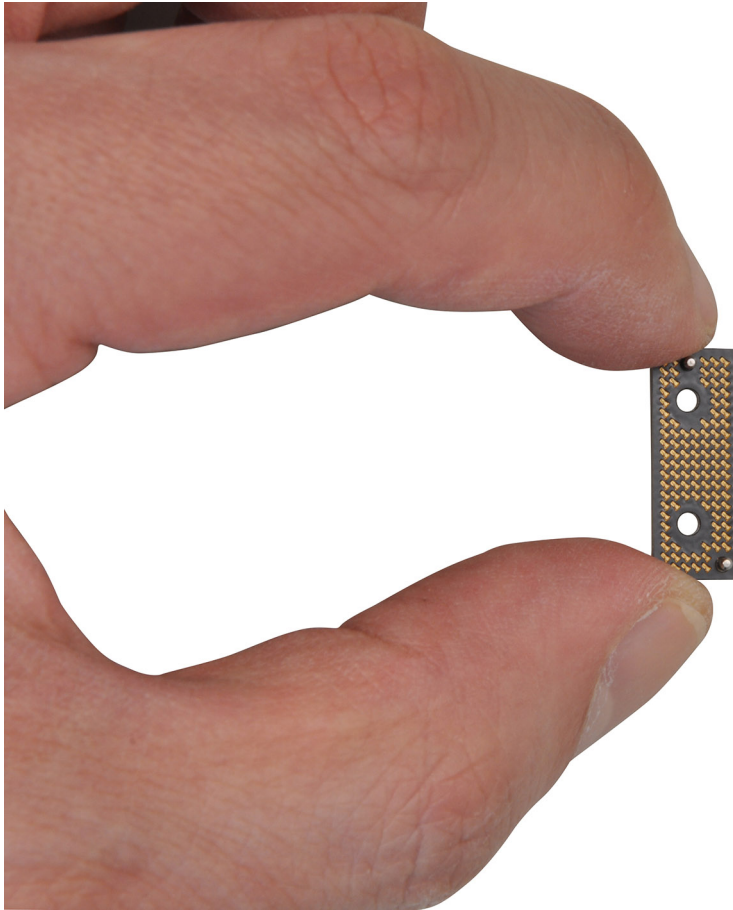
Abbildung 67. Interposer-Platine
