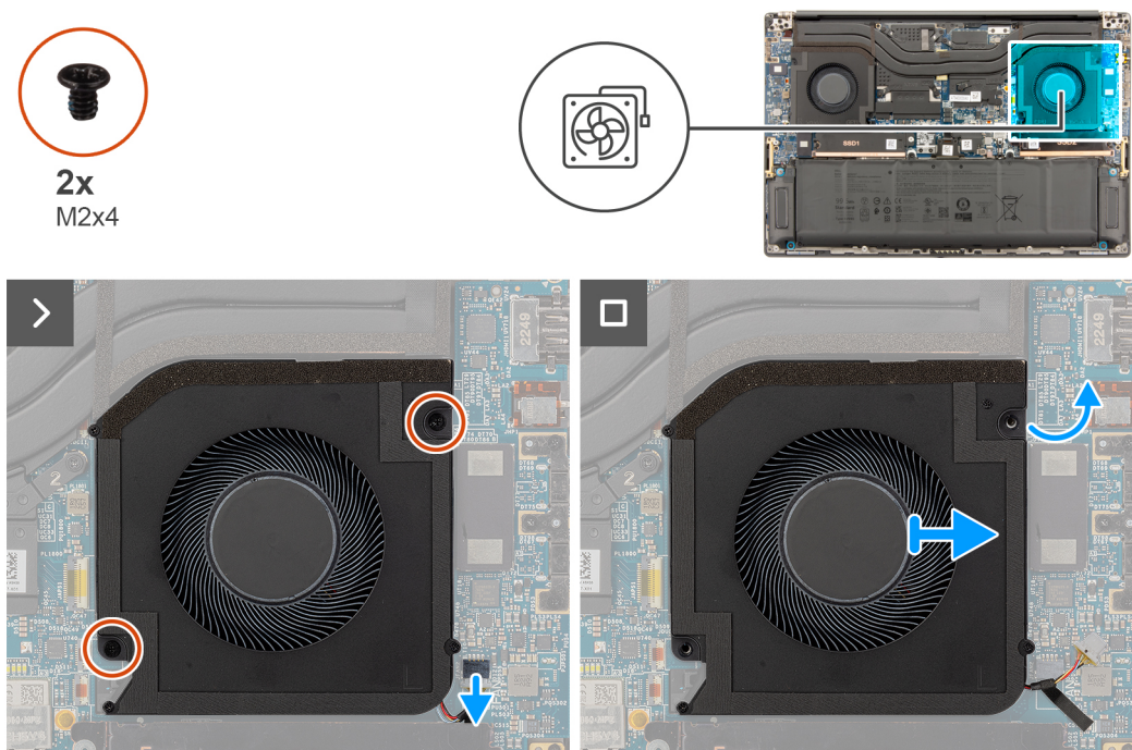
Abbildung 22. Entfernen des Prozessorlüfters
