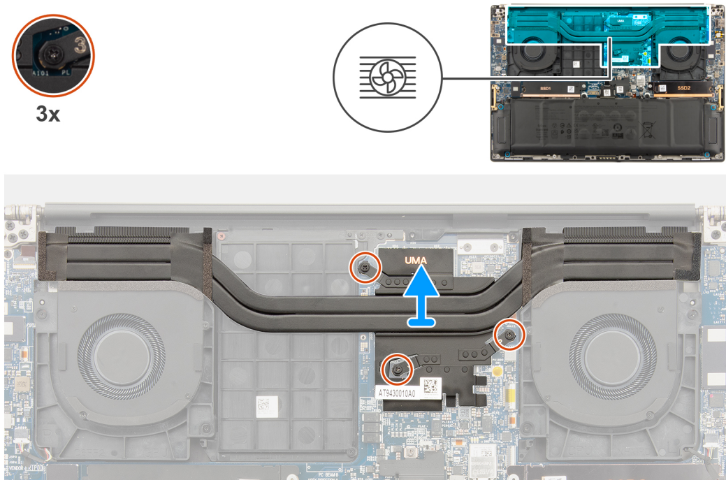
Abbildung 26. Entfernen des Kühlkörpers für die integrierte Grafikkarte
