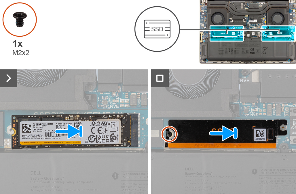
Abbildung 19. Installieren der M.2-2280-SSD
