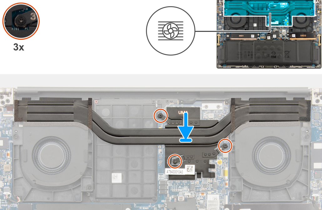
Abbildung 27. Installieren des Kühlkörpers für die integrierte Grafikkarte
