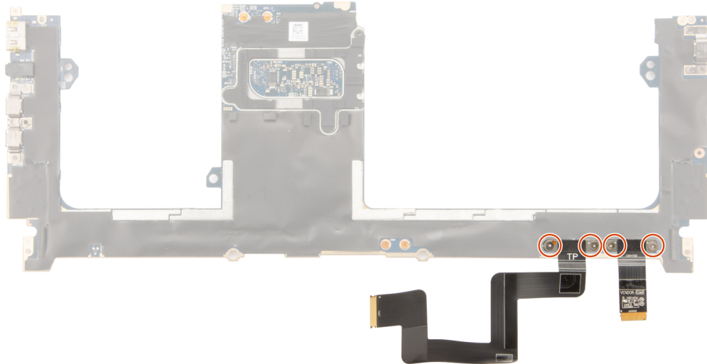
Abbildung 60. FPC-Kabel des Touchpads und FPC-Kabel der USH-Platine
