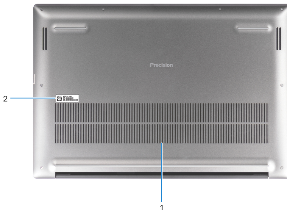
Abbildung 8. Unterseite
