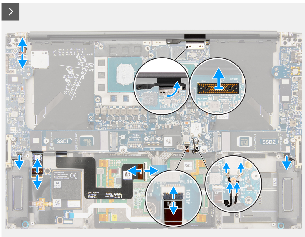
Abbildung 57. Entfernen der Hauptplatine
