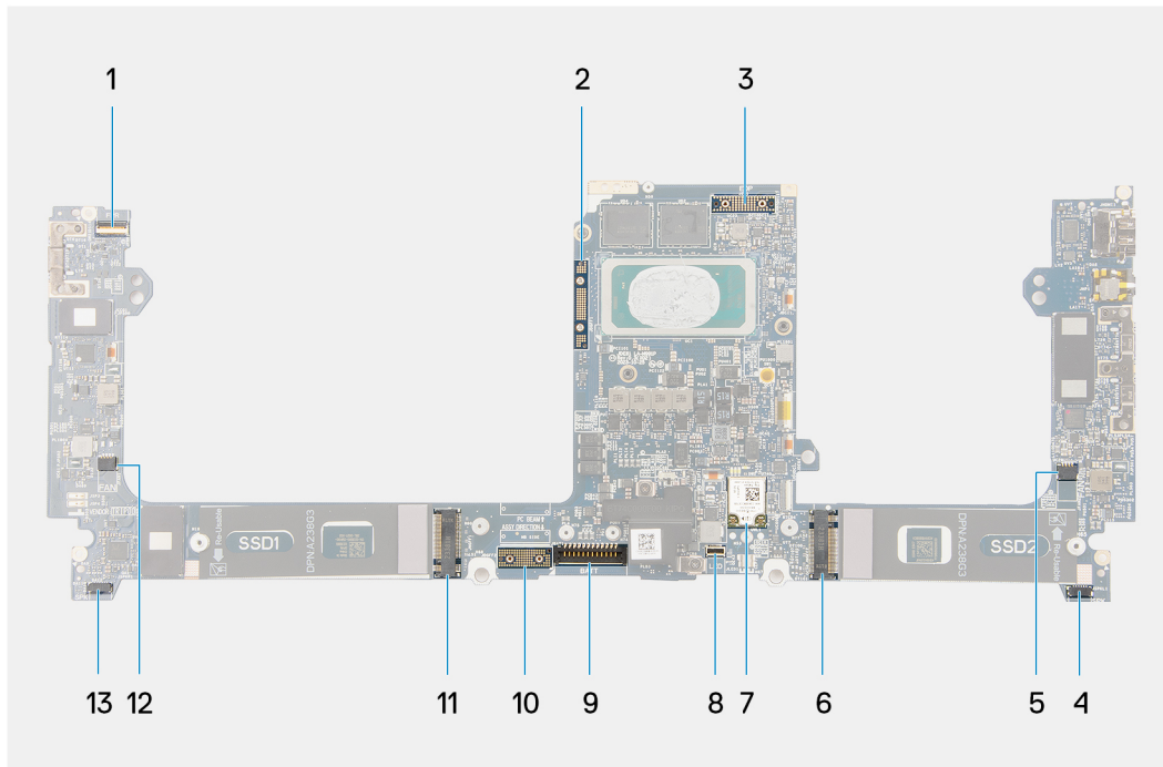
Abbildung 53. Anschlüsse auf der Hauptplatine
