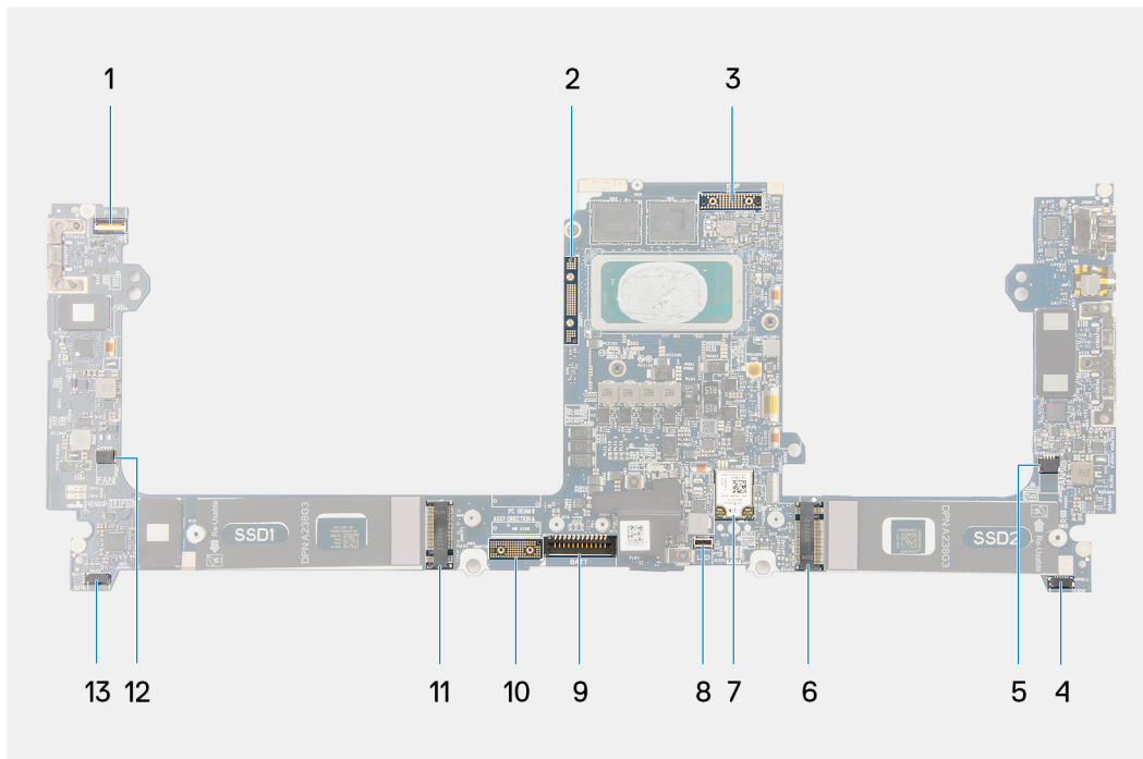
Abbildung 61. Anschlüsse auf der Hauptplatine
