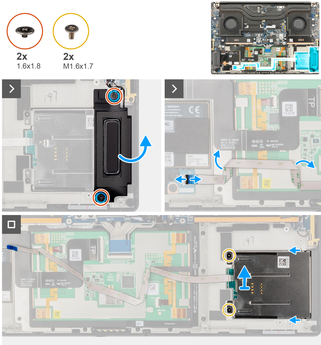
Abbildung 43. Entfernen des Smartcardlesegeräts
