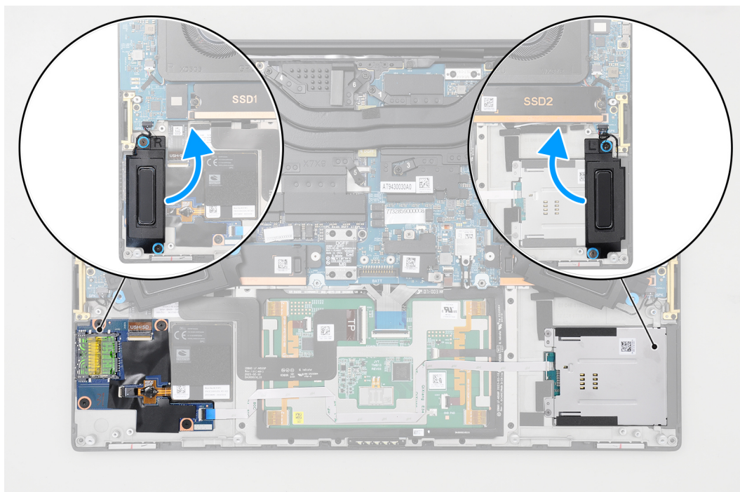
Abbildung 38. Lautsprecher
