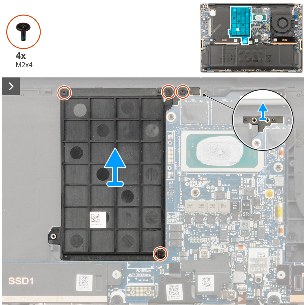
Abbildung 51. Entfernen des Grafikkartenplatzhalters
