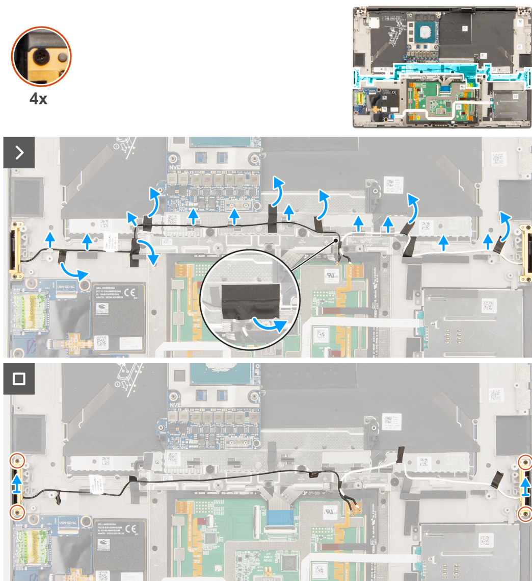
Abbildung 77. Entfernen des WLAN-Antennenmoduls
