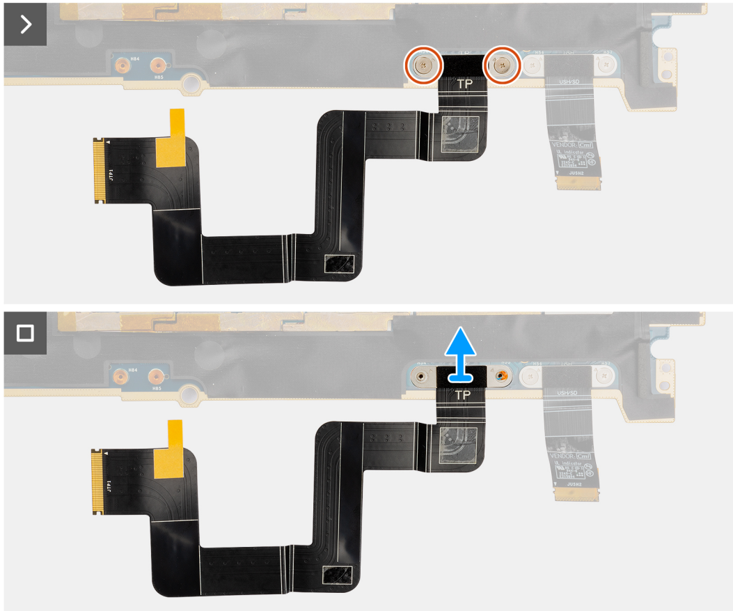
Abbildung 71. Installieren der haptischen Touchpad-FPC
