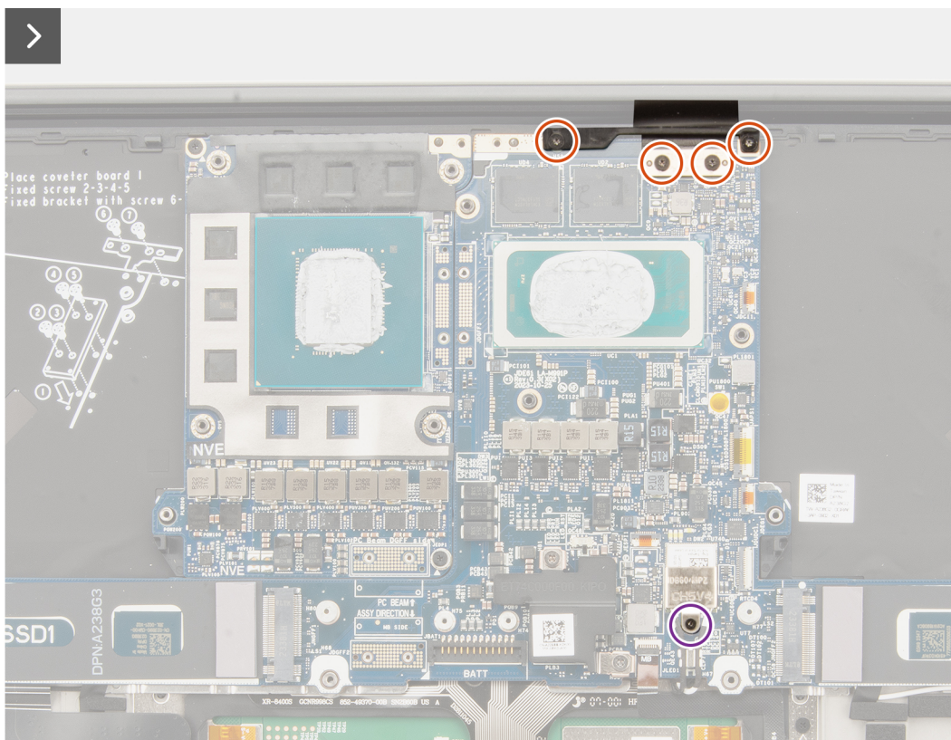
Abbildung 65. Installieren der Hauptplatine
