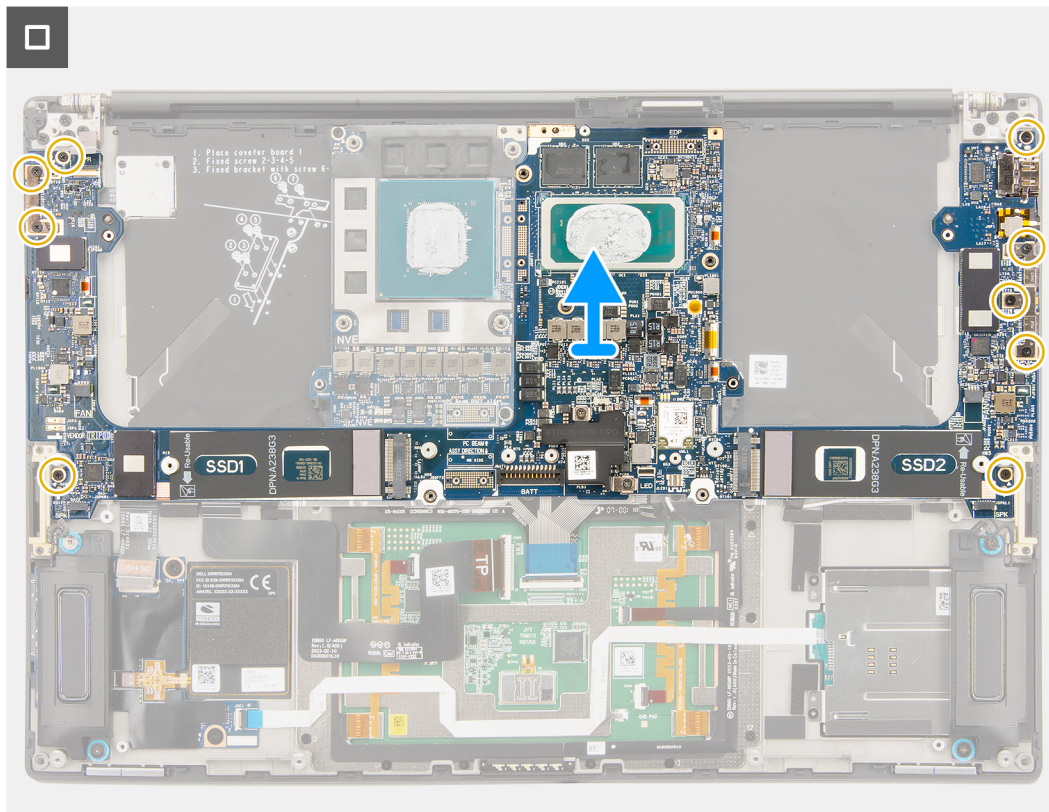
Abbildung 58. Entfernen der Hauptplatine
