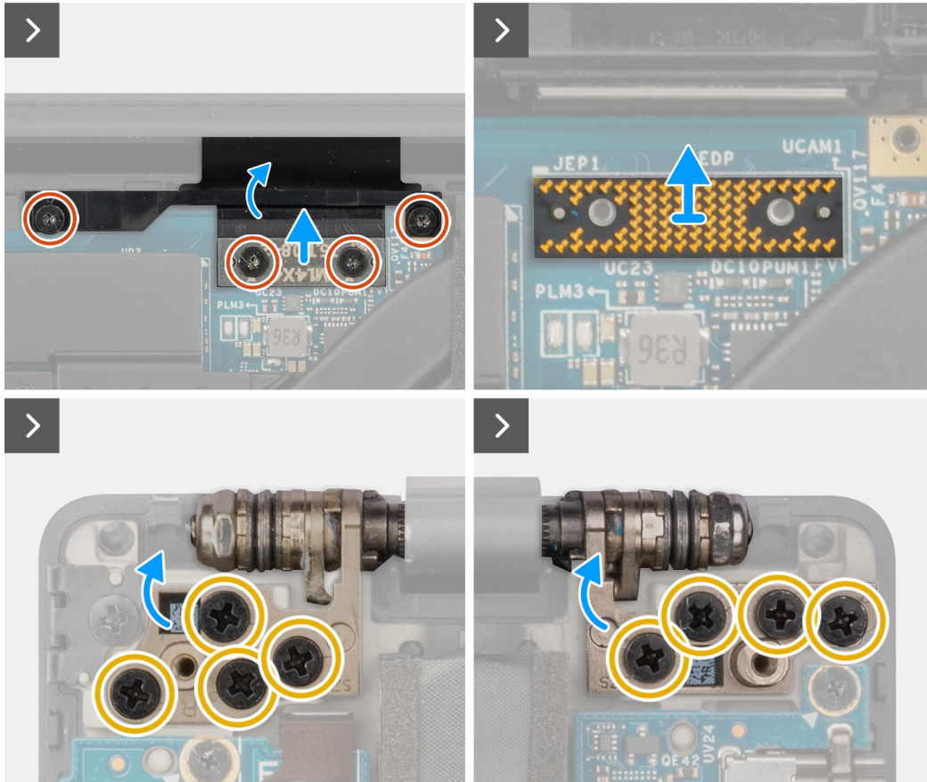
Abbildung 30. Entfernen der Displaybaugruppe
