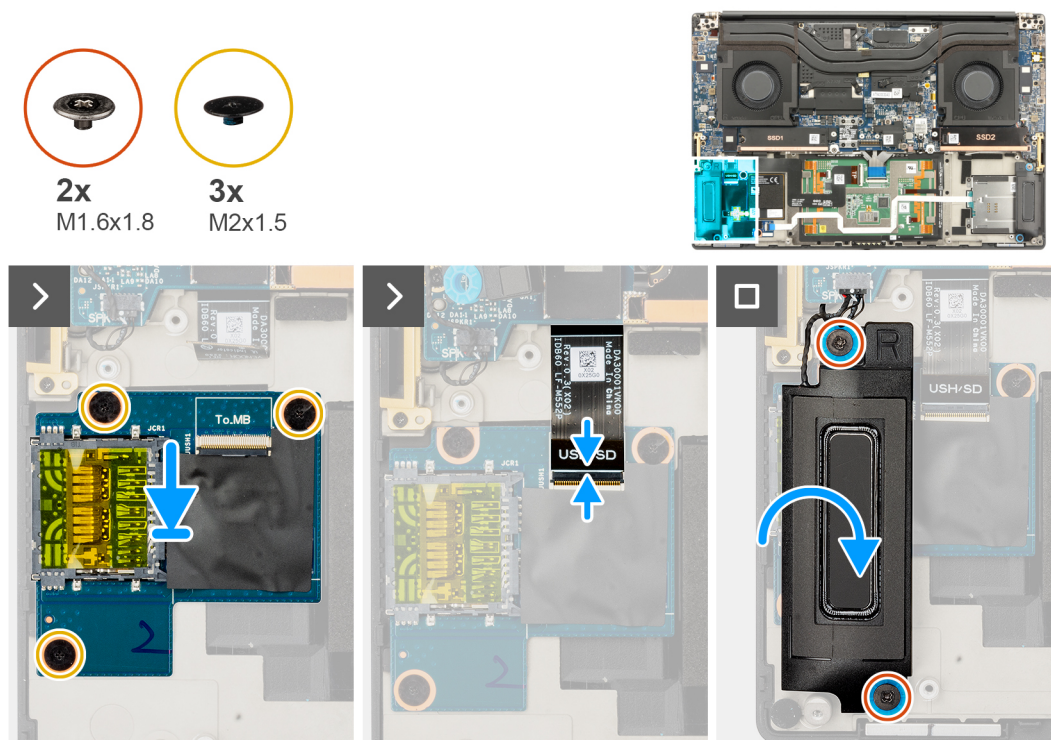
Abbildung 39. Installieren der SD-Karten-Zusatzplatine
