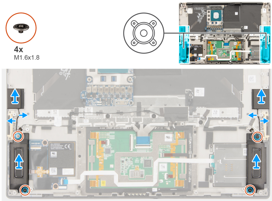
Abbildung 68. Entfernen der Lautsprecher
