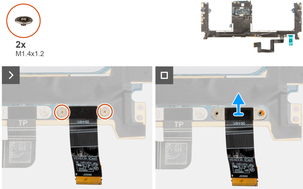
Abbildung 75. Entfernen des FPC-Kabels für die USH/SD-Karten-Zusatzplatine
