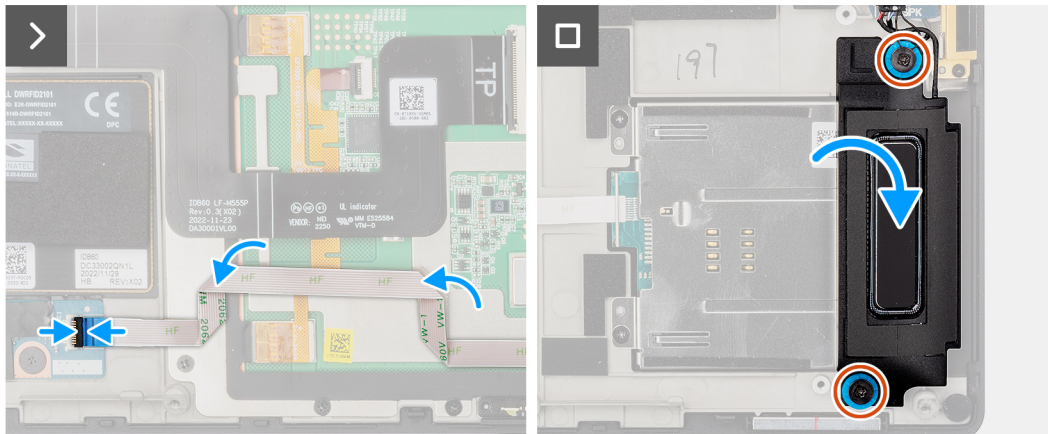
Abbildung 45. Installieren des Smartcardlesegeräts
