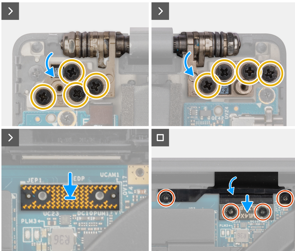
Abbildung 34. Installieren der Displaybaugruppe
