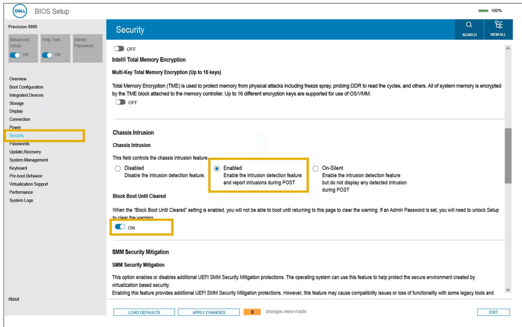
Abbildung 83. Löschen von Gehäuseeingriffswarnungen
