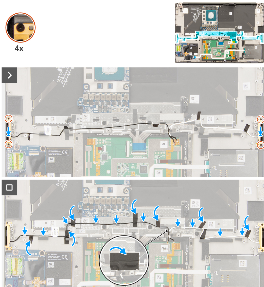
Abbildung 78. Installieren des WLAN-Antennenmoduls
