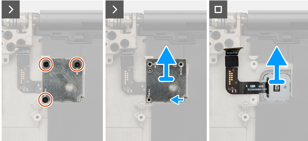
Abbildung 79. Entfernen der Baugruppe aus Netzschalter und Fingerabdruck-Lesegerät
