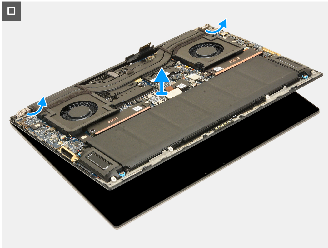
Abbildung 31. Entfernen der Displaybaugruppe
