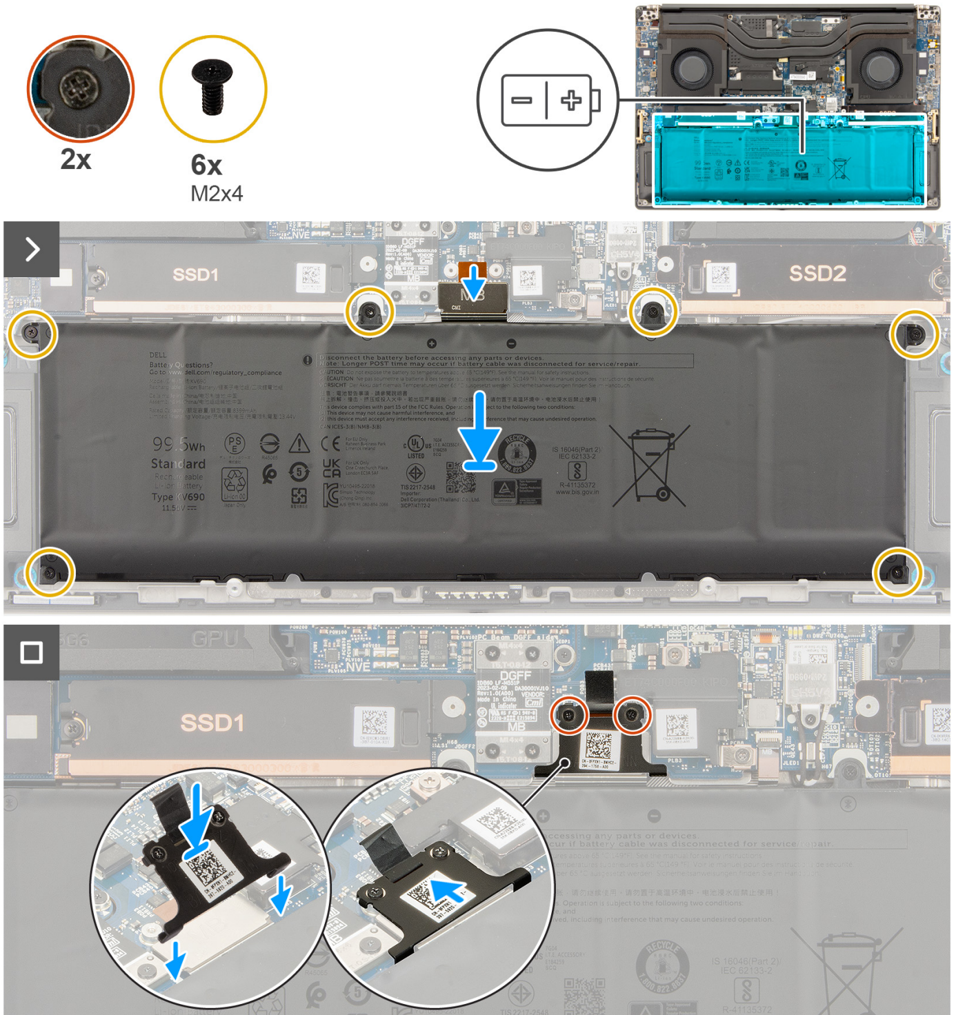
Abbildung 21. Installieren des Akkus
