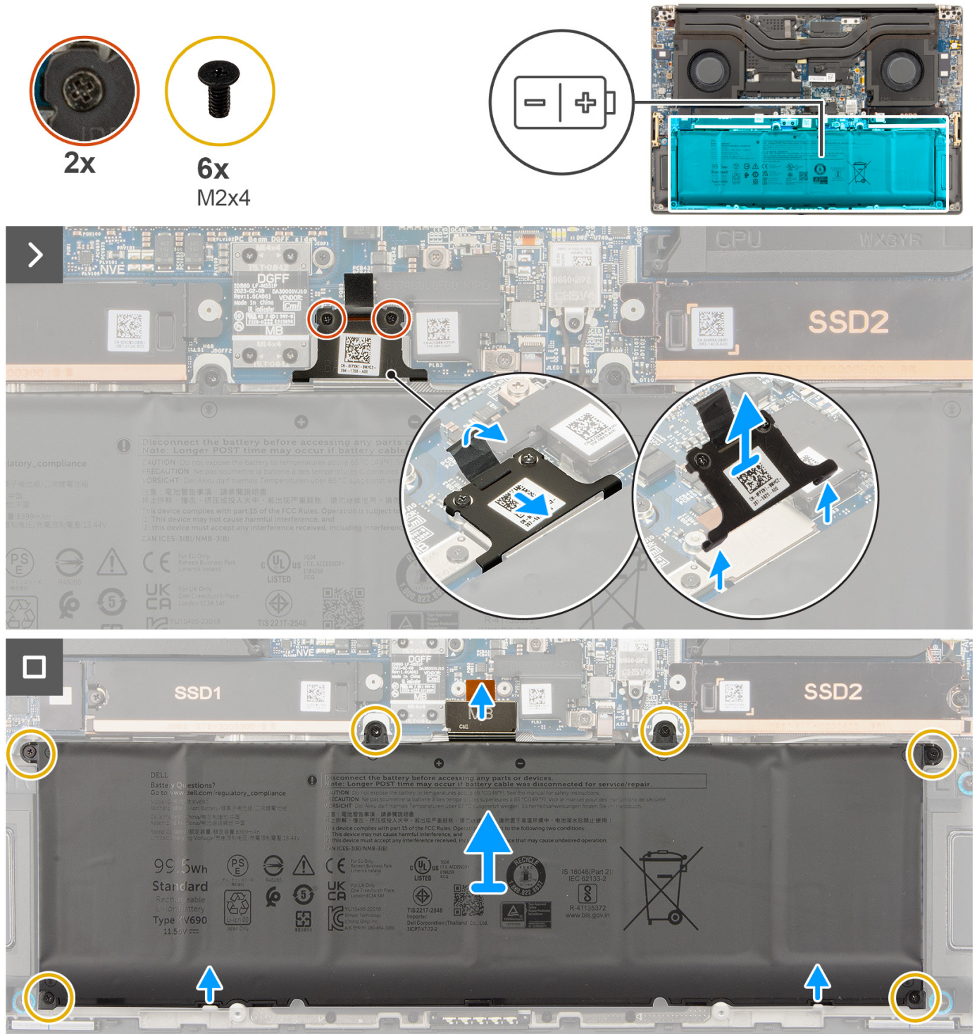
Abbildung 20. Entfernen des Akkus
