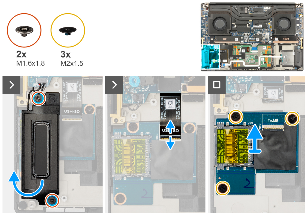
Abbildung 37. Entfernen der SD-Karten-Zusatzplatine
