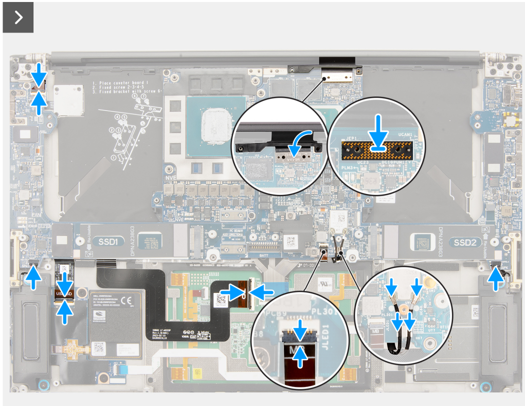
Abbildung 64. Installieren der Hauptplatine
