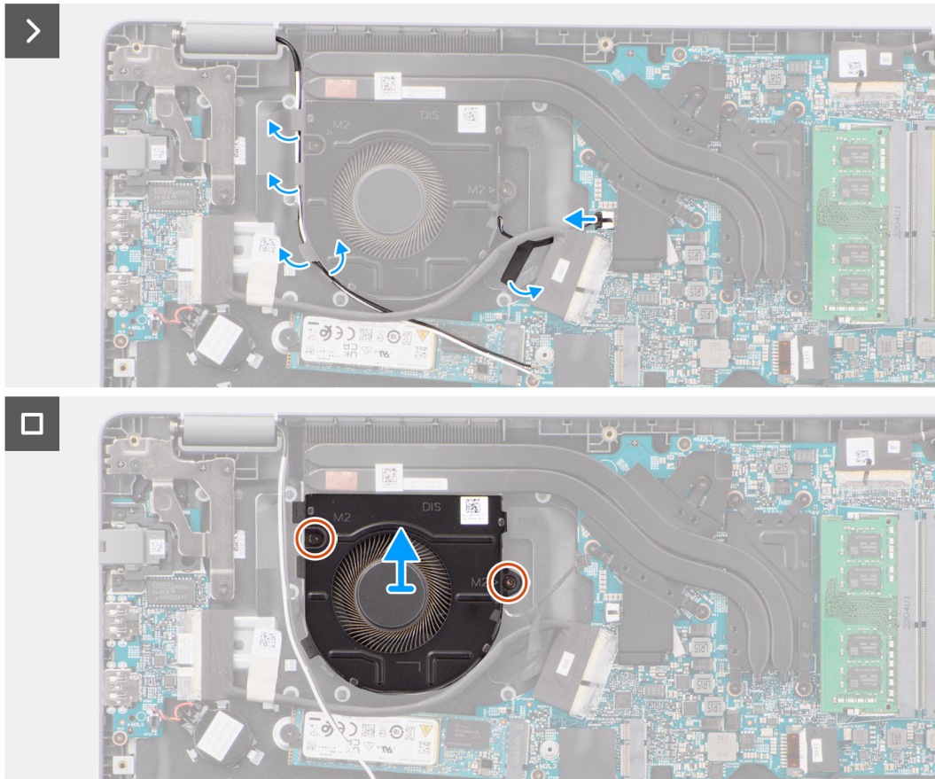
Afbeelding 33. De ventilator verwijderen
