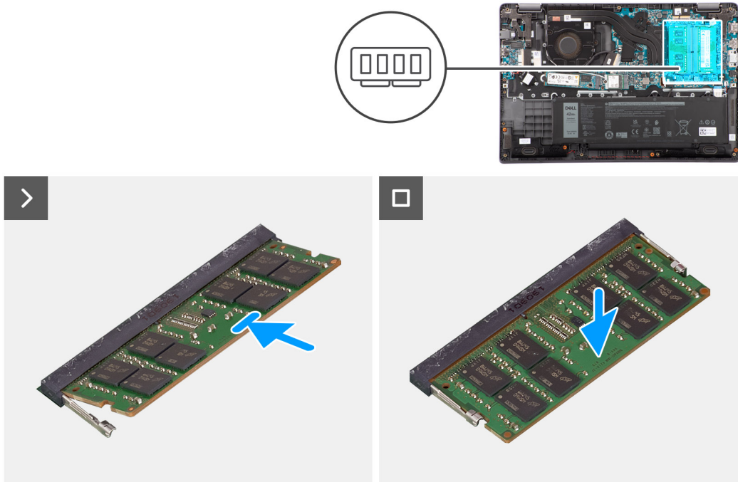
Afbeelding 12. De geheugenmodule verwijderen
