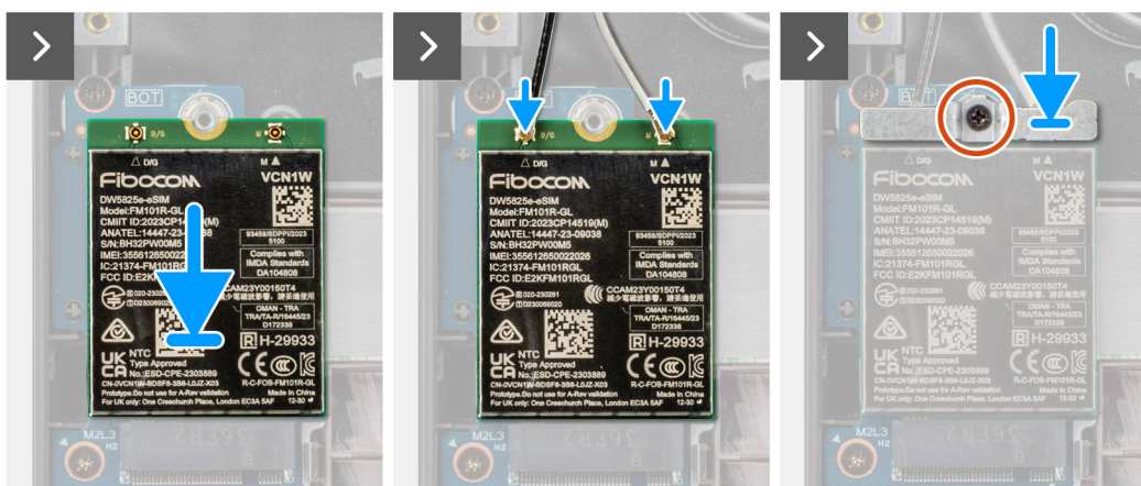
Afbeelding 17. De WWAN-kaart installeren
