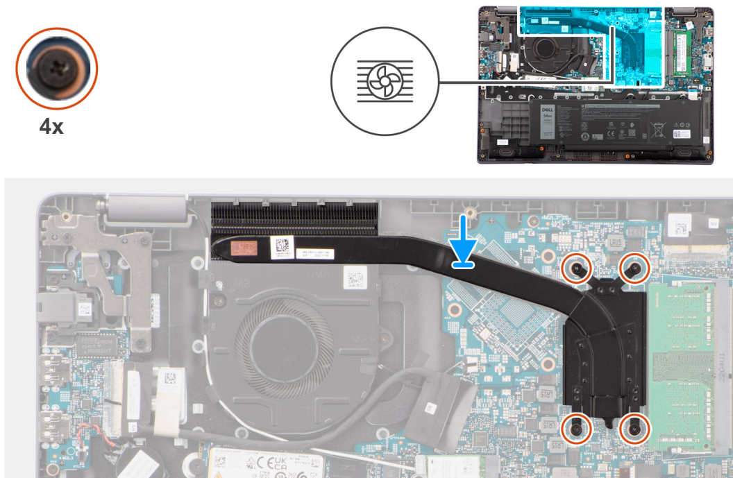
Afbeelding 30. De koelplaat van de geïntegreerde grafische kaart installeren
