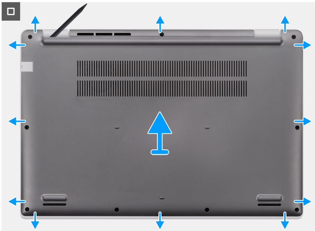
Afbeelding 9. De onderplaat verwijderen
