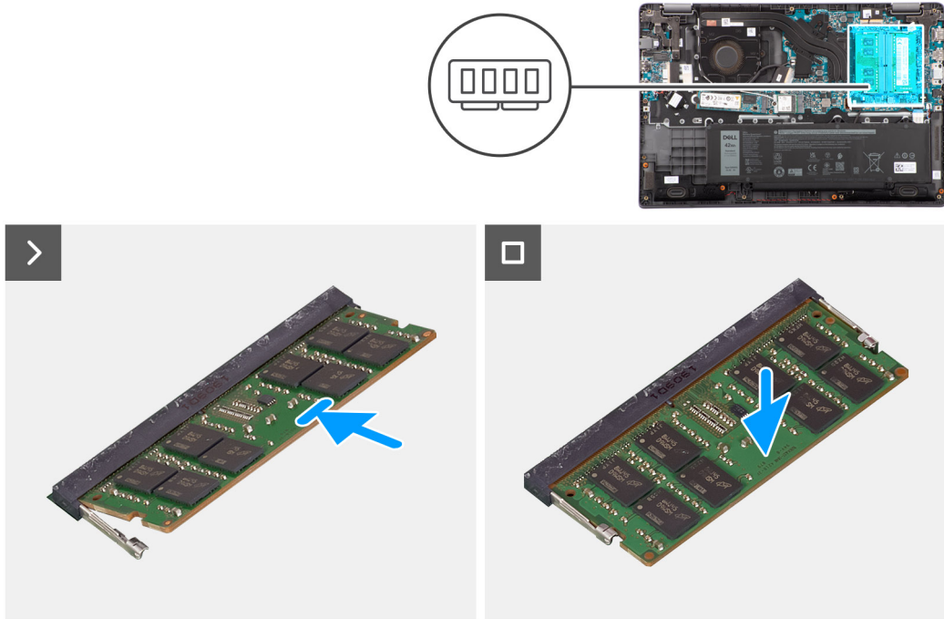
Afbeelding 13. De geheugenmodules plaatsen
