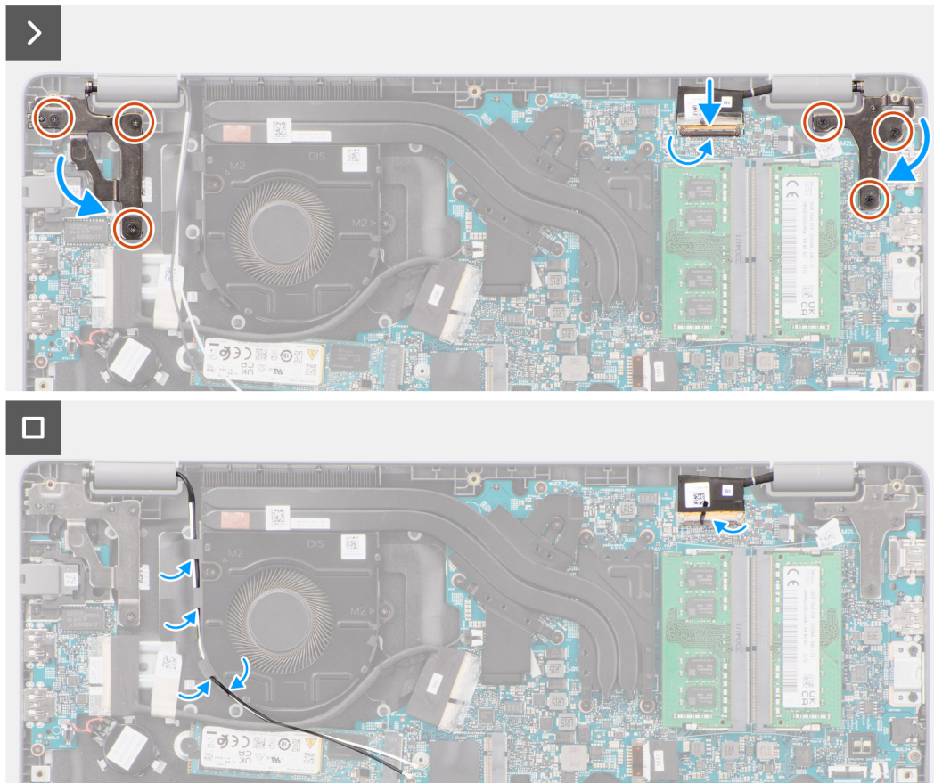
Afbeelding 52. De beeldschermenheid plaatsen
