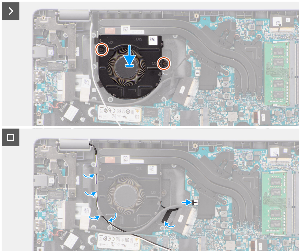
Obrázek 34. Montáž ventilátoru
