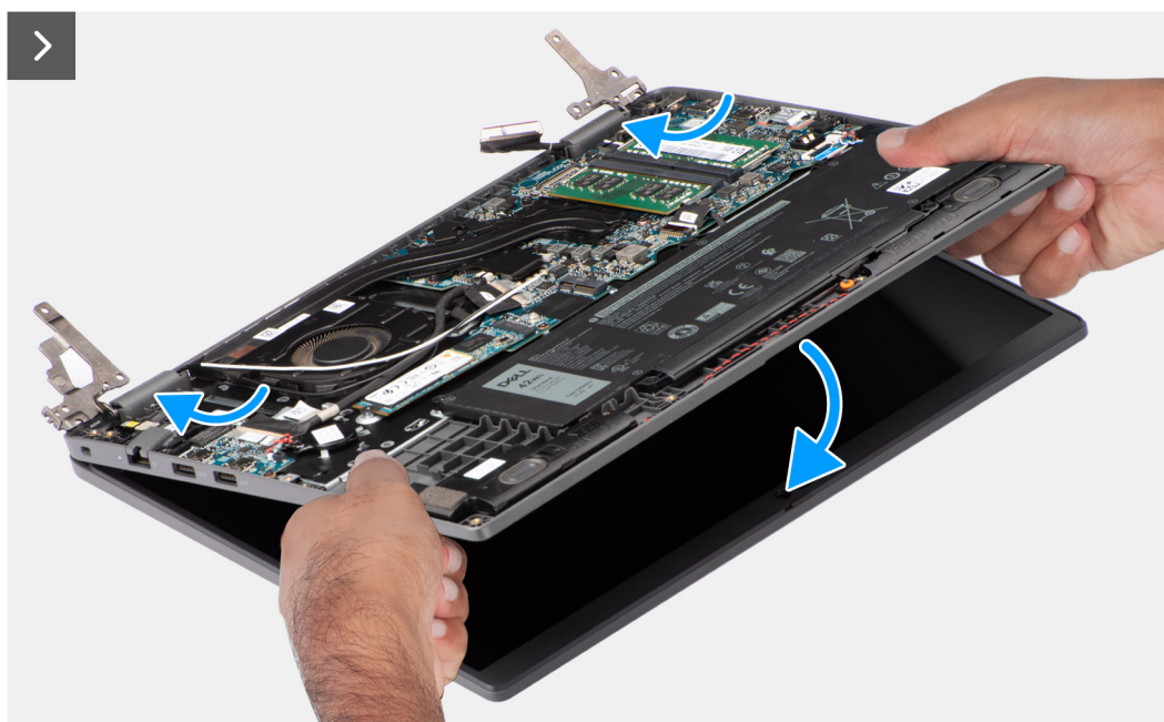
Obrázek 51. Montáž sestavy displeje
