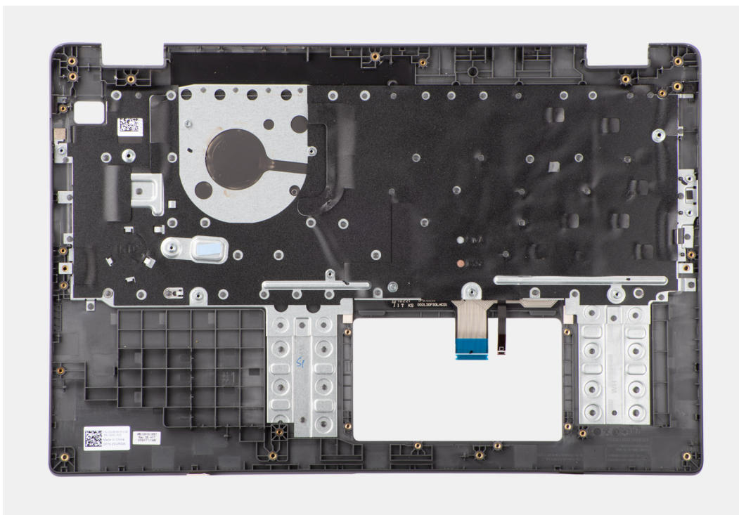
Obrázek 46. Demontáž sestavy opěrky pro dlaň a klávesnice
