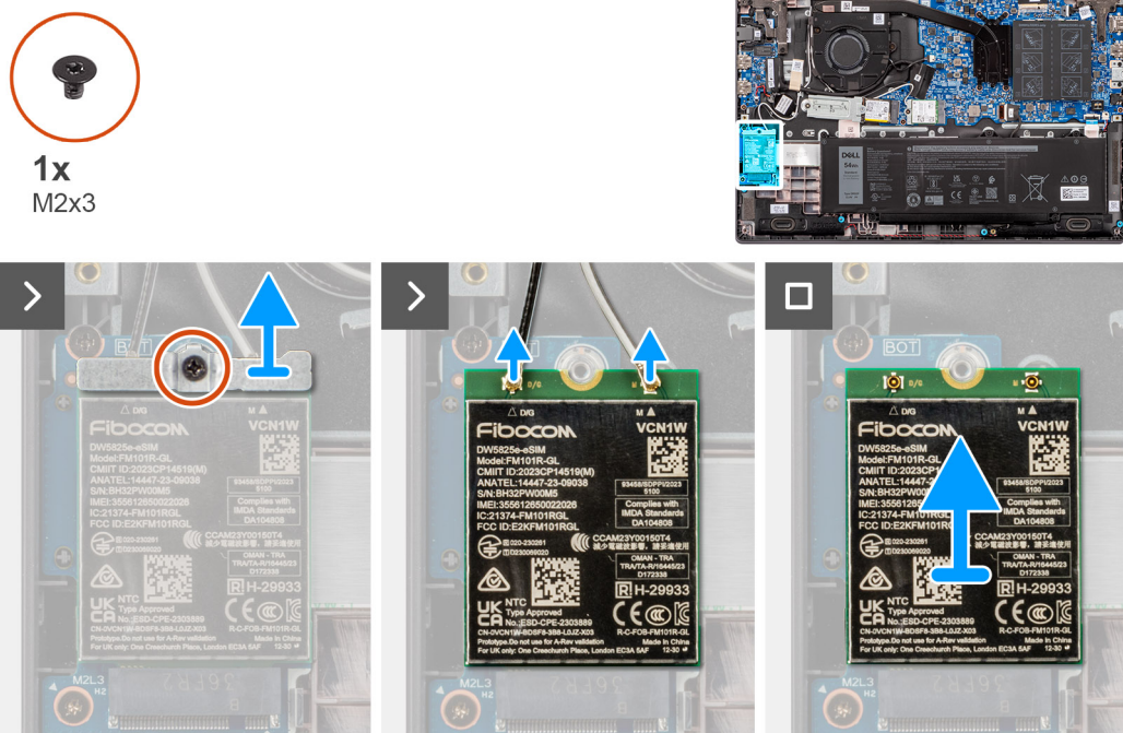
Obrázek 16. Vyjmutí karty sítě WWAN
