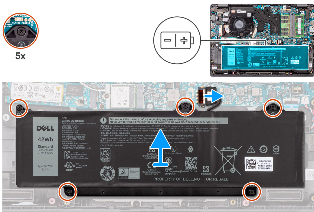
Obrázek 24. Vyjmutí baterie
