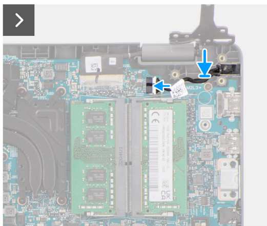
Obrázek 28. Montáž portu napájecího adaptéru
