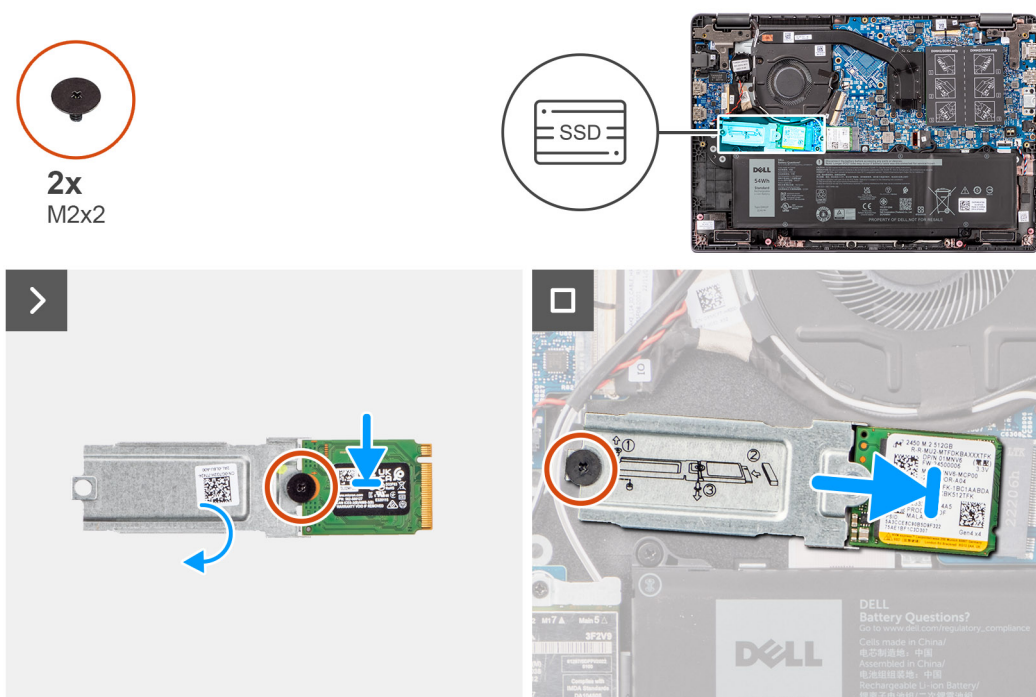
Obrázek 23. Montáž disku SSD M.2 2230
