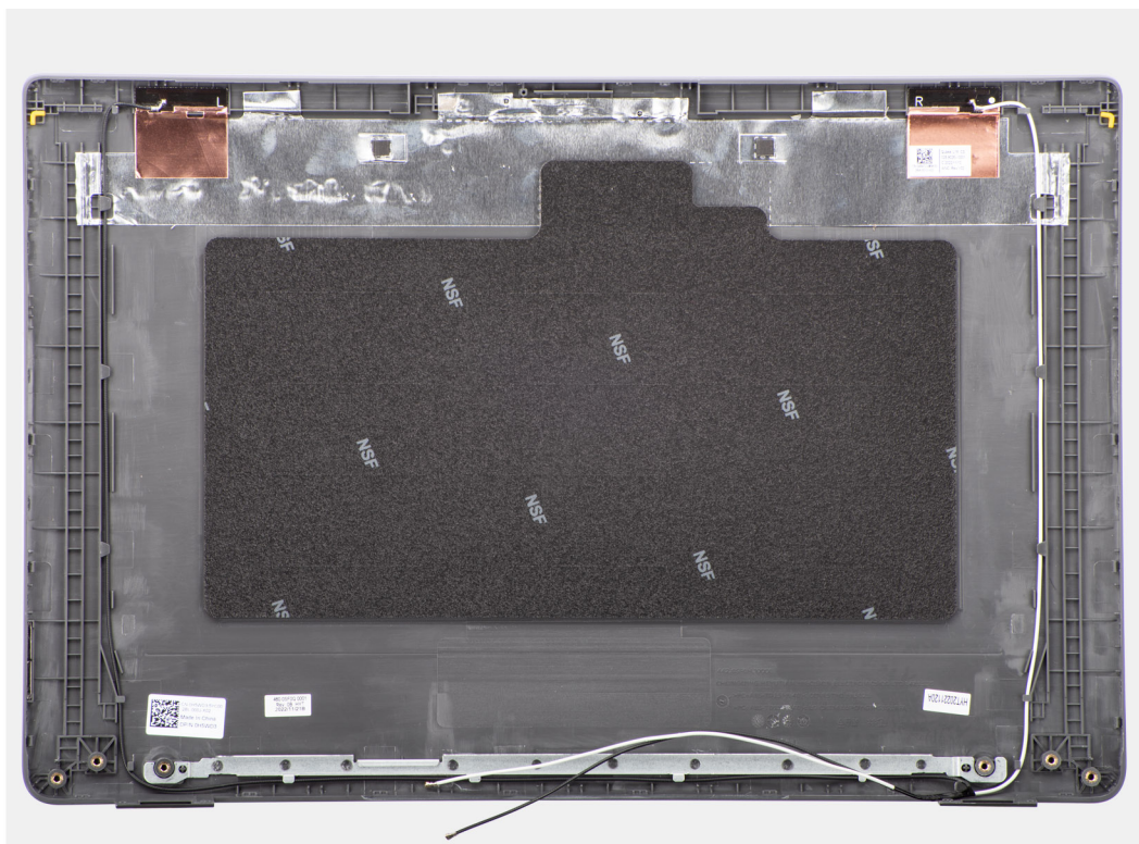
Obrázek 70. Demontáž zadního krytu displeje
