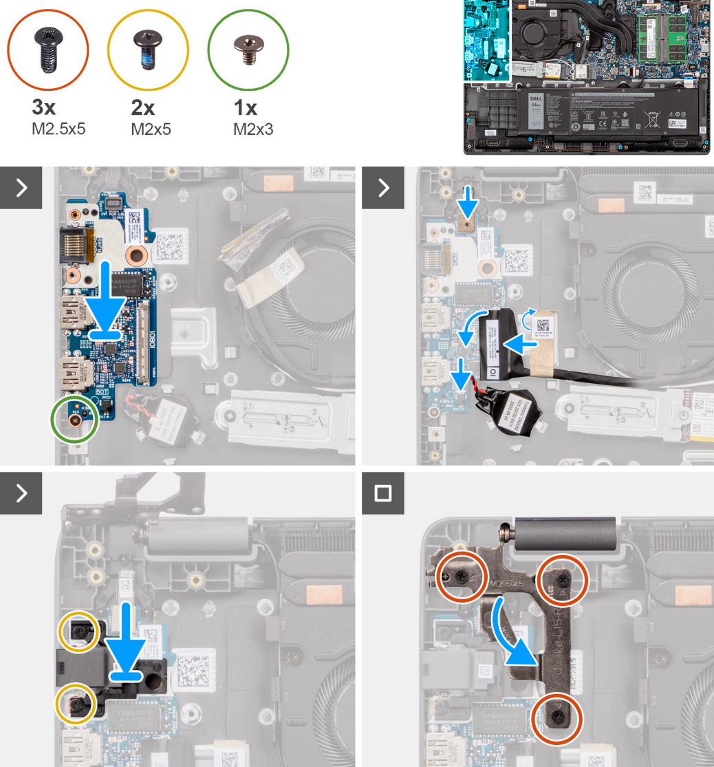
Obrázek 38. Vložení desky I/O
