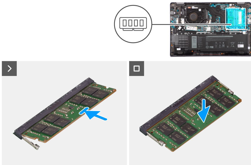
Obrázek 12. Vyjmutí paměťového modulu
