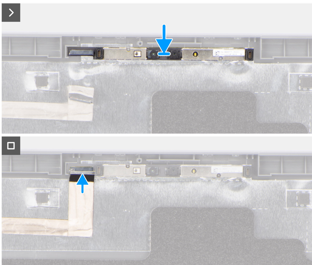
Obrázek 67. Montáž kamery
