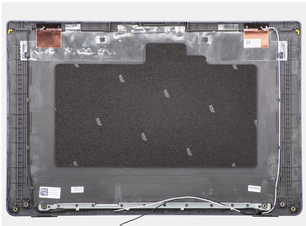
Obrázek 71. Montáž zadního krytu displeje
