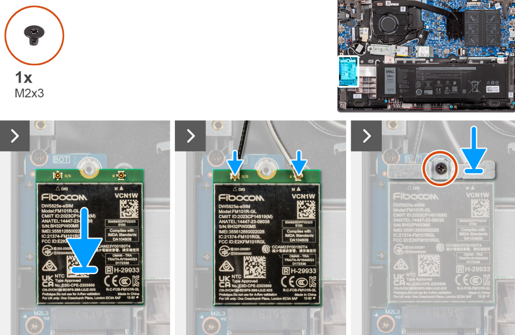
Obrázek 17. Montáž karty sítě WWAN
