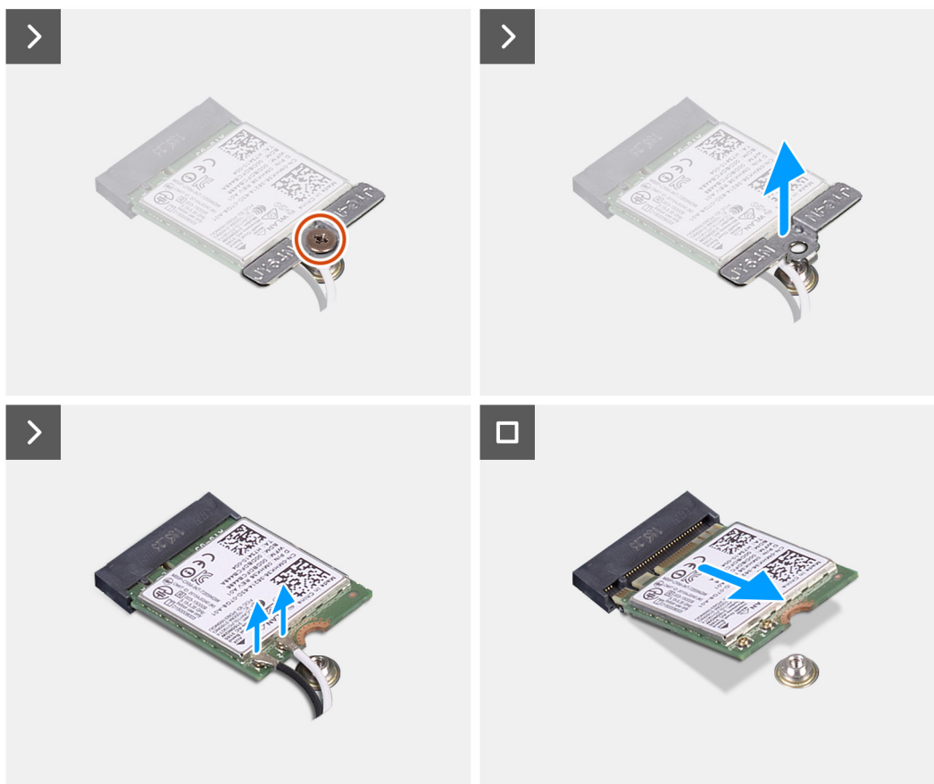
Obrázek 14. Demontáž bezdrátové karty
