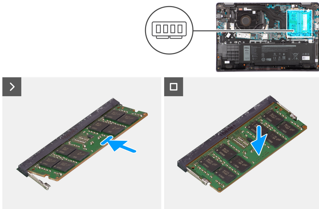
Obrázek 13. Vložení paměťových modulů
