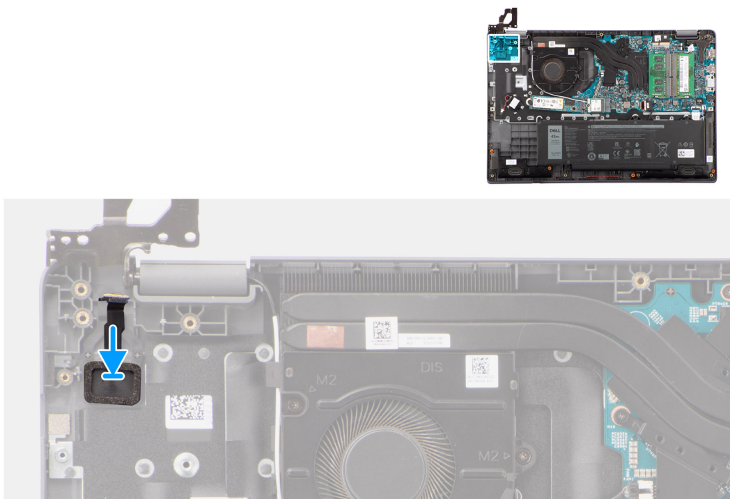
Obrázek 40. Montáž vypínače
