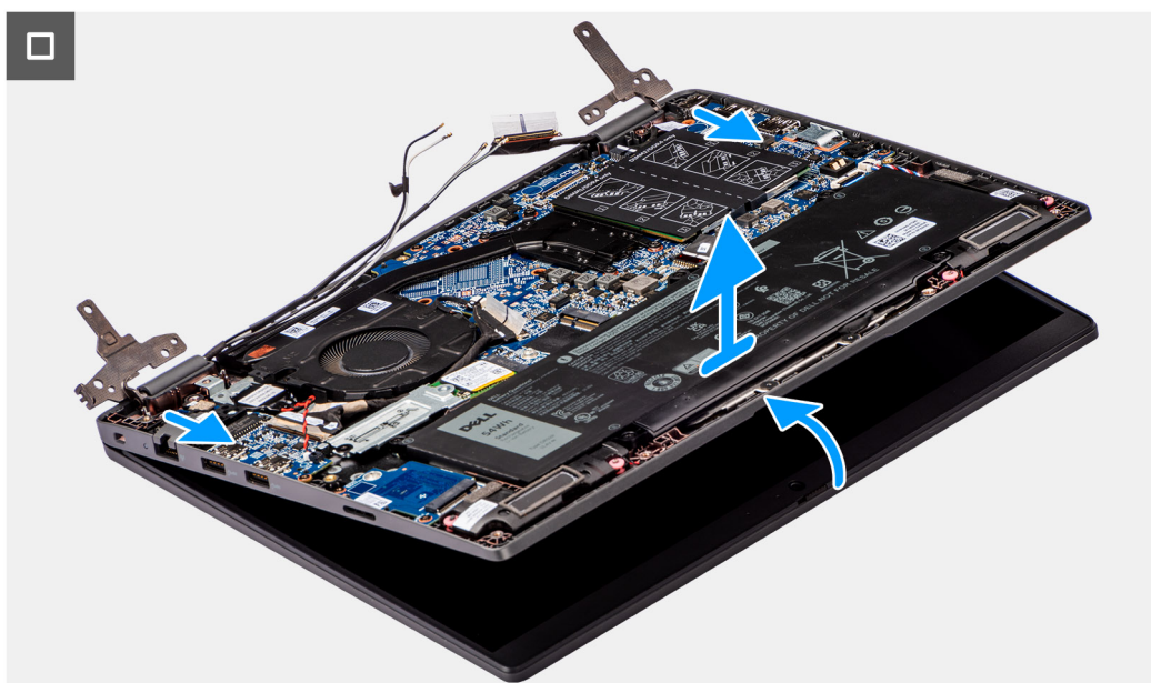
Obrázek 49. Demontáž sestavy displeje
