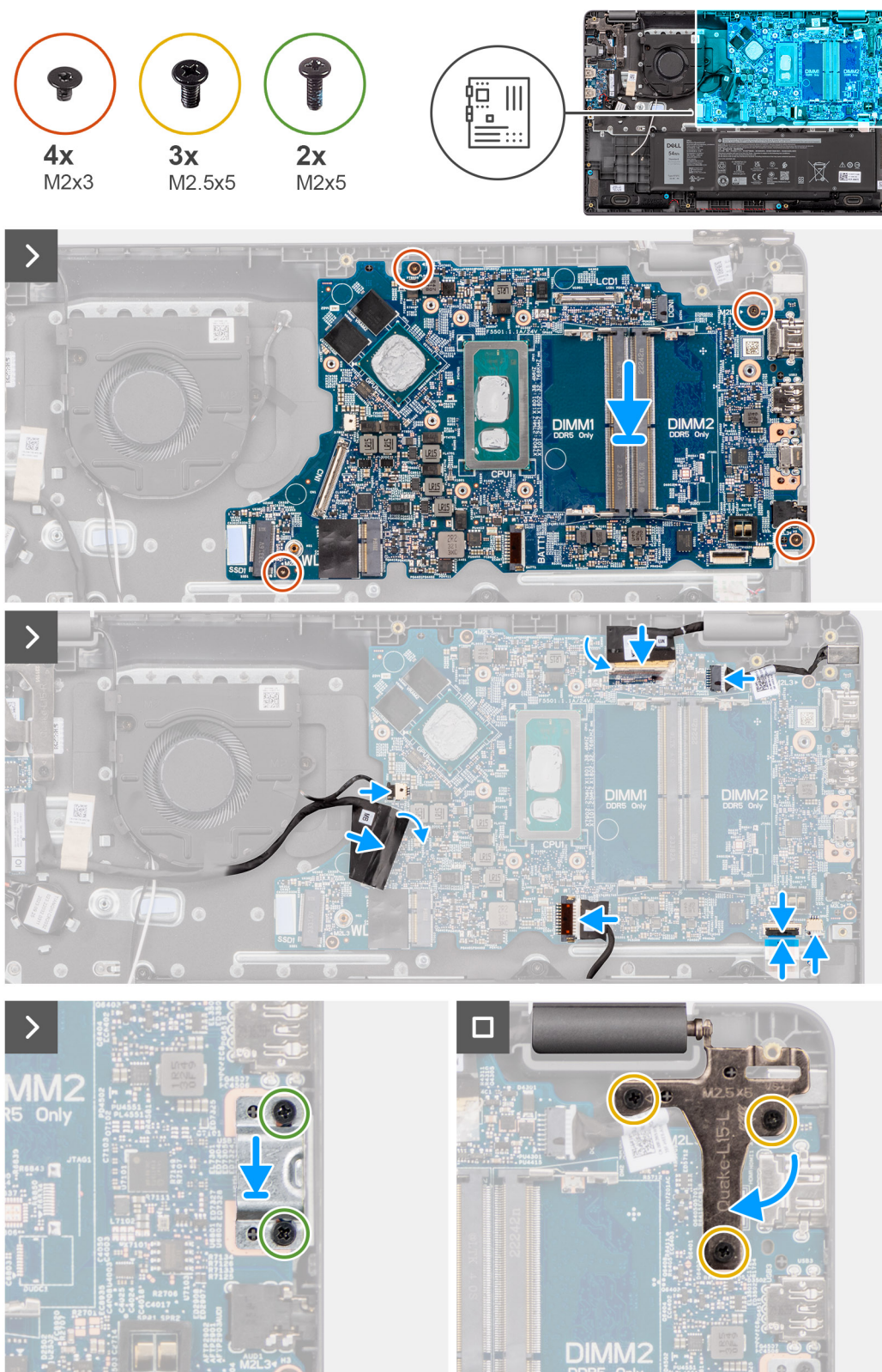
Obrázek 45. Montáž základní desky
