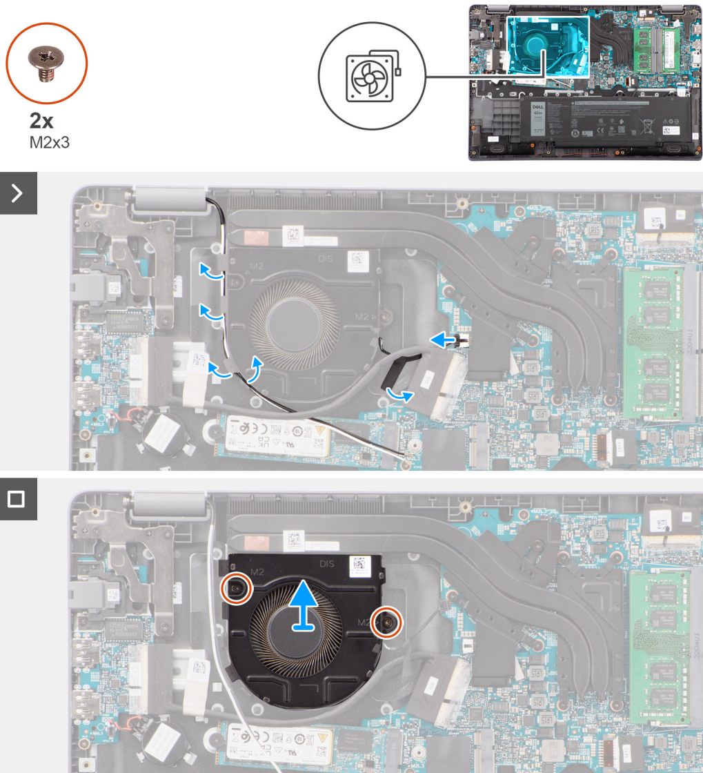
Obrázek 33. Demontáž ventilátoru
