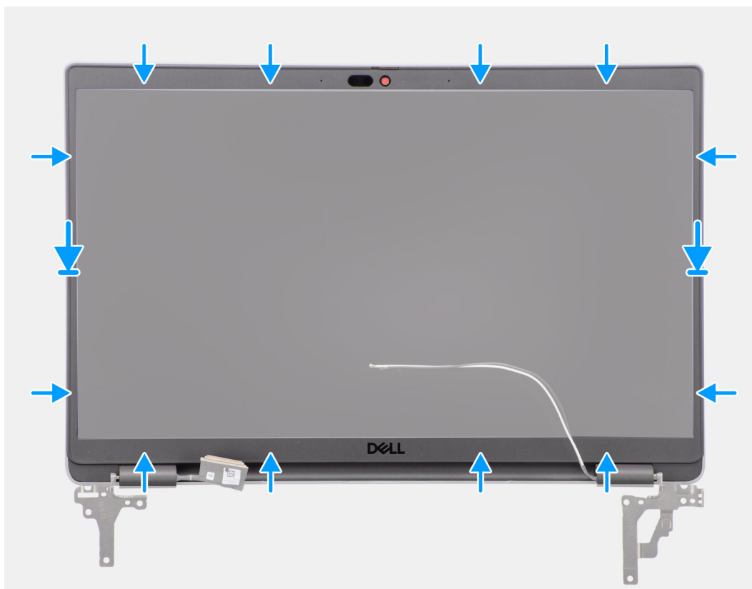
Obrázek 54. Montáž čelního krytu displeje
