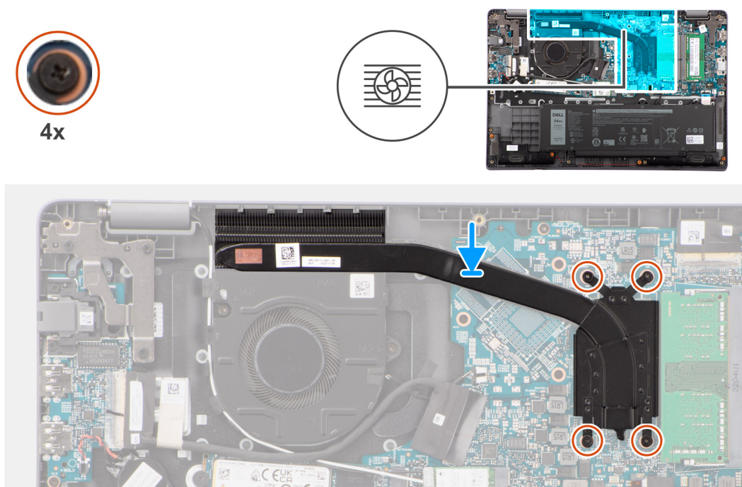
Obrázek 30. Montáž chladiče pro integrované grafické karty
