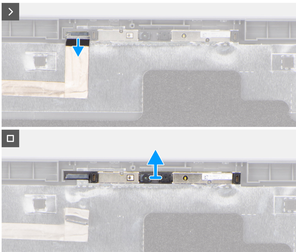
Obrázek 66. Demontáž kamery
