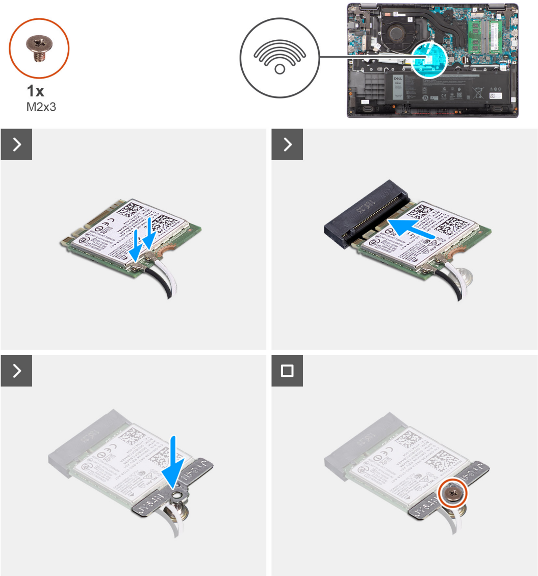
Obrázek 15. Montáž bezdrátové karty
