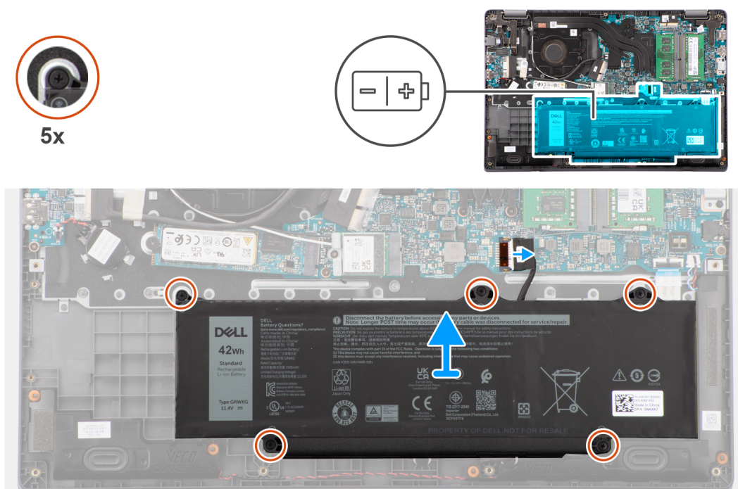
Obrázek 24. Vyjmutí baterie
