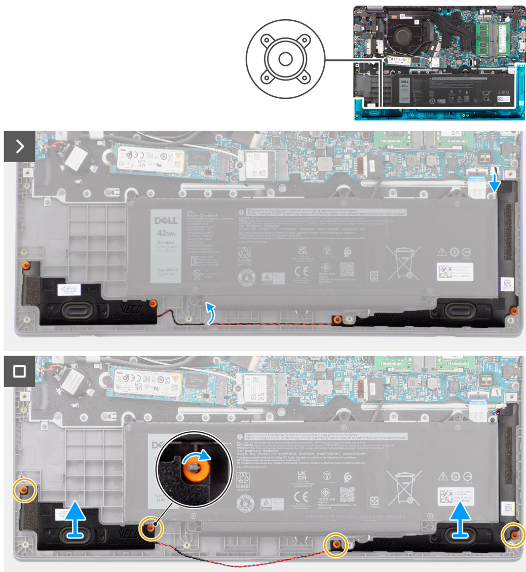
Obrázek 20. Demontáž reproduktorů
