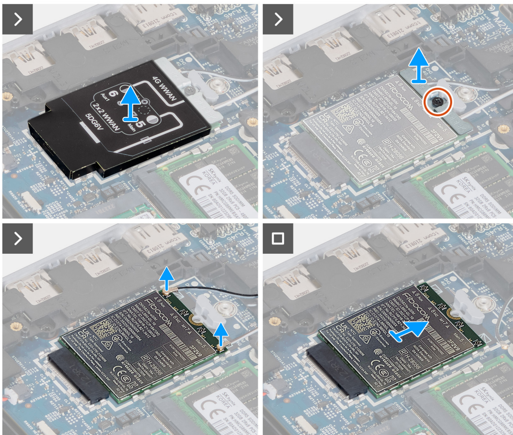
Afbeelding 21. De 4G WWAN-kaart verwijderen
