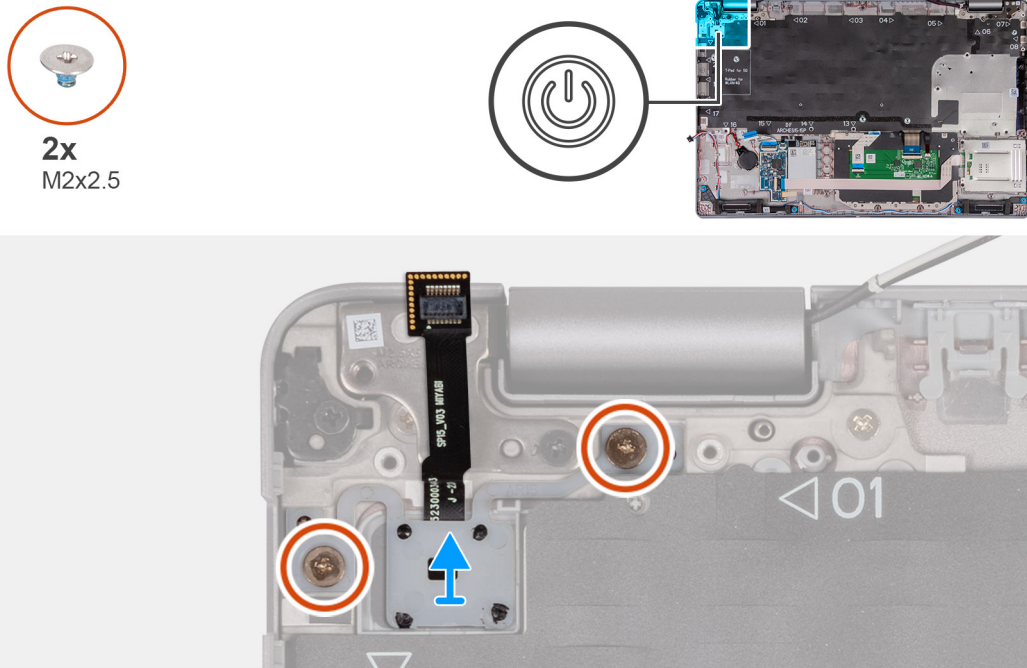
Afbeelding 65. De aan/uit-knop verwijderen
