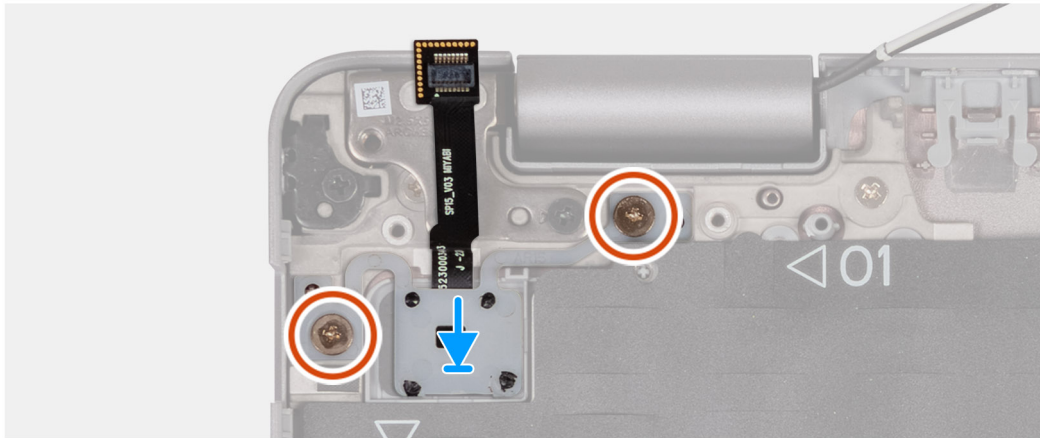
Afbeelding 66. De aan/uit-knop plaatsen
