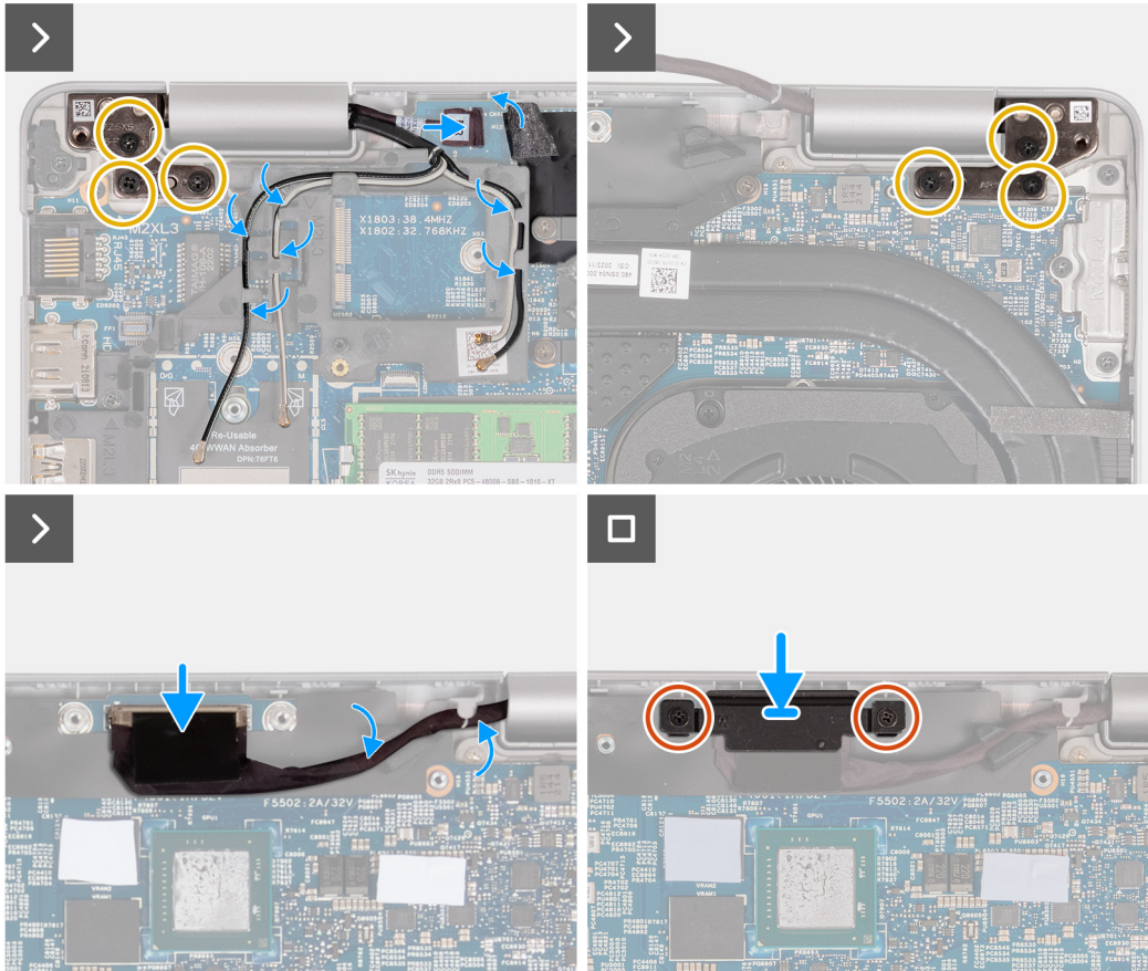
Afbeelding 77. De beeldschermenheid plaatsen
