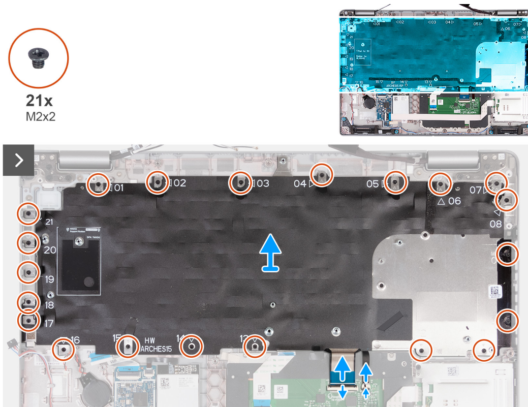
Afbeelding 69. Het toetsenbord verwijderen
