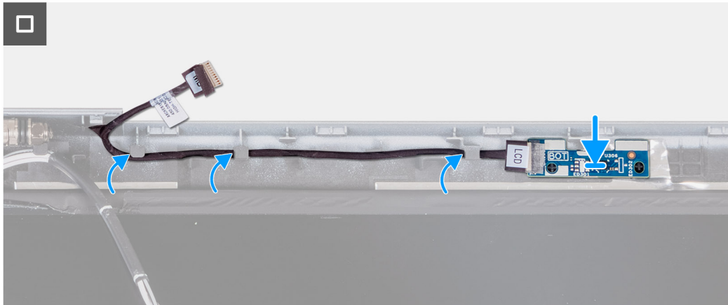
Afbeelding 97. De sensorkaart plaatsen
