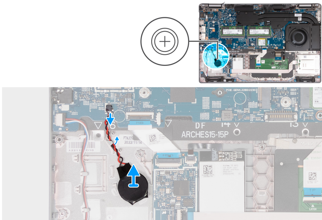
Afbeelding 50. De knoopcelbatterij verwijderen
