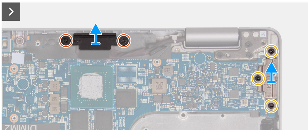
Afbeelding 57. De systeemkaart verwijderen
