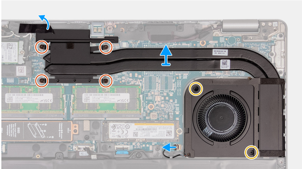
Afbeelding 54. De ventilator- en koelplaateneheid verwijderen (geïntegreerde GPU)
