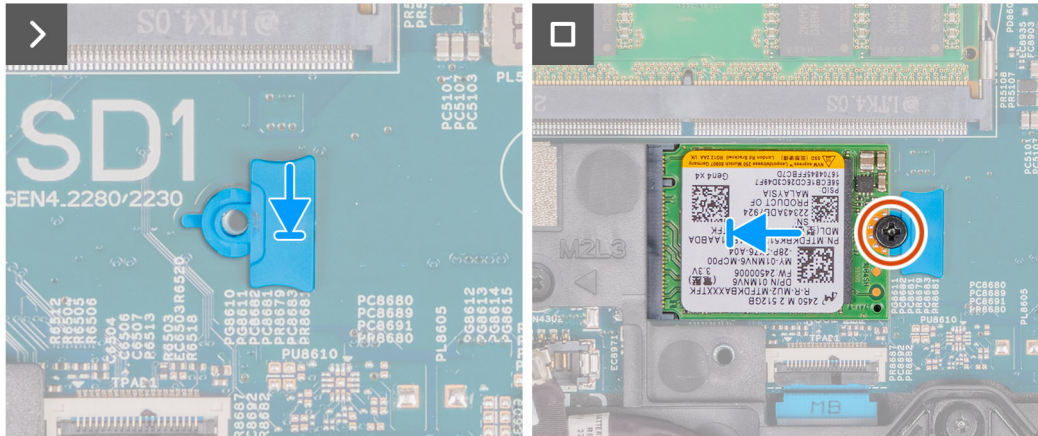
Afbeelding 28. De M.2 2230 SSD in slot 1 installeren
