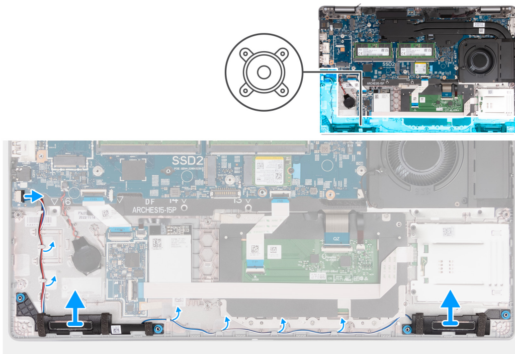
Afbeelding 47. De luidsprekers verwijderen
