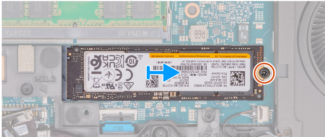
Afbeelding 29. De M.2 2280 SSD verwijderen uit slot 1
