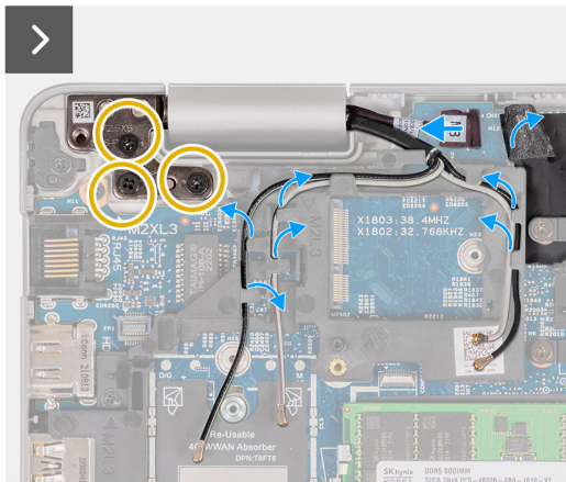
Afbeelding 73. De beeldschermenunit verwijderen
