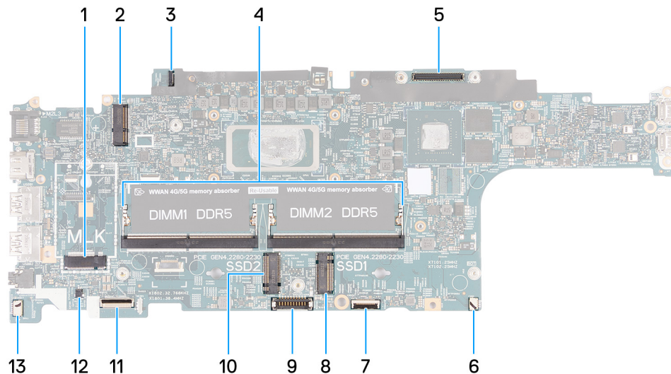
Afbeelding 61. Systeemkaartconnectoren
