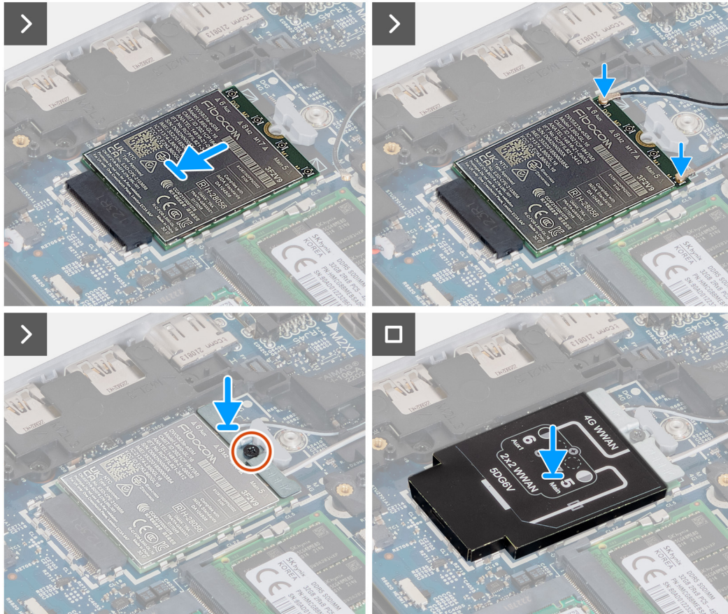
Afbeelding 22. De 4G WWAN-kaart installeren
