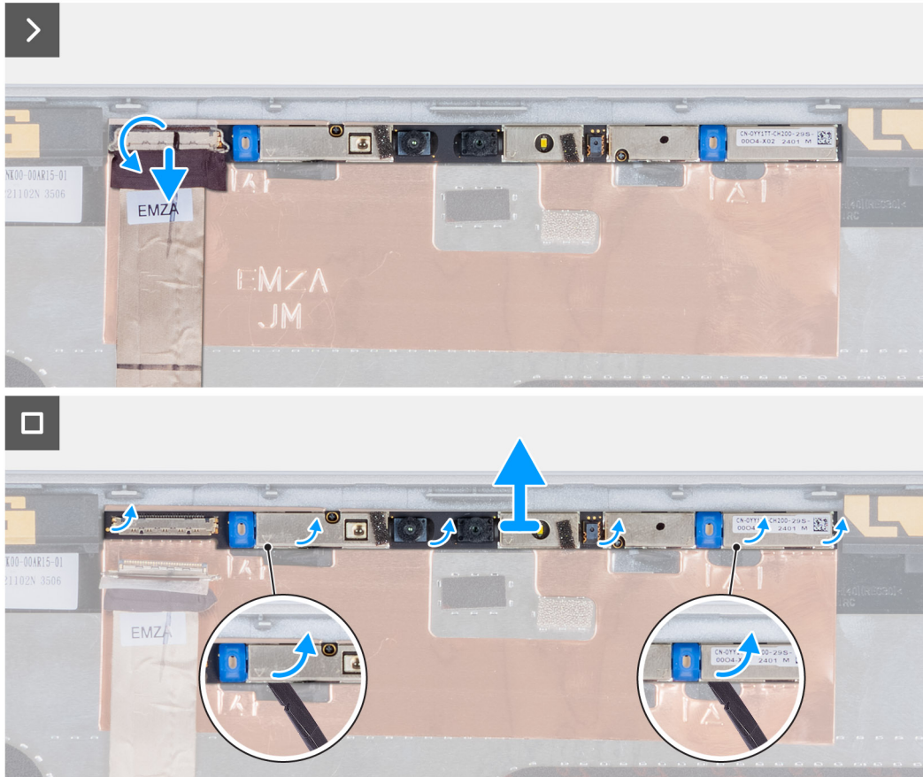
Afbeelding 88. De cameramodule verwijderen
