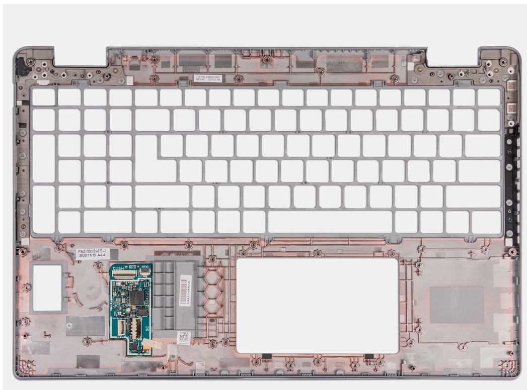
Afbeelding 102. De palmsteuneenheid verwijderen
