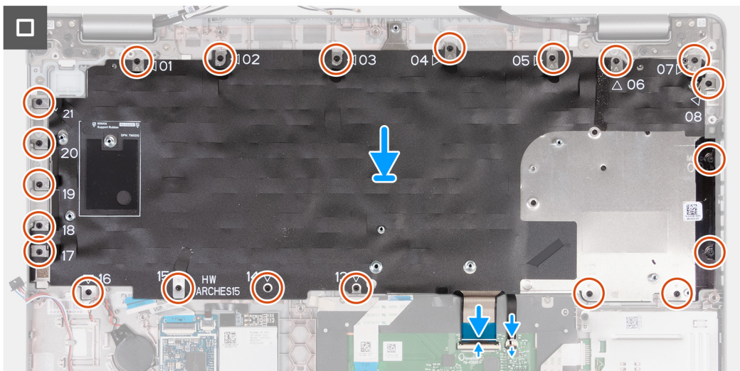
Afbeelding 72. Het toetsenbord plaatsen
