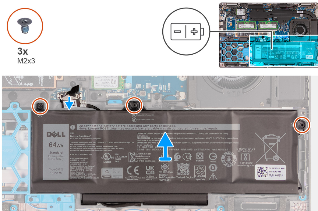
Afbeelding 37. De batterij verwijderen - 64 Whr
