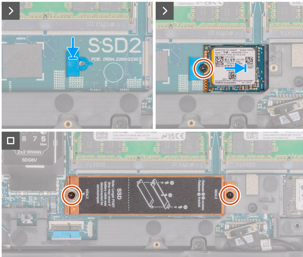
Afbeelding 32. De M.2 2230 SSD in slot 2 installeren
