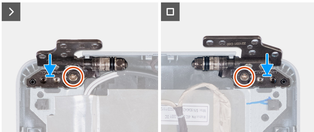
Afbeelding 91. De beeldschermcharnieren installeren
