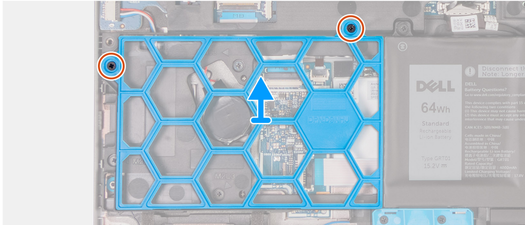
Afbeelding 35. Het plastic inzetstuk verwijderen
