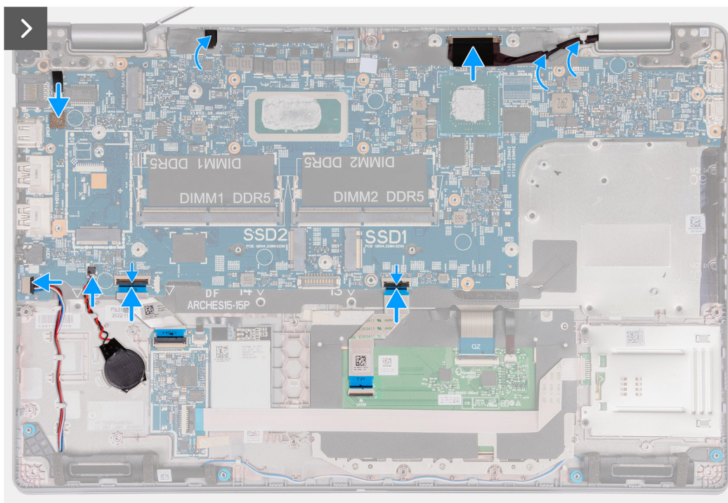
Afbeelding 63. De systeemkaart installeren
