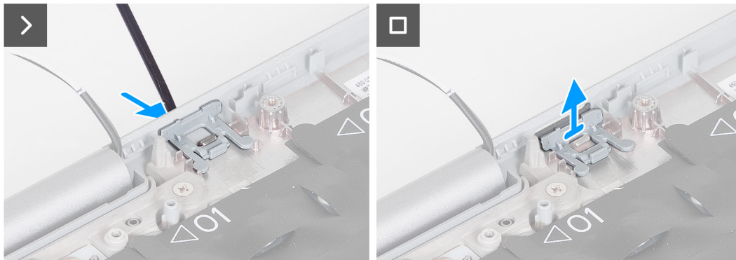
Afbeelding 100. De dummy simkaartslotvuller verwijderen
