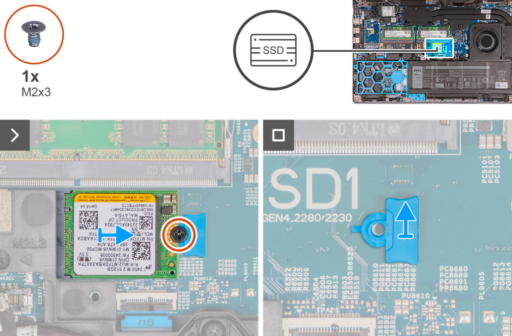
Afbeelding 27. De M.2 2230 SSD verwijderen uit slot 1
