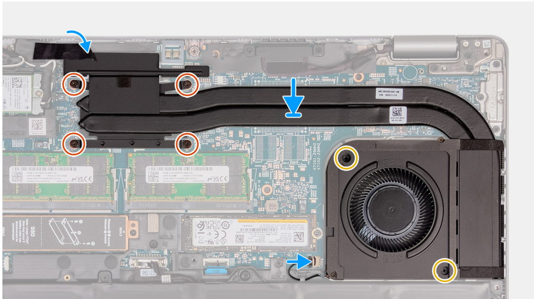
Afbeelding 55. De ventilator- en koelplaateneheid plaatsen (geïntegreerde GPU)
