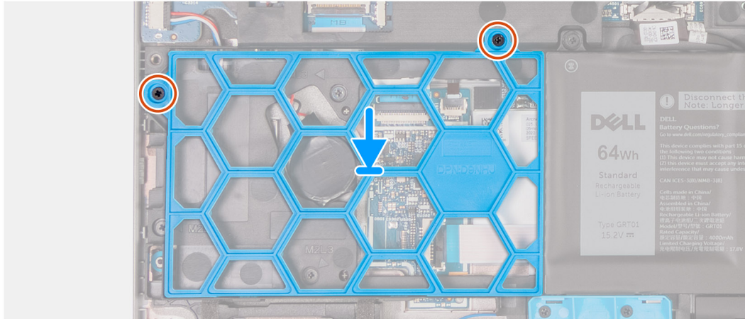
Afbeelding 36. Het plastic inzetstuk installeren
