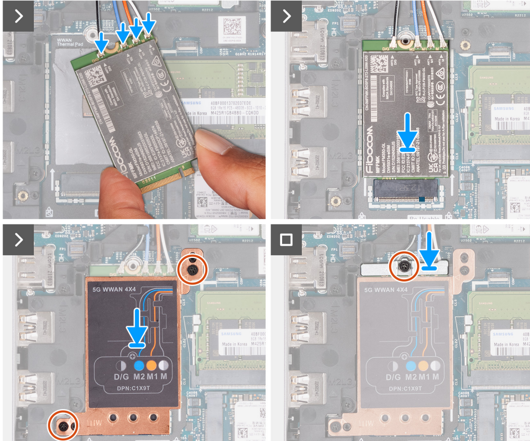
Afbeelding 24. De 5G WWAN-kaart installeren
