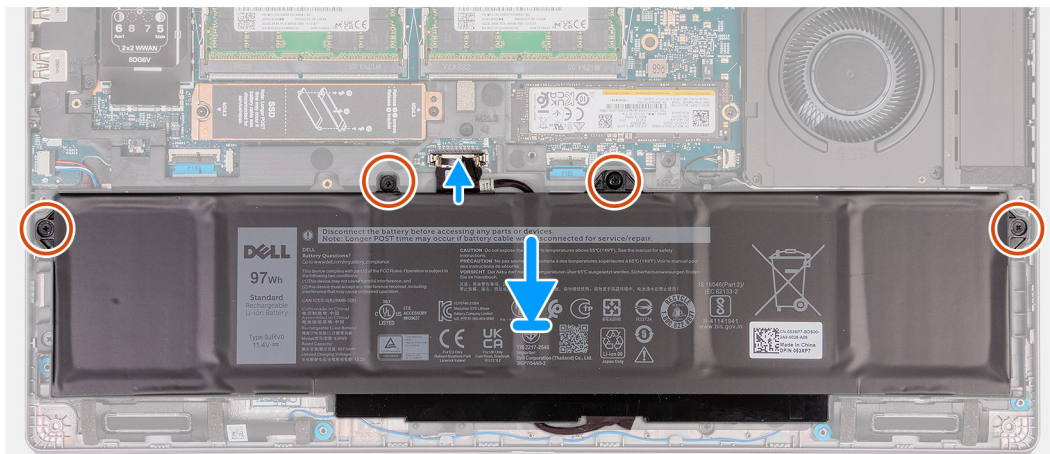
Afbeelding 40. De 97 Whr batterij installeren
