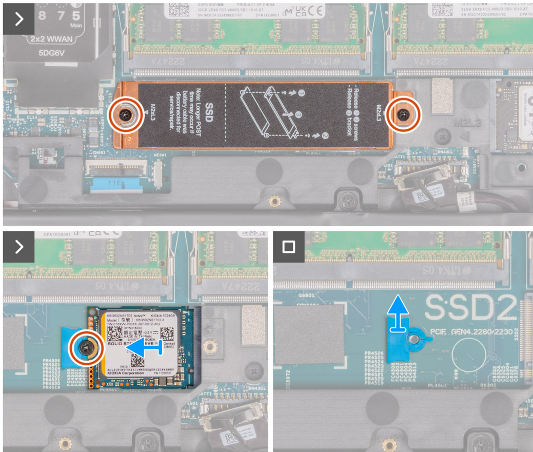
Afbeelding 31. De M.2 2230 SSD verwijderen uit slot 2
