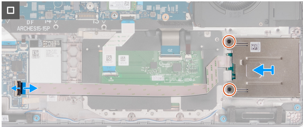
Afbeelding 98. De smartcardlezer verwijderen
