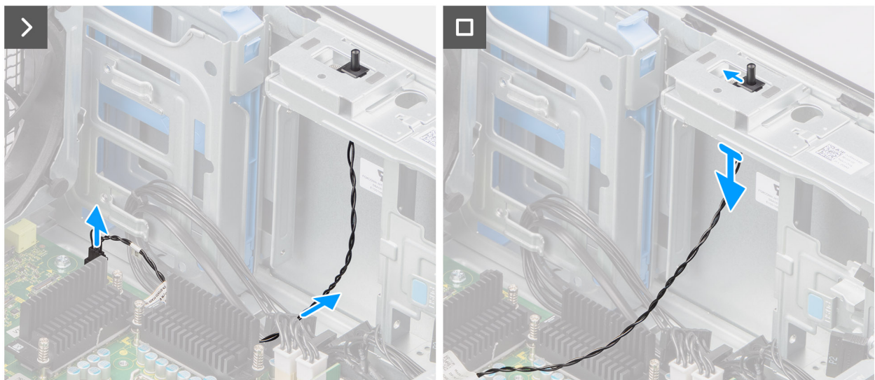
Figure 70. Retrait du commutateur d'intrusion
