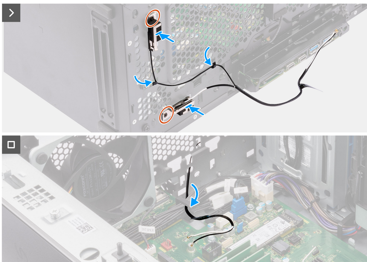
Figure 29. Installation de l'antenne interne WLAN
