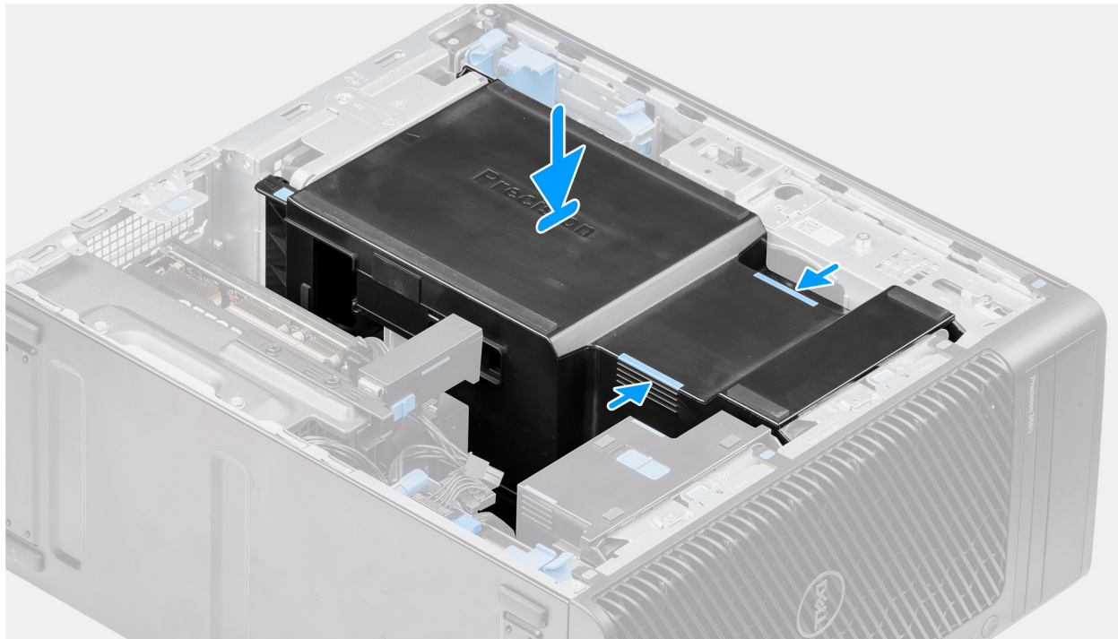
Figure 15. Installation du carénage à air
