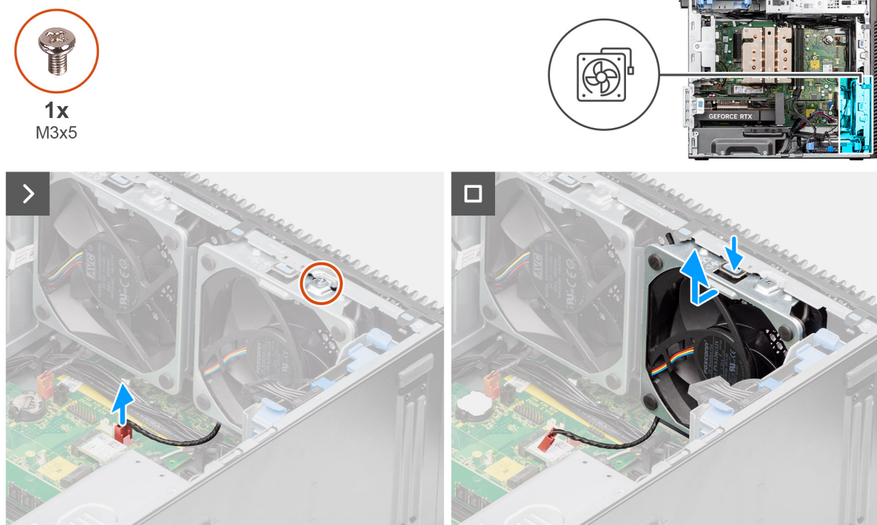
Figure 60. Ventilateur avant 1
