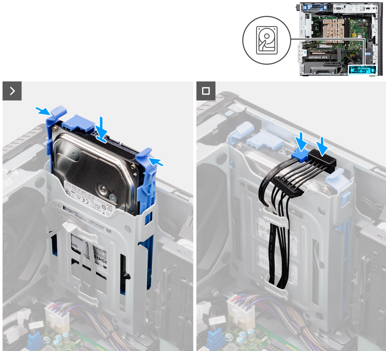
Figure 21. Installation de l'assemblage de disque dur de 3,5 pouces de la baie 1
