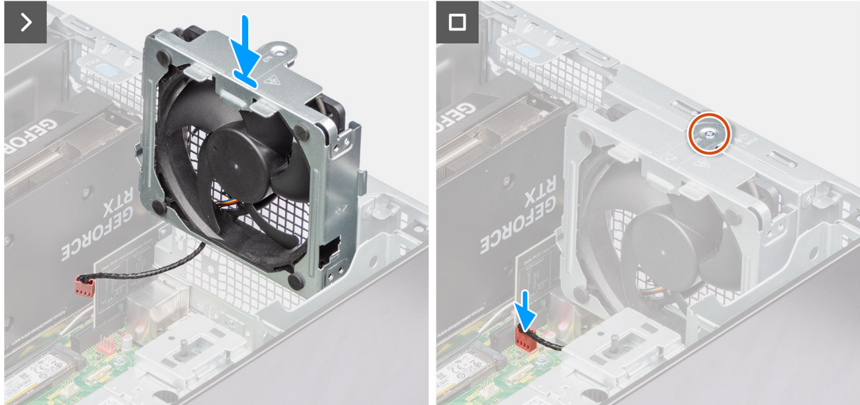
Figure 67. Installation du ventilateur arrière (bloc d'alimentation de 1 000 W)
