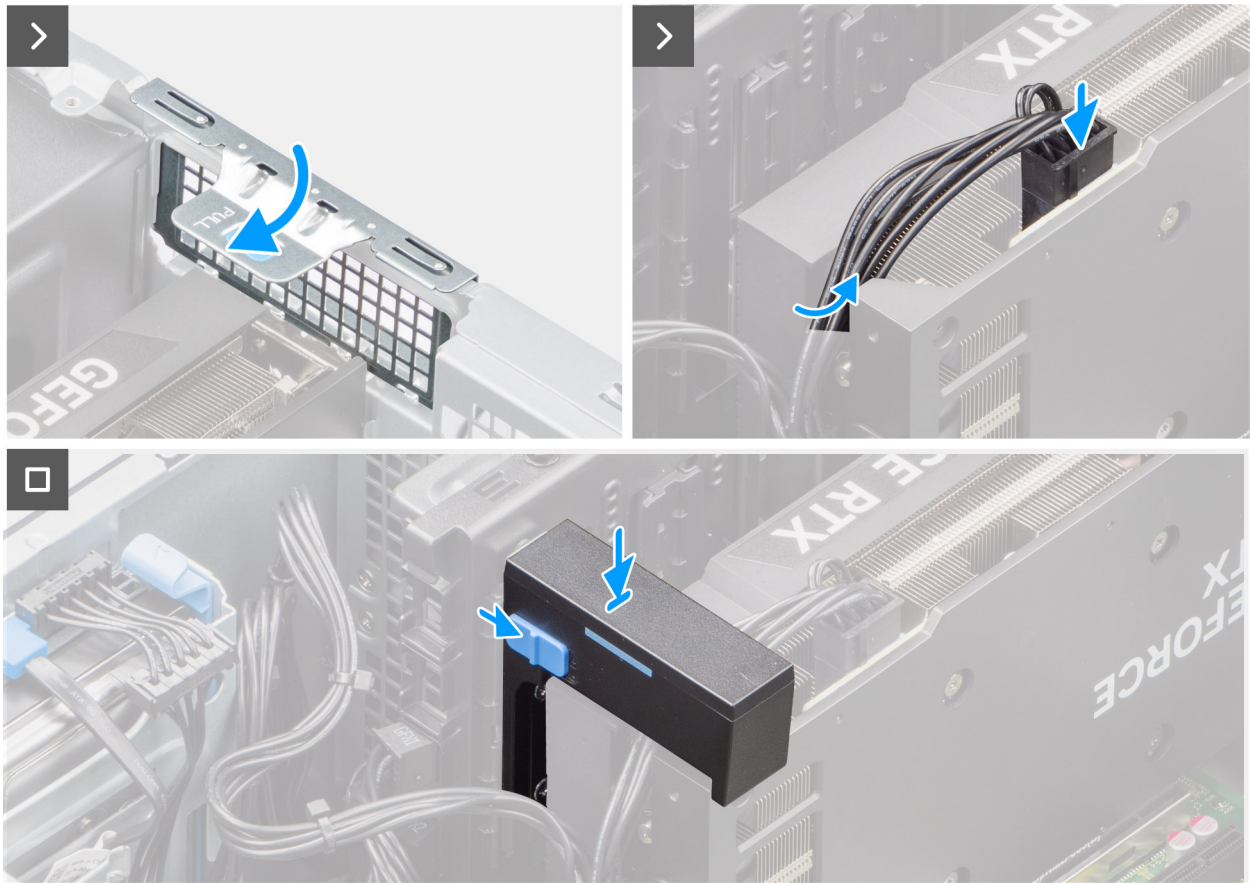
Figure 45. Installation du processeur graphique alimenté
