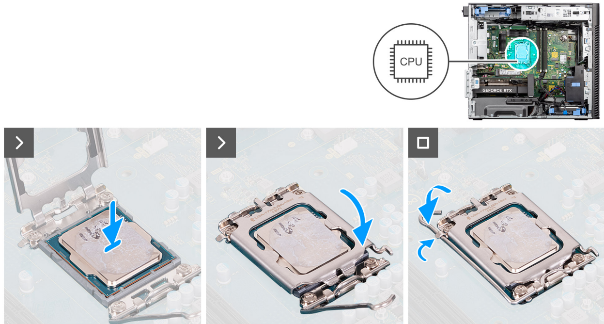
Figure 57. Installation du processeur
