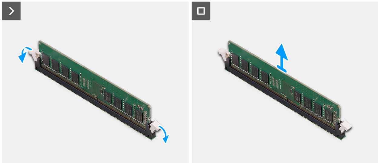
Figure 32. Retrait du module de mémoire
