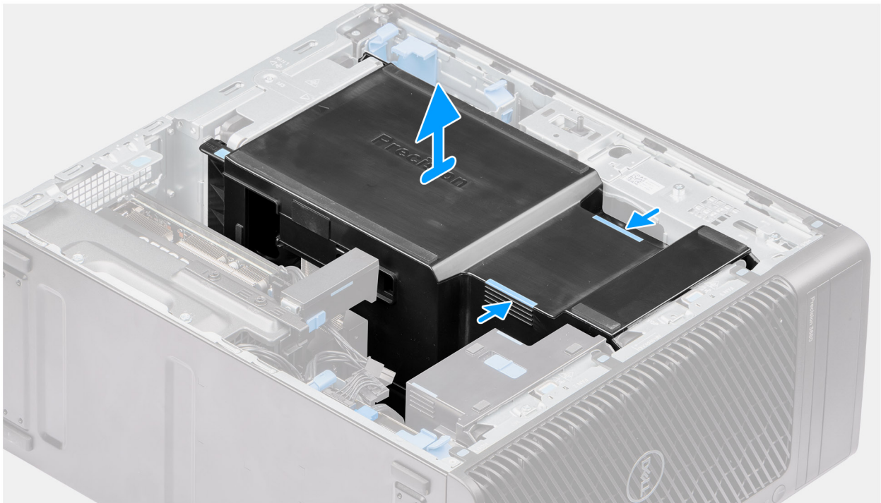
Figure 14. Retrait du carénage à air
