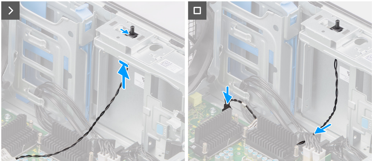
Figure 71. Installation du commutateur d'intrusion
