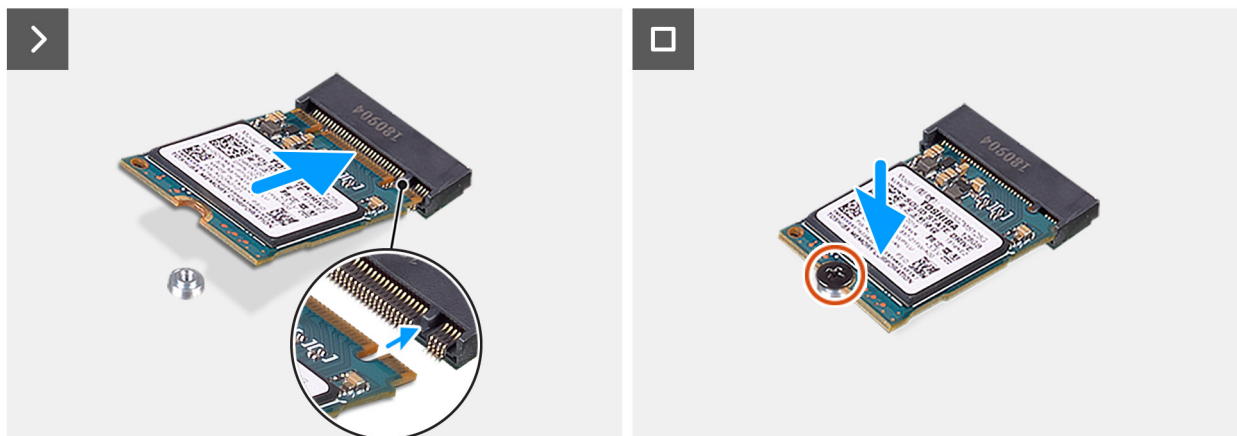
Figure 23. Installation du disque SSD M.2 2230 PCIe
