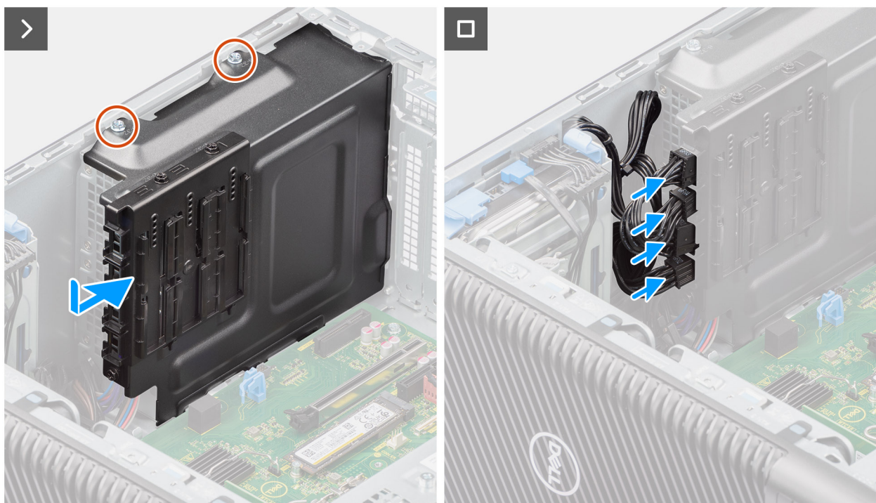
Figure 47. Installation du capot du bloc d'alimentation
