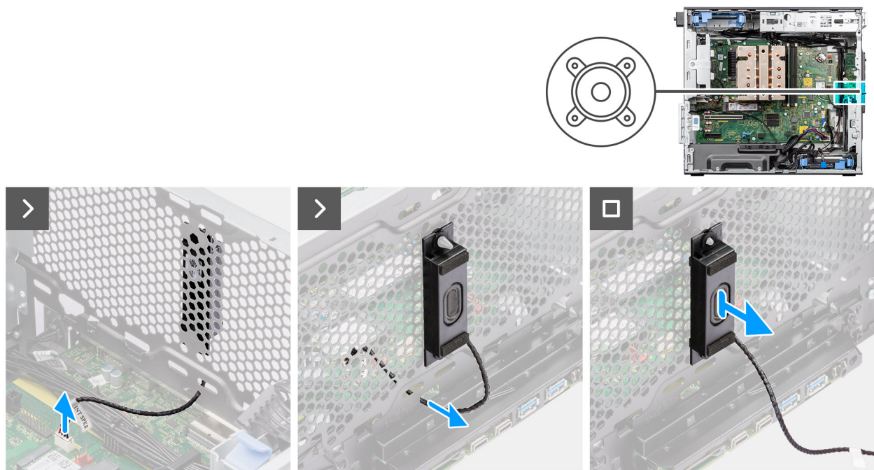
Figure 72. Retrait du haut-parleur interne
