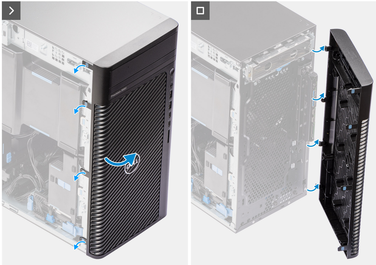
Figure 12. Retrait du panneau avant
