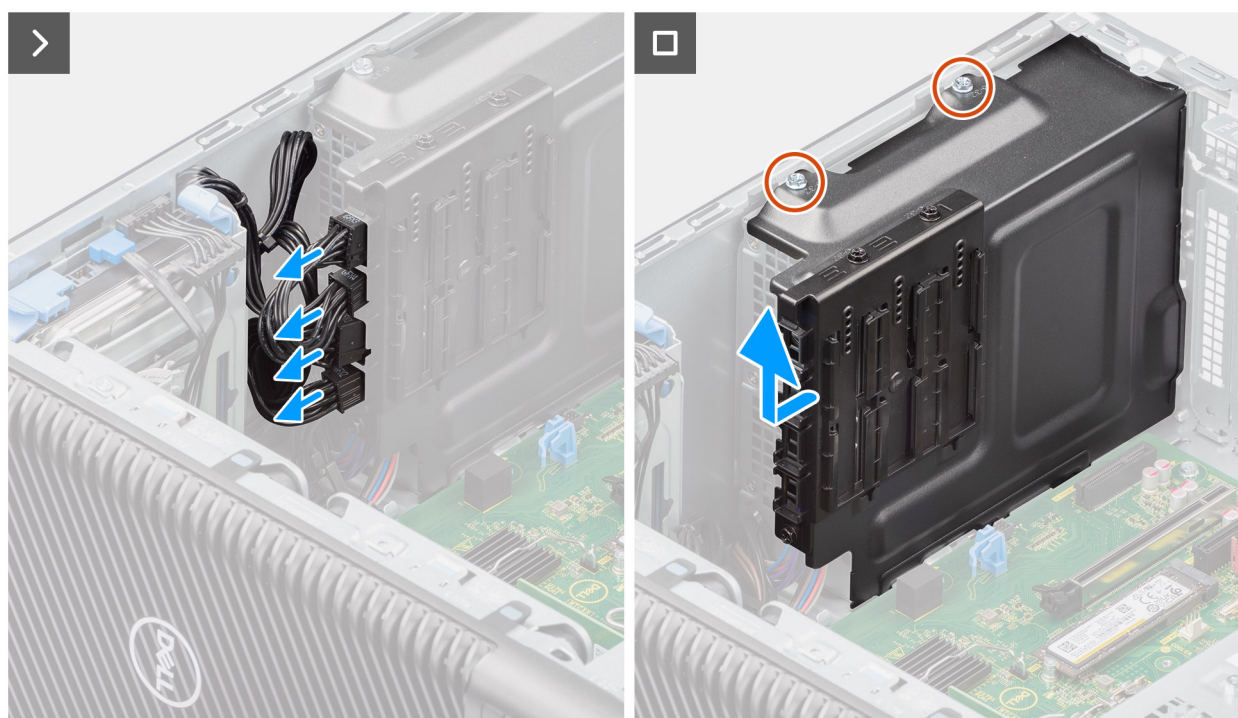
Figure 46. Retrait du capot du bloc d'alimentation
