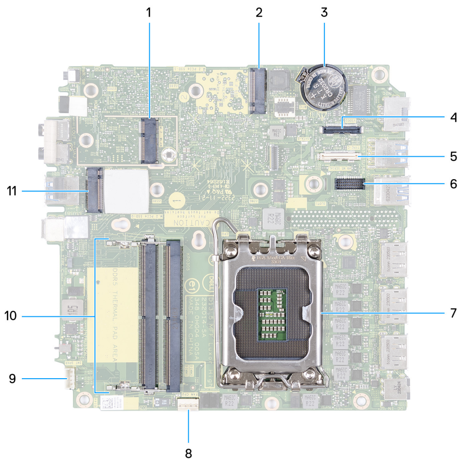
Figur 47. Kontakter på moderkortet
