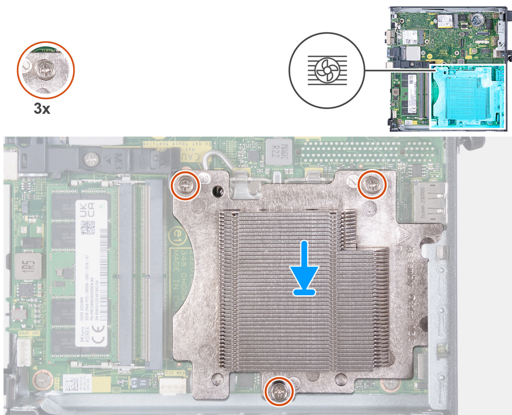
Figur 41. Installera kylflänsen
