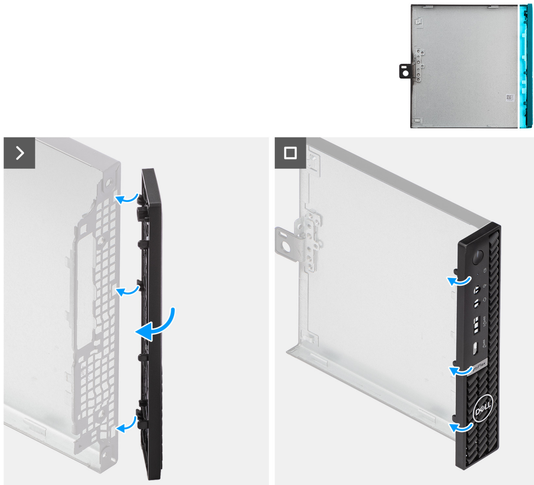
Figur 16. Installera frontramen
