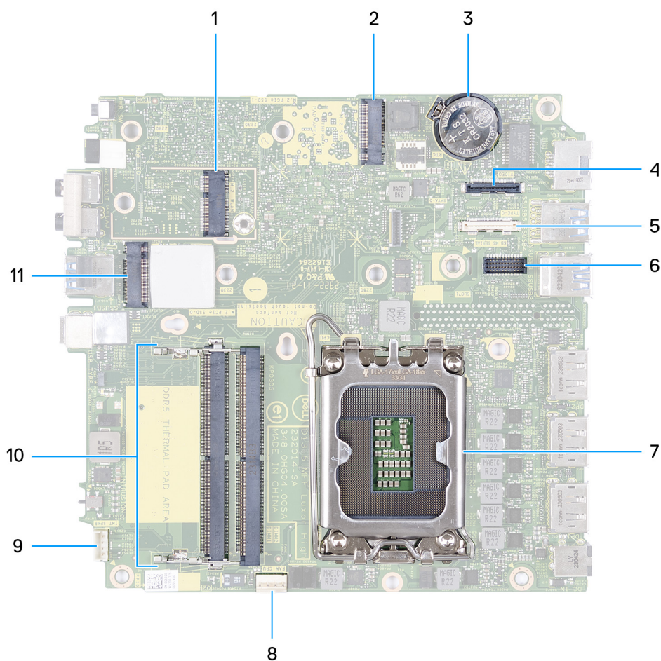
Figur 44. Kontakter på moderkortet
