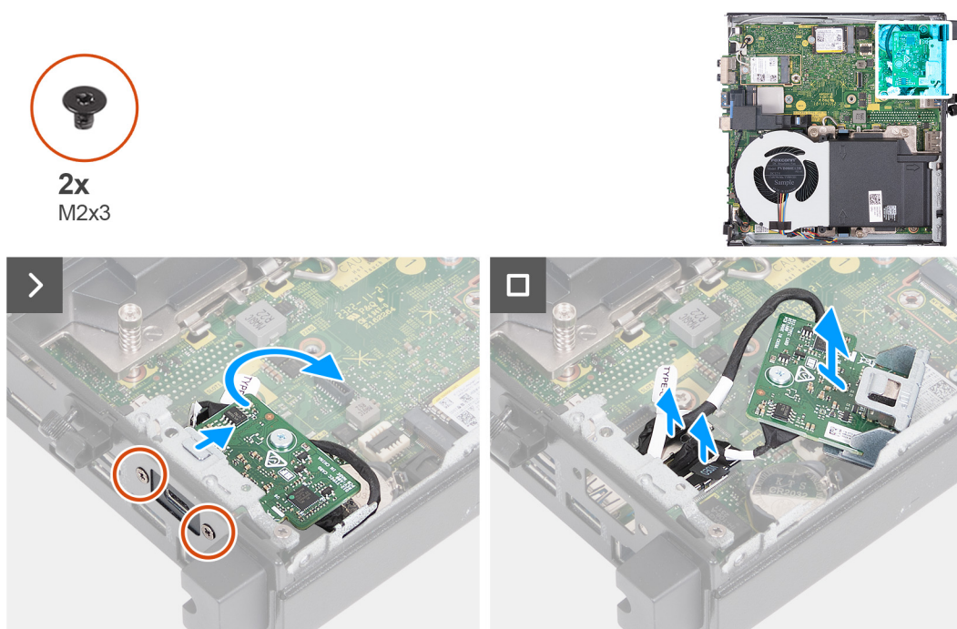
Figur 38. Ta bort Typ C-modulen (tillval)
