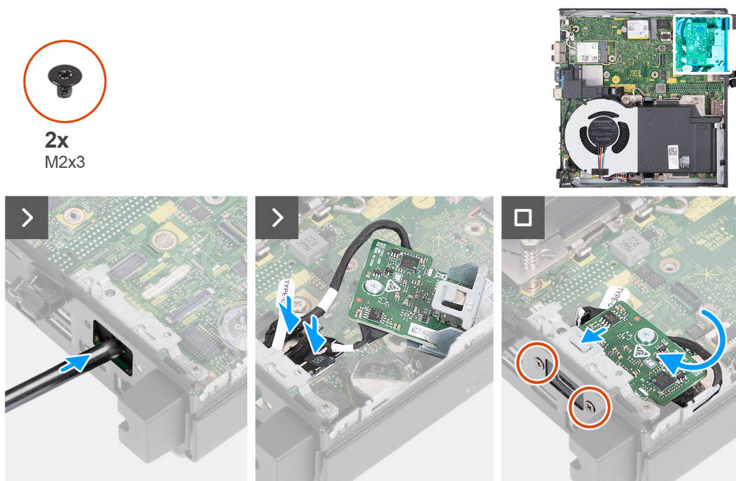
Figur 39. Installera Typ C-modulen (tillval)
