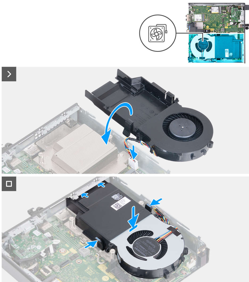
Figur 31. Installera fläkten
