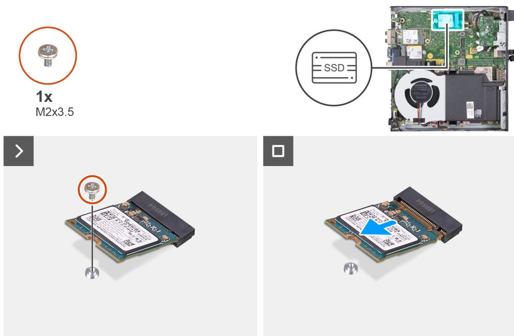
Figur 21. Ta bort M.2 2230 SSD-disk från kortplats 1
