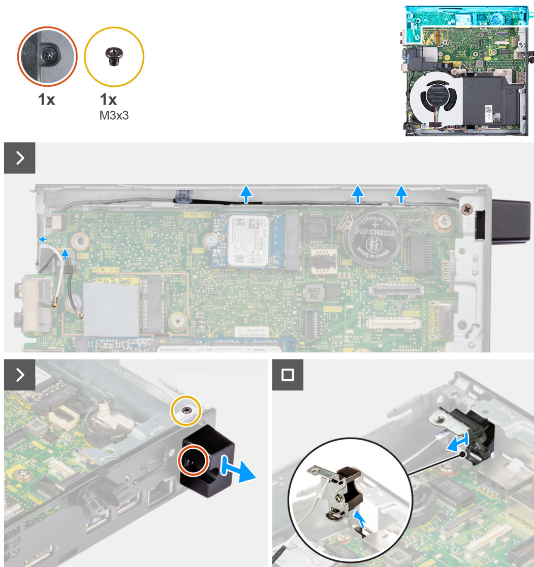
Figur 50. Ta bort antennenmodulen (vit kabel)
