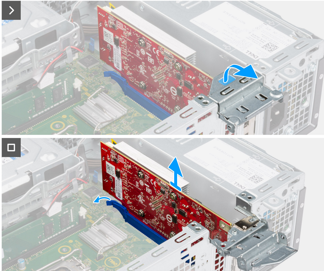
Figure 29. Retrait de la carte graphique
