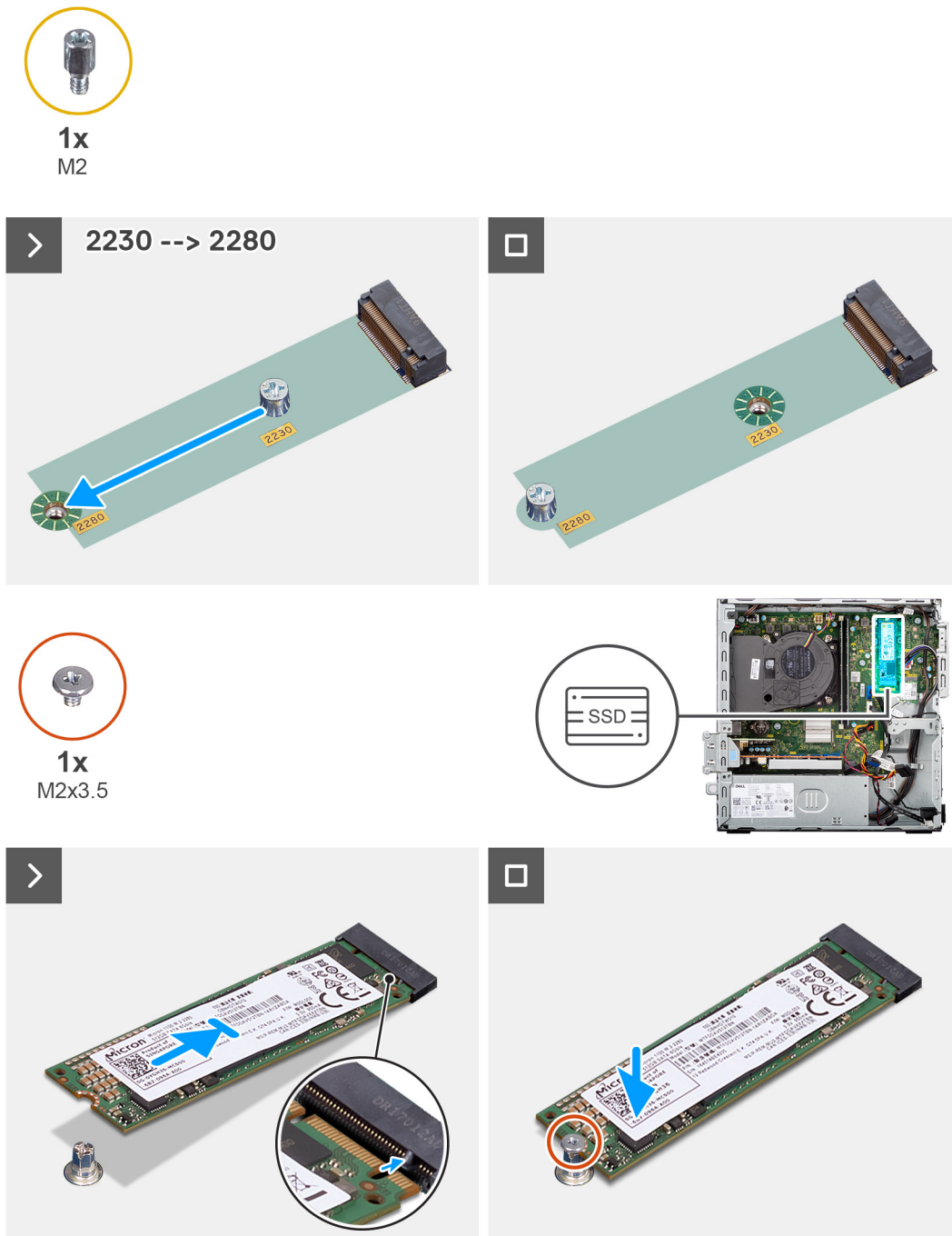
Figure 20. Installation du disque SSD M.2 2280
