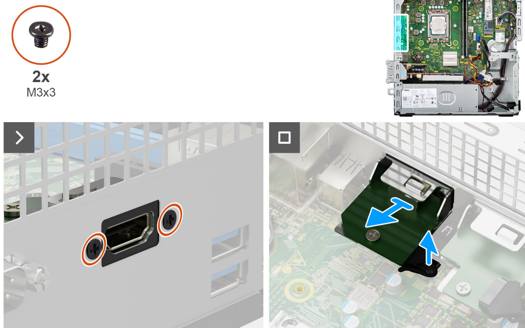
Figure 54. Retrait du module HDMI
