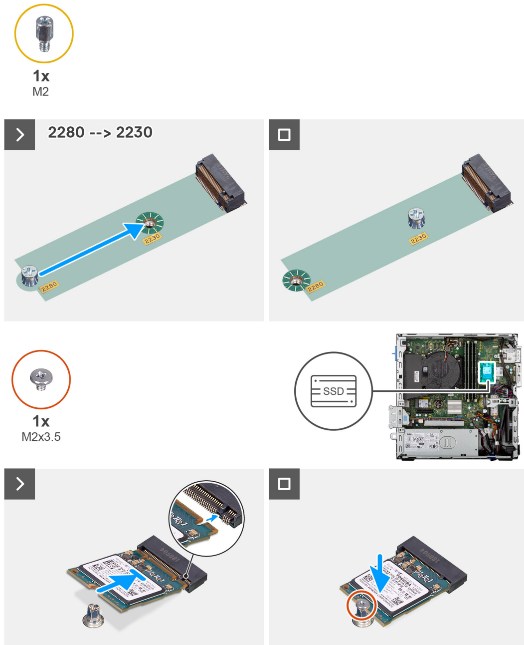
Figure 18. Installation des disques SSD M.2 2230
