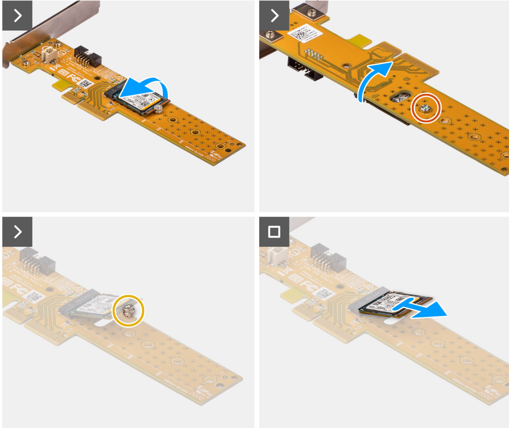
Figure 22. Retrait du disque SSD M.2 2230 de la carte Dell Ultra Speed Drive Gen 3
