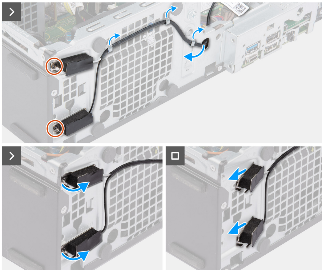
Figure 37. Retrait du module d'antenne interne
