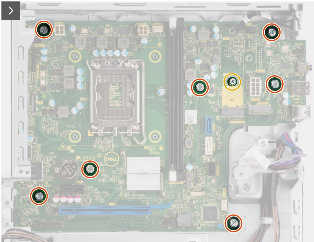
Figura 63. Installazione della scheda di sistema
