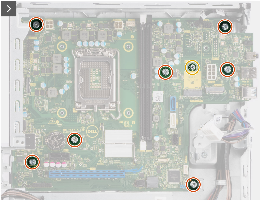
Figura 59. Rimozione della scheda di sistema
