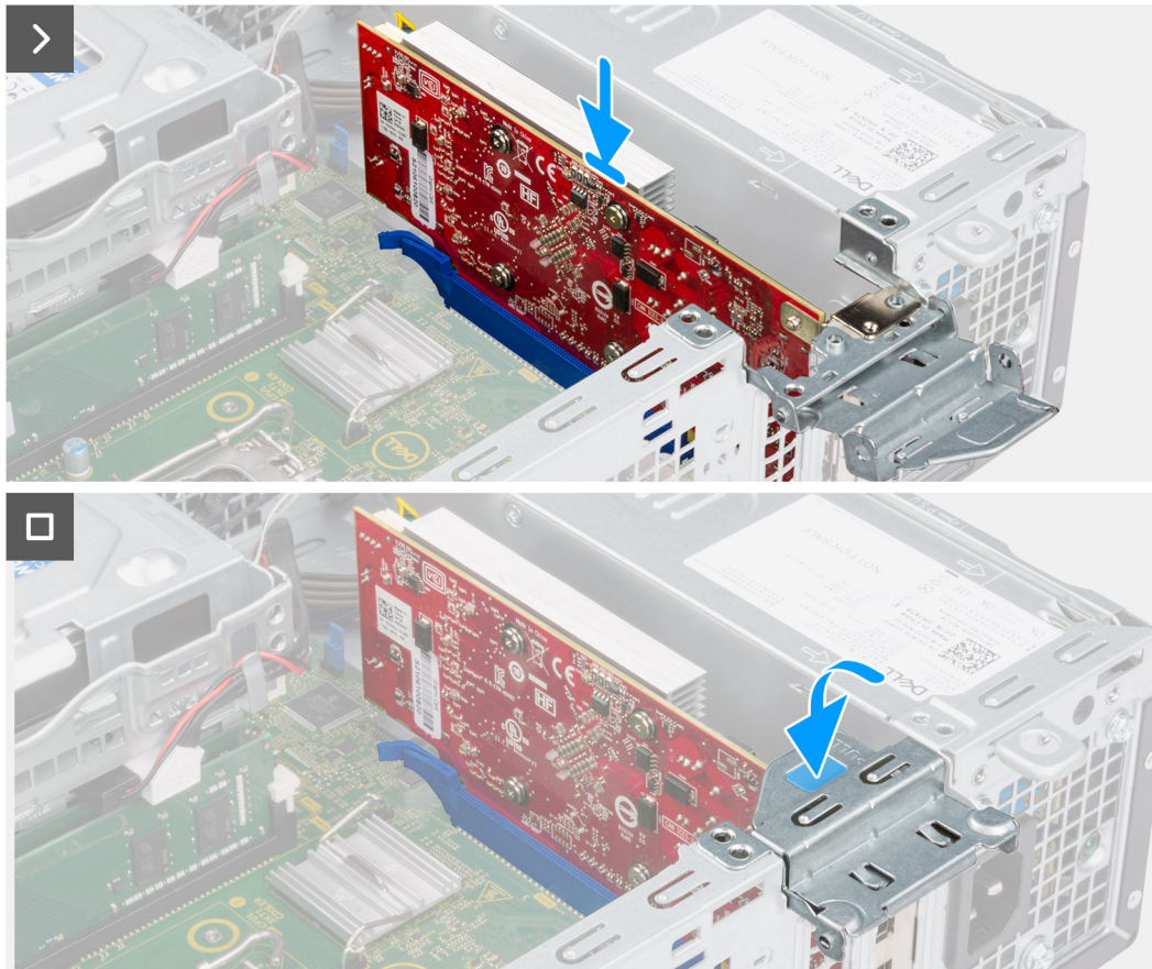
Figura 30. Installazione della scheda grafica
