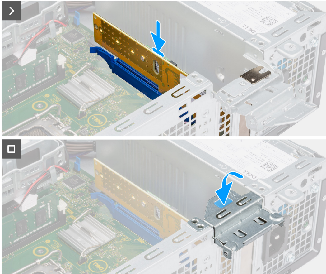
Figura 26. Installazione della scheda Dell Ultra Speed Drive Gen3
