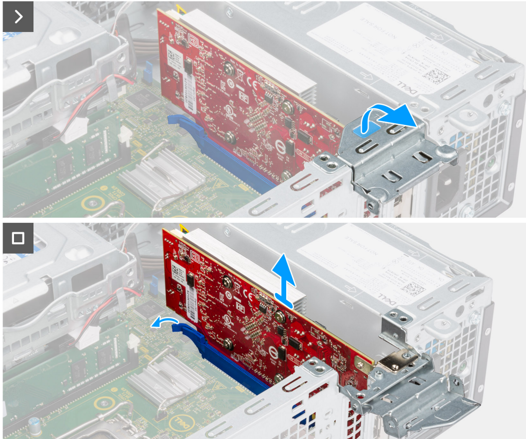
Figura 29. Rimozione della scheda grafica
