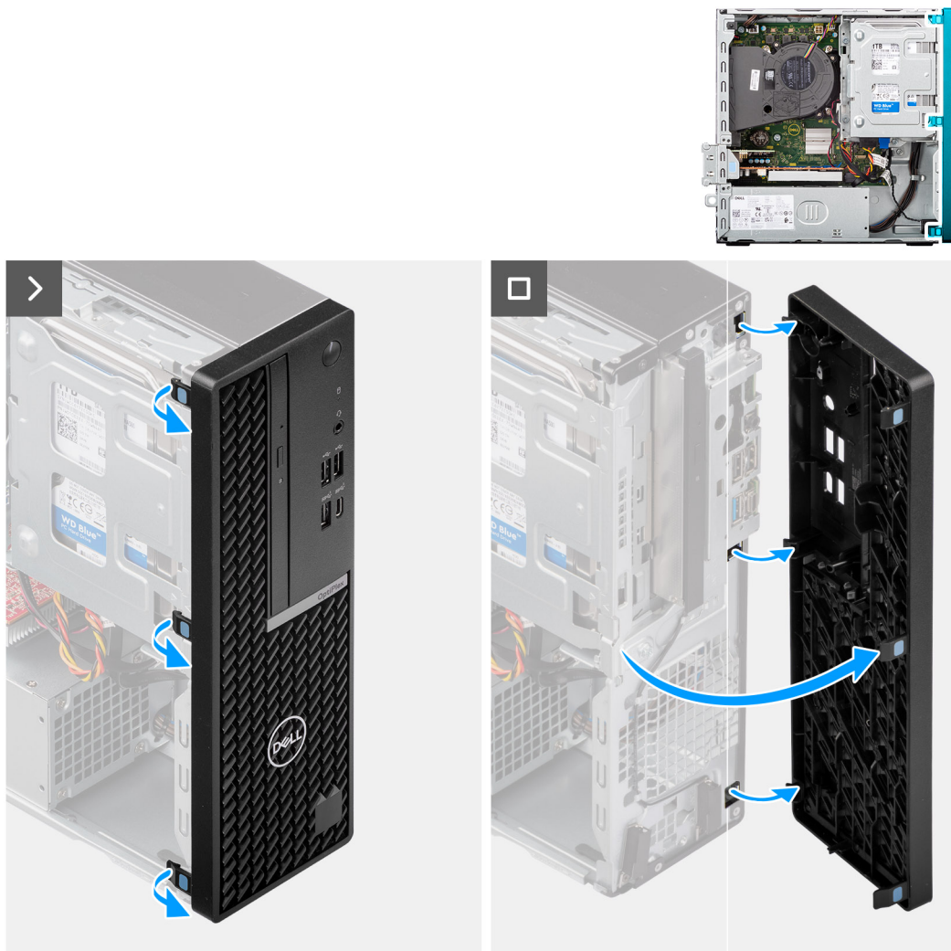
Figura 7. Rimozione del pannello anteriore
