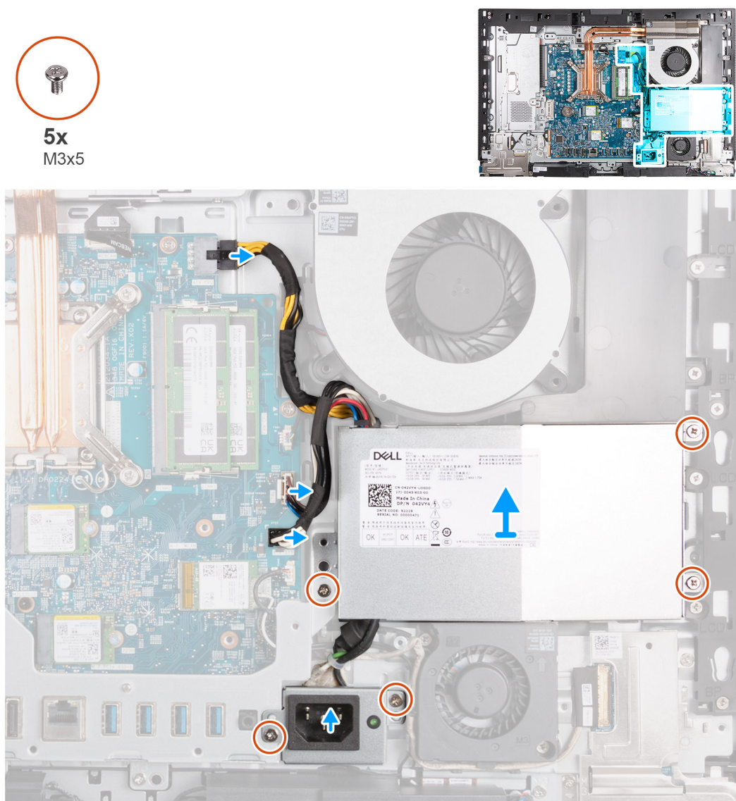
Figura 49. Rimozione dell'unità di alimentazione
