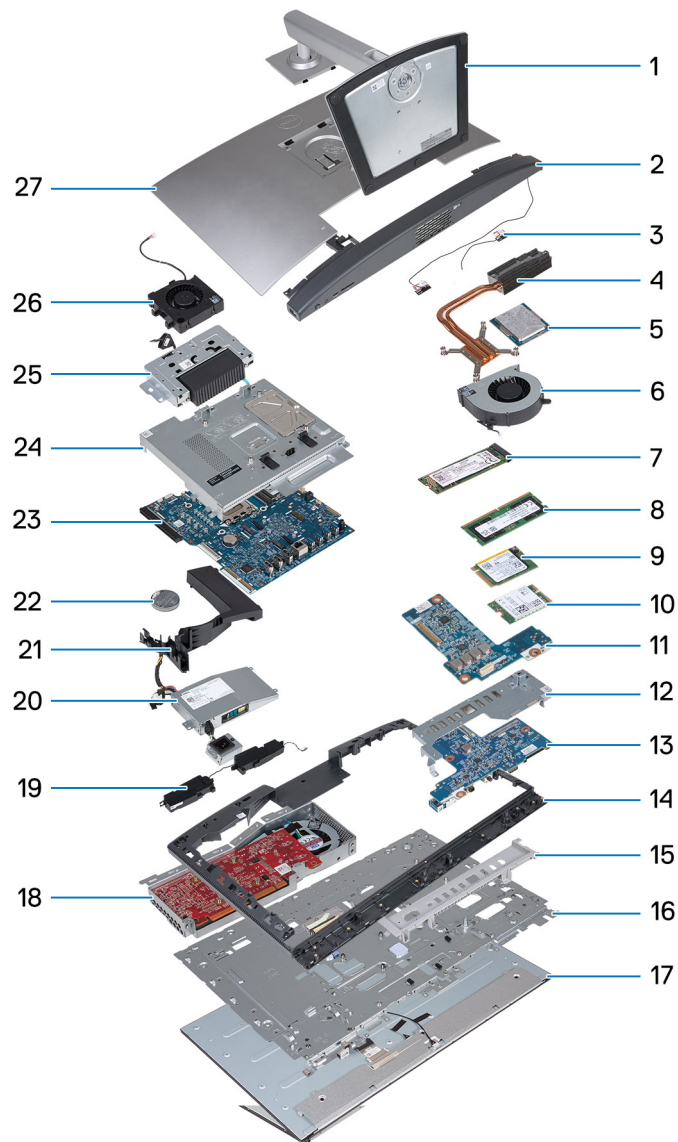
Figure 14. Principaux composants de votre ordinateur OptiPlex All-in-One Plus 7420
