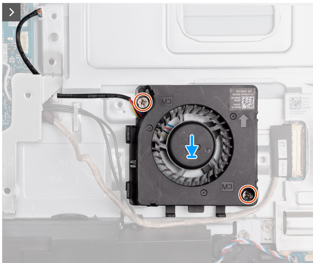
Figure 54. Installation du ventilateur du bloc d'alimentation
