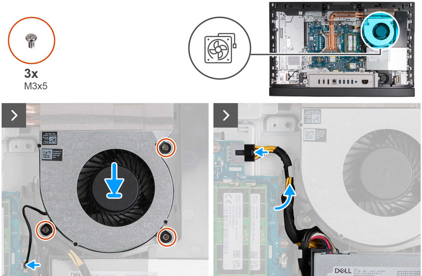
Figure 48. Installation du ventilateur
