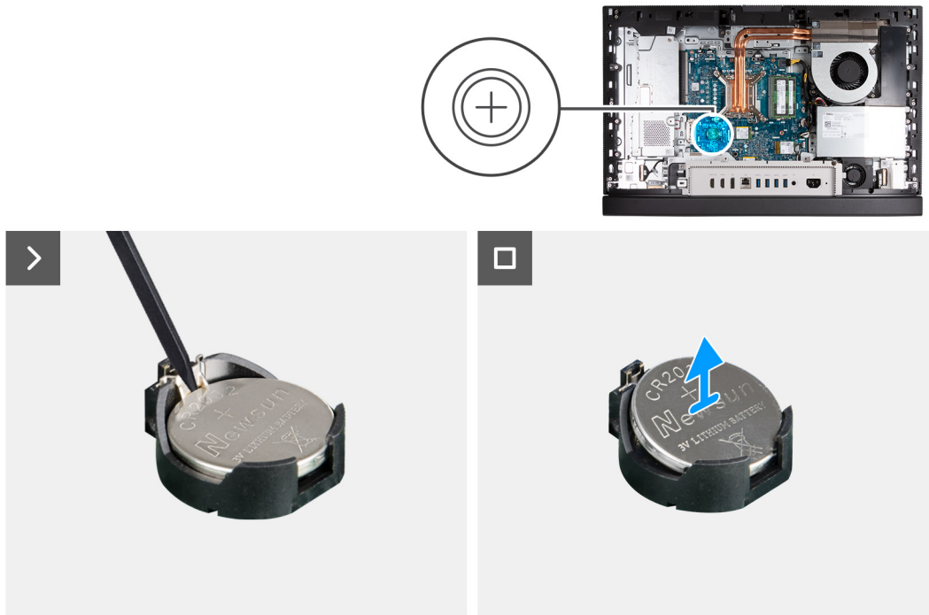
Figure 39. Retrait de la pile bouton
