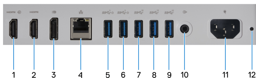
Figure 8. Vue du panneau arrière de l'ordinateur OptiPlex All-in-One Plus 7420
