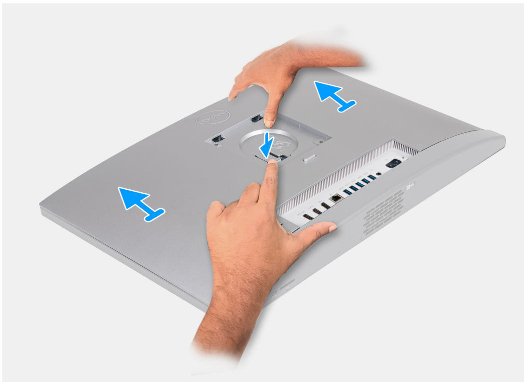
Figure 19. Retrait du capot arrière
