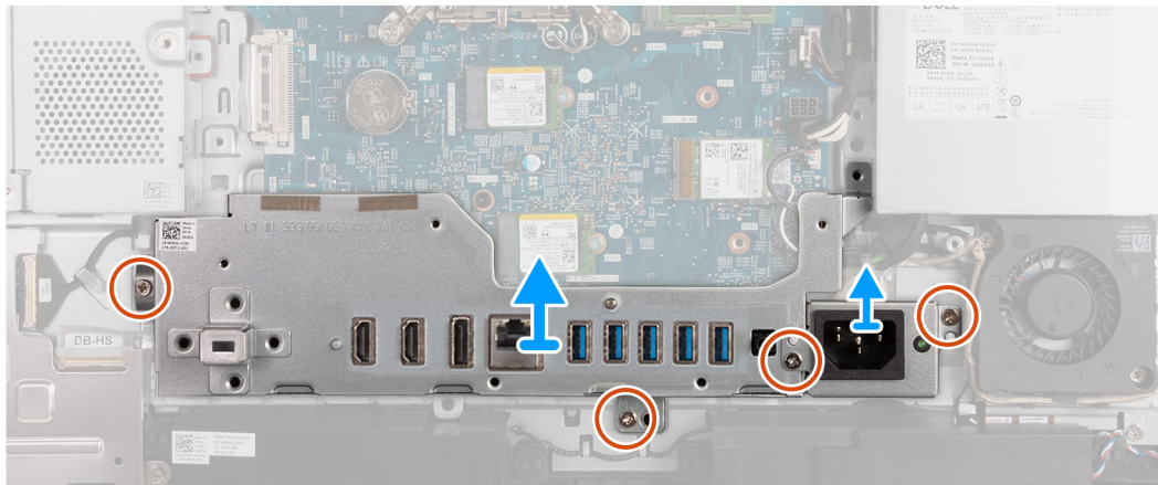
Figure 57. Retrait du support d'E/S
