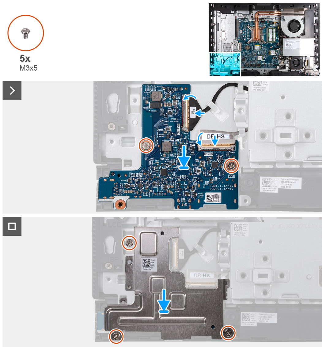
Figure 72. Installation du bouton d'alimentation et de la carte d'E/S
