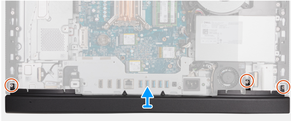
Figure 43. Retrait du cache inférieur
