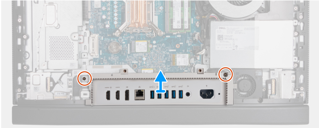
Figure 41. Retrait du cache d'E/S
