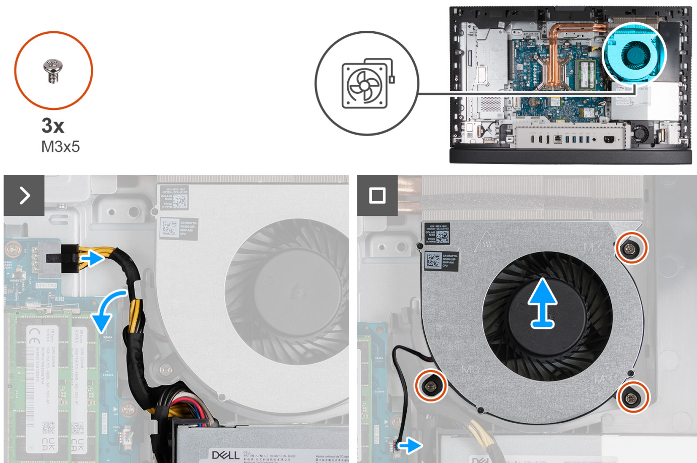
Figure 47. Retrait du ventilateur
