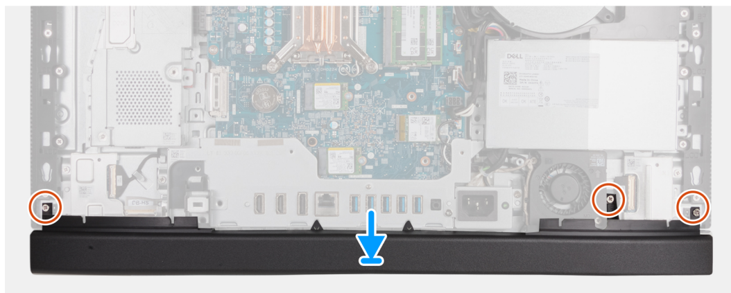
Figure 44. Installation du capot inférieur
