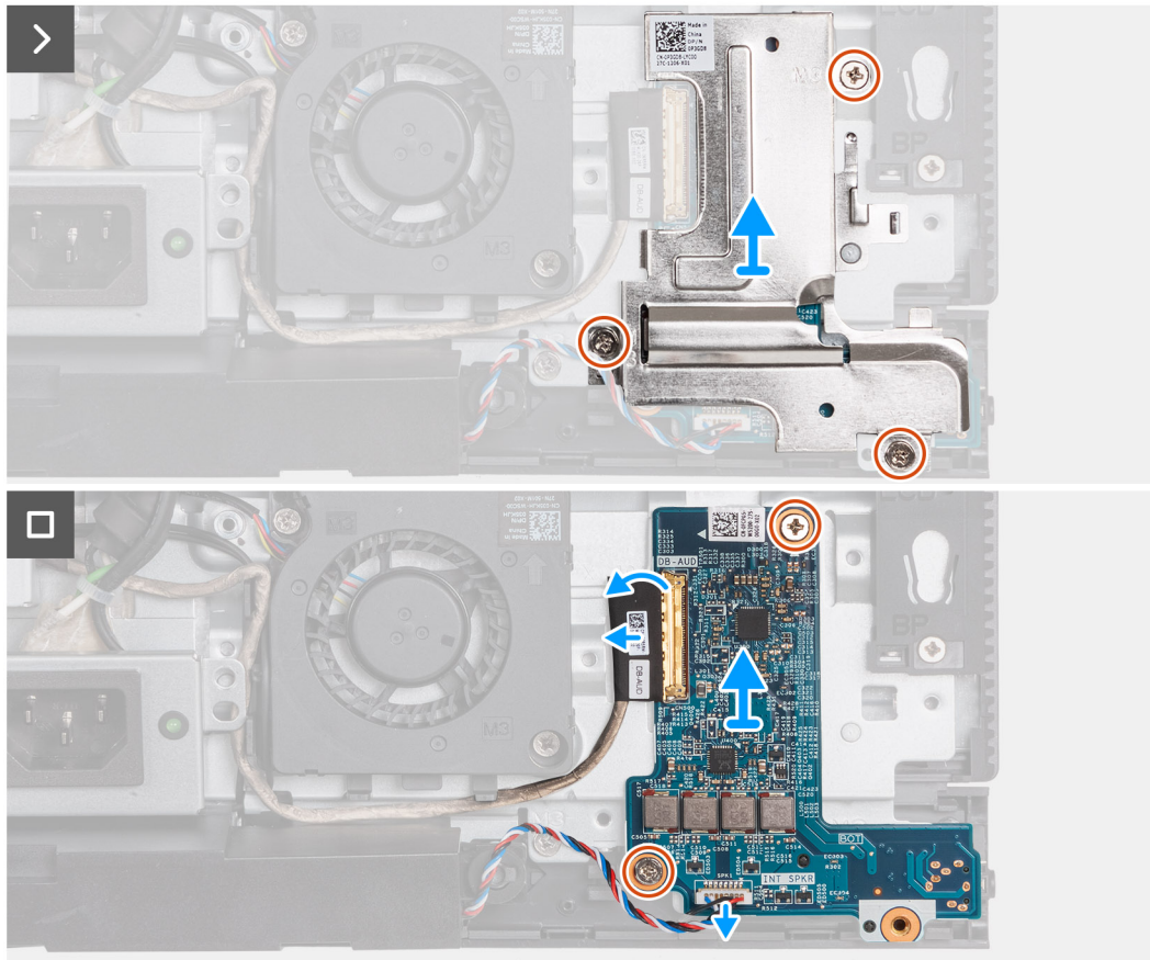
Figure 73. Retrait de la carte audio
