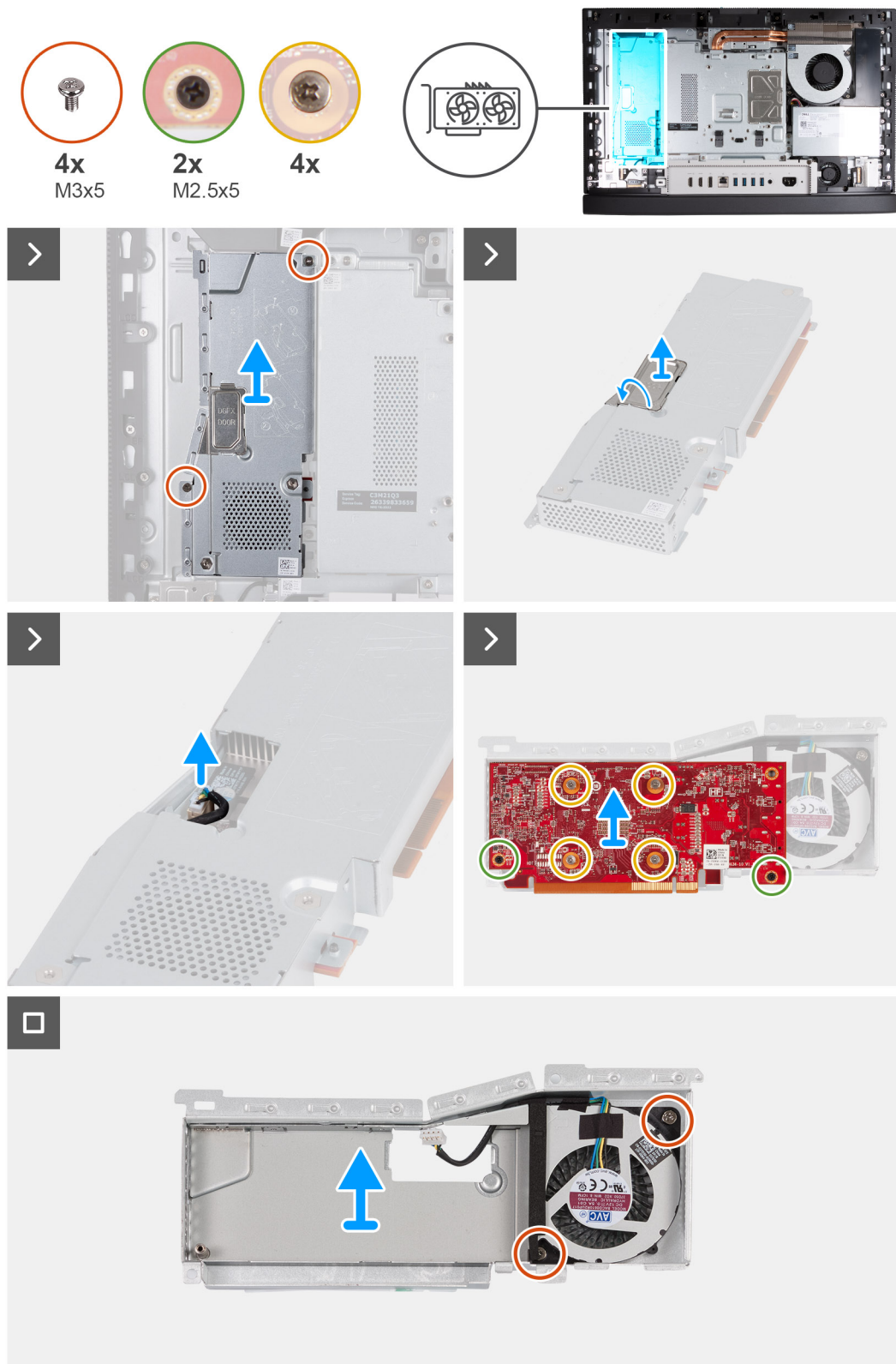
Figure 23. Retrait de la carte graphique
