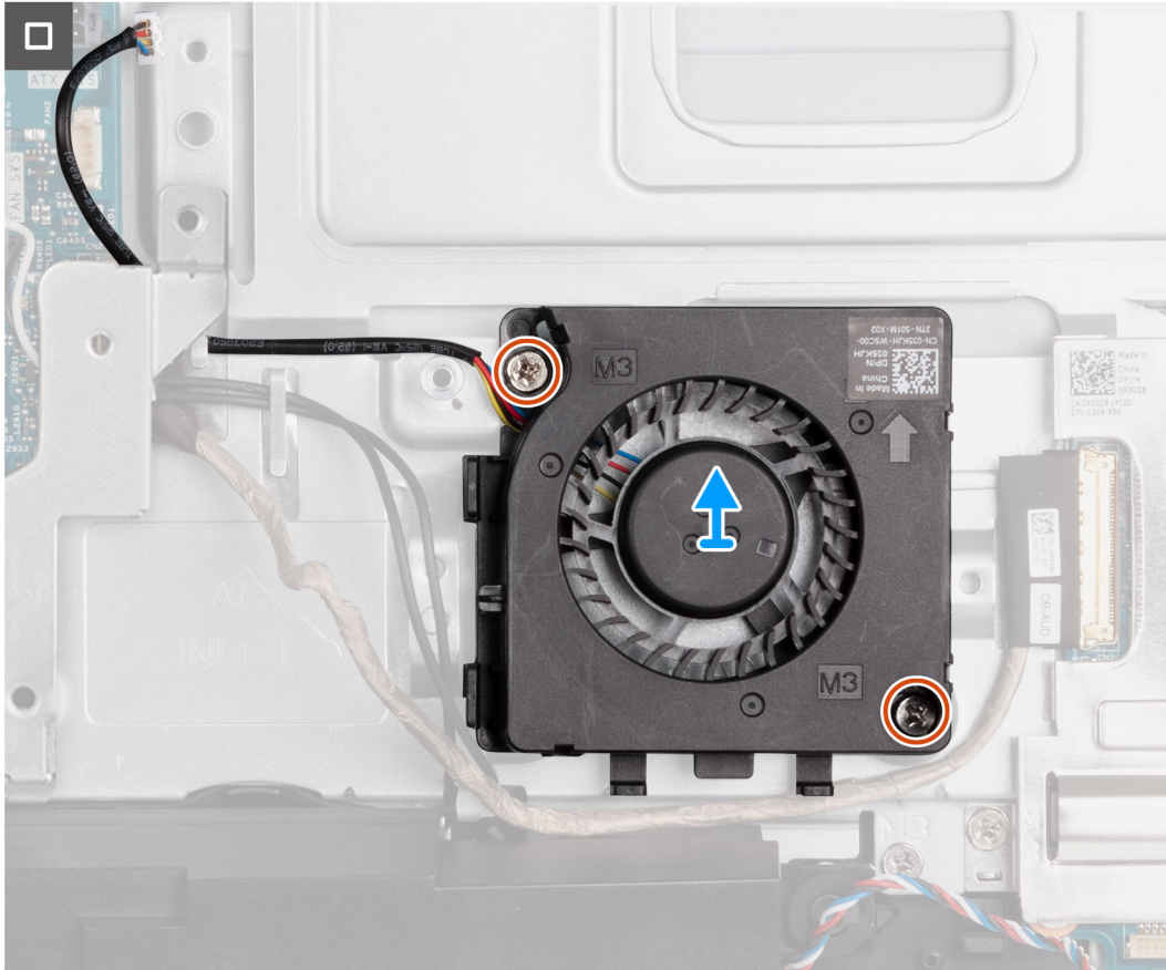
Figure 53. Retrait du ventilateur du bloc d'alimentation
