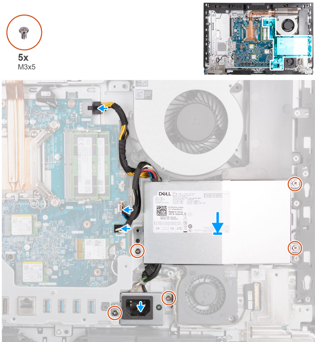
Figure 50. Installation du bloc d'alimentation
