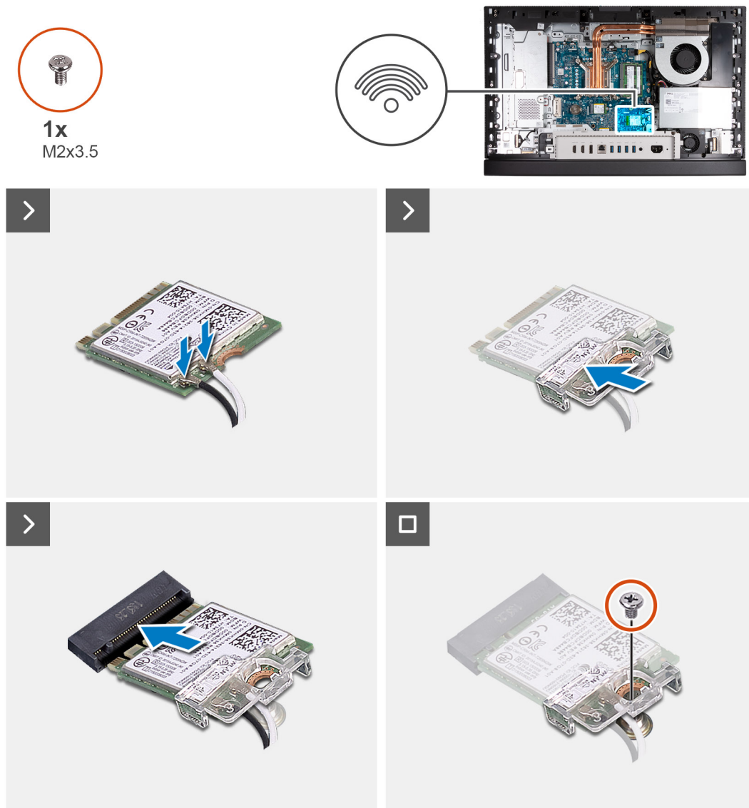
Figure 28. Installation de la carte sans fil
