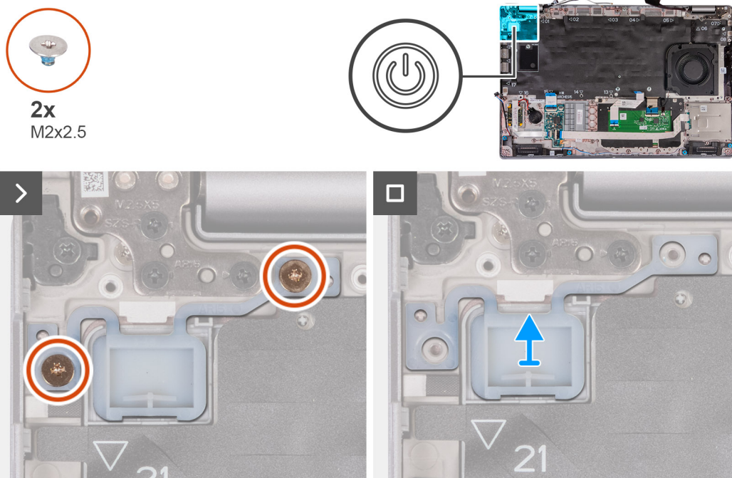
Figura61. Retirar o botão de alimentação
