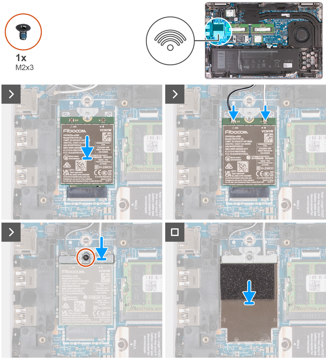
Figura22. Instalar a placa WWAN 4G
