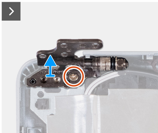
Figura86. Retirar as dobradiças do ecrã
