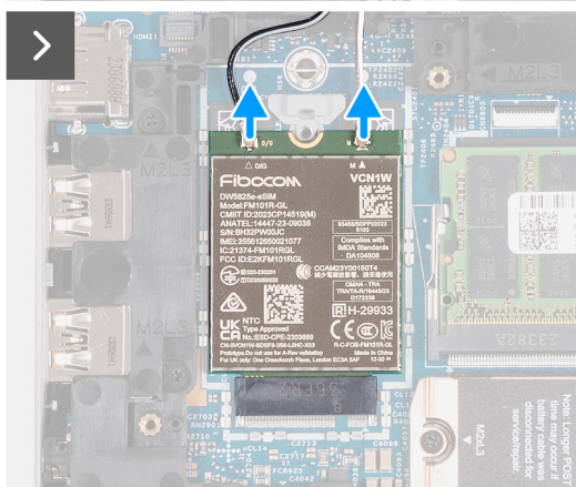
Figura21. Retirar a placa WWAN 4G
