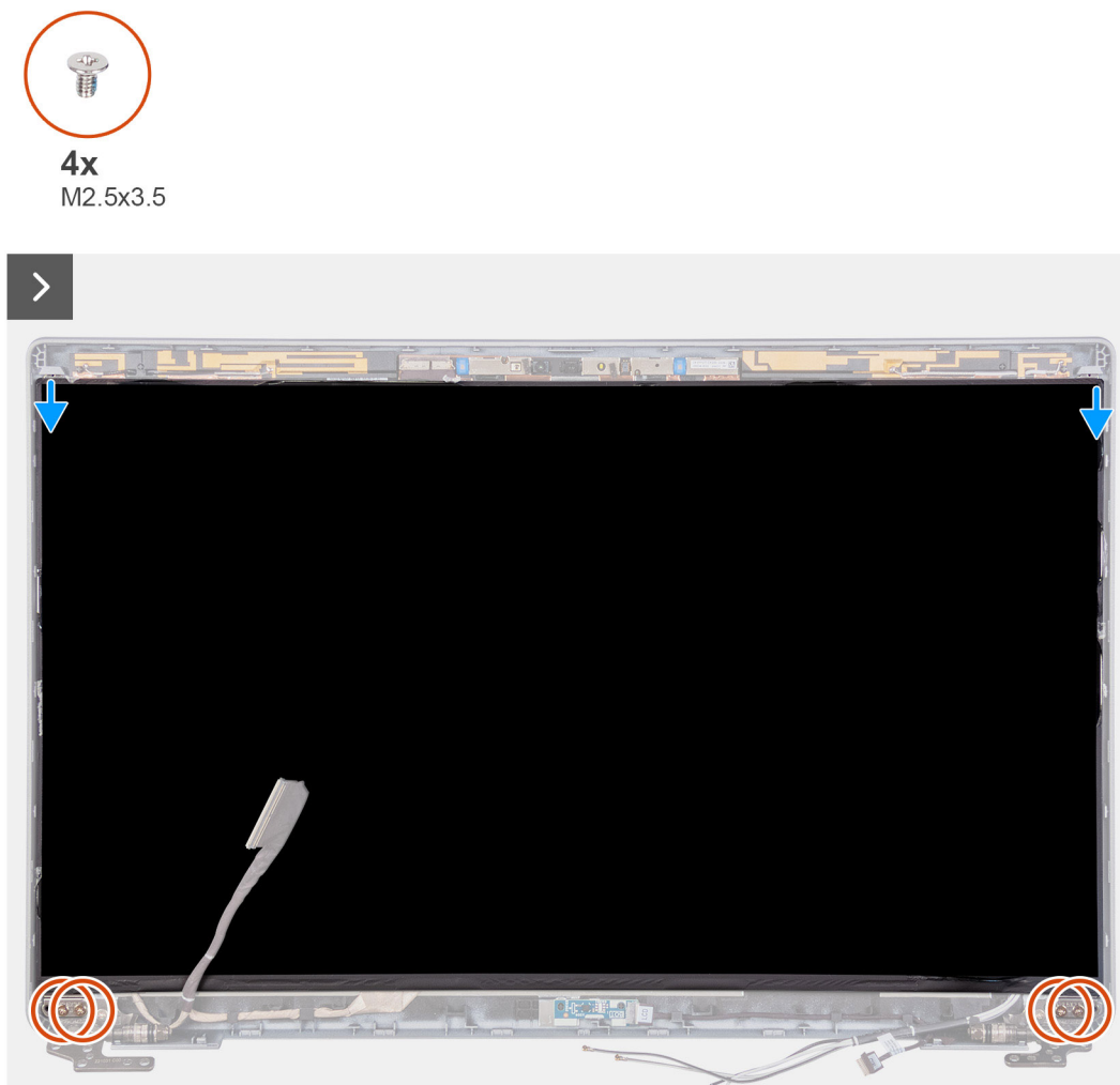
Figura76. Retirar o ecrã
