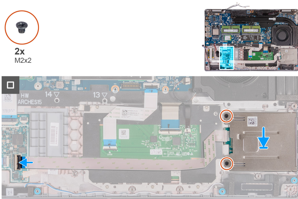
Figura97. Instalar o leitor de Smart Card
