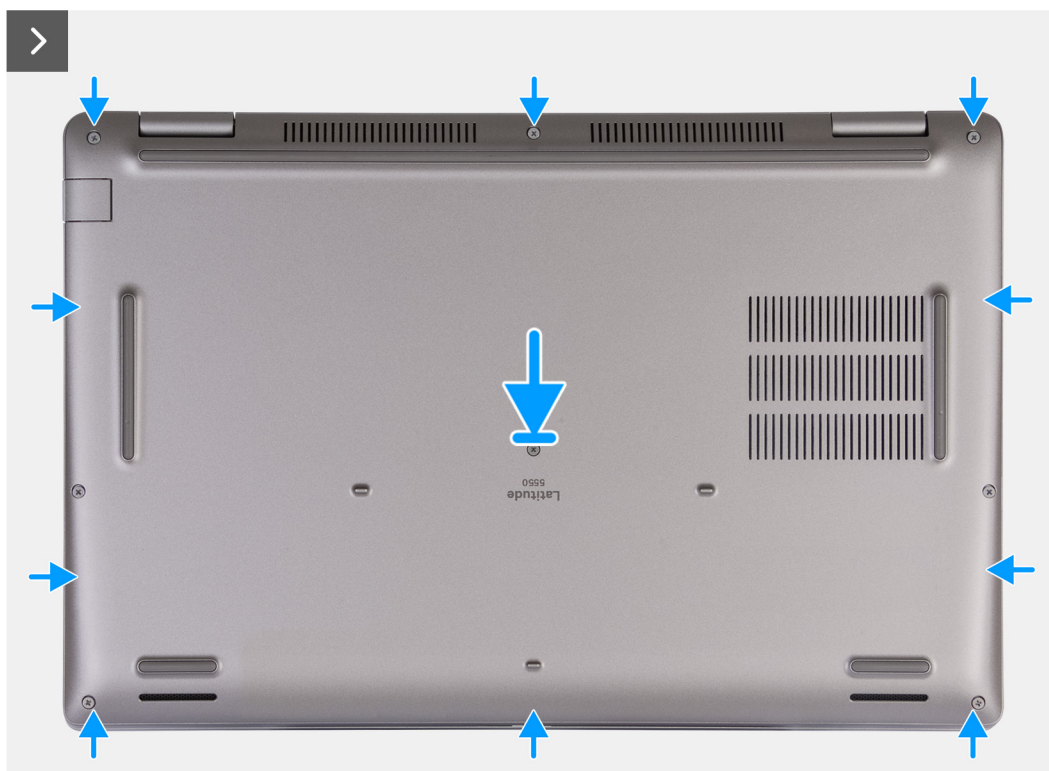
Figura17. Instalar a tampa da base
