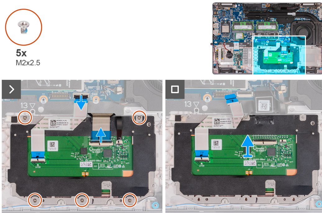
Figura41. Retirar o touchpad
