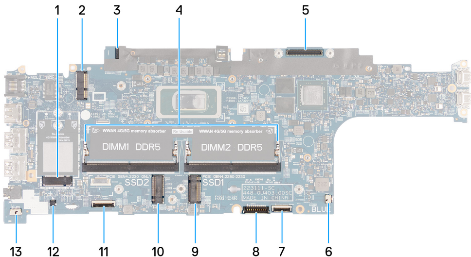
Figura57. Conectores da placa de sistema
