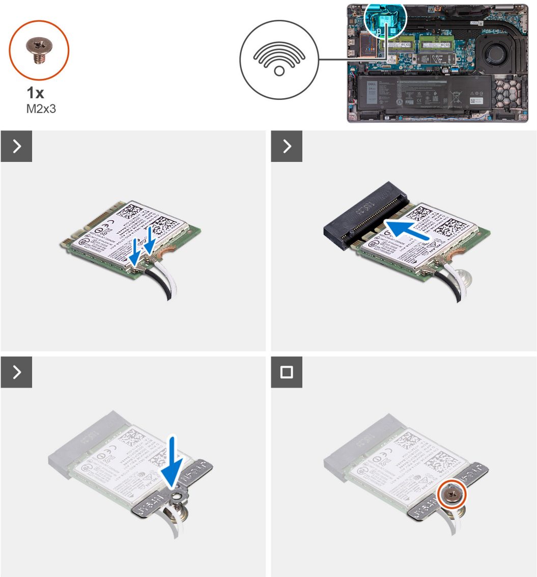
Figura20. Instalar a placa de comunicação sem fios
