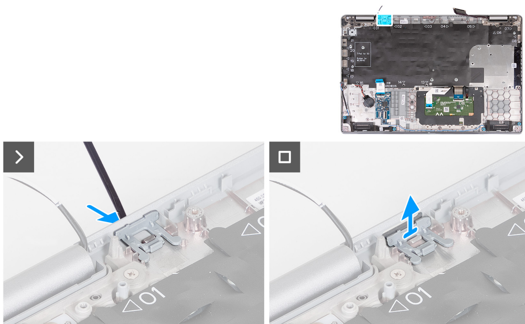
Figura98. Retirar o enchimento da ranhura do cartão SIM fictício
