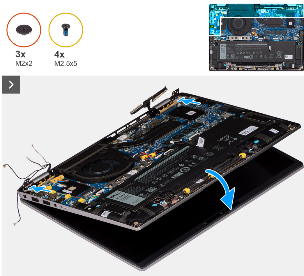
Figur 53. Installera bildskärmsenheten
