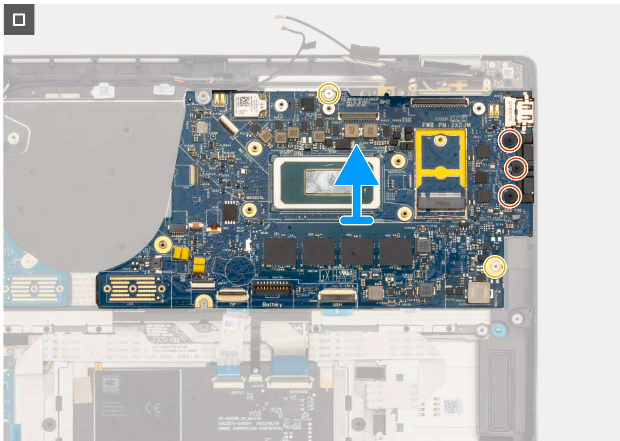
Figur 60. Ta bort moderkortet
