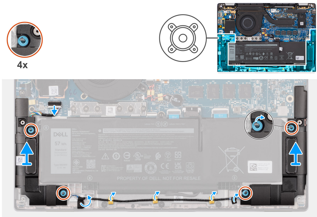
Figur 33. Ta bort högtalarna för vanliga enheter
