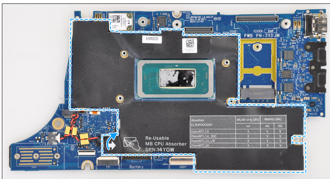
Figur 61. CPU-absorberare
