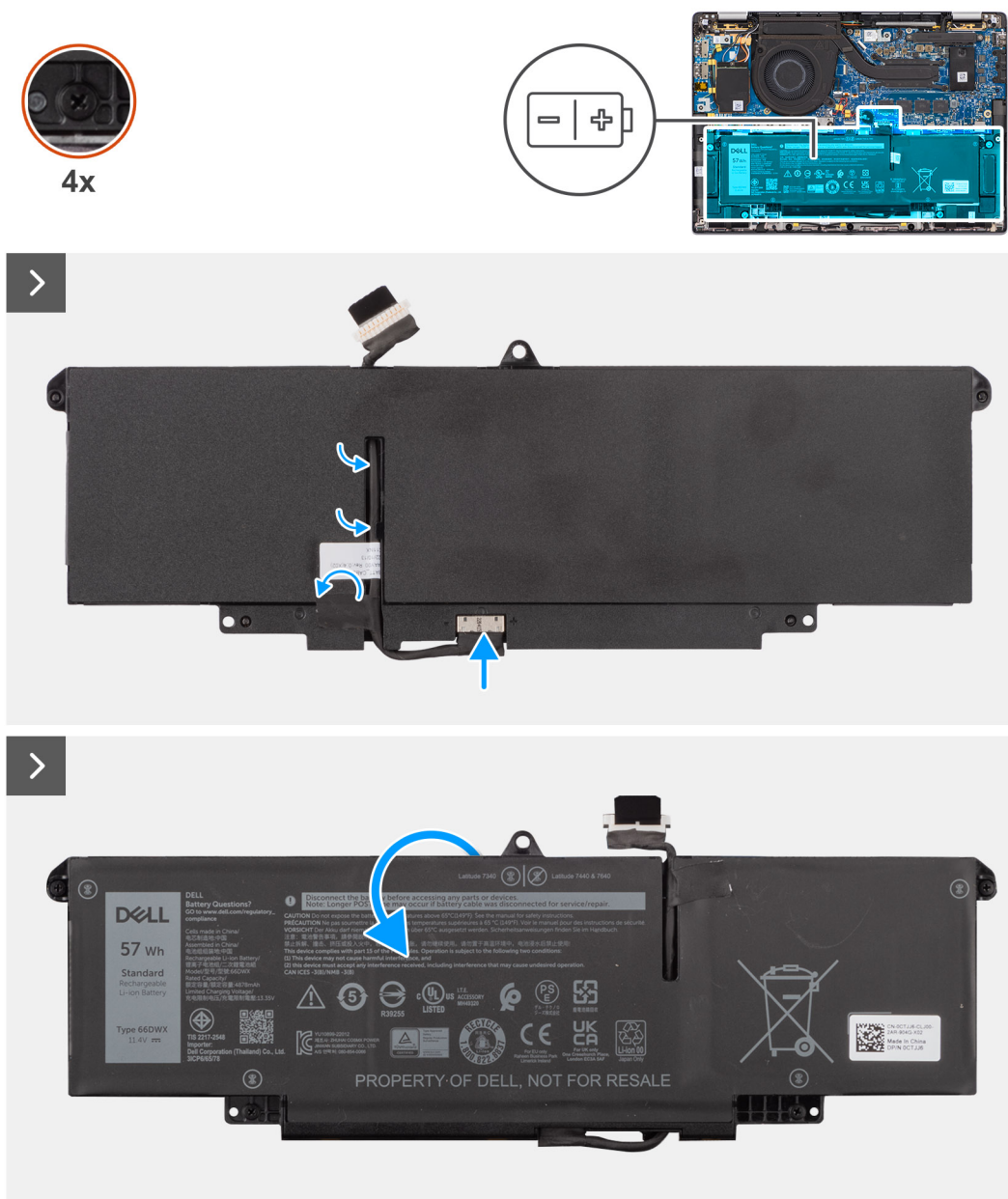
Figur 45. Installera batterikabeln
