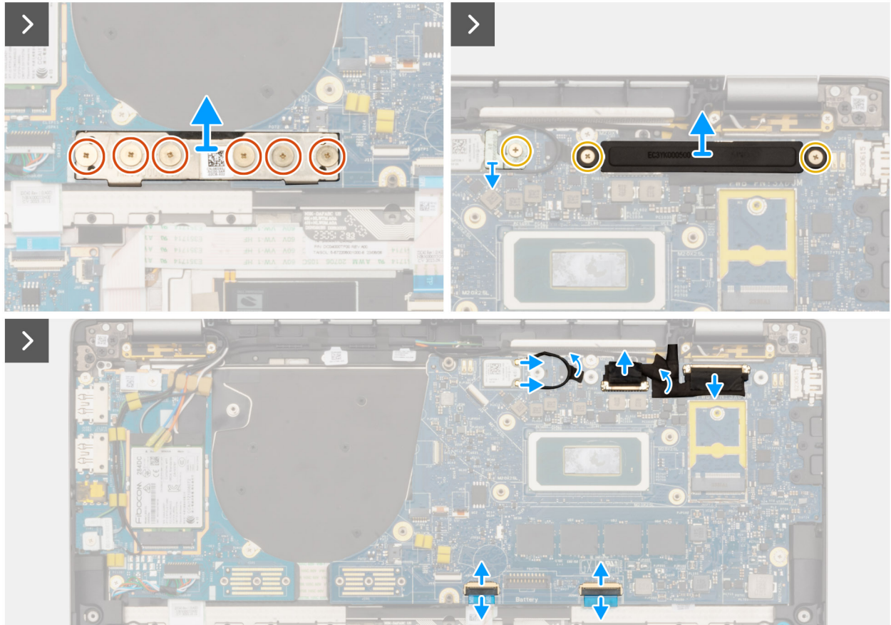
Figur 59. Ta bort moderkortet
