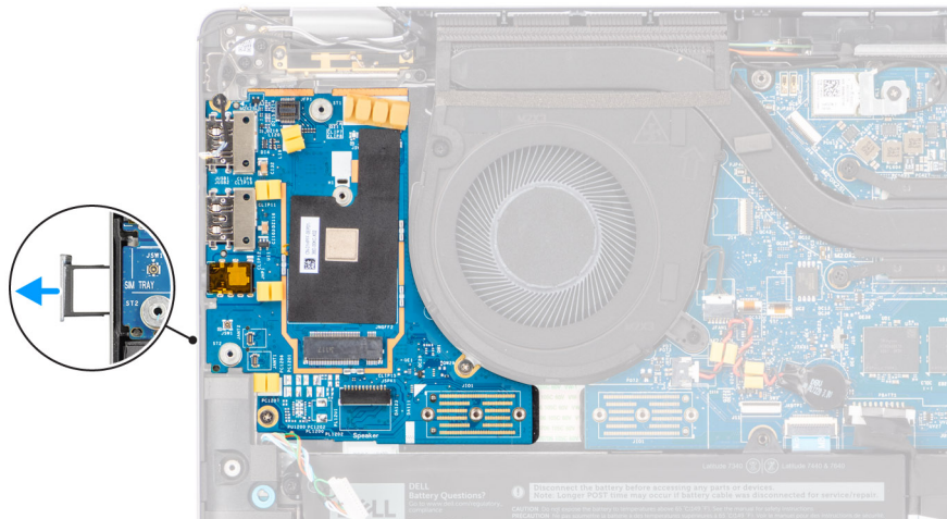
Figur 14. Borttagning av I/O-dotterkort
