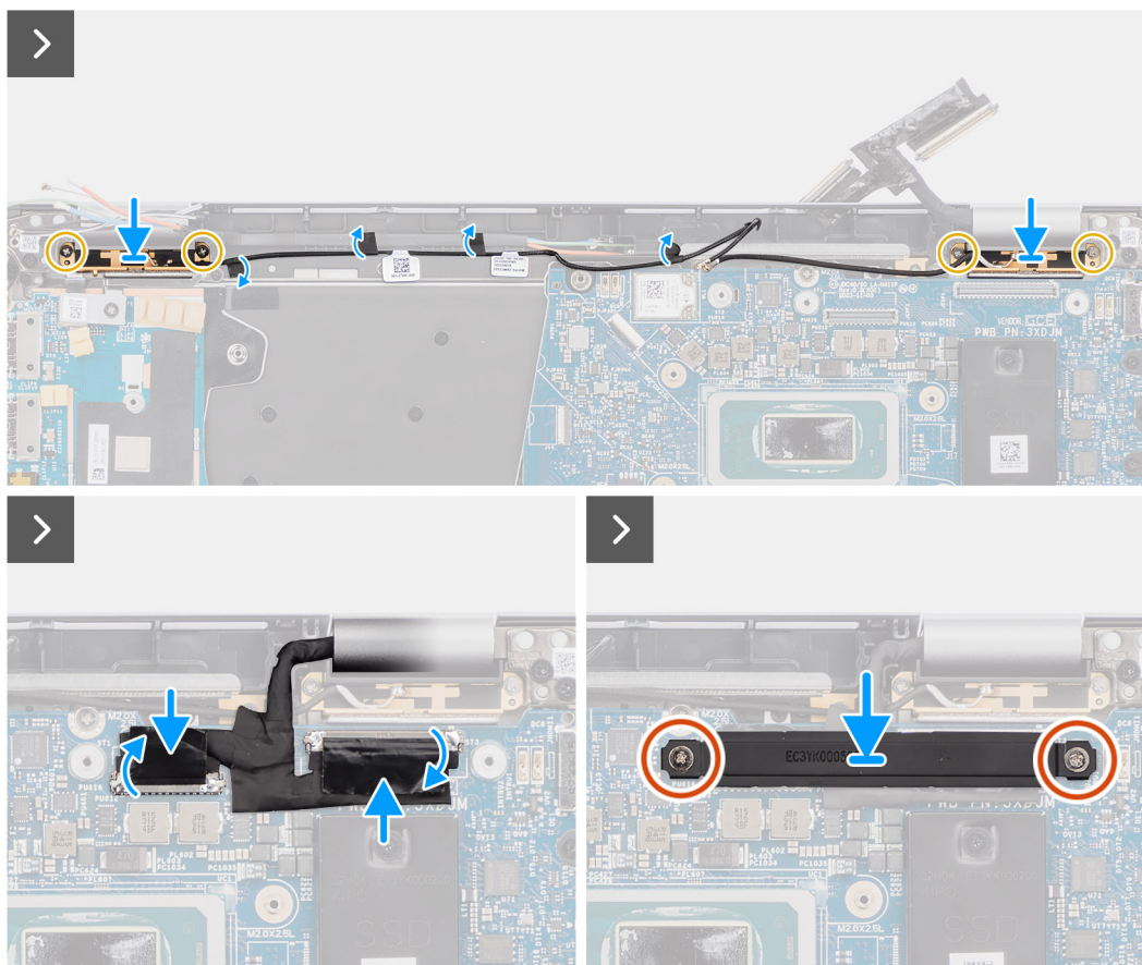
Figur 68. Installera WLAN-antenmodulen
