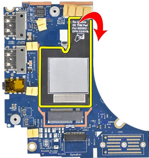
Figur 74. Latitude 7450 5G WWAN-konfiguration (klistermärke för värmeplatta)
