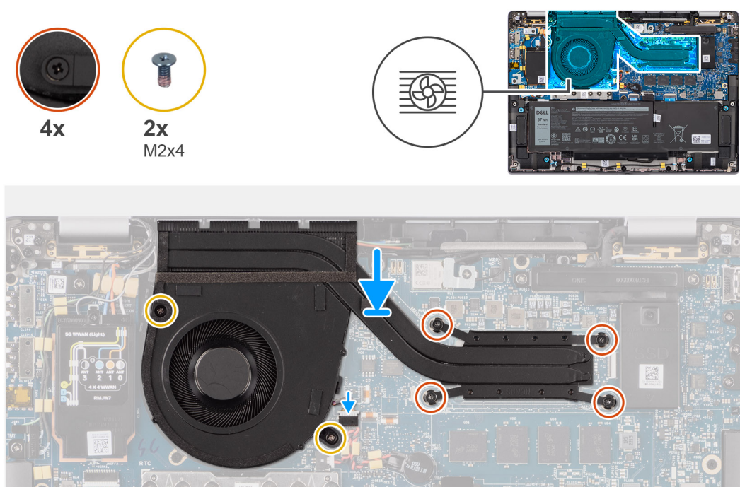
Figur 47. Installera fläkt- och kylflänsmonteringen
