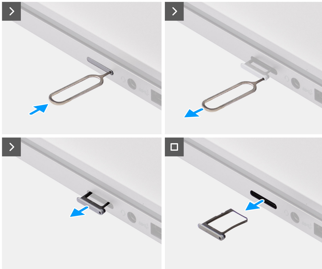
Figur 13. Ta bort SIM-kortsfacket
