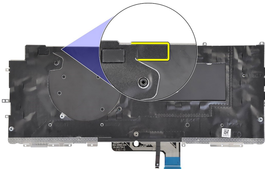
Figur 83. Installera tangentbordets mylartejp
