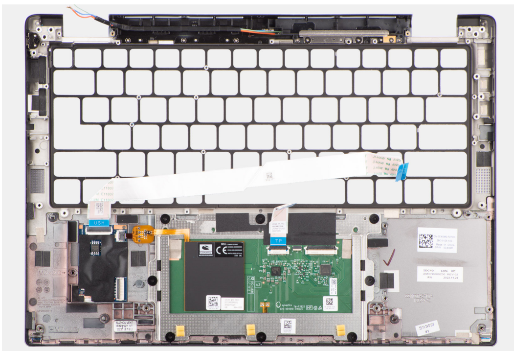
Figur 85. Installera handledsstödet
