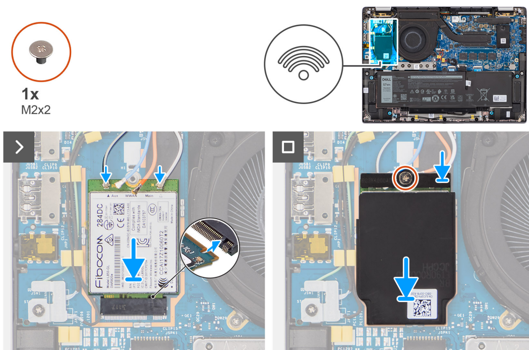
Figur 25. Installera 4G WWAN-kortet
