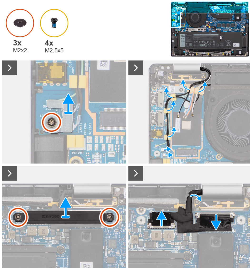
Figur 48. Ta bort bildskärmsenheten
