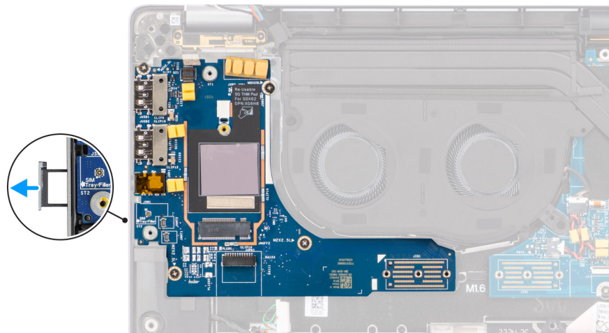
Figur 70. Ta bort I/O-dotterkortet
