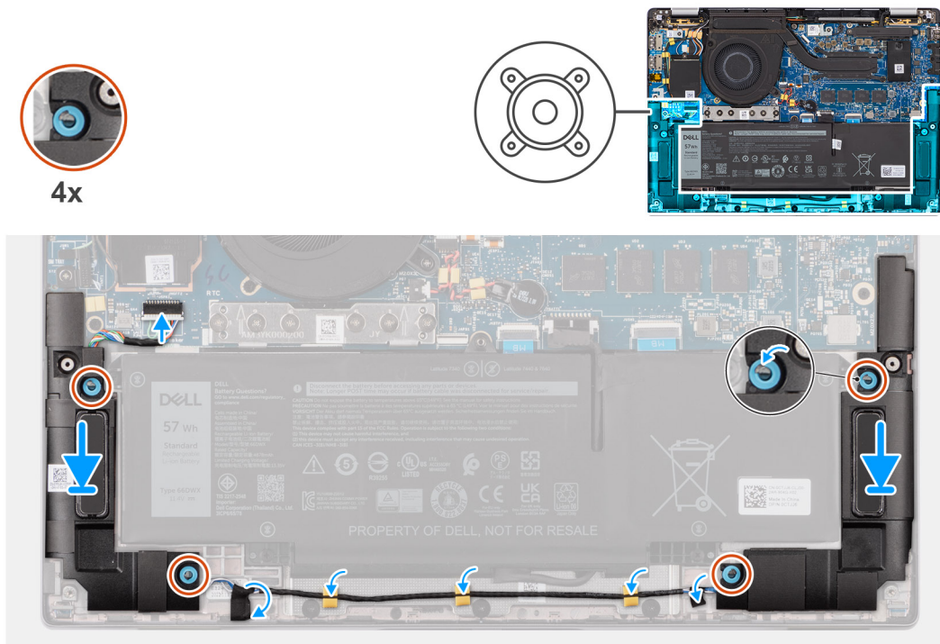
Figur 34. Installera högtalarna för mainstream
