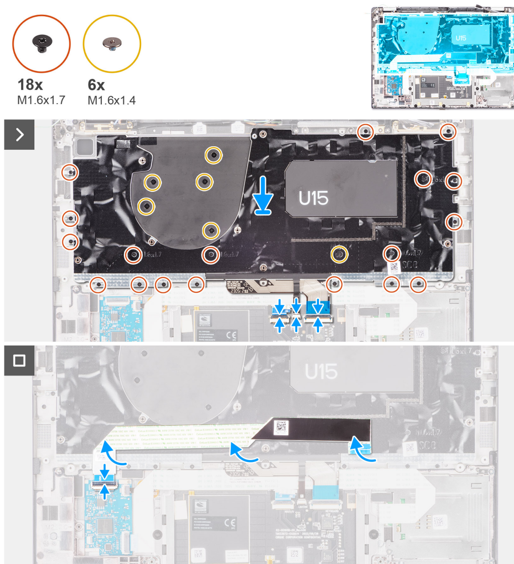
Figur 81. Installera tangentbordet
