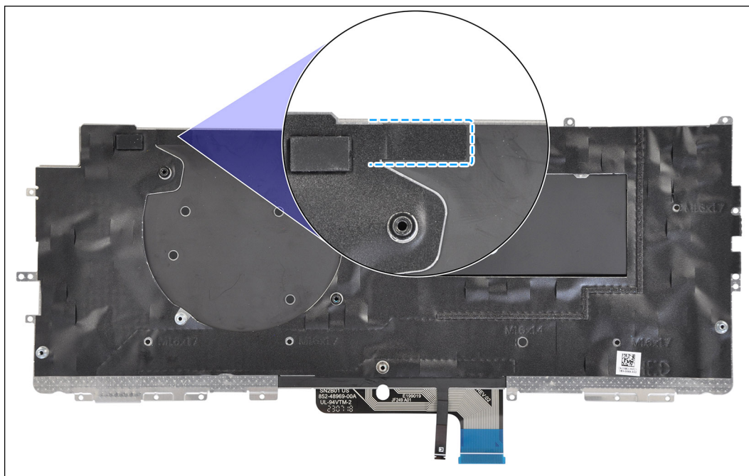
Figur 80. Ta bort tangentbordets mylartejp
