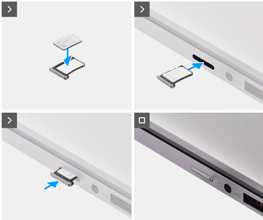
Figur 15. Installera SIM-kortsfacket
