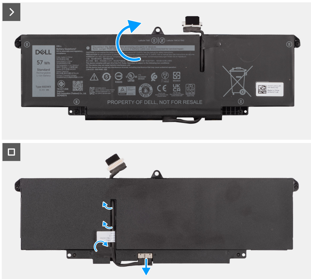
Figur 44. Ta bort batterikabeln
