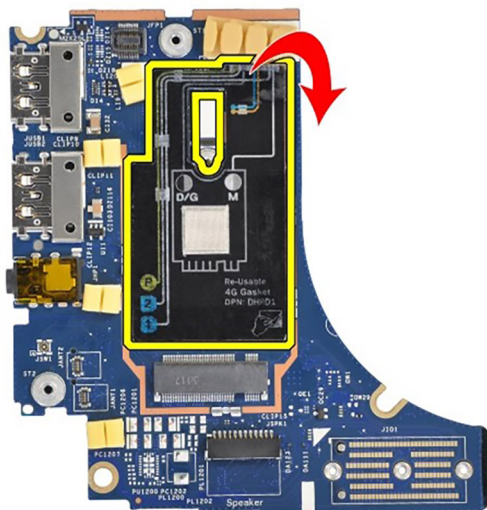
Figur 72. Latitude 7450 hopvikbar 4G WWAN-konfiguration (packningsklistermärke)
