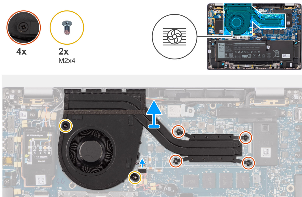
Figur 46. Ta bort kylfläns- och fläktmonteringen
