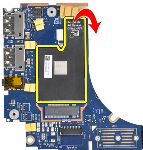
Figur 73. Latitude 7450 2-i-1 4G WWAN-konfiguration (packningsklistermärke)
