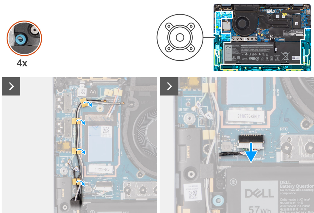
Figur 29. Ta bort högtalarna för ultralight
