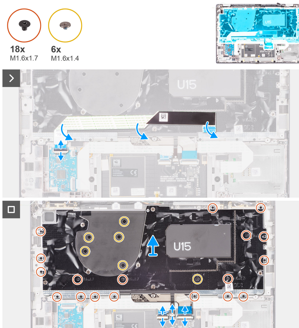
Figur 78. Ta bort tangentbordet
