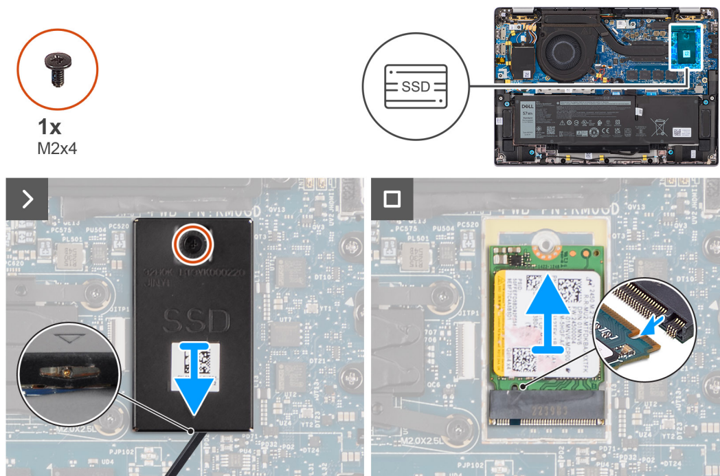
Figur 22. Ta bort M.2 2230 SSD-disken
