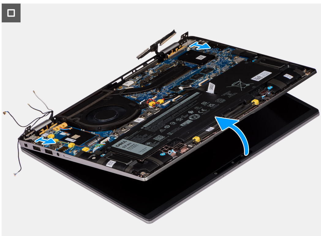
Figur 50. Ta bort bildskärmsenheten
