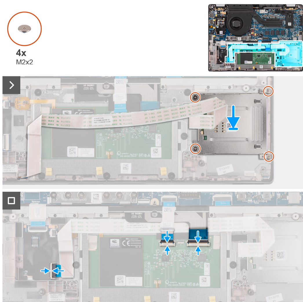
Figur 57. Installera smartkortläsaren
