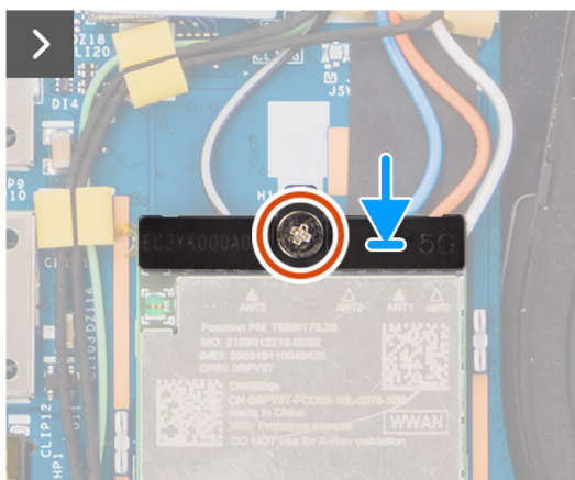
Figur 27. Installera 5G WWAN-kortet
