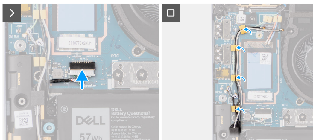
Figur 32. Installera högtalarna för ultralight
