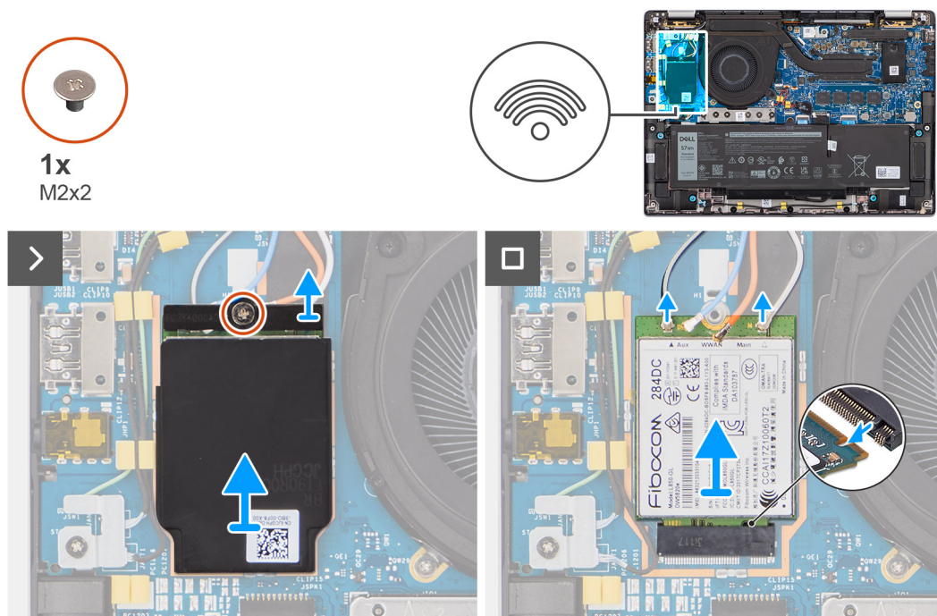
Figur 24. Ta bort 4G WWAN-kortet
