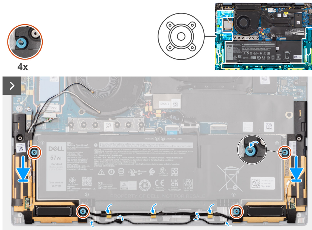
Figur 31. Installera högtalarna för ultralight
