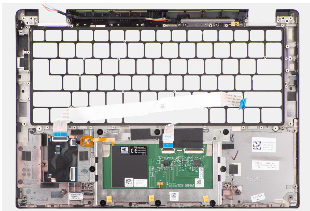
Figur 84. Ta bort handledsstödet
