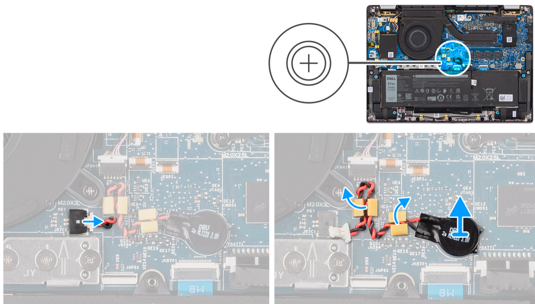
Figur 35. Ta bort knappcellsbatteriet
