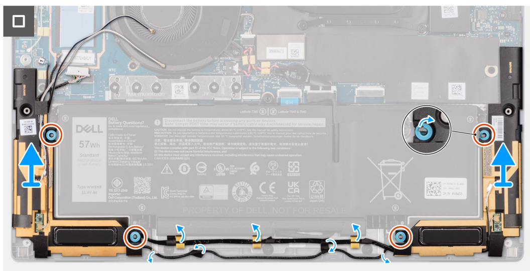
Figur 30. Ta bort högtalarna för ultralight
