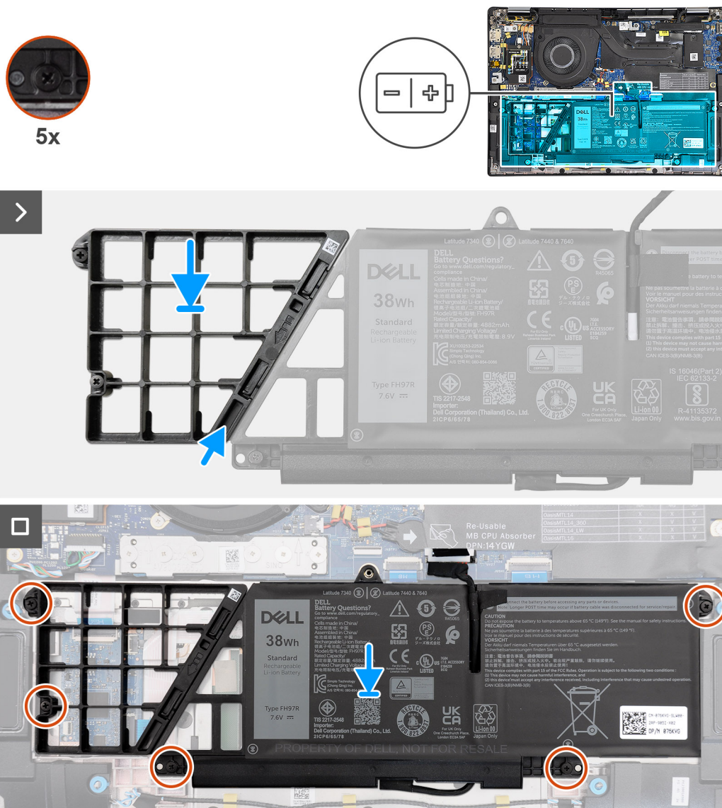
Figur 39. Installera 2-cellsbatteriet
