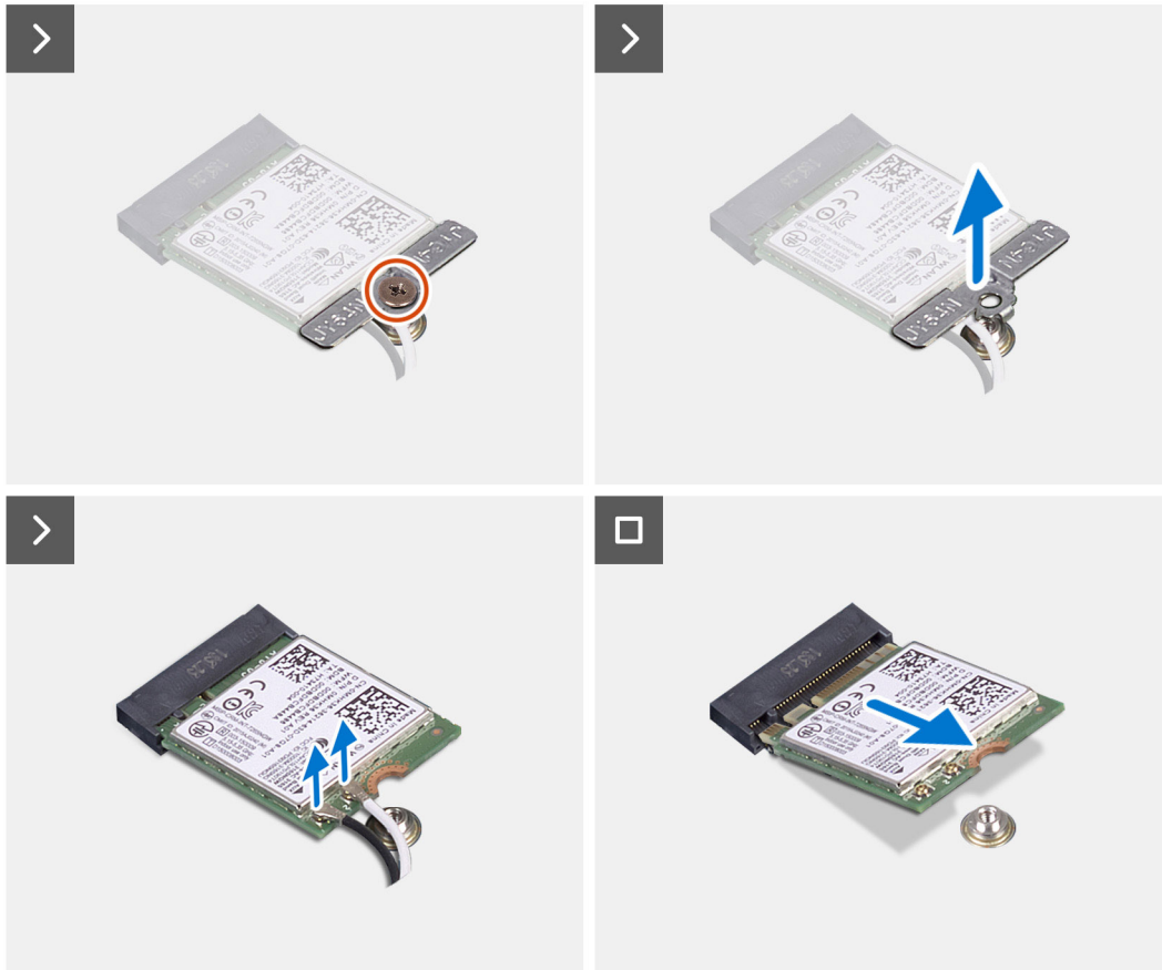
Afbeelding 19. De draadloze kaart verwijderen
