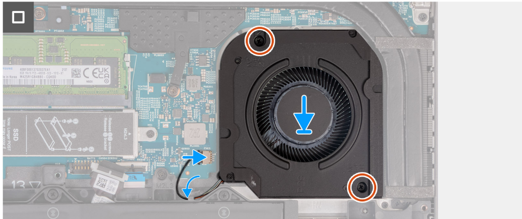
Afbeelding 34. De ventilator installeren
