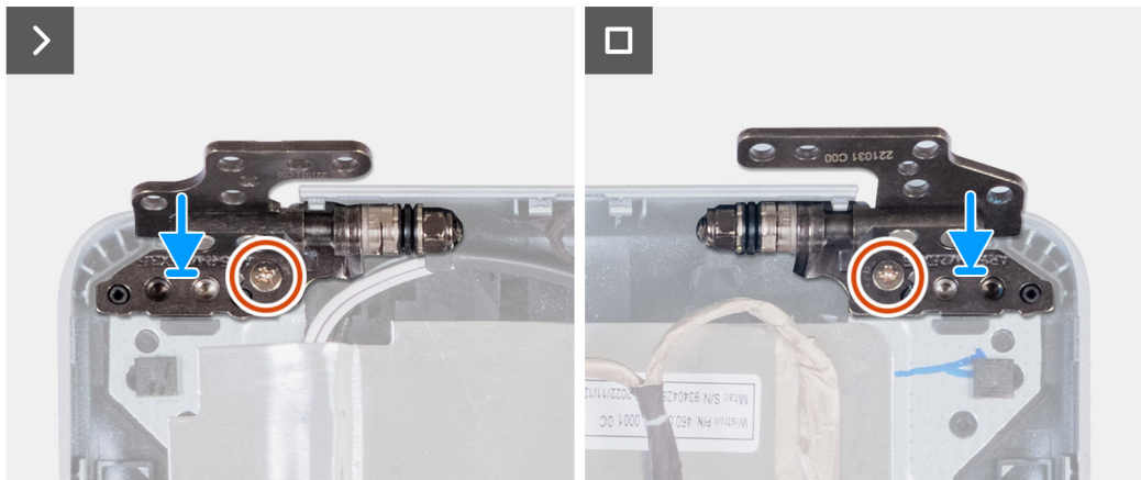
Afbeelding 87. De beeldschermsharnieren installeren
