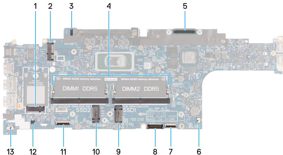
Afbeelding 57. Systeemkaartconnectoren
