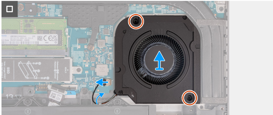
Afbeelding 33. De ventilator verwijderen
