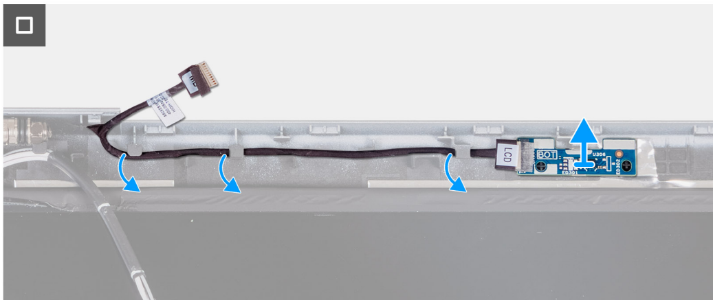
Afbeelding 92. De sensorkaart verwijderen
