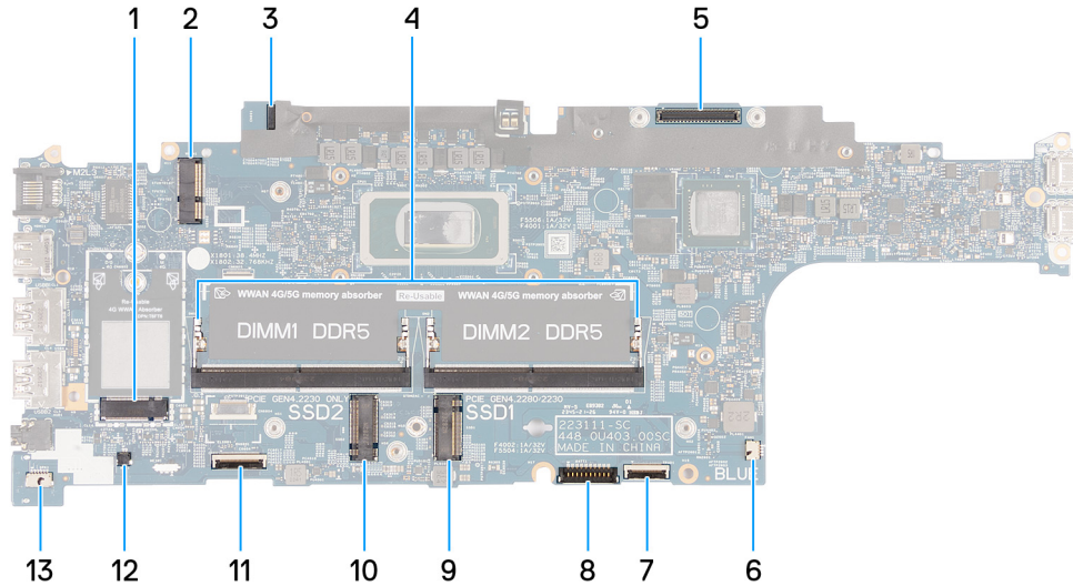
Afbeelding 52. Systeemkaartconnectoren
