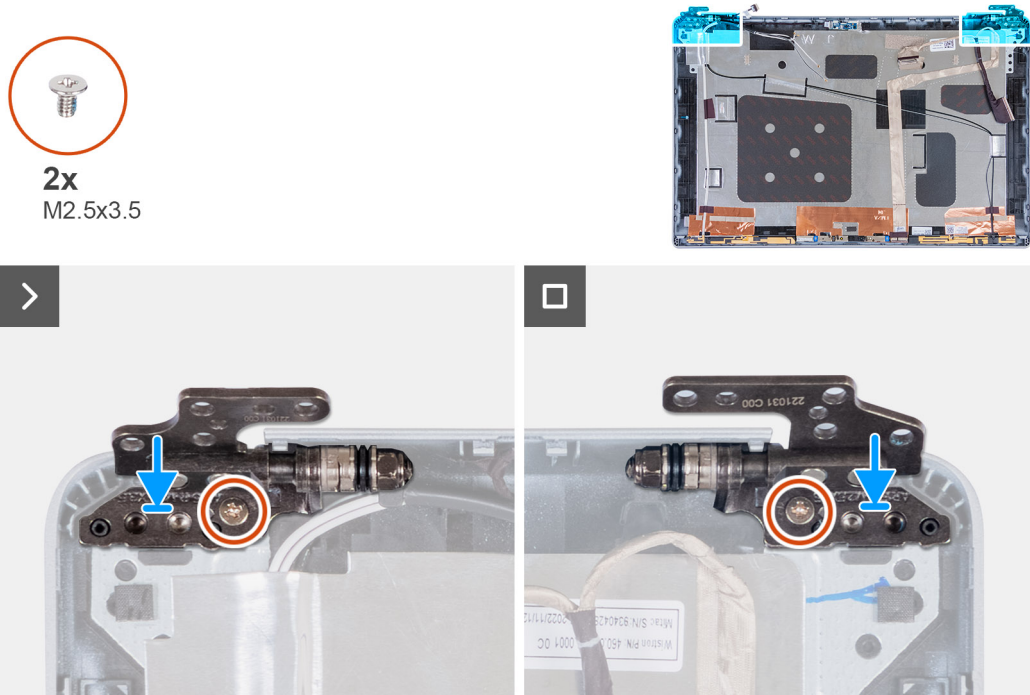
Figura 91. Installazione delle cerniere del display
