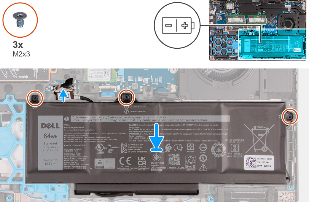
Figura 39. Installazione della batteria da 64 Wh
