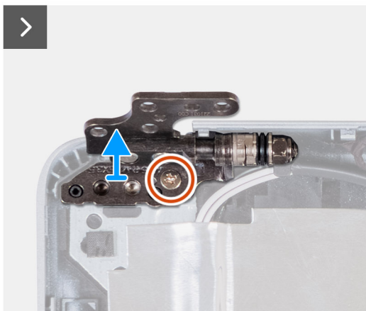
Figura 90. Rimozione delle cerniere del display
