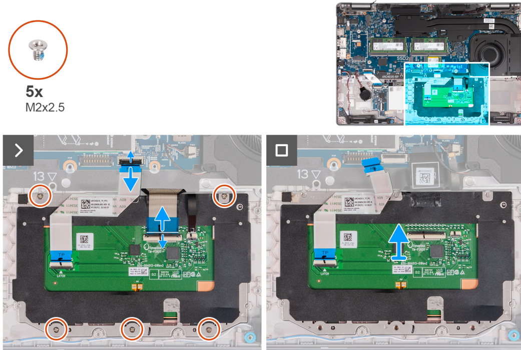
Figura 45. Rimozione del trackpad
