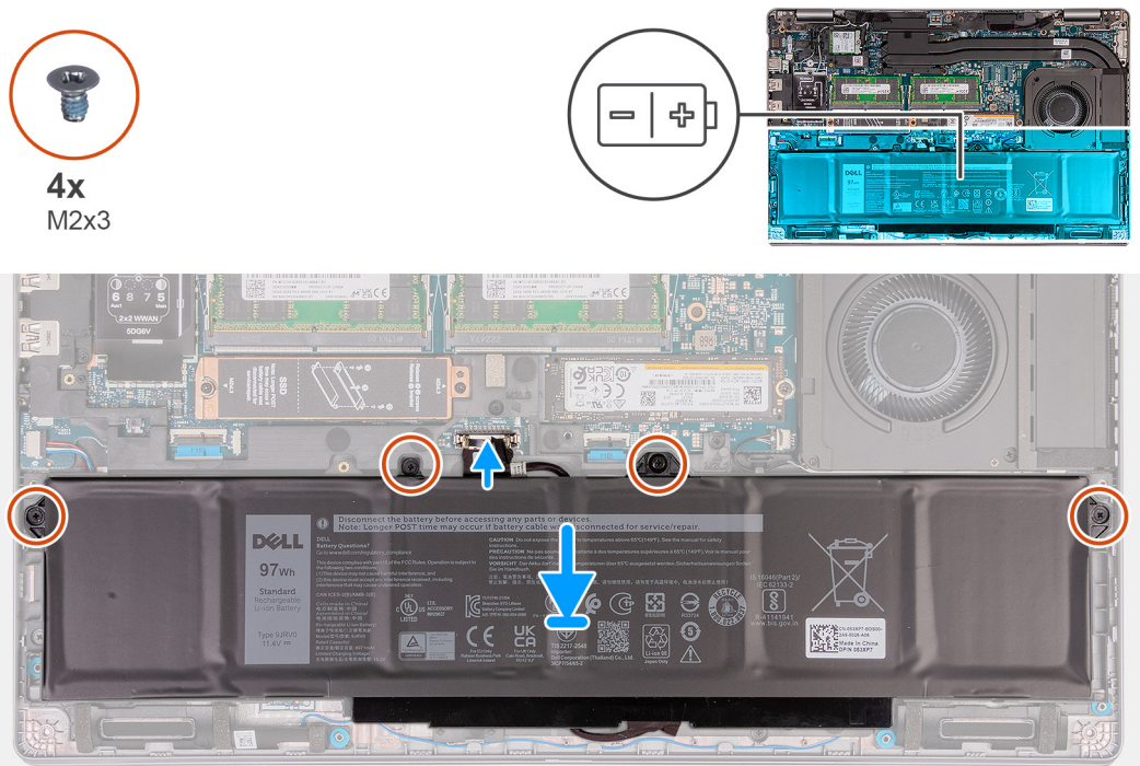
Figura 40. Installazione della batteria da 97 Wh
