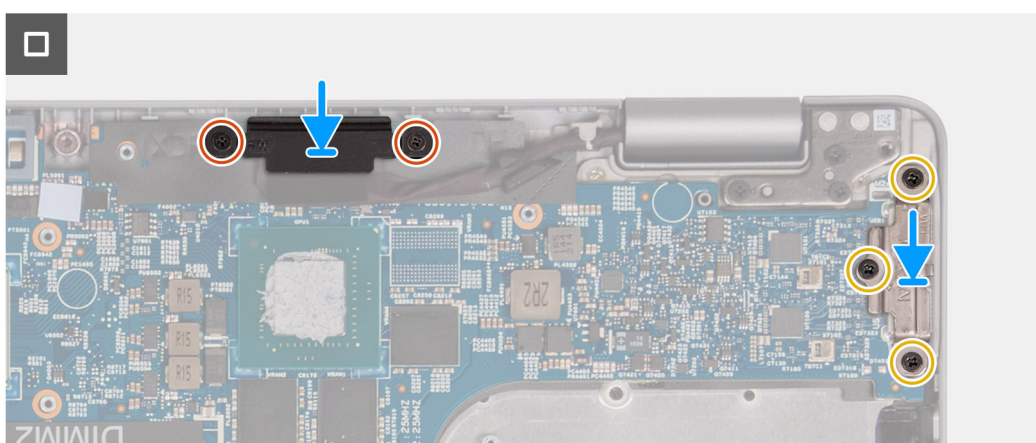
Figura 64. Installazione della scheda di sistema
