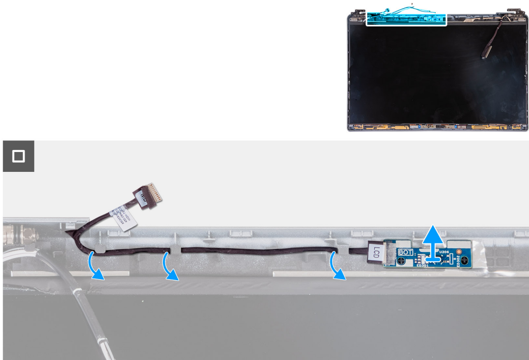
Figura 96. Rimozione della scheda sensore
