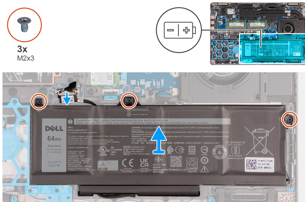
Figura 37. Rimozione della batteria: 64 Wh
