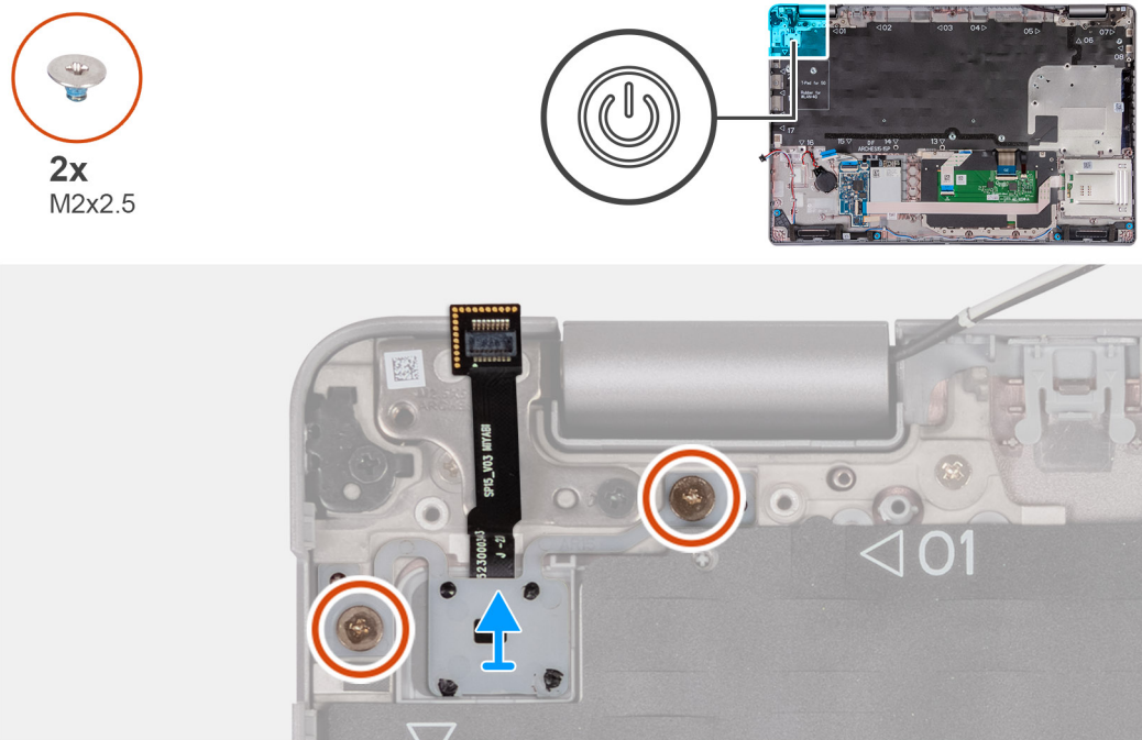
Figura 65. Rimozione del pulsante di accensione
