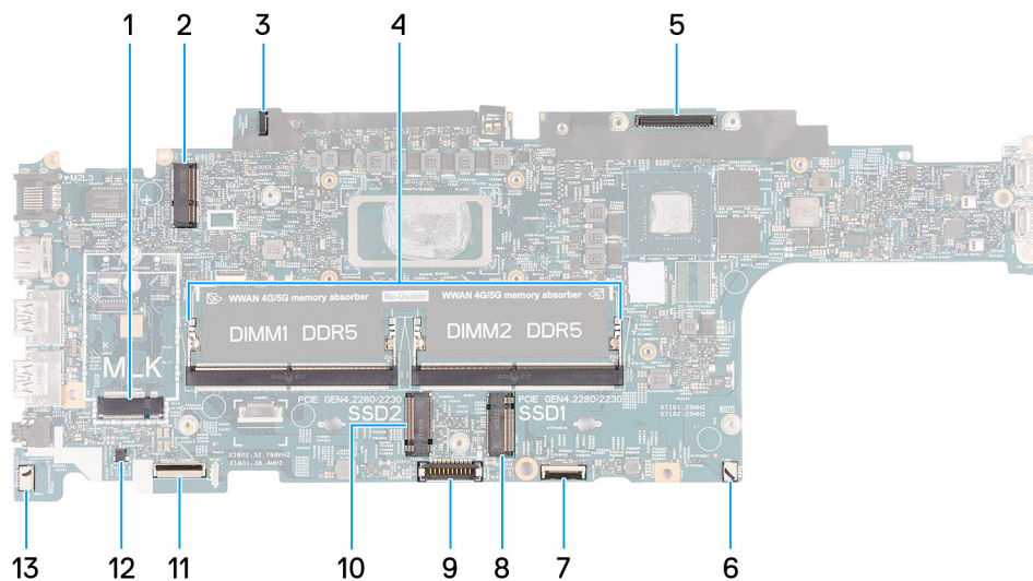
Figura 56. Connettori della scheda di sistema
