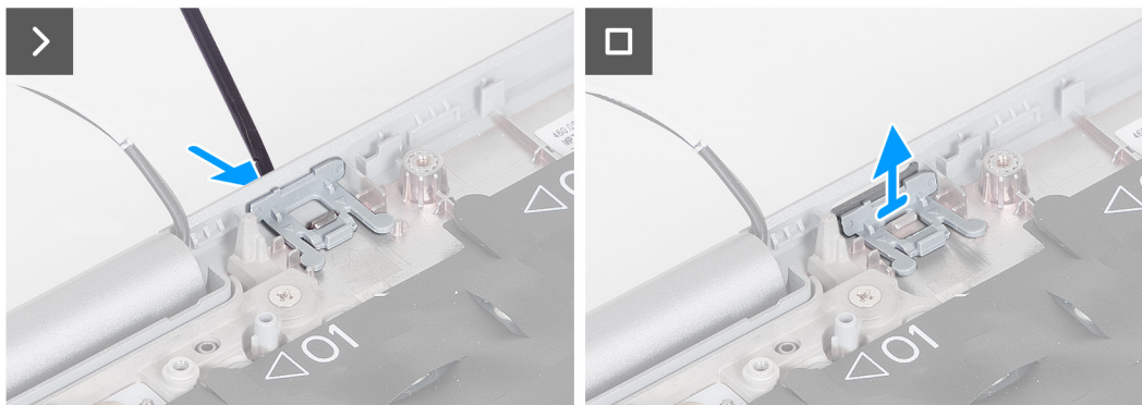
Figura 100. Rimozione del riempimento dello slot per schede SIM fittizie
