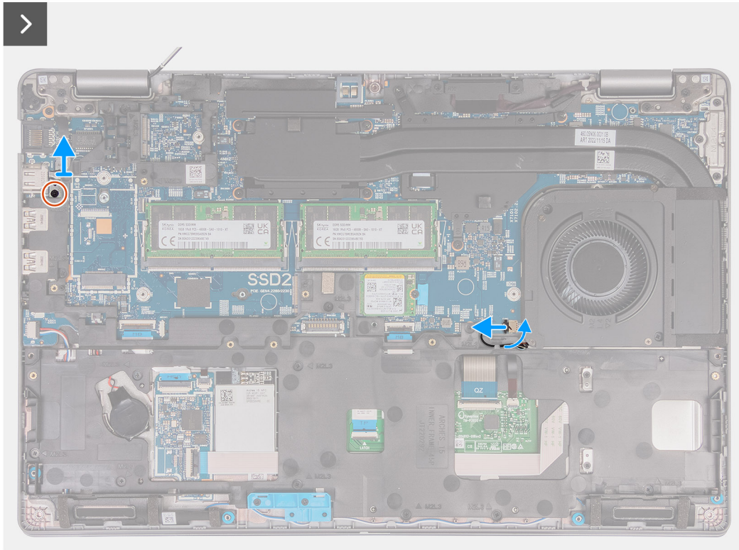
Figura 41. Rimozione del telaio interno del gruppo
