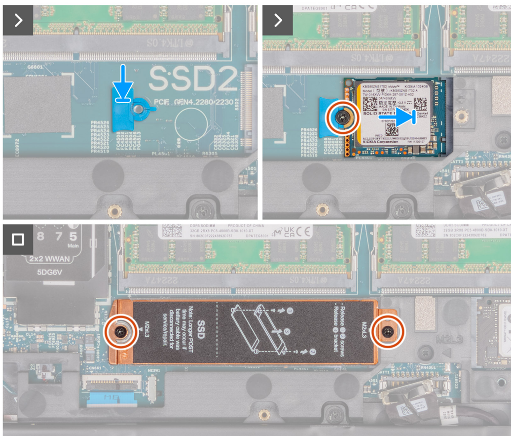
Figura 32. Installazione dell'SSD M.2 2230 nello slot 2
