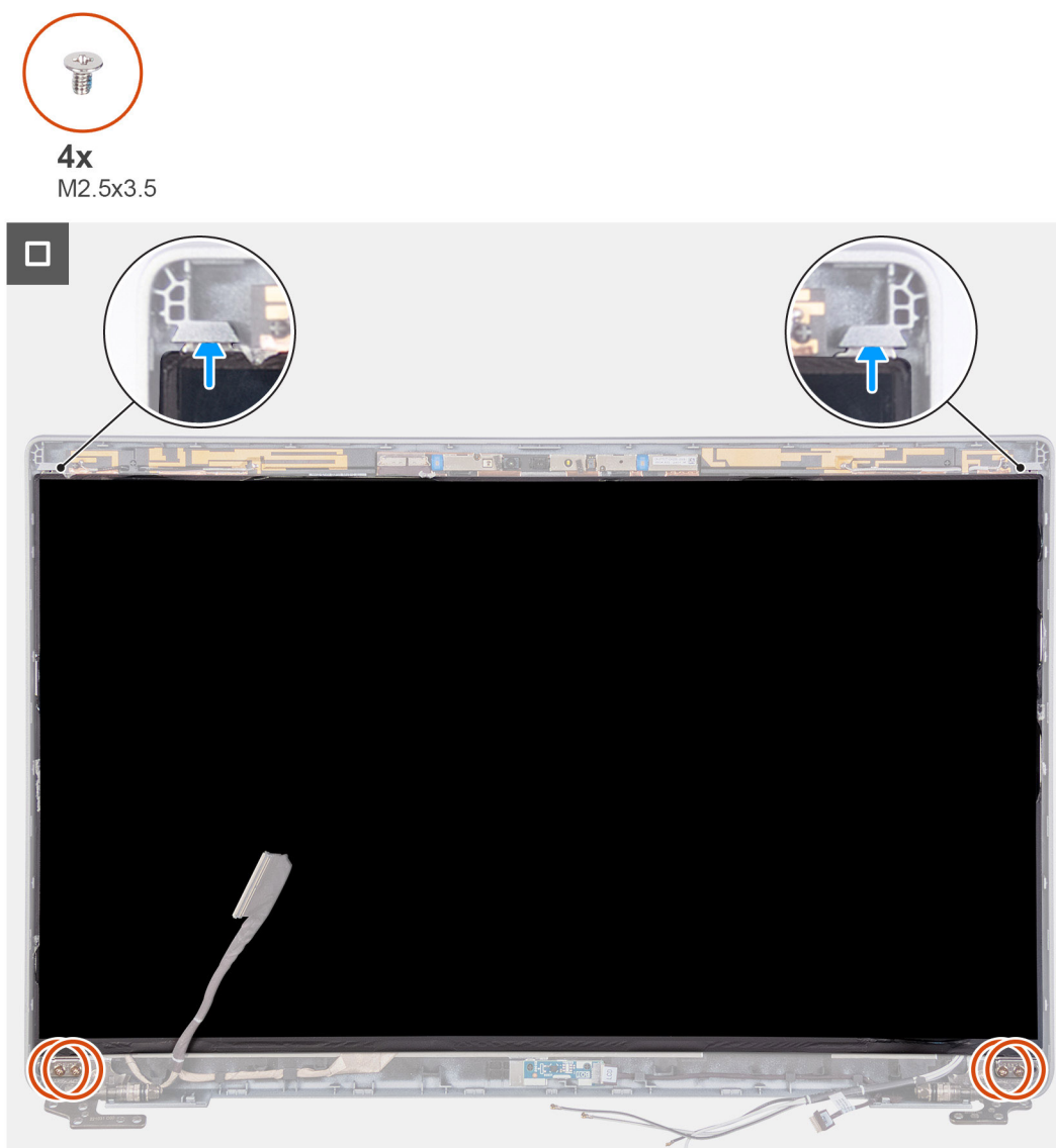
Figura 87. Installazione del pannello del display
