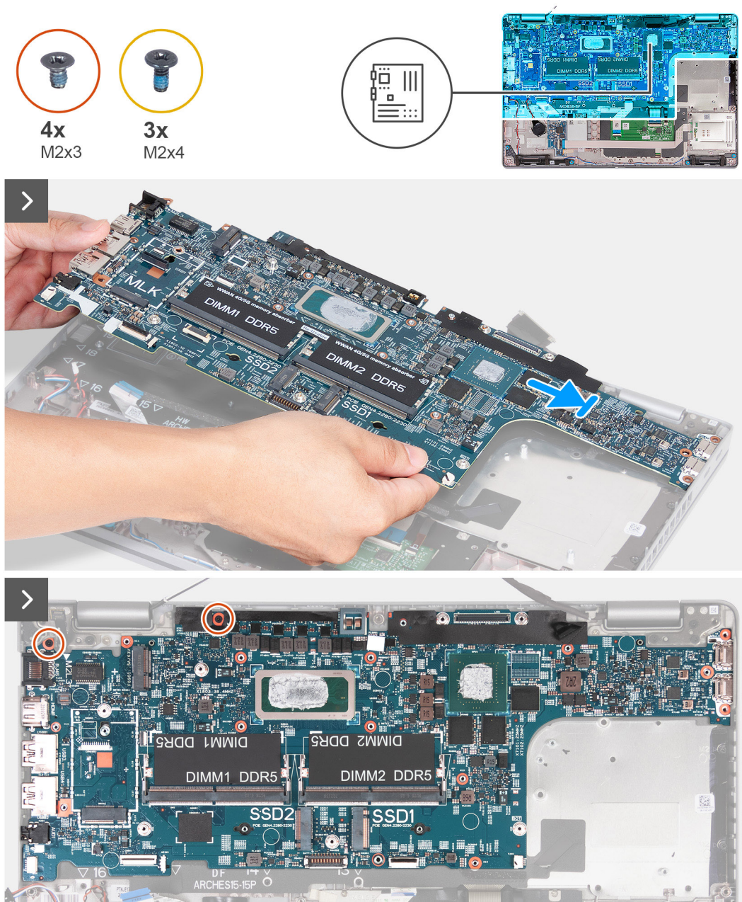
Figura 62. Installazione della scheda di sistema
