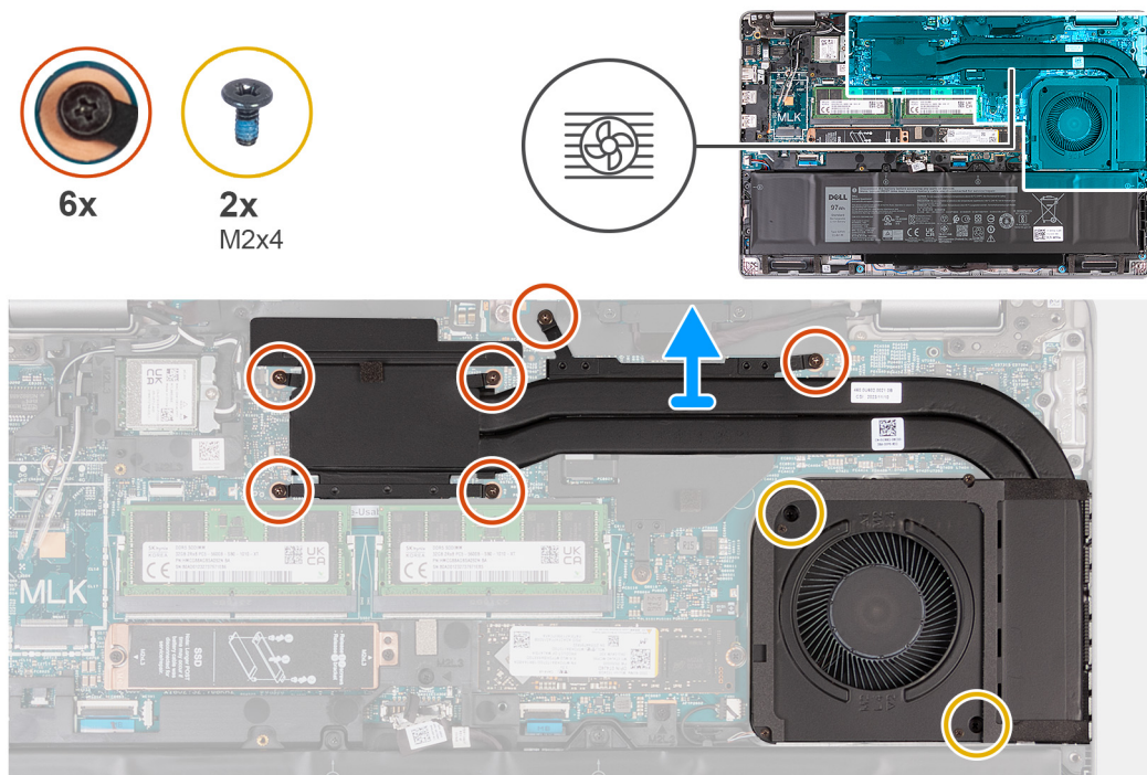
Figura 52. Rimozione del dissipatore di calore (GPU dedicata)
