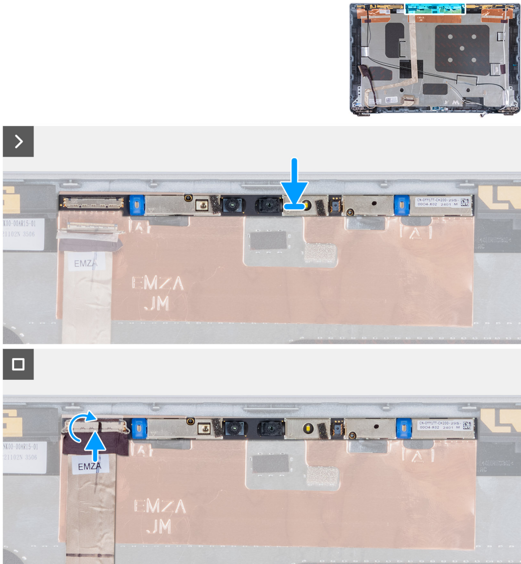
Figura 89. Installazione del modulo della fotocamera
