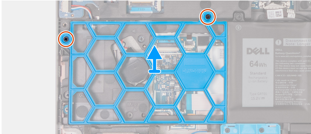
Figura 35. Rimozione del riempimento in plastica
