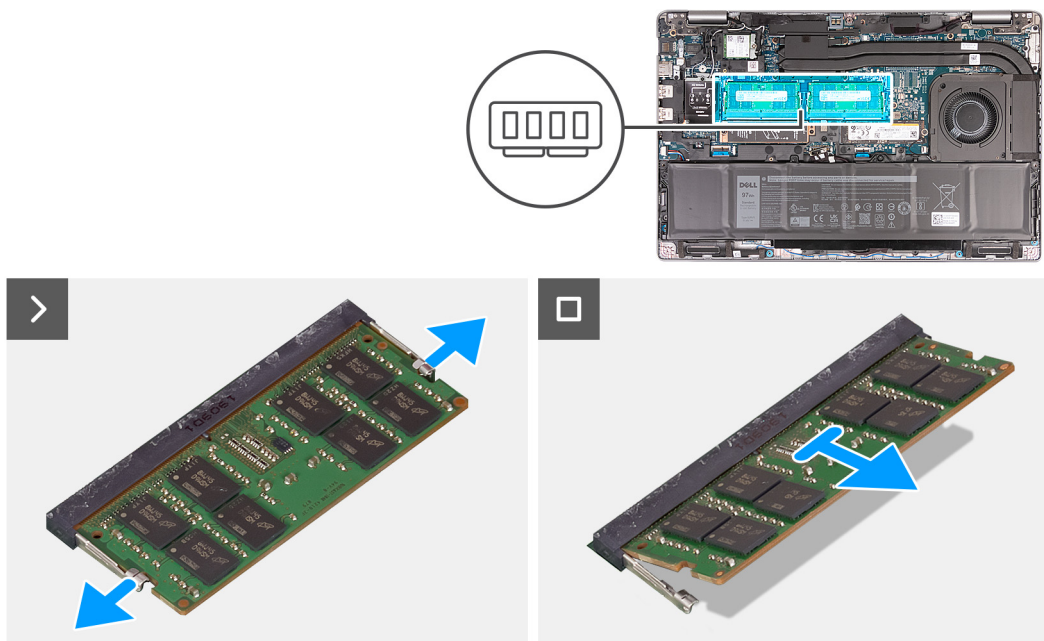
Figura 25. Rimozione del modulo di memoria
