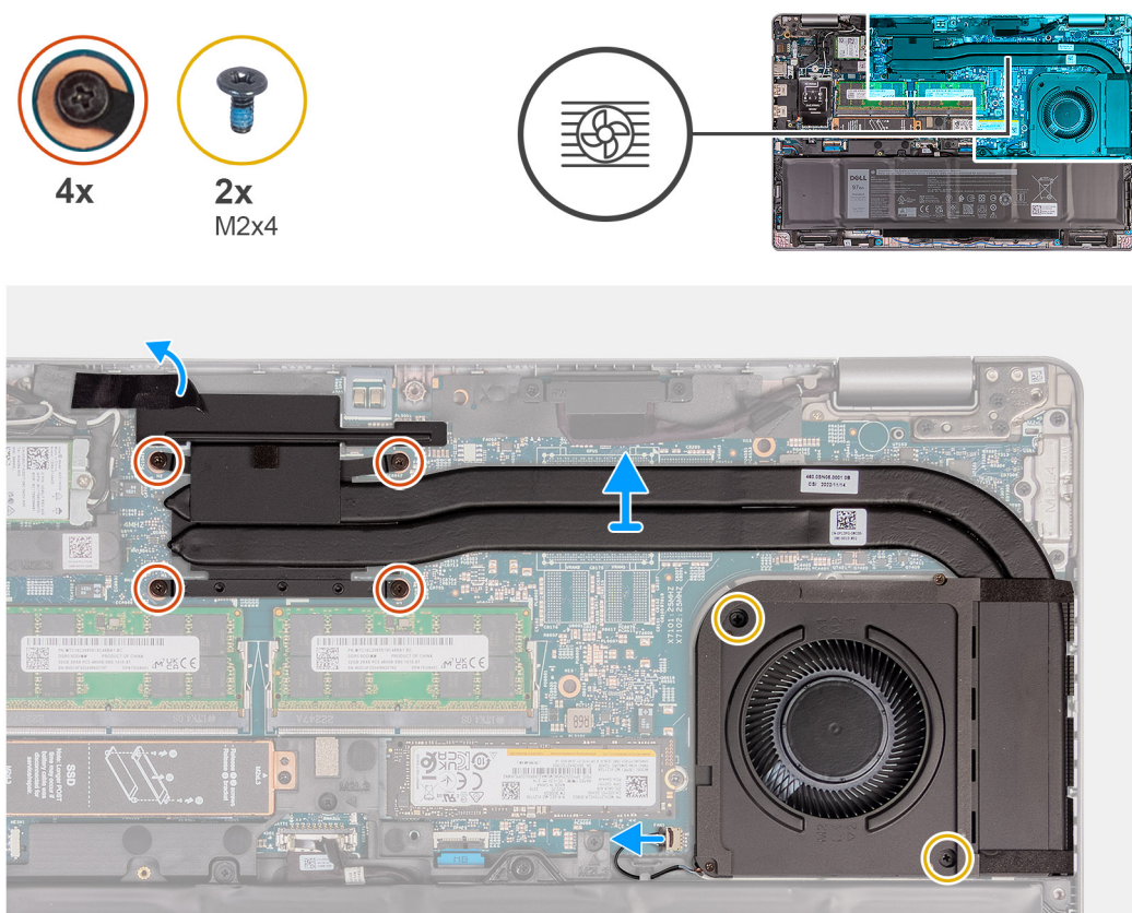
Figura 54. Rimozione del gruppo ventola e dissipatore di calore (GPU integrata)
