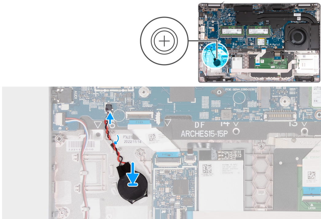
Figura 51. Installazione della batteria a bottone
