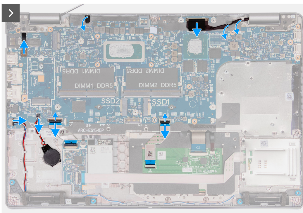
Figura 58. Rimozione della scheda di sistema
