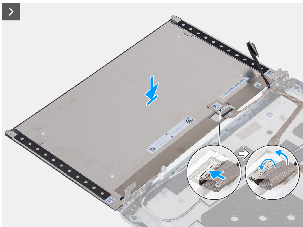
Figura 85. Installazione del pannello del display
