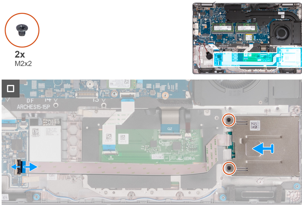
Figura 98. Rimozione del lettore di smart card
