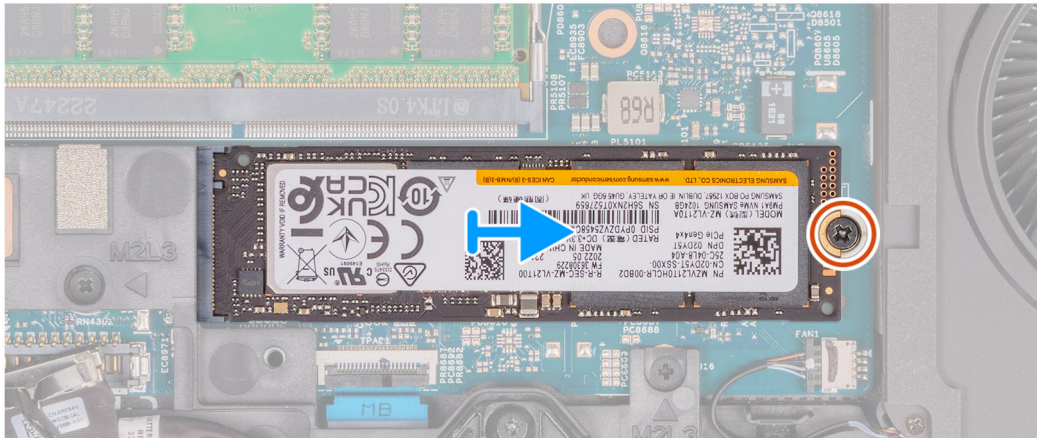
Figura 29. Rimozione dell'SSD M. 2 2280 dallo slot 1
