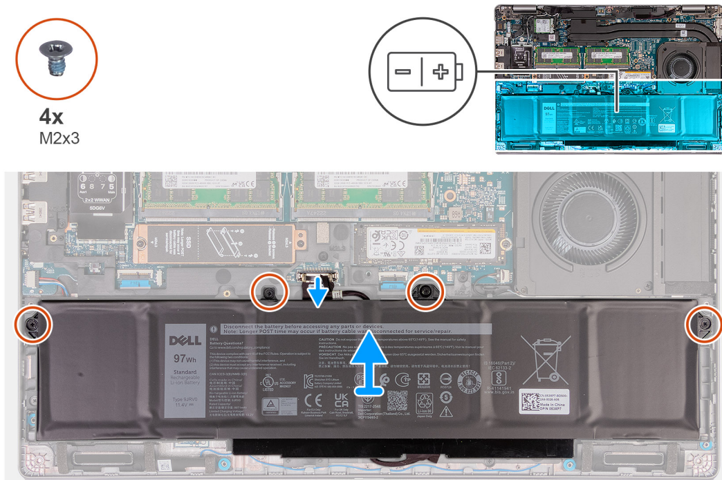
Figura 38. Rimozione della batteria: 97 Wh
