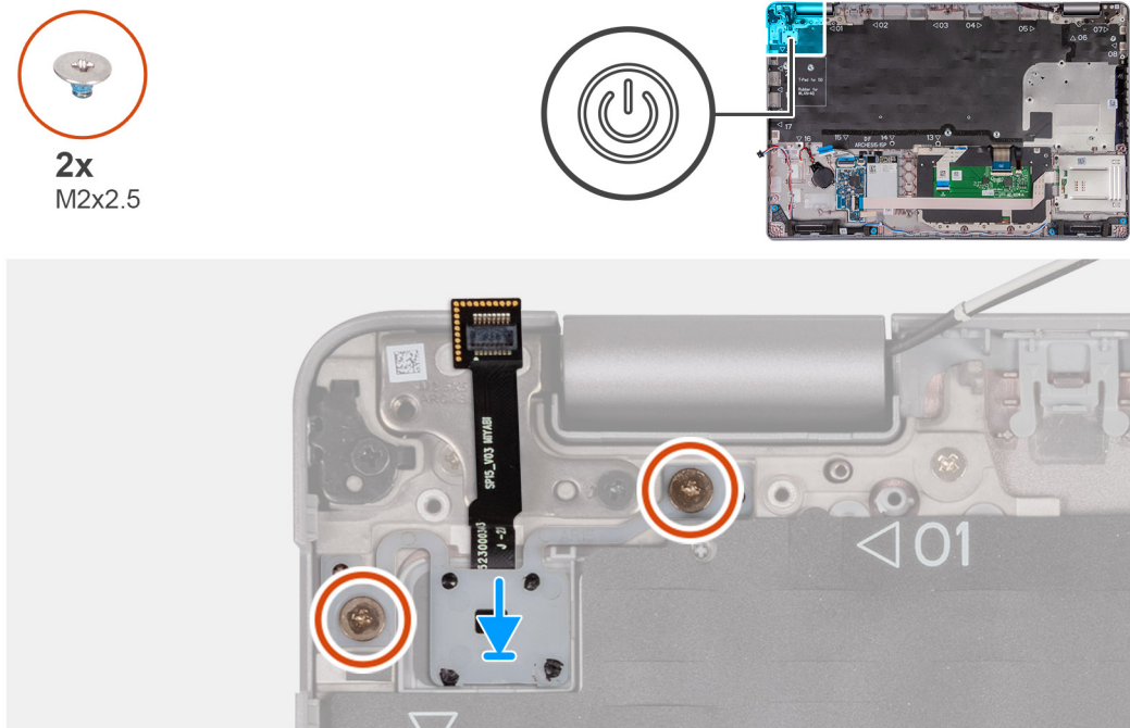
Figura 68. Installazione del pulsante di accensione con lettore di impronte digitali opzionale
