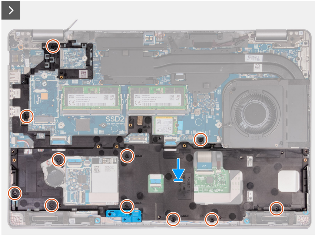
Figura 43. Installazione del telaio interno del gruppo
