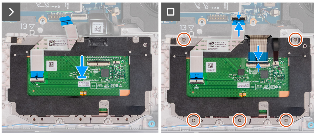
Figura 46. Installazione del trackpad
