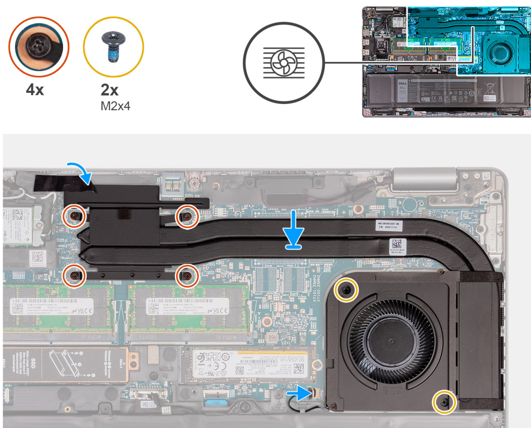
Figura 55. Installazione del gruppo ventola e dissipatore di calore (GPU integrata)
