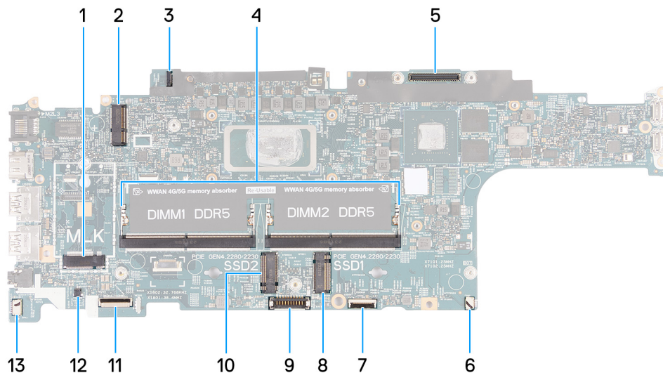
Figura 61. Connettori della scheda di sistema
