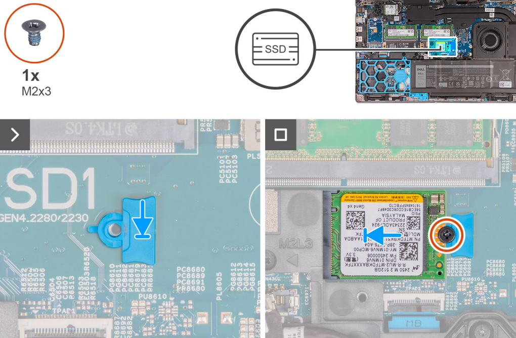
Figura 28. Installazione dell'SSD M.2 2230 nello slot 1
