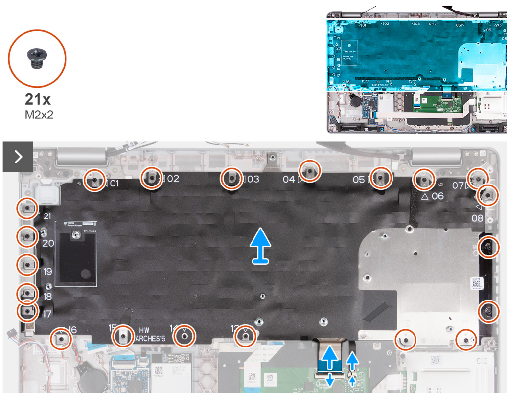
Figura 69. Rimozione della tastiera
