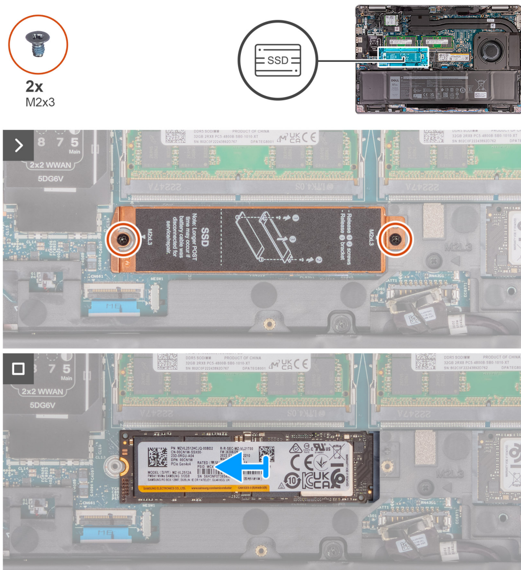
Figura 33. Rimozione dell'SSD M.2 2280 dallo slot 2
