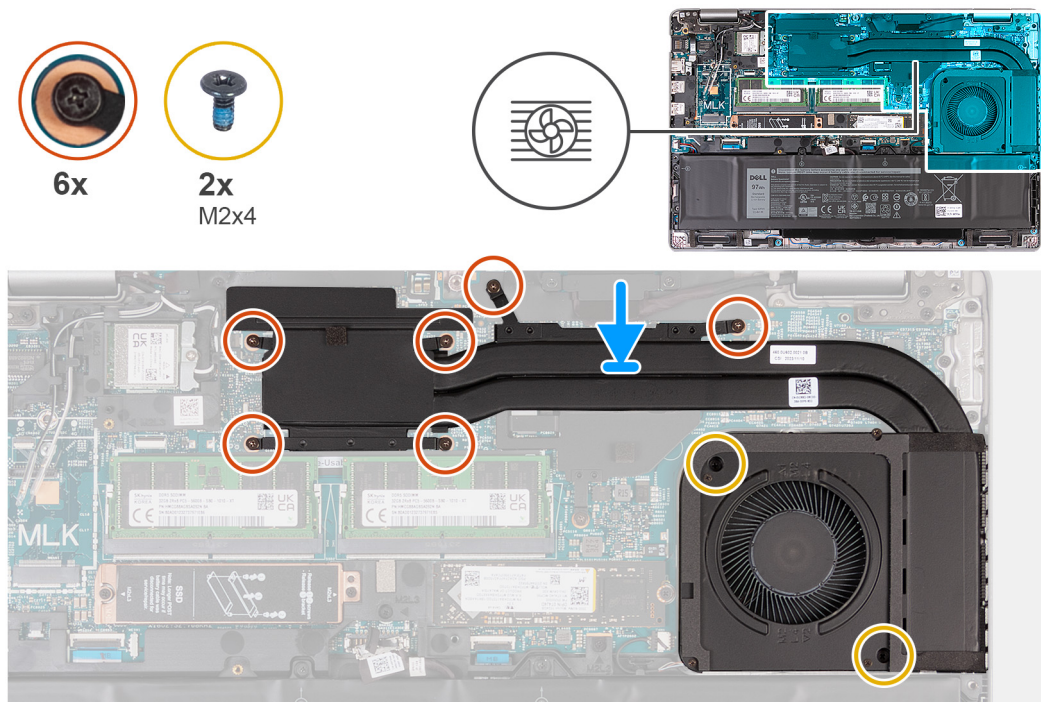
Figura 53. Installazione del dissipatore di calore (GPU dedicata)
