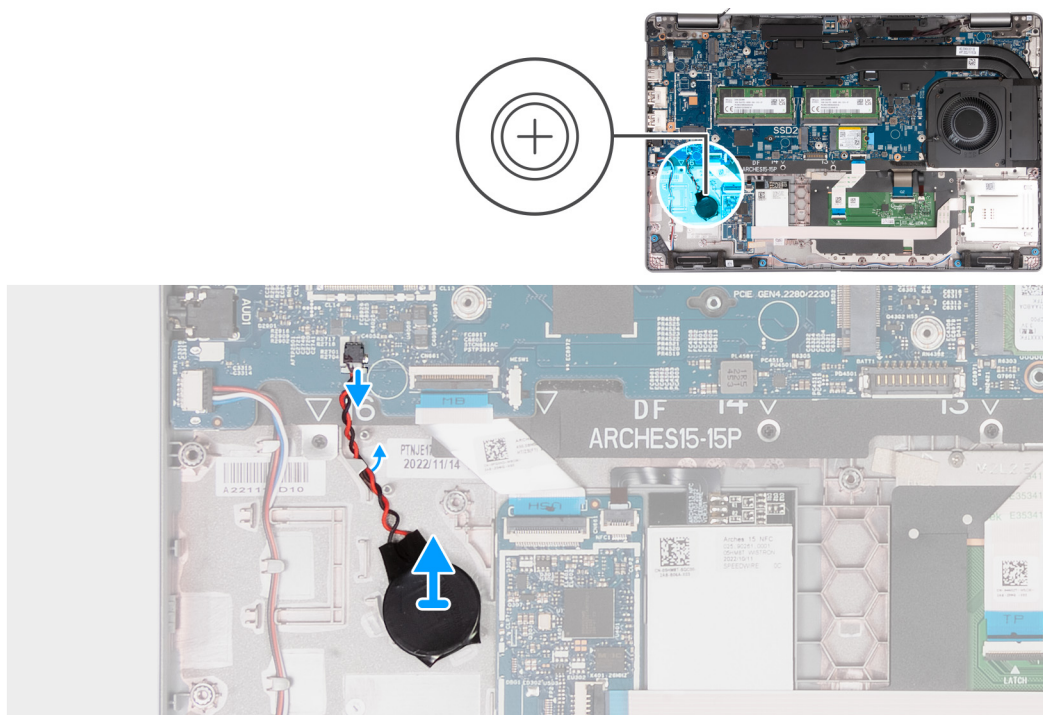
Figura 50. Rimozione della batteria a bottone
