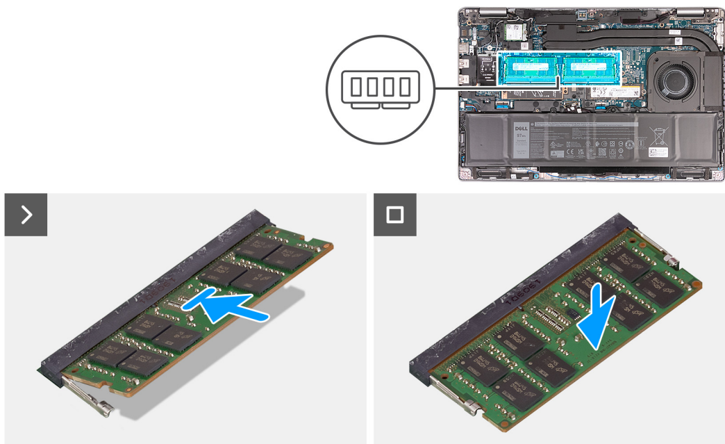
Figura 26. Installazione del modulo di memoria
