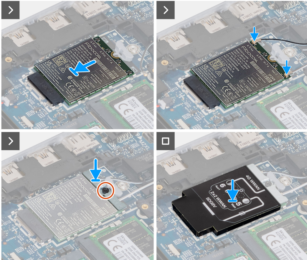
Figura 22. Installazione della scheda WWAN 4G
