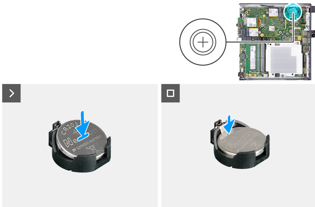
Obrázek 14. Montáž knoflíkové baterie
