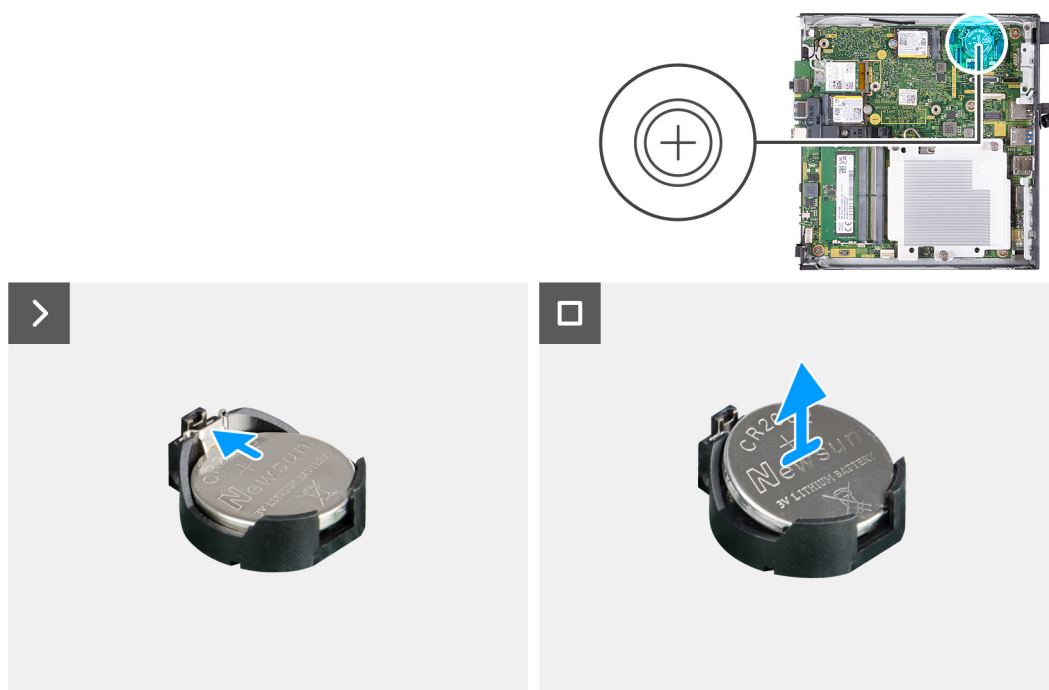
Obrázek 13. Vyjmutí knoflíkové baterie
