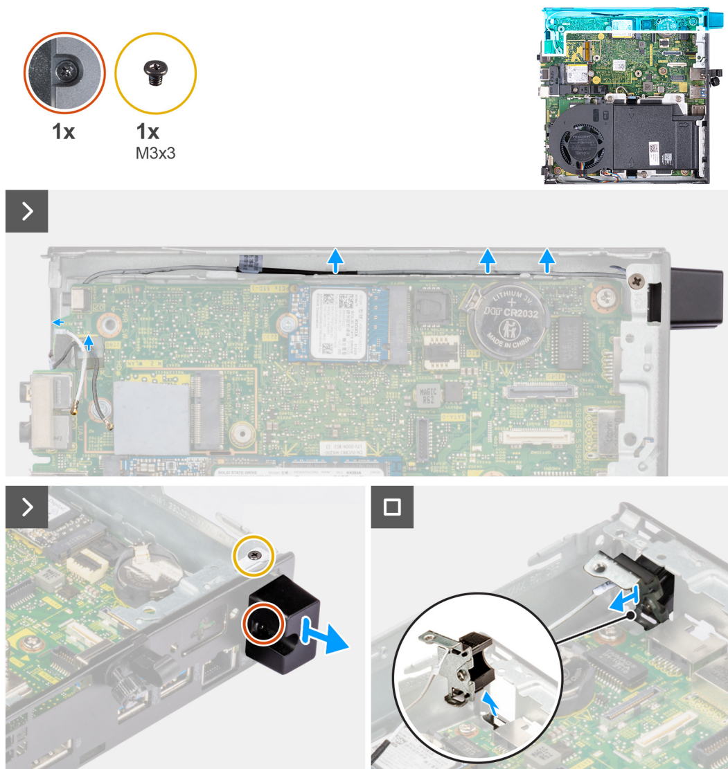
Obrázek 50. Demontáž anténního modulu (bílý kabel)
