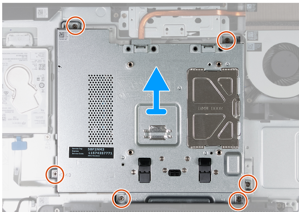
Obrázek 25. Demontáž krytu základní desky
