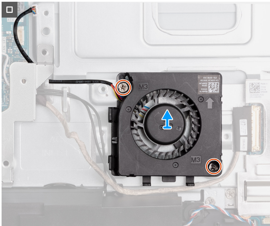
Obrázek 53. Demontáž jednotky ventilátoru napájecího zdroje
