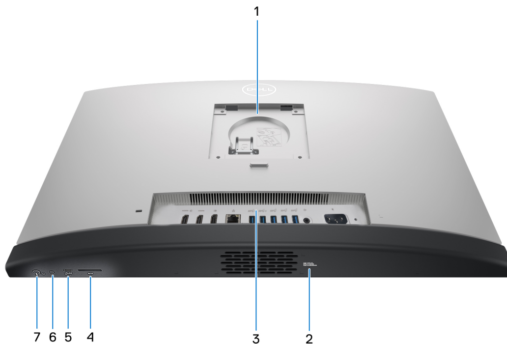
Obrázek 7. Pohled zespodu na počítač OptiPlex All-in-One Plus 7420
