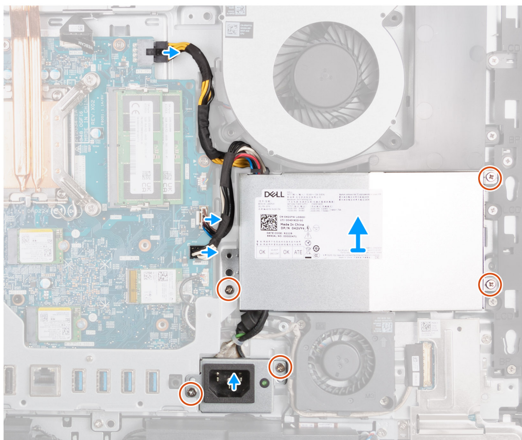
Obrázek 49. Demontáž napájecí jednotky
