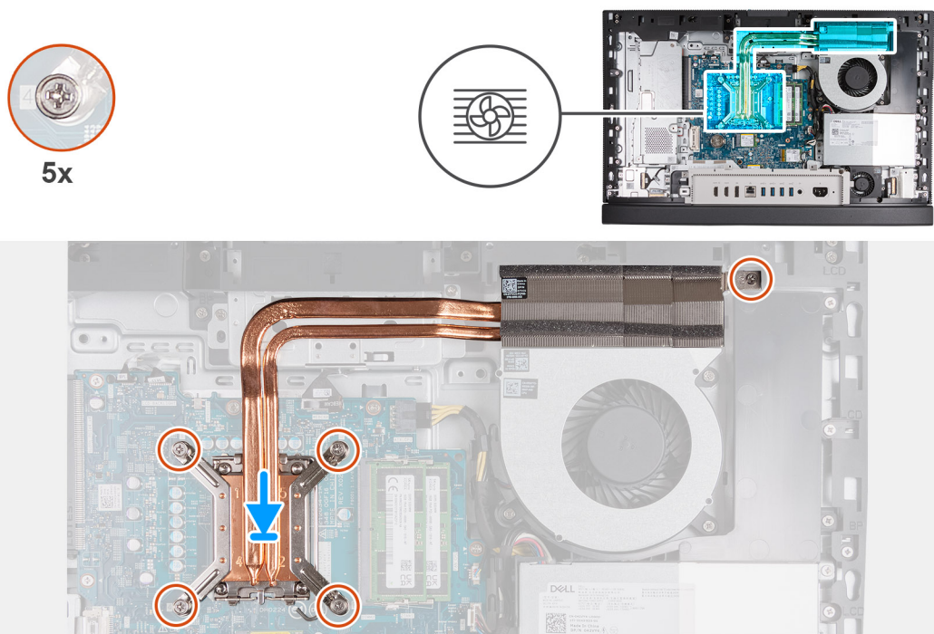
Obrázek 62. Montáž chladiče
