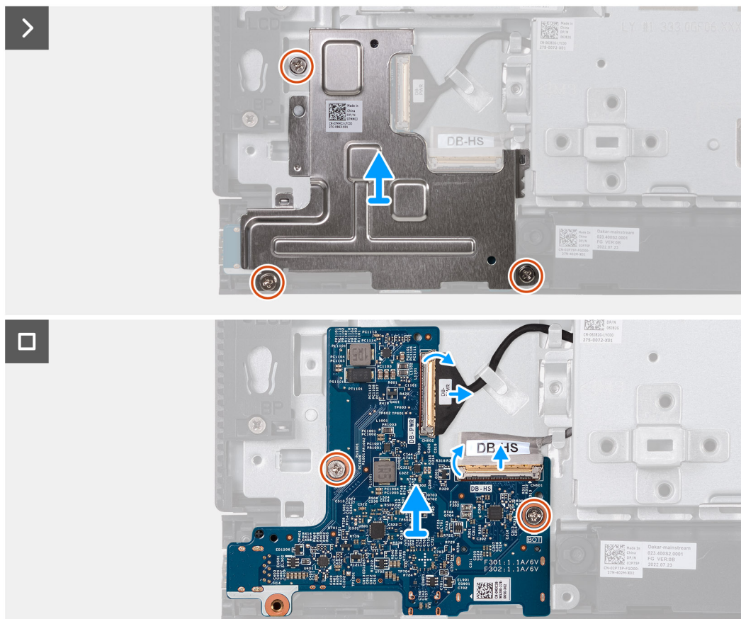
Obrázek 71. Demontáž desky vypínače a I/O
