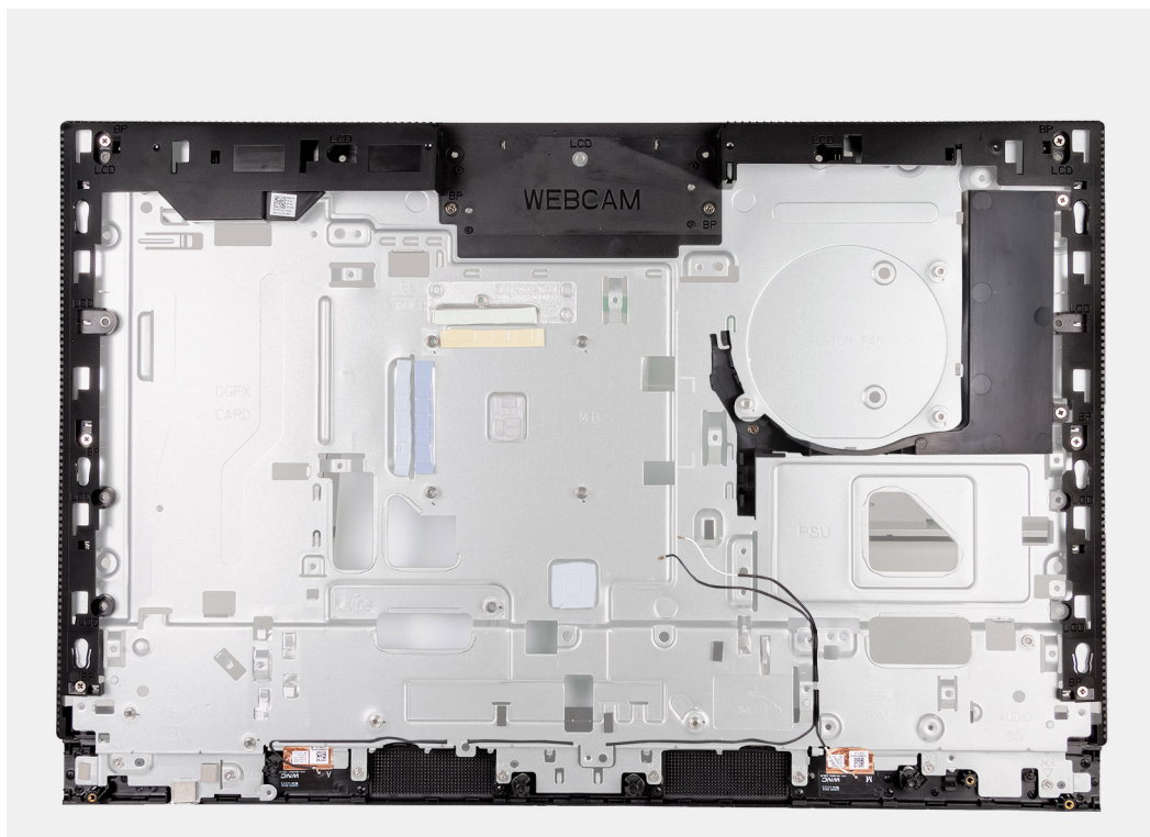
Obrázek 75. Demontáž základny sestavy displeje
