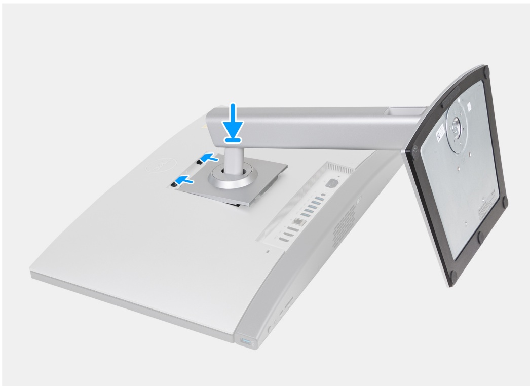
Obrázek 17. Instalace výškově nastavitelného stojanu (HAS)
