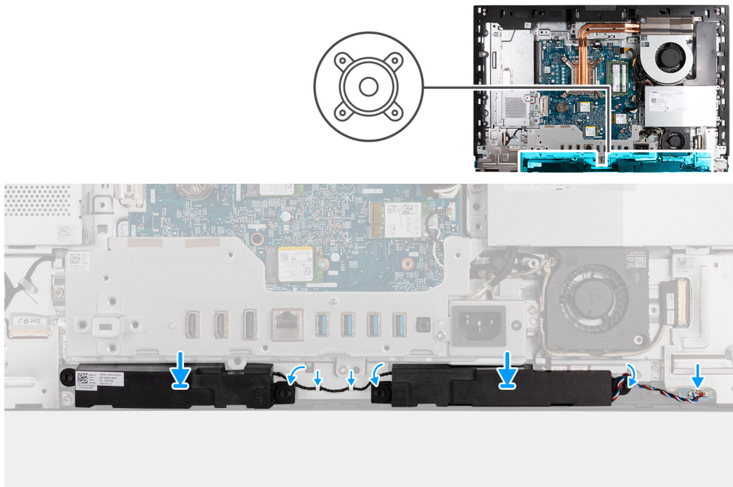
Obrázek 60. Montáž reproduktorů
