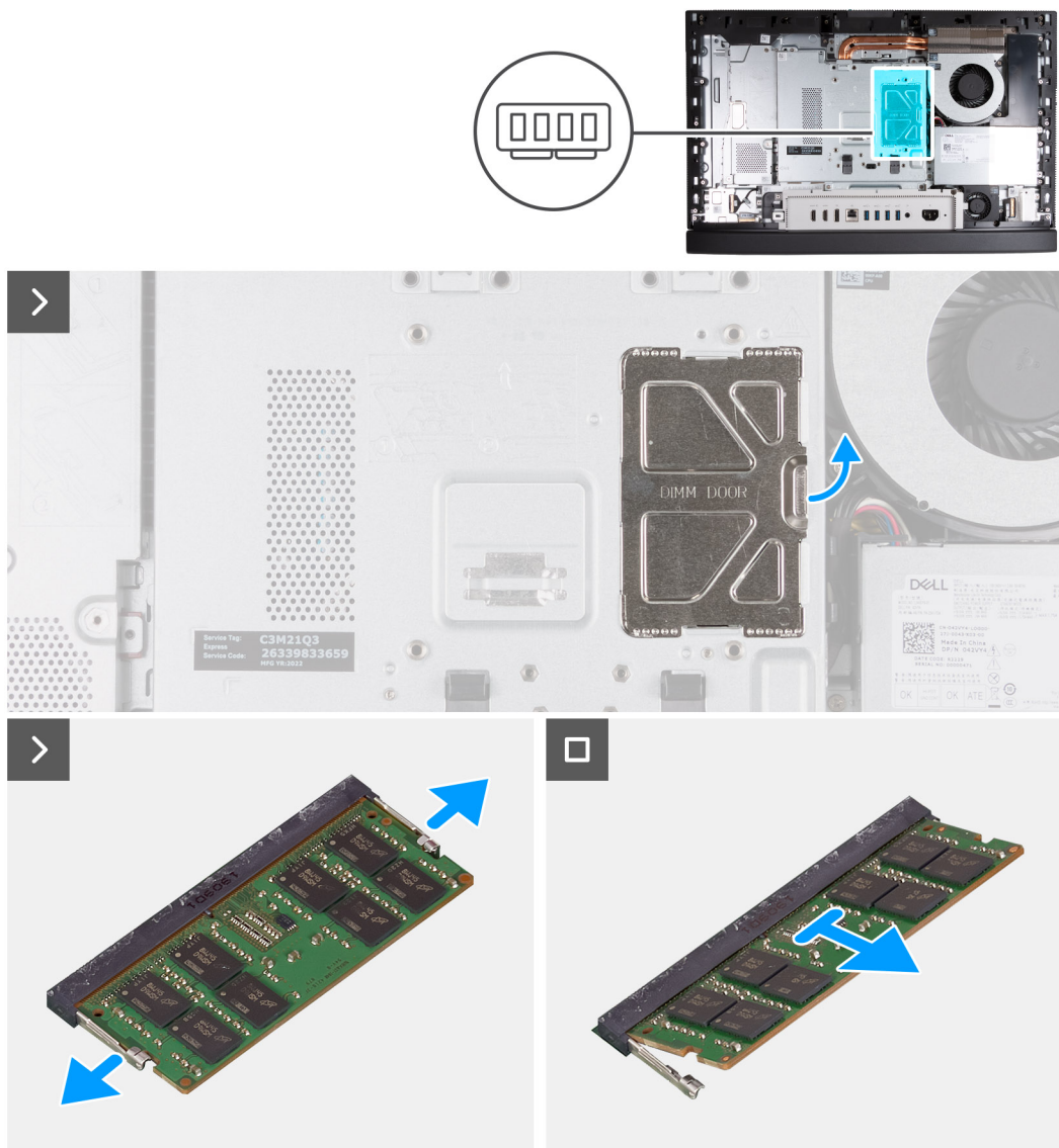
Obrázek 21. Vyjmutí paměti
