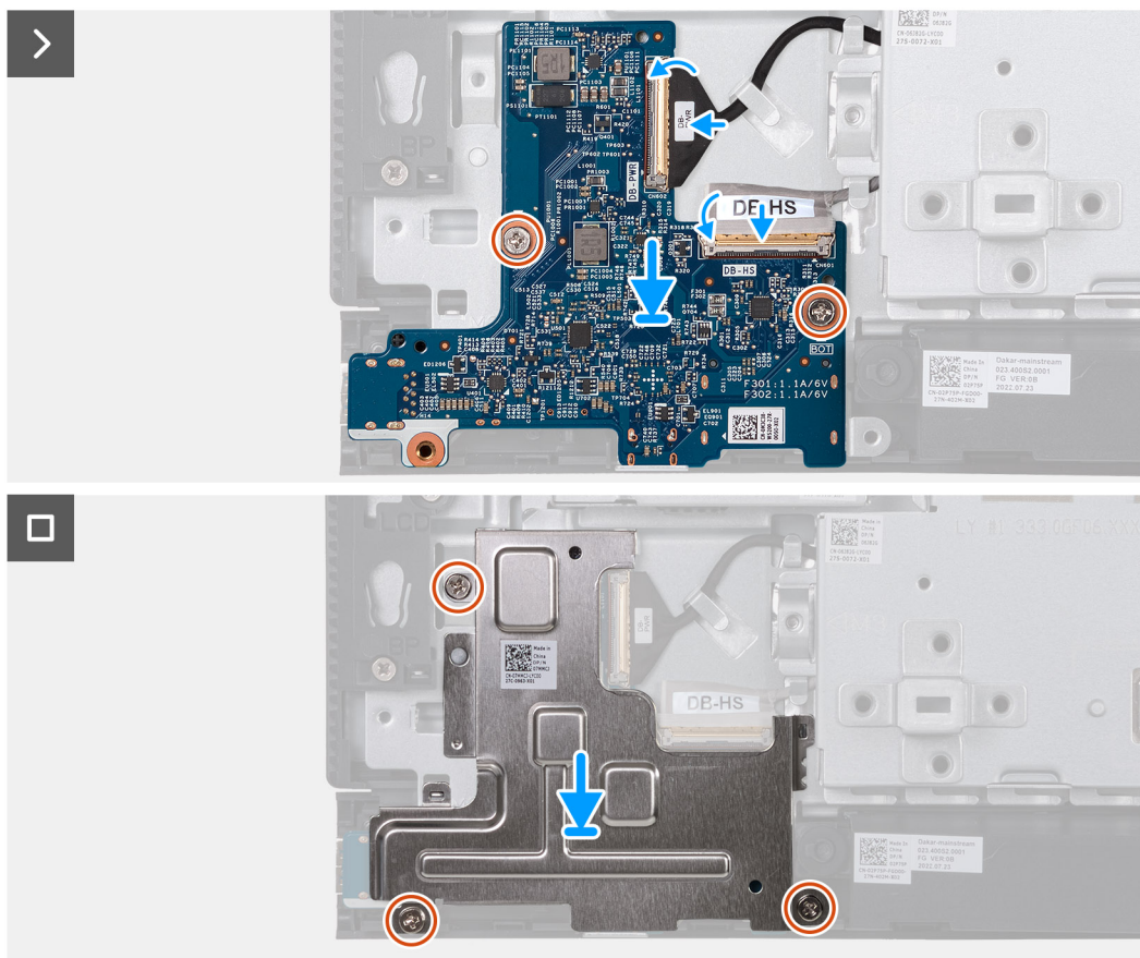
Obrázek 72. Montáž vypínače a desky I/O
