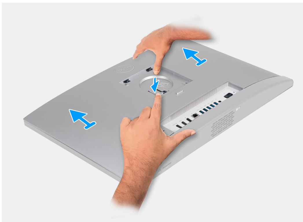
Obrázek 19. Demontáž zadního krytu
