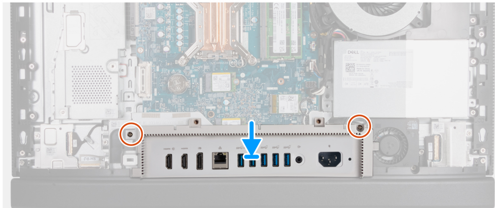
Obrázek 42. Montáž krytu I/O
