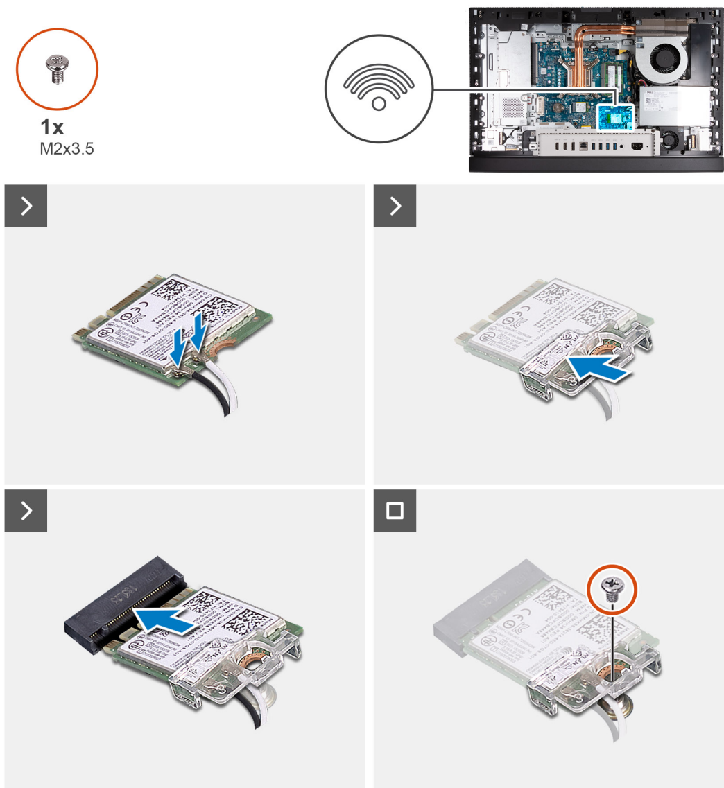
Obrázek 28. Montáž bezdrátové karty
