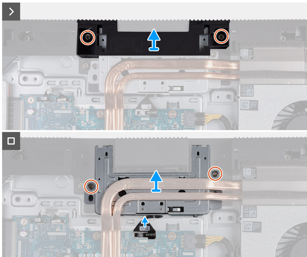
Obrázek 45. Demontáž sestavy zasouvací kamery
