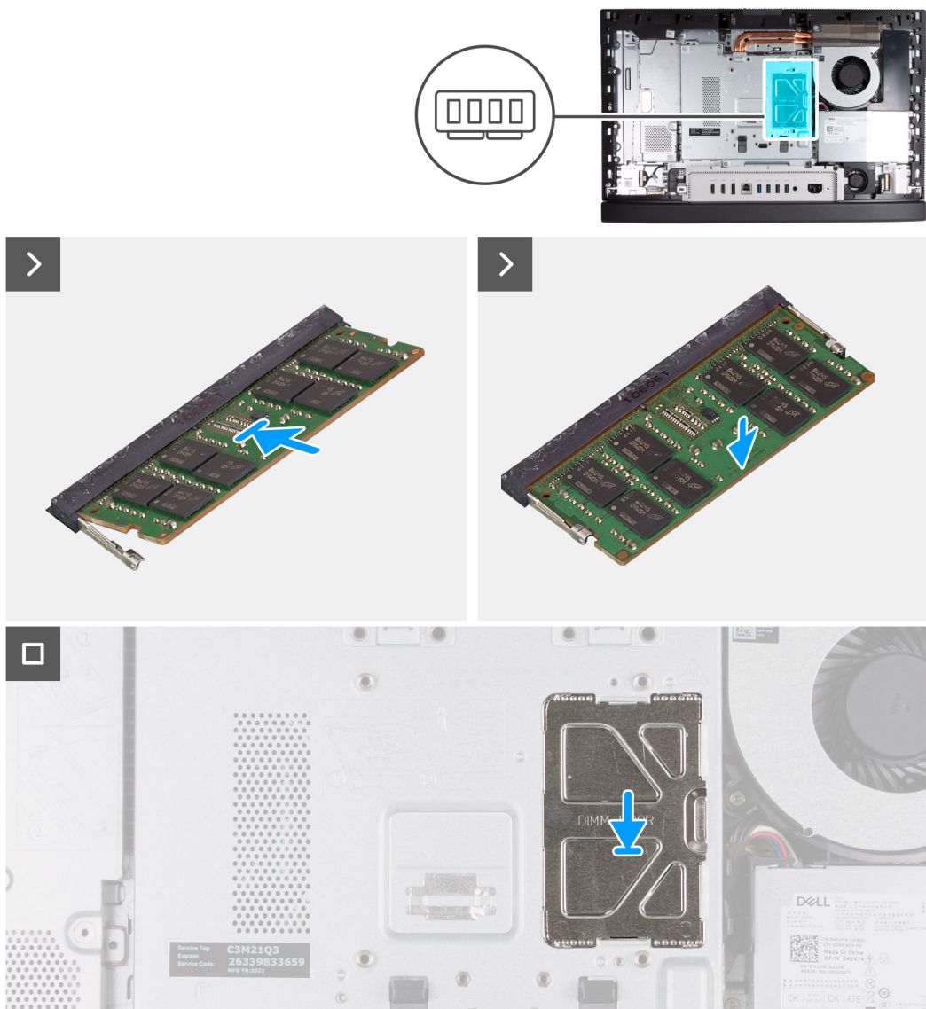
Obrázek 22. Instalace paměti
