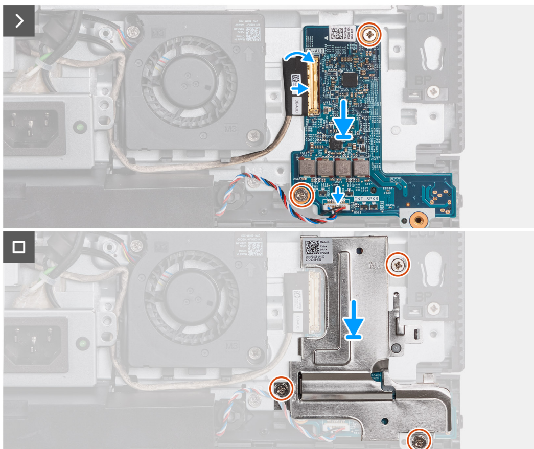
Obrázek 74. Montáž zvukové karty
