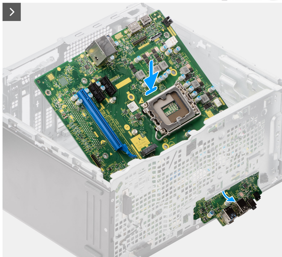
Obrázek 88. Montáž základní desky
