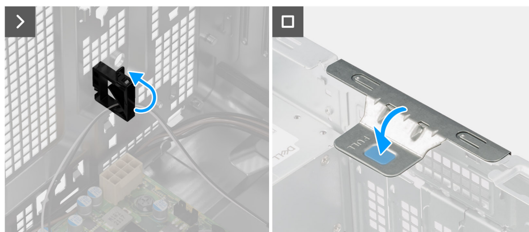
Obrázek 59. Montáž modulu externí antény SMA
