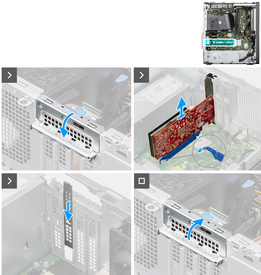
Obrázek 33. Demontáž grafické karty
