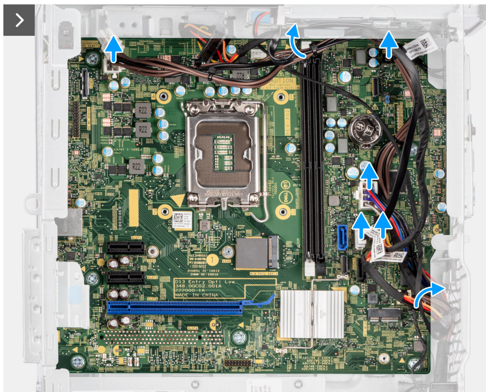
Obrázek 84. Demontáž základní desky
