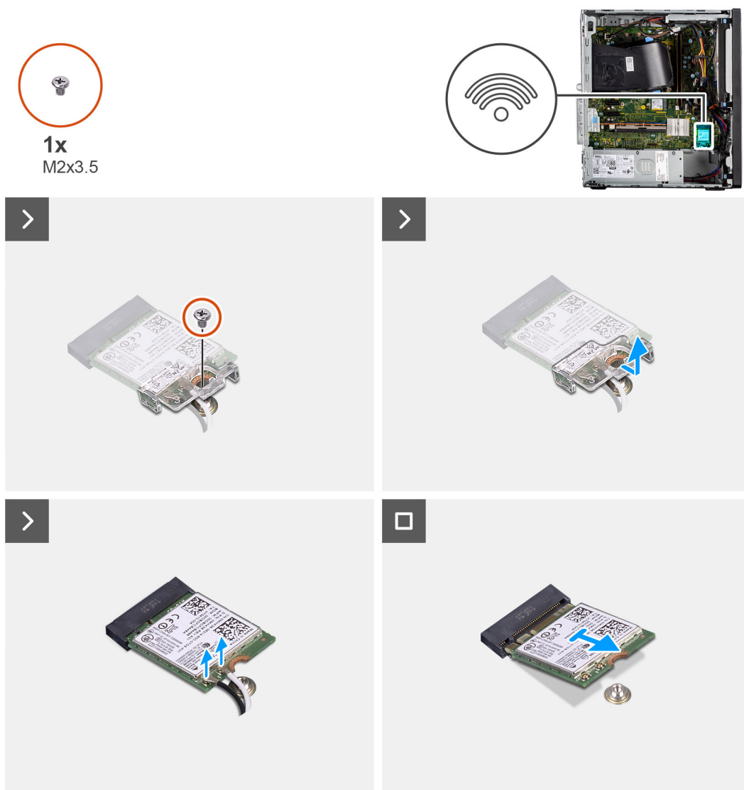
Obrázek 31. Demontáž bezdrátové karty
