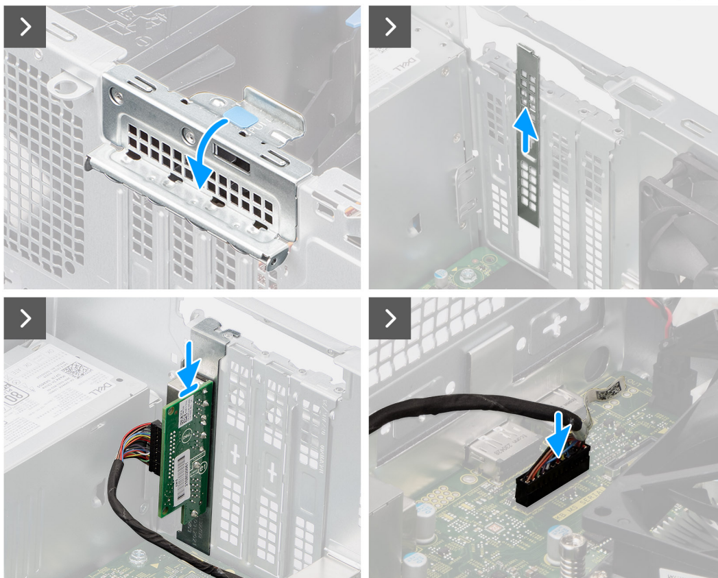
Obrázek 74. Montáž volitelného modulu PS2 a sériového modulu
