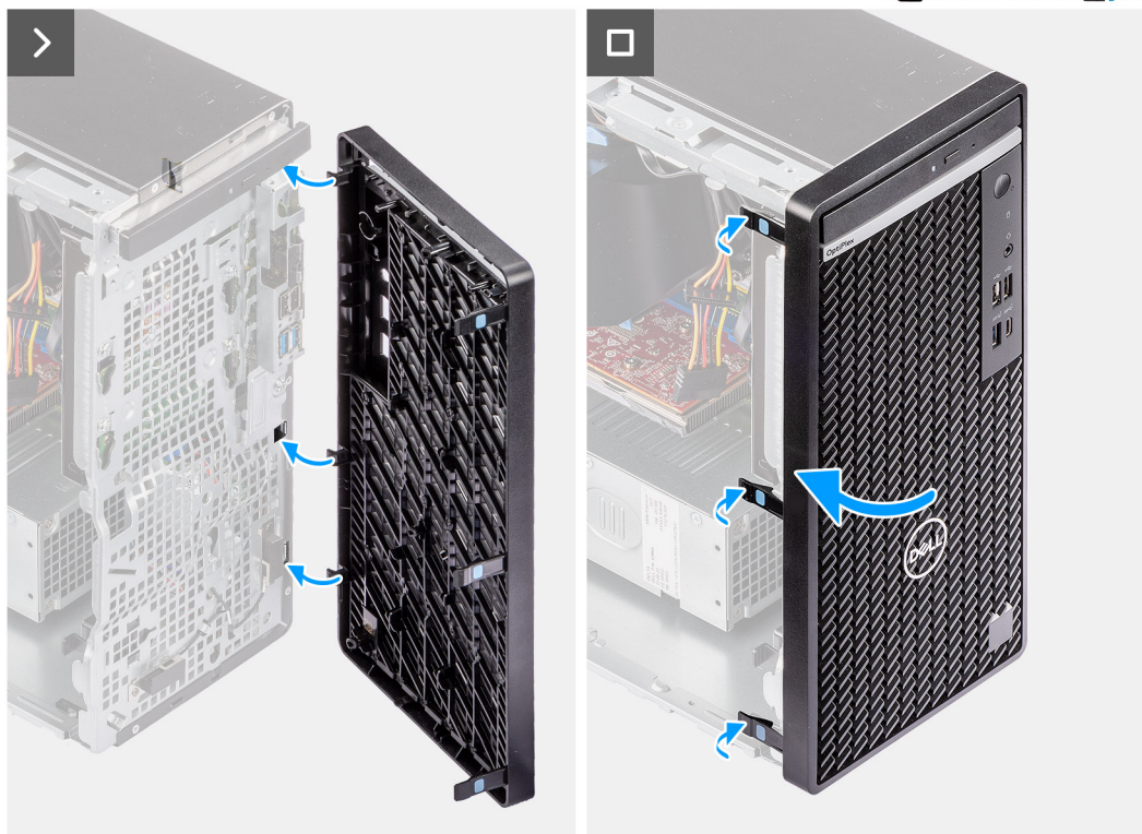
Obrázek 16. Montáž čelního krytu
