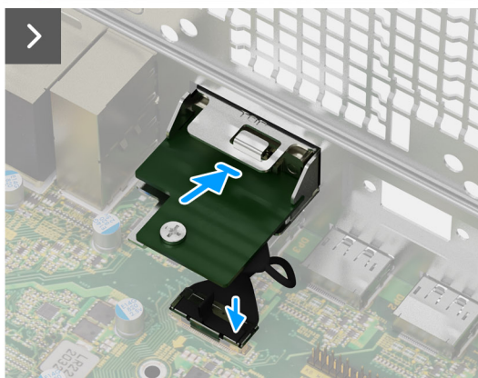
Obrázek 81. Montáž volitelného modulu VGA
