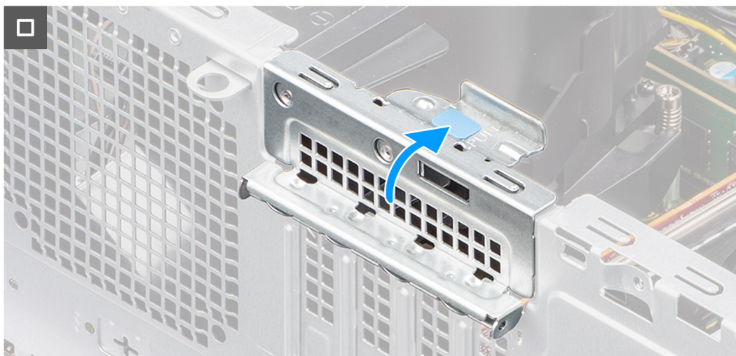
Obrázek 73. Demontáž volitelného modulu PS2 a sériového modulu
