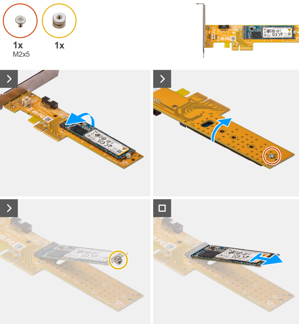
Obrázek 27. Demontáž karty Dell Ultra Speed 3. generace s diskem M.2 2280
