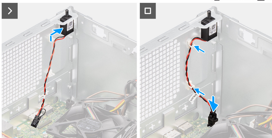
Obrázek 48. Montáž spínače detekce vniknutí do šasi
