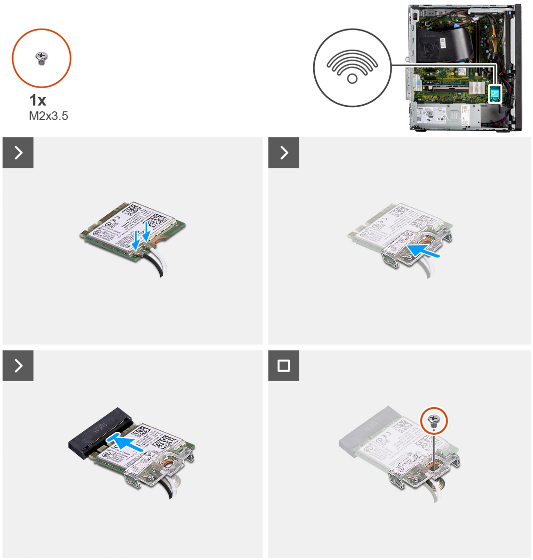
Obrázek 32. Montáž bezdrátové karty
