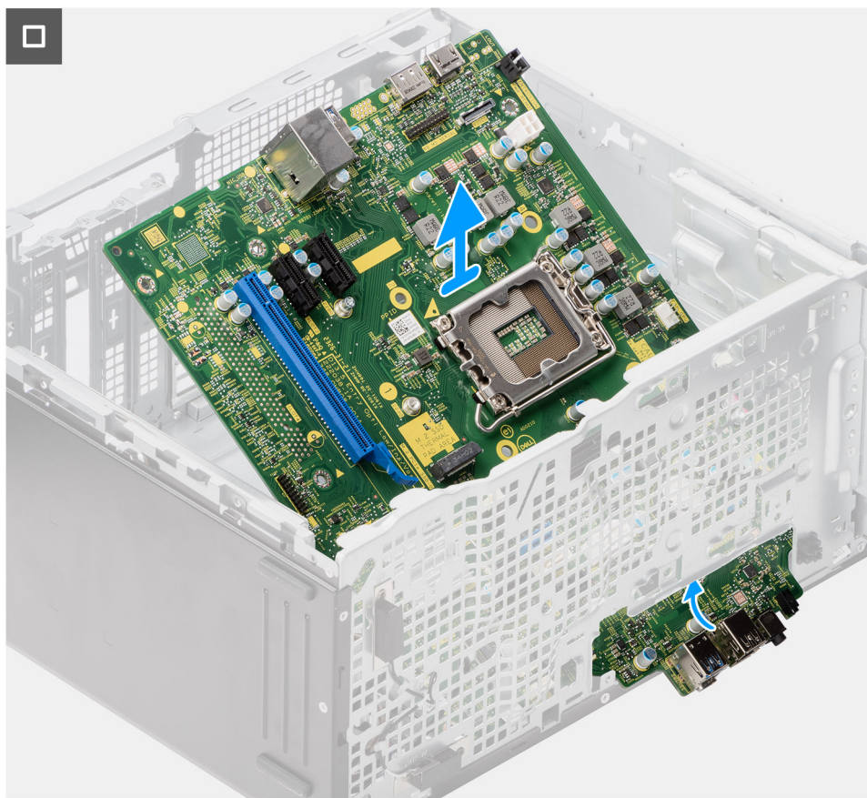
Obrázek 86. Demontáž základní desky
