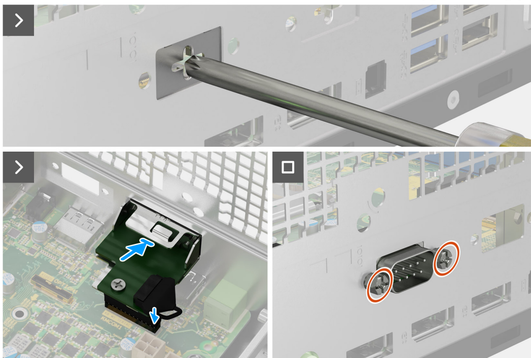
Obrázek 71. Montáž volitelného modulu sériového rozhraní
