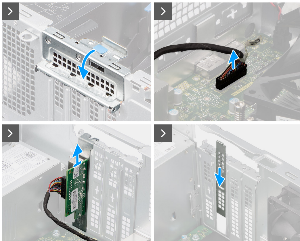
Obrázek 72. Demontáž volitelného modulu PS2 a sériového modulu
