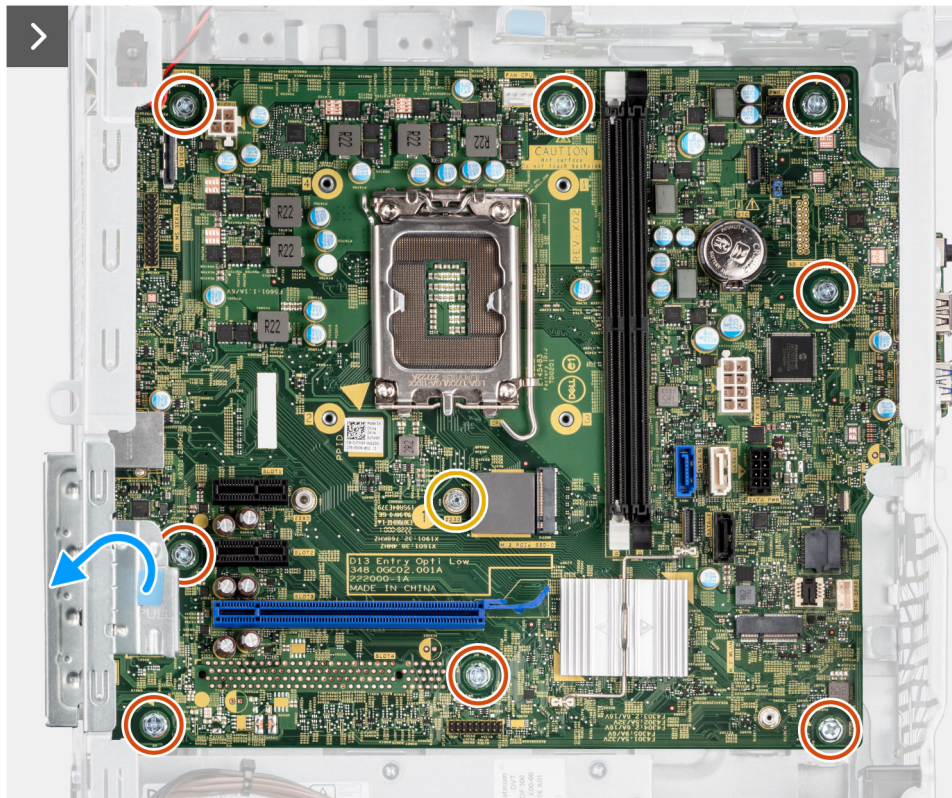
Obrázek 85. Demontáž základní desky
