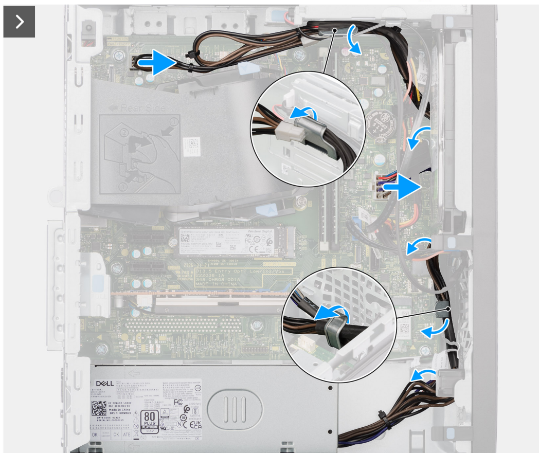
Obrázek 64. Demontáž napájecí jednotky
