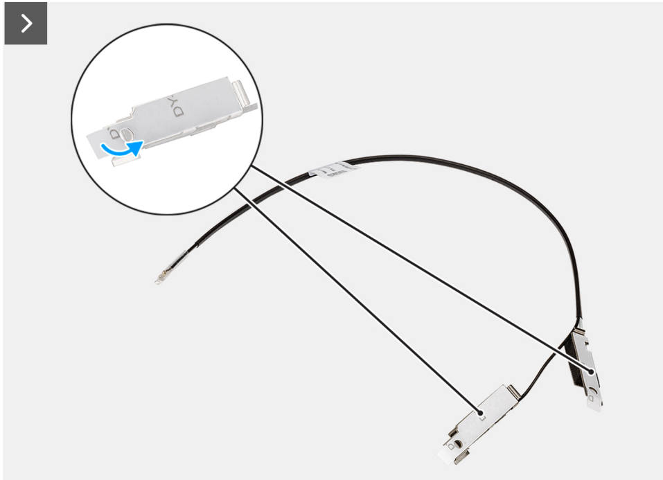
Obrázek 54. Montáž modulu interní antény
