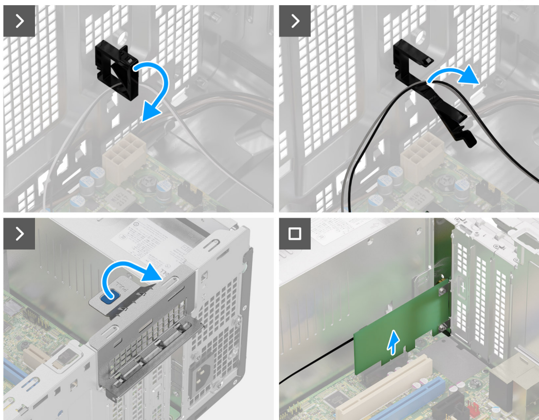
Obrázek 56. Demontáž modulu externí antény SMA
