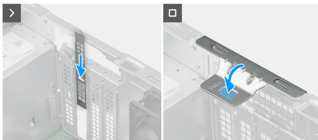
Obrázek 44. Demontáž karty sériového/paralelního portu
