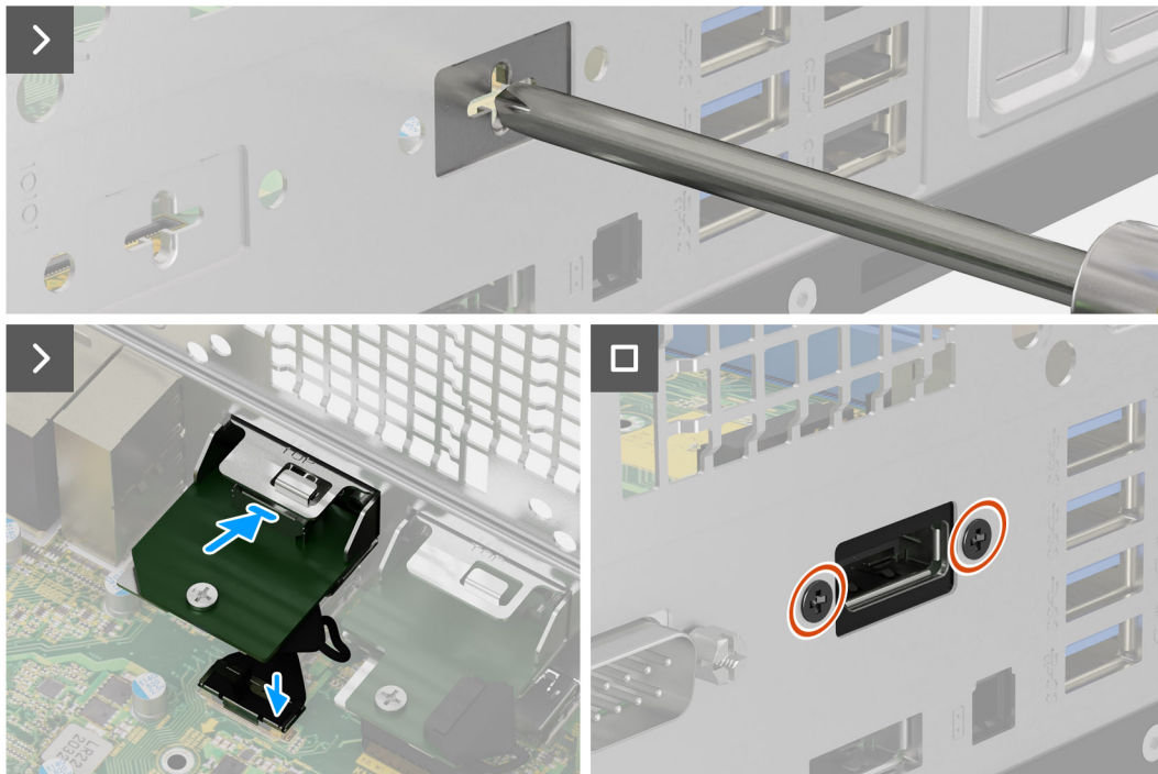
Obrázek 79. Instalace volitelného modulu DisplayPort
