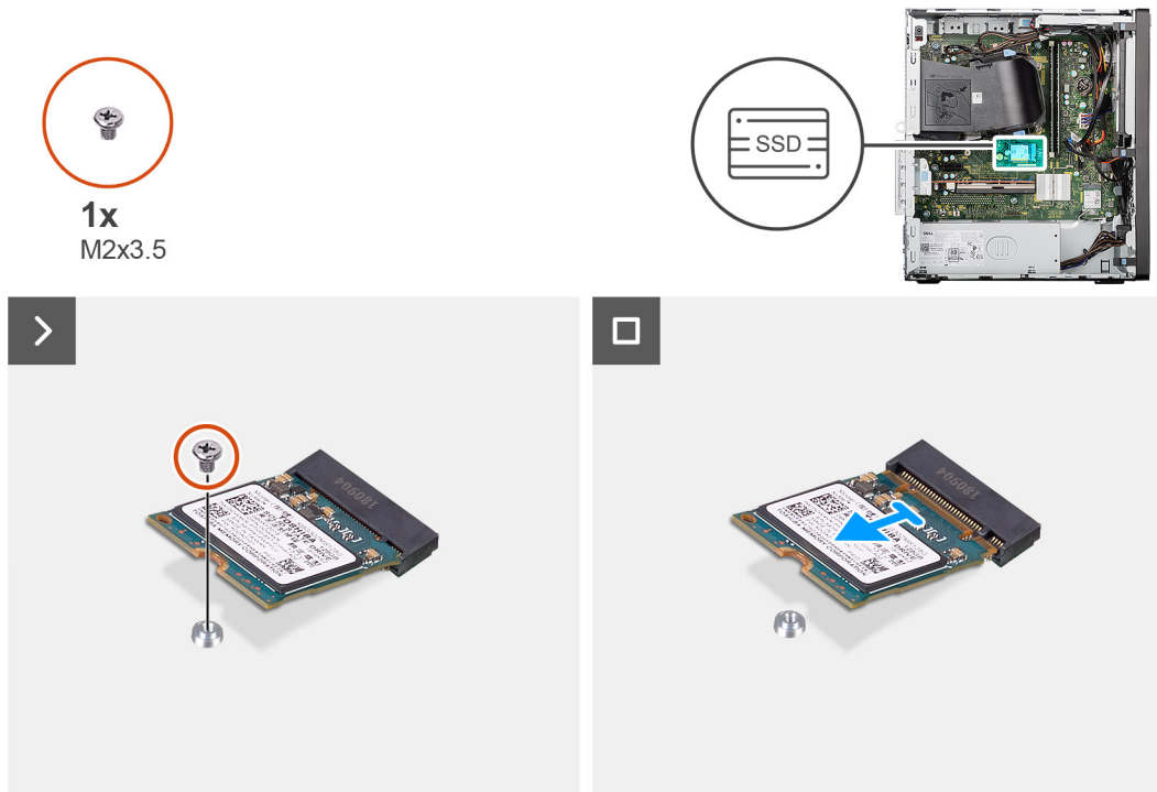
Obrázek 19. Demontáž disku SSD M.2 2230
