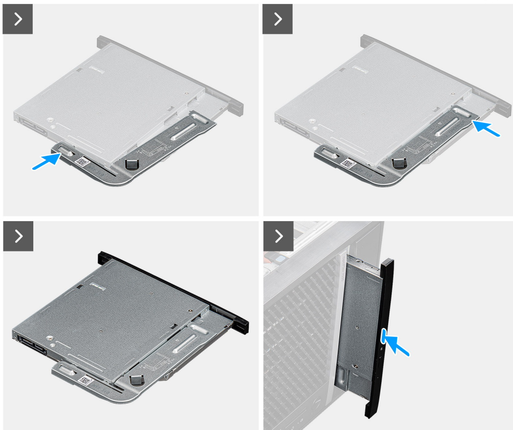
Obrázek 39. Montáž tenké optické jednotky
