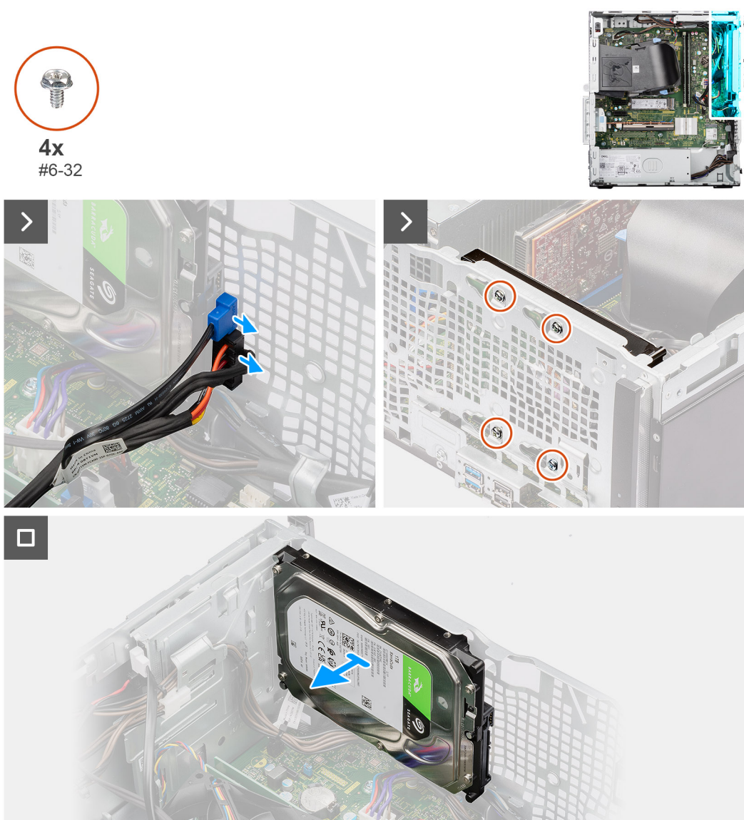
Obrázek 35. Vyjmutí 3,5palcového pevného disku
