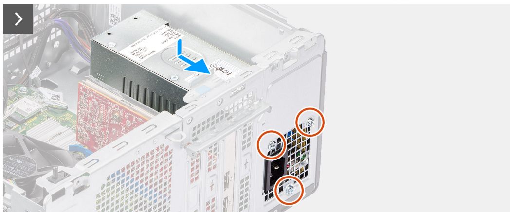
Obrázek 66. Montáž napájecí jednotky
