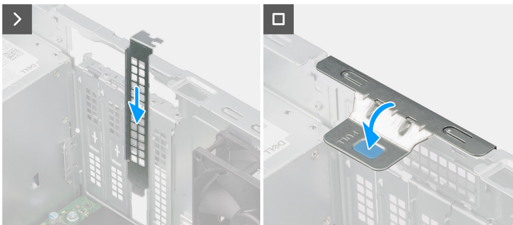
Obrázek 57. Demontáž modulu externí antény SMA
