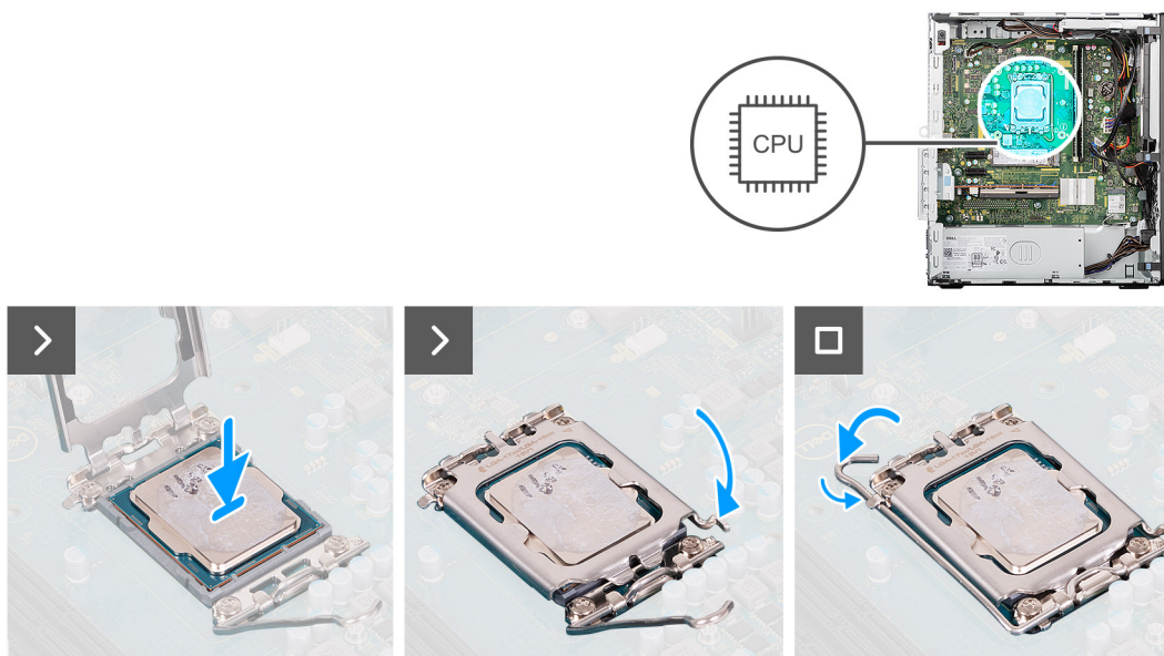
Obrázek 69. Montáž procesoru
