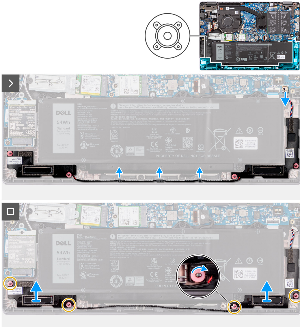
Figura21. Retirar os altifalantes
