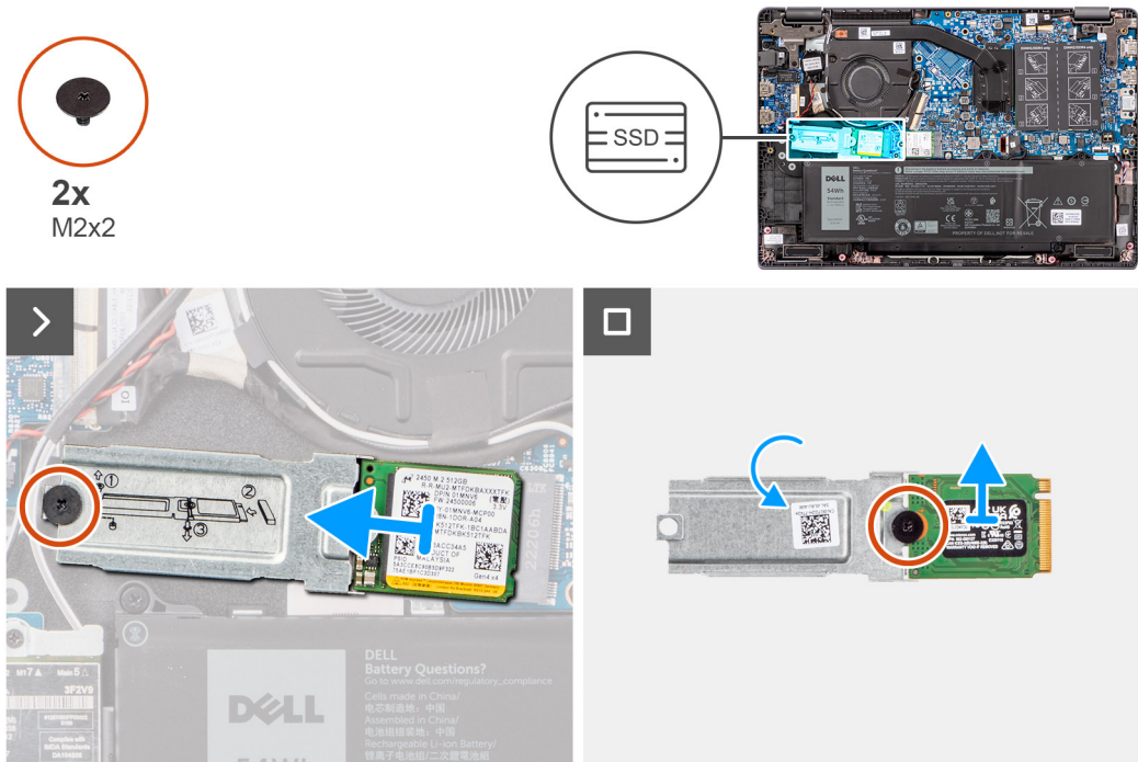
Figura19. Retirar o disco de estado sólido M.2 2230
