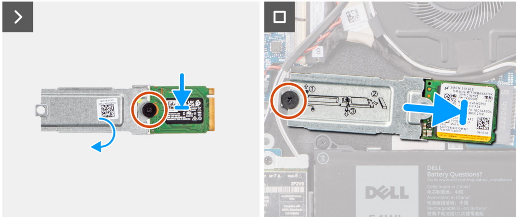
Figura20. Instalar o disco de estado sólido M.2 2230
