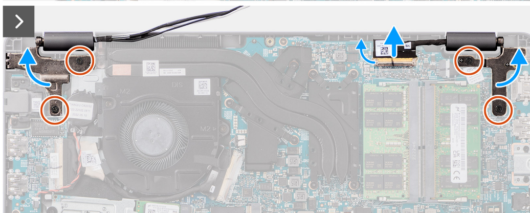
Figura47. Retirar o conjunto do ecrã
