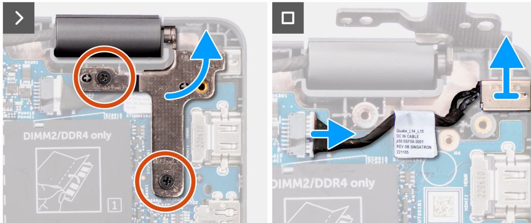
Figura27. Retirar a porta do transformador
