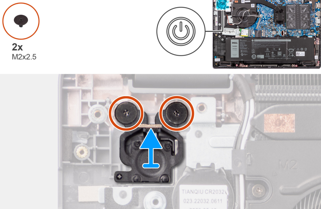
Figura39. Retirar o botão de alimentação
