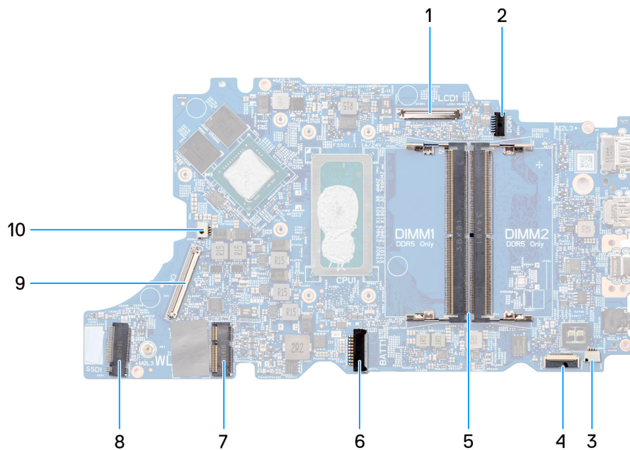
Figura41. Conectores da placa de sistema
