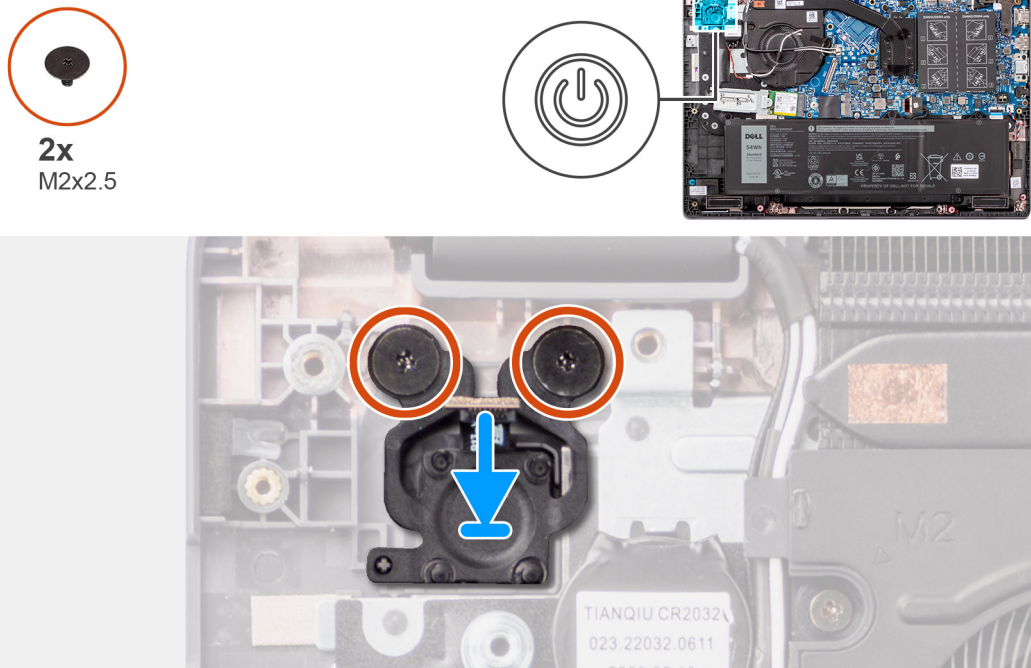
Figura40. Instalar o botão de alimentação
