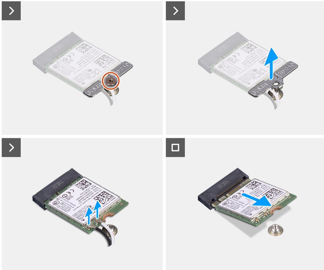
Figura15. Retirar a placa de comunicação sem fios
