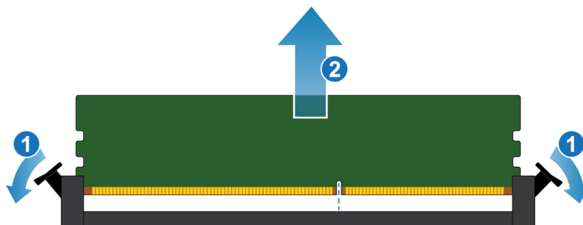
Ilustración 130. Extracción del DIMM
