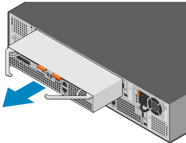
Ilustración 128. Extracción del Módulo de acceso
