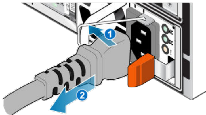
Ilustración 49. Extracción del cable de alimentación
