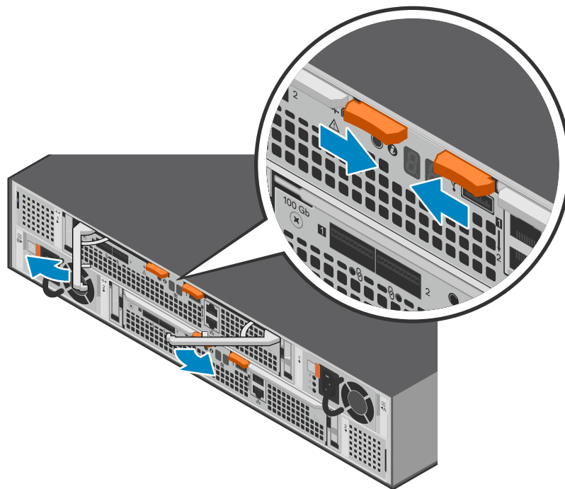
Ilustración 127. Liberación del Módulo de acceso
