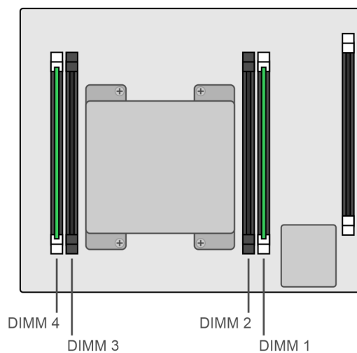
Ilustración 129. Vista superior del Módulo de acceso
