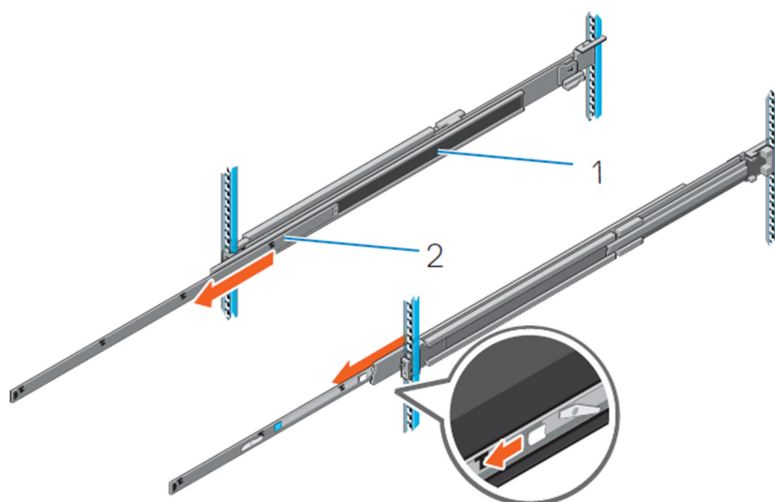
Ilustración 10. Tire de la guía intermedia
