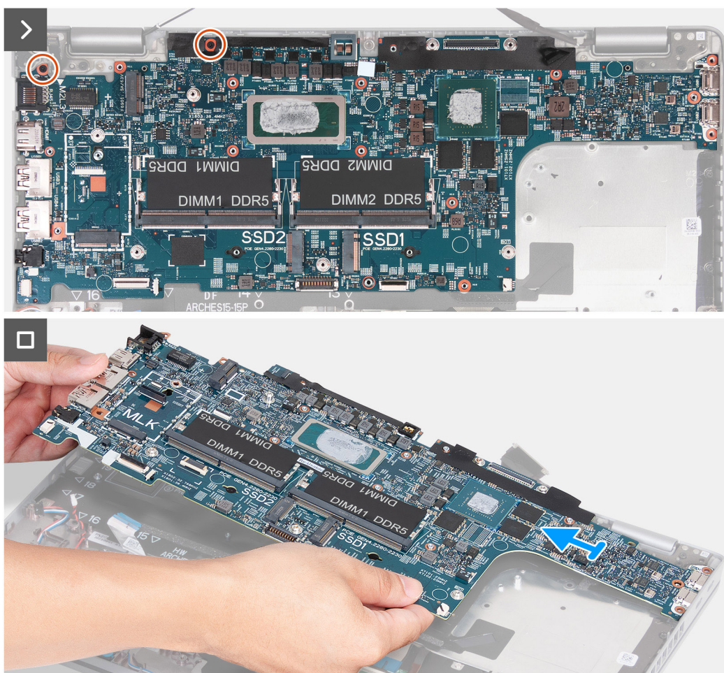
Figura 59. Rimozione della scheda di sistema
