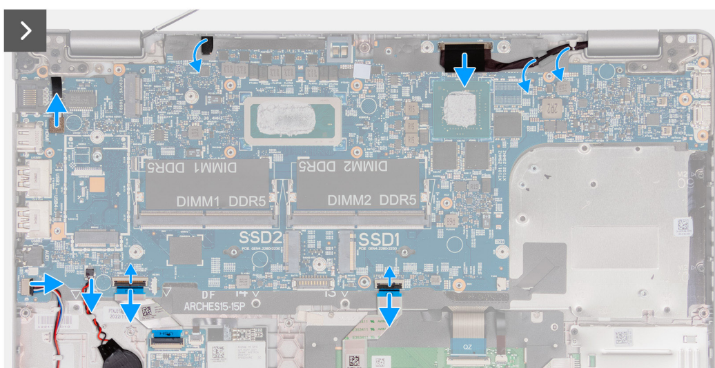
Figura 58. Rimozione della scheda di sistema
