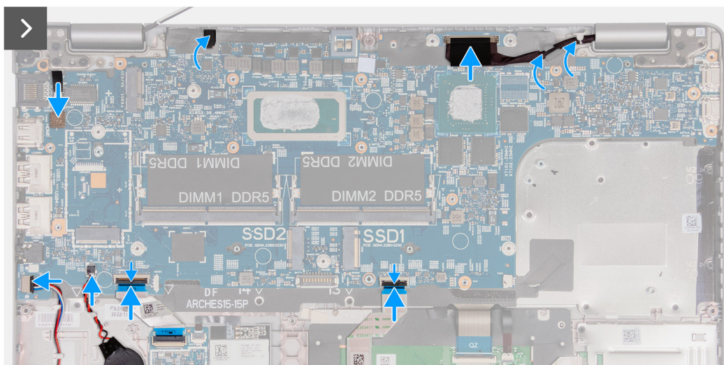
Figura 63. Installazione della scheda di sistema
