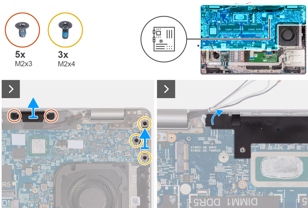
Figura 53. Rimozione delle viti
