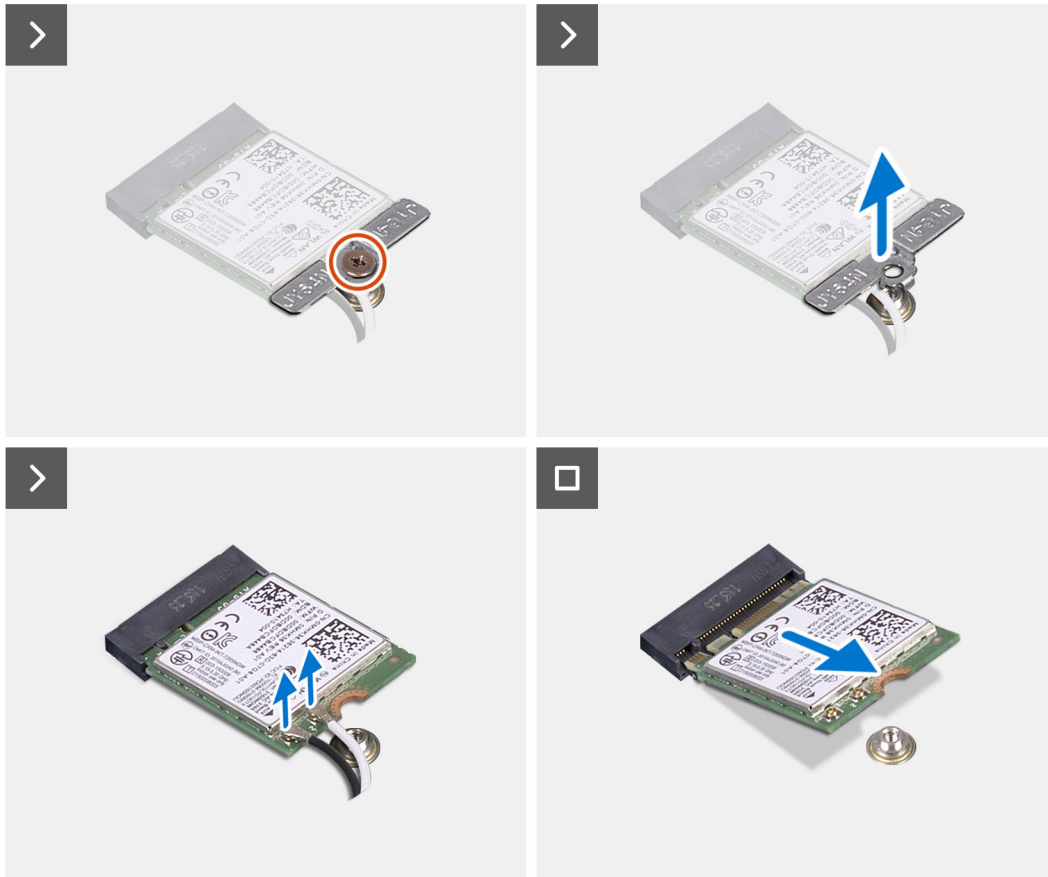
Figura 19. Rimozione della scheda wireless
