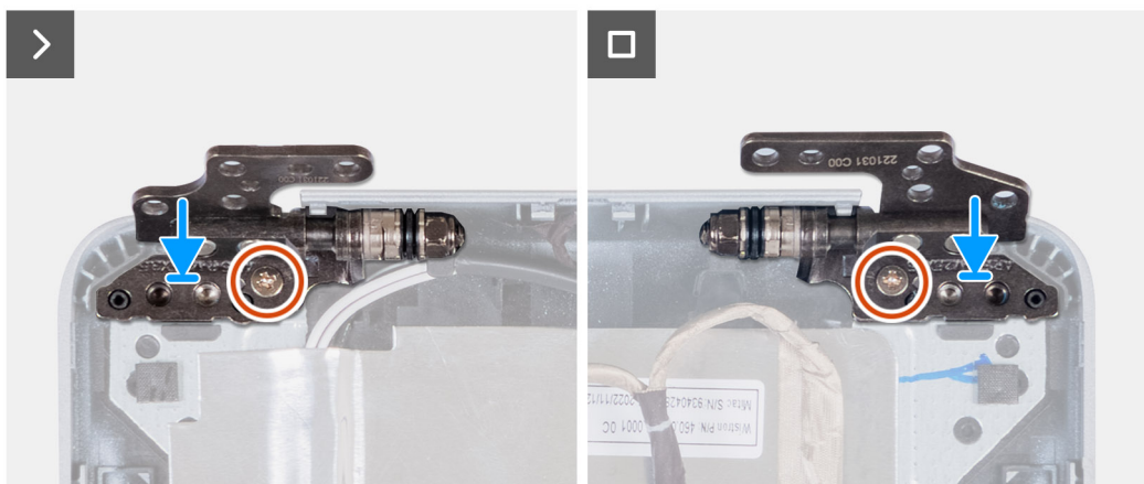
Figura 87. Installazione delle cerniere del display
