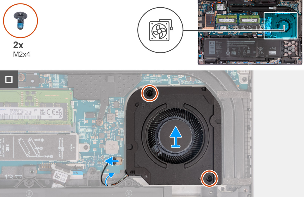
Figura 33. Rimozione della ventola
