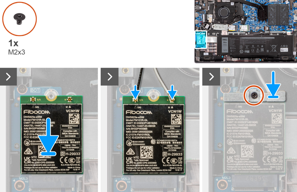
Figure 17. Installation de la carte WWAN
