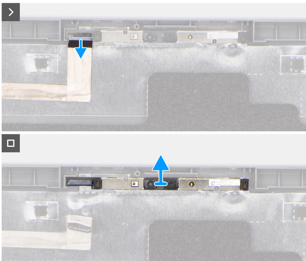
Figure 66. Retrait de la caméra
