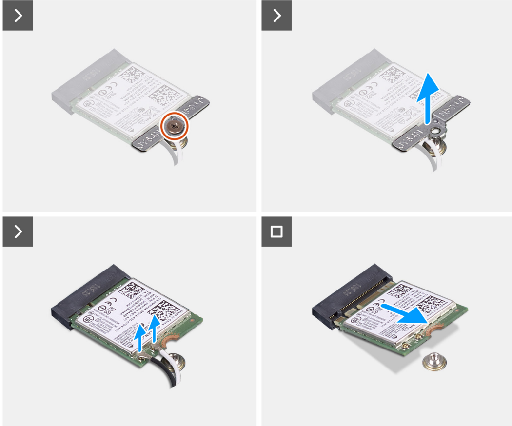
Figure 14. Retrait de la carte sans fil
