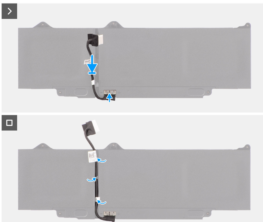
Figure 26. Installation du câble de la batterie
