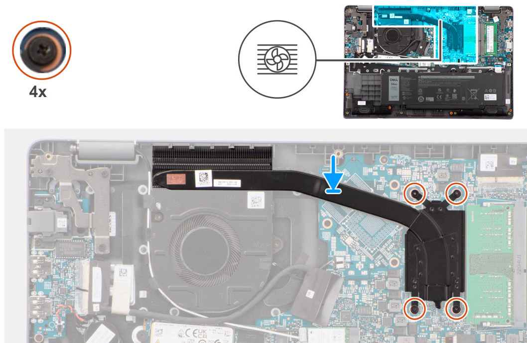
Figure 30. Installation du dissipateur de chaleur pour carte graphique intégrée
