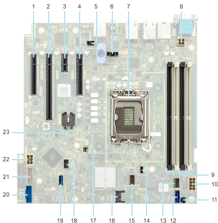
Figure 101. Disposition de la carte système
