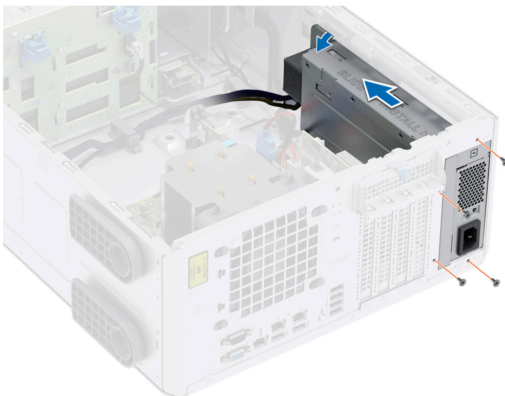
Figure 80. Retrait du bâti du bloc d'alimentation
