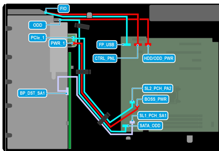
Figure 47. Acheminement des câbles : système à 4 disques de 3,5 pouces
