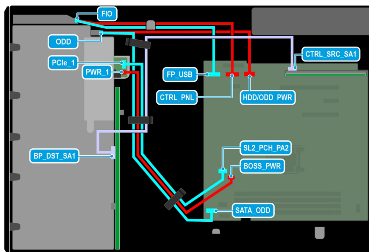
Figure 46. Système à 8 disques de 3,5 pouces
