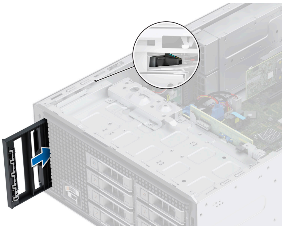
Figure 35. Installation du cache de lecteur optique dans le bâti du lecteur optique
