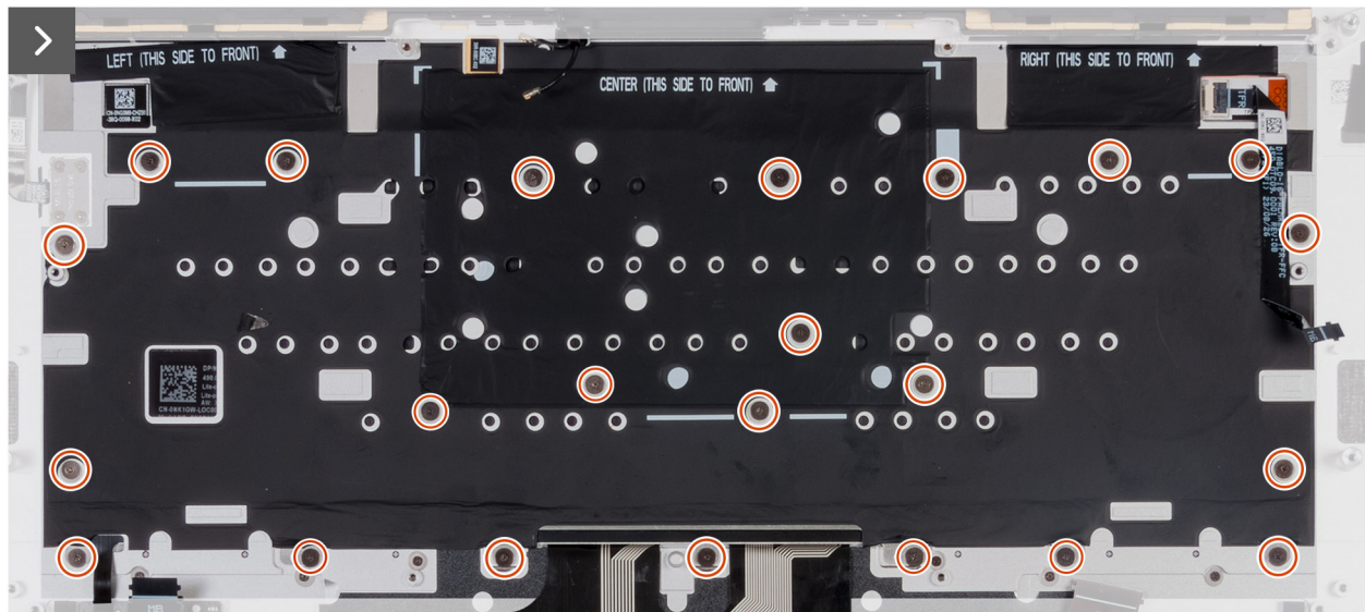
Ilustración 60. Instalación del teclado
