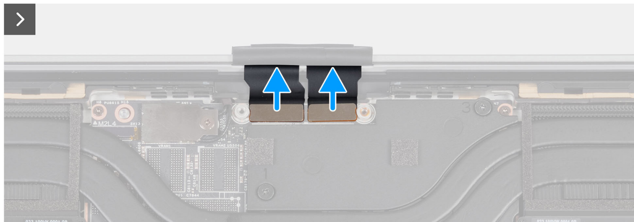
Ilustración 47. Extracción de la tarjeta madre
