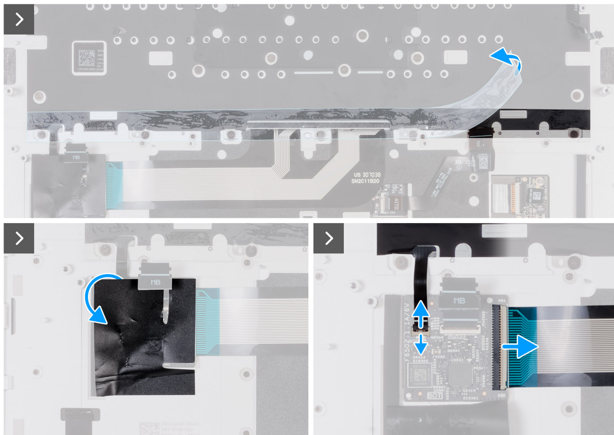
Ilustración 56. Extracción del teclado
