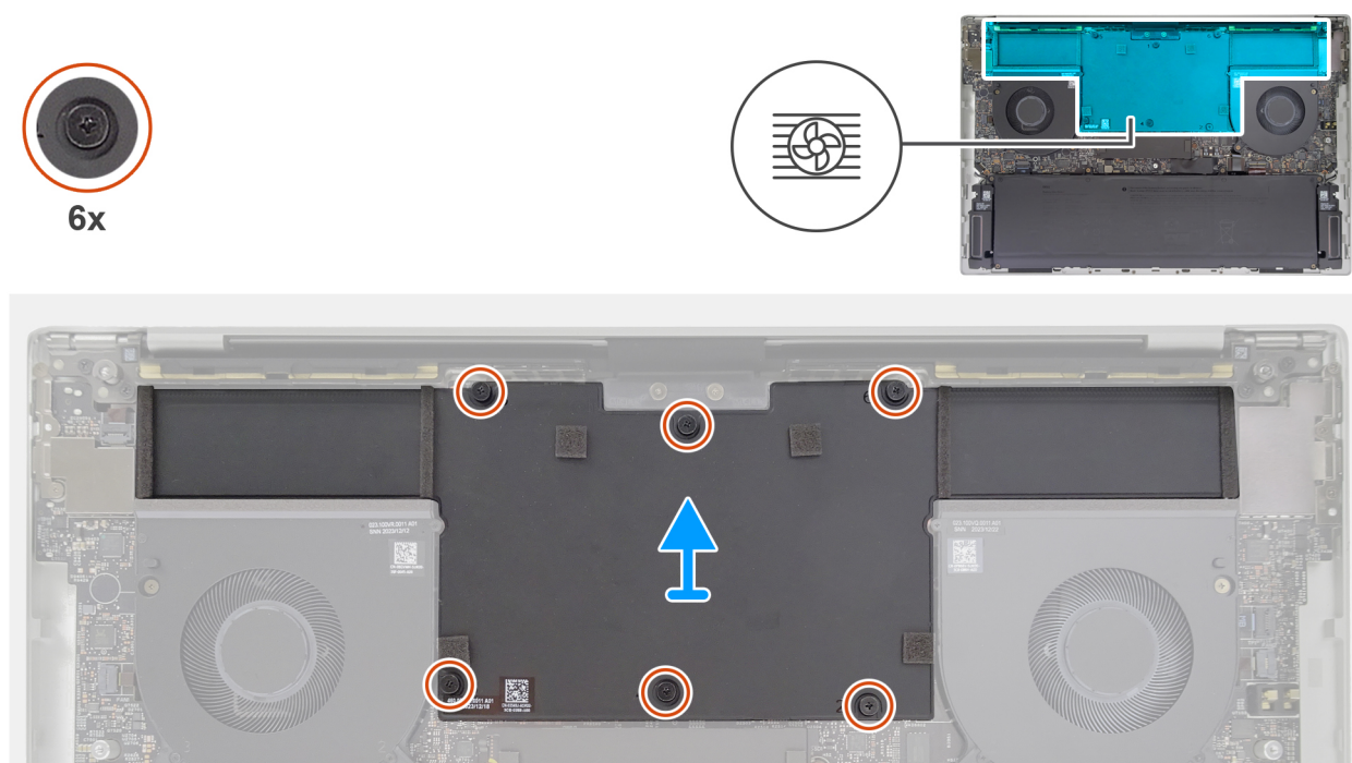
Ilustración 34. Extracción del disipador de calor: GPU discreta (cámara de vapor)
