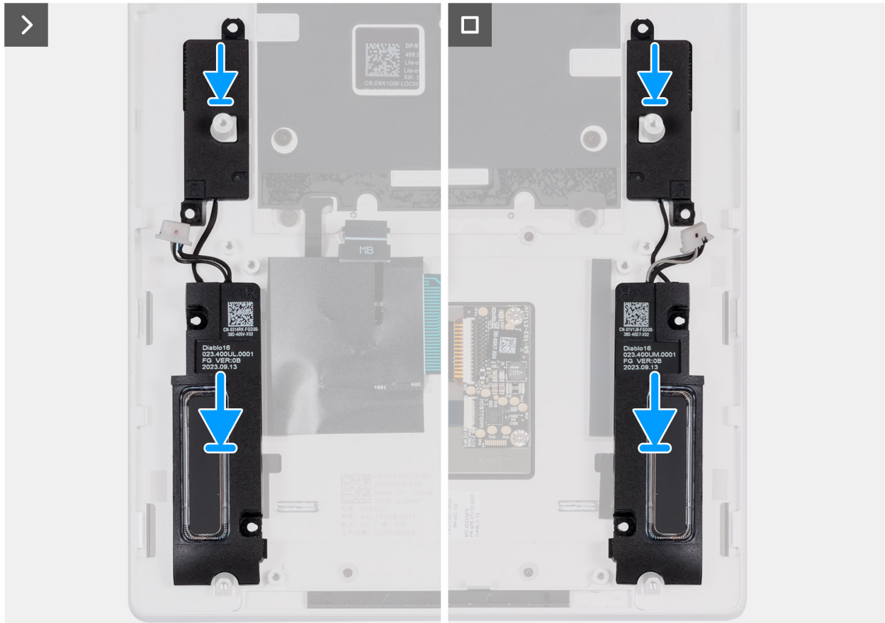
Ilustración 55. Instalación de los parlantes
