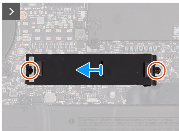
Ilustración 28. Extracción de la unidad de estado sólido M.2 2280
