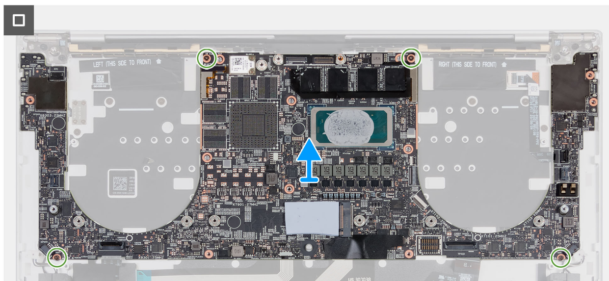
Ilustración 49. Extracción de la tarjeta madre
