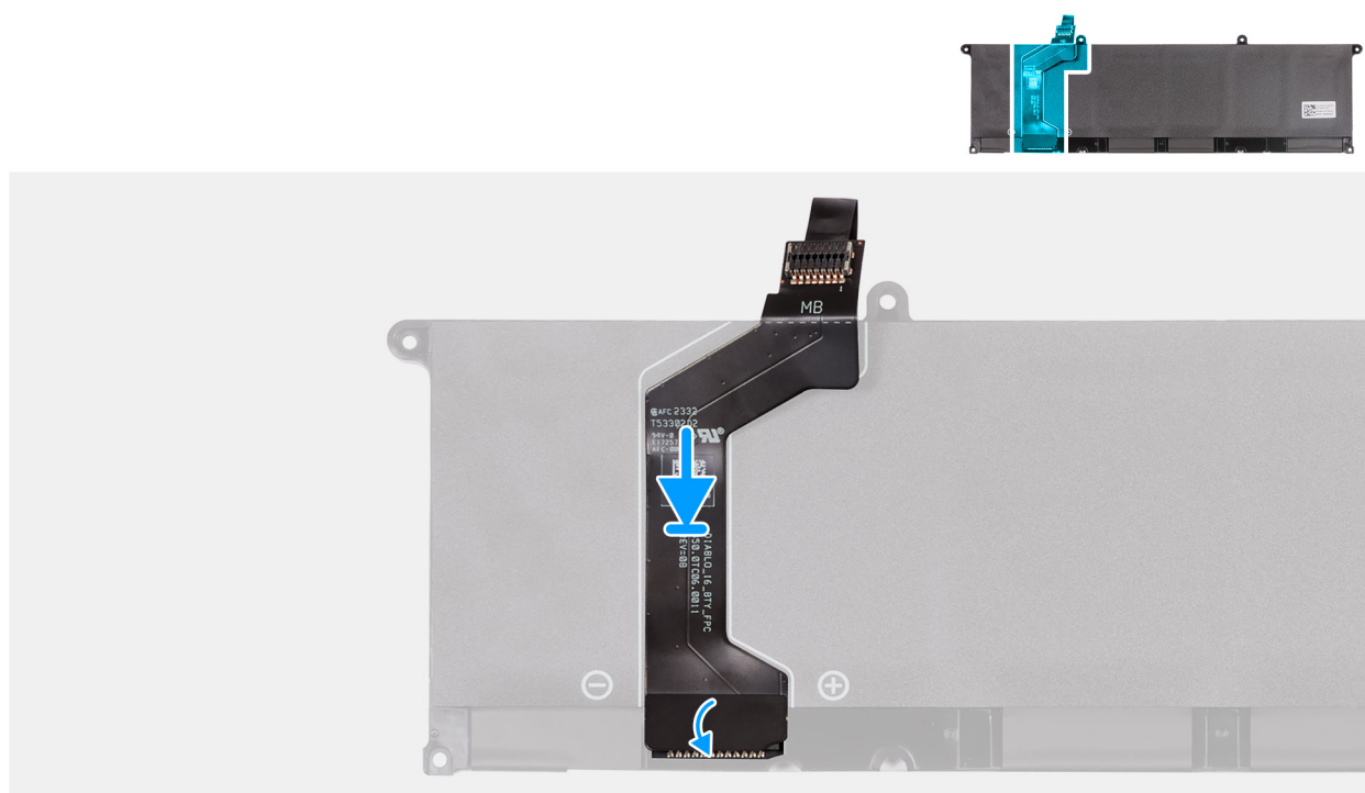
Ilustración 22. Instalación del cable de la batería
