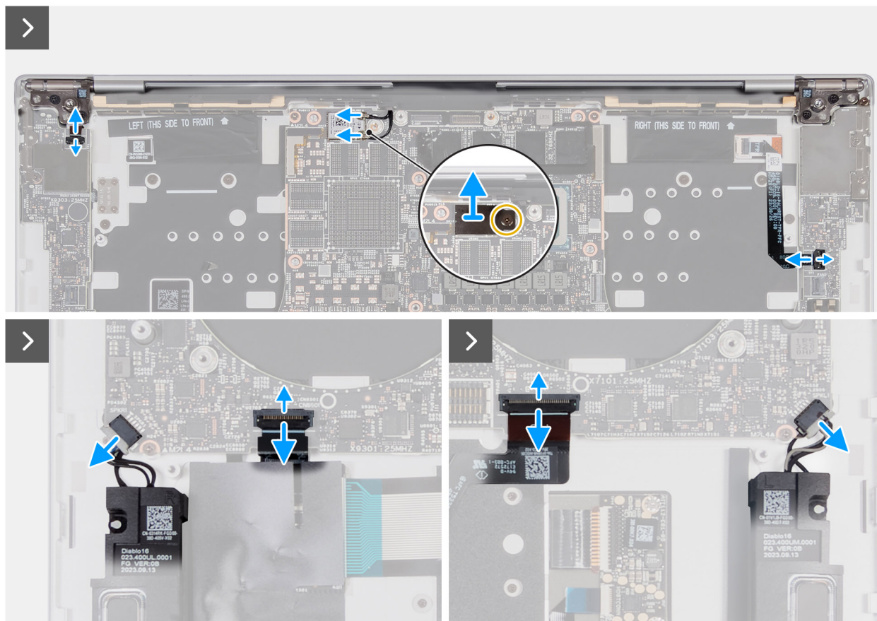
Ilustración 48. Extracción de la tarjeta madre
