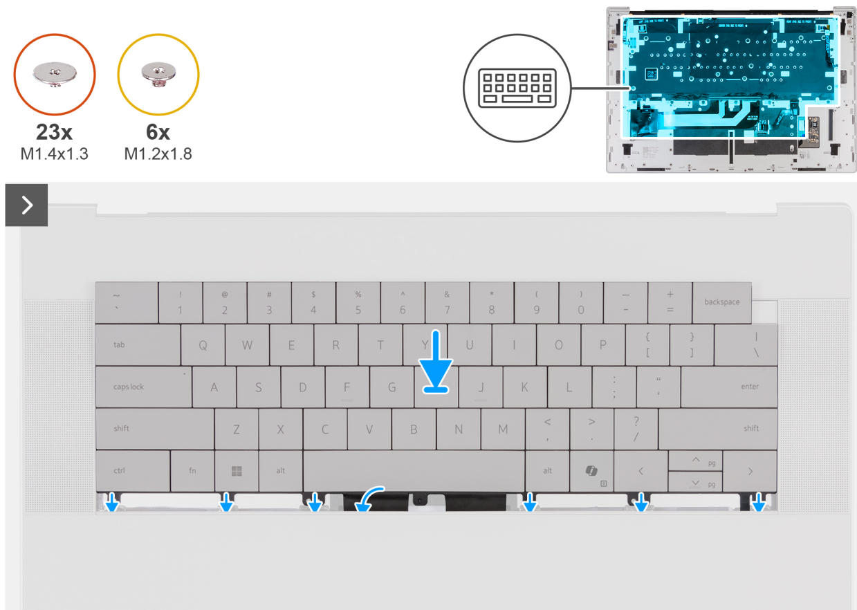
Ilustración 59. Instalación del teclado
