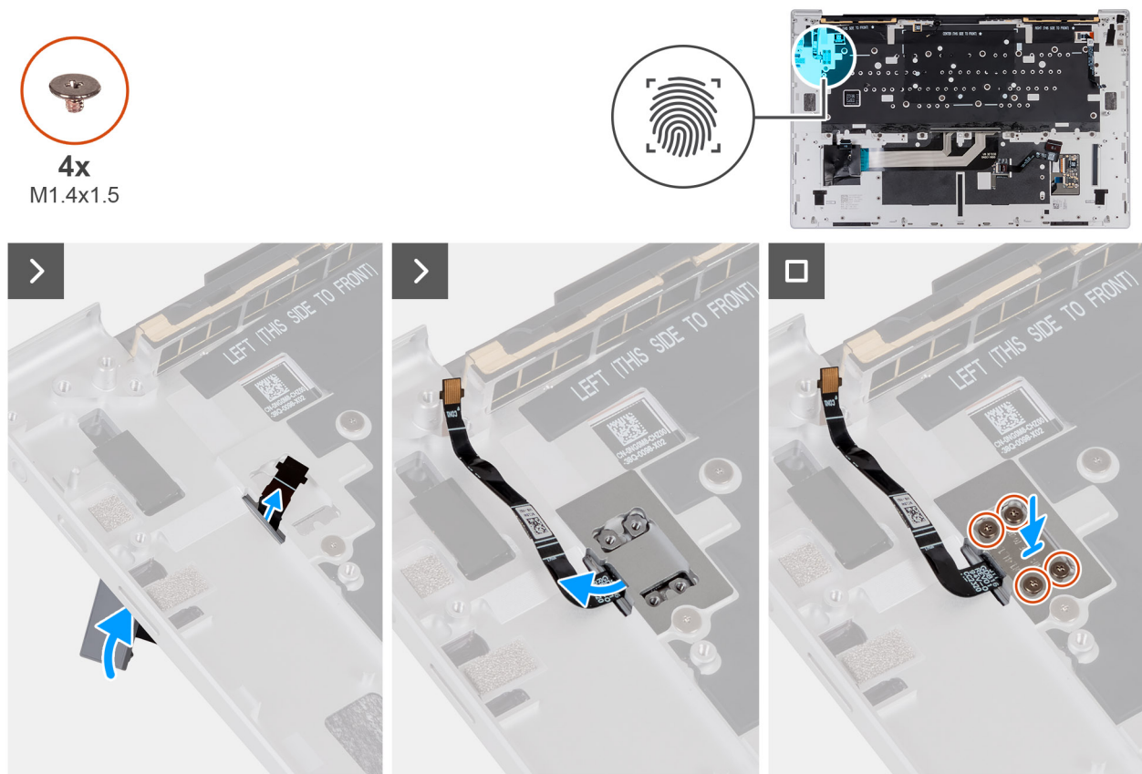
Ilustración 63. Instalación del botón de encendido con lector de huellas digitales
