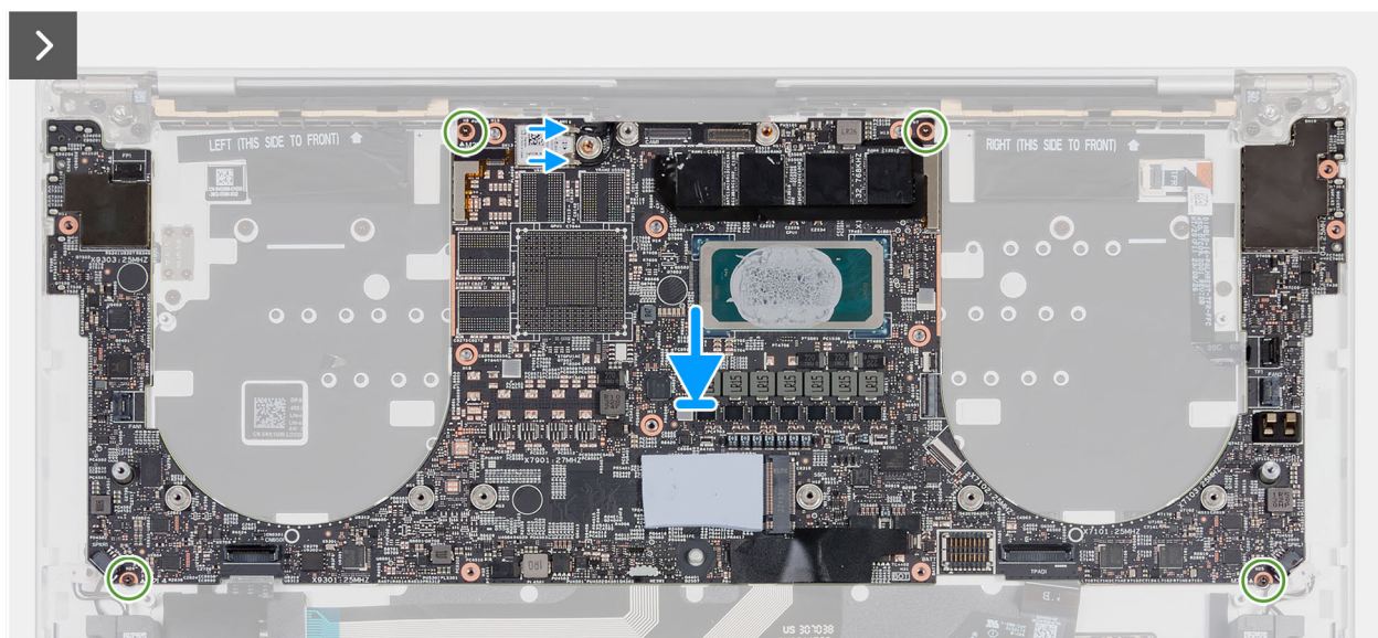
Ilustración 51. Instalación de la tarjeta madre
