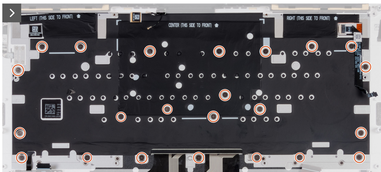
Ilustración 57. Extracción del teclado
