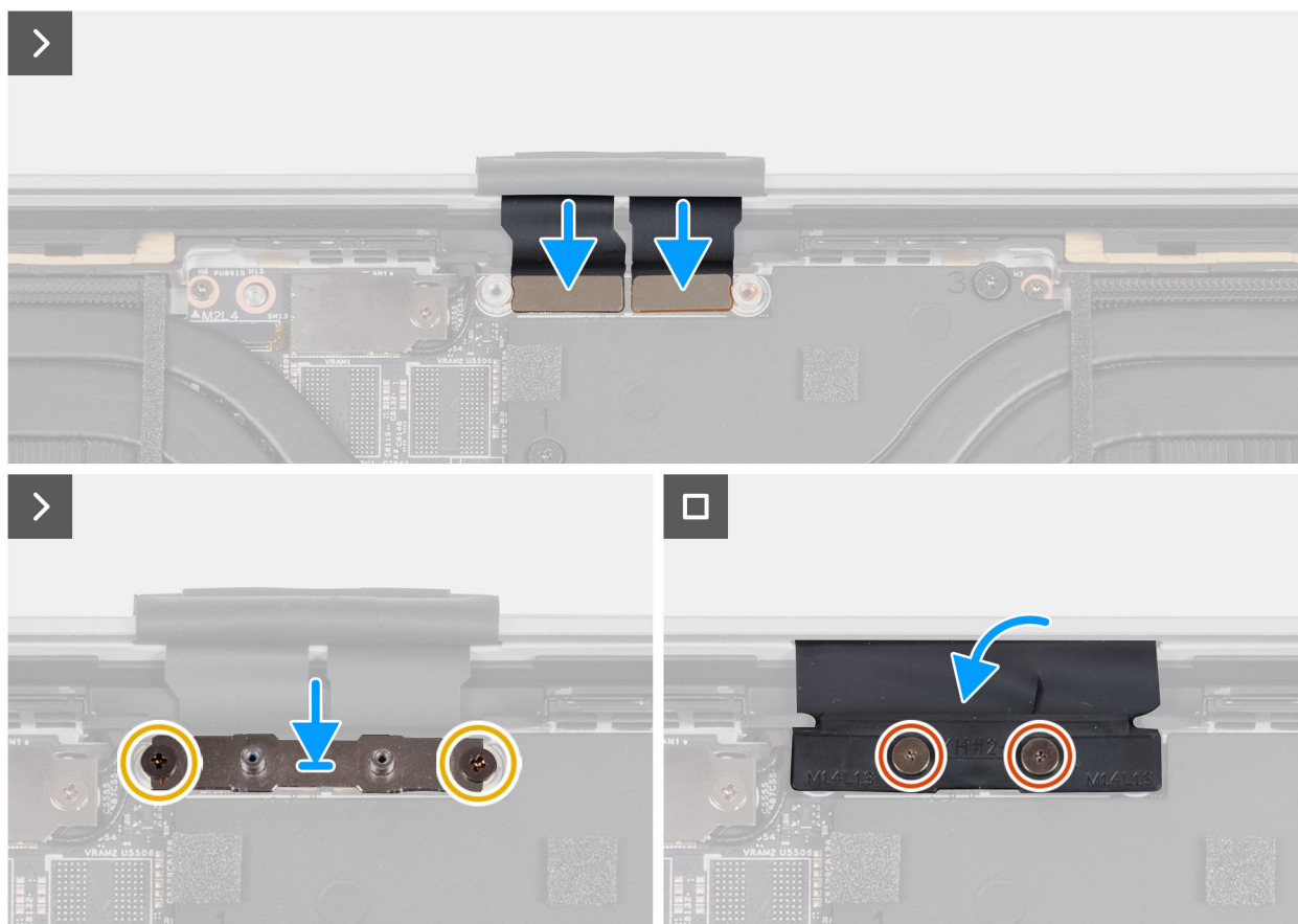
Ilustración 53. Instalación de la tarjeta madre
