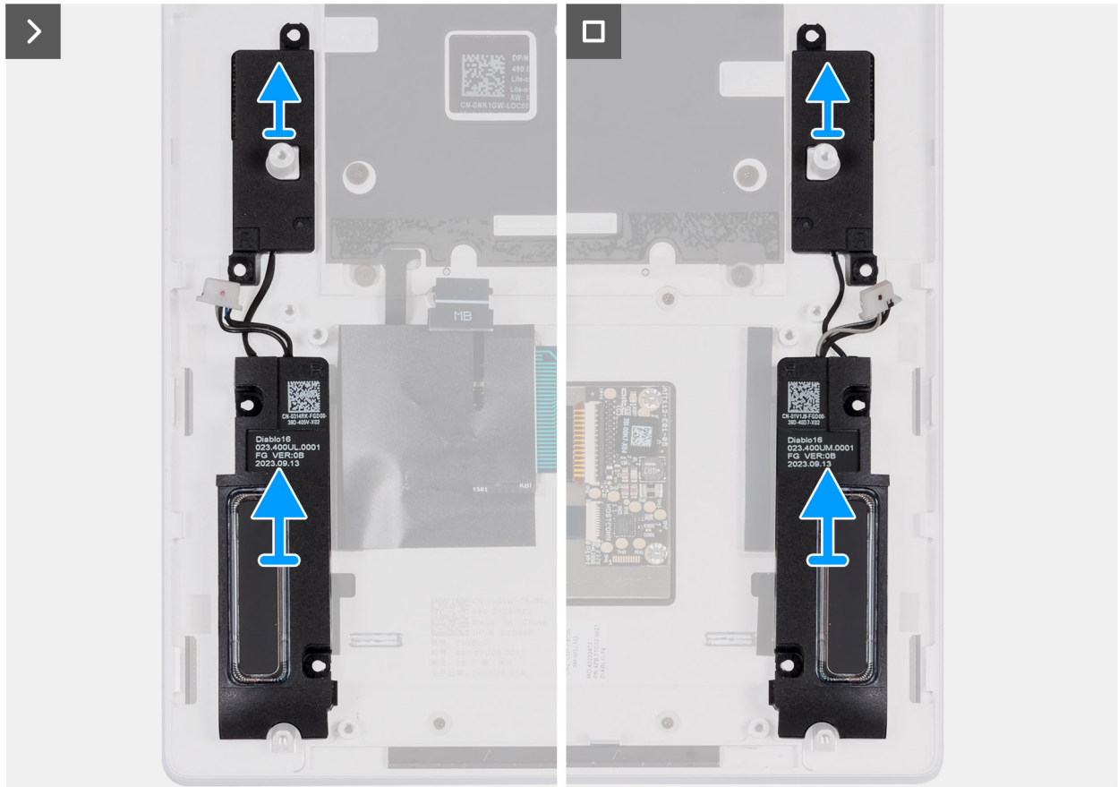
Ilustración 54. Extracción de los parlantes
