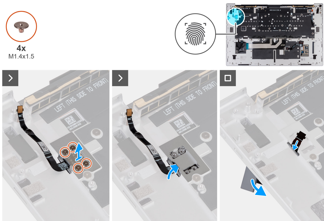
Ilustración 62. Extracción del botón de encendido con lector de huellas digitales
