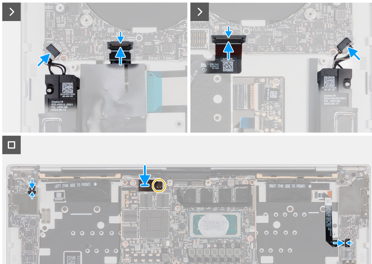
Ilustración 52. Instalación de la tarjeta madre
