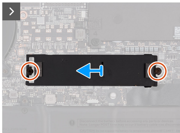
Ilustración 27. Extracción de la unidad de estado sólido M.2 2230
