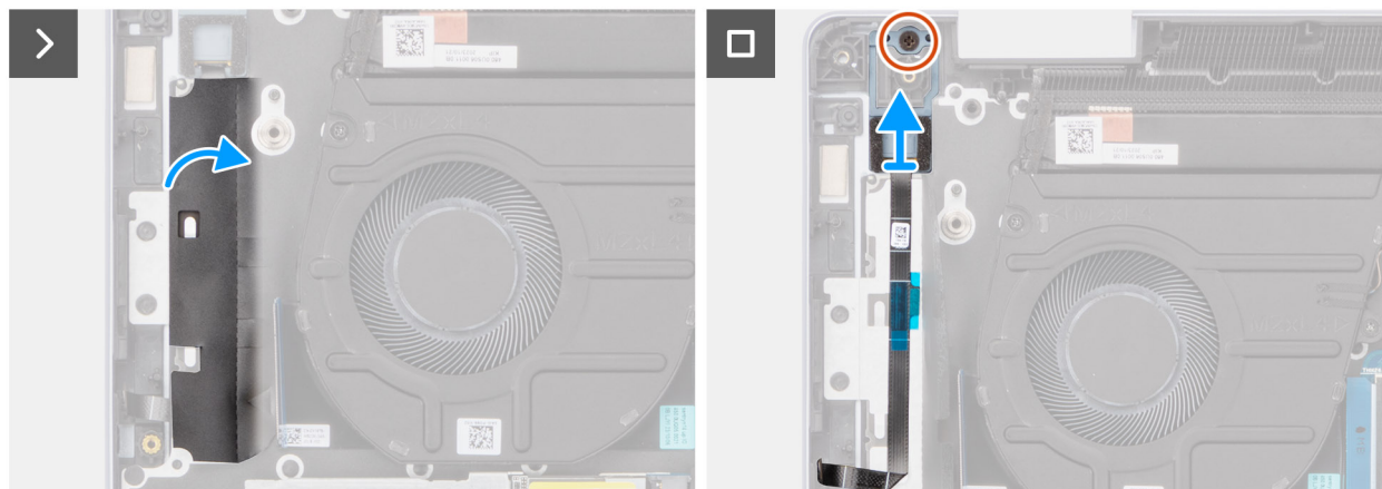
Ilustración 35. Extracción del botón de encendido con lector de huellas digitales
