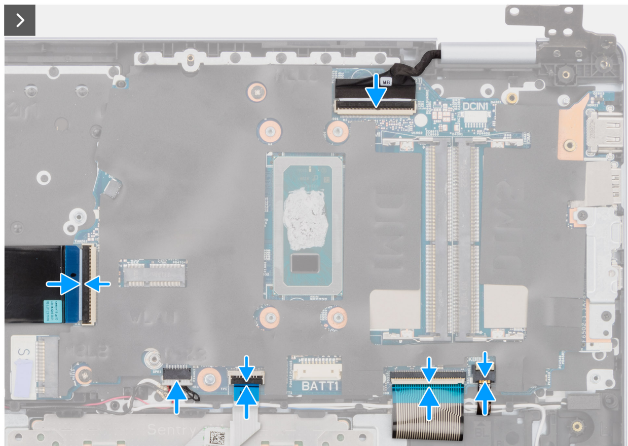
Ilustración 52. Reemplazo de los conectores del cable
