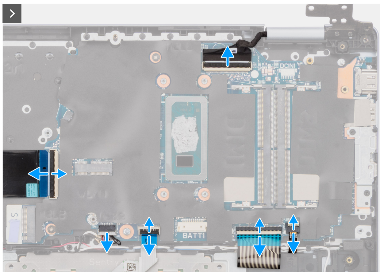
Ilustración 47. Extracción de los conectores del cable
