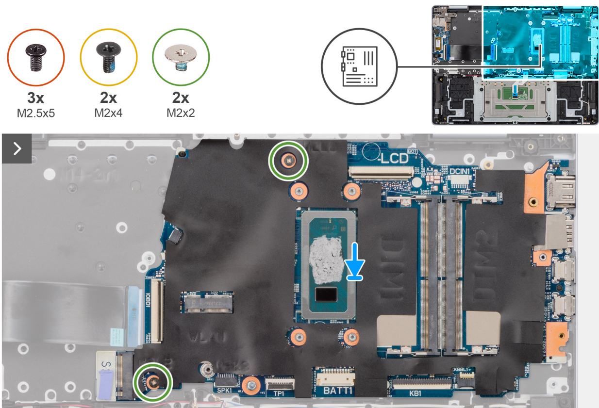
Ilustración 50. Instalación de la tarjeta madre
