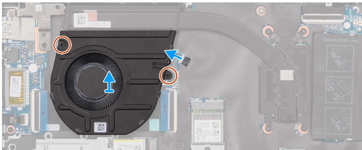
Ilustración 23. Extracción del ventilador
