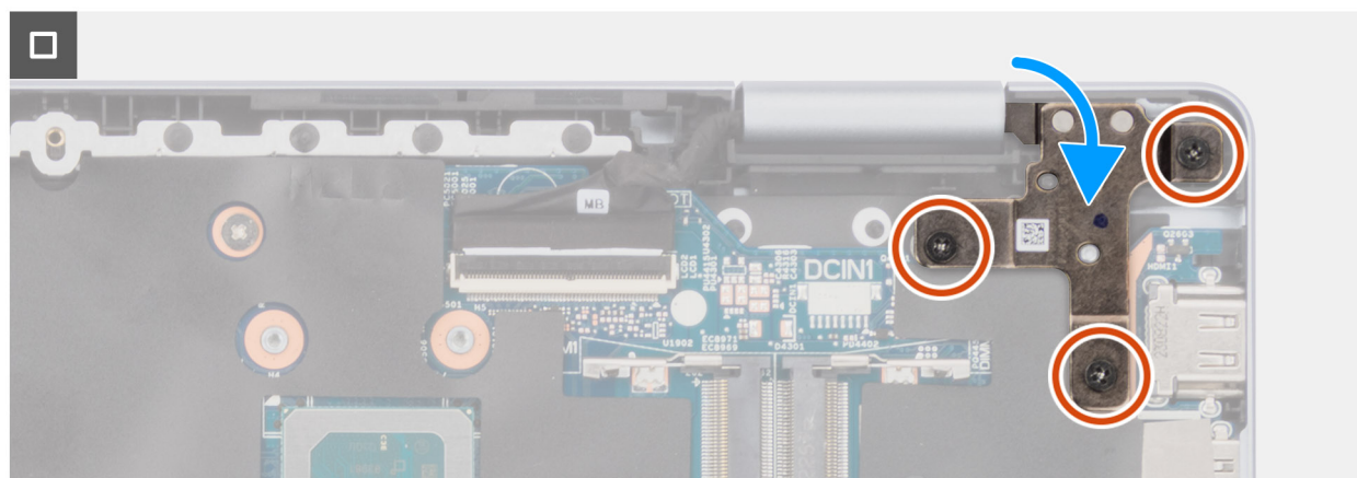
Ilustración 53. Reemplazo de los tornillos de las bisagras
