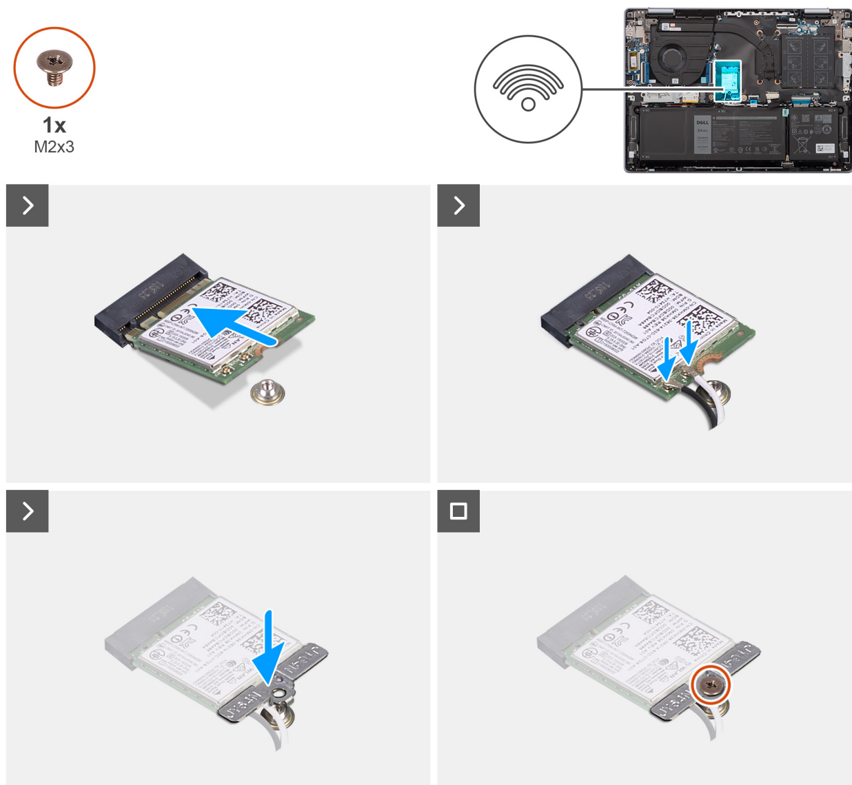
Ilustración 22. Instalación de la tarjeta inalámbrica
