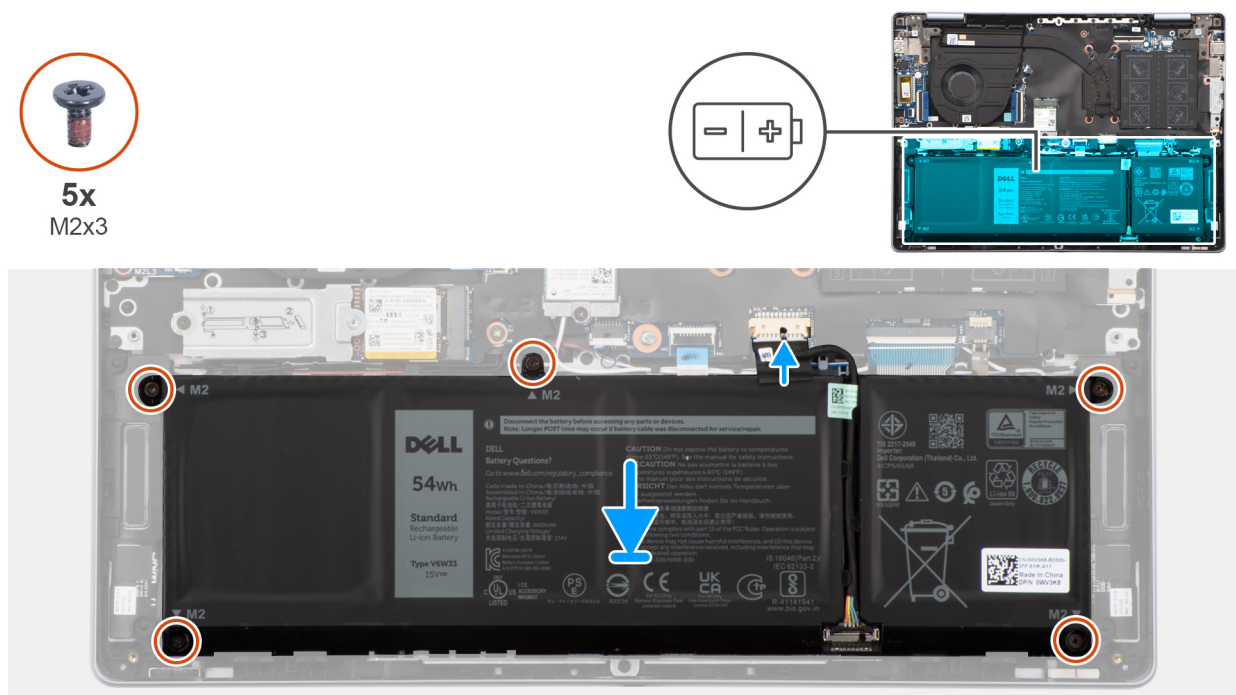
Ilustración 26. Instalación de la batería
