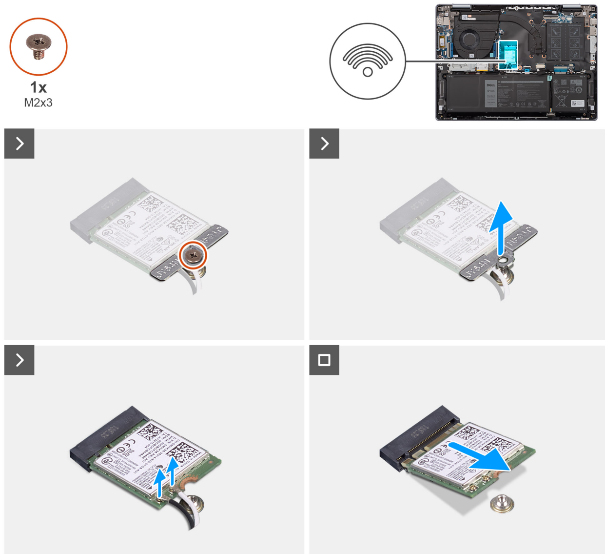
Ilustración 21. Extracción de la tarjeta inalámbrica
