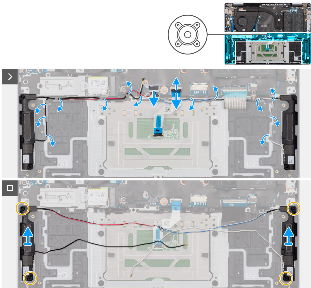
Ilustración 39. Extracción de los parlantes
