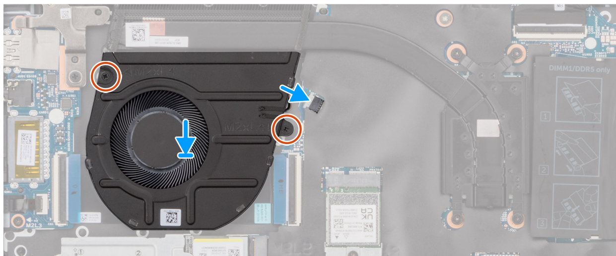
Ilustración 24. Instalación del ventilador
