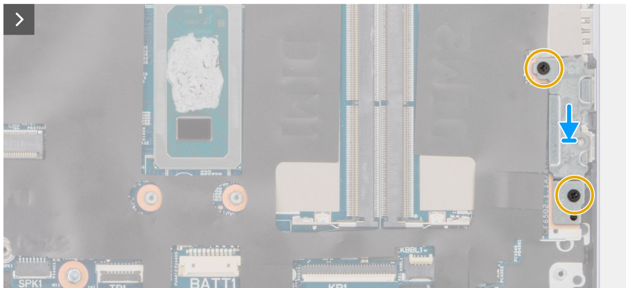
Ilustración 51. Reemplazo del soporte de USB Type C
