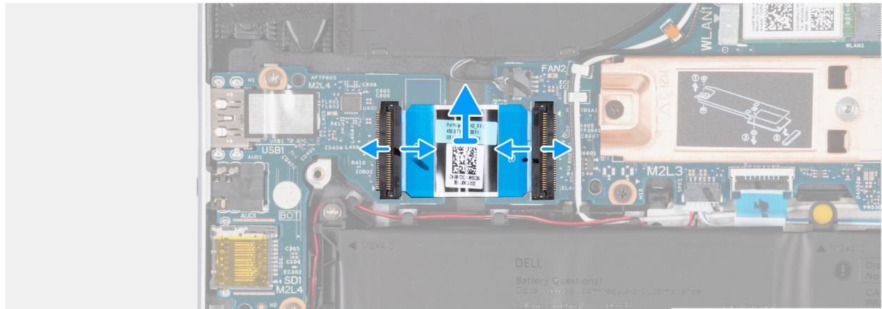
איור 38. הסרת כבל לוח השמע
