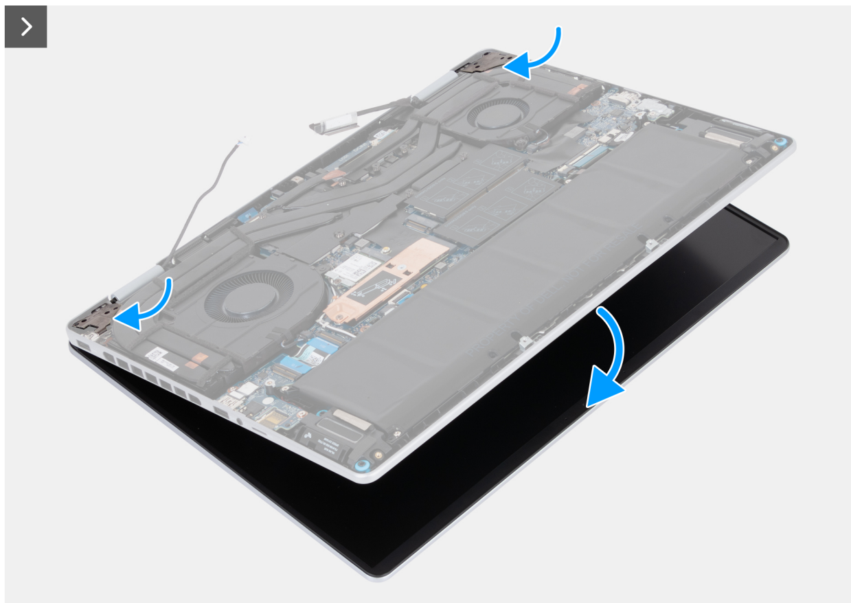
איור 34. התקנת מכלול הצג
