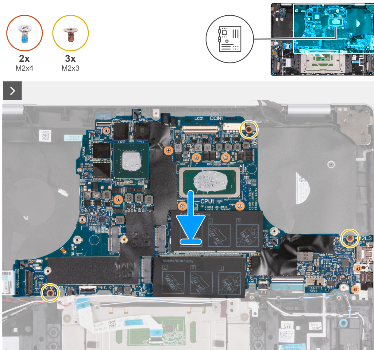
איור 58. התקנת לוח המערכת 1
