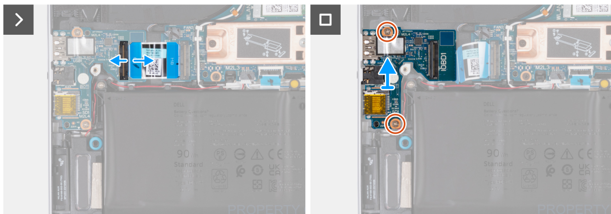
איור 36. הסרת לוח השמע
