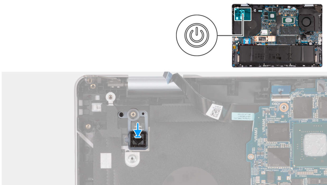
איור 51. התקנת לחצן ההפעלה
