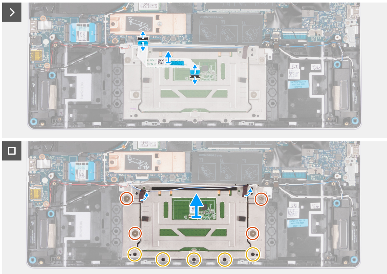
איור 60. הסרת משטח המגע
