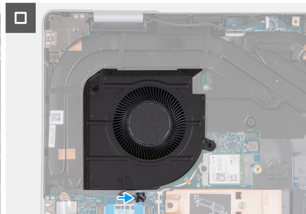
איור 22. התקנת המאוורר של יחידת העיבוד הגרפי
