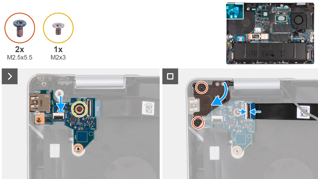
איור 45. התקנת לוח הקלט/פלט
