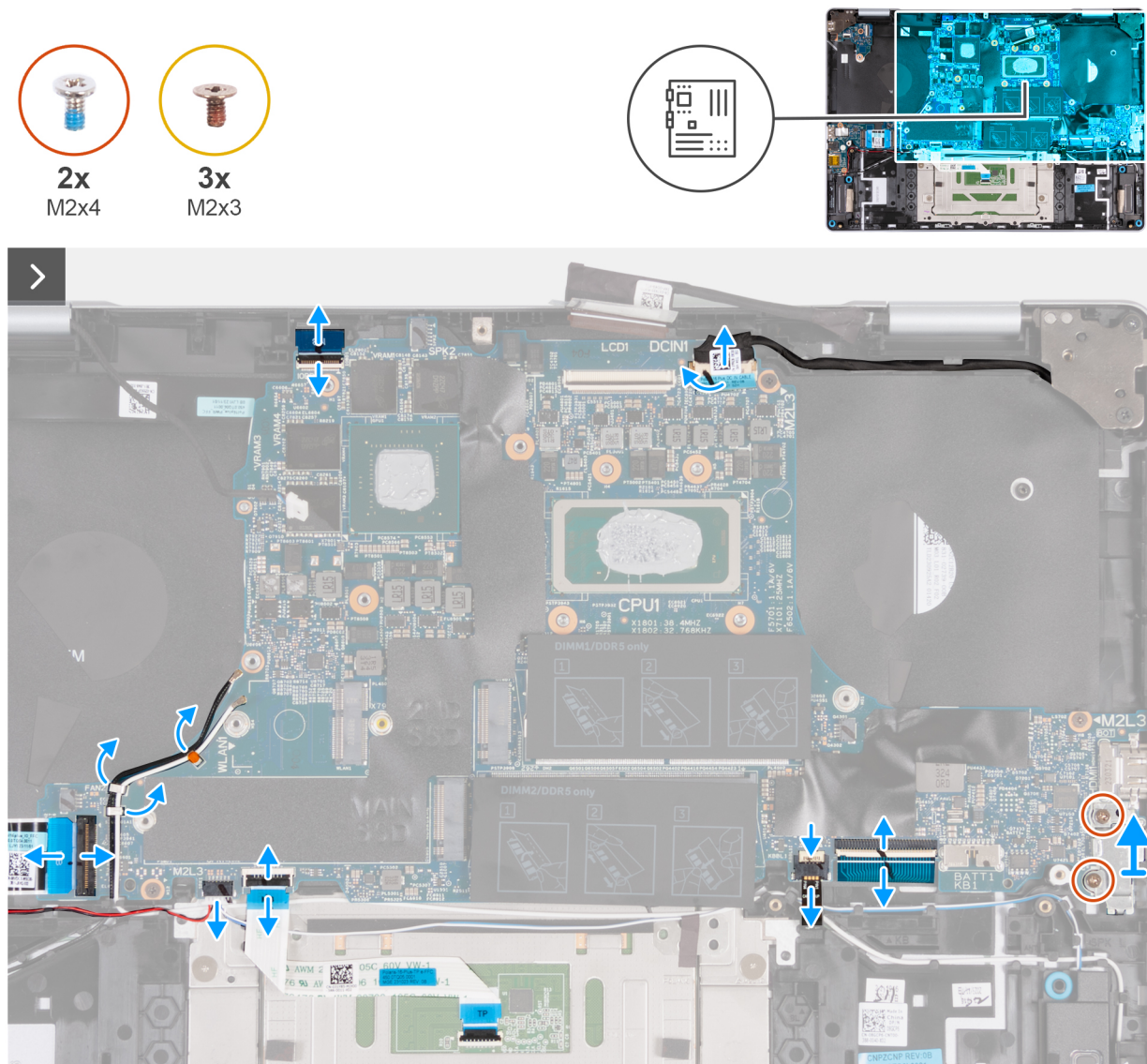
איור 55. הסרת לוח המערכת
