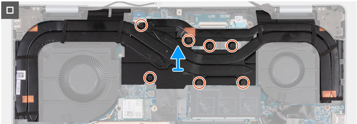
איור 41. הסרת גוף הקירור
