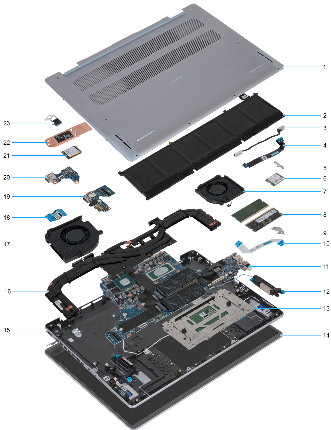
איור 8. הרכיבים העיקריים של Inspiron 16 Plus 7640
