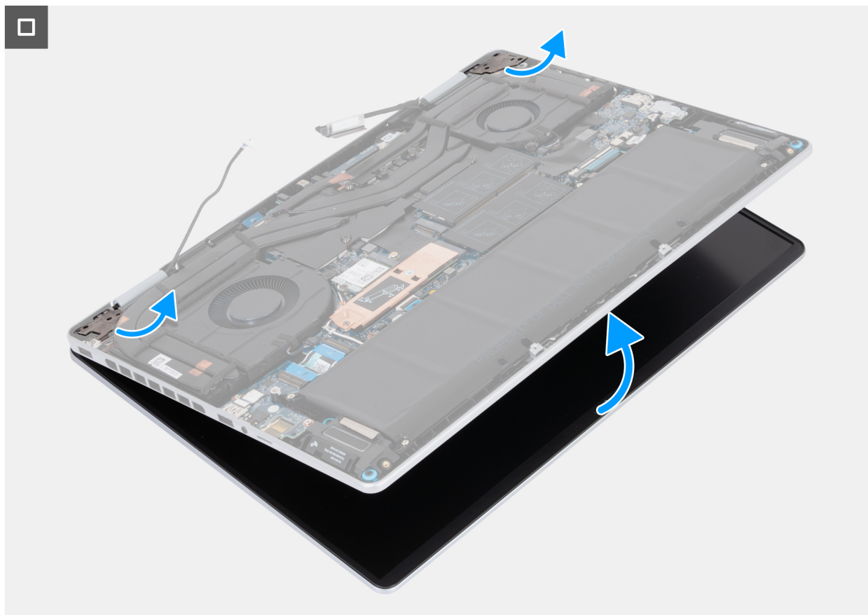
איור 32. הסרת מכלול הצג
