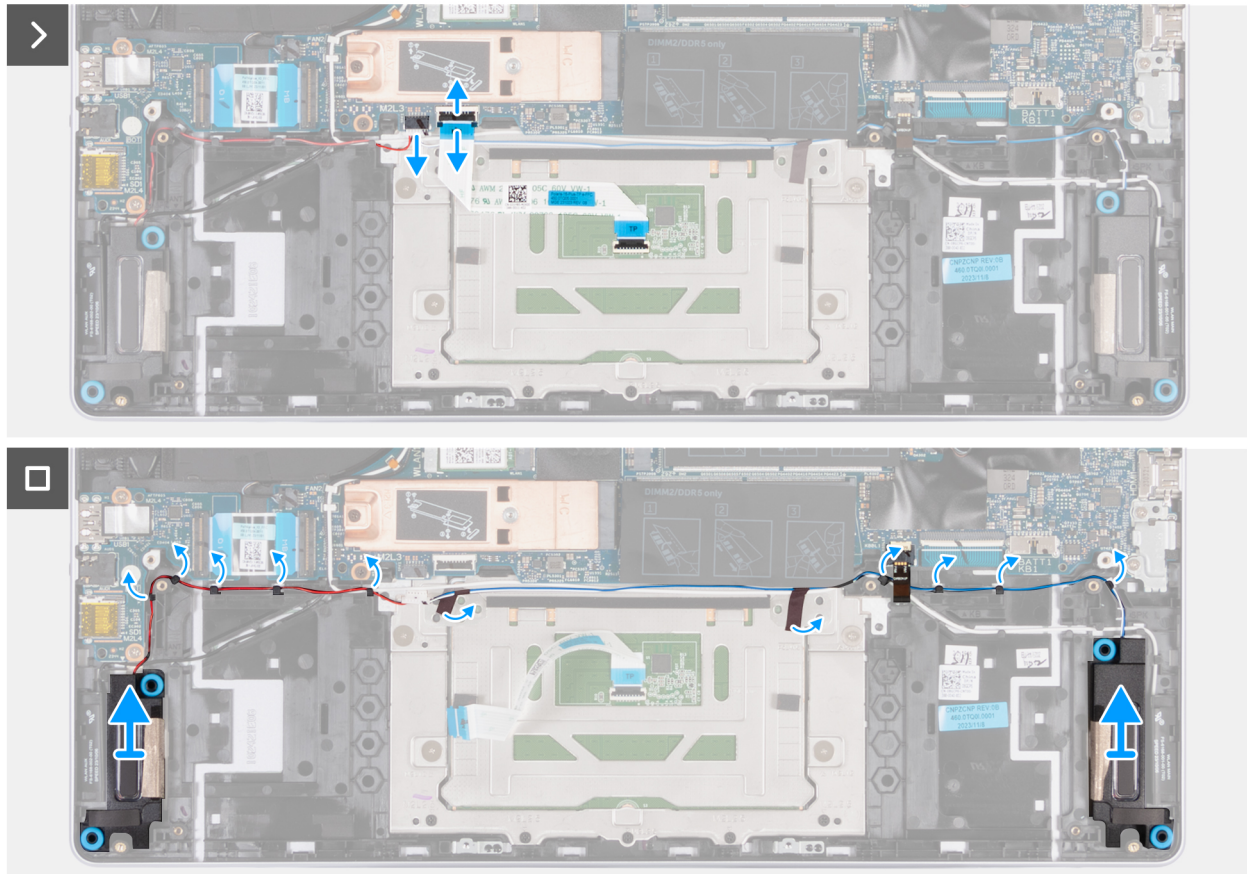
איור 29. הסרת הרמקולים
