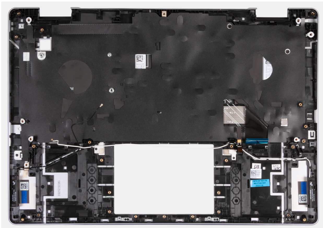
איור 62. מכלול משענת כף היד והמקלדת
