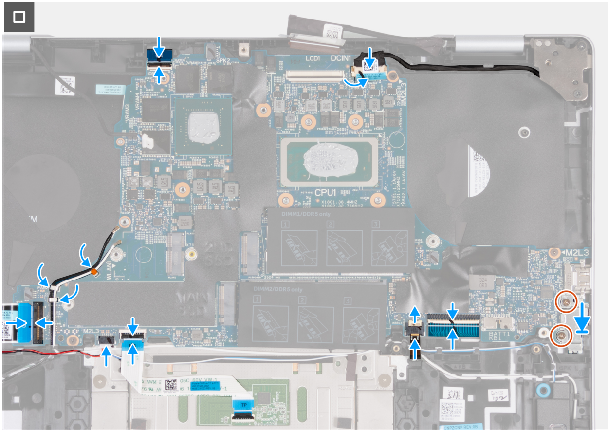
איור 59. התקנת לוח המערכת 2
