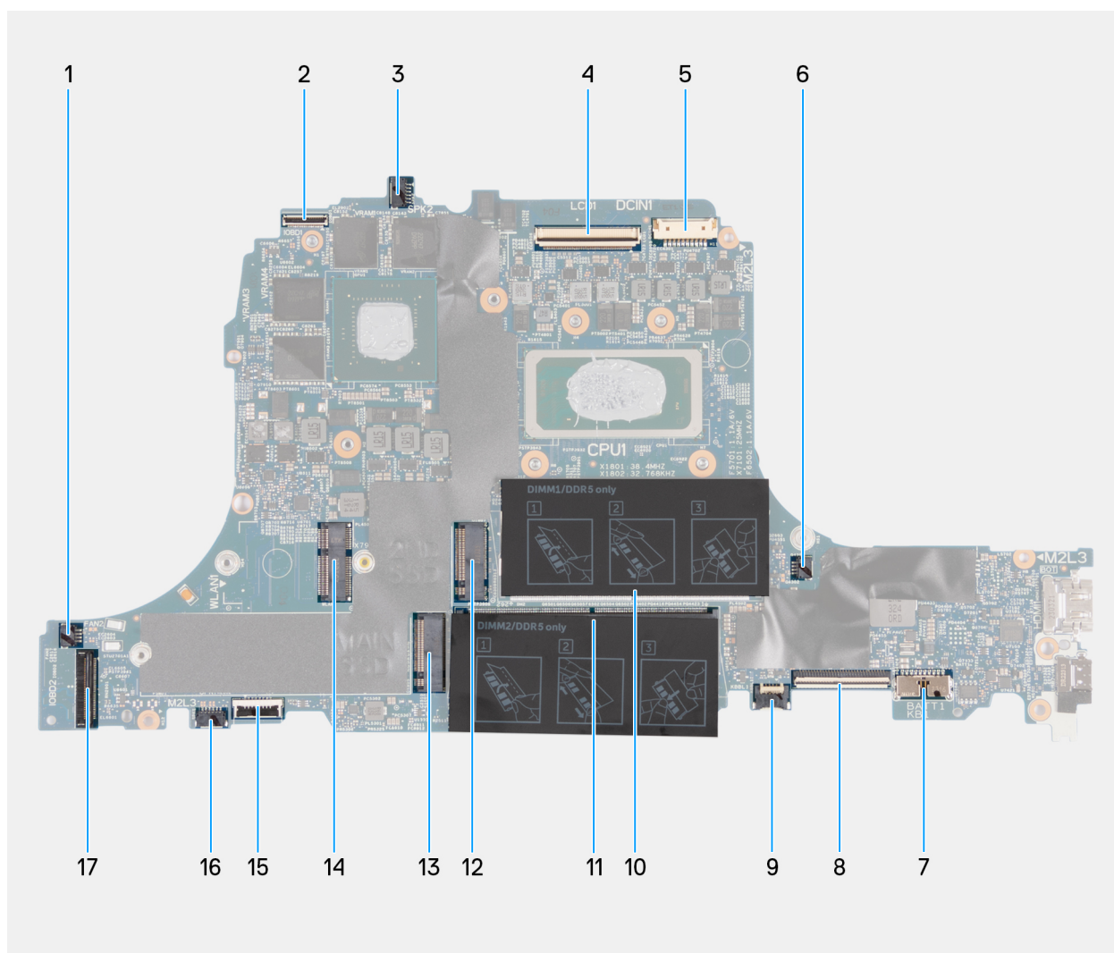
איור 57. מחברי לוח מערכת
