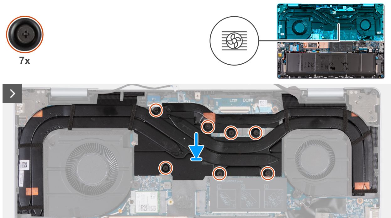
איור 42. התקנת גוף הקירור
