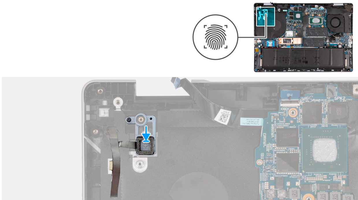
איור 50. התקנת לחצן הפעלה עם קורא טביעות אצבעות אופציונלי
