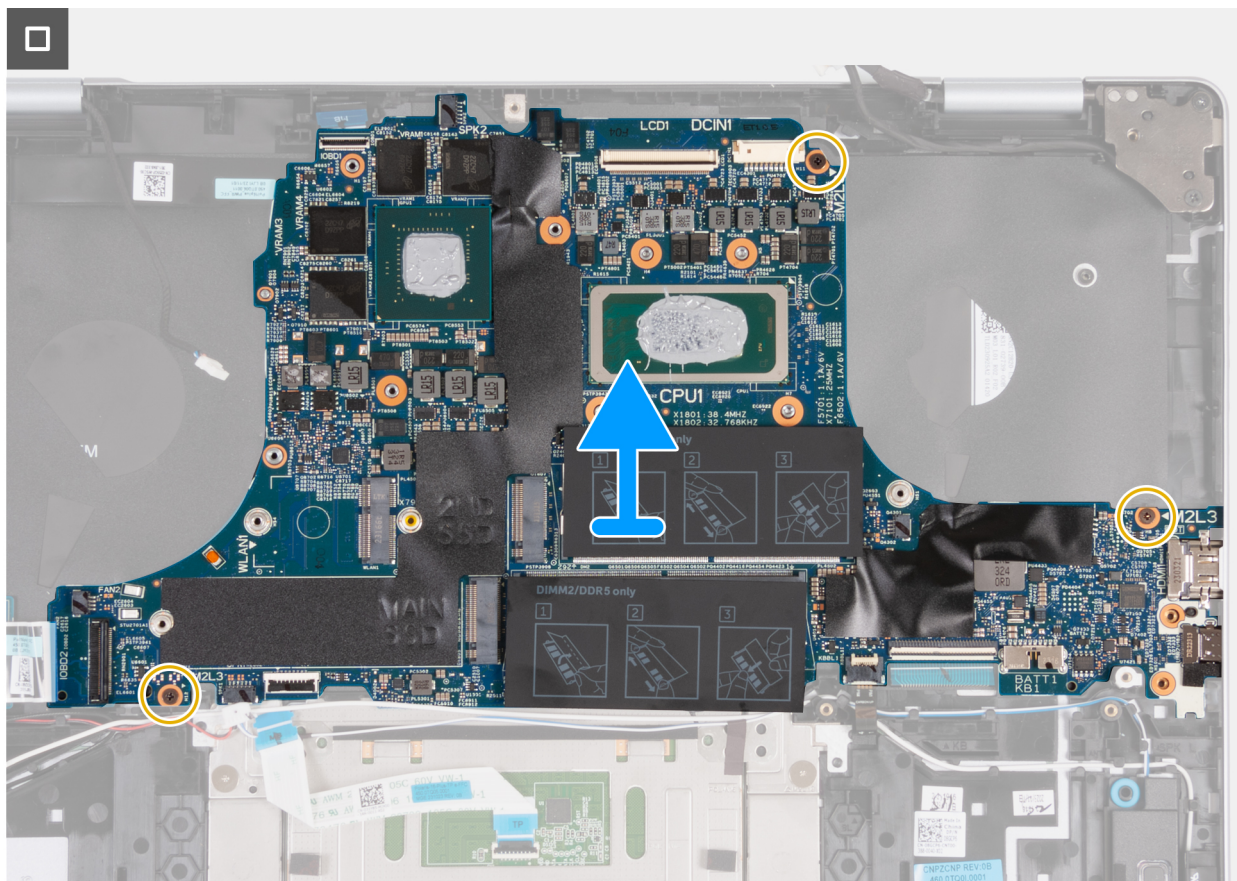
איור 56. הסרת לוח המערכת
