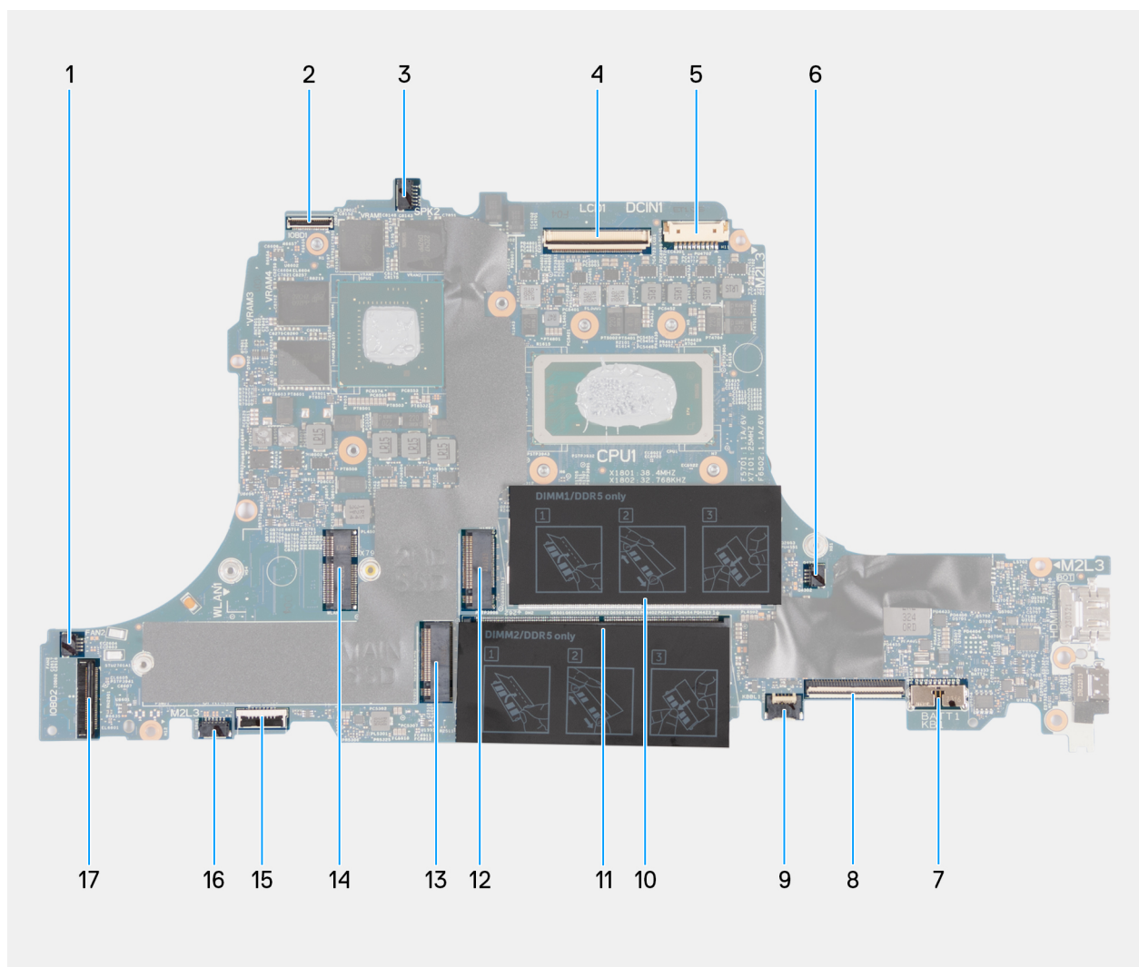
איור 54. מחברי לוח מערכת
