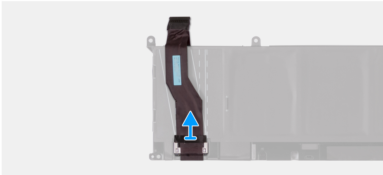
איור 27. הסרת כבל הסוללה
